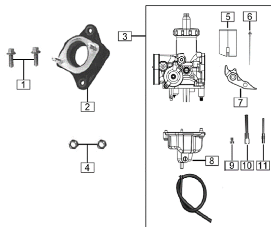
FIG. Nº 13 CARBURADOR
