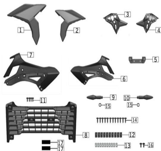
FIG. Nº 16 ENFOCADORES-DIRECCIONALES
