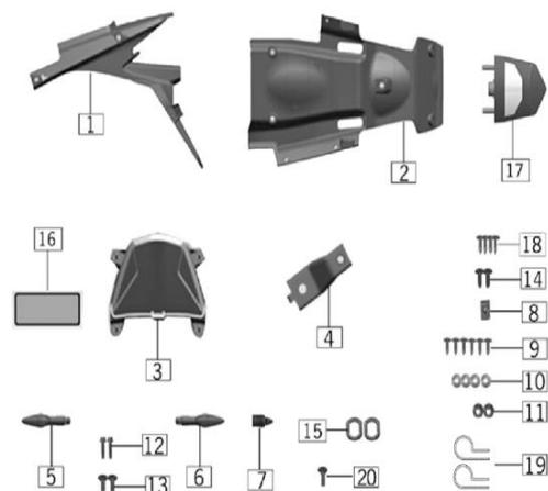
FIG. Nº 31 GUARDABARRO TRASERO-DIRECCIONALES
