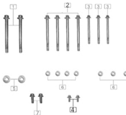
FIG. Nº 35 SOPORTE MOTOR
