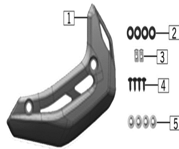
FIG. Nº 18 CUBIERTA INFERIOR
