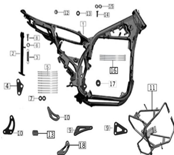
FIG. Nº 34 COMPLEMENTOS CHASIS-GATO LATERAL
