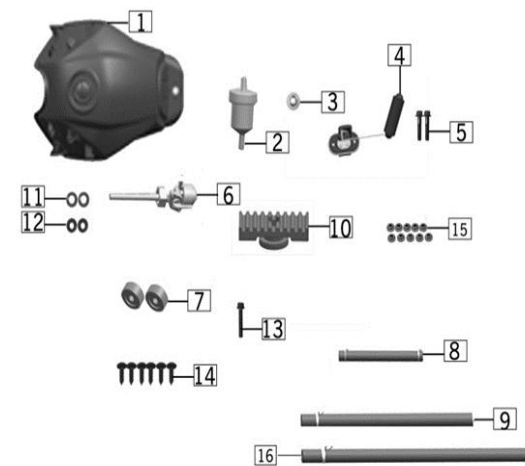
FIG. Nº 15 TANQUE GASOLINA
