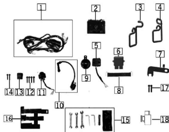
FIG. Nº 32 PARTES ELÉCTRICAS
