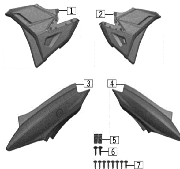
FIG. Nº 17 CUBIERTAS LATERALES
