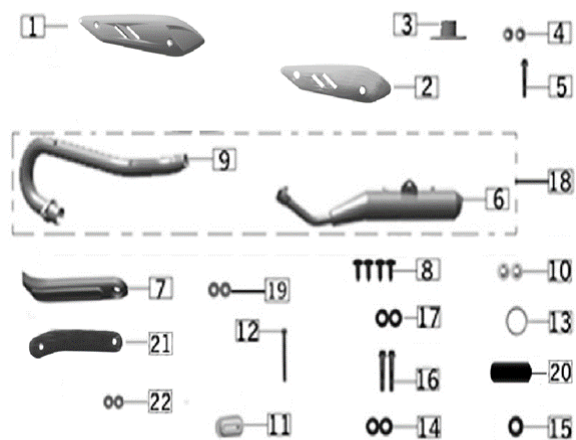
FIG. N° 14 MOFLE
