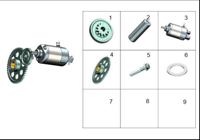
FIGURA 129: ARRANQUE ELÉCTRICO
