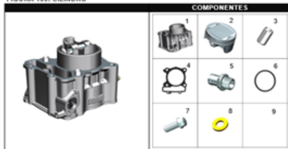
FIGURA 109: CILINDRO
