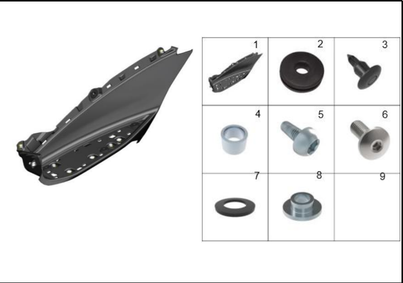
FIGURA 22: REPOSAPIE IZQUIERDO
