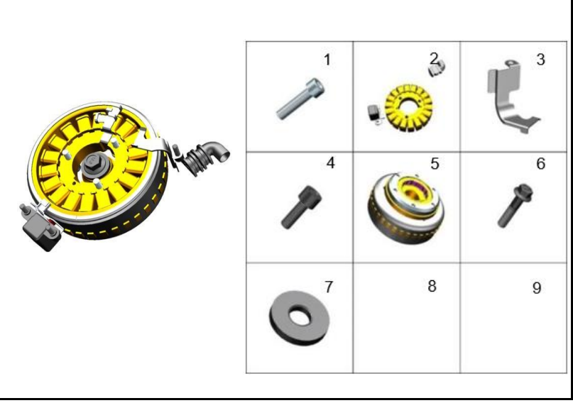
FIGURA 130: PLATO BOBINA
