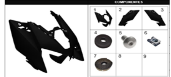
FIGURA 12: CUBIERTA FRONTAL
