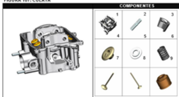
FIGURA 107: CULATA
