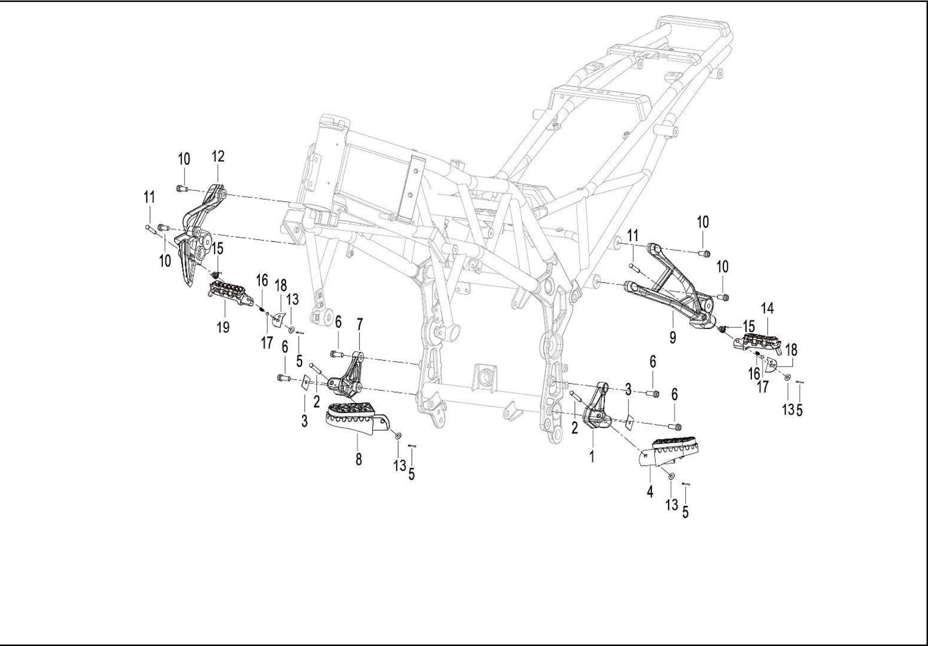
FIGURA N° 28: REPOSAPIES
