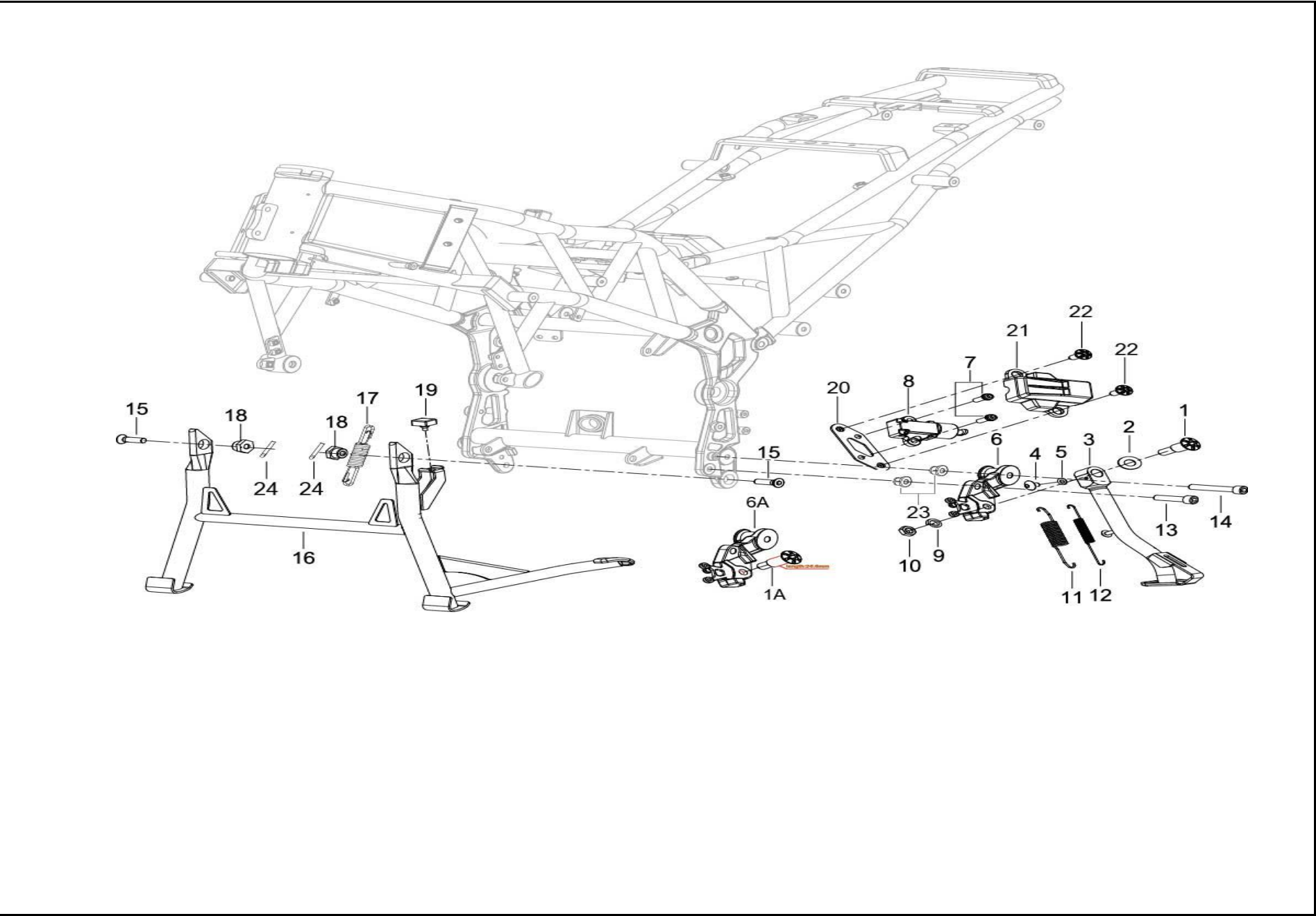
FIGFIGURA N° 29: GATO CENTRAL - GATO LATERAL
