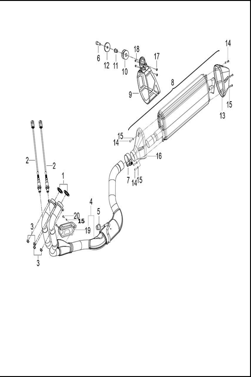
FIGURA N° 32: SILENCIADOR
