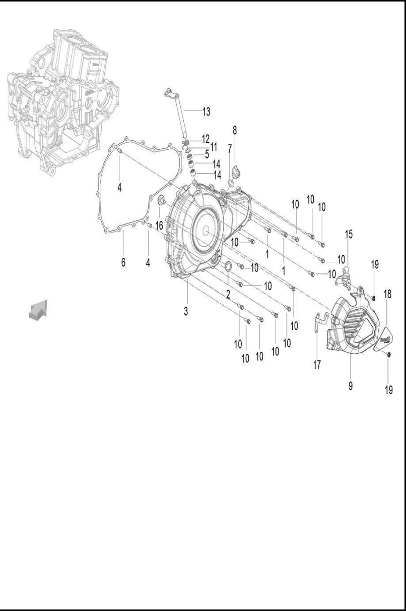
FIGURA N° 7: CUBIERTA CLUTCH
