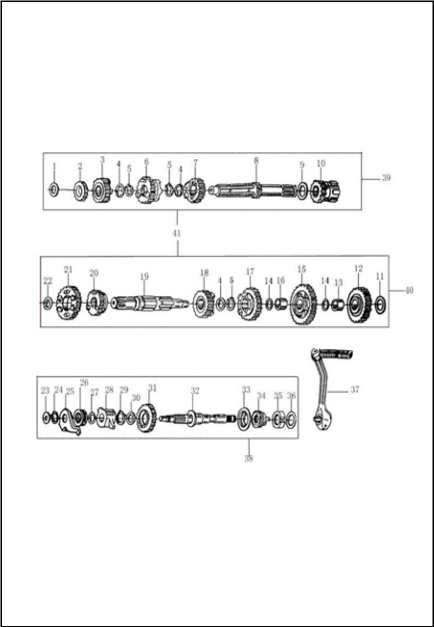
FIGURA N°8: TRANSMISIÓN (1/2)
