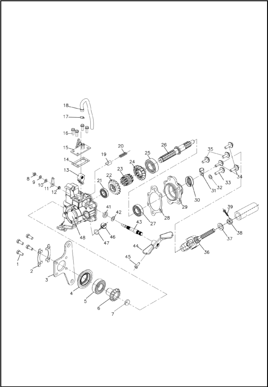
FIGURA N° 42: CAJA REVERSA (2/2)
