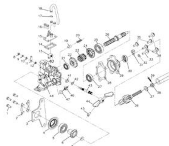
FIGURA N° 42: CAJA REVERSA
