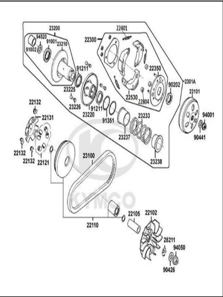
FIGURA N° 5: CLUTCH CENTRIFUGO 1/2
