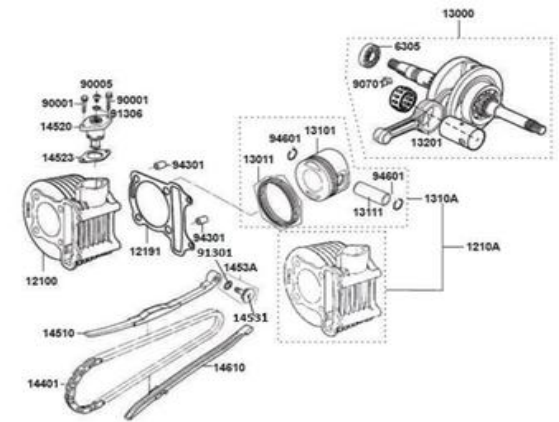
FIG. N° 3 CILINDRO - PISTÓN - CIGÜEÑAL
