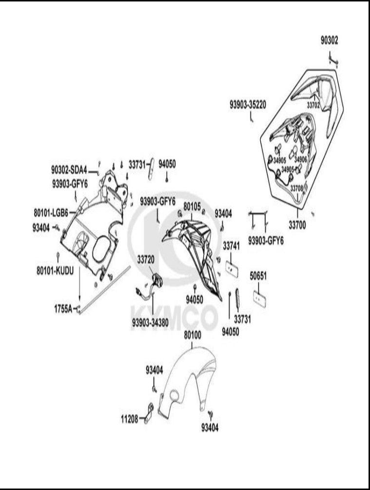
FIGURA N° 27: GUARDABARRO TARSERO
