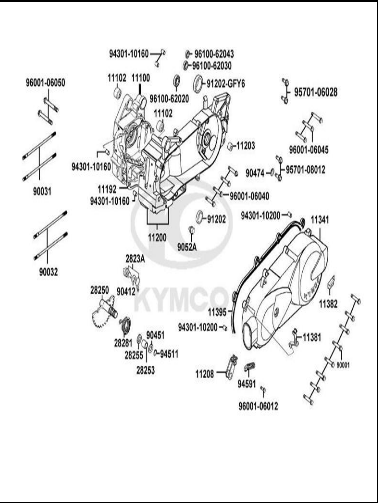
FIGURA N° 1: CARCASAS 1/2
