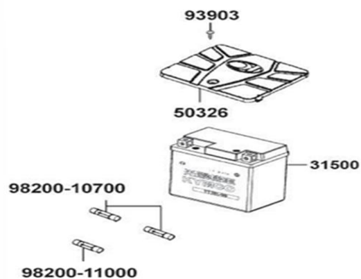
FIG. N° 20 BATERIA
