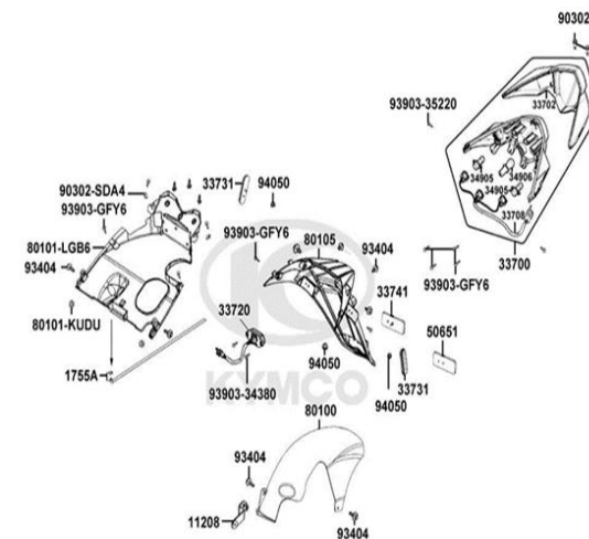
FIG. N° 27 GUARDABARRO TARSERO
