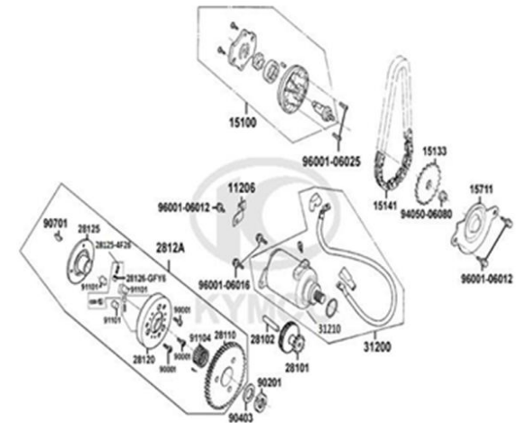
FIG. Nº 6 MOTOR DE ARRANQUE - BOMBA DE ACEITE
