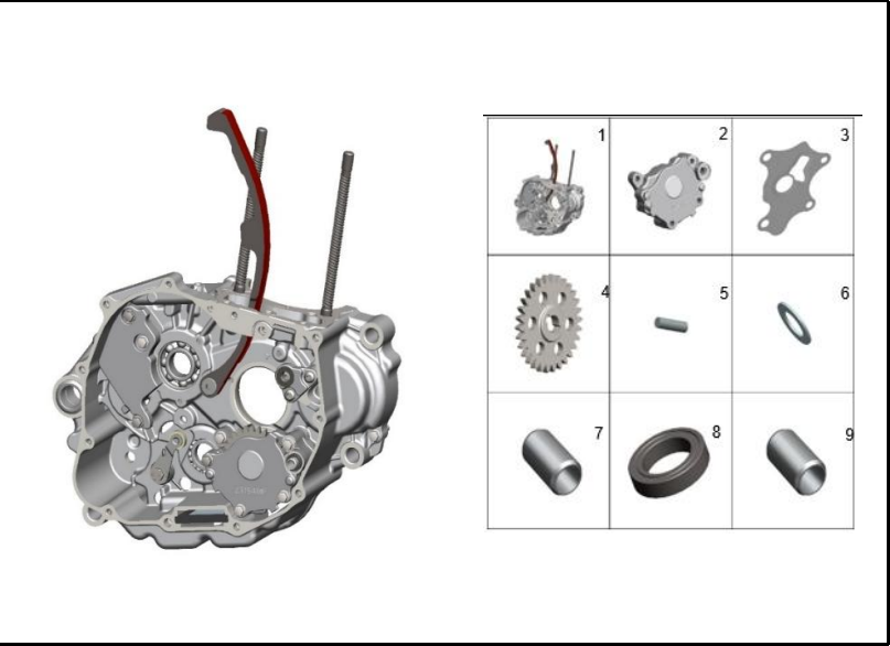
FIGURA 111: CARCASA DERECHA
