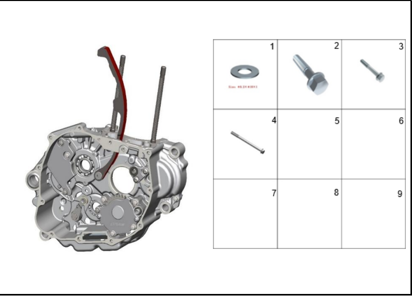
FIGURA 111: CARCASA DERECHA 2
