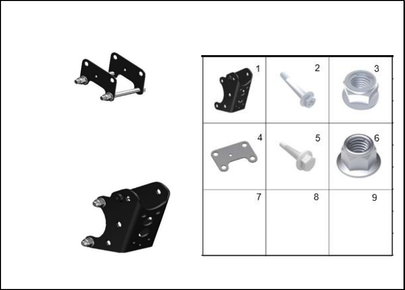
FIGURA 66: SOPORTE MOTOR
