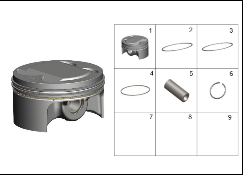
FIGURA 100: PISTON
