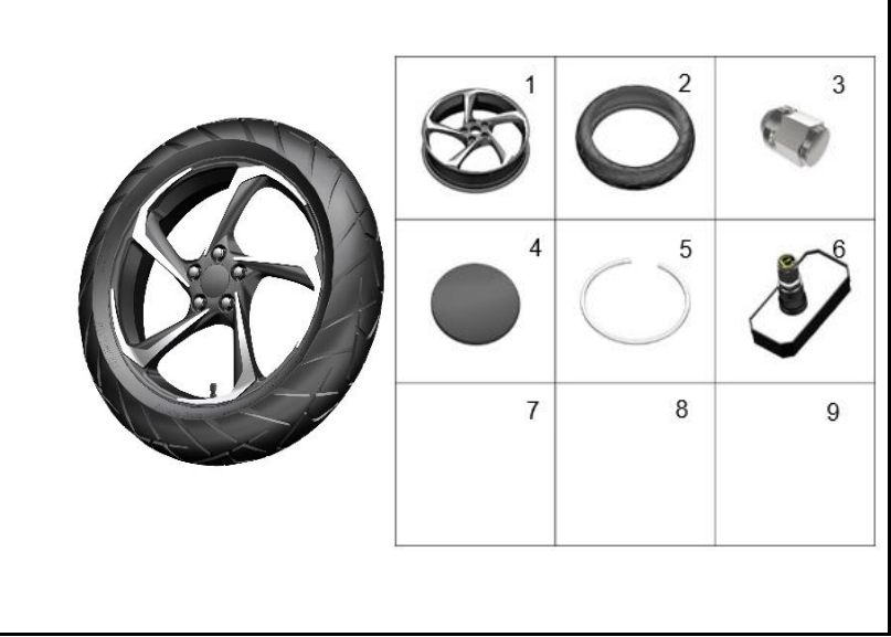
FIGURA 63: RUEDA TRASERA
