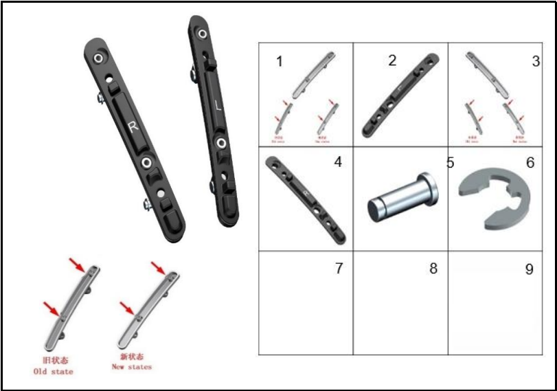
FIGURA 2: SOPORTES VISOR
