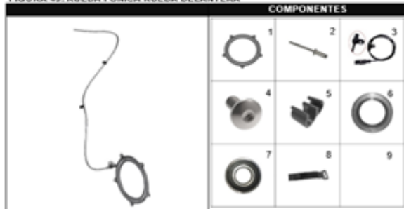
FIGURA 49: RUEDA FONICA RUEDA DELANTERA
