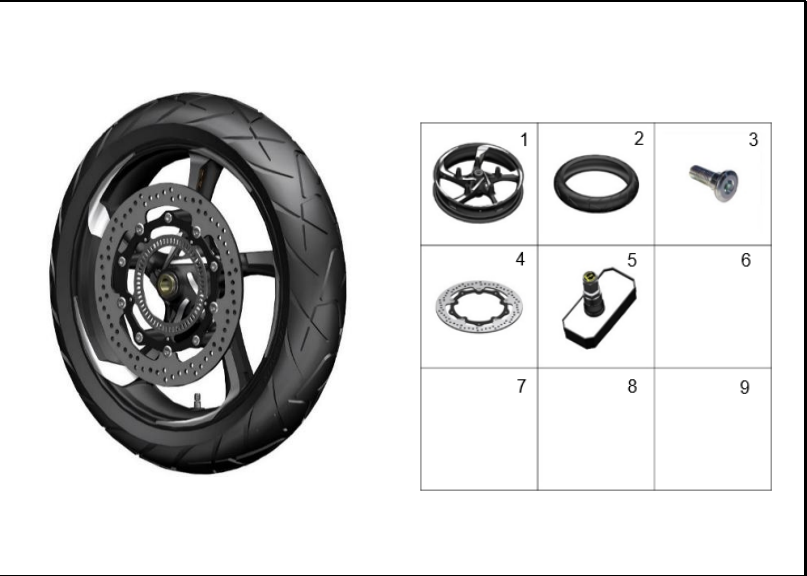
FIGURA 48: RUEDA DELANTERA
