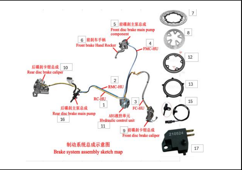
FIGURA 129: SISTEMA DE FRENOS
