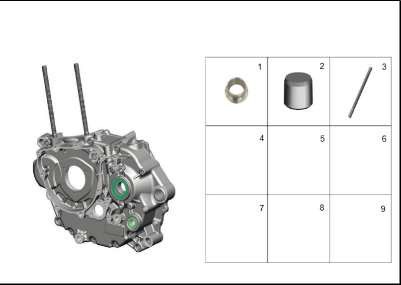
FIGURA 116: CARCASA IZQUIERDA 5
