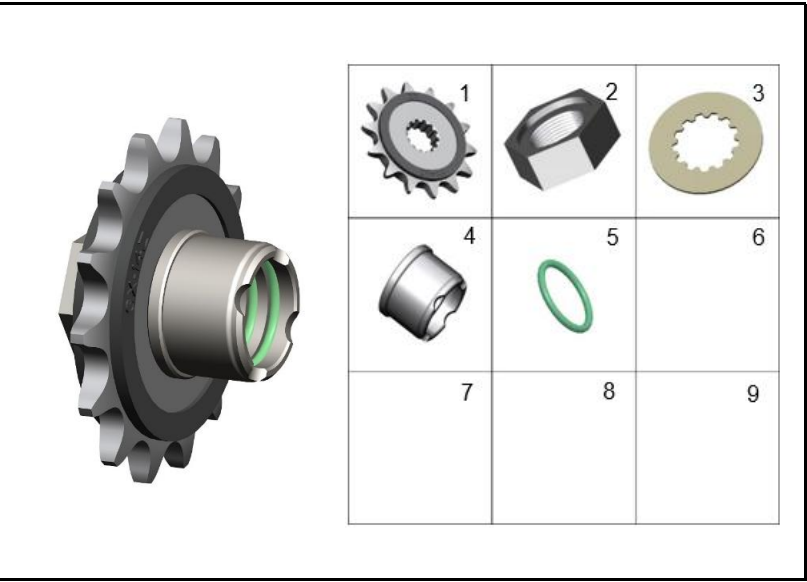
FIGURA 112: PIÑON DE SALIDA
