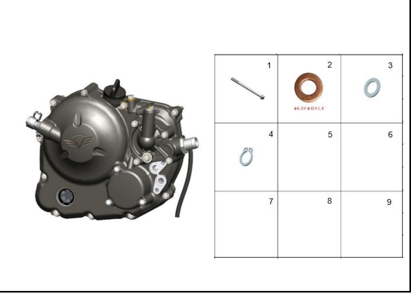
FIGURA 124: TAPA CARTER DERECHA 2
