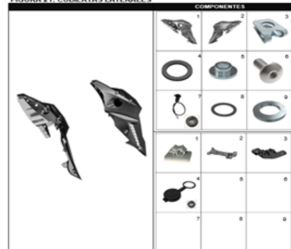
FIGURA 21: CUBIERTAS LATERALES
