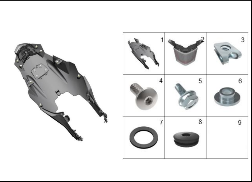
FIGURA 28: COLA INFERIOR
