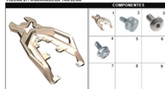
FIGURA 27: AGARRADERA TRASERA
