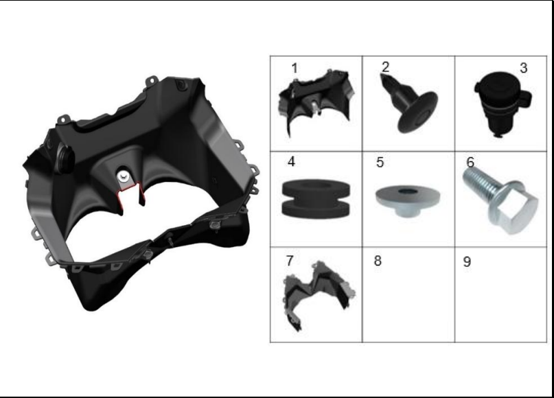
FIGURA 12: CUBIERTA INTERIOR FRONTAL
