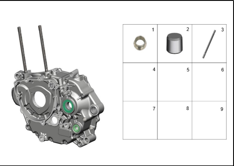
FIGURA 121: CARCASA IZQUIERDA
