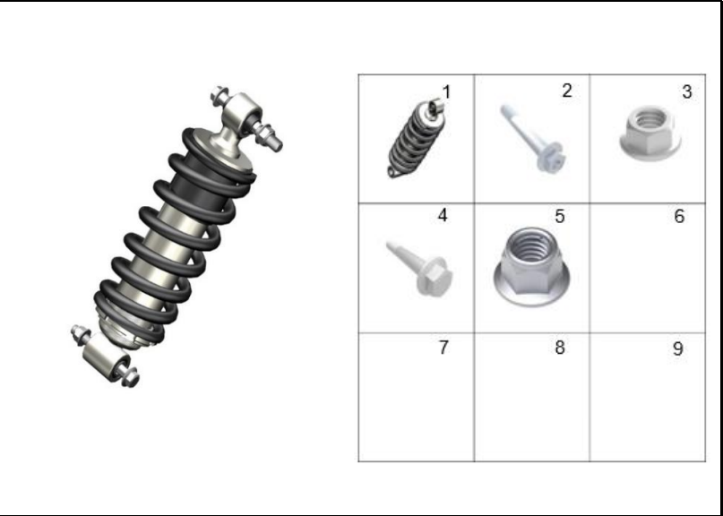
FIGURA 58: AMORTIGUADOR TRASERO
