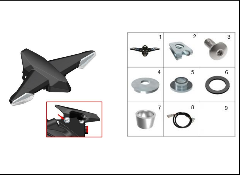
FIGURA 40: SOPORTE DIRECCIONALES 2
