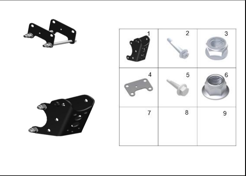
FIGURA 76: SOPORTE MOTOR
