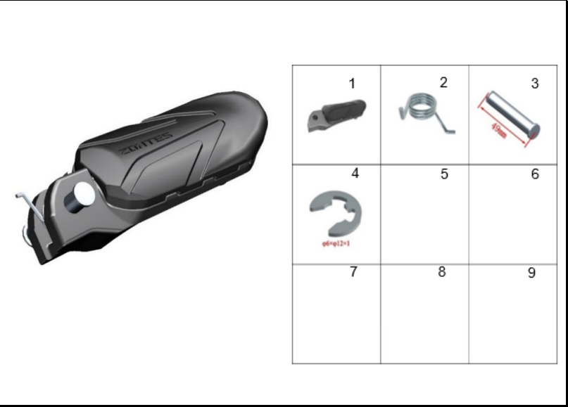
FIGURA 86: REPOSAPIE DELANTERO IZQUIERDO COMPLETO
