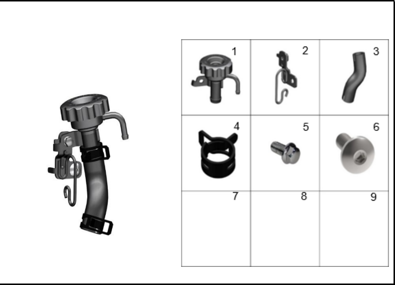
FIGURA 98: TAPA RADIADOR
