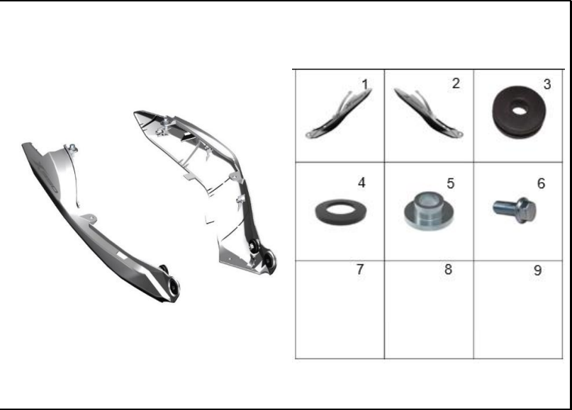
FIGURA 34: CUBIERTAS DE SILLIN
