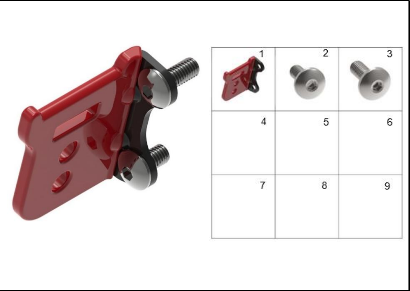
FIGURA 87: SOPORTE DE BLOQUEO DEL FRENO DE DISCO
