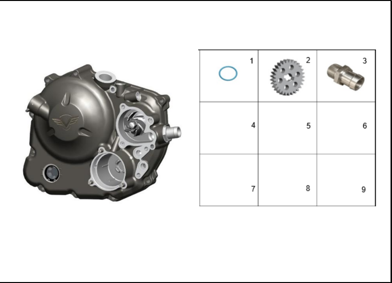
FIGURA 131: CUBIERTA CARCASA MOTOR DERECHA
