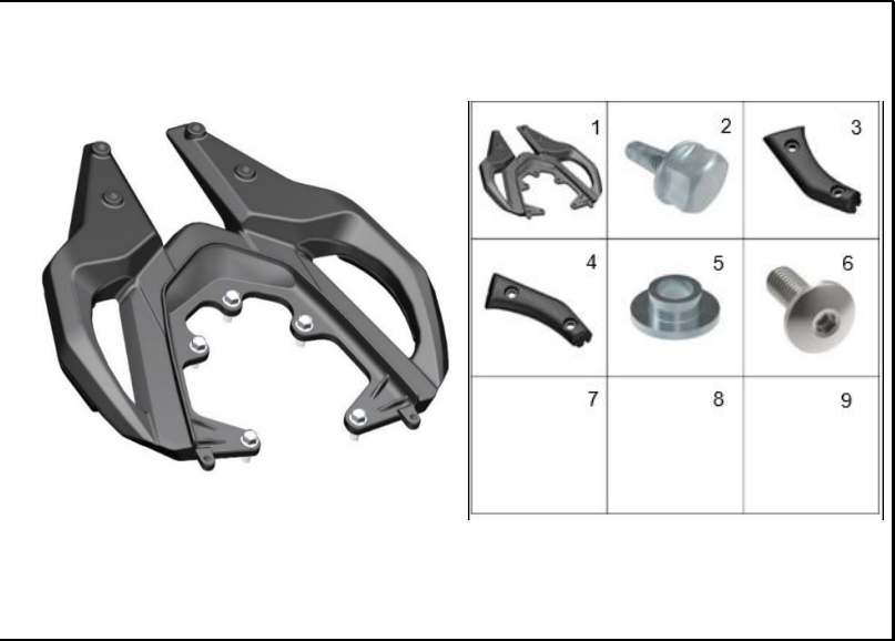
FIGURA 37: AGARRADERA TRASERA
