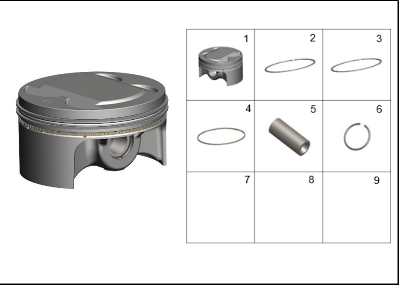
FIGURA 112: PISTON
