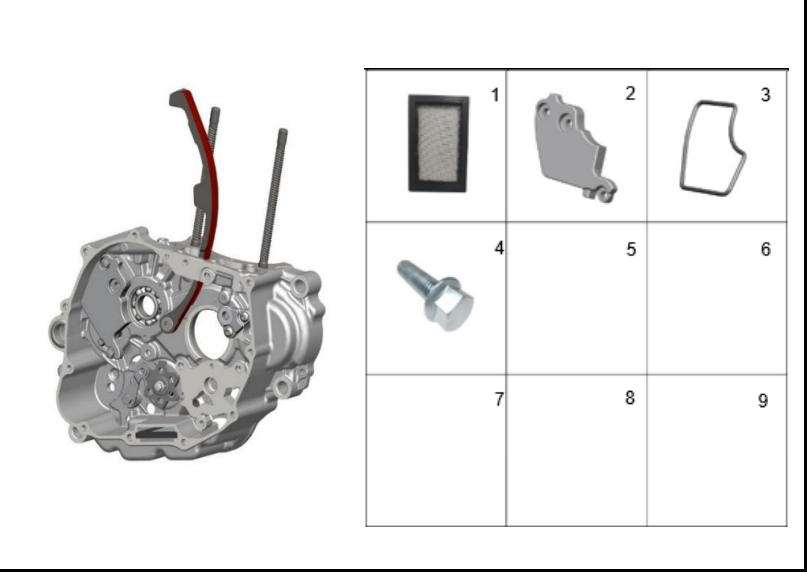
FIGURA 124: CARCASA DERECHA 2
