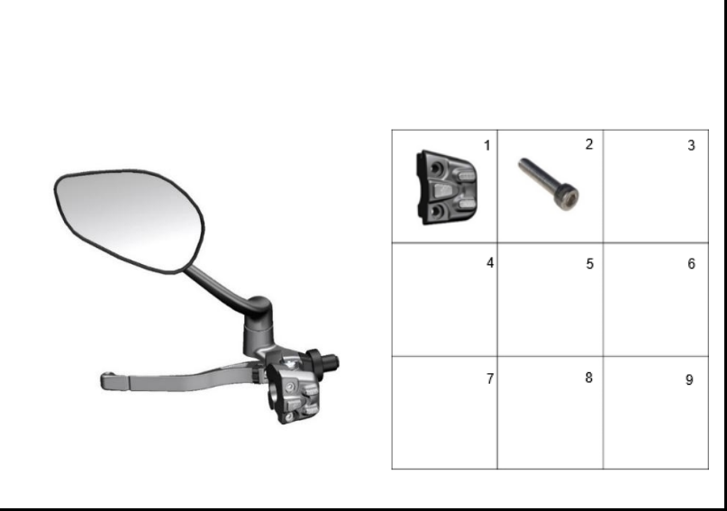
FIGURA 46: LEVA DE CLUTCH-ESPEJO IZQUIERDO 2
