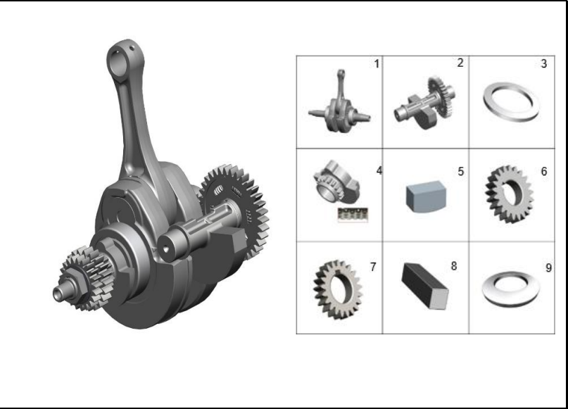
FIGURA 122: CIGÜEÑAL
