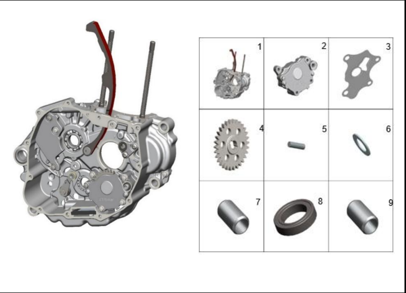
FIGURA 123: CARCASA DERECHA
