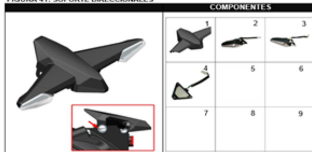
FIGURA 41: SOPORTE DIRECCIONALES
