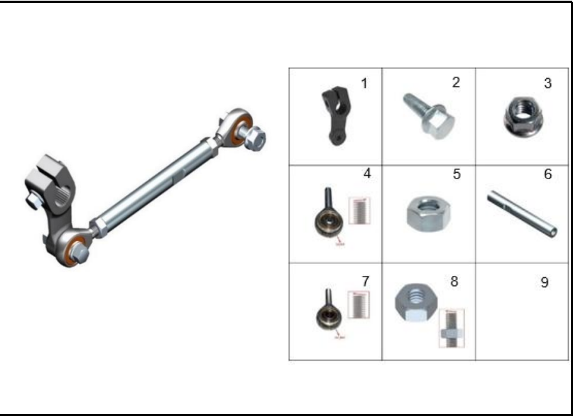
FIGURA 88: VARILLA MUÑÓN PEDAL DE CAMBIOS
