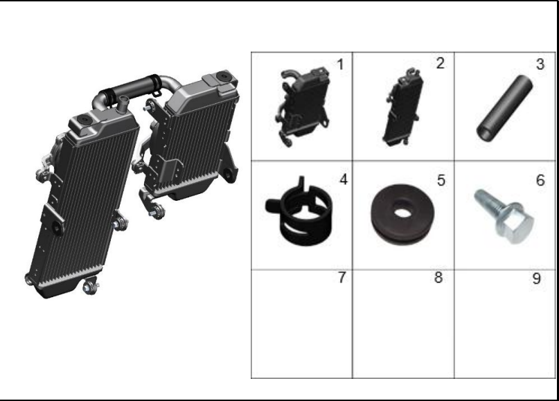
FIGURA 97: RADIADOR
