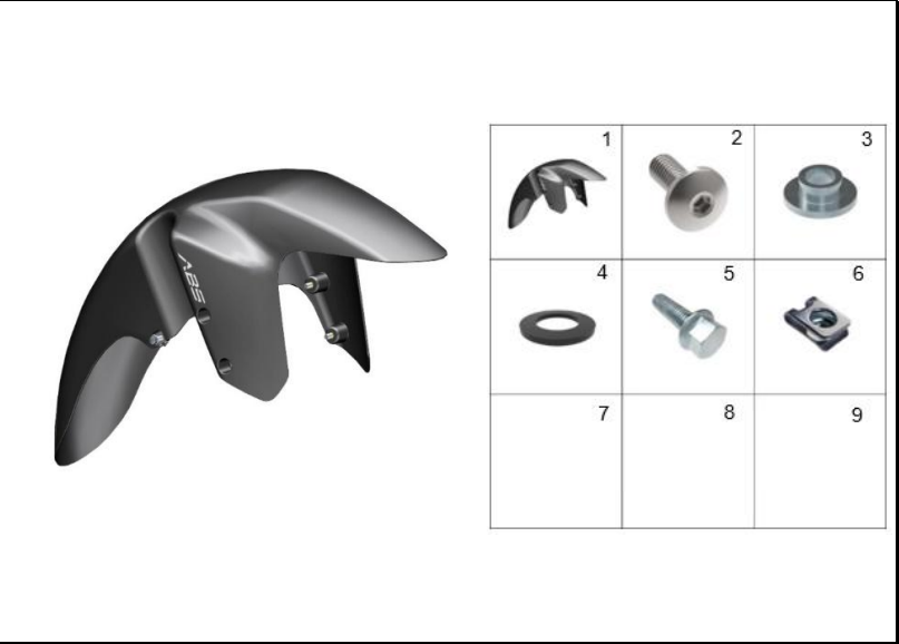
FIGURA 14: GUARDABARRO DELANTERO
