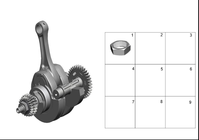
FIGURA 122: CIGÜEÑAL
