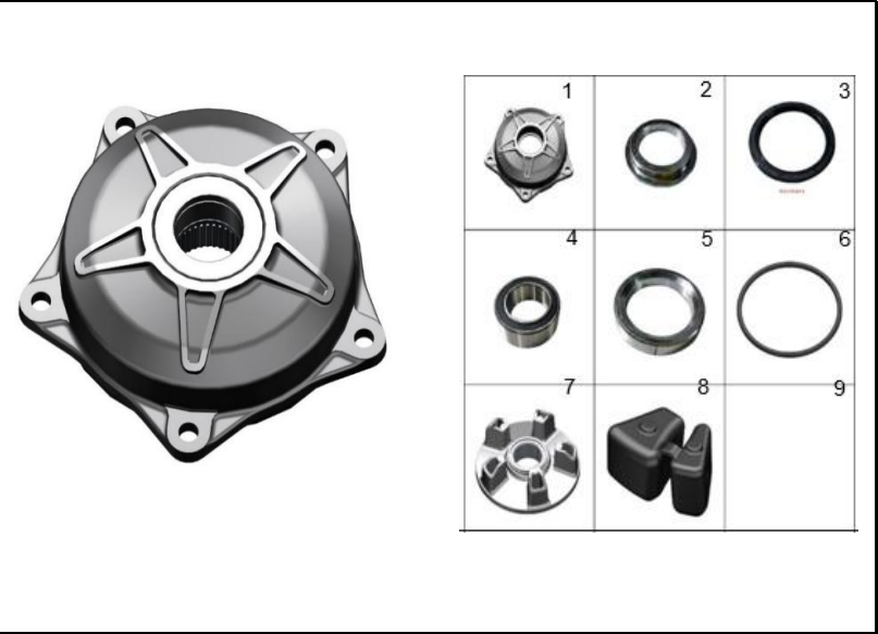
FIGURA 64: PROTECTOR SPROCKET
