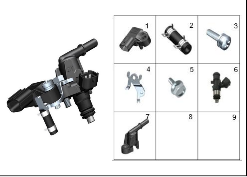
FIGURA 80: SOPORTE INYECTOR
