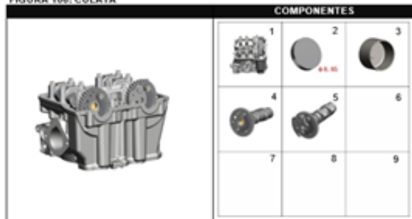
FIGURA 106: CULATA
