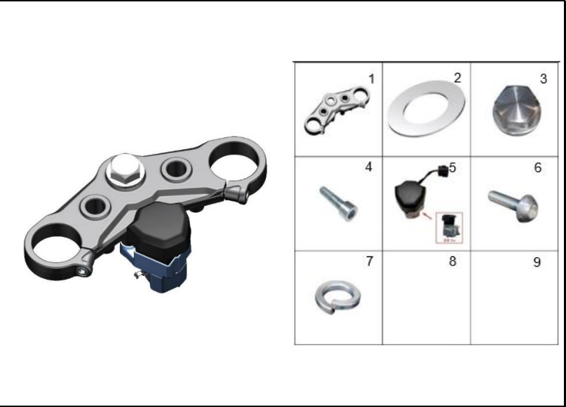
FIGURA 50: SOPORTE TUBOS SUSPENSIÓN DELANTERA
