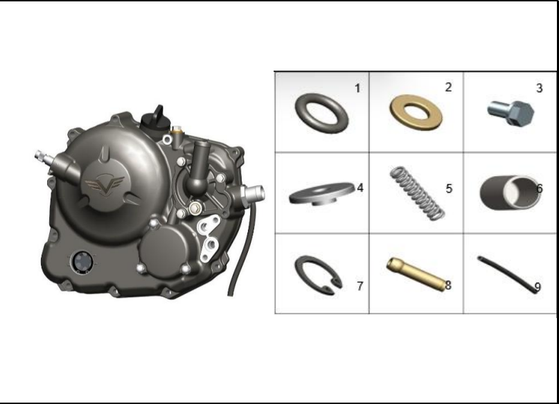
FIGURA 130: TAPA CARTER DERECHA 2
