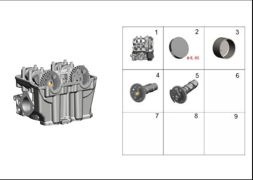
FIGURA 106: CULATA 3
