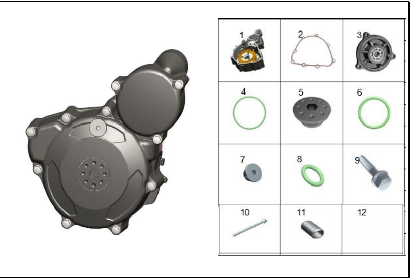
FIGURA 126: TAPA CÁRTER IZQ
