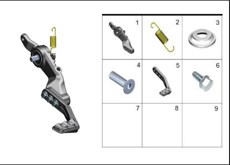
FIGURA 95: PEDAL DE FRENO
