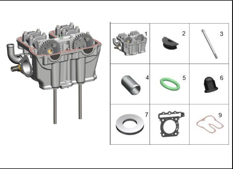
FIGURA 104: CULATA
