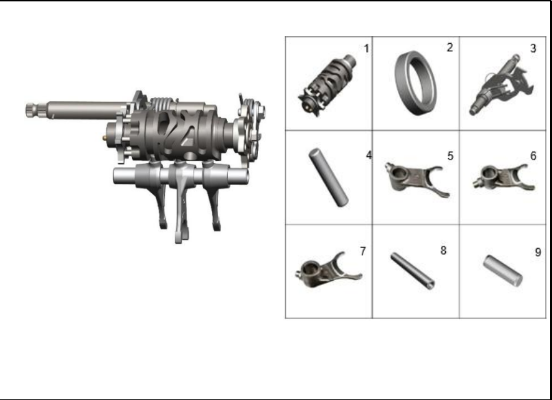
FIGURA 118: EJE DE CAMBIOS
