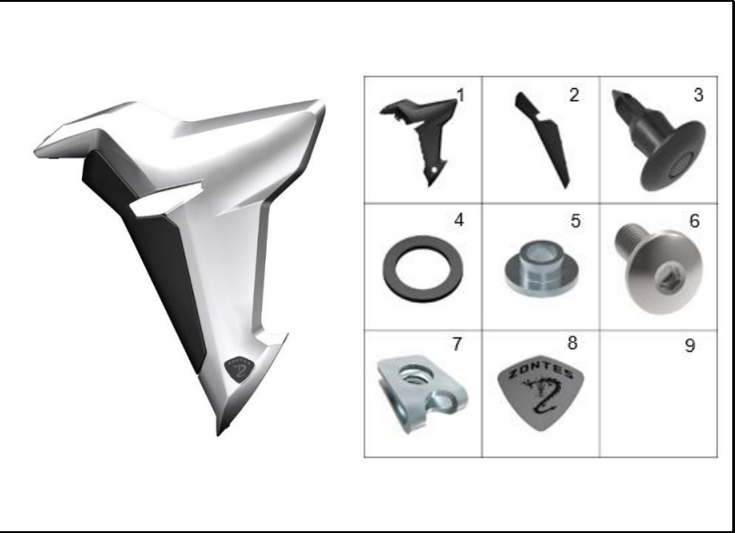
FIGURA 21: CUBIERTA TANQUE IZQUIERDA
