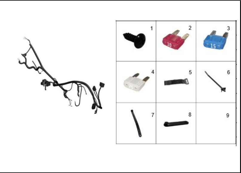
FIGURA 71: PARTES ELECTRICAS 2
