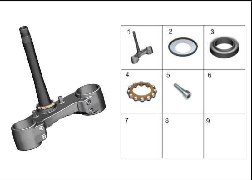
FIGURA 52: HORQUILLA DIRECCIÓN
