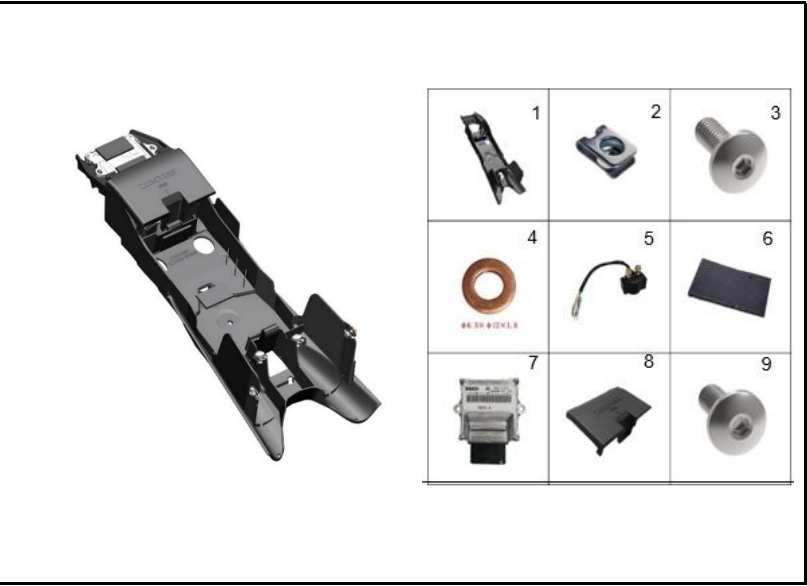
FIGURA 30: CAJA DISPOSITIVOS ELÉCTRICOS
