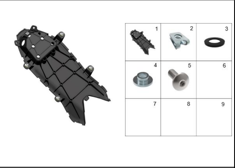
FIGURA 35: GUARDABARRO TRASERO
