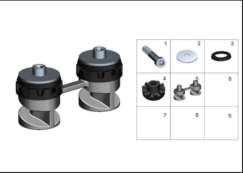
FIGURA 16: SOPORTE TANQUE DE COMBUSTIBLE
