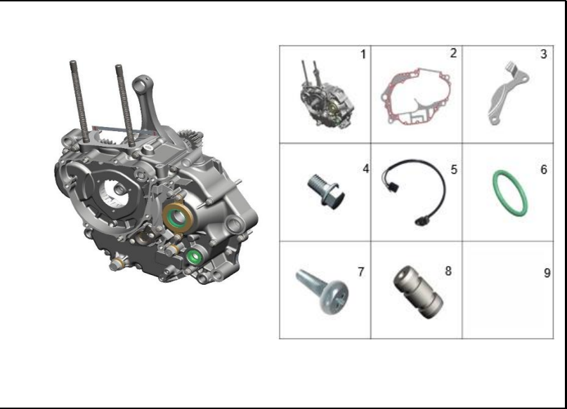
FIGURA 119: CARCASA IZQUIERDA
