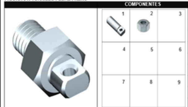
FIGURA 91: TORNILLO PEDAL FRENO
