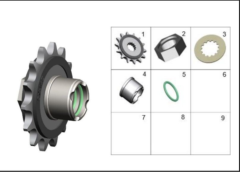
FIGURA 117: PIÑÓN DE SALIDA
