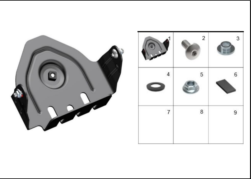
FIGURA 32: SOPORTE BATERÍA
