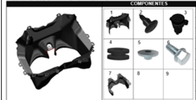
FIGURA 12: CUBIERTA INTERIOR FRONTAL
