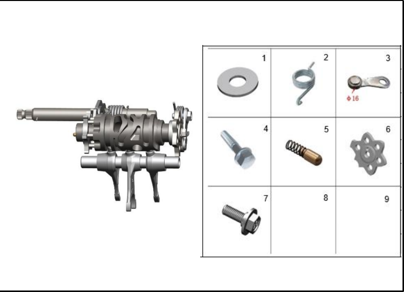
FIGURA 118: EJE DE CAMBIOS 2
