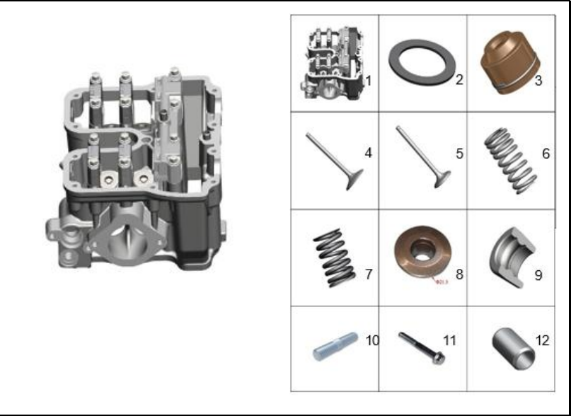
FIGURA 107: CULATA 4
