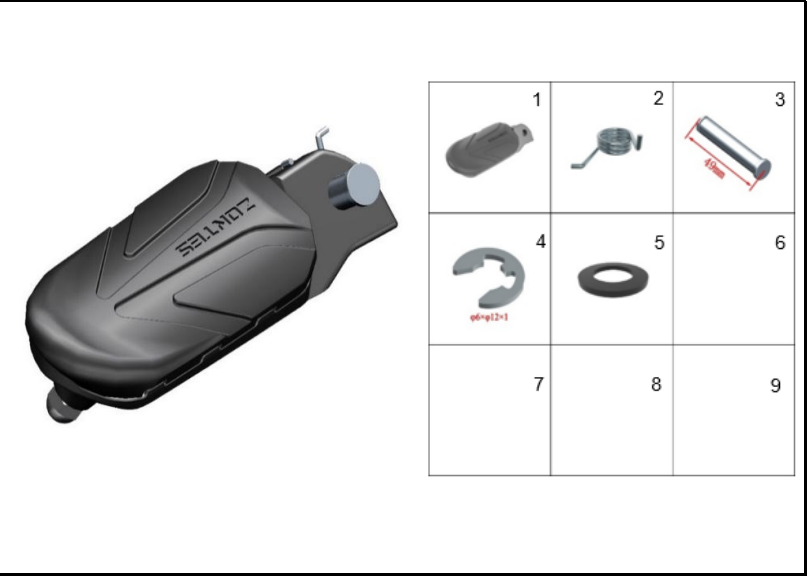
FIGURA 92: REPOSAPIE DELANTERO DERECHO COMPLETO
