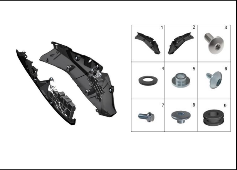
FIGURA 33: CUBIERTAS LATERALES TRASERAS
