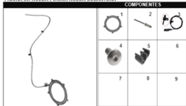
FIGURA 55: RUEDA FONICA RUEDA DELANTERA
