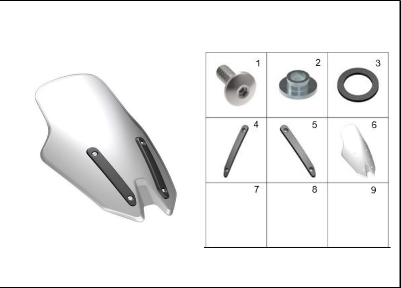
FIGURA 1: VISOR
