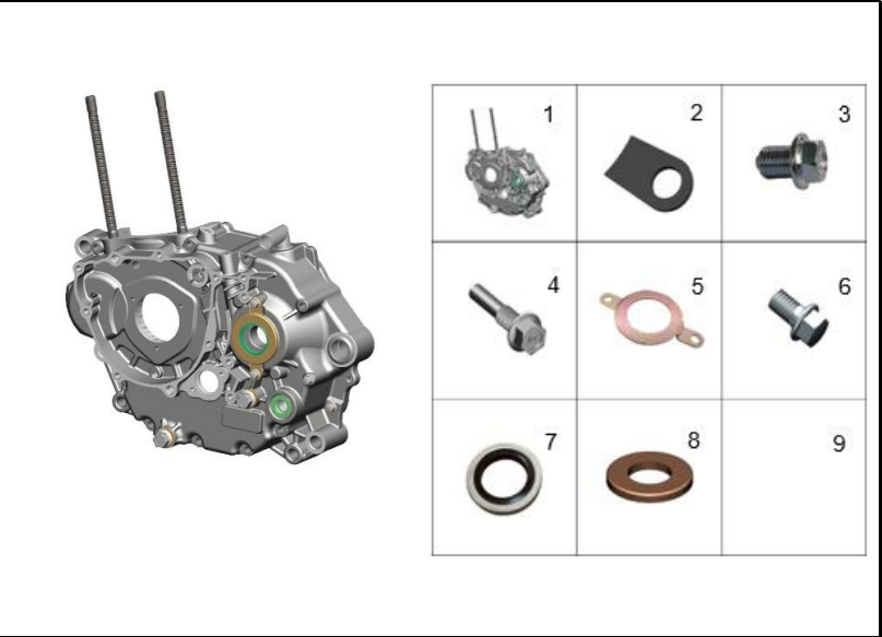
FIGURA 120: CARCASA IZQUIERDA
