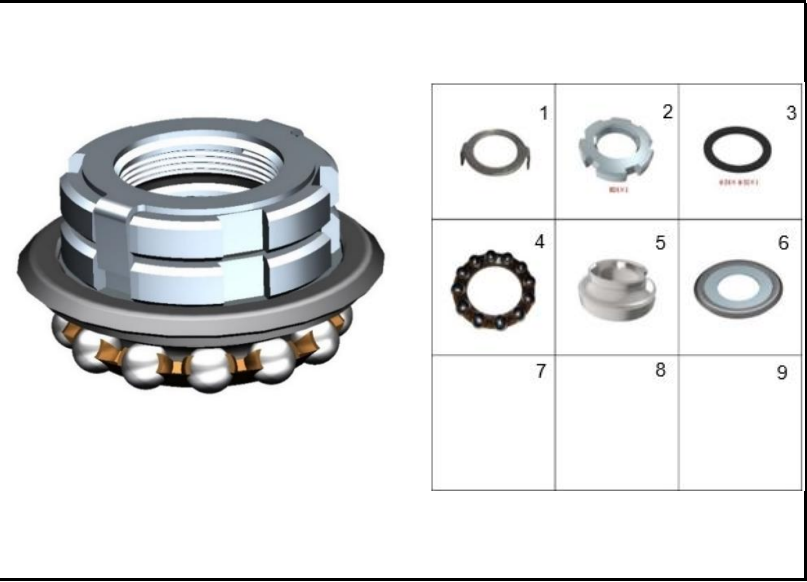
FIGURA 51: CUNAS DIRECCIÓN
