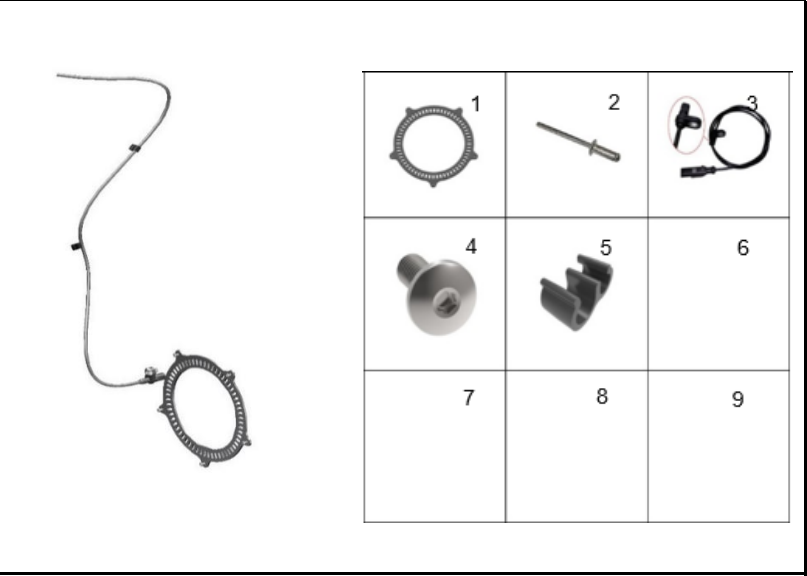
FIGURA 55: RUEDA FONICA RUEDA DELANTERA
