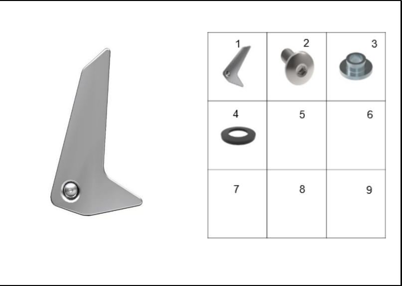
FIGURA 60: SOPORTE SPROCKET
