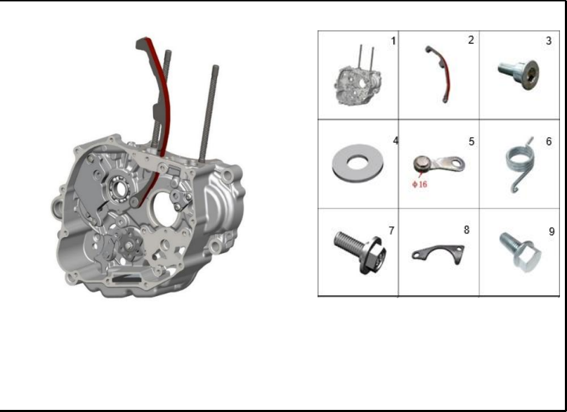
FIGURA 124: CARCASA DERECHA 2
