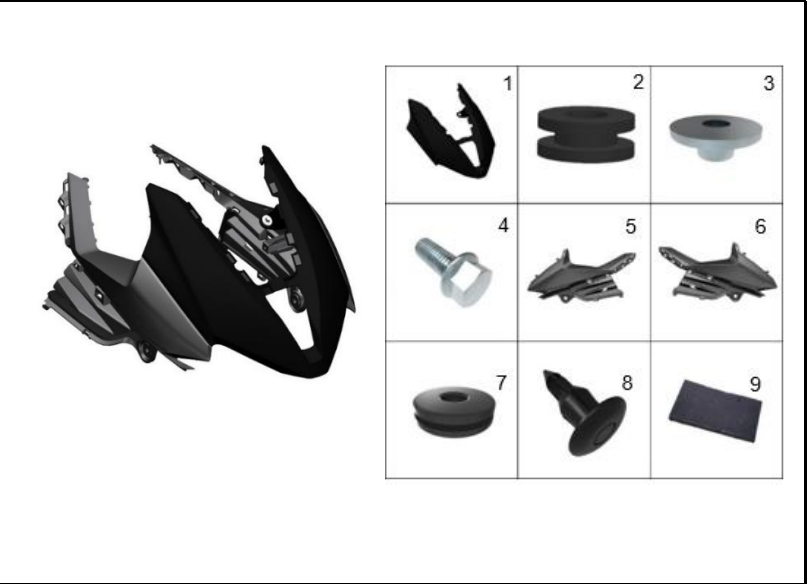
FIGURA 9: CUBIERTA CARENAJE FRONTAL
