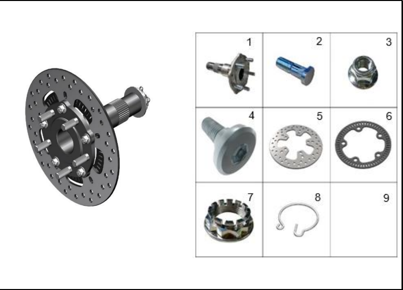
FIGURA 68: EJE RUEDA TRASERA
