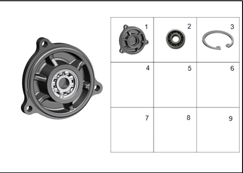
FIGURA 128: TAPA PIÑÓN REDUCTOR ARRANQUE
