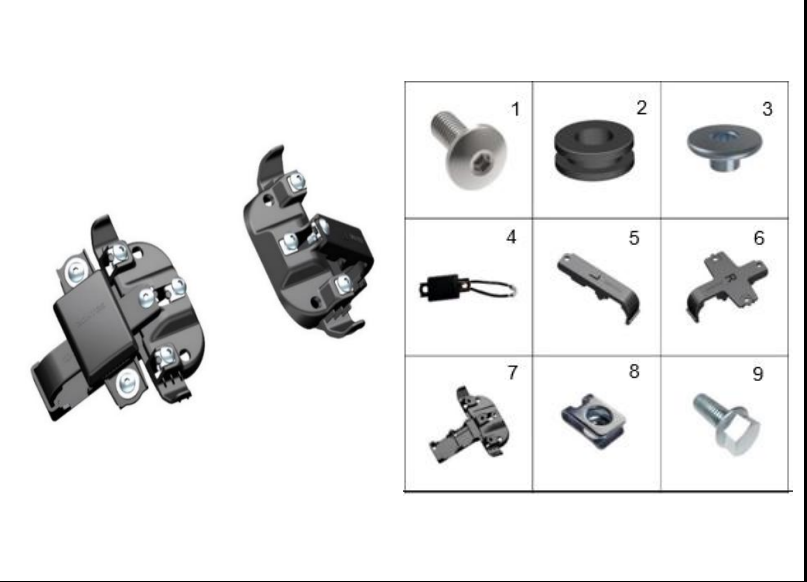
FIGURA 8: CUBIERTA
