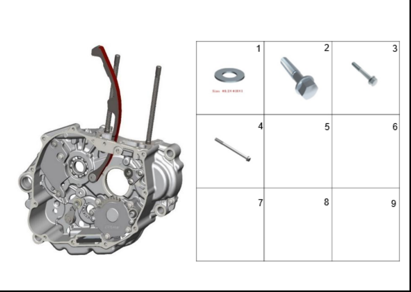
FIGURA 123: CARCASA DERECHA
