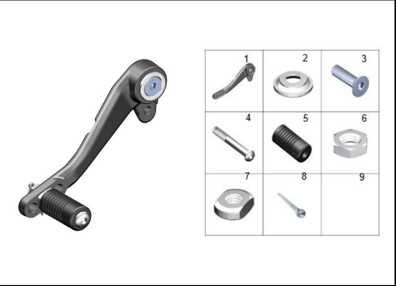
FIGURA 89: PEDAL DE CAMBIOS
