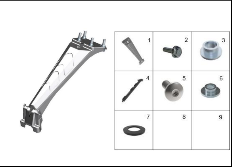
FIGURA 38: SOPORTE GUARDABARRO TRASERO
