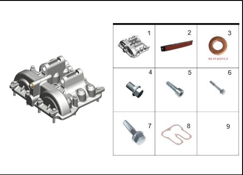
FIGURA 108: TAPA CULATA
