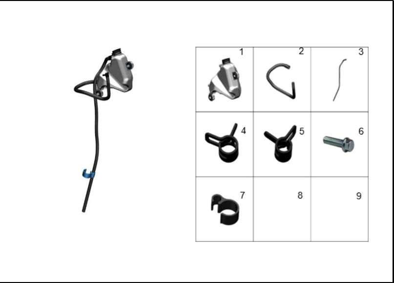
FIGURA 99: TANQUE RESERVORIO
