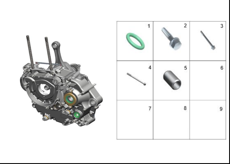
FIGURA 119: CARCASA IZQUIERDA
