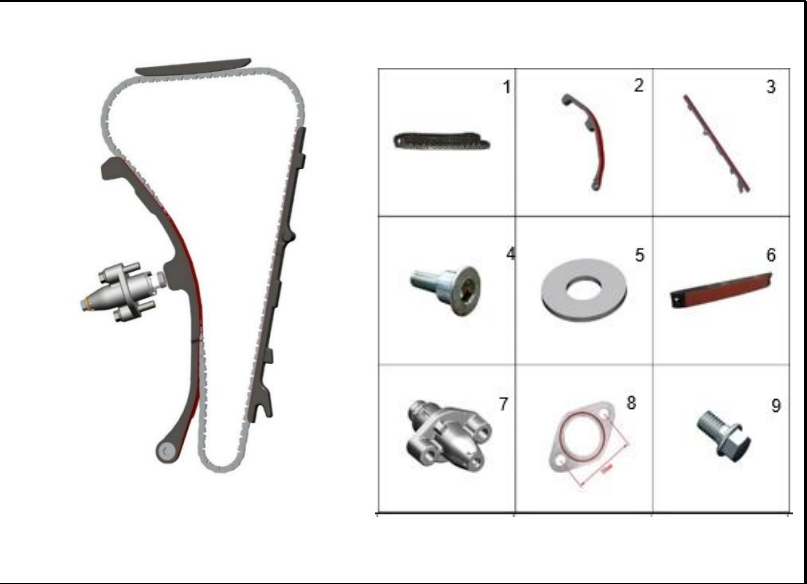
FIGURA 133: CADENILLA DE DISTRIBUCIÓN
