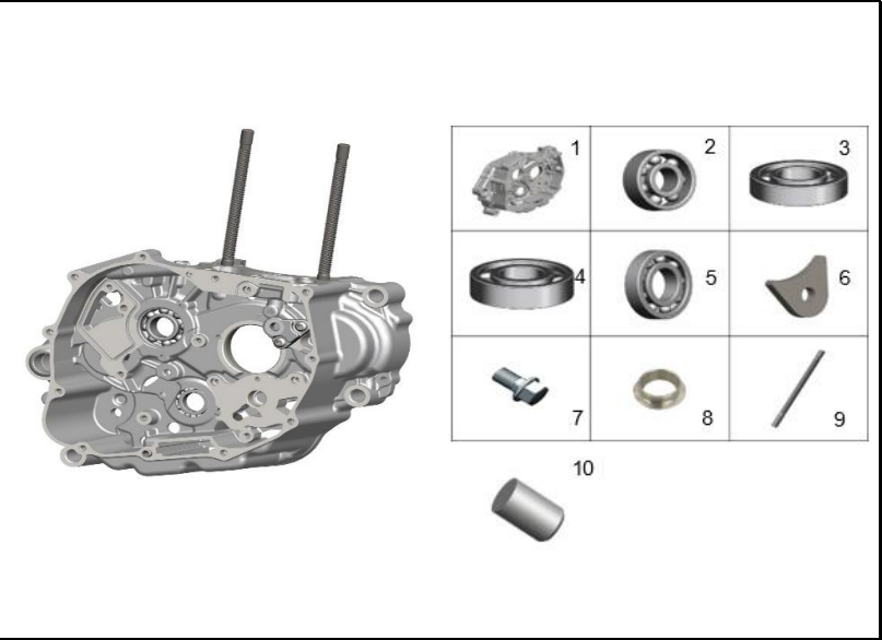
FIGURA 125: CARCASA DERECHA 3
