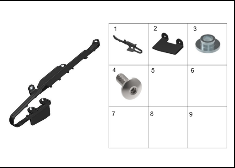
FIGURA 57: DESLIZADOR DE CADENA
