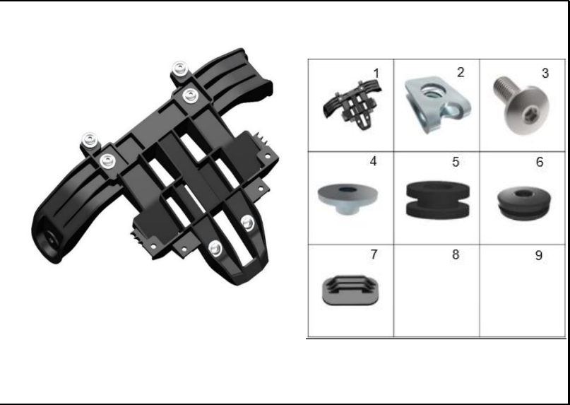
FIGURA 17: SOPORTE TANQUE COMBUSTIBLE 2
