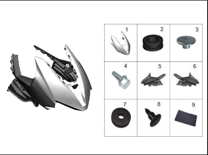
FIGURA 10: CUBIERTA SUPERIOR FAROLA
