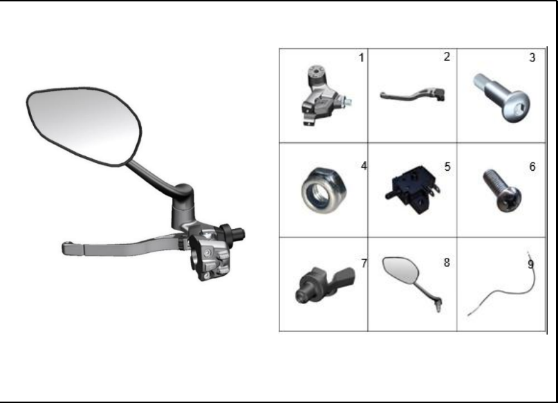
FIGURA 46: LEVA DE CLUTCH-ESPEJO IZQUIERDO
