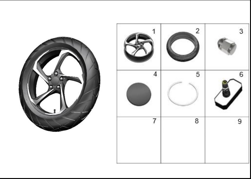
FIGURA 69: LLANTA TRASERA
