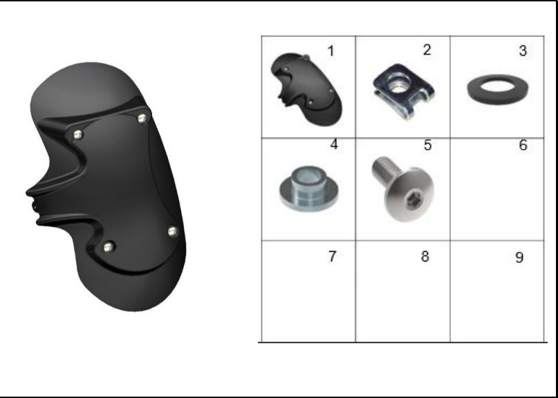
FIGURA 63: GUARDABARRO LLANTA
