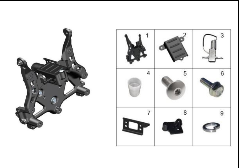
FIGURA 6: SOPORTE PARABRISAS
