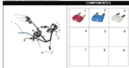
FIGURA N° 76: PARTES ELECTRICAS
