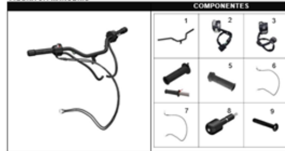
FIGURA 57: MANUBRIO
