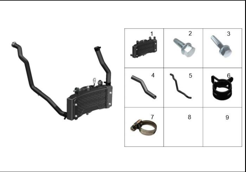
FIGURA 102: RADIADOR INFERIOR
