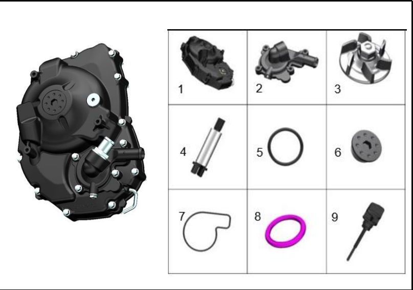
FIGURA 125: TAPA CARCASA DERECHA
