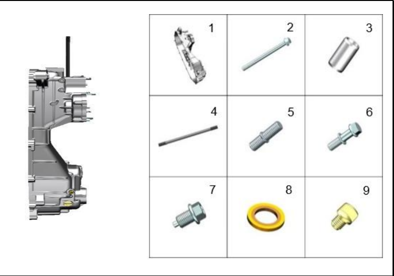
FIGURA 115: CARCASA IZQUIERDA MOTOR
