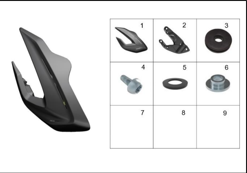
FIGURA 88: CUBIERTA TRASERA INFERIOR
