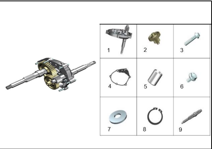
FIGURA 119: TRANSMISIÓN
