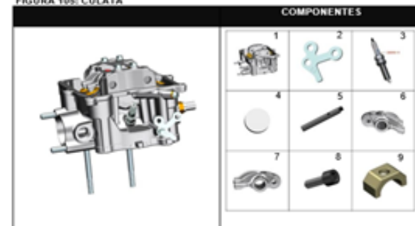
FIGURA 105: CULATA
