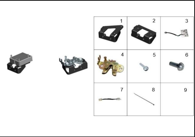
FIGURA 37: SEGURO SILLIN
