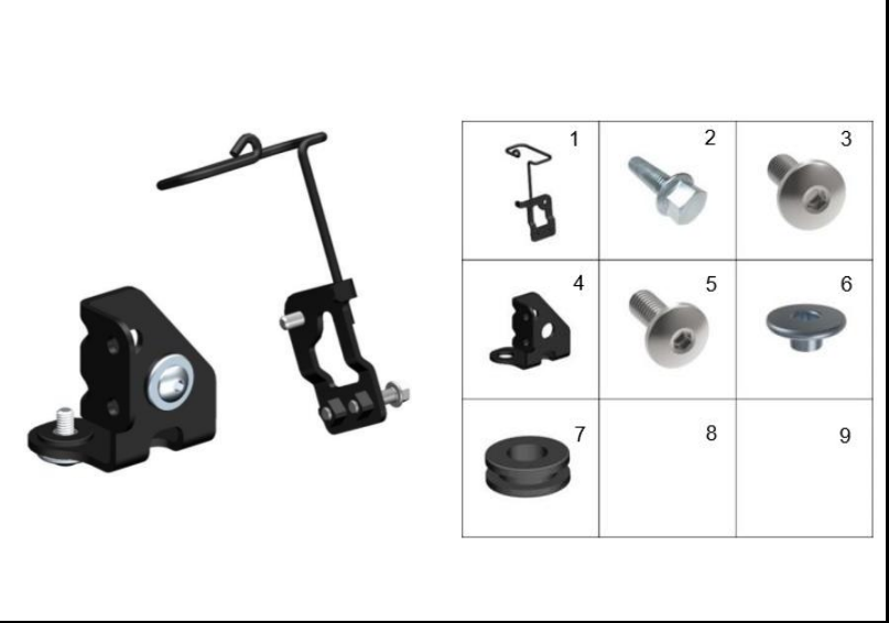
FIGURA 63: SOPORTE MANGUERA DE FRENO
