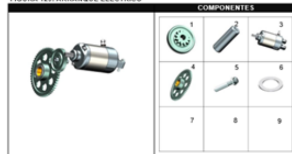
FIGURA 129: ARRANQUE ELECTRICO
