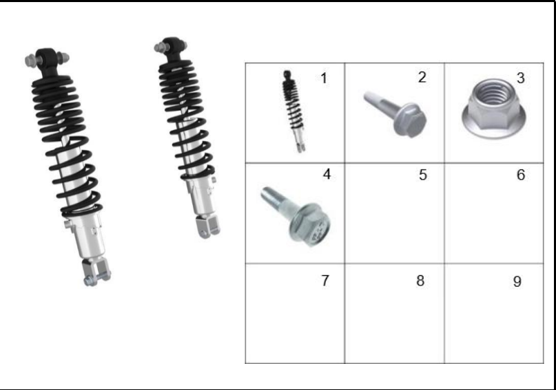
FIGURA 71: AMORTIGUADORES TRASEROS
