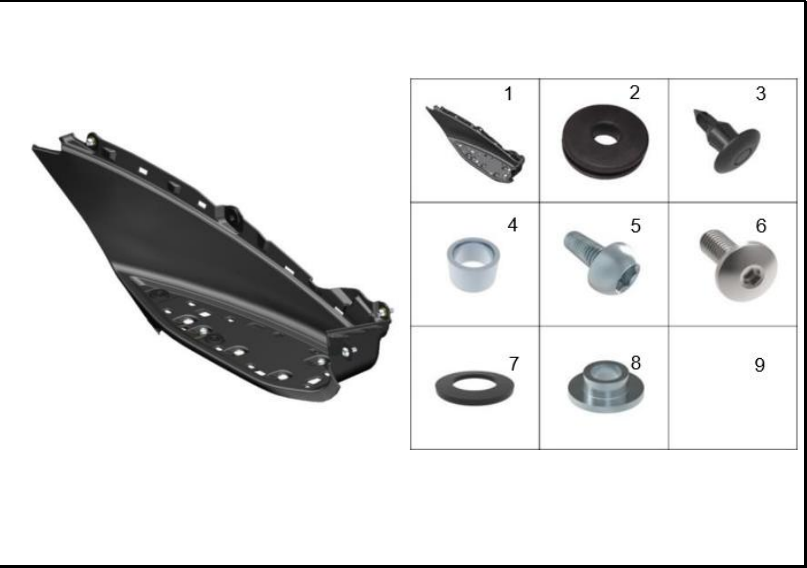
FIGURA 23: REPOSAPIE DERECHO
