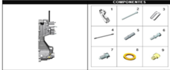
FIGURA 116: CARCASA IZQUIERDA MOTOR
