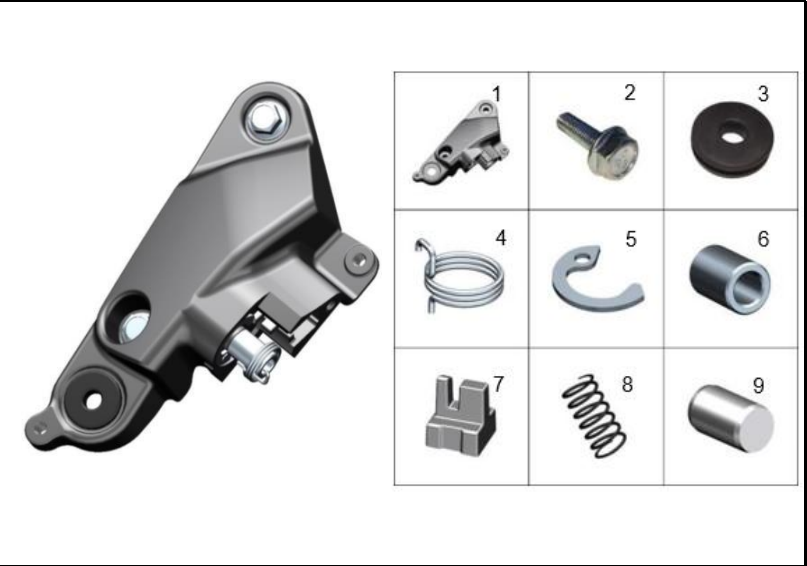
FIGURA 94: PLATINA REPOSAPIES IZQ
