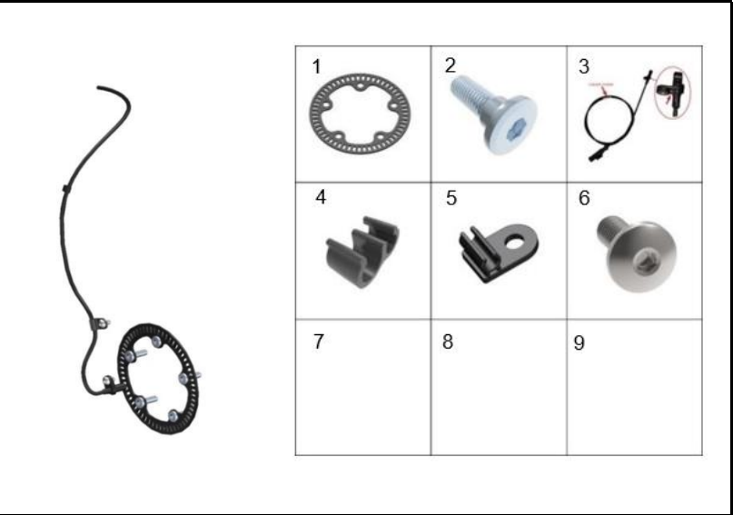
FIGURA 69: RUEDA FONICA ABS FRENO DELANTERO
