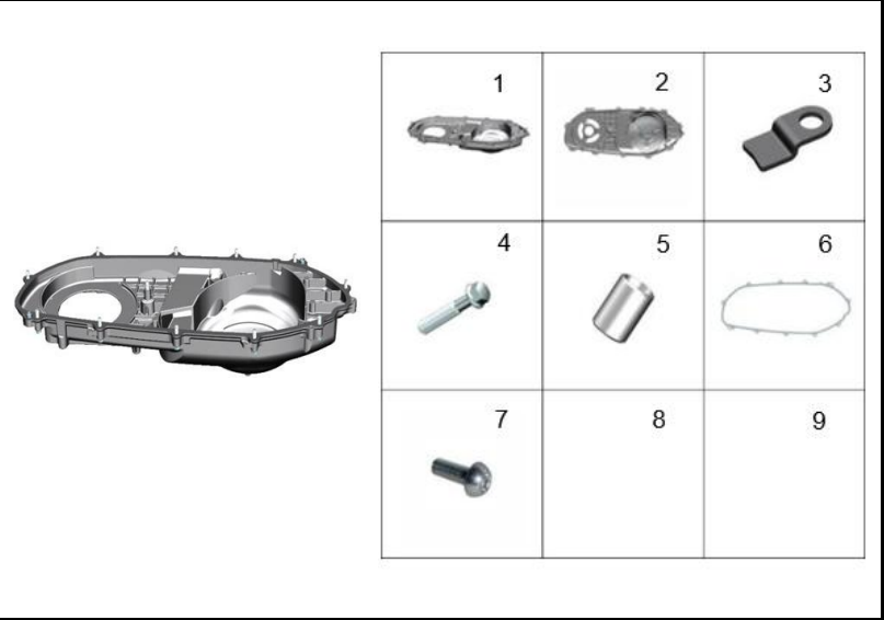
FIGURA 123: CARCASA MOTOR IZQUIERDA 2
