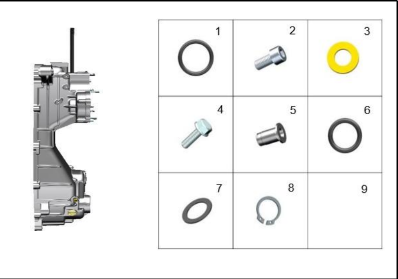
FIGURA 115A: CARCASA IZQUIERDA MOTOR 2
