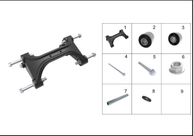
FIGURA 81: SOPORTE MOTOR
