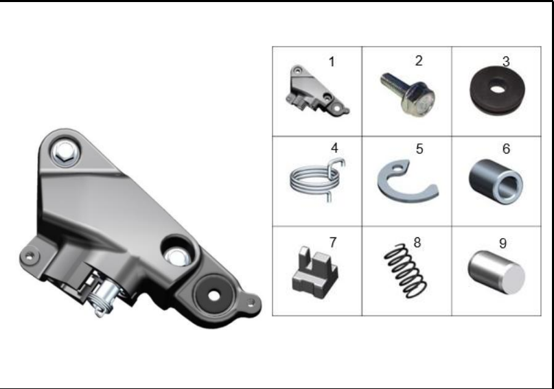
FIGURA 95: PLATINA REPOSAPIES DER
