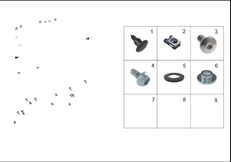
FIGURA 27: PARTES DE SUJECION
