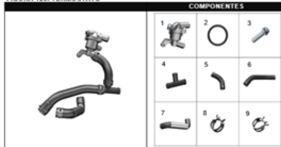
FIGURA 128: TERMOSTATO
