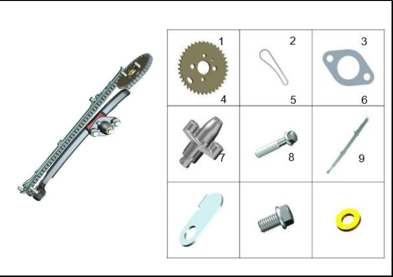
FIGURA 131: SISTEMA DE TRANSMISION
