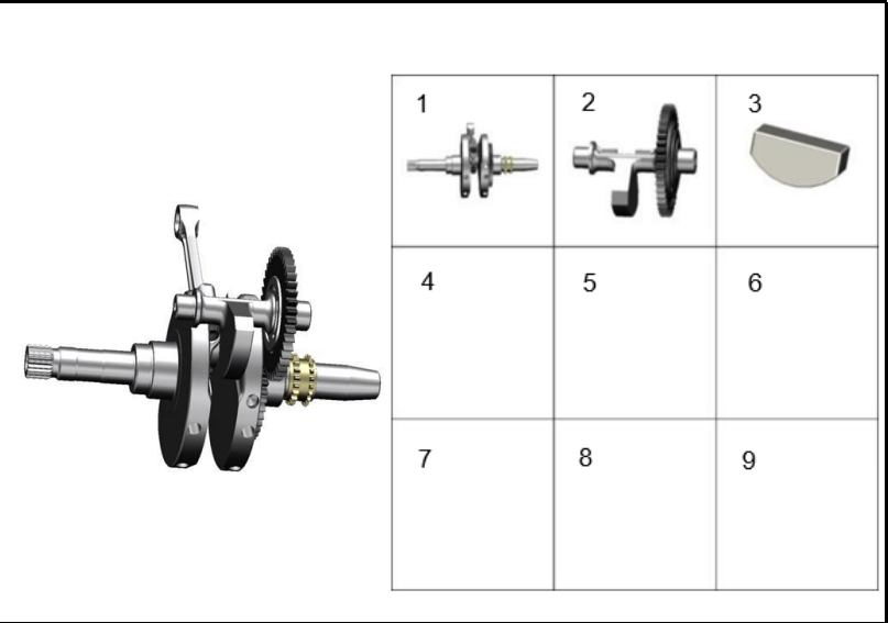
FIGURA 114: CIGÜEÑAL
