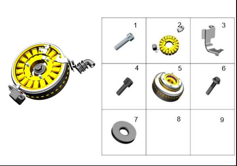
FIGURA 130: PLATO BOBINA
