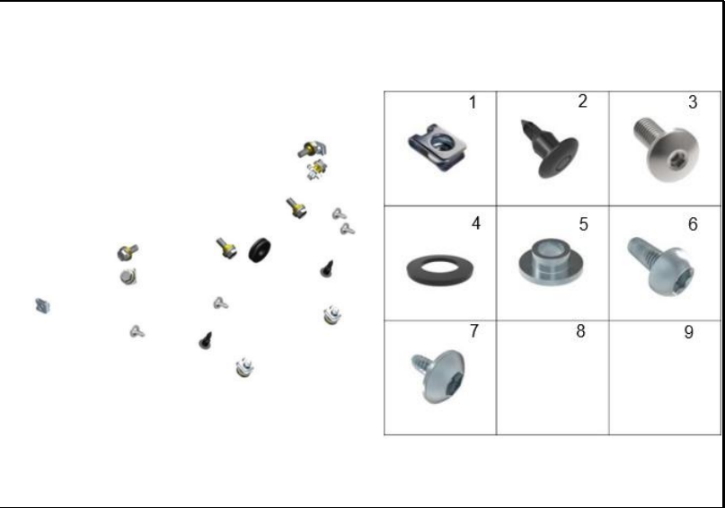
FIGURA 56: PARTES DE SUJECION 3
