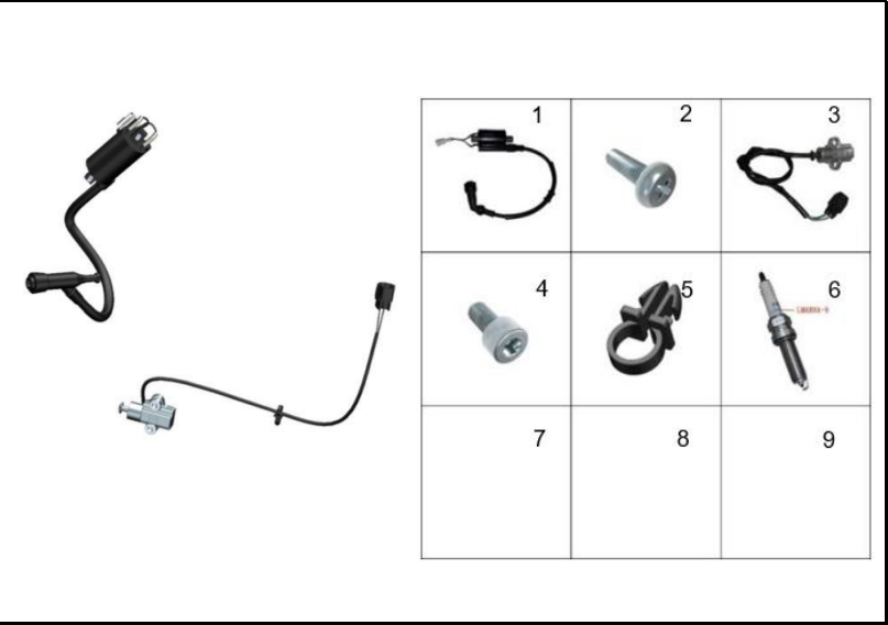
FIGURA 79: PARTES ELECTRICAS
