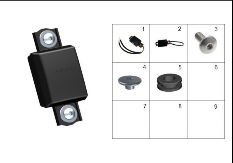
FIGURA 3: CONTROLADOR PARABRISAS
