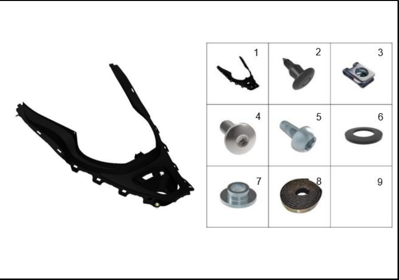
FIGURA 40: CUBIERTA CENTRAL TANQUE
