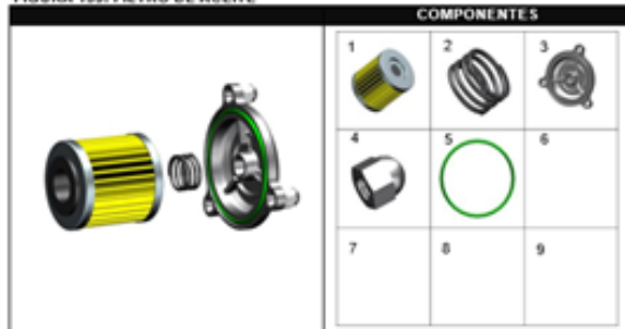
FIGURA 133: FILTRO DE ACEITE
