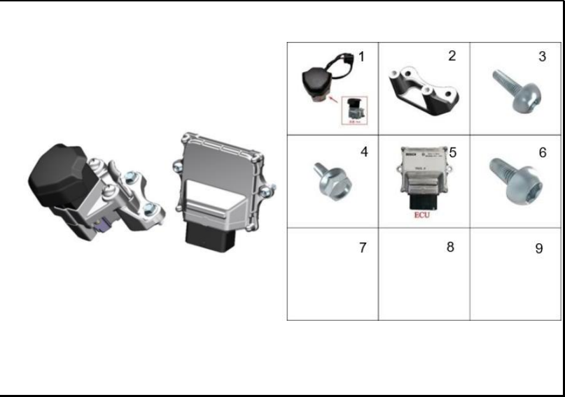
FIGURA 77: ECU - CERRADURA ELECTRÓNICA
