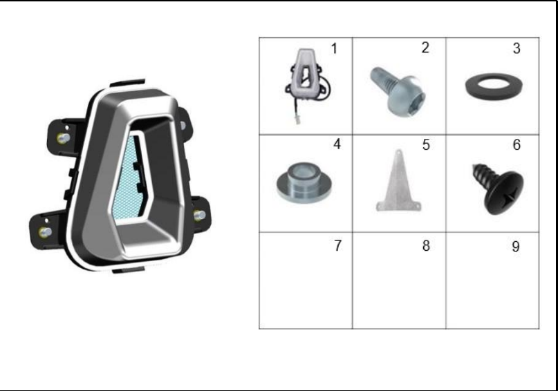
FIGURA 17: LUZ POSICION
