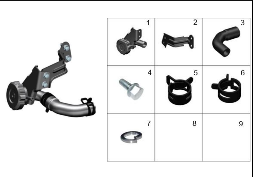
FIGURA 100: TAPA RADIADOR
