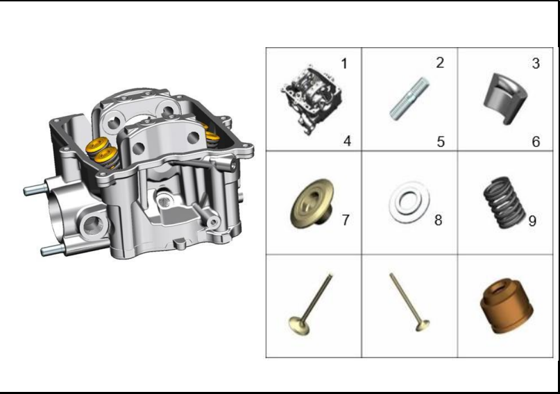
FIGURA 107: CULATA - VALVULAS
