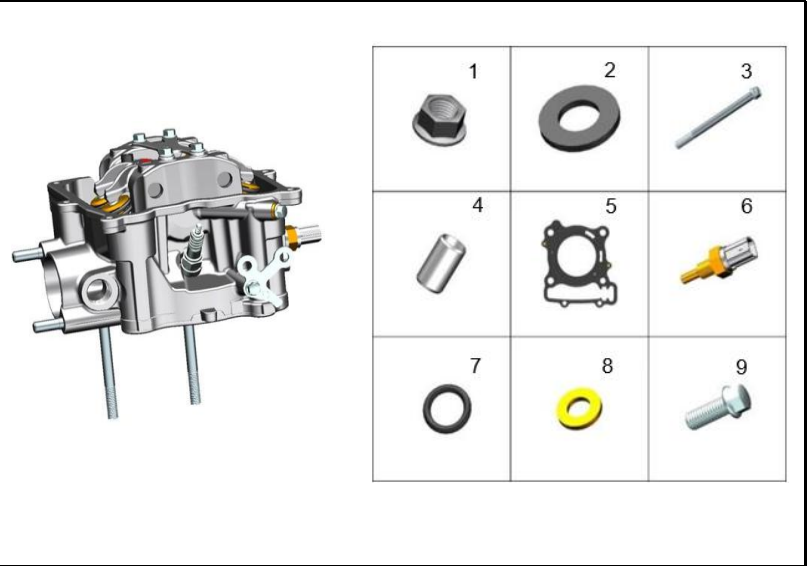
FIGURA 106: CULATA - EMPAQUE CULATA
