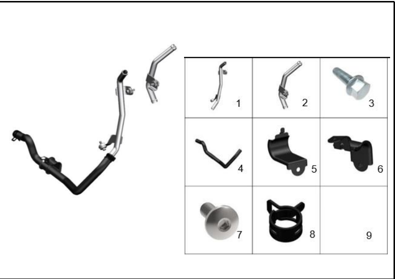
FIGURA 103: DUCTOS DE REFRIGERACIÓN
