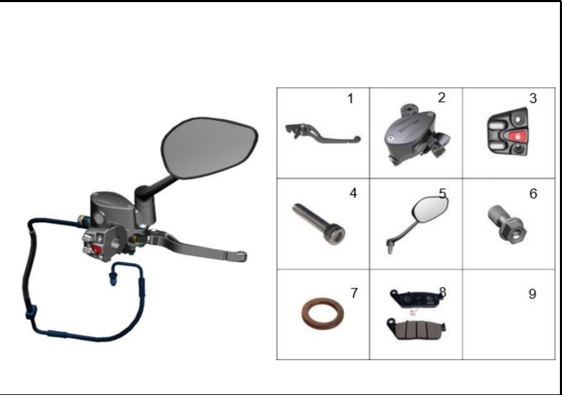
FIGURA 61: LEVA DE FRENO DELANTERO
