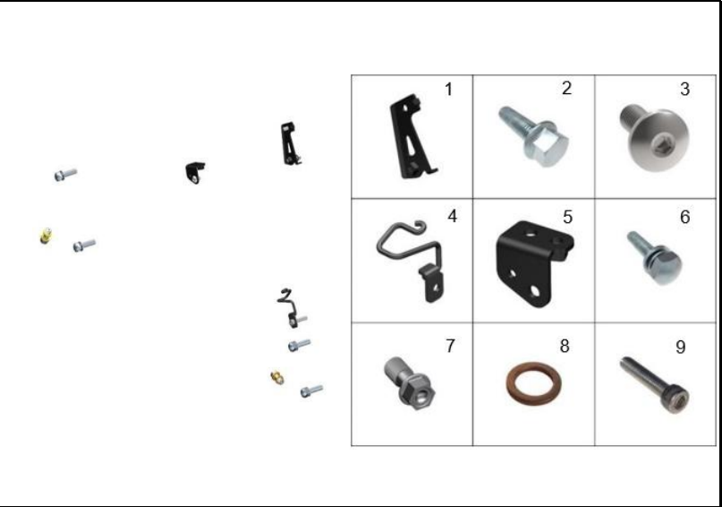
FIGURA 64: SOPORTE MANGUERA DE FRENO DELANTERO
