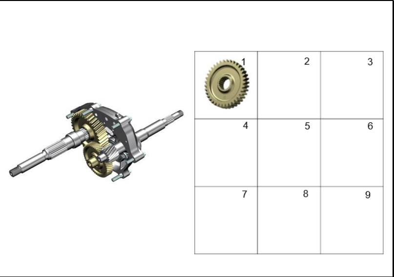
FIGURA 120: TRANSMISIÓN 2
