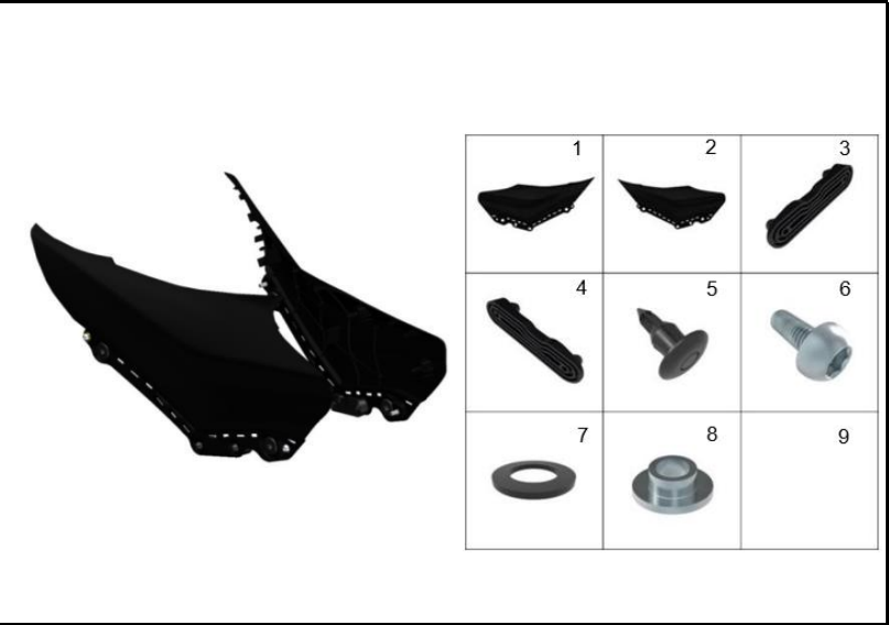
FIGURA 41: CUBIERTAS LATERALES TANQUE
