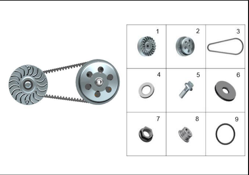
FIGURA 111: TRASMISIÓN
