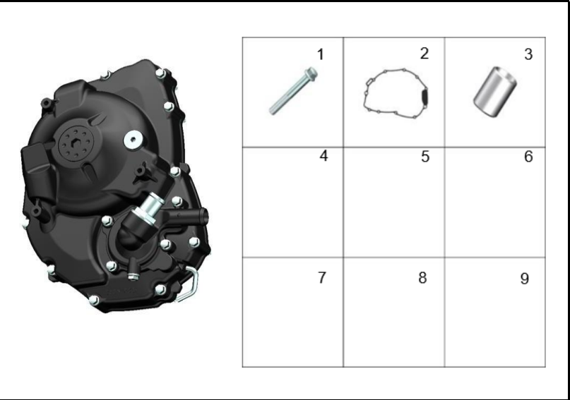
FIGURA 126A: TAPA CARCASA DERECHA 2
