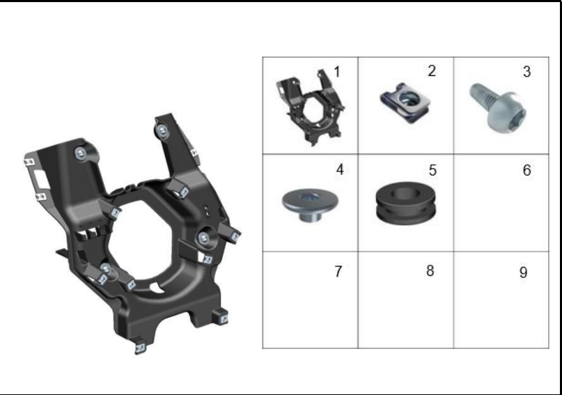
FIGURA 10: SOPORTE FAROLA
