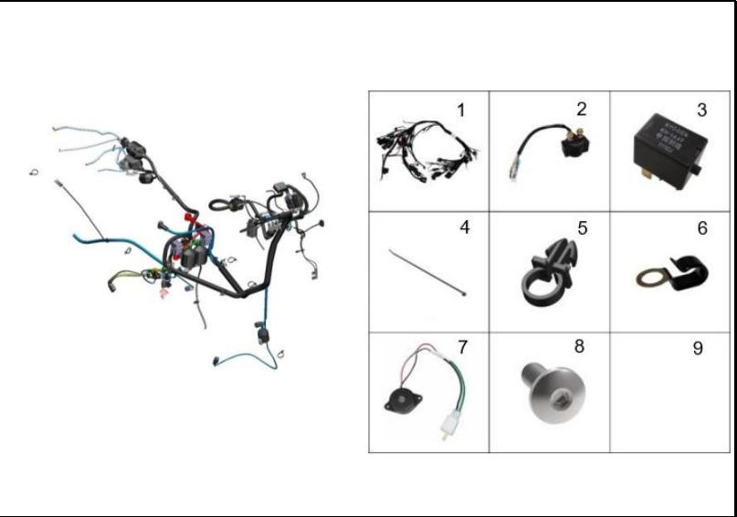
FIGURA 76: PARTES ELÉCTRICAS 1
