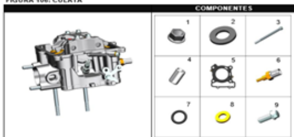
FIGURA 106: CULATA
