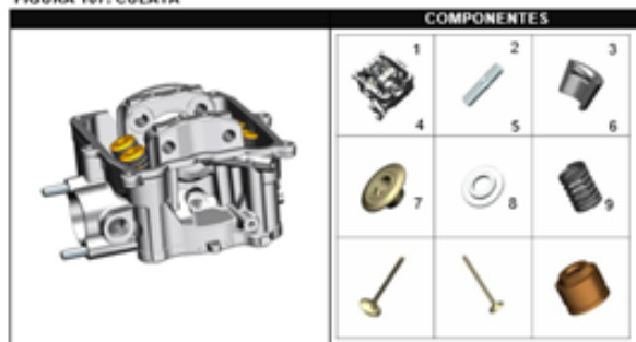
FIGURA 107: CULATA
