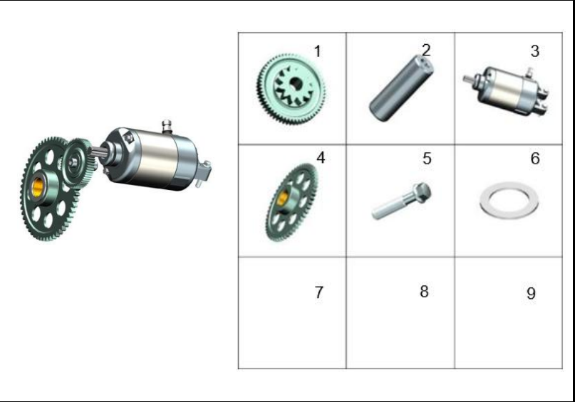
FIGURA 129: ARRANQUE ELÉCTRICO
