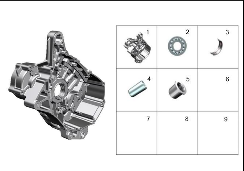
FIGURA 118: CARCASA MOTOR DERECHA 3
