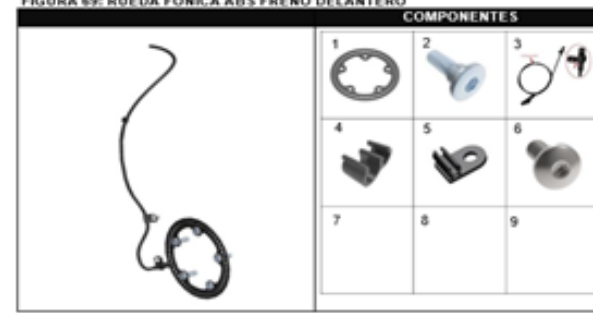
FIGURA 69: RUEDA FONICA ABS FRENO DELANTERO
