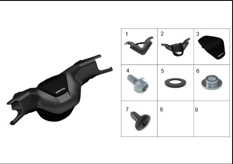
FIGURA 59: CUBIERTA MANUBRIO
