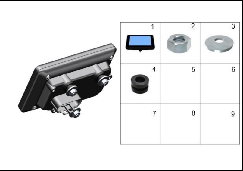
FIGURA 7: VELOCIMETRO
