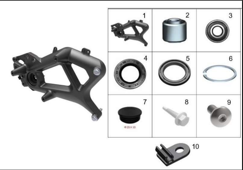
FIGURA 74: SOPORTE MOTOR
