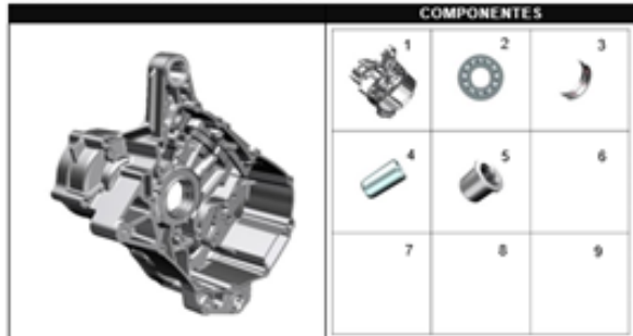
FIGURA 118: CARCASA MOTOR DERECHA
