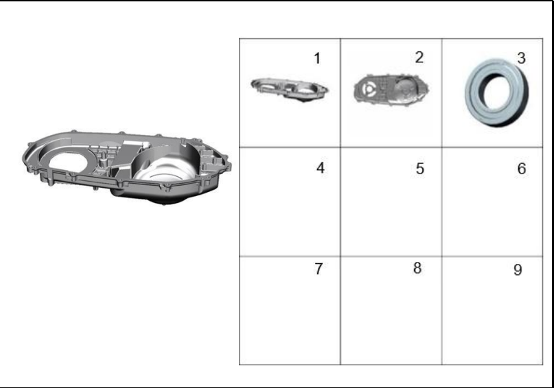
FIGURA 124: CARCASA MOTOR IZQUIERDA 3
