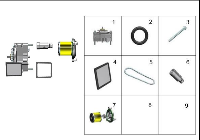
FIGURA 132: BOMBA DE ACEITE
