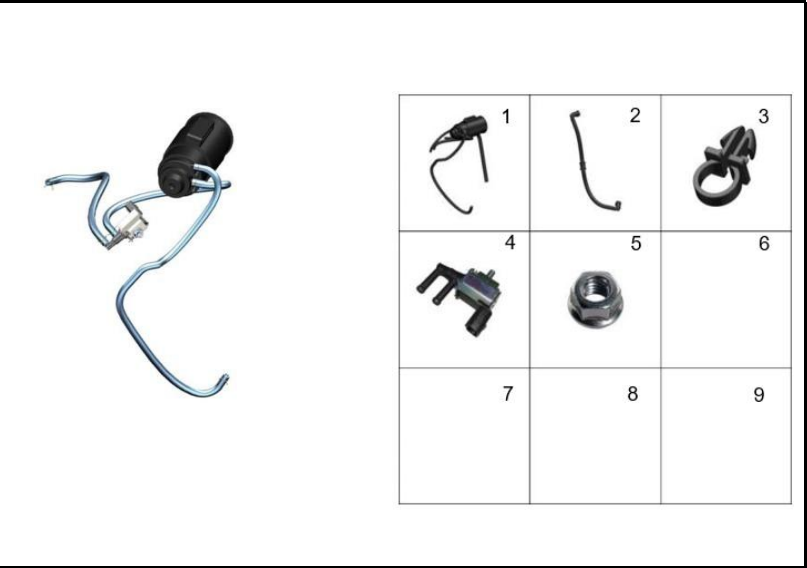
FIGURA 84: CANISTER
