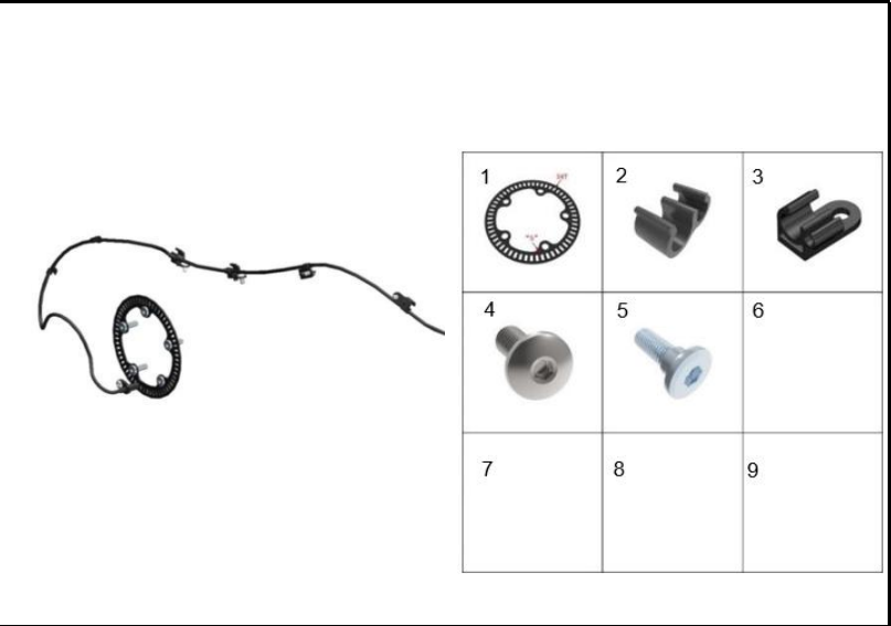
FIGURA 73: RUEDA FONICA ABS FRENO TRASERO
