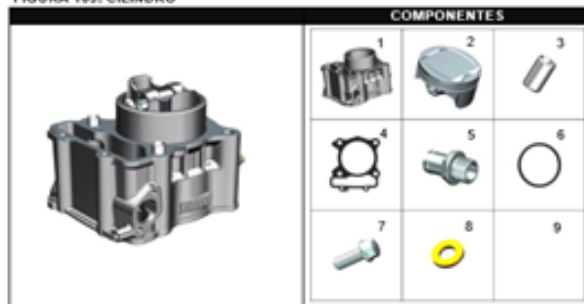
FIGURA 109: CILINDRO
