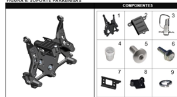
FIGURA 6: SOPORTE PARABRISAS
