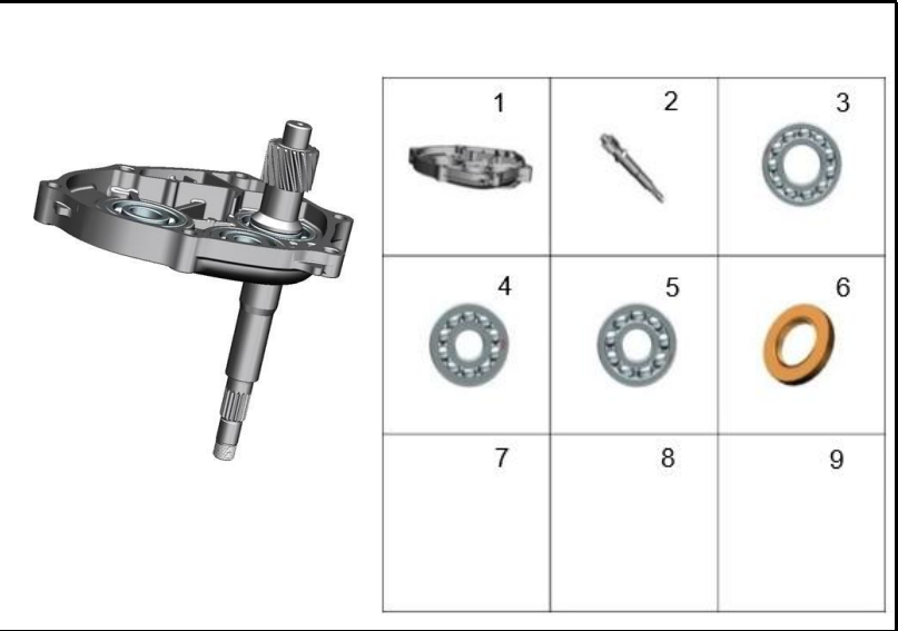
FIGURA 121: CUBIERTA TRANSMISION
