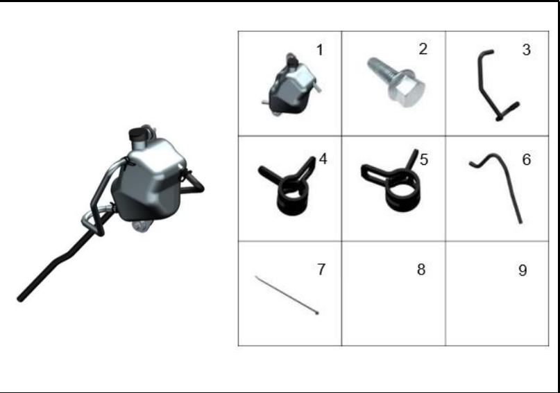
FIGURA 101: RESERVORIO REFRIGERANTE
