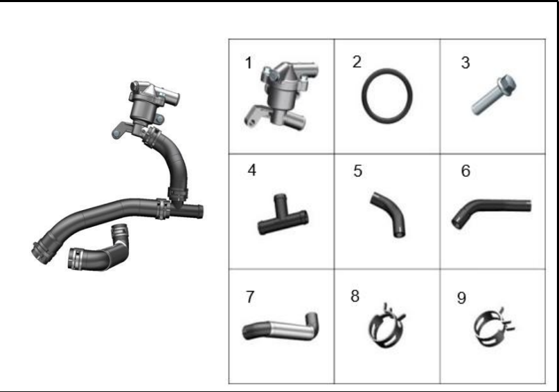
FIGURA 128: TERMOSTATO
