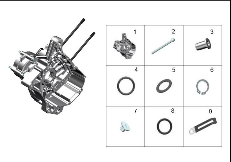
FIGURA 117: CARCASA MOTOR DERECHA
