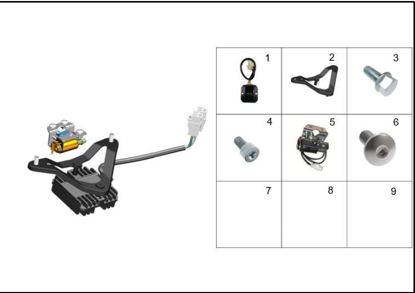
FIGURA 80: REGULADOR - SEGURO ELECTRÓNICO SILLÍN®
