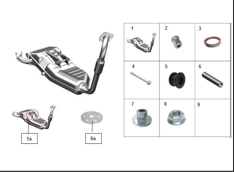
FIGURA 73: SILENCIADOR
