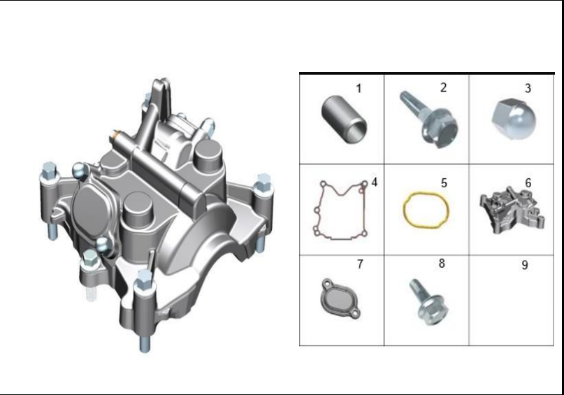
FIGURA 88: CUBIERTA CULATA
