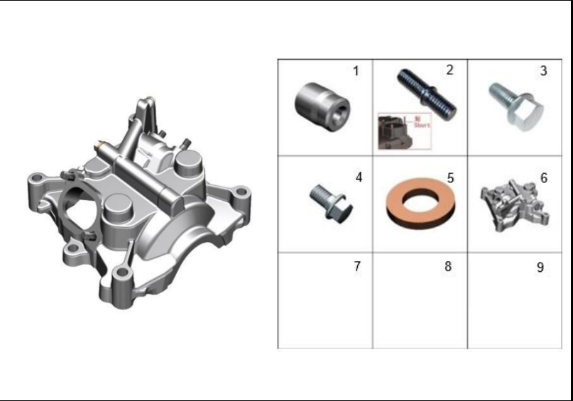
FIGURA 89: CUBIERTA CULATA 2
