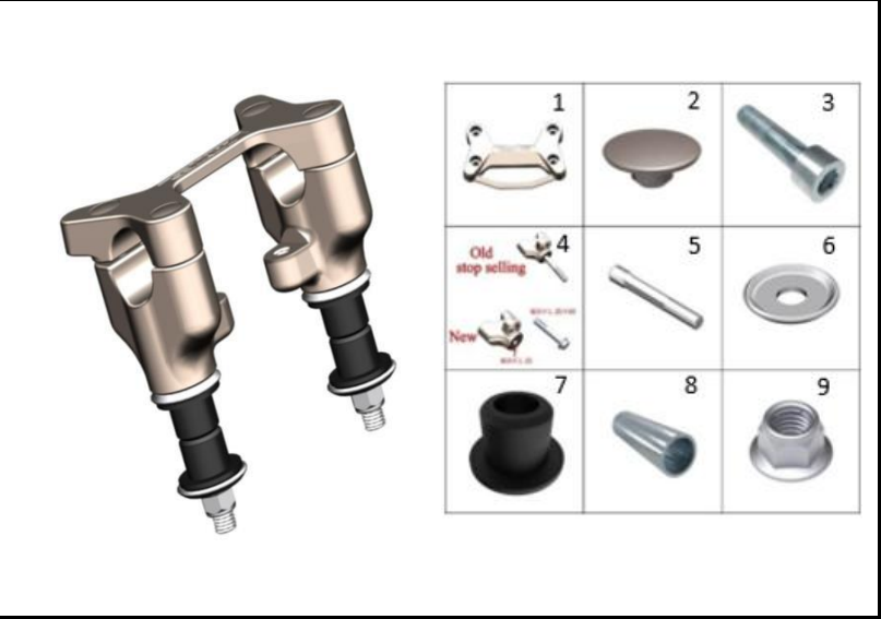
FIGURA 34: SOPORTES MANUBRIO
