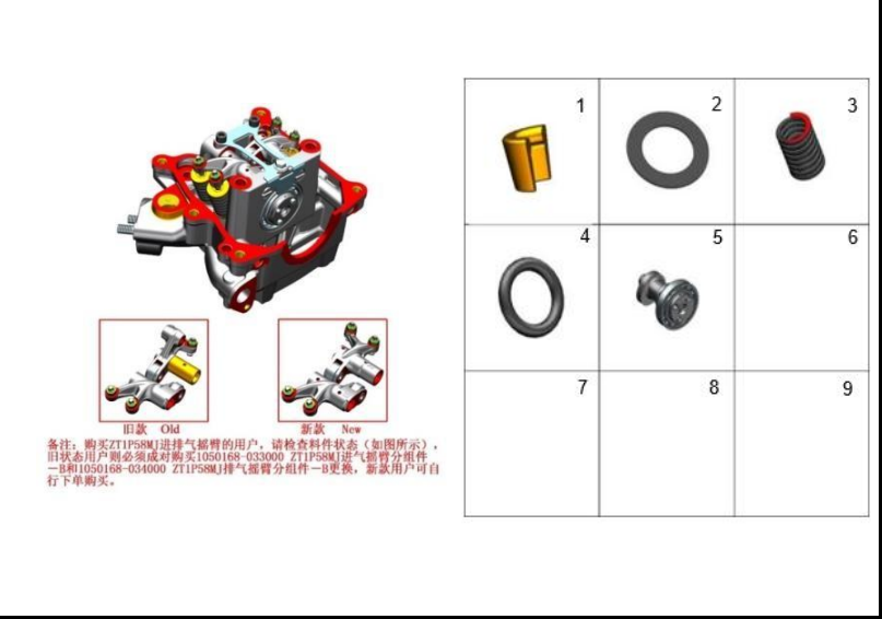
FIGURA 93: VALVULAS 3
