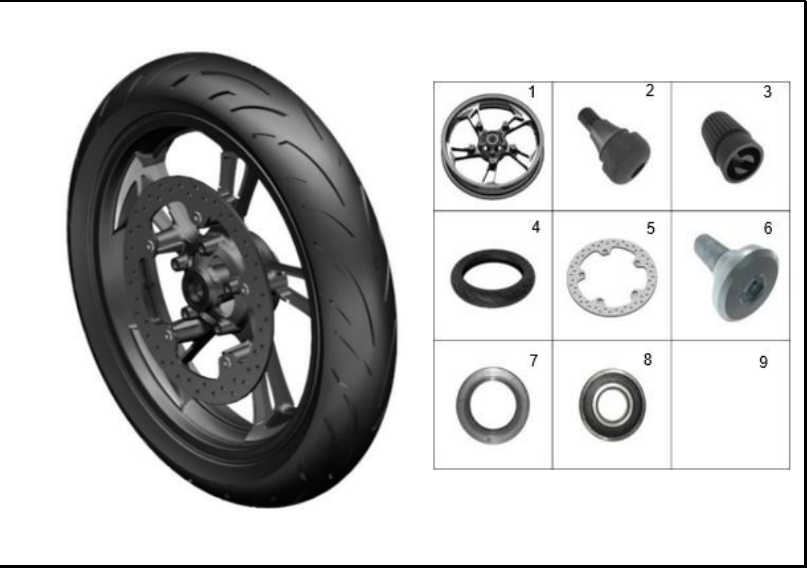
FIGURA 44: RUEDA DELANTERA
