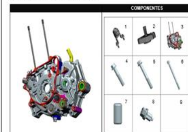
FIGURA 108: CARCASA IZQUIERDA
