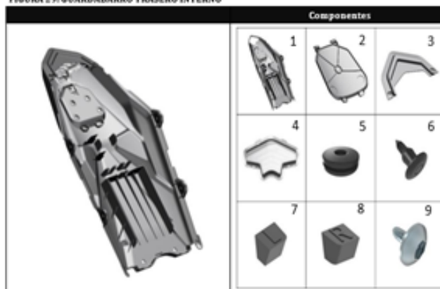
FIGURA 29: GUARDABARRO TRASERO INTERNO
