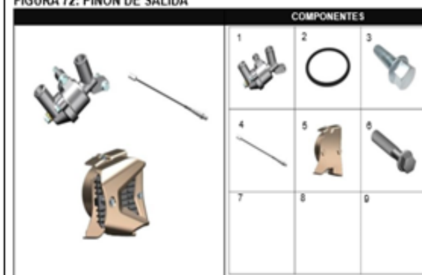
FIGURA 72: PIÑÓN DE SALIDA
