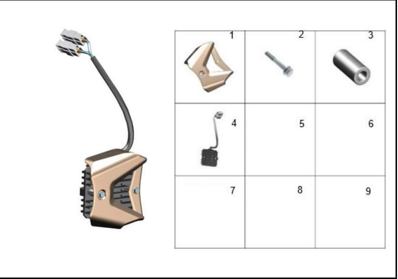
FIGURA 62: PARTES ELÉCTRICAS 3
