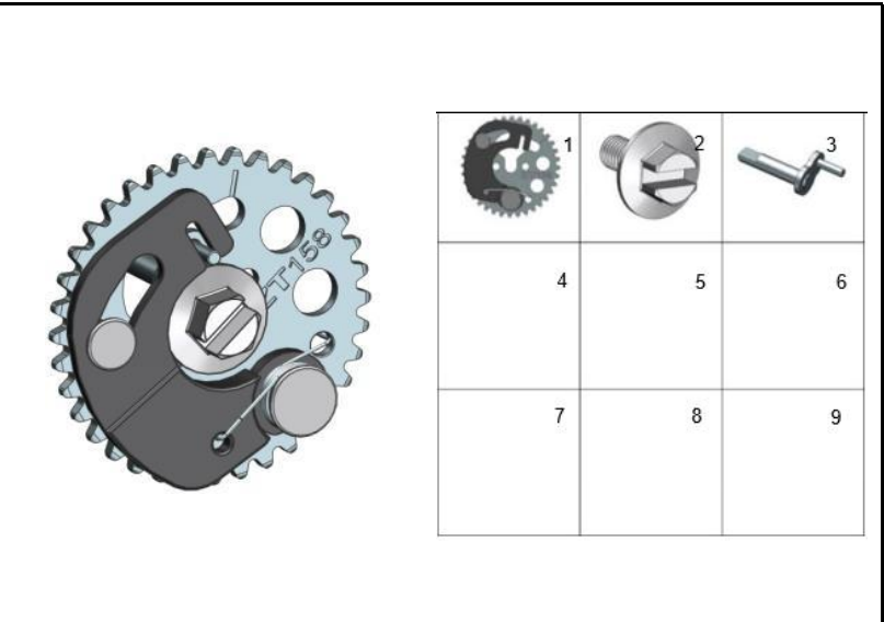
FIGURA 131: DESCOMPRESOR
