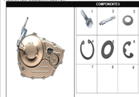
FIGURA 120: CUBIERTA CLUTCH
