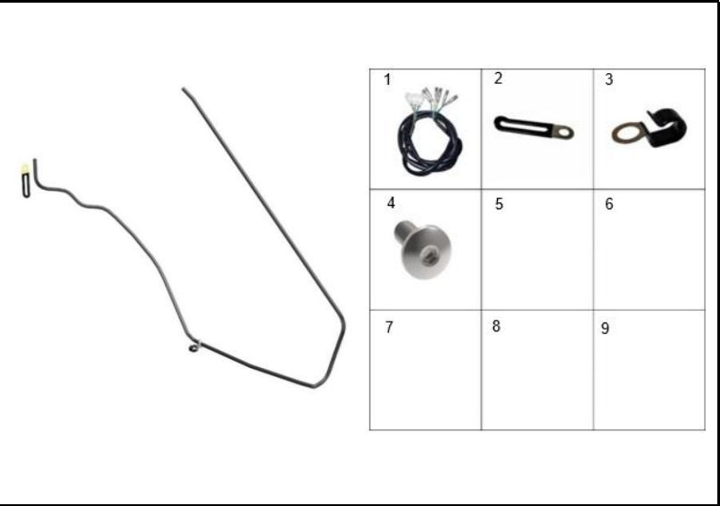
FIGURA 58: RAMAL ELÉCTRICO
