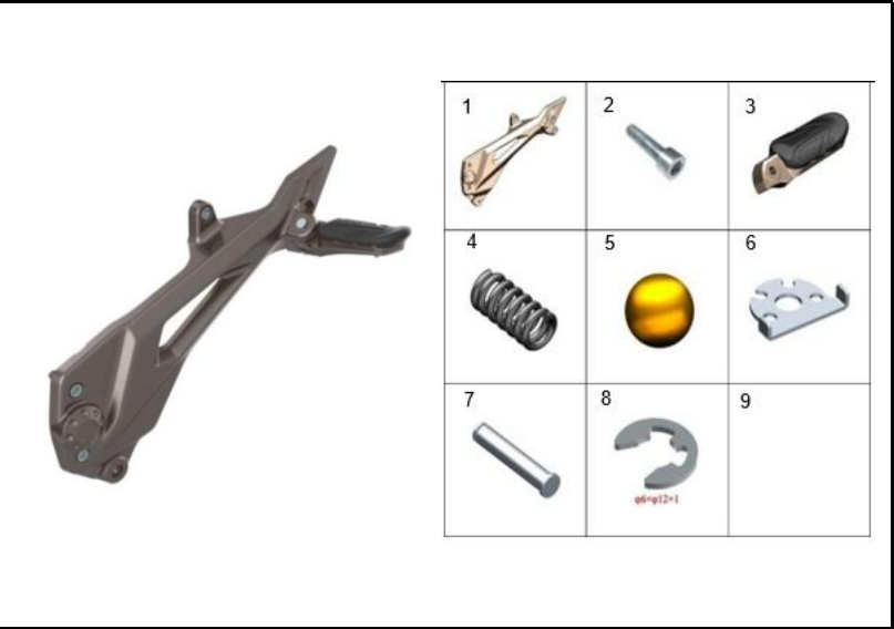
FIGURA 75: SOPORTE REPOSAPIE TRASERO IZQUIERDO
