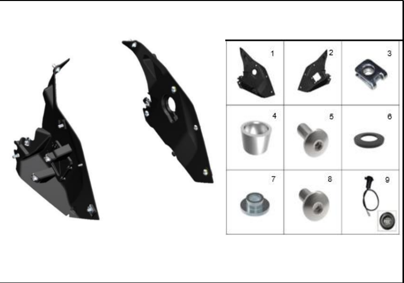
FIGURA 16 : SOPORTES CUBIERTAS TANQUE COMBUSTIBLE
