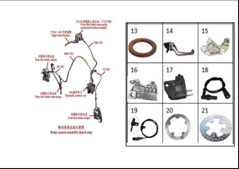
FIGURA 37: CALIPER DELANTERO Y TRASERO 2
