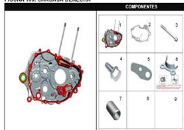
FIGURA 106: CARCASA DERECHA
