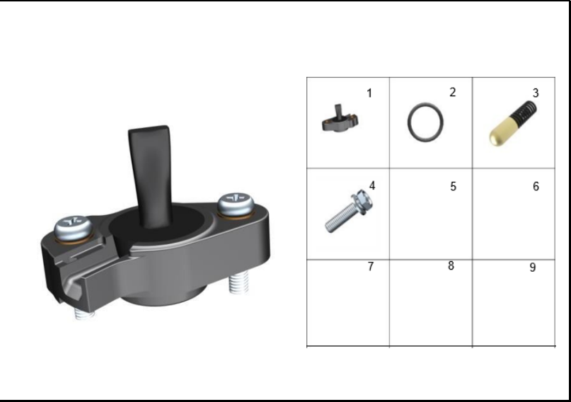
FIGURA 112: SENSOR DE CAMBIOS
