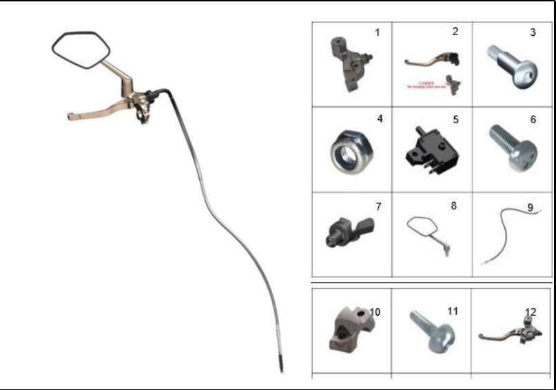
FIGURA 33: LEVA DE CLUTCH-ESPEJO IZQUIERDO
