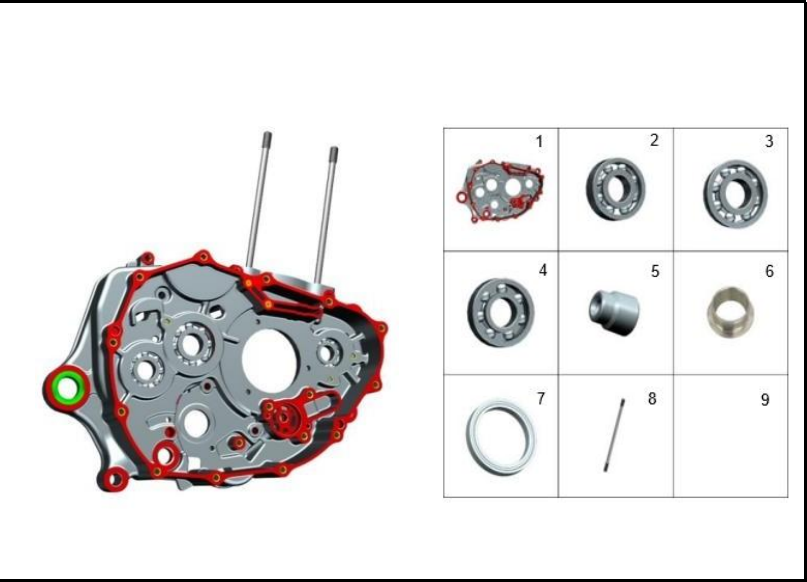
FIGURA 107: CARCASA DERECHA 2
