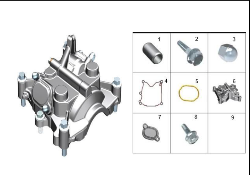
FIGURA 88: CUBIERTA CULATA
