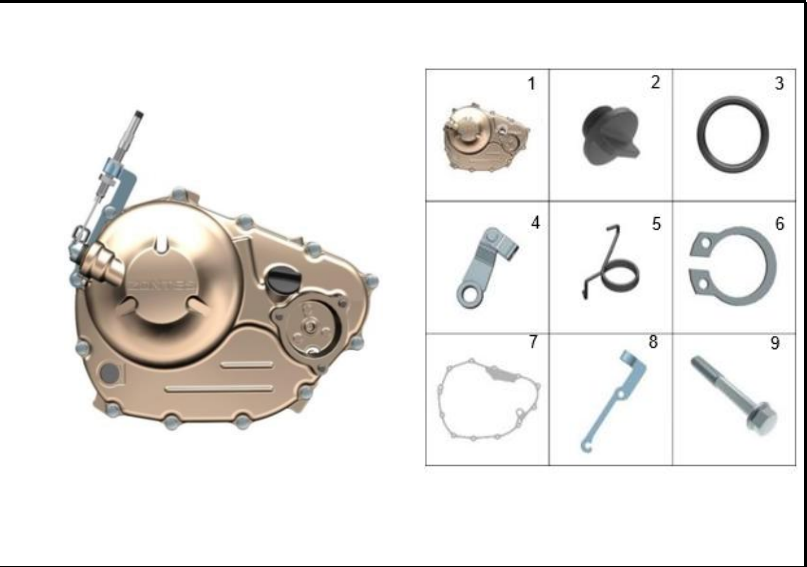
FIGURA 119: CUBIERTA CLUTCH
