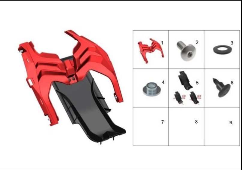
FIGURA 30: CUBIERTAS SILLÍN TRASERO
