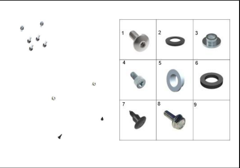
FIGURA 28: TORNILLERIA
