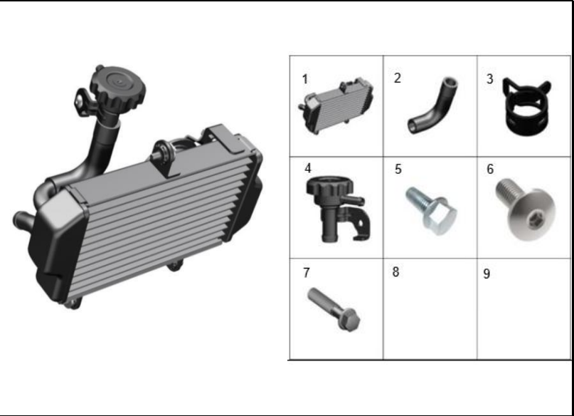
FIGURA 84: RADIADOR
