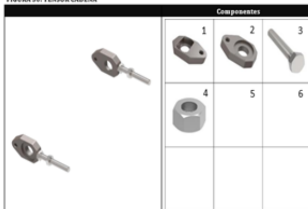
FIGURA 50: TENSOR CADENA
