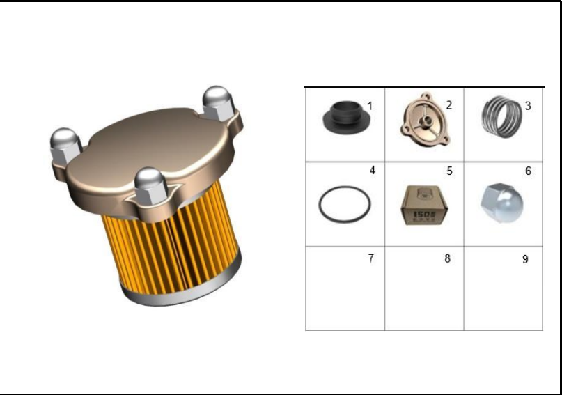
FIGURA 123: FILTRO DE ACEITE
