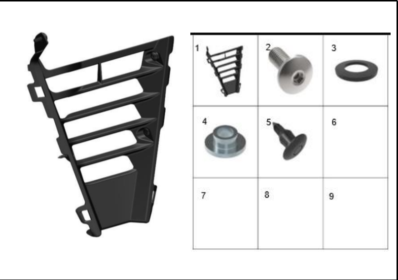
FIGURA 19: REJILLA FRONTAL MOTOR
