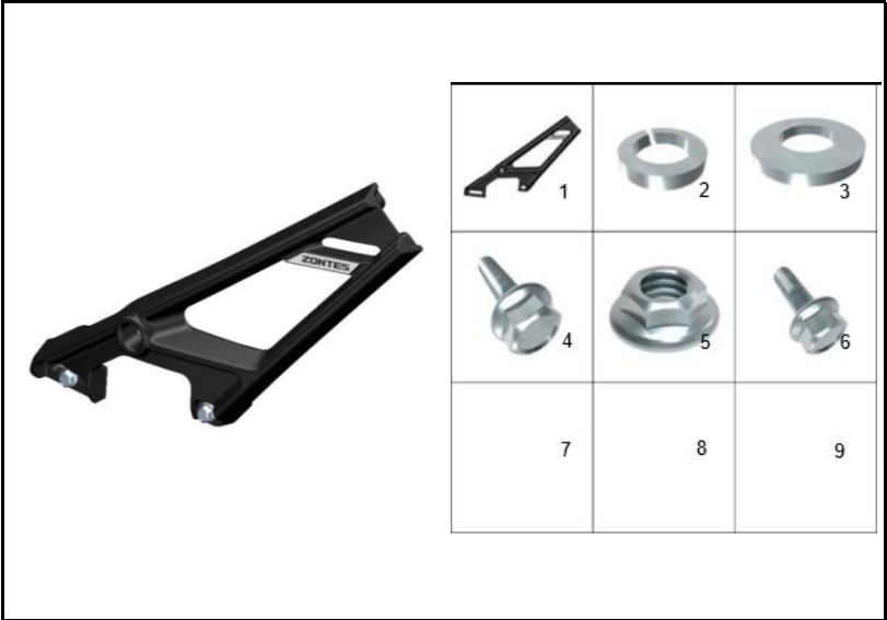
FIGURA 54: SOPORTE GUARDABARRO LLANTA TRASERA
