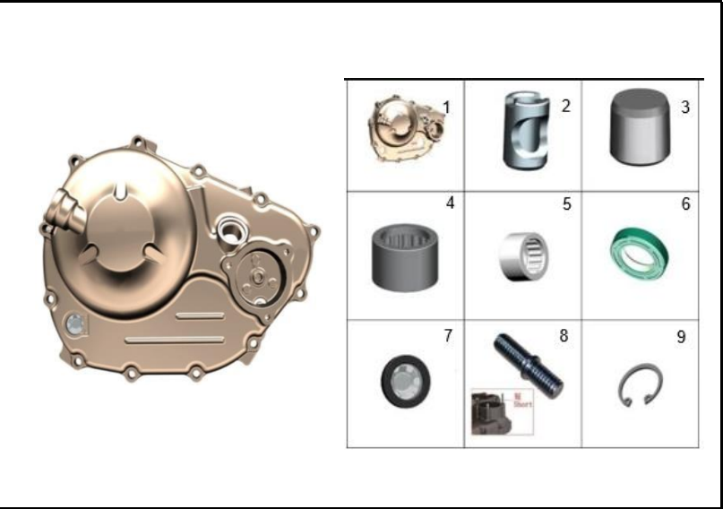
FIGURA 121: CUBIERTA CLUTCH 3
