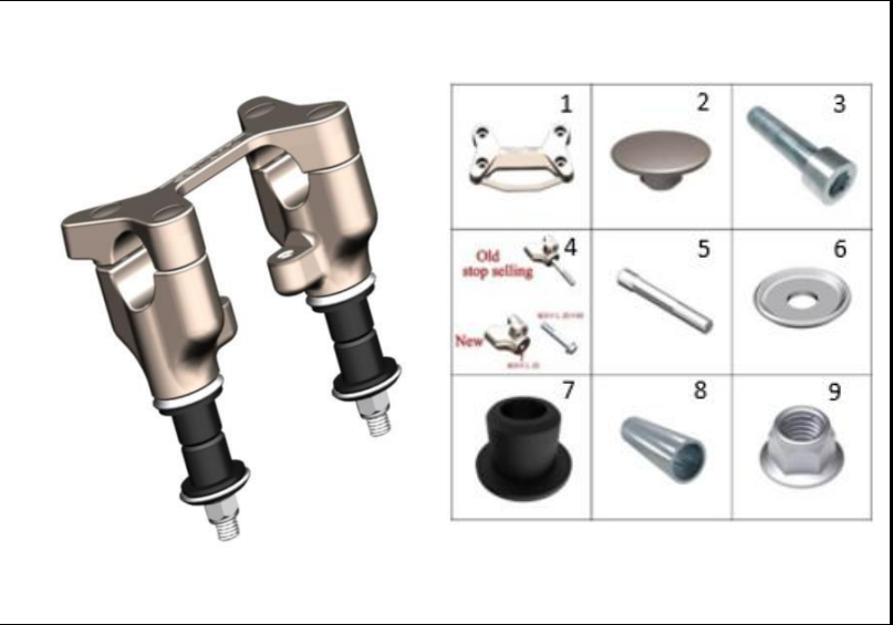
FIGURA 34: SOPORTES MANUBRIO
