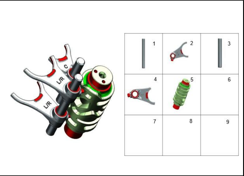
FIGURA 102: HORQUILLA DE CAMBIOS
