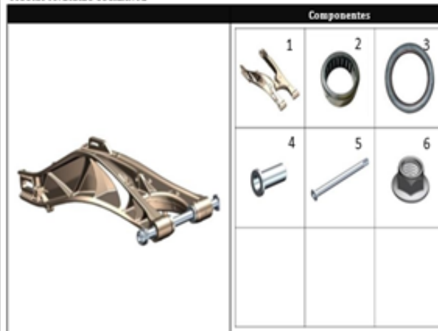
FIGURA 46: BRAZO OSCILANTE
