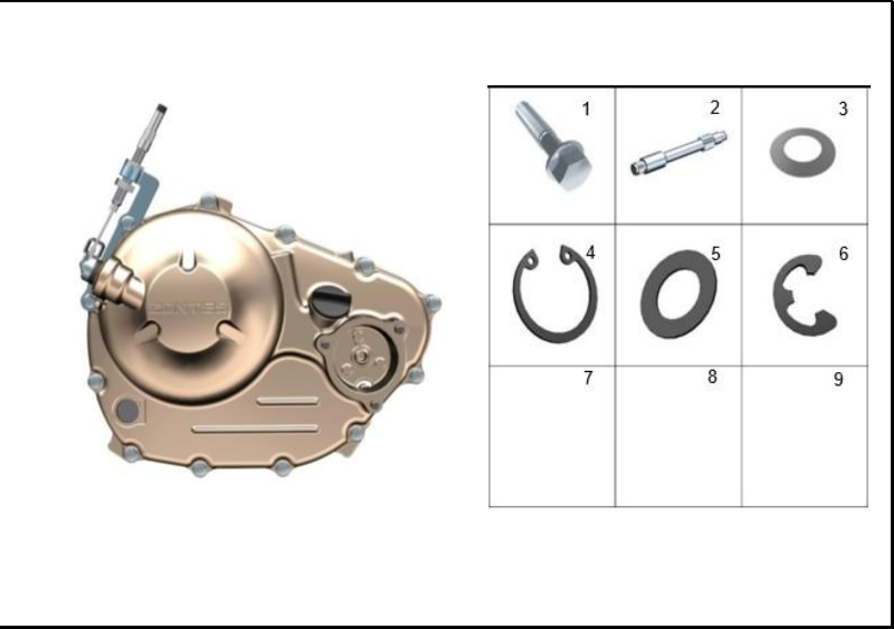
FIGURA 120: CUBIERTA CLUTCH 2
