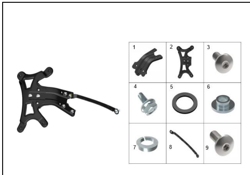
FIGURA 56: SOPORTE GUARDABARRO LLANTA TRASERA 2
