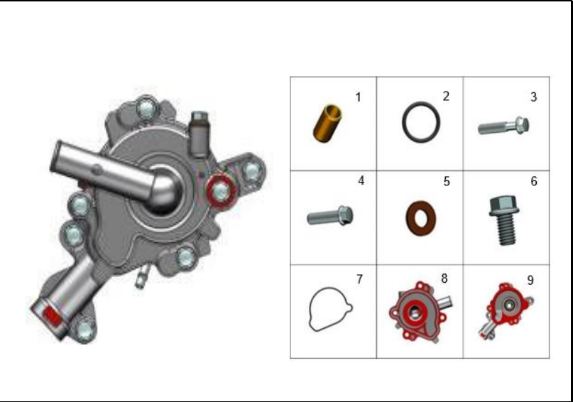
FIGURA 94: BOMBA DE AGUA
