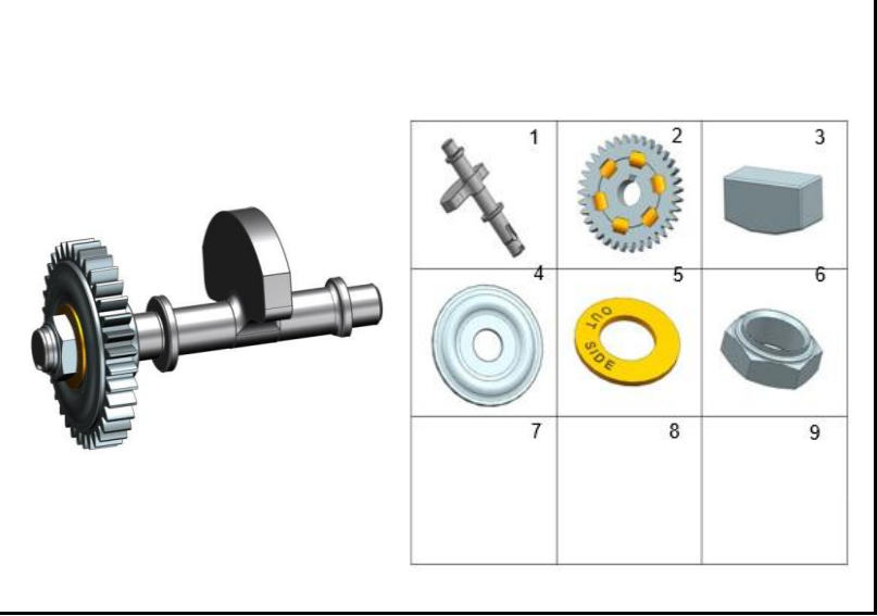
FIGURA 117: BALANCEADOR
