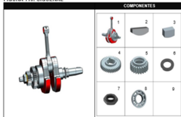
FIGURA 116: CIGUEÑAL
