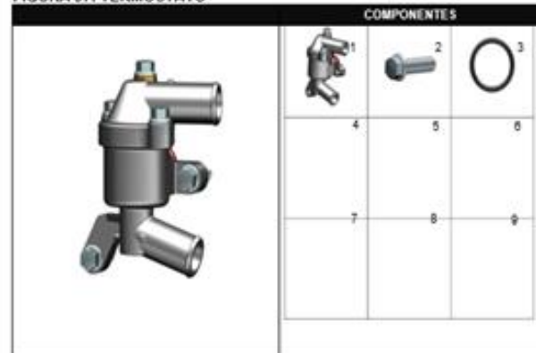
FIGURA 97: TERMOSTATO
