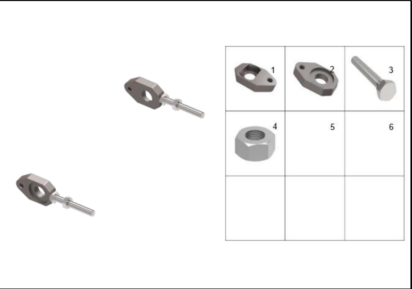
FIGURA 50: TENSOR CADENA
