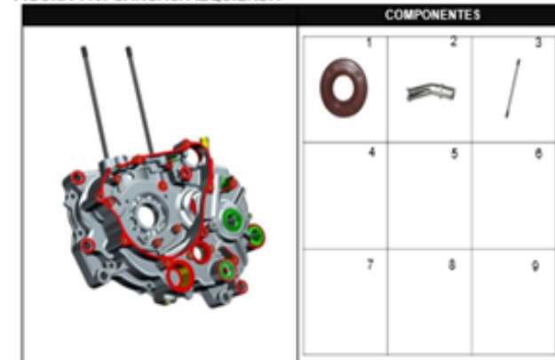
FIGURA 110: CARCASA IZQUIERDA
