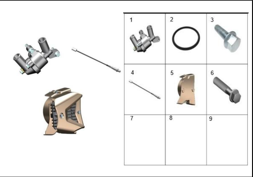
FIGURA 72: PIÑÓN DE SALIDA
