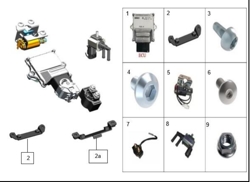
FIGURA 63: ECU - ARRANQUE
