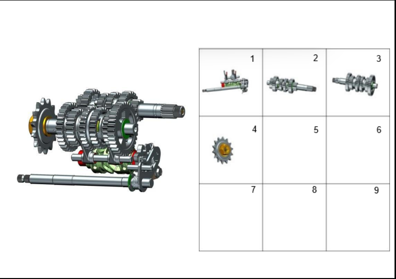
FIGURA 101: TRANSMISIÓN
