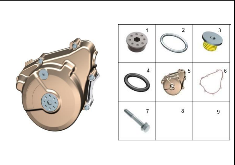
FIGURA 122: CUBIERTA VOLANTE
