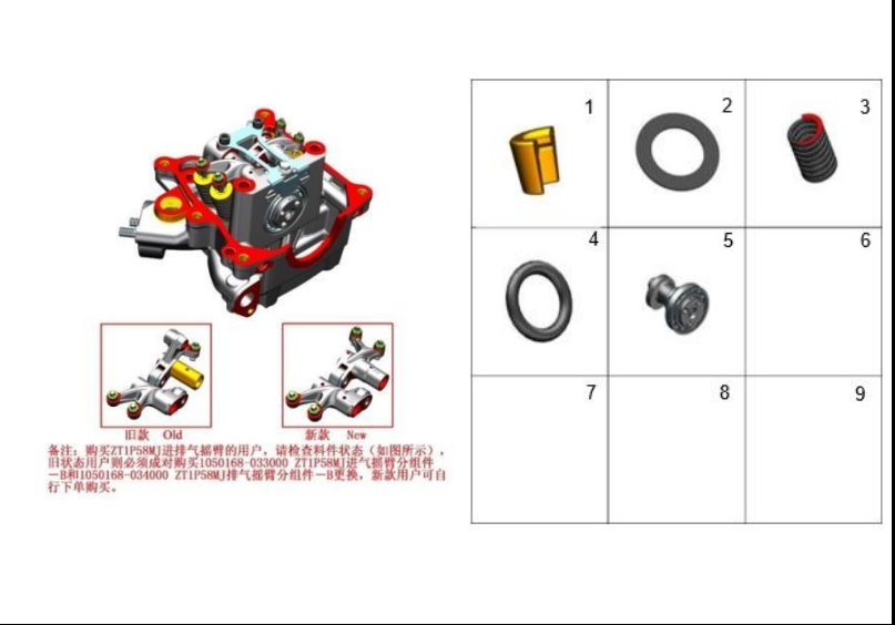
FIGURA 93: VALVULAS 3
