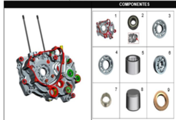
FIGURA 109: CARCASA IZQUIERDA
