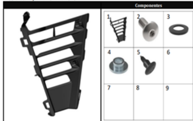
FIGURA 19: REJILLA FRONTAL MOTOR
