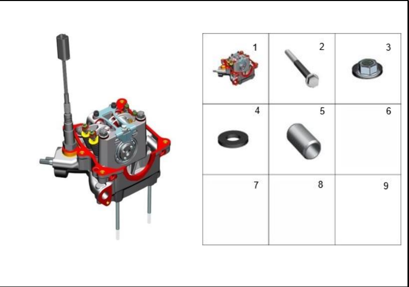
FIGURA 90: CULATA
