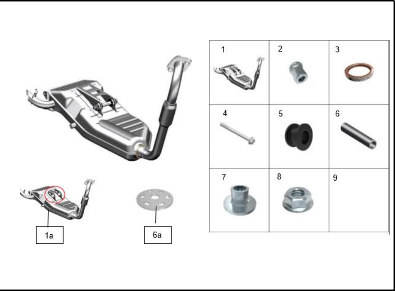
FIGURA 73: SILENCIADOR
