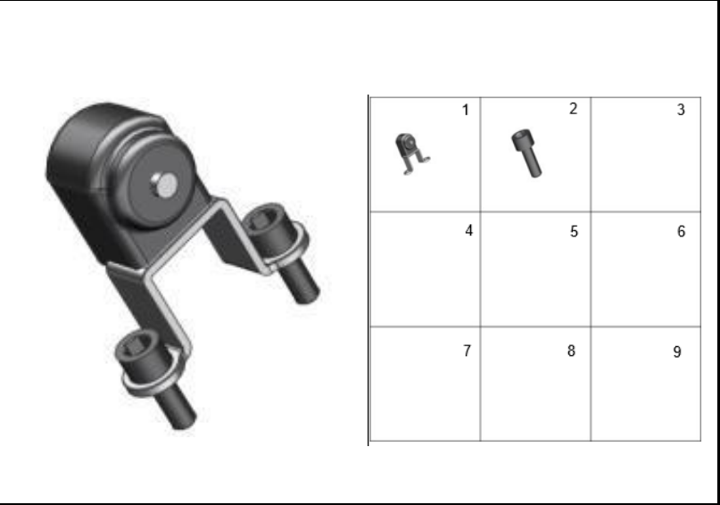
FIGURA 111: SENSOR DE POSICIÓN DEL CIGUEÑAL
