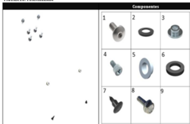
FIGURA 28: TORNILLERIA
