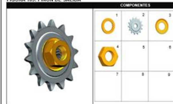
FIGURA 105: PIÑÓN DE SALIDA
