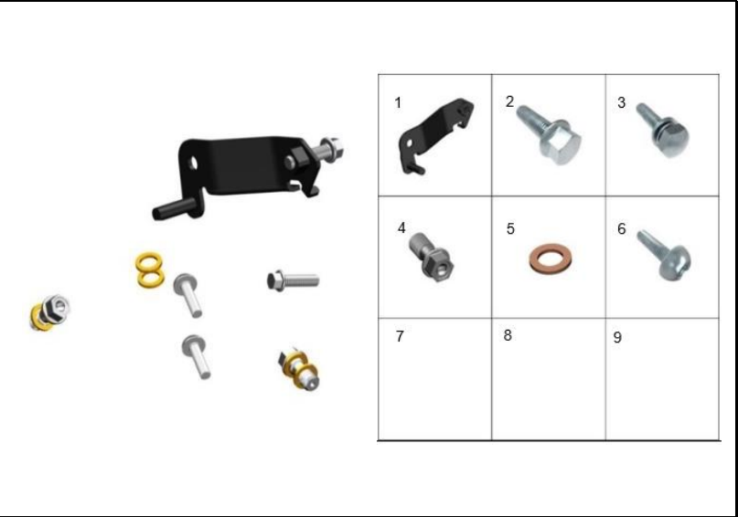
FIGURA 38: PLATINA FRENO DELANTERO
