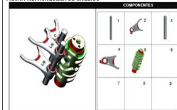
FIGURA 102: HORQUILLA DE CAMBIOS
