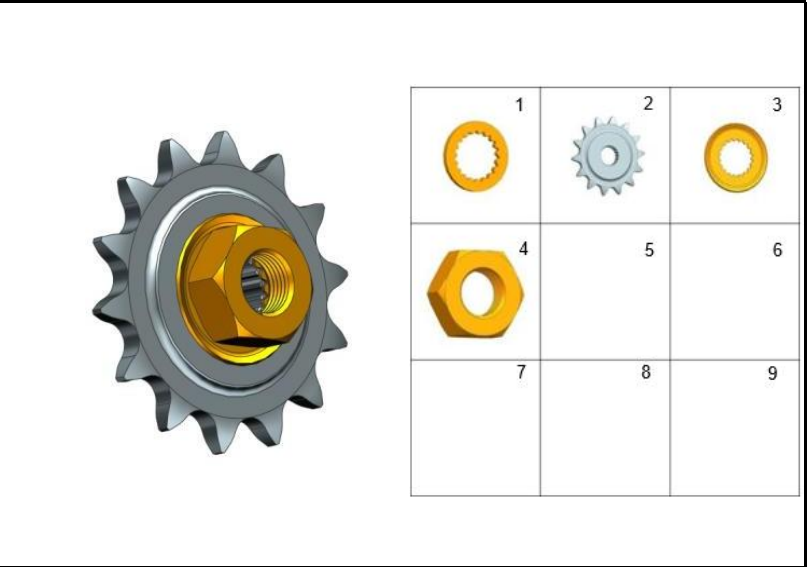
FIGURA 105: PIÑÓN DE SALIDA 2
