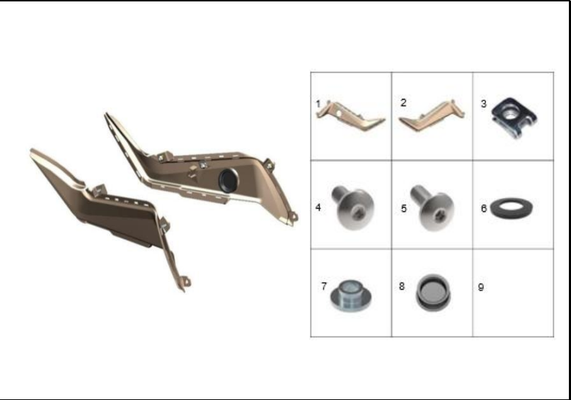
FIGURA 14: CUBIERTAS LATERALES
