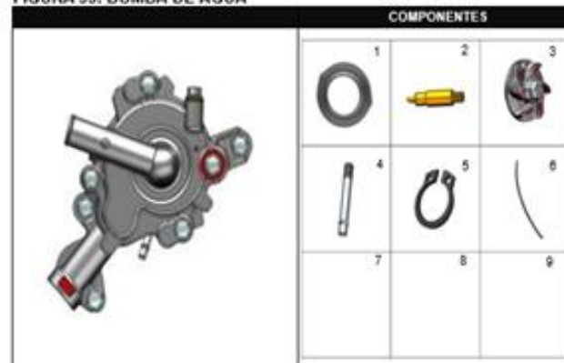
FIGURA 95: BOMBA DE AGUA
