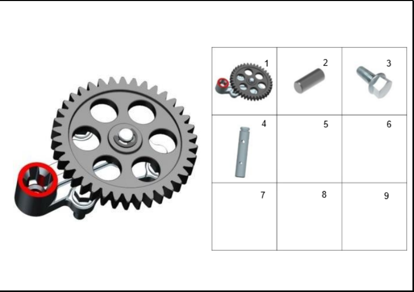
FIGURA 126: PIÑÓN DE BOMBA ACEITE
