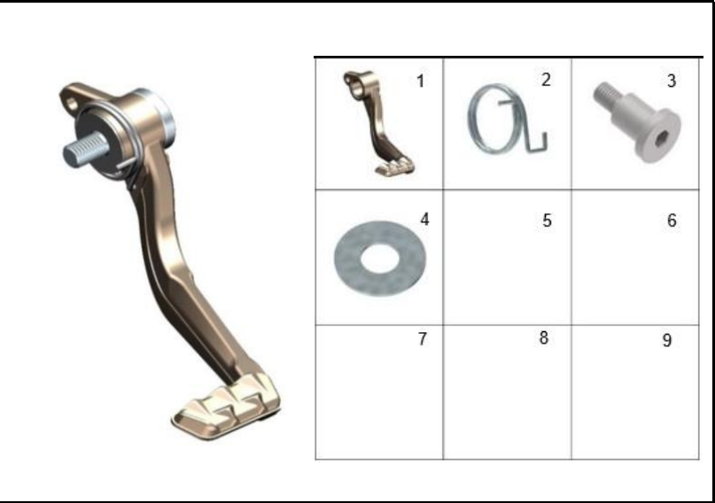
FIGURA 81: PEDAL DE FRENO
