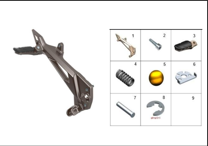
FIGURA 79: SOPORTE REPOSAPIE TRASERO DERECHO
