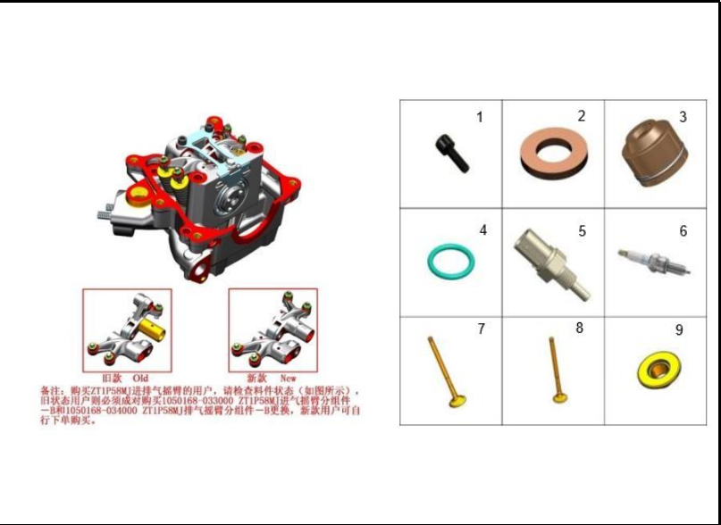
FIGURA 92: VALVULAS 2
