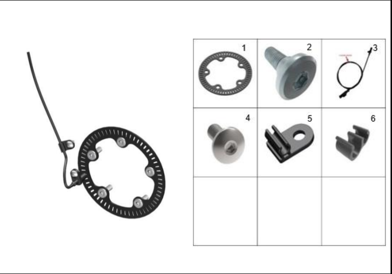
FIGURA 45: RUEDA FÓNICA RUEDA DELANTERA
