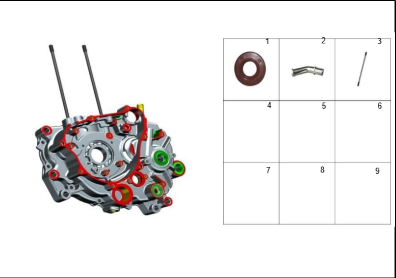
FIGURA 110: CARCASA IZQUIERDA 3
