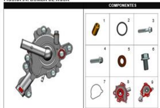
FIGURA 94: BOMBA DE AGUA
