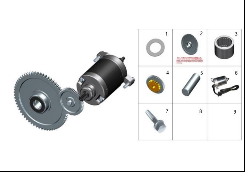
FIGURA 127: MOTOR DE ARRANQUE
