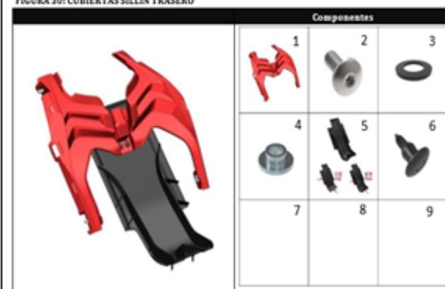
FIGURA 30: CUBIERTAS SILLÍN TRASERO
