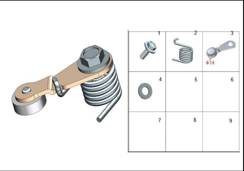
FIGURA 104: LEVA ESTRELLA SELECTORA
