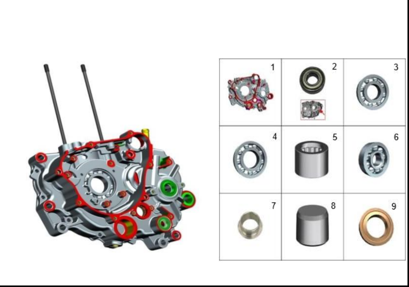
FIGURA 109: CARCASA IZQUIERDA 2
