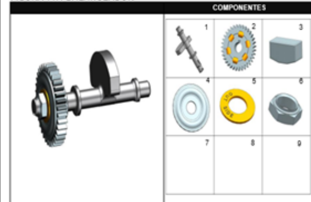
FIGURA 117: BALANCEADOR
