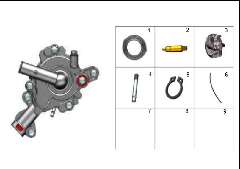
FIGURA 95: BOMBA DE AGUA 2
