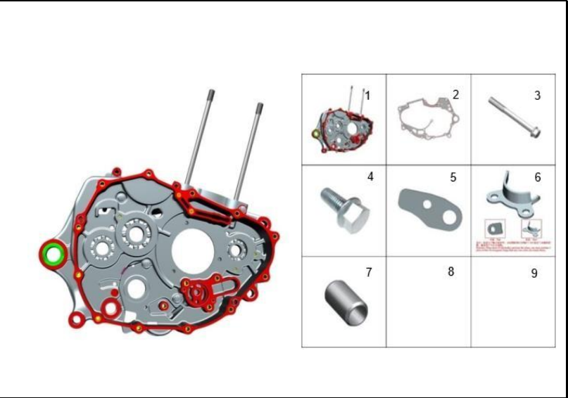
FIGURA 106: CARCASA DERECHA
