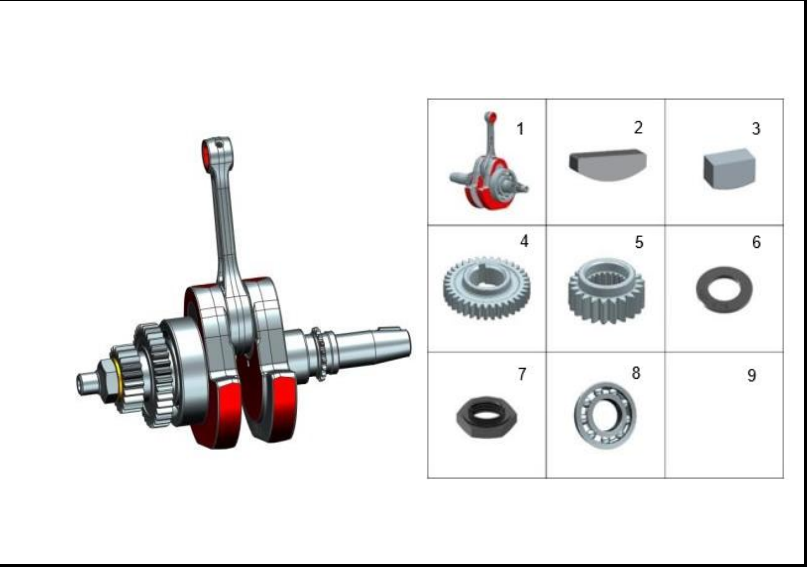
FIGURA 116: CIGUEÑAL
