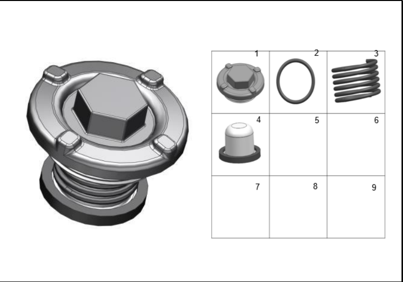
FIGURA 118: COMPLEMENTO TAPÓN ACEITE
