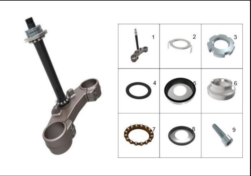
FIGURA 42: HORQUILLA DIRECCIÓN
