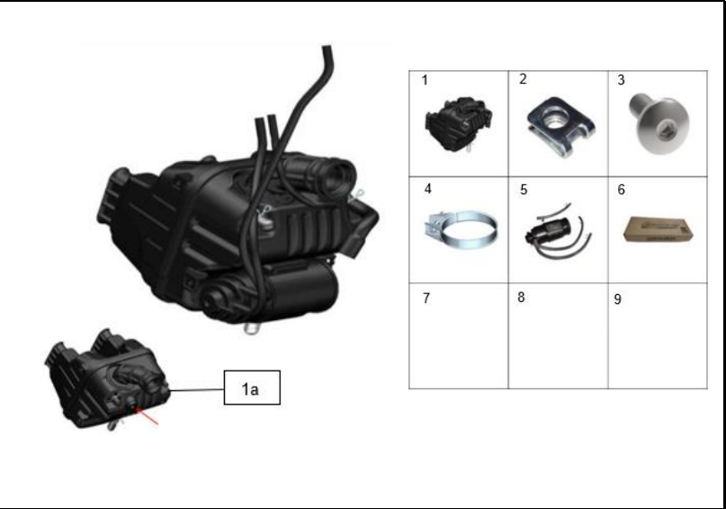
FIGURA N 68: CAJA FILTRO DE AIRE
