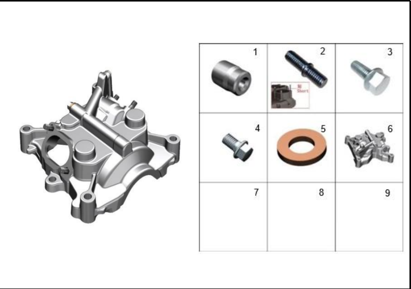
FIGURA 89: CUBIERTA CULATA 2
