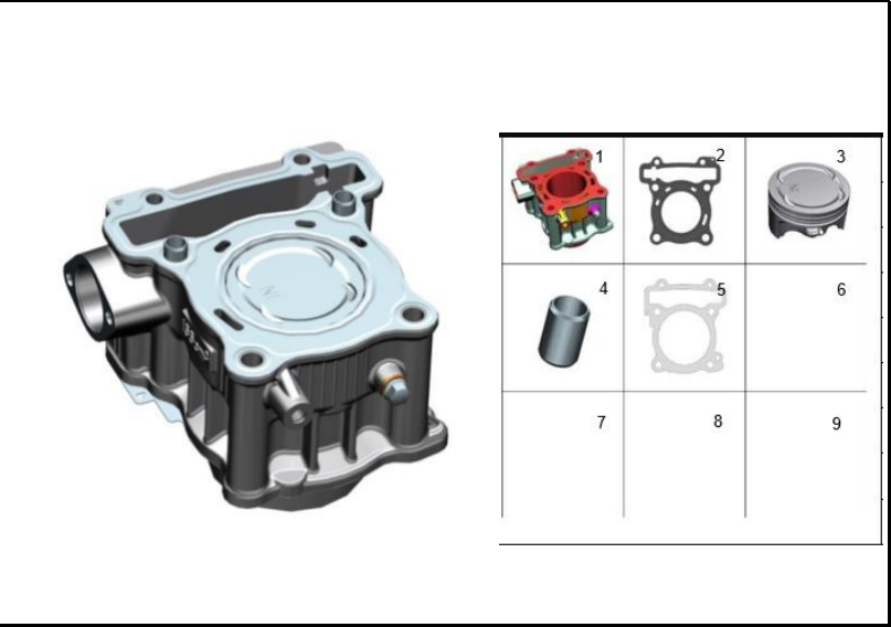
FIGURA 98: CILINDRO
