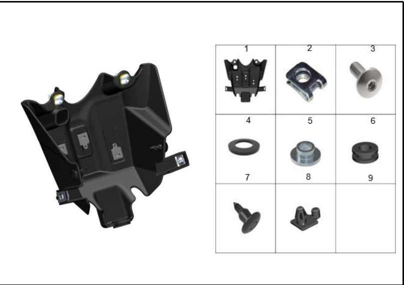
FIGURA 4: CUBIERTA TRASERA FAROLA
