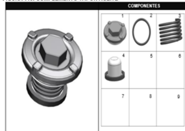
FIGURA 118: COMPLEMENTO TAPÓN ACEITE
