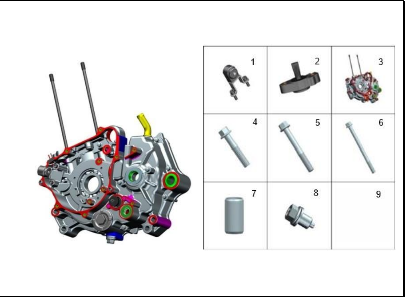
FIGURA 108: CARCASA IZQUIERDA
