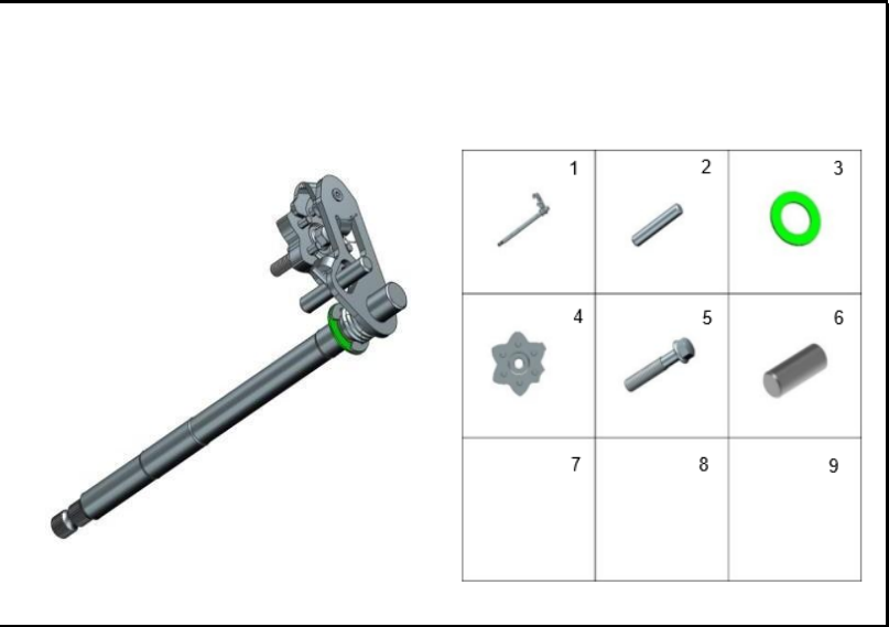
FIGURA 103: EJE DE CAMBIOS
