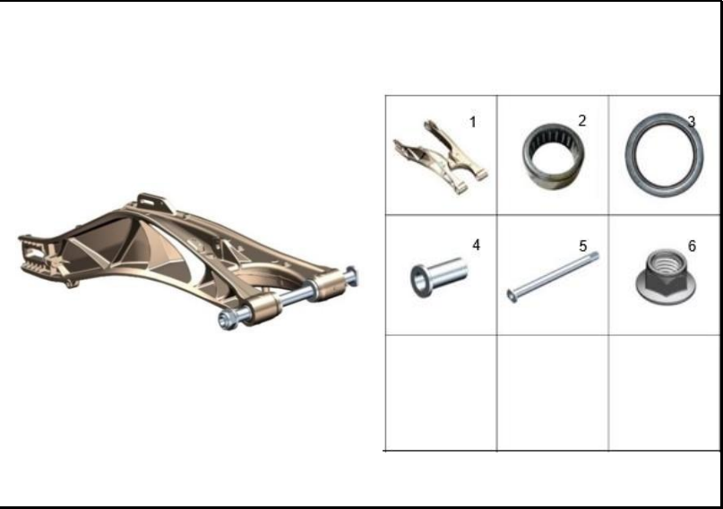
FIGURA 46: BRAZO OSCILANTE
