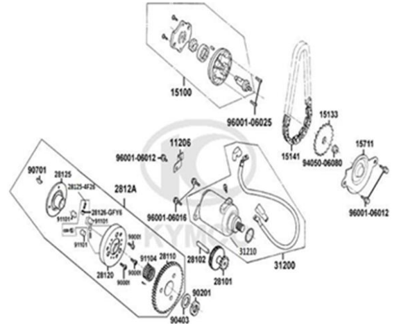
FIG. Nº 6 MOTOR DE ARRANQUE - BOMBA DE ACEITE
