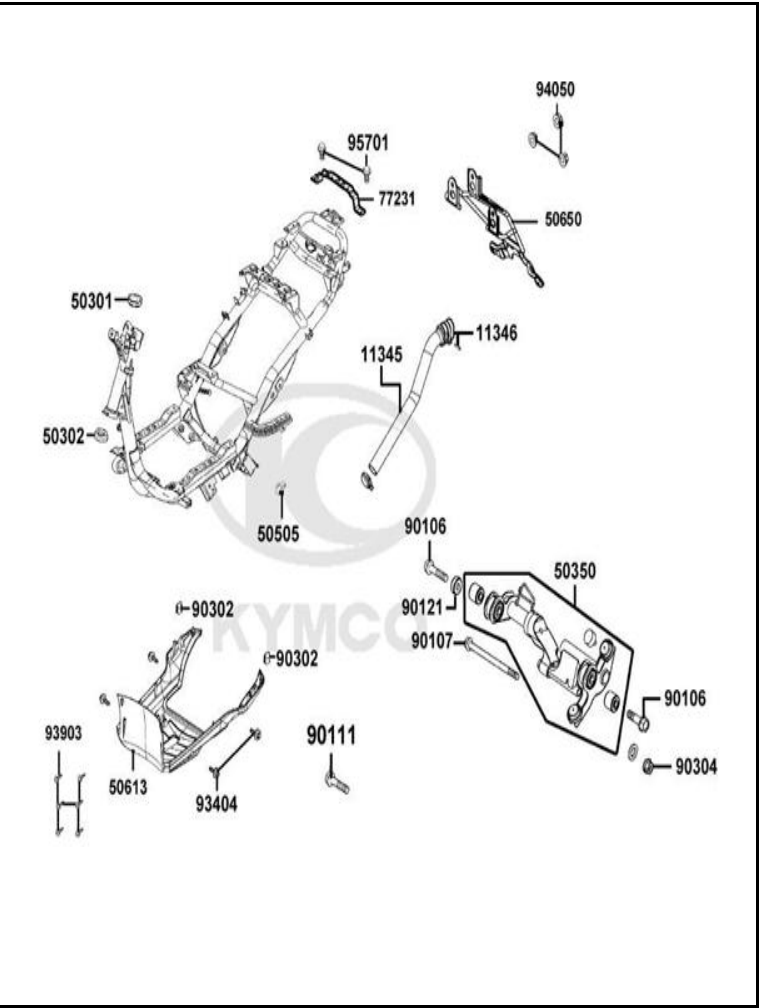
FIGURA N° 29: CHASIS
