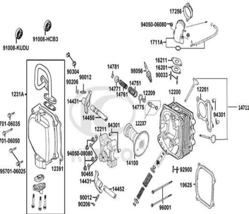
FIG. N° 2 CULATA
