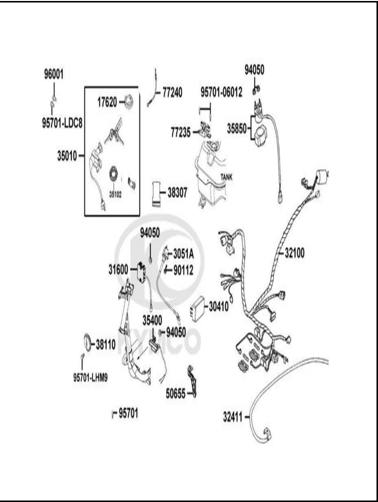
FIGURA N° 28: SISTEMA ELECTRICO
