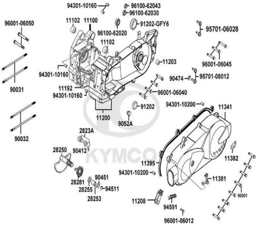
FIG. N° 1 CARCASAS
