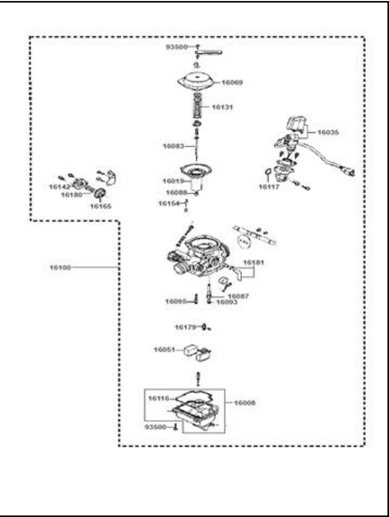
FIGURA N° 9: CARBURADOR
