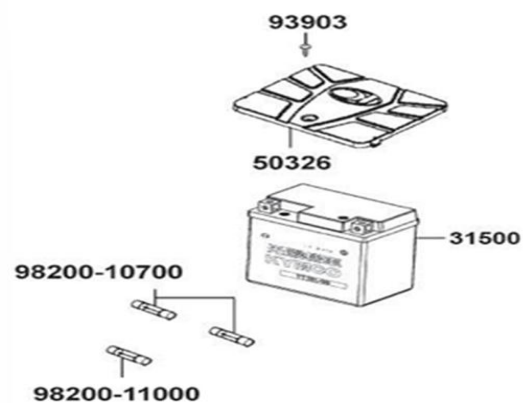
FIG. N° 20 BATERIA
