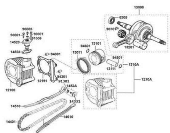
FIG. N° 3 CILINDRO - PISTÓN - CIGÜEÑAL
