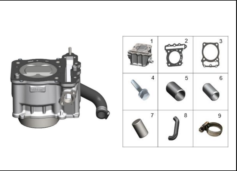
FIGURA 97: KIT CILINDRO
