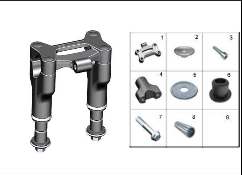
FIGURA 39: SOPORTE MANUBRIO
