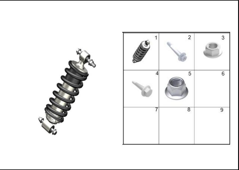
FIGURA 52: AMORTIGUADOR TRASERO
