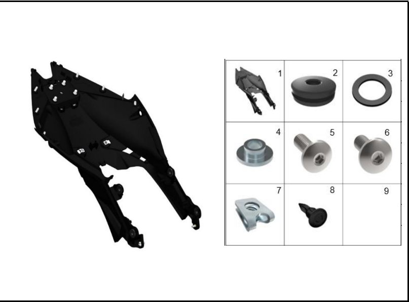
FIGURA 25: CUBIERTA INFERIOR SILLÍN
