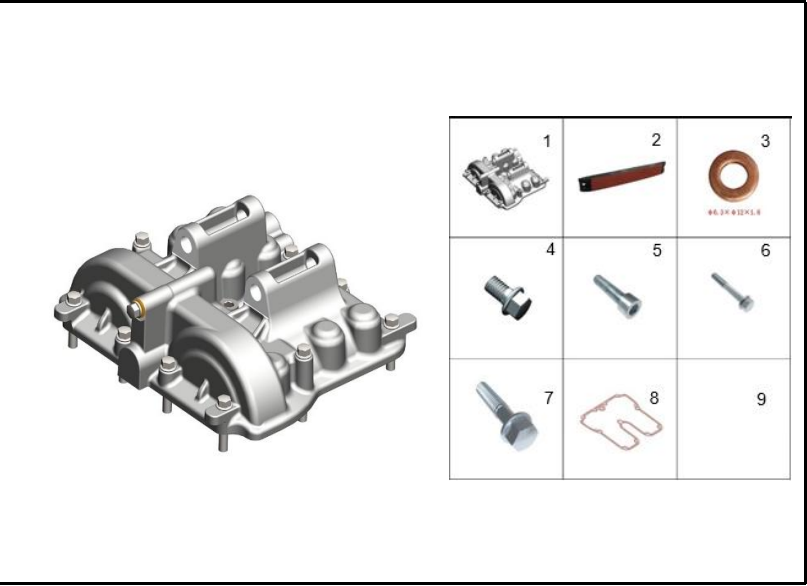
FIGURA 96: TAPA CULATA
