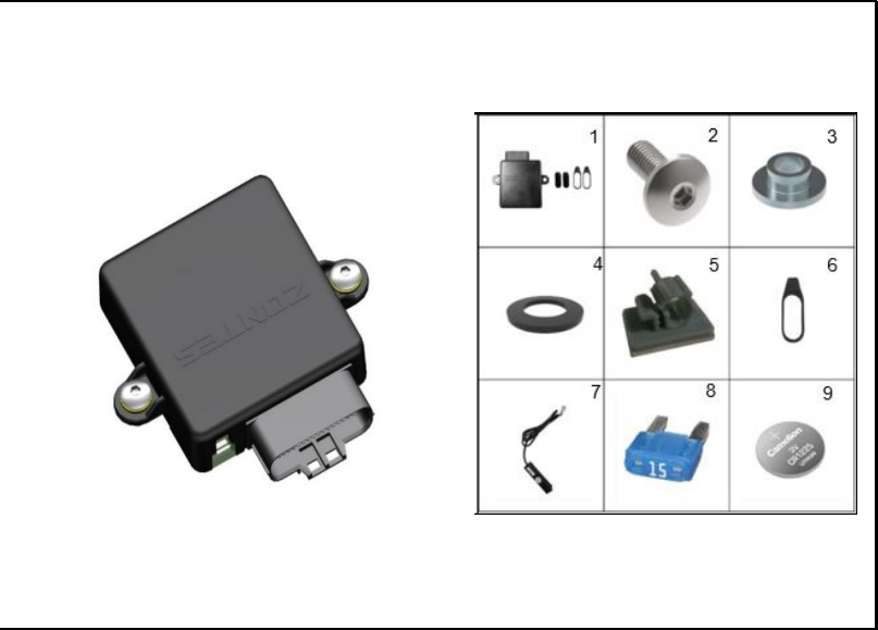
FIGURA 64: CONTROLADOR ENCENDIDO Y CONTROLES
