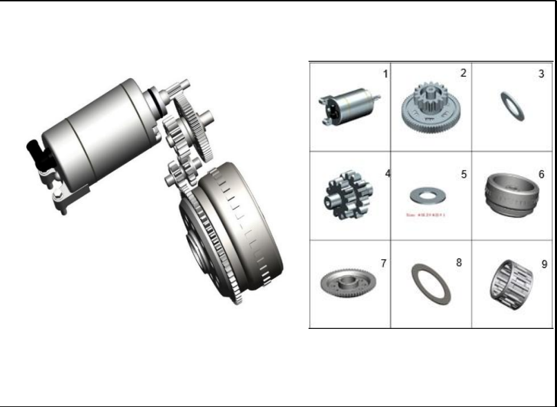
FIGURA 120: MOTOR DE ARRANQUE
