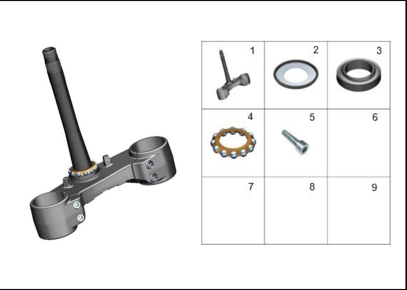
FIGURA 45: HORQUILLA DIRECCIÓN
