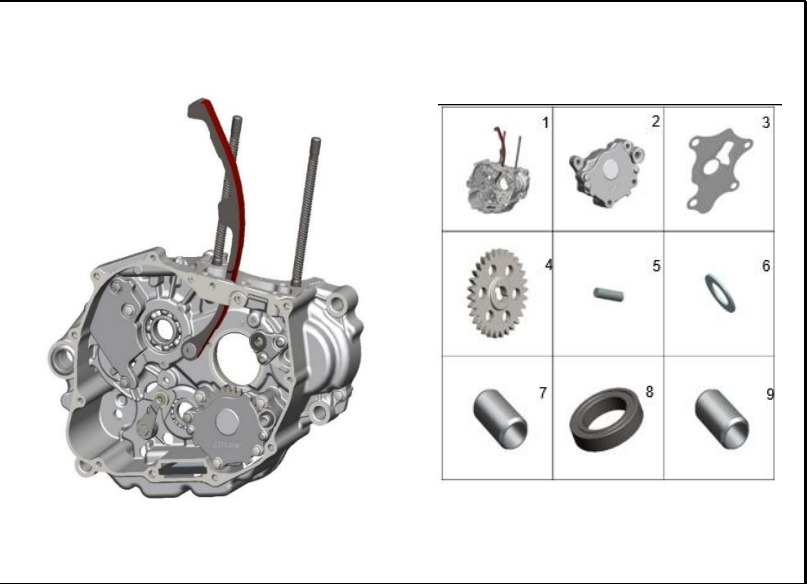
FIGURA 111: CARCASA DERECHA
