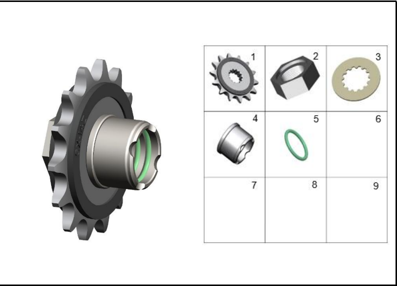
FIGURA 105: PIÑÓN DE SALIDA
