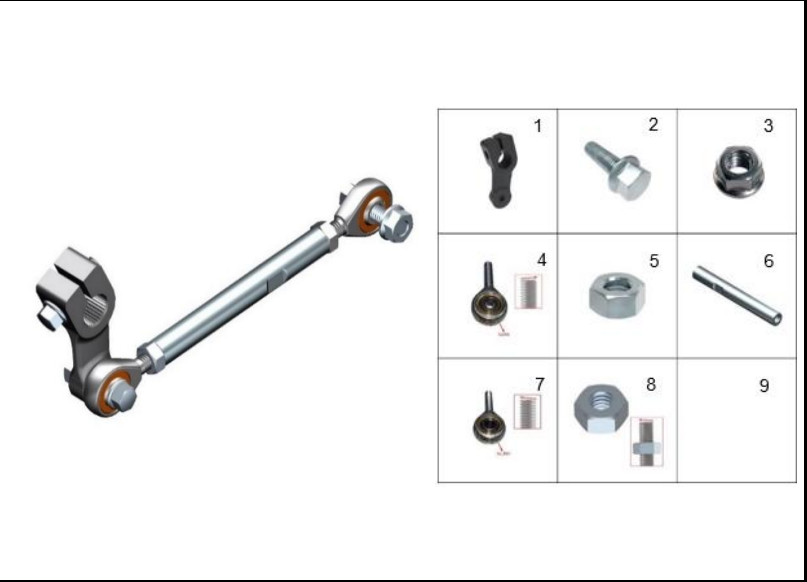
FIGURA 78: MUÑON PEDAL DE CAMBIOS
