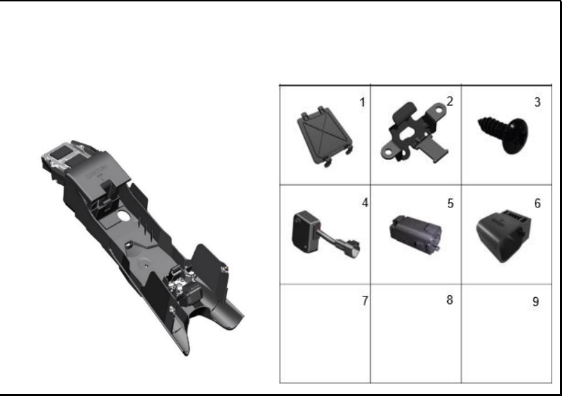
FIGURA N°19: CAJA DISPOSITIVOS ELECTRICOS 2
