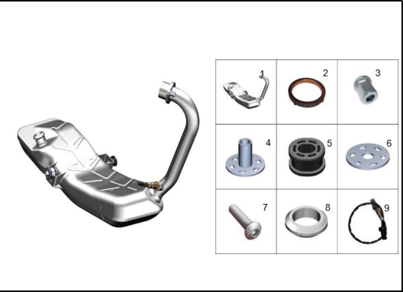
FIGURA 73: SILENCIADOR
