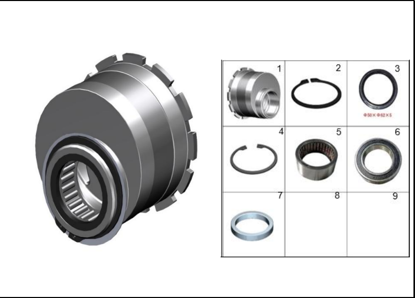
FIGURA 56: SOPORTE DENTADO BRAZO OSCILANTE
