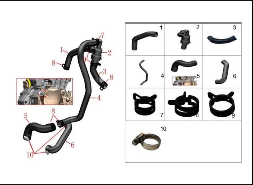
FIGURA 89: TERMOSTATO Y MANGUERAS
