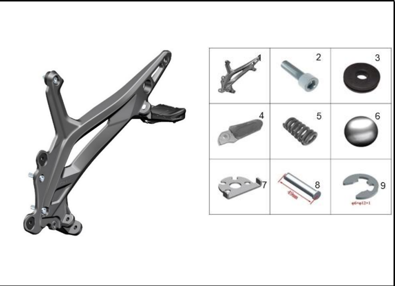
FIGURA 75: SOPORTE REPOSAPIES IZQUIERDO
