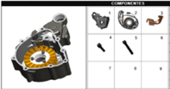
FIGURA N° 115: CUBIERTA CARCASA MOTOR IZQUIERDA
