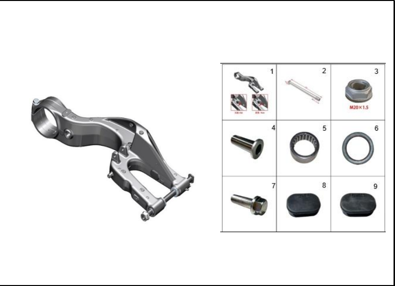
FIGURA 49: BRAZO OSCILANTE
