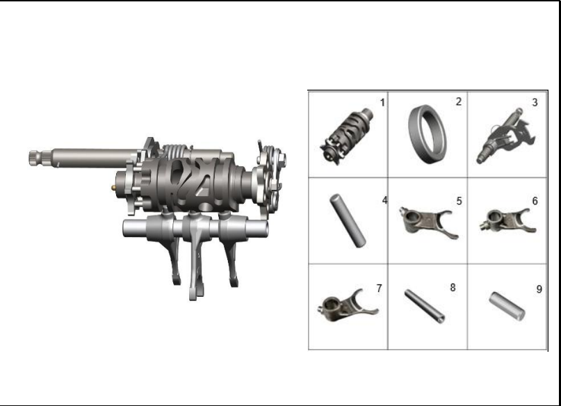
FIGURA 106: EJE DE CAMBIOS
