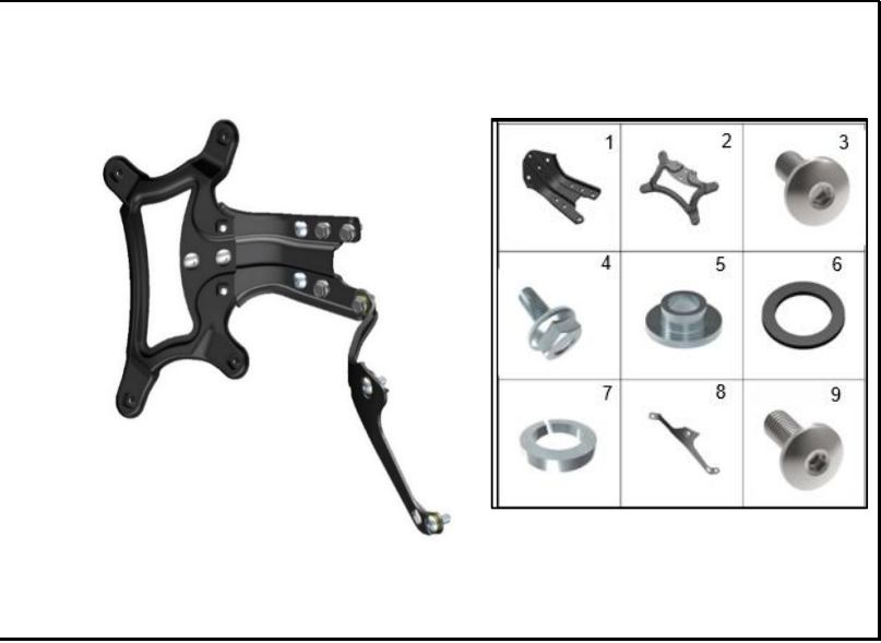
FIGURA 29: SOPORTE GUARDABARRO TRASERO 2
