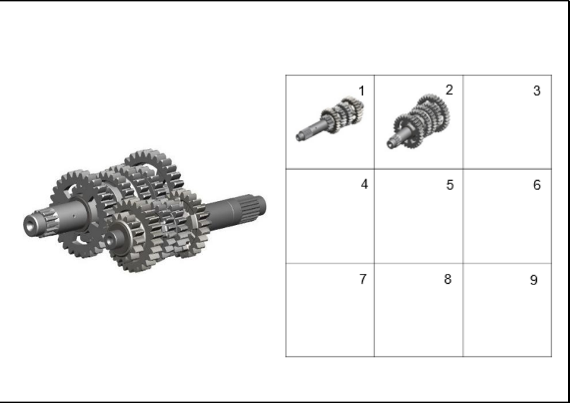
FIGURA 104: TRANSMISIÓN
