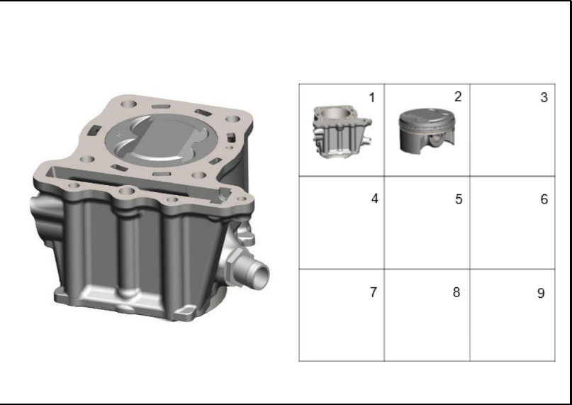
FIGURA 98: CILINDRO COMPLETO
