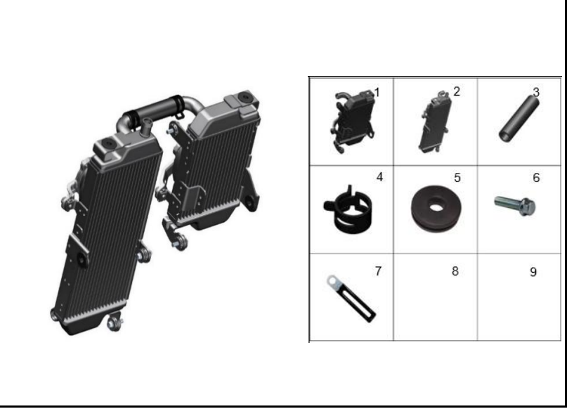
FIGURA 86: RADIADOR
