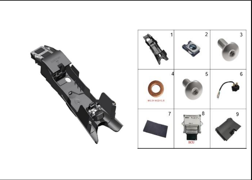
FIGURA N°19: CAJA DISPOSITIVOS ELECTRICOS
