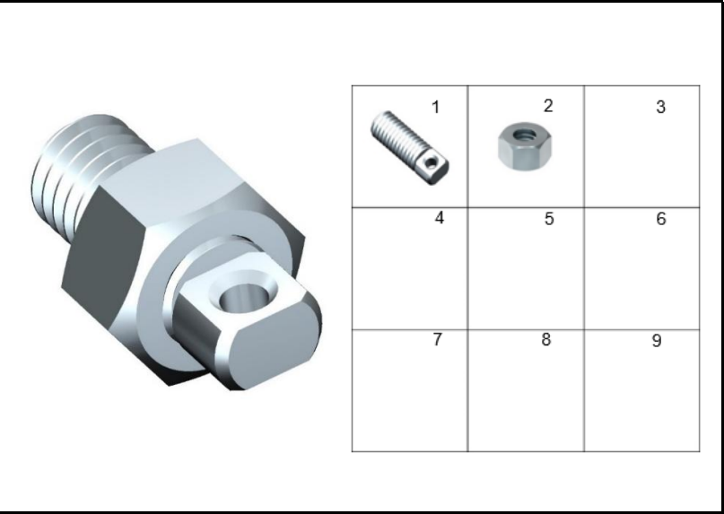
FIGURA 81: TORNILLO PEDAL FRENO
