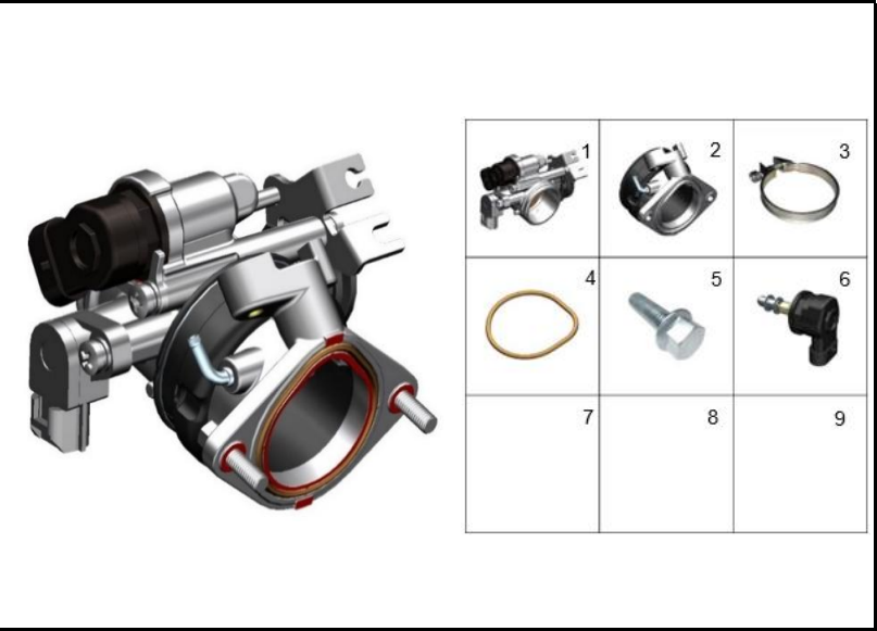
FIGURA 69: CUERPO DE INYECCIÓN
