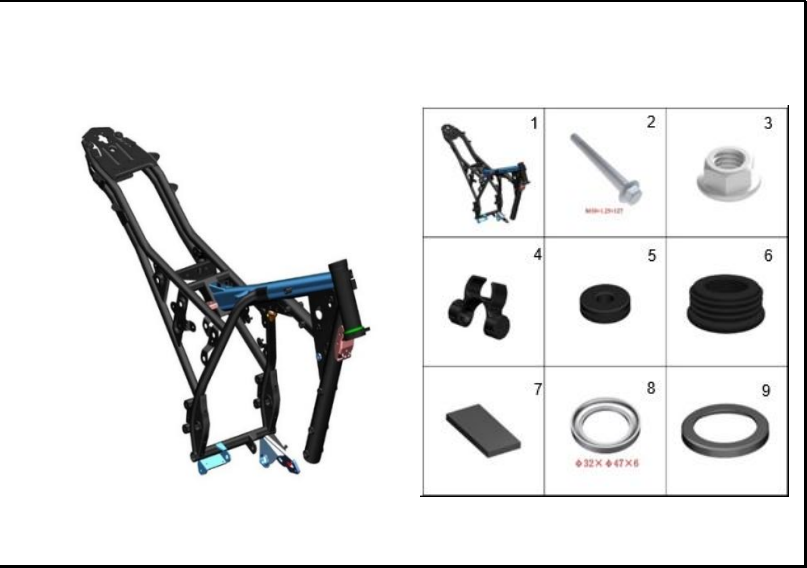
FIGURA 60: PARTES CHASIS
