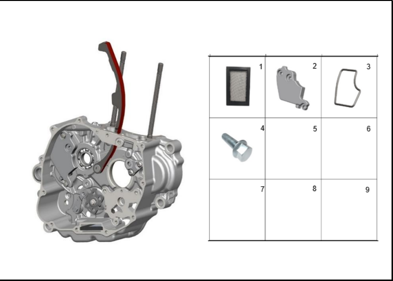
FIGURA 112: CARCASA DERECHA 4
