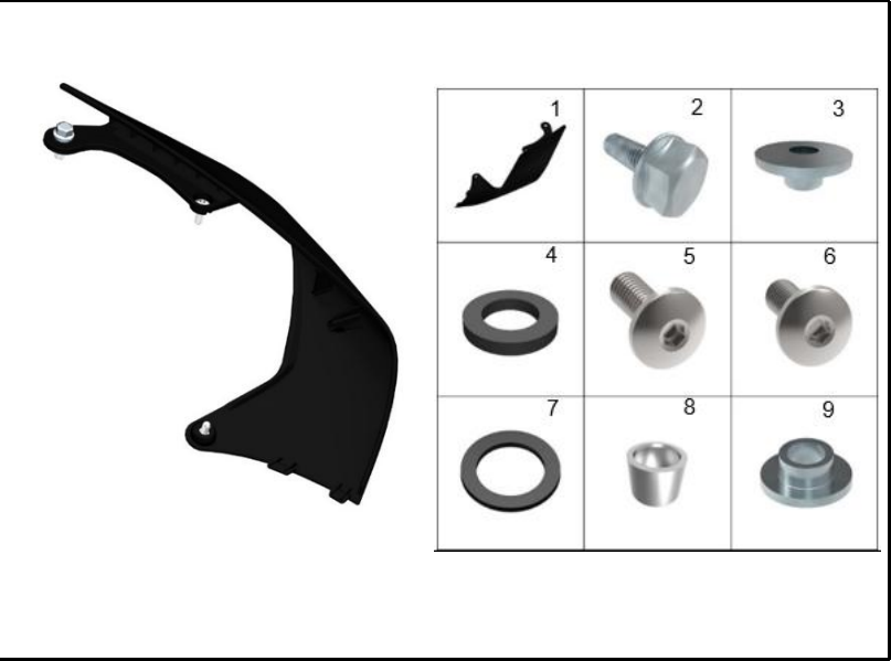
FIGURA 22: CUBIERTA IZQUIERDA SILLÍN
