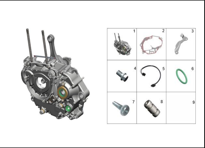
FIGURA 107: CARCASA IZQUIERDA
