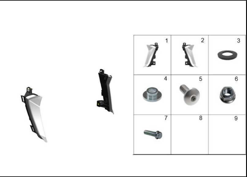
FIGURA 17: DIRECCIONALES DELANTERAS
