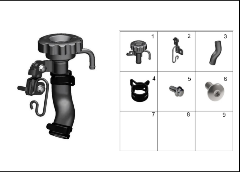
FIGURA 87: TAPA RADIADOR
