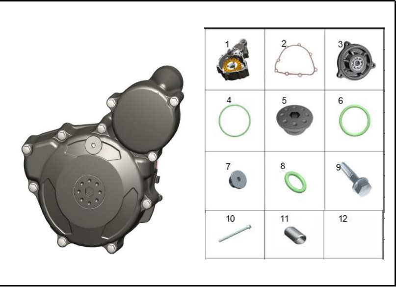
FIGURA 114: TAPA CÁRTER IZQ
