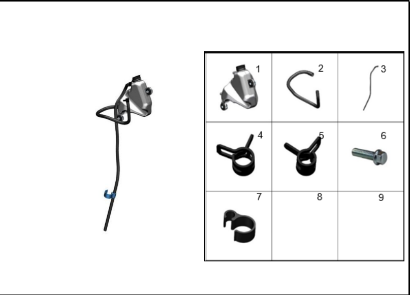
FIGURA 88: TANQUE RESERVORIO
