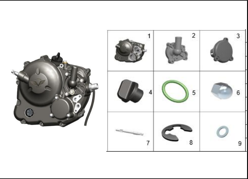
FIGURA 118: TAPA CARTER DERECHA 3
