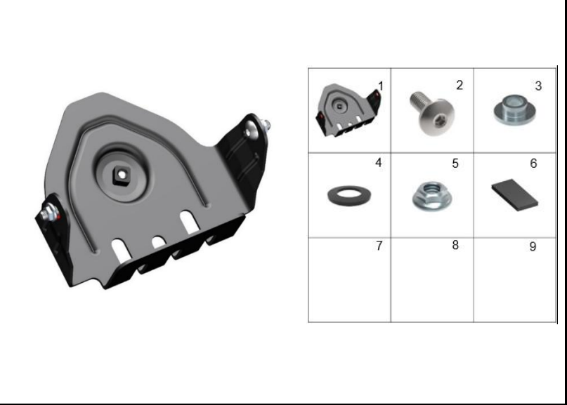
FIGURA 21: SOPORTE BATERÍA
