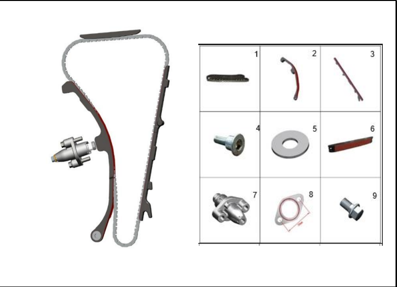
FIGURA 121: CADENILLA DE DISTRIBUCIÓN
