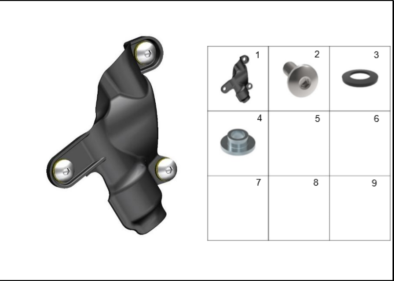
FIGURA 83: CUBIERTA BOMBA DE FRENO TRASERO
