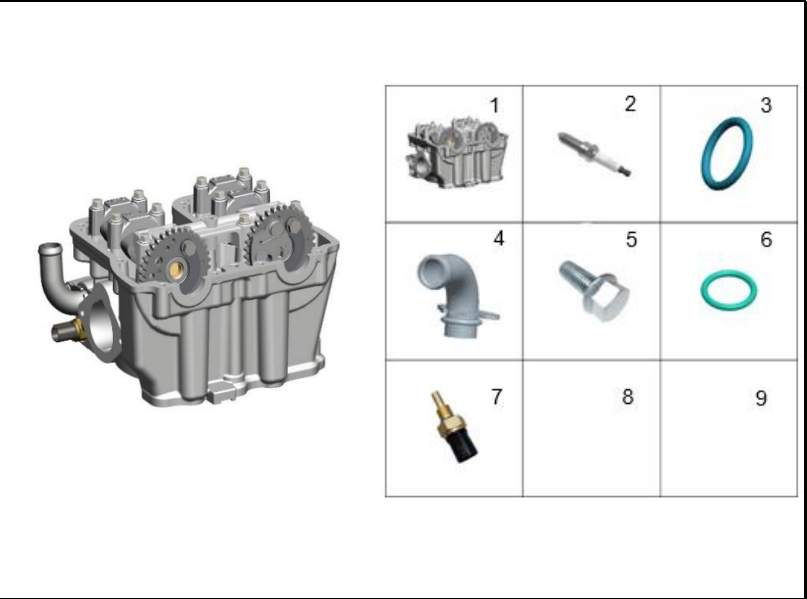
FIGURA 93: CULATA 2
