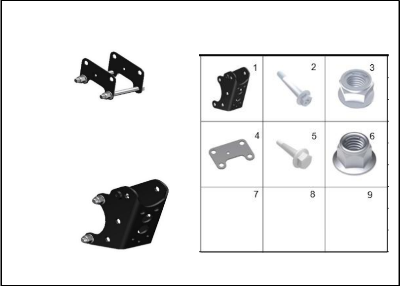
FIGURA 66: SOPORTE MOTOR
