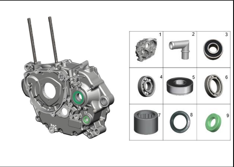
FIGURA 109: CARCASA IZQUIERDA 4
