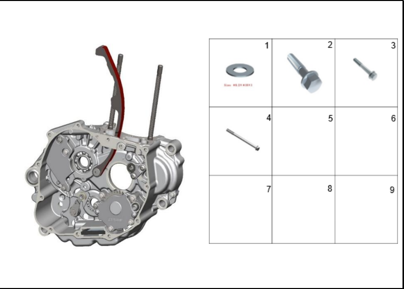
FIGURA 111: CARCASA DERECHA 2
