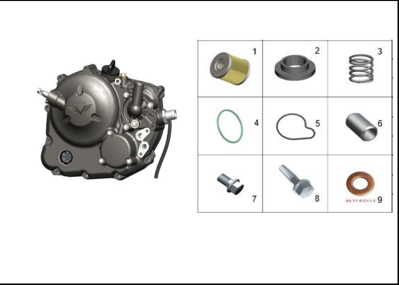
FIGURA 118: TAPA CARTER DERECHA 4
