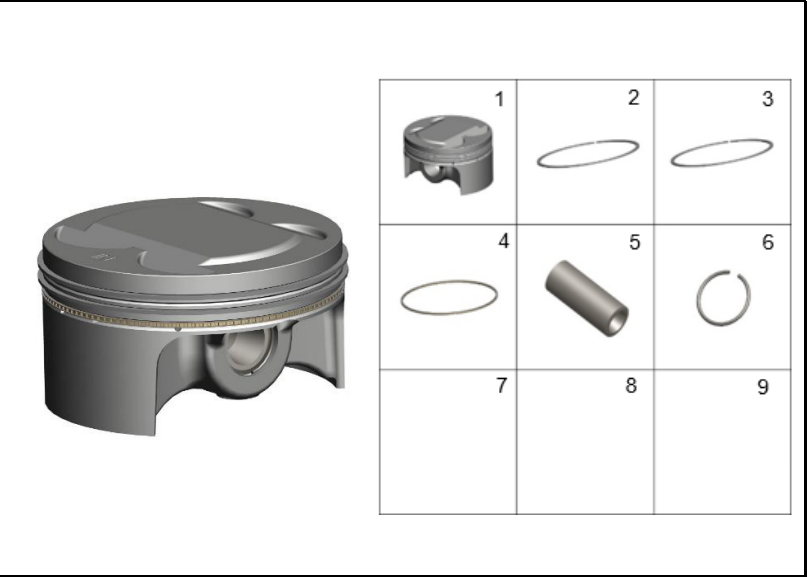
FIGURA 100: PISTON
