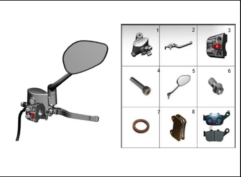
FIGURA 40: LEVA DE FRENO
