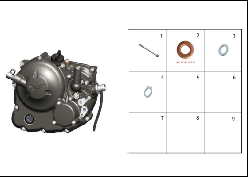
FIGURA 117: TAPA CARTER DERECHA 2
