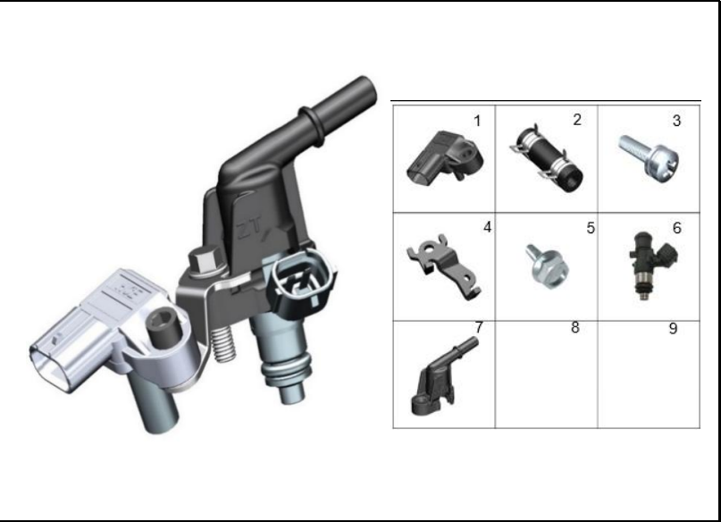
FIGURA 70: SOPORTE INYECTOR
