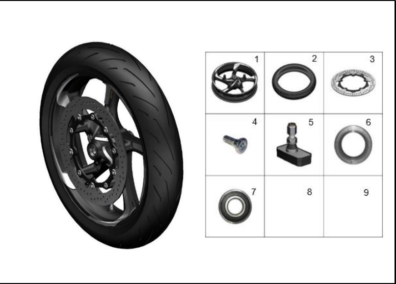
FIGURA 47: RUEDA DELANTERA
