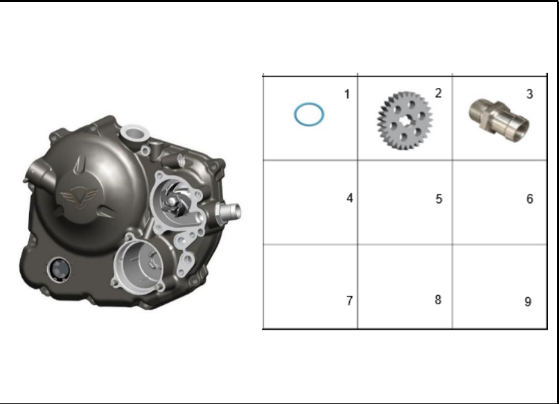
FIGURA 119: CUBIERTA CARCASA MOTOR DERECHA 3
