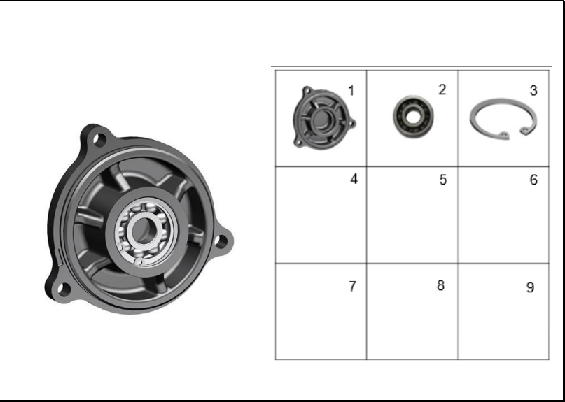
FIGURA 116: TAPA PIÑÓN REDUCTOR ARRANQUE
