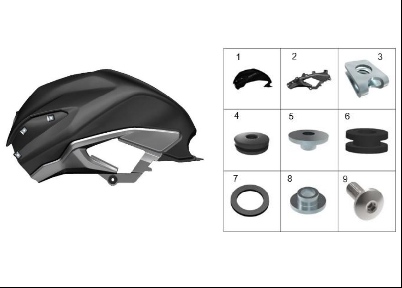
FIGURA 12: CUBIERTA TANQUE IZQUIERDO
