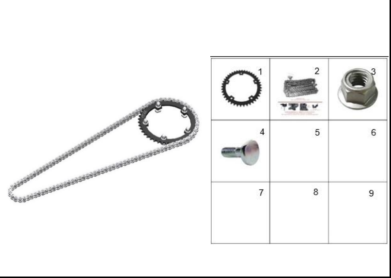
FIGURA 55: CADENA
