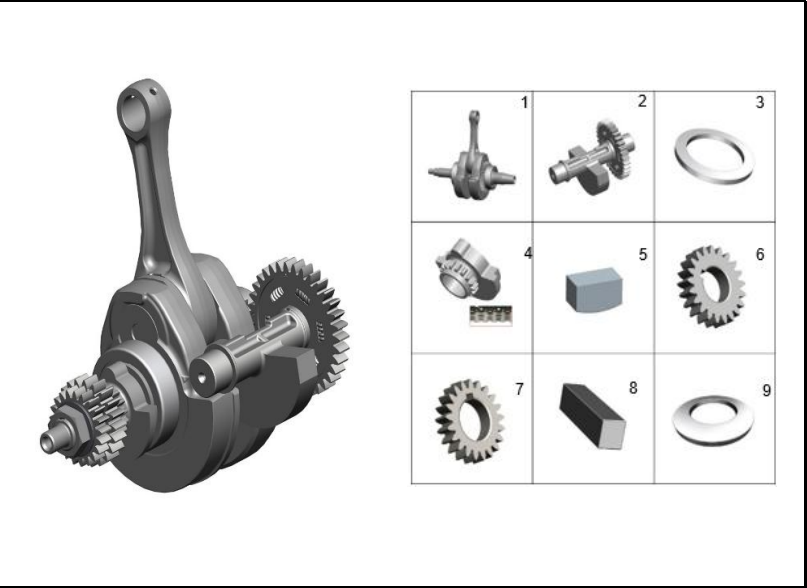
FIGURA 110: CIGÜEÑAL
