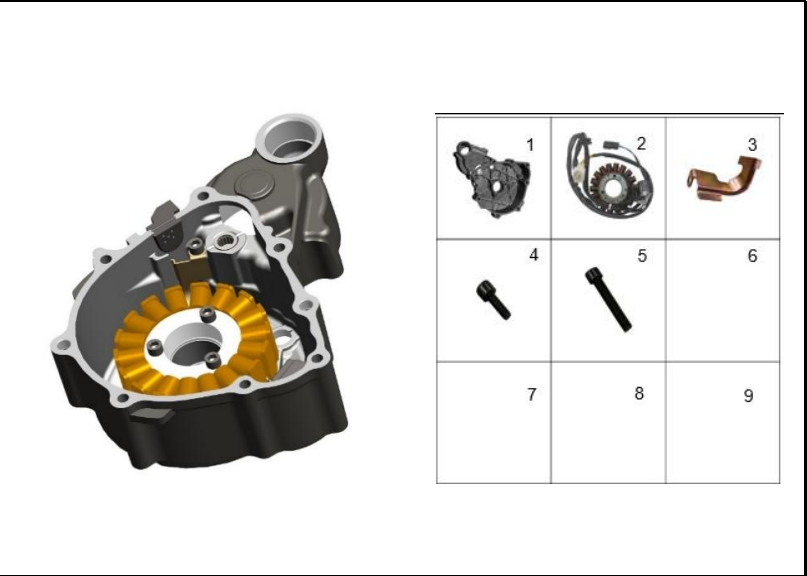
FIGURA 115: CUBIERTA CARCASA MOTOR IZQUIERDA
