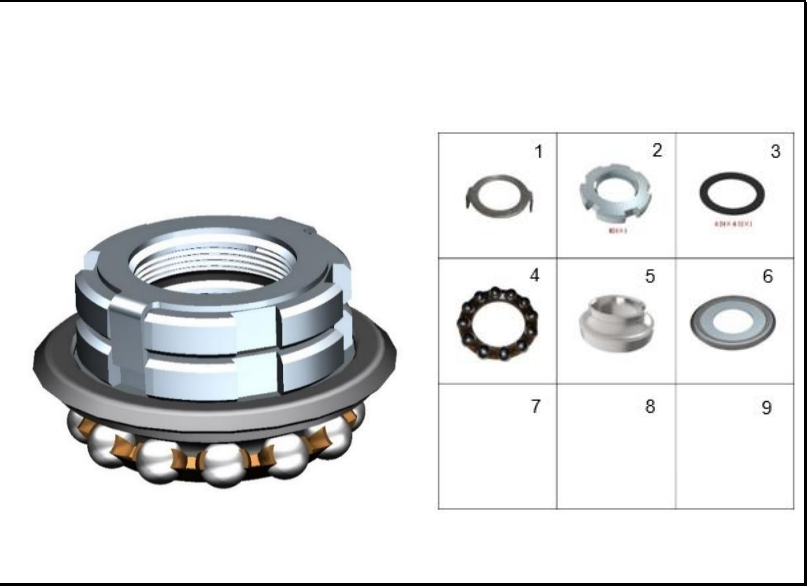
FIGURA 44: CUNAS DIRECCIÓN
