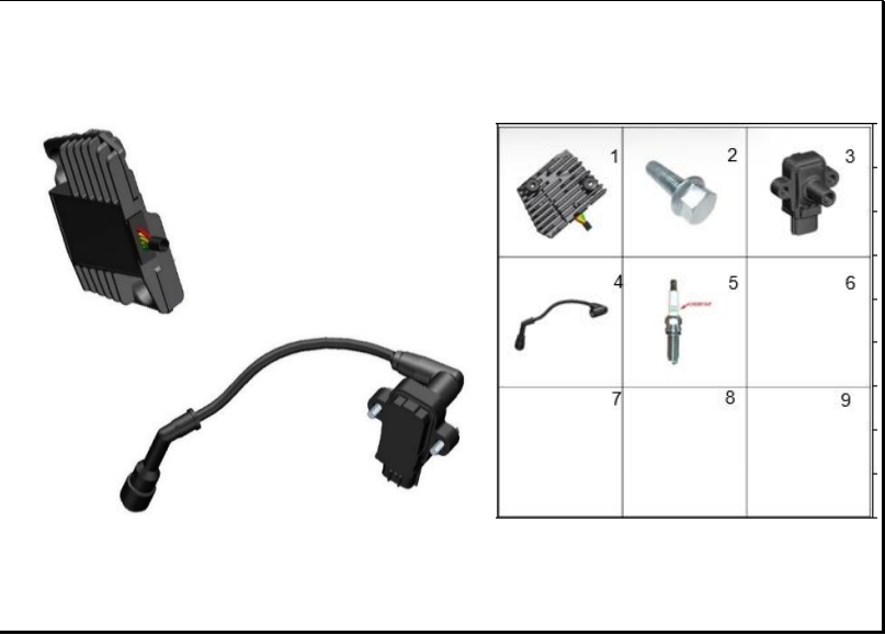
FIGURA 63: REGULADOR
