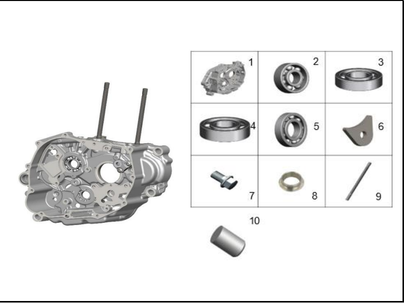
FIGURA 113: CARCASA DERECHA 5
