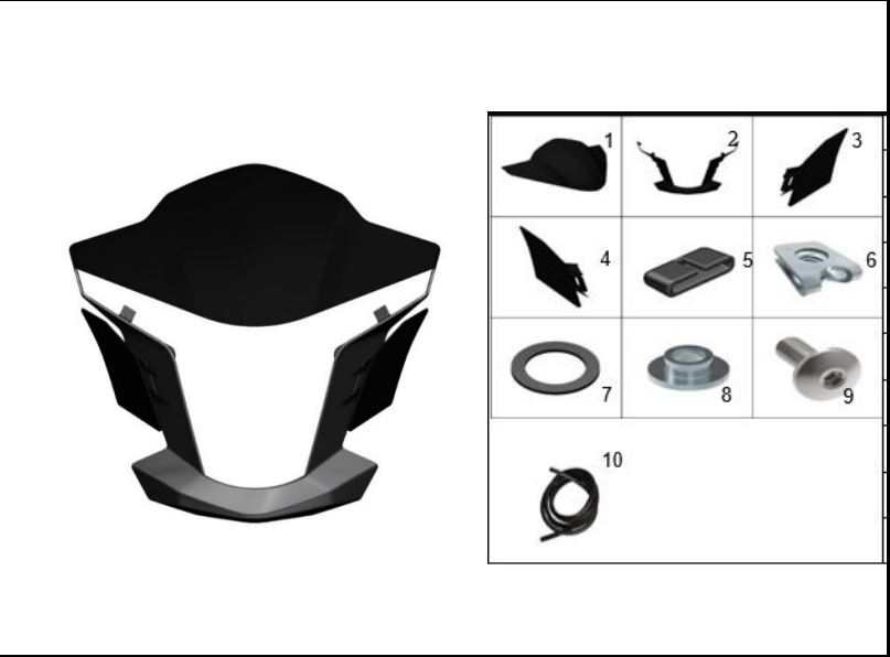
FIGURA 3: CUBIERTA FAROLA
