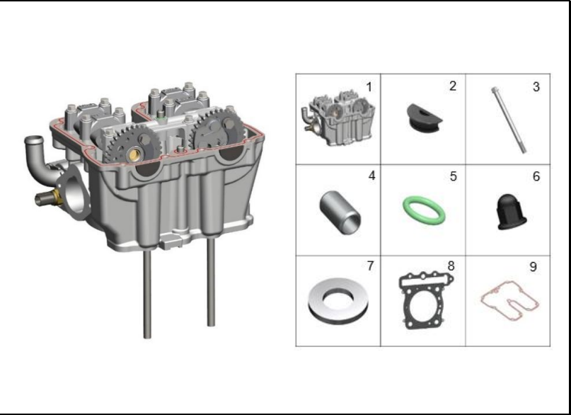
FIGURA 92: CULATA
