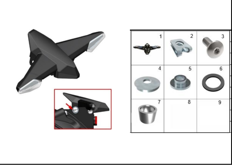
FIGURA 31: SOPORTE DIRECCIONALES COMPLETO
