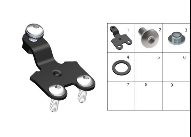
FIGURA 27: SOPORTE STOP TRASERO
