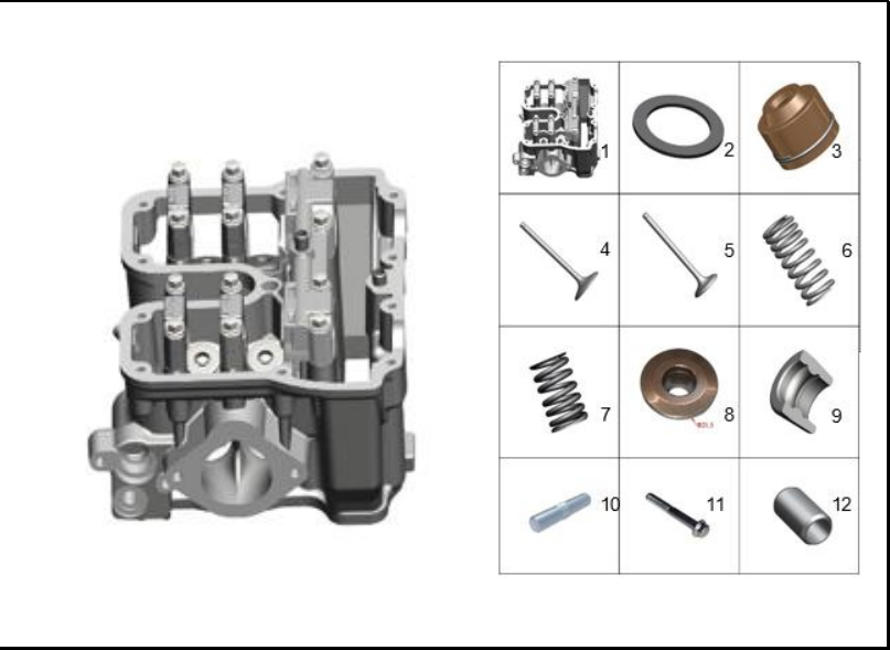
FIGURA 95: CULATA 4
