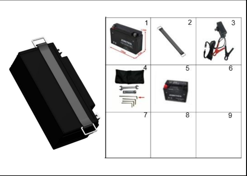
FIGURA 20: BATERÍA
