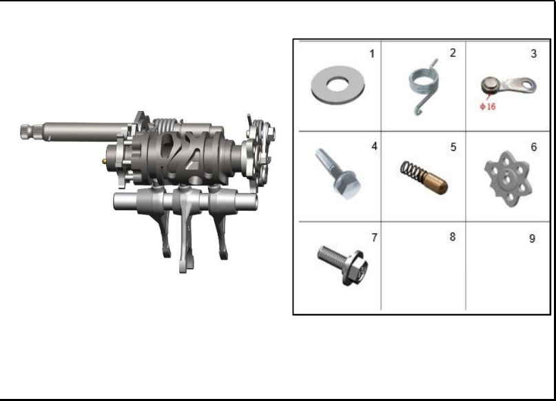
FIGURA 106: EJE DE CAMBIOS 2
