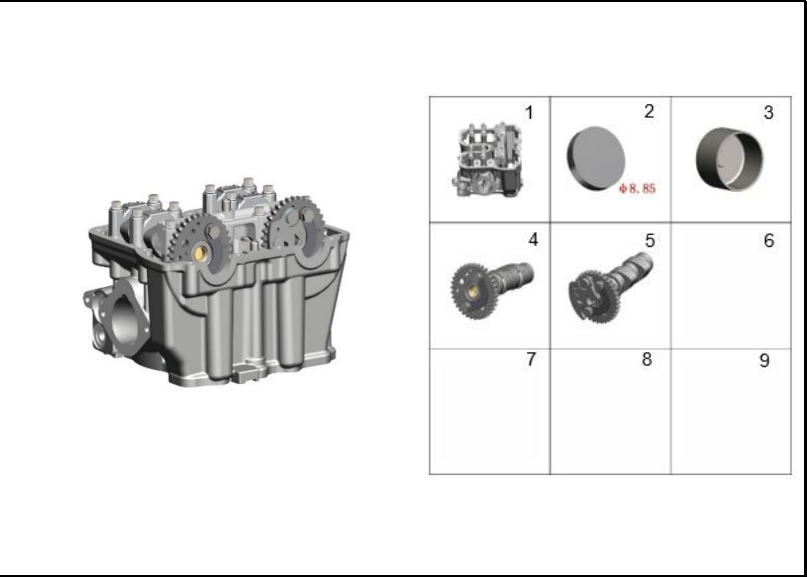
FIGURA 94: CULATA 3
