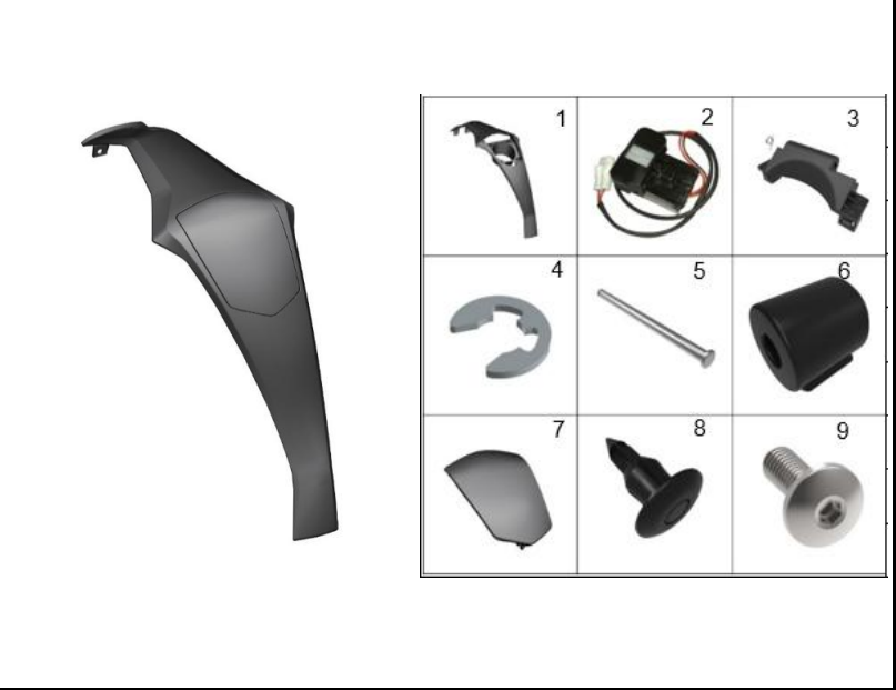
FIGURA 14: CUBIERTA CENTRAL TANQUE
