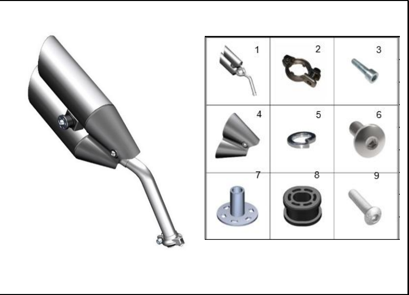
FIGURA 74: PARTE TRASERA SILENCIADOR
