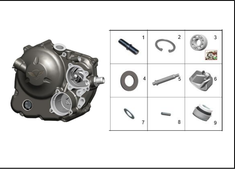
FIGURA 119: CUBIERTA CARCASA MOTOR DERECHA 2
