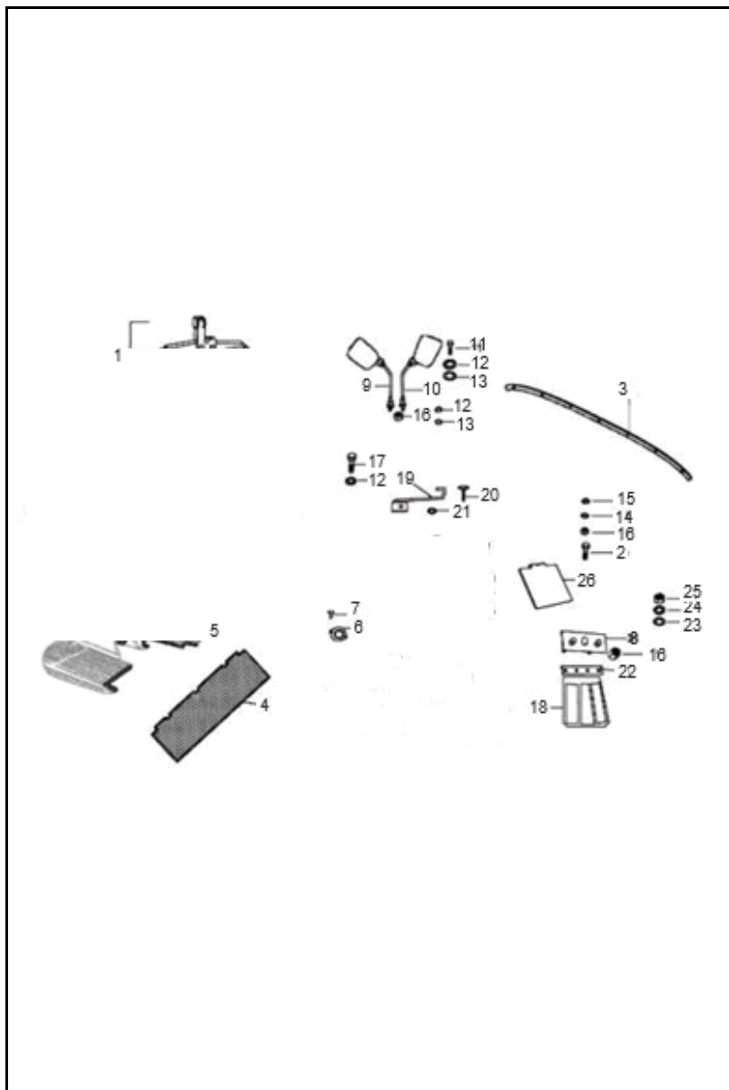
FIGURA N° 33: ESPEJOS - COMPLEMENTOS CARROCERIA (2/2)
