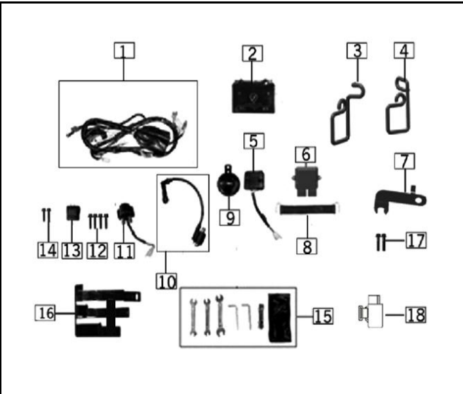
FIG. Nº 32 PARTES ELÉCTRICAS
