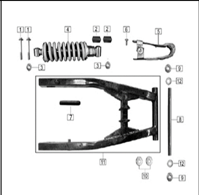
FIG. Nº 36 BRAZO OSCILANTE-MONOSHOCK
