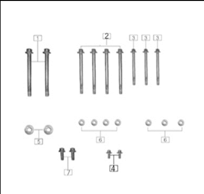
FIG. Nº 35 SOPORTE MOTOR
