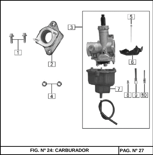
FIG. N° 24: CARBURADOR
