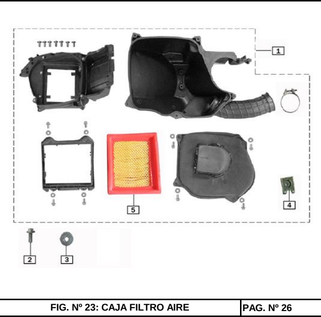
FIG. N° 23: CAJA FILTRO AIRE
