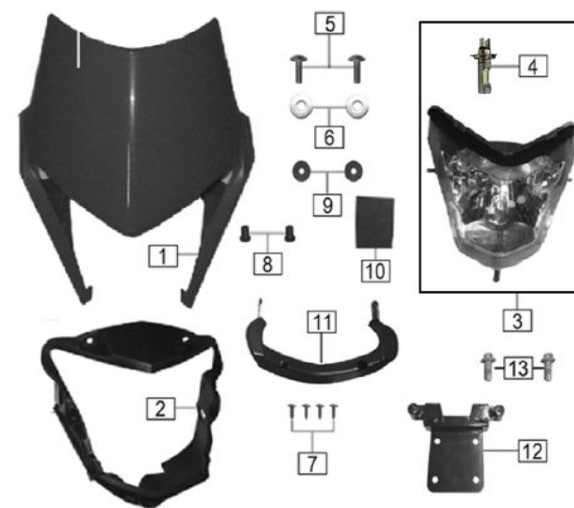
FIG. N° 12: FAROLA - CARENAJE FAROLA
