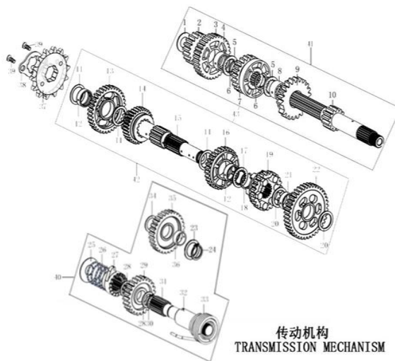
FIG. N° 8: TRANSMISION
