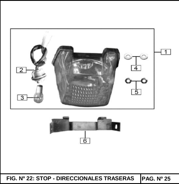
FIG. N° 22: STOP - DIRECCIONALES TRASERAS
