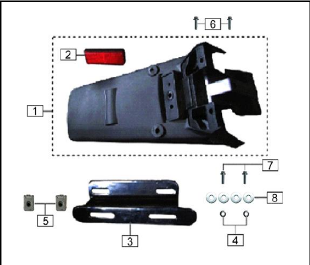
FIG. N° 21: GUARDABARRO TRASERO
