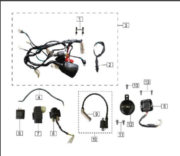
FIG. N° 19: SISTEMA ELECTRICO
