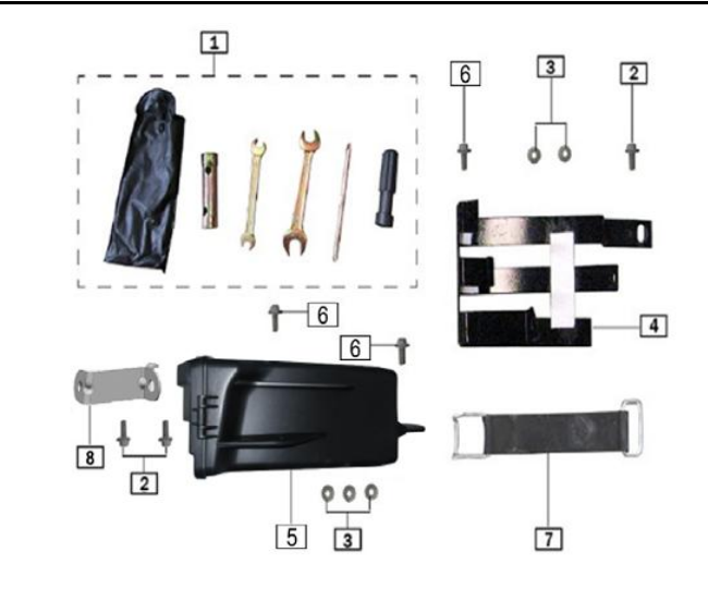
FIG. N° 20: CAJA HERRAMIENTAS
