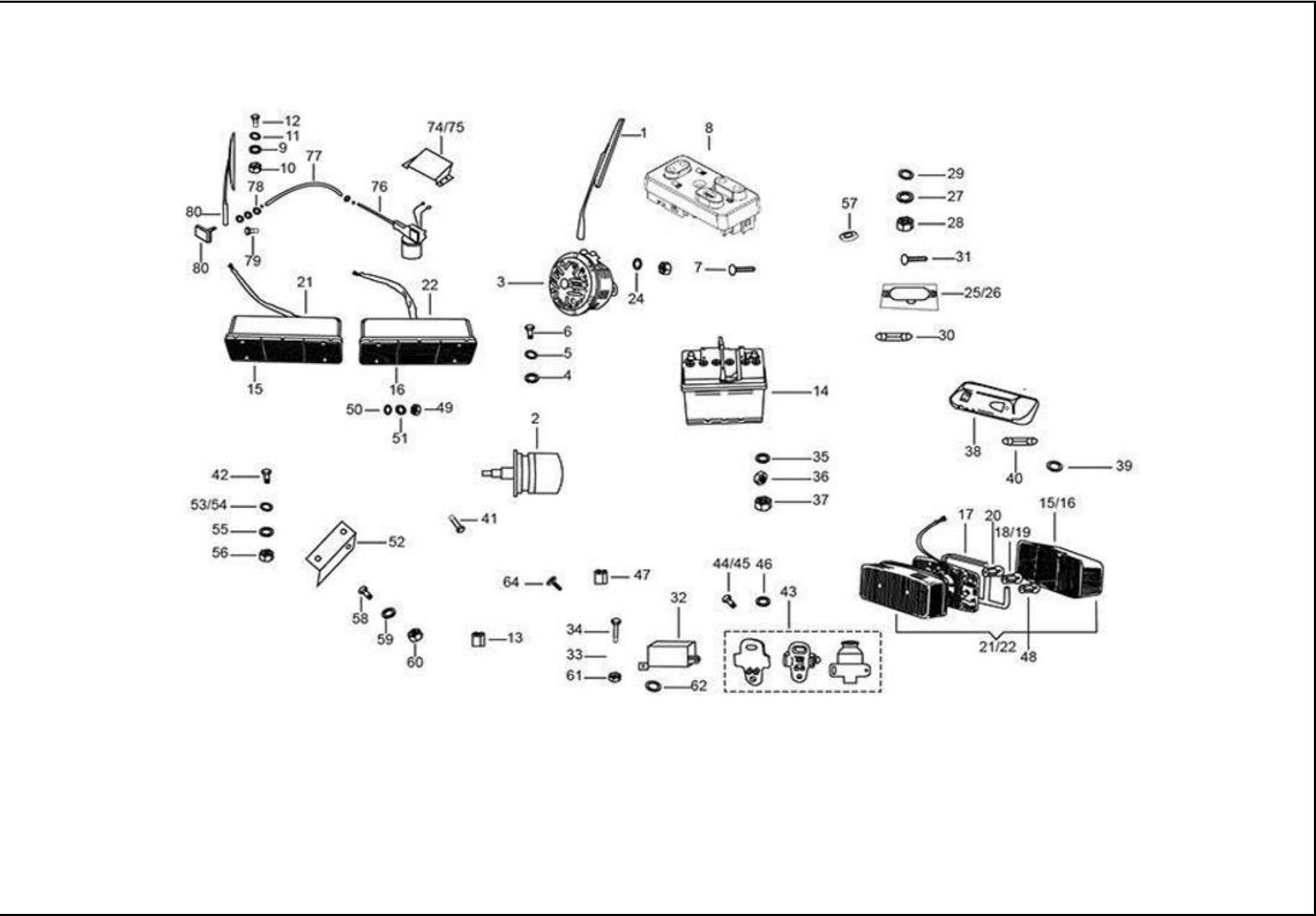
FIGURA N° 29 COMPONENTES ELÉCTRICOS
