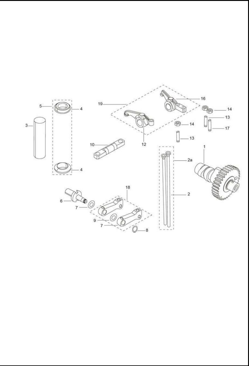
FIGURA N° 5 ARBOL LEVAS, VARILLAS, EMPUJADOR, LEVAS.
