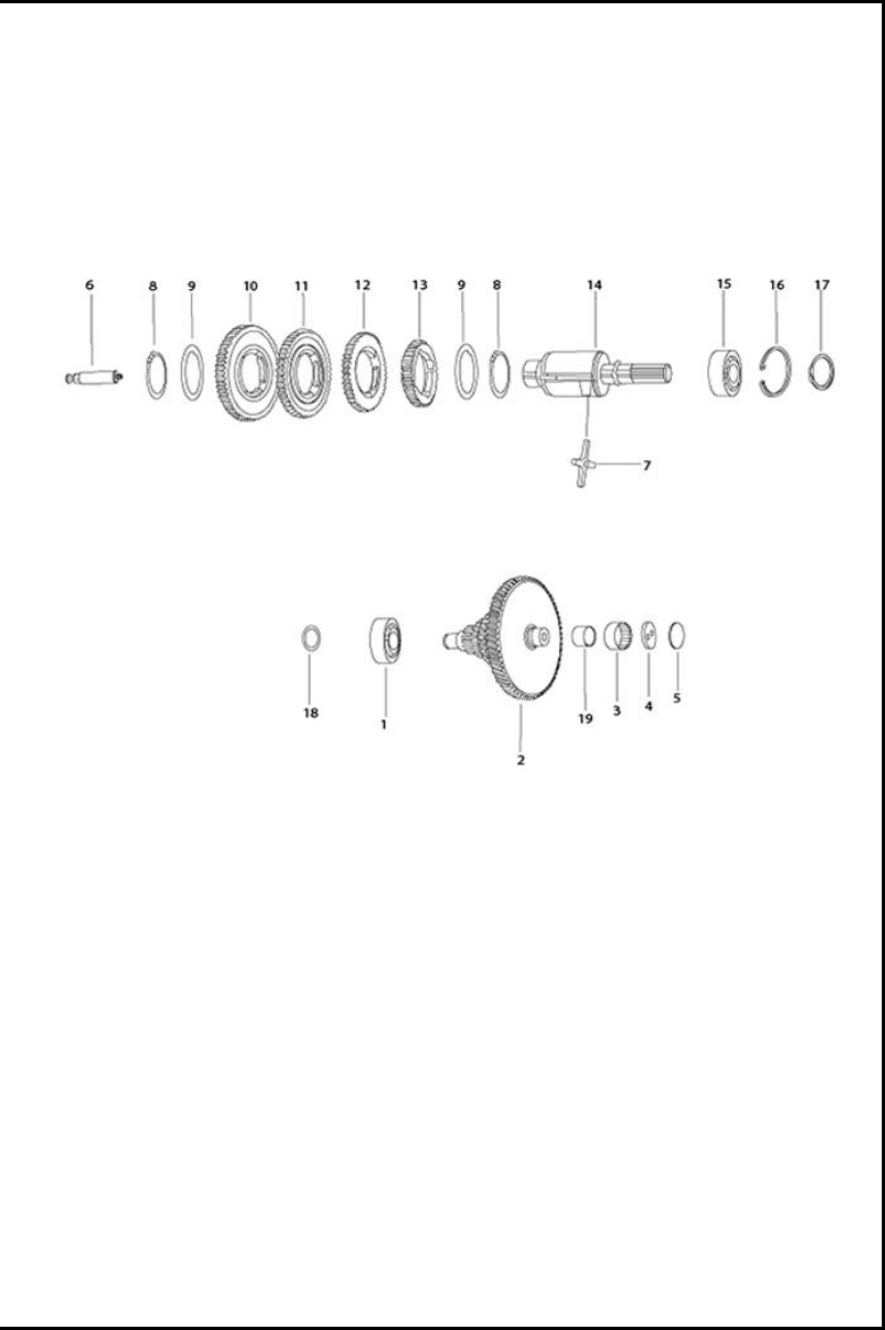
FIGURA N° 14 EJE PRIMARIO Y CAJA CAMBIOS
