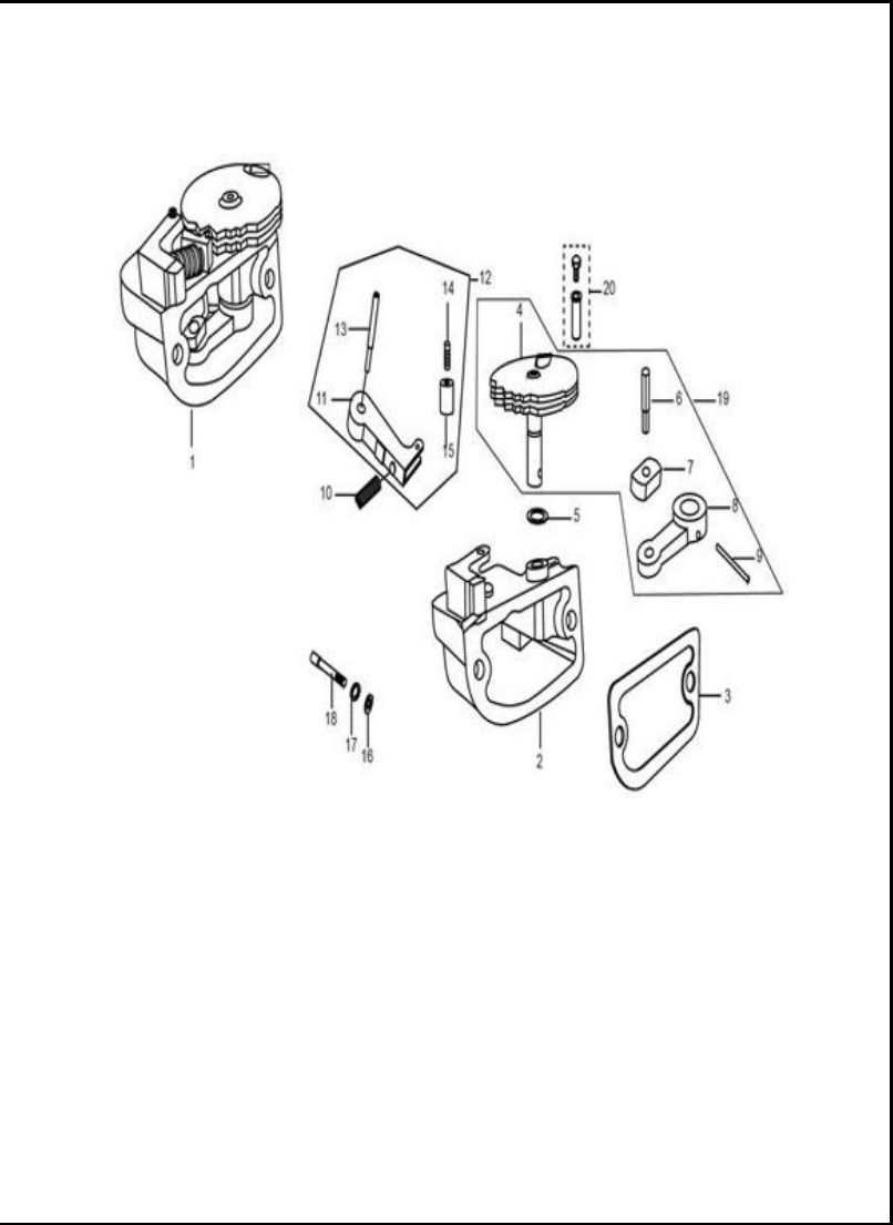
FIGURA N° 17 CAJA CAMBIOS Y MECANISMO DE CONTROL
