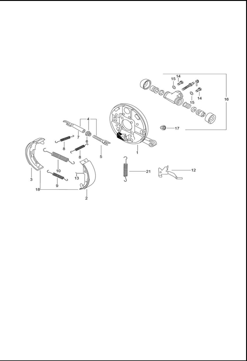
FIGURA N° 32 CONJUNTO FRENO DELANTERO AUTO AJUSTABLE
