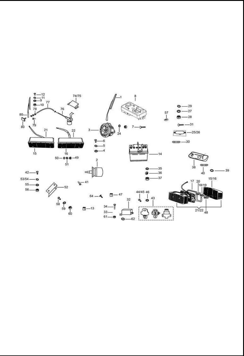
FIGURA N° 29 COMPONENTES ELÉCTRICOS
