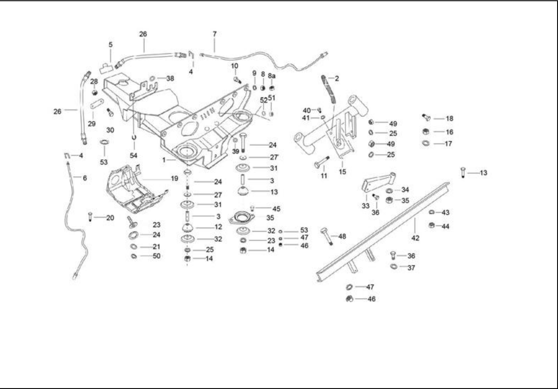
FIGURA N° 24 SOPORTE MOTOR
