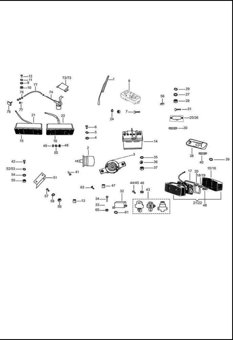
FIGURA N° 31 COMPONENTES ELÉCTRICOS
