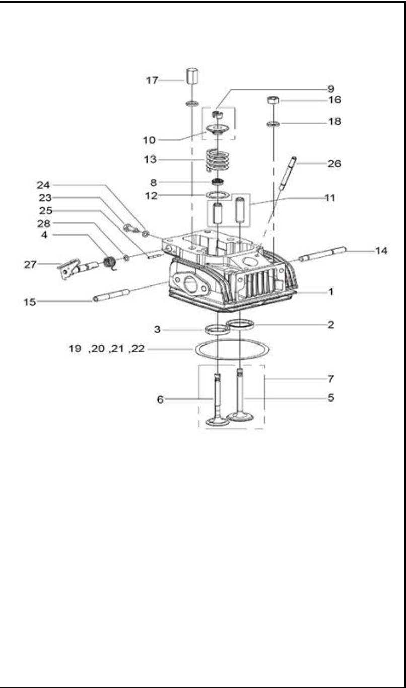
FIGURA N° 5 CULATA Y LEVA DESCOMPRESIÓN
