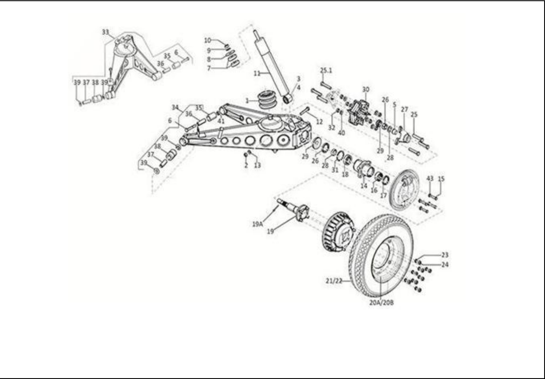
FIGURA N° 27 SUSPENSIÓN TRASERA
