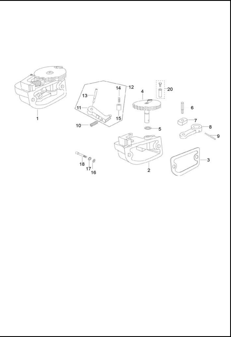
FIGURA N° 22 CAJA CAMBIOS Y MECANISMO CONTROL
