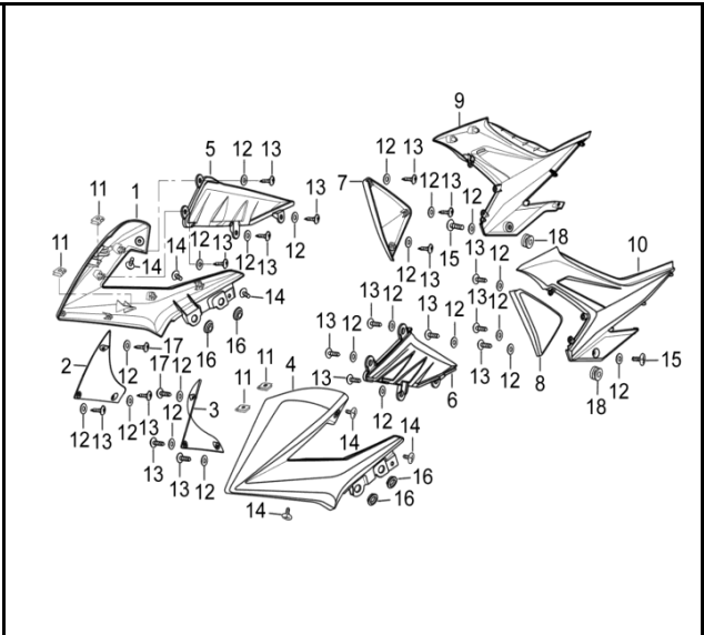
PAG. Nº 29 FIG. Nº 27: CUBIERTAS PAG. Nº 30
