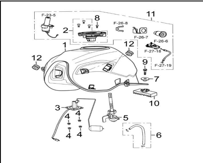
PAG. Nº 28 FIG. Nº 26: TANQUE GASOLINA
