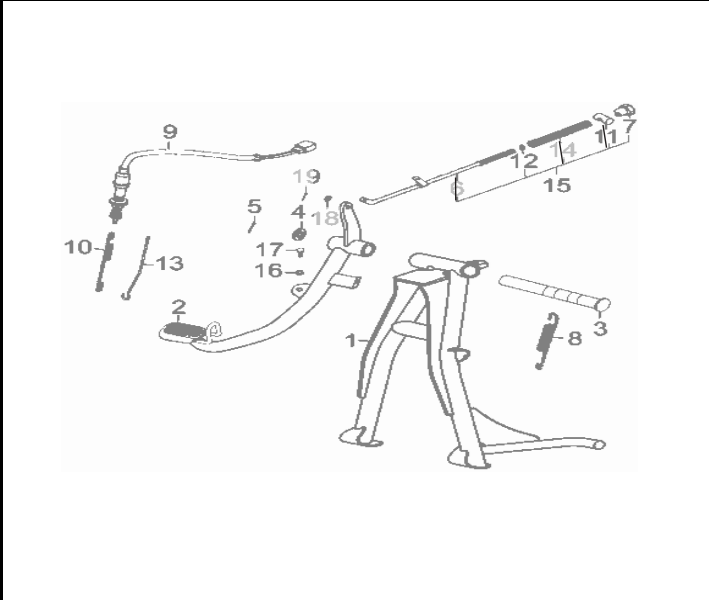
PAG. Nº 31 FIG. Nº 29: GATO CENTRAL - PEDAL FRENO
