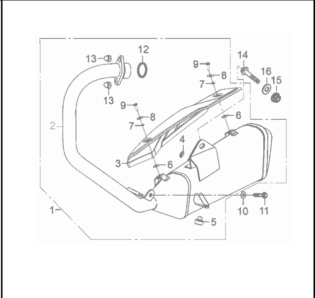
PAG. Nº 32 FIG. Nº 30: SILENCIADOR PAG. Nº 33
