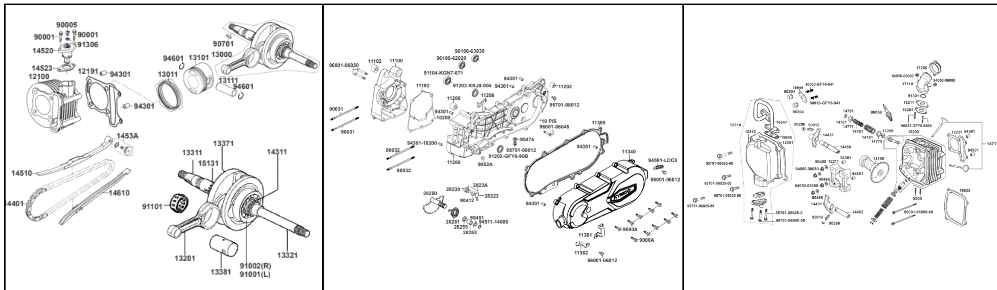
FIG. Nº 1 CILINDRO - PISTÓN - CIGÜEÑAL PAG. Nº 1 FIG. Nº 2 CARCASAS PAG. Nº 2-3 FIG. Nº 3 CULATA PAG. Nº 4-5
