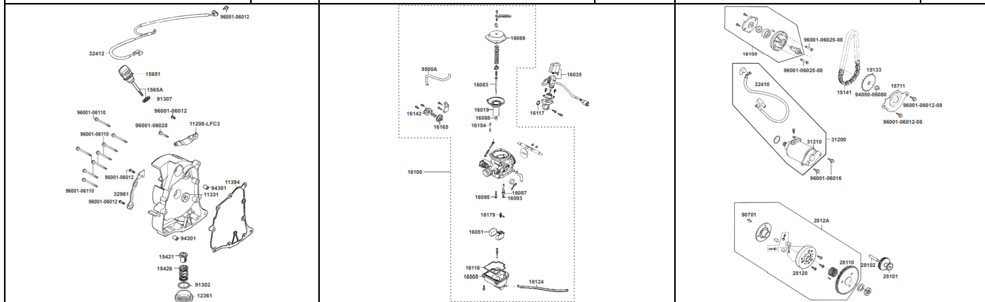
FIG. Nº 4 CUBIERTA MOTOR DERECHA PAG. Nº 6 FIG. Nº 5 CARBURADOR PAG. Nº 7 FIG. Nº 6 MOTOR DE ARRANQUE - BOMBA DE ACEITE PAG. Nº 8
