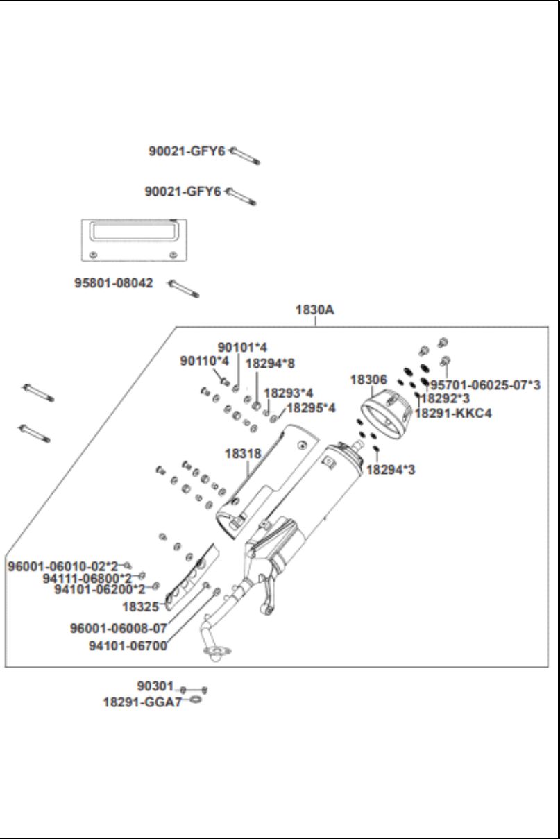
FIGURA N° 23: SILENCIADOR
