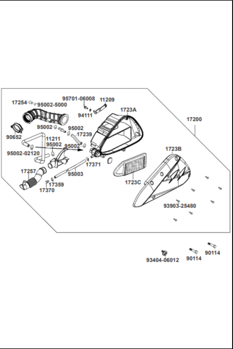
FIGURA N° 22: FILTRO DE AIRE
