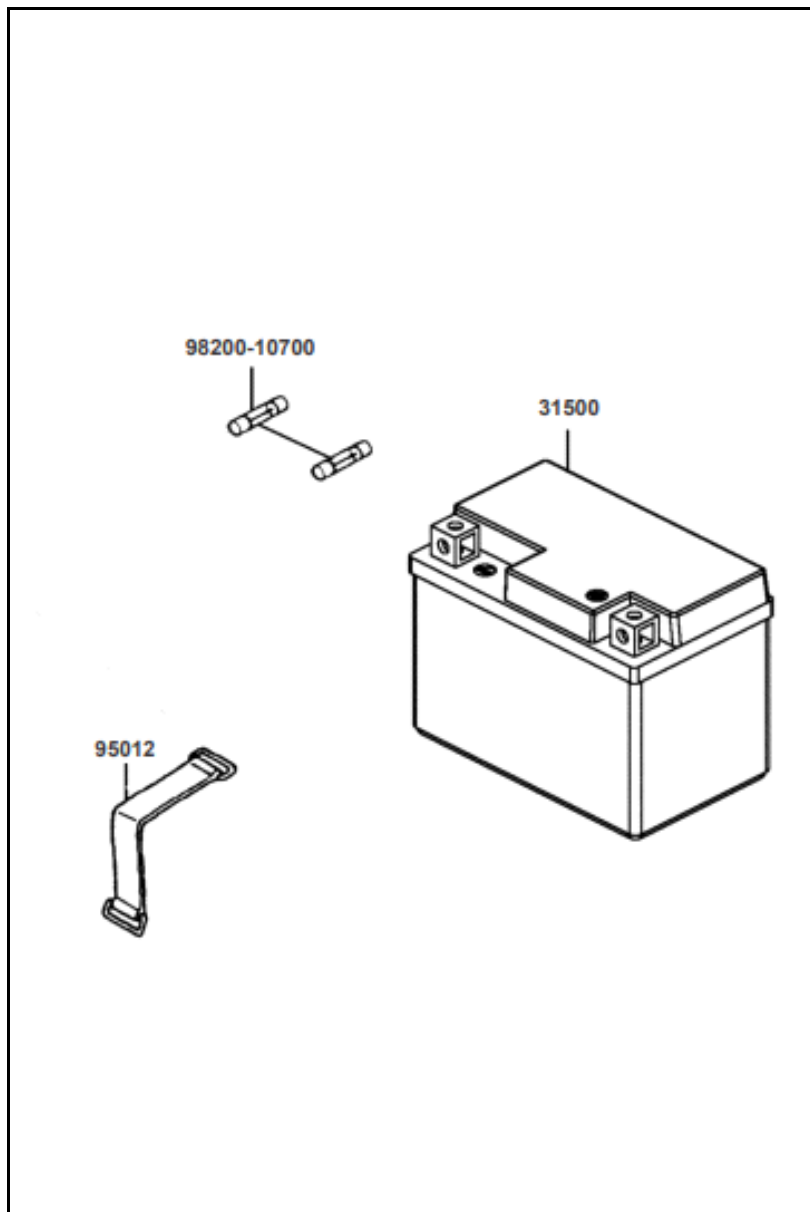
FIGURA N° 20: BATERÍA
