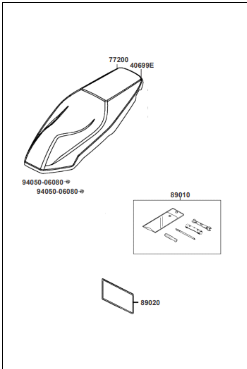
FIGURA N° 16: SILLÍN
