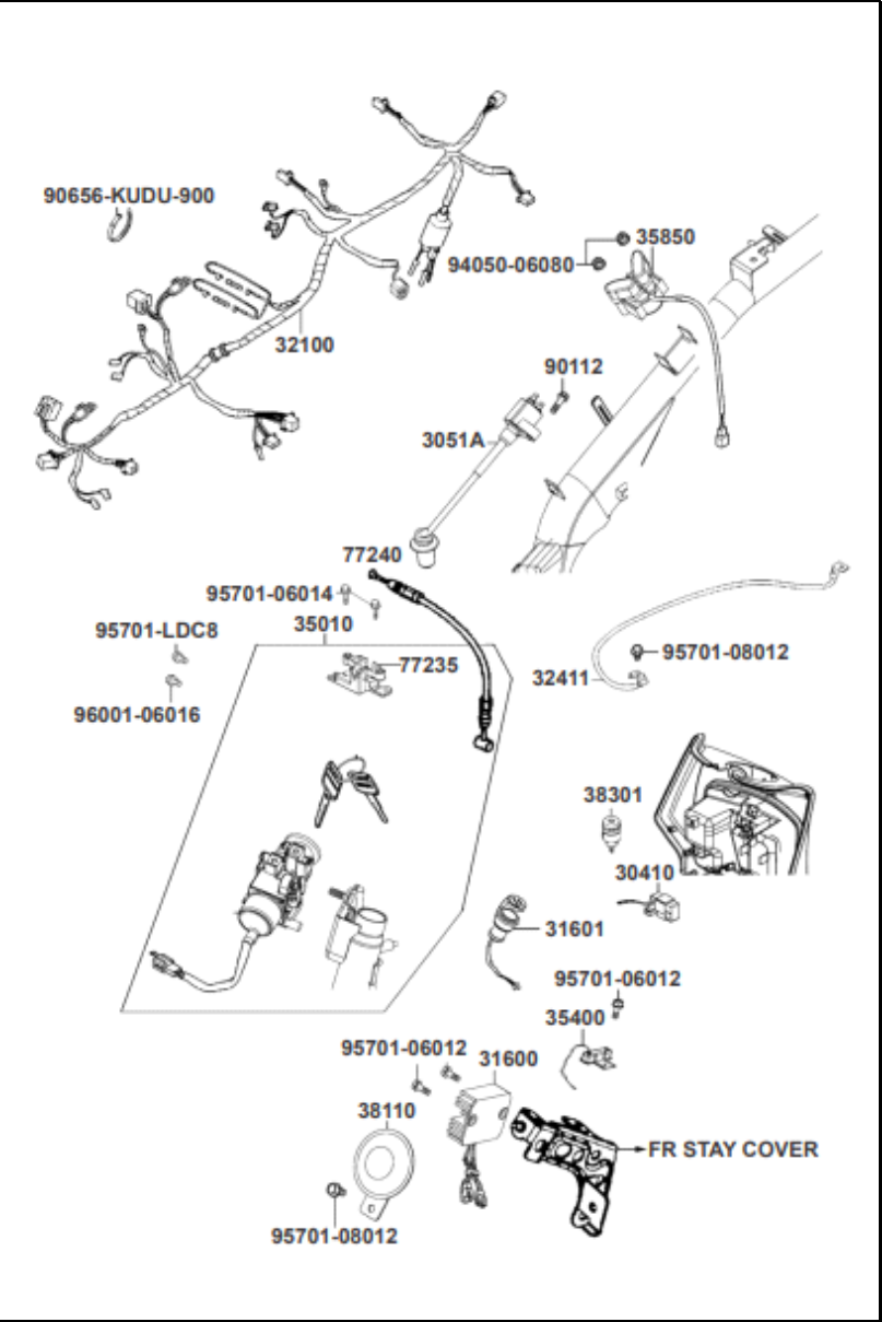
FIGURA N° 28: SISTEMA ELÉCTRICO
