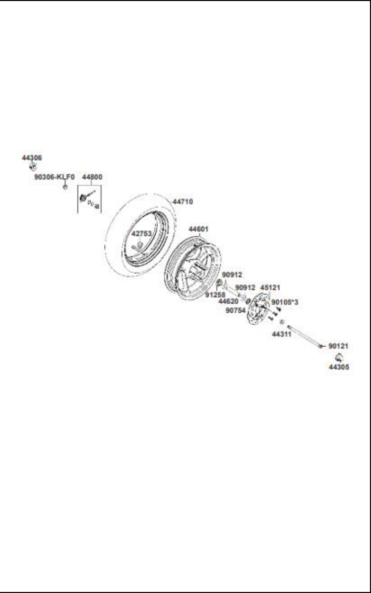
FIGURA 16: RIN DELANTERO
