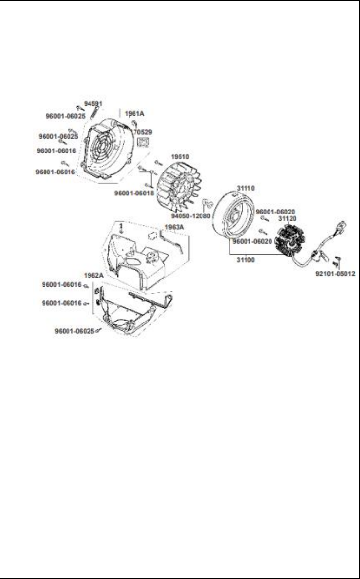
FIGURA 07: CUBIERTA VENTILADOR - MAGNETO
