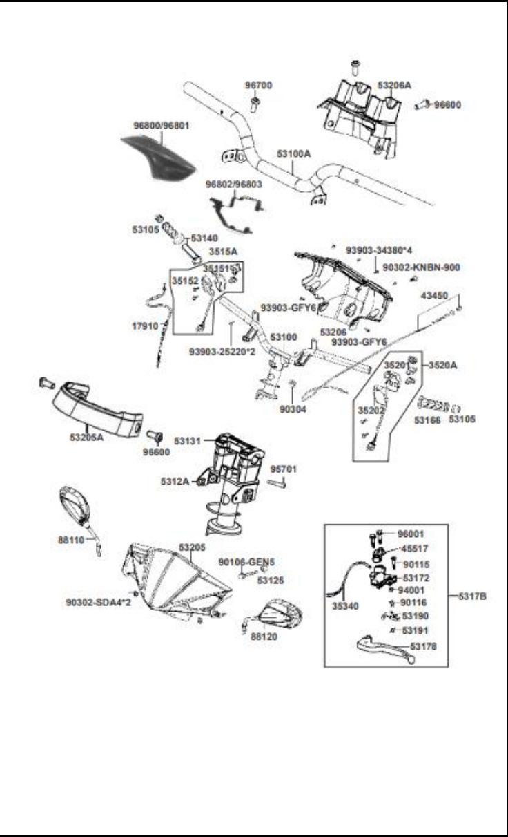
FIGURA 11 MANUBRIO - CUBIERTAS MANUBRIO (2/3)
