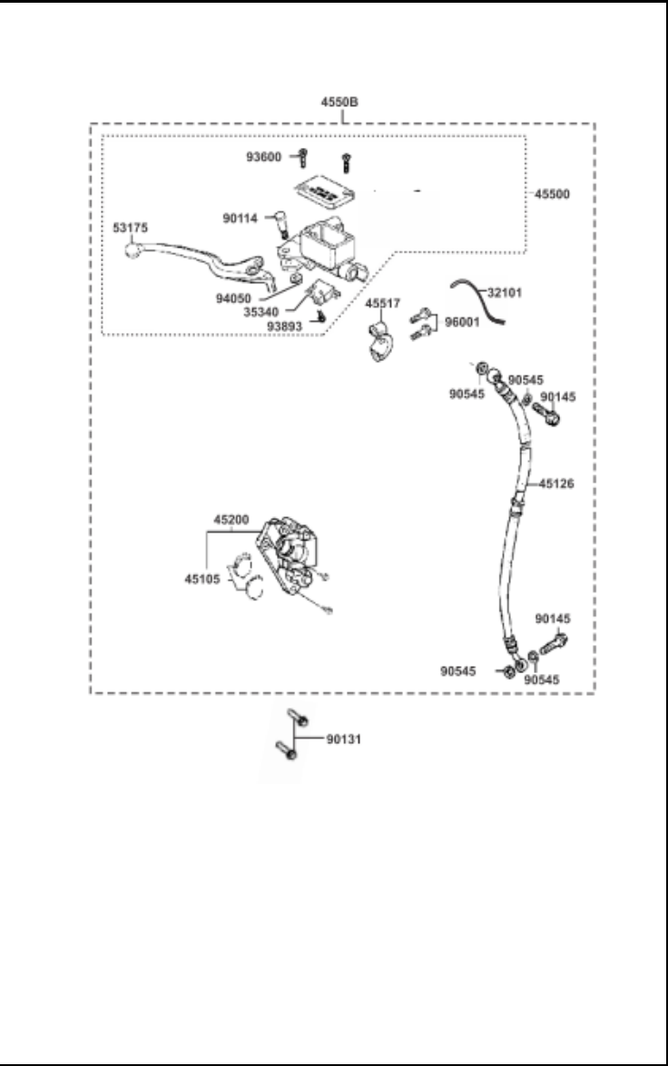
FIGURA 13: BOMBA DE FRENO
