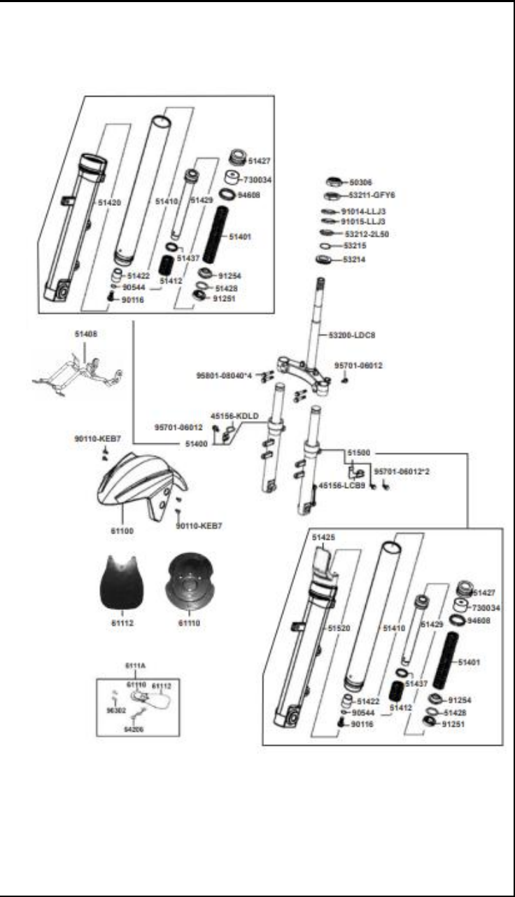
FIGURA 15: SUSPENSIÓN DELANTERA (1/2)
