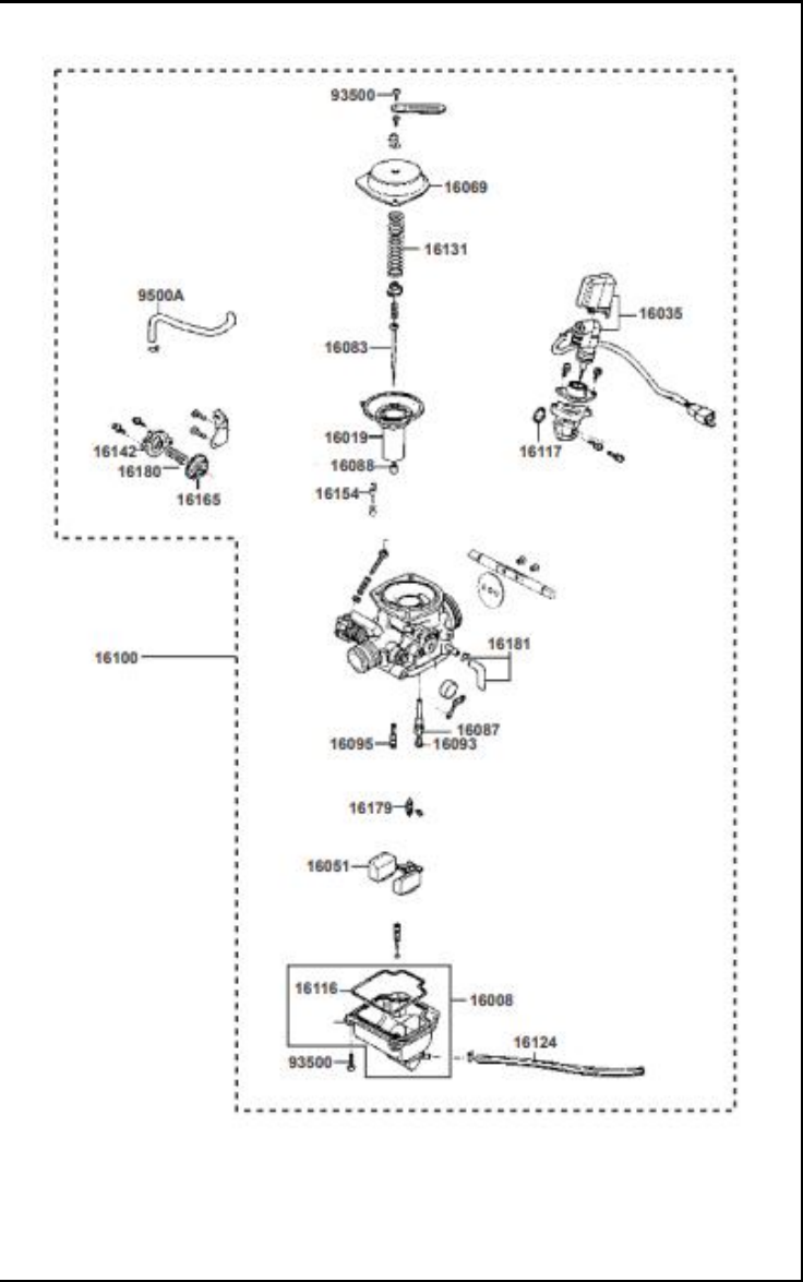
FIGURA 05: CARBURADOR
