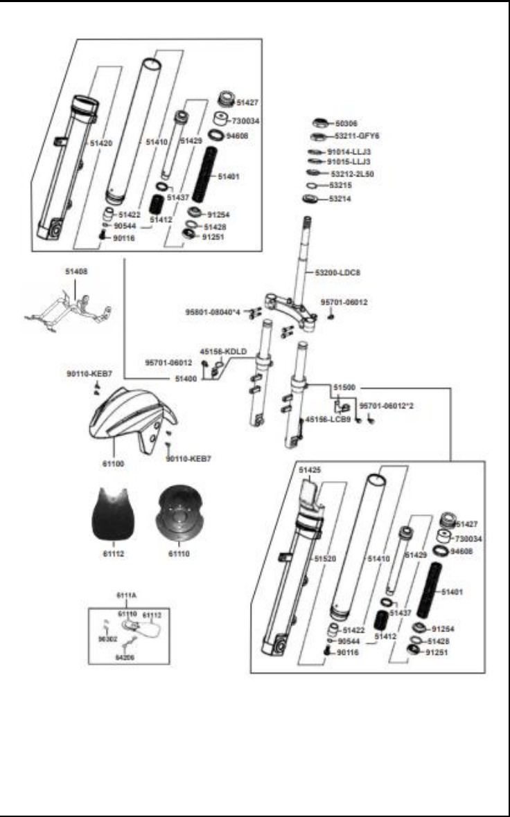
FIGURA 15 : SUSPENSIÓN DELANTERA (2/2)
