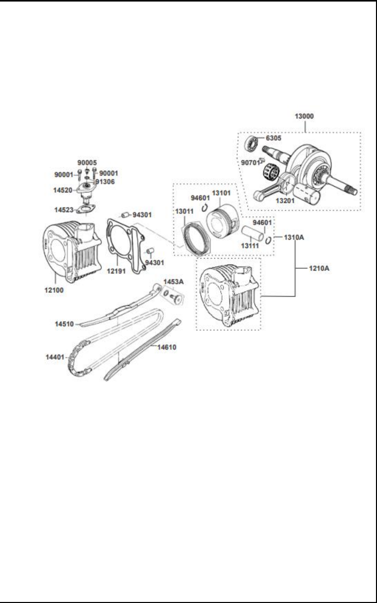
FIGURA 01: CILINDRO - PISTÓN - CIGÜEÑAL
