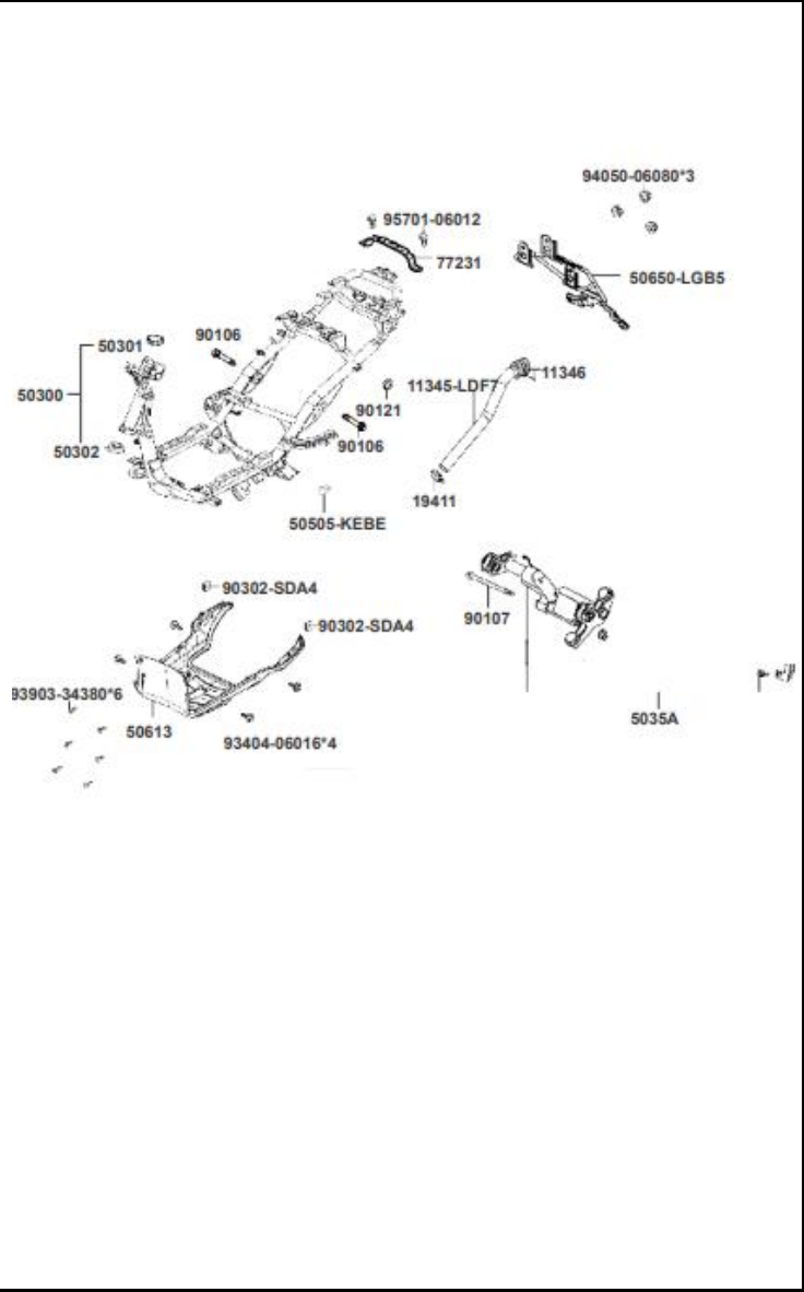
FIGURA 29 : CHASIS
