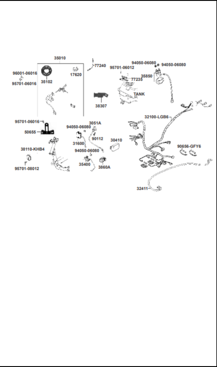
FIGURA 28:SISTEMA ELÉCTRICO (1/2)
