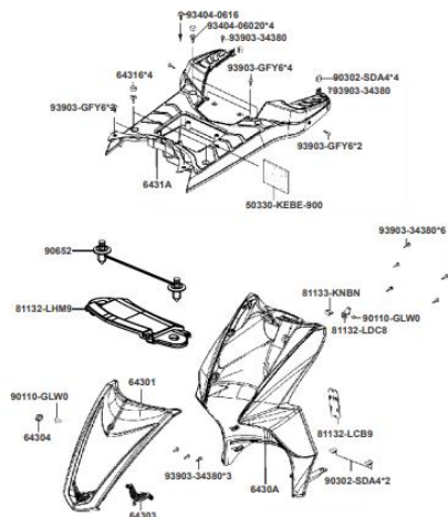
FIG. Nº 13: BOMBA DE FRENO PAG. Nº 18 FIG. Nº 14: CUBIERTA FRONTAL
