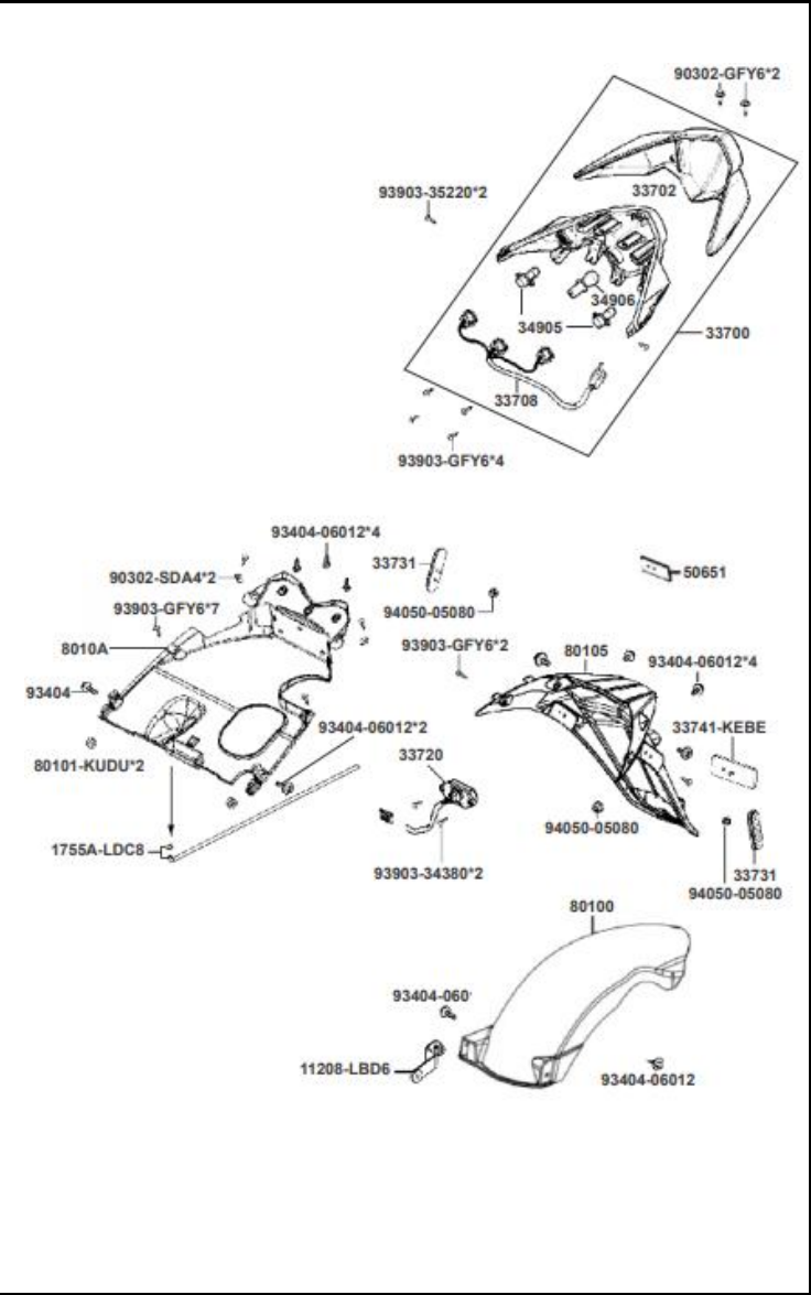
FIGURA 27: STOP - GUARDABARRO TRASERO
