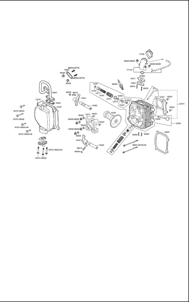
FIGURA 03 CULATA
