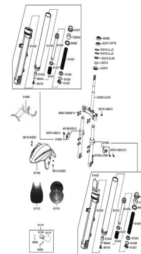
PAG. Nº 19 FIG. Nº 15: SUSPENSIÓN DELANTERA
