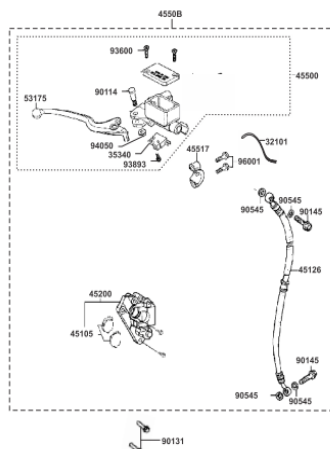
FIG. Nº 13: BOMBA DE FRENO
