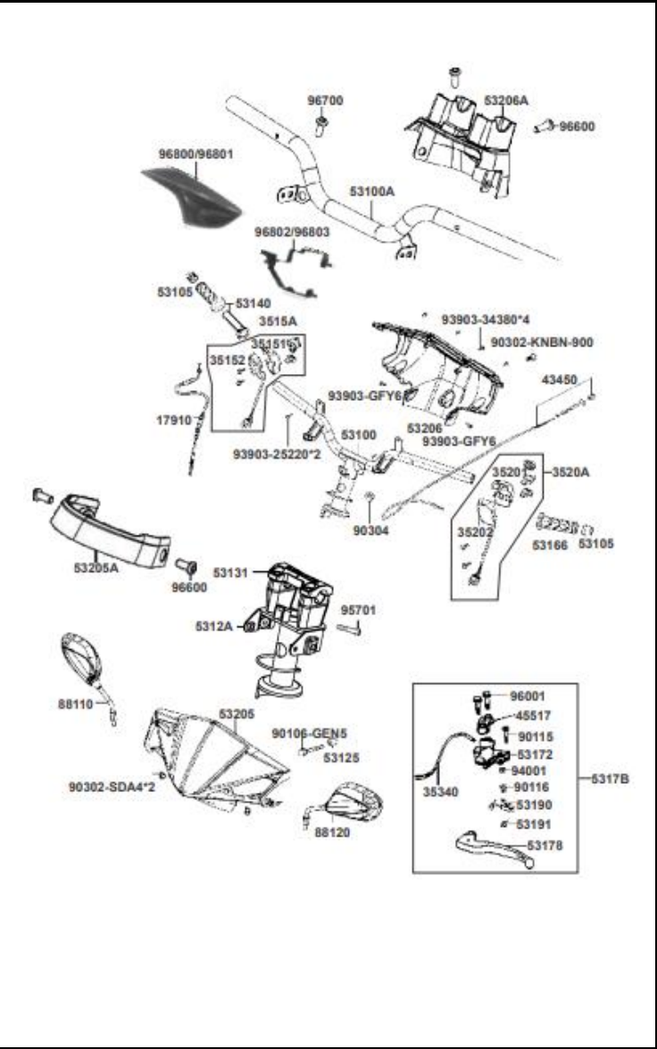
FIGURA 11 MANUBRIO - CUBIERTAS MANUBRIO (1/ 3)
