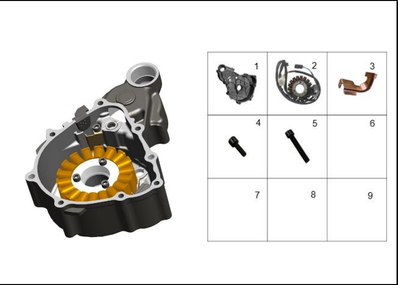
FIGURA 118: CUBIERTA CARCASA MOTOR IZQUIERDA
