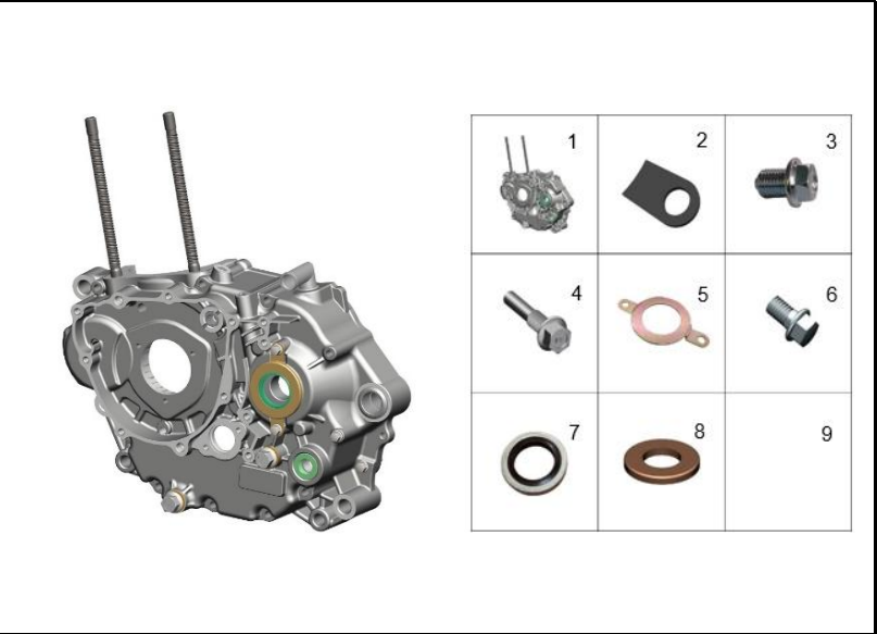
FIGURA 111: CARCASA IZQUIERDA 3
