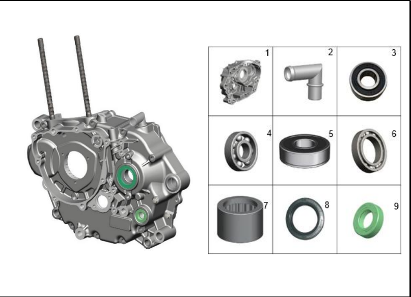
FIGURA 112: CARCASA IZQUIERDA 4
