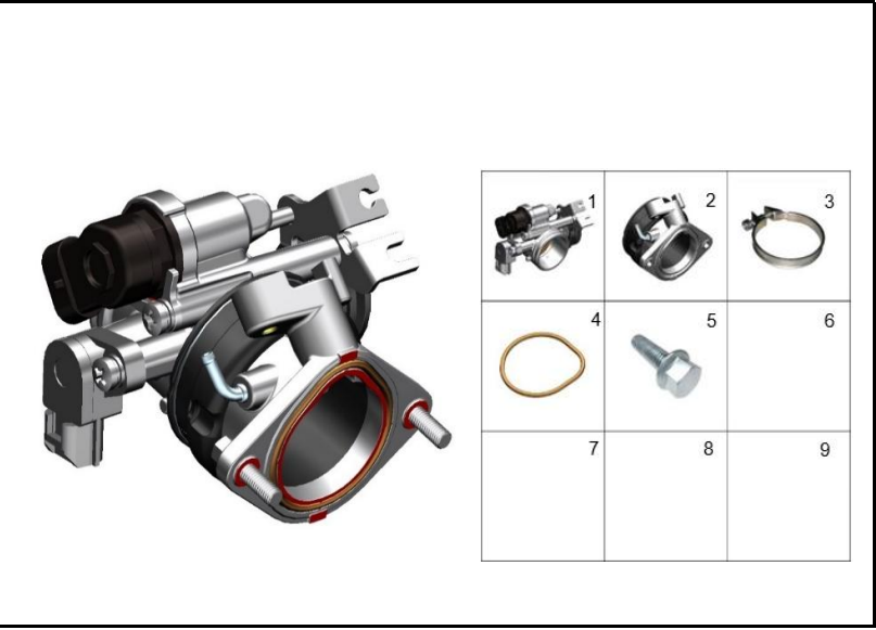
FIGURA 70: CUERPO DE INYECCIÓN
