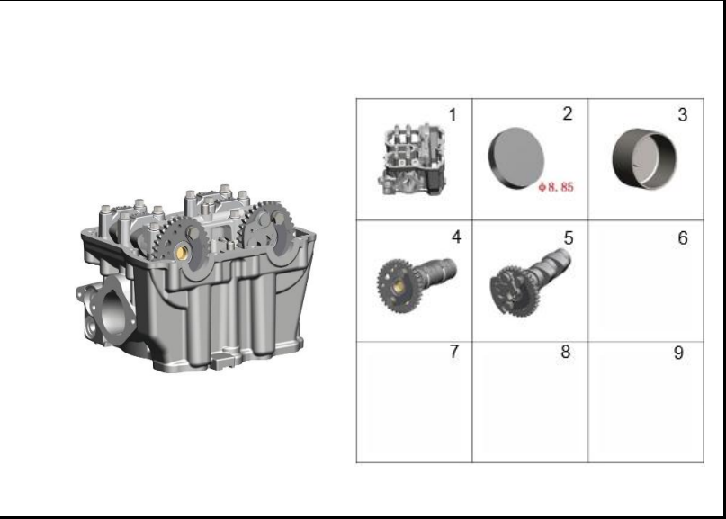
FIGURA 97: CULATA 3
