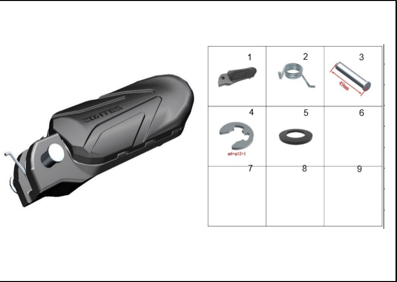
FIGURA 77: REPOSAPIE DELANTERO IZQUIERDO
