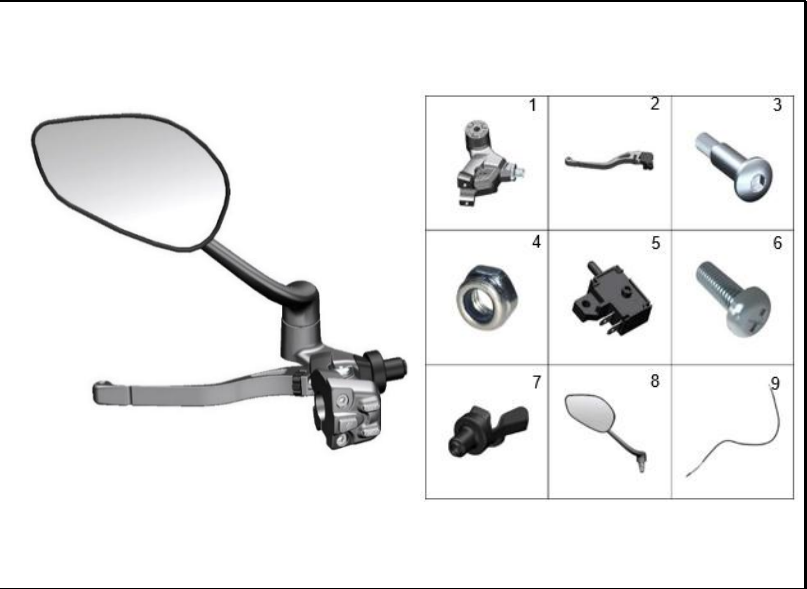
FIGURA 41: LEVA DE CLUTCH – ESPEJO IZQUIERDO
