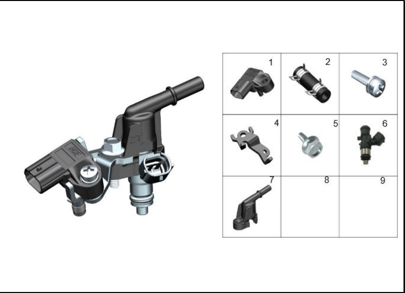
FIGURA 71: SOPORTE INYECTOR
