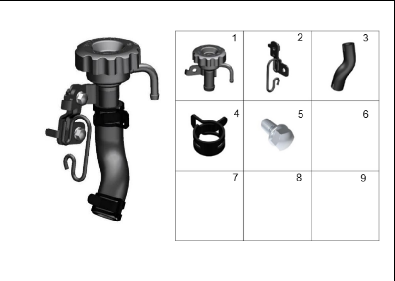
FIGURA 89: TAPA RADIADOR
