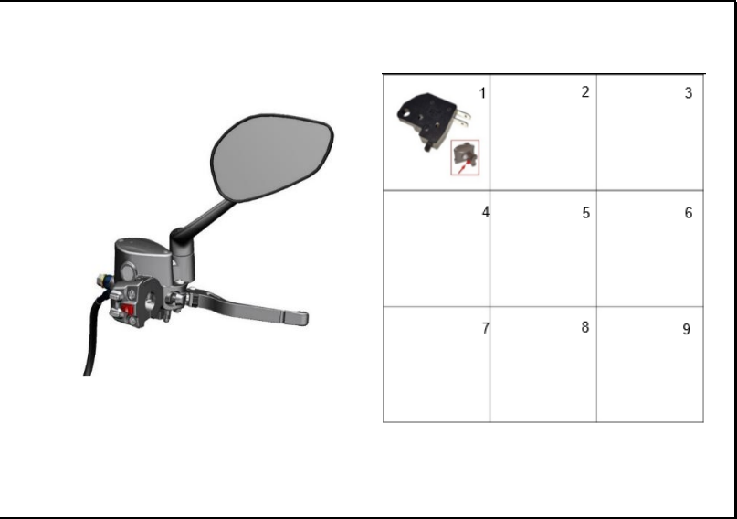
FIGURA 43: LEVA DE FRENO – ESPEJO DERECHO 2
