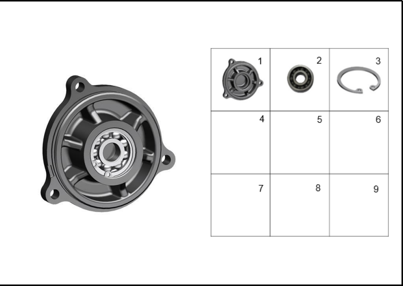
FIGURA 119: TAPA PIÑÓN REDUCTOR ARRANQUE
