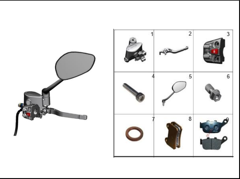
FIGURA 43: LEVA DE FRENO – ESPEJO DERECHO
