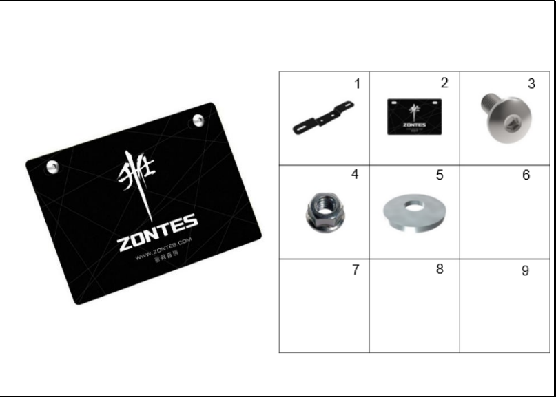
FIGURA 38: PORTA PLACA
