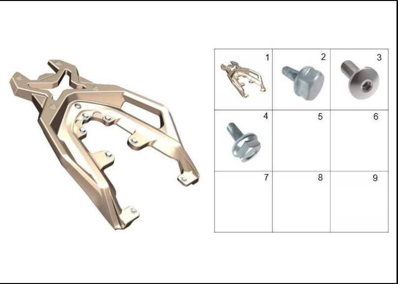
FIGURA 29: AGARRADERA TRASERA
