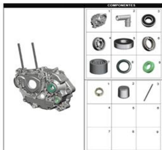
FIGURA N° 112: CARCA SA IZQUIERDA
