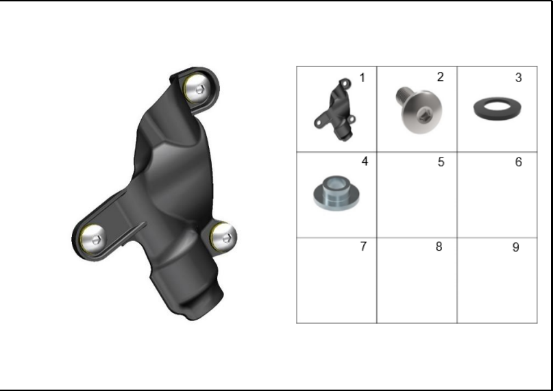
FIGURA 85: CUBIERTA BOMBA DE FRENO TRASERO
