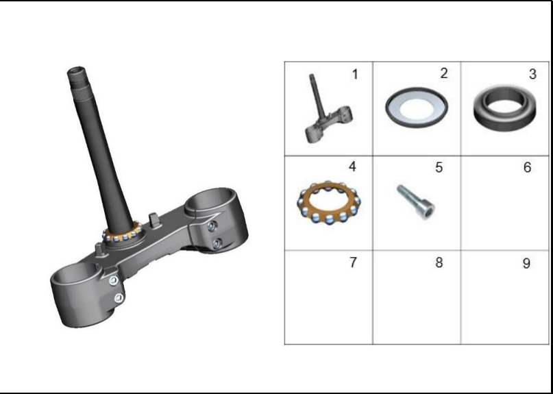
FIGURA 48: HORQUILLA DIRECCIÓN
