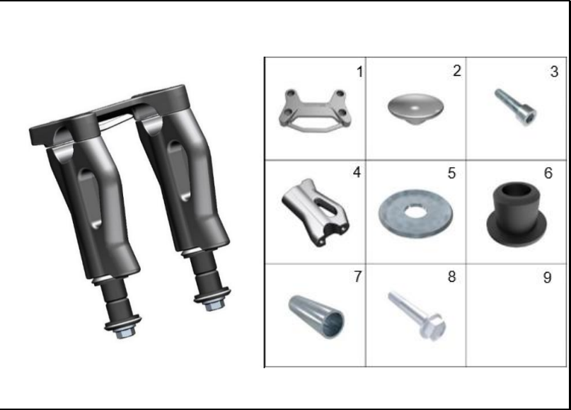
FIGURA 42: SOPORTE MANUBRIO
