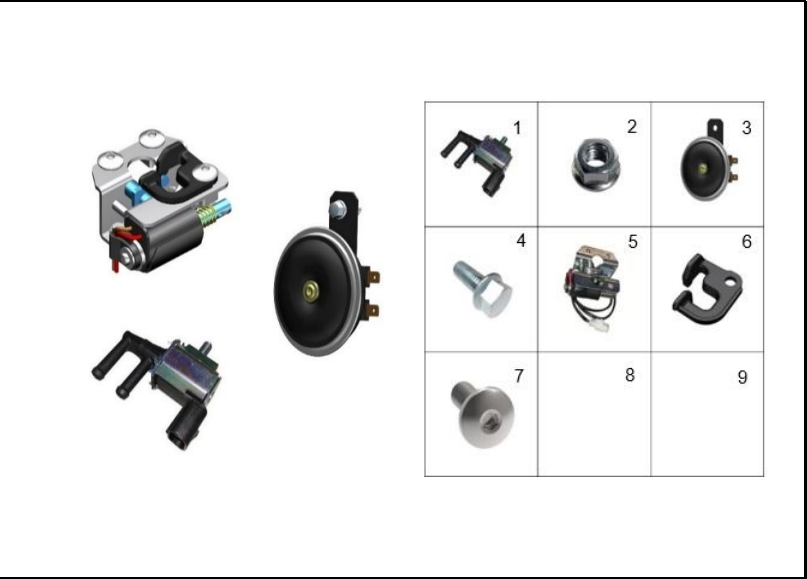
FIGURA 63: PITO Y SEGURO SILLIN
