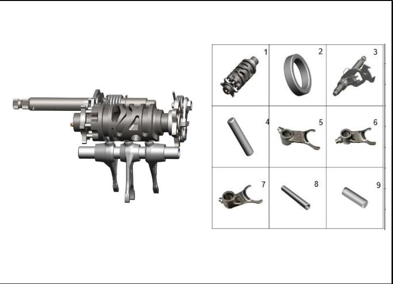
FIGURA 109: EJE DE CAMBIOS
