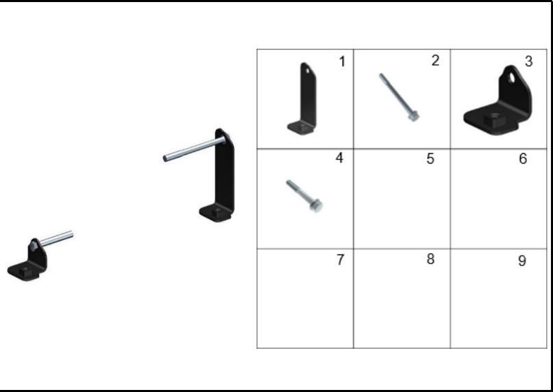
FIGURA 16: PLATINA IZQUIERDA CUBIERTA INFERIOR
