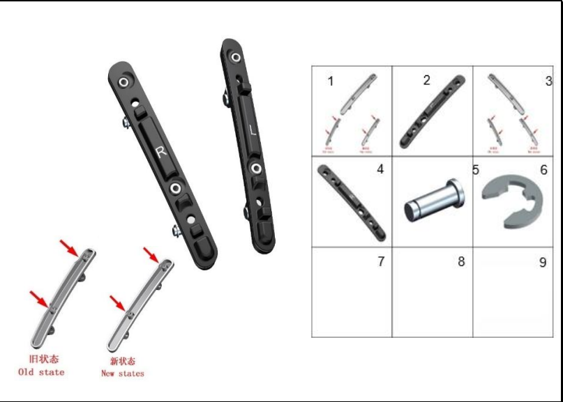
FIGURA 2: SOPORTES VISOR
