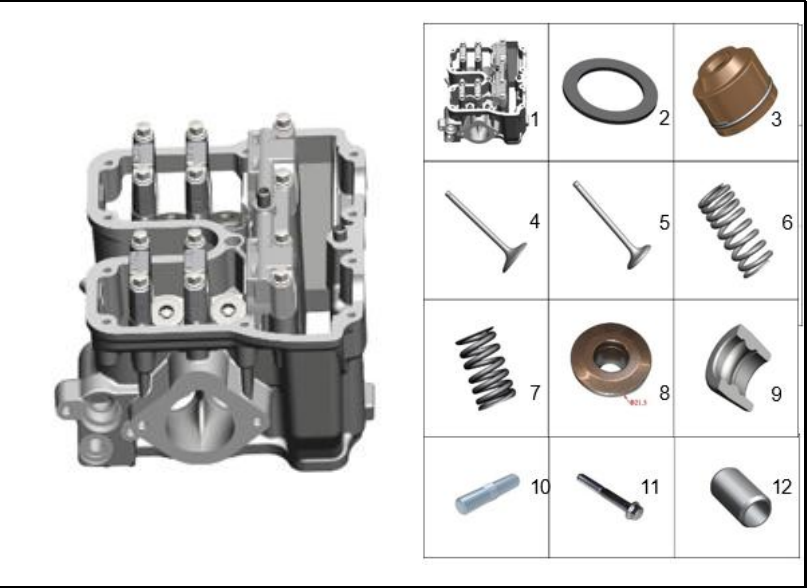
FIGURA 98: CULATA 4
