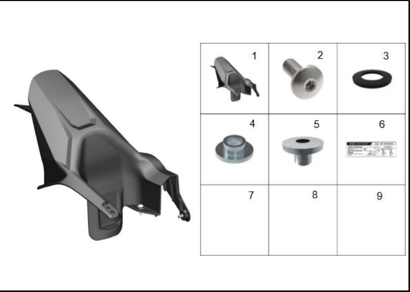
FIGURA 54: GUARDABARRO TRASERO INFERIOR INTERNO
