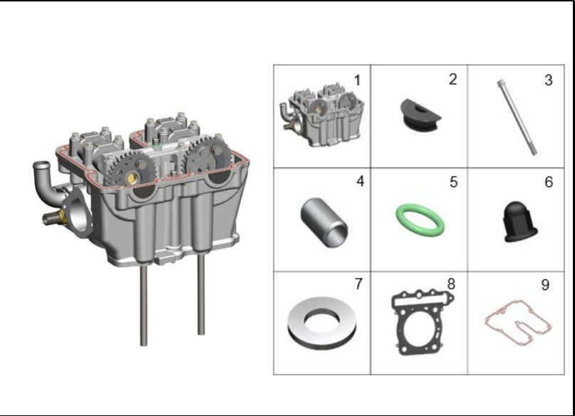
FIGURA 95: CULATA
