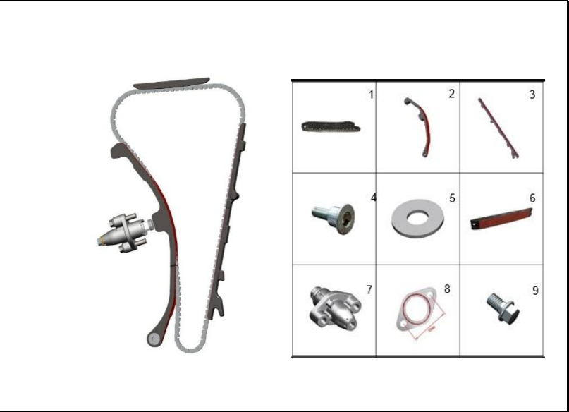
FIGURA 124: CADENILLA DE DISTRIBUCIÓN
