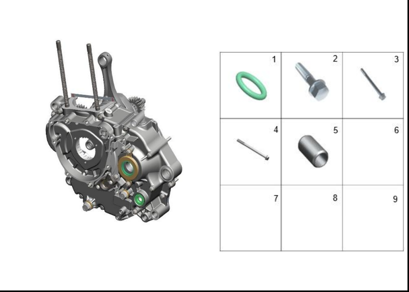
FIGURA 110: CARCASA IZQUIERDA 2
