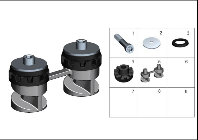
FIGURA 18: SOPORTE TANQUE DE COMBUSTIBLE
