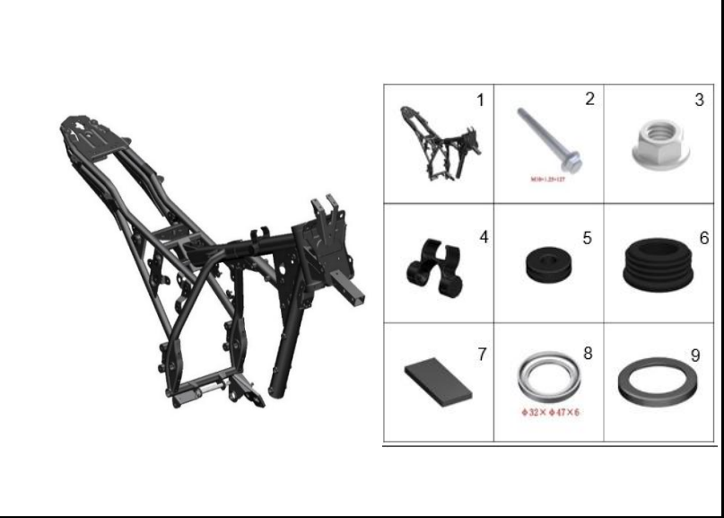
FIGURA 60: PARTES CHASIS
