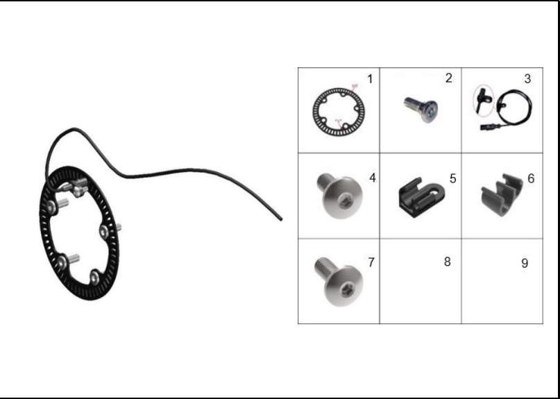
FIGURA 59: RUEDA FÓNICA ABS
