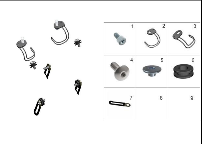
FIGURA 9: GUIAS
