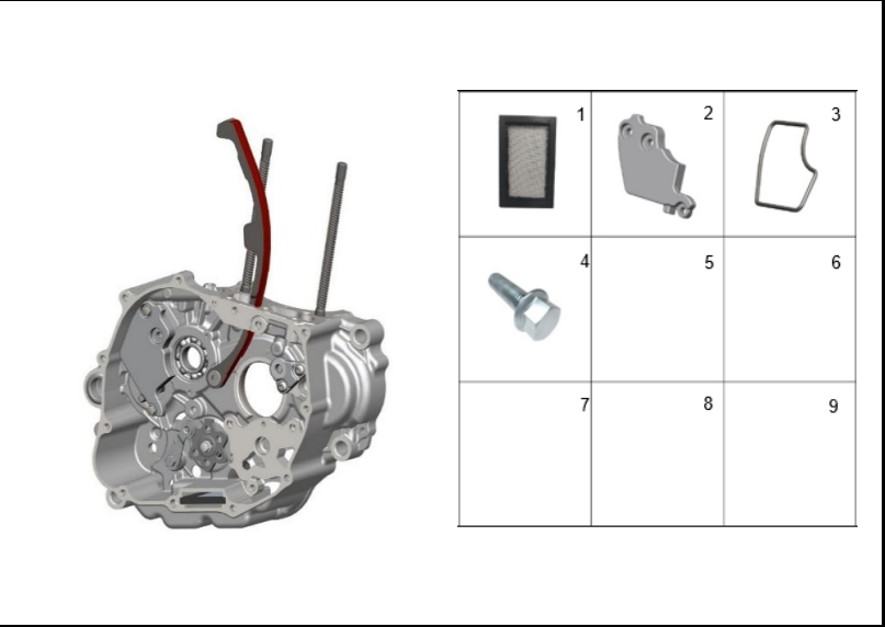
FIGURA 115: CARCASA DERECHA 4
