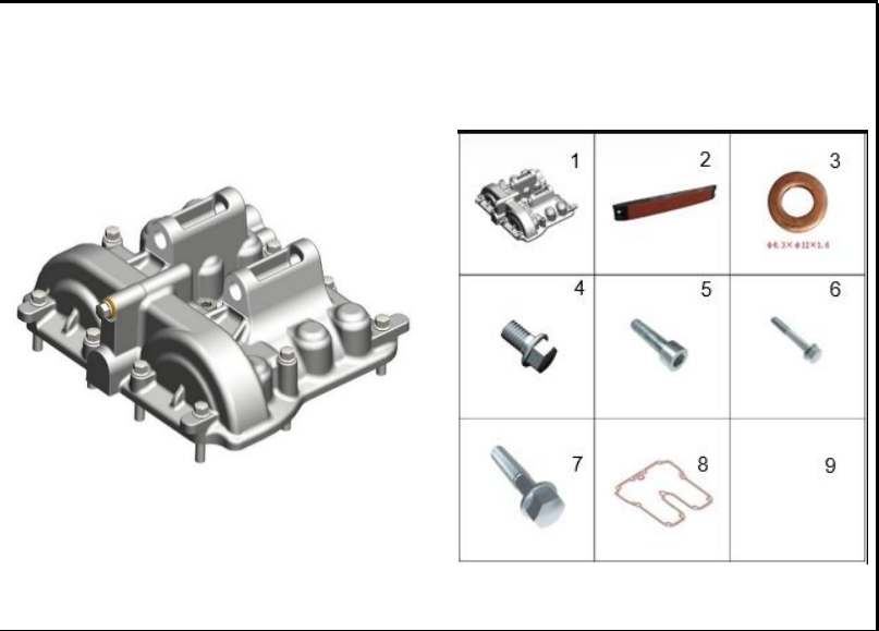
FIGURA 99: TAPA CULATA
