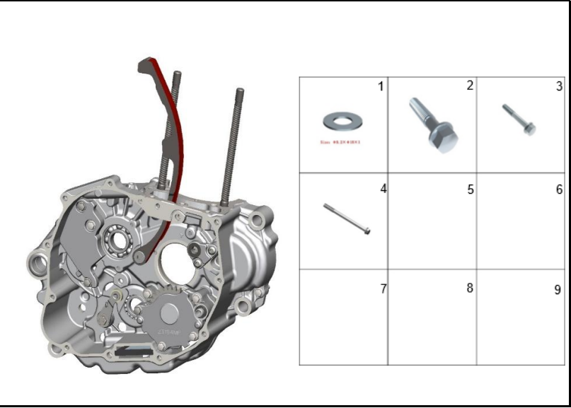
FIGURA 114: CARCASA DERECHA 2
