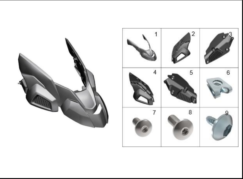
FIGURA 10: GUARDABARRO SUPERIOR
