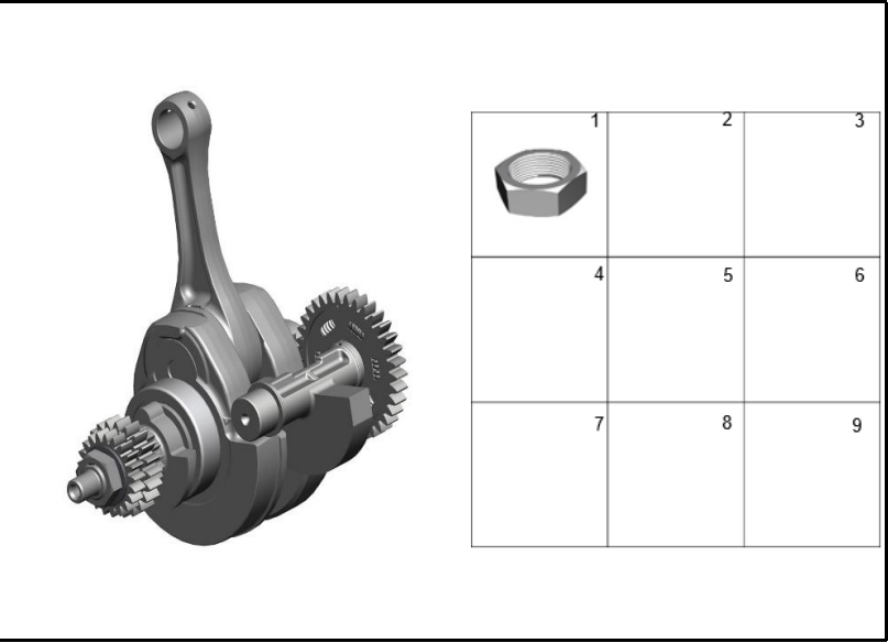
FIGURA 113: CIGÜEÑAL 2
