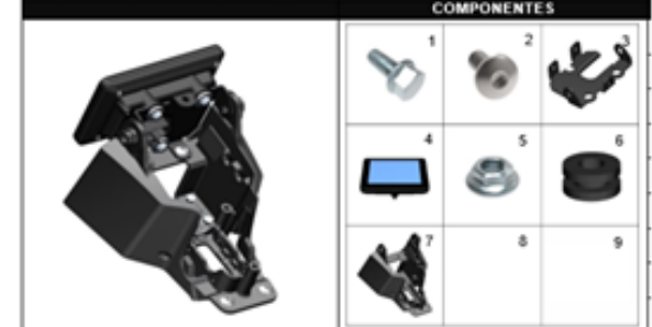
FIGURA 6: CUBIERTA INFERIOR VELOCIMETRO
