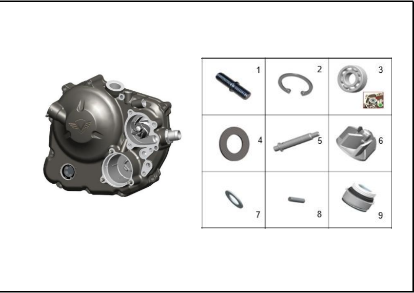
FIGURA 122: CUBIERTA CARCASA MOTOR DERECHA 2
