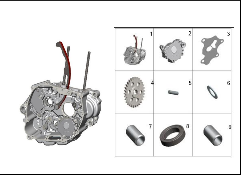
FIGURA 114: CARCASA DERECHA
