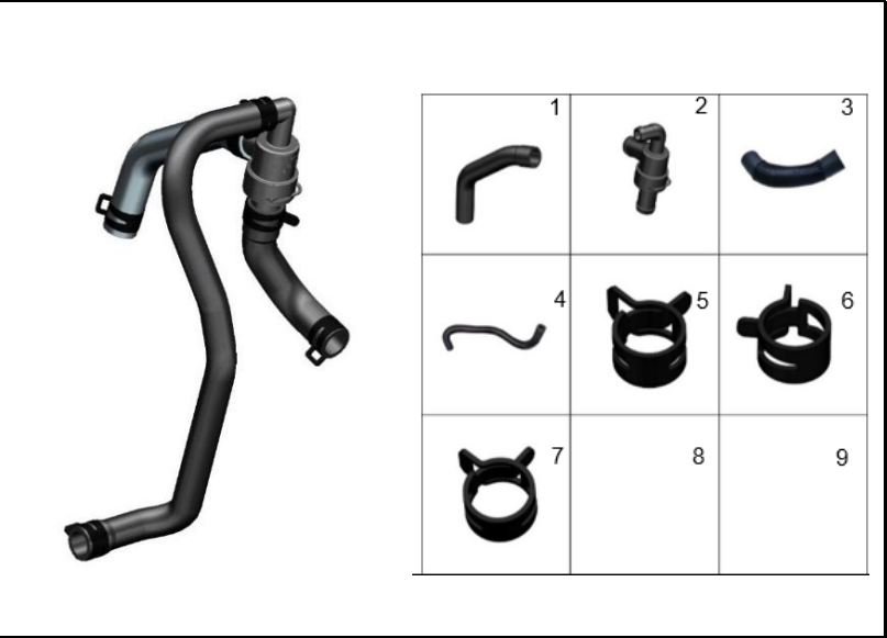
FIGURA 91: TERMOSTATO
