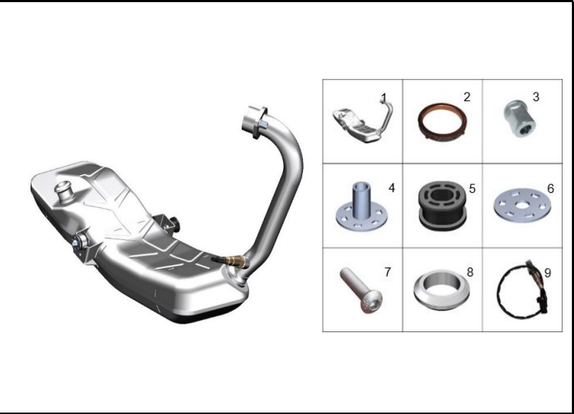
FIGURA 74: SILENCIADOR
