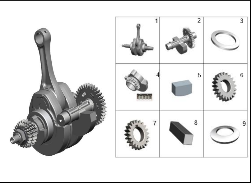
FIGURA 113: CIGÜEÑAL
