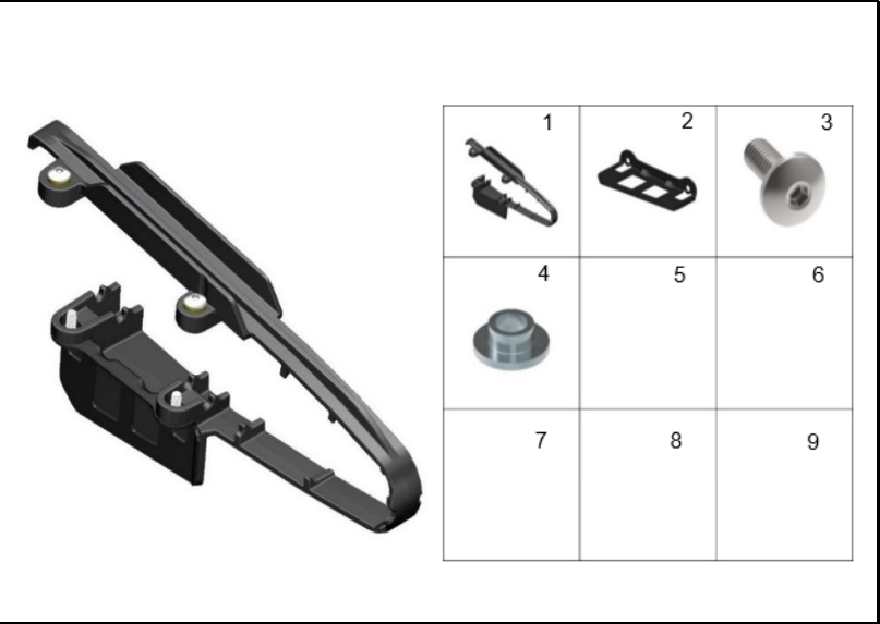
FIGURA 53: DESLIZADOR CADENA
