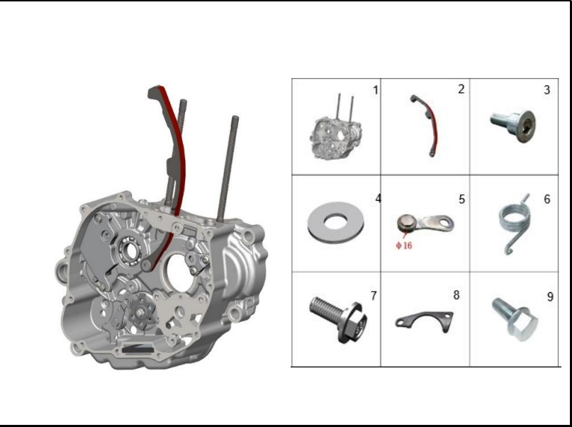
FIGURA 115: CARCASA DERECHA 3
