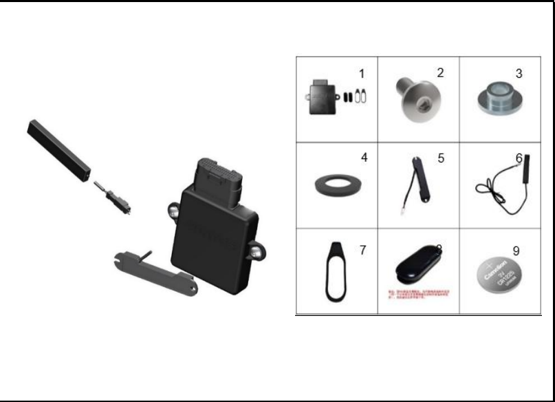
FIGURA 66: CONTROLADOR ENCENDIDO Y CONTROLES
