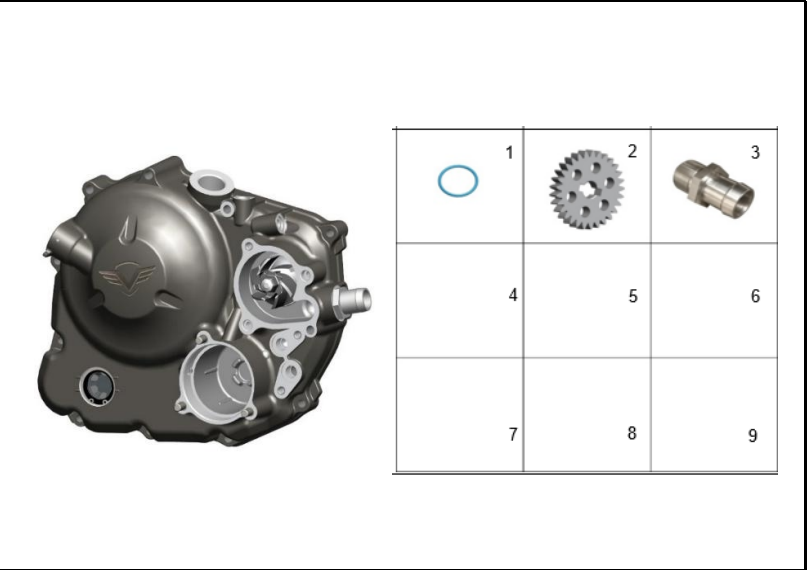
FIGURA 122: CUBIERTA CARCASA MOTOR DERECHA 3
