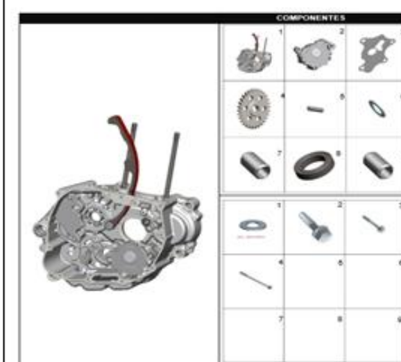
FIGURA N° 114: CARCA SA DERECHA
