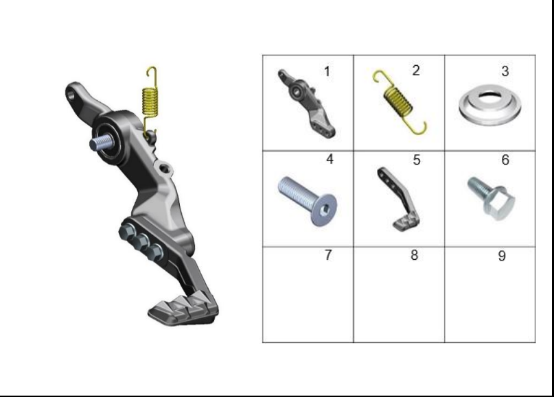
FIGURA 84: PEDAL DE FRENO
