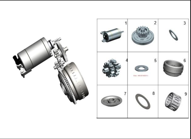
FIGURA 123: MOTOR DE ARRANQUE
