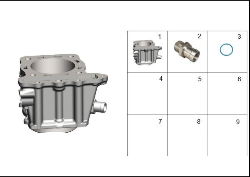
FIGURA 102: CILINDRO SOLO
