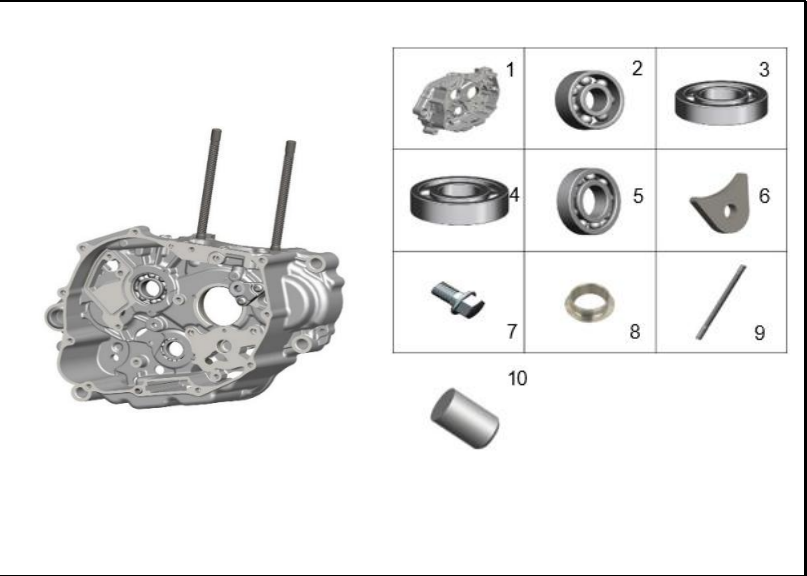
FIGURA 116: CARCASA DERECHA 5
