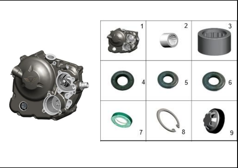
FIGURA 122: CUBIERTA CARCASA MOTOR DERECHA
