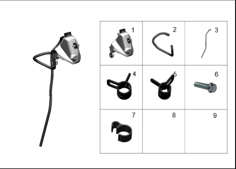
FIGURA 90: TANQUE RESERVORIO
