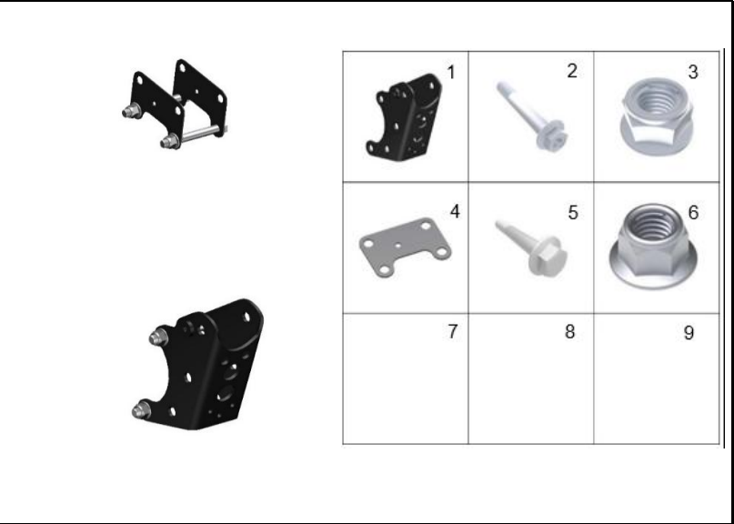
FIGURA 67: SOPORTE MOTOR
