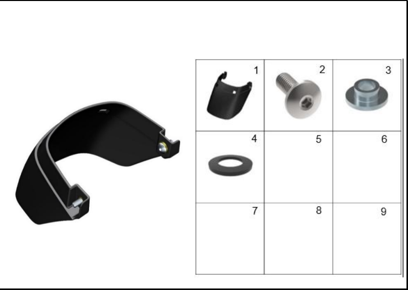
FIGURA 14: COMPLEMENTO GUARDABARRO DELANTERO 2
