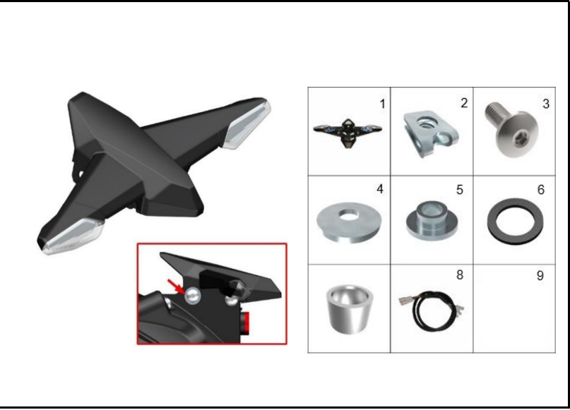
FIGURA 36: SOPORTE DIRECCIONALES COMPLETO
