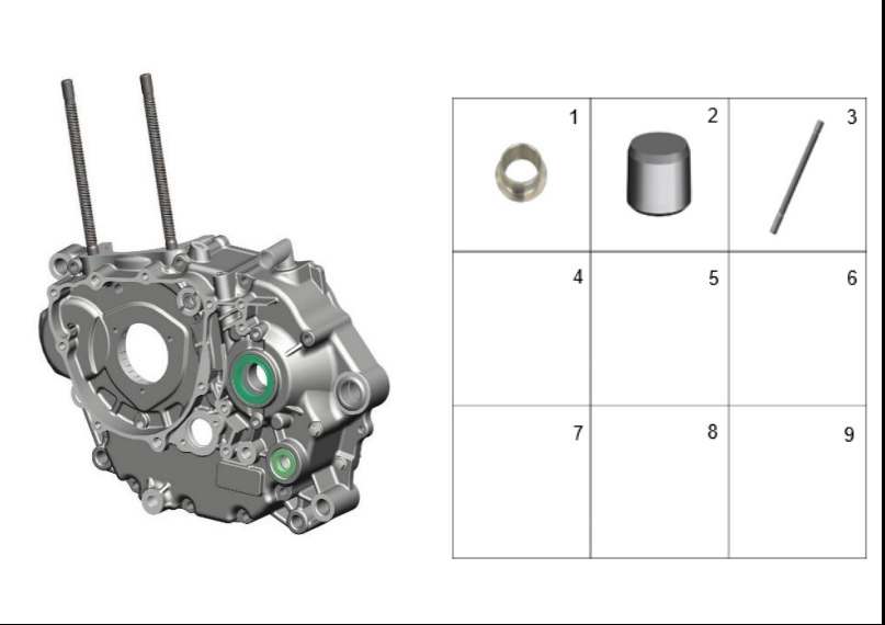
FIGURA 112: CARCASA IZQUIERDA 5
