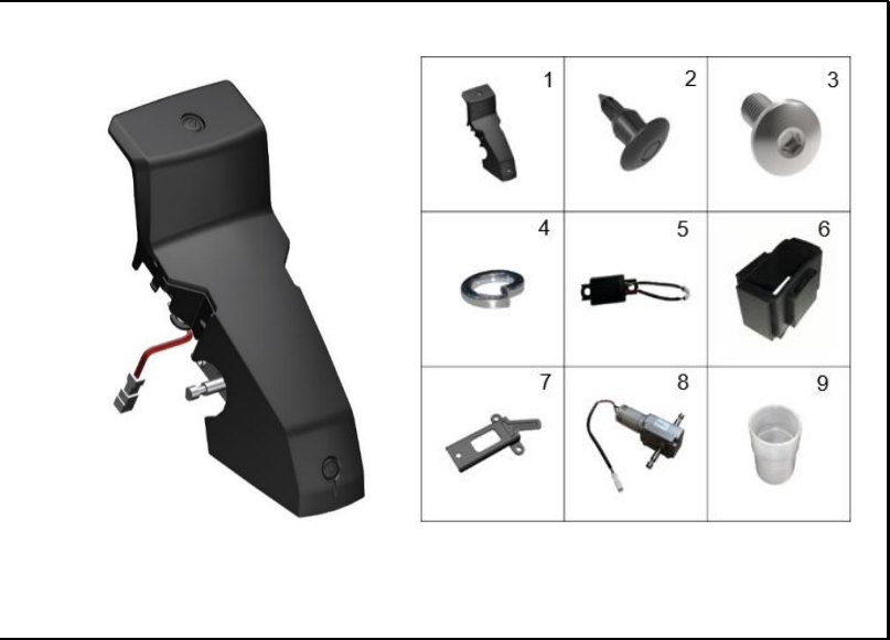
FIGURA 5: CUBIERTA CENTRAL
