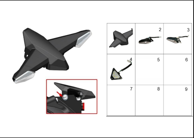
FIGURA 37: SOPORTE DIRECCIONALES TRASERAS
