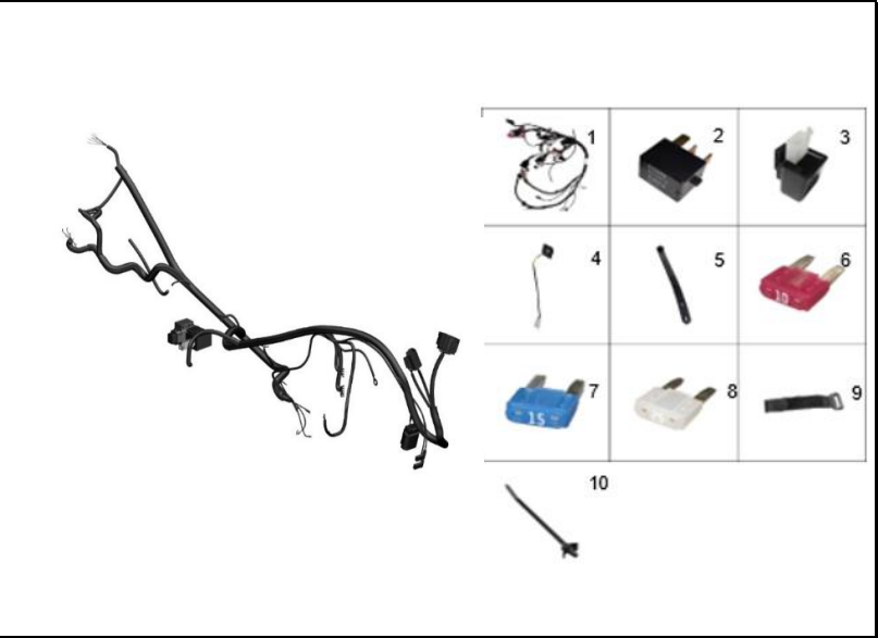
FIGURA 62: PARTES ELECTRICAS
