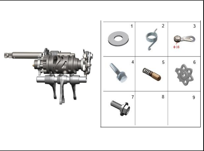
FIGURA 109: EJE DE CAMBIOS 2
