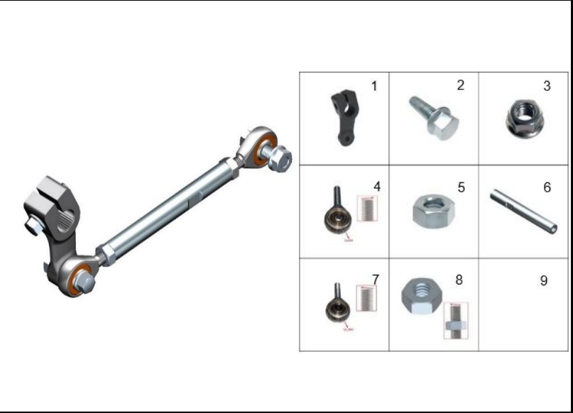
FIGURA 79: MUÑON PEDAL DE CAMBIOS
