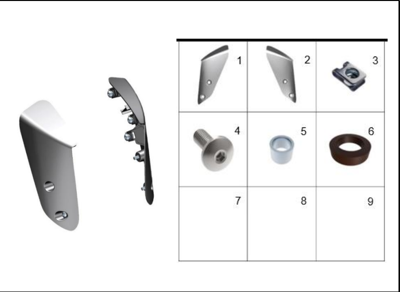
FIGURA 13: COMPLEMENTOS GUARDABARRO DELANTERO
