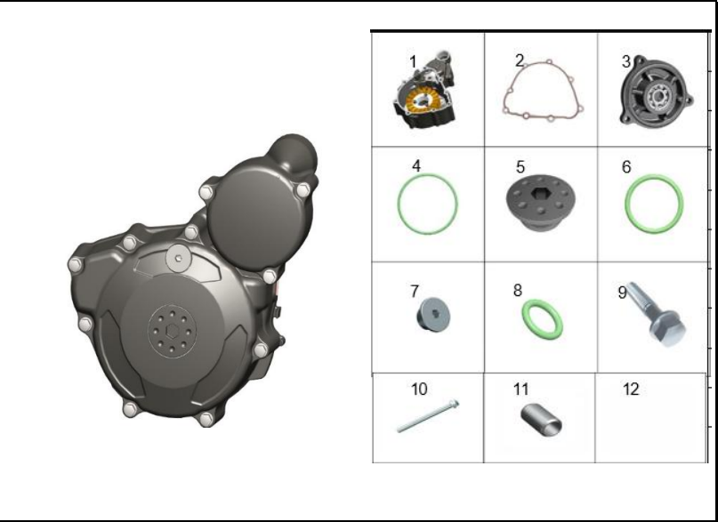
FIGURA 117: TAPA CÁRTER IZQ
