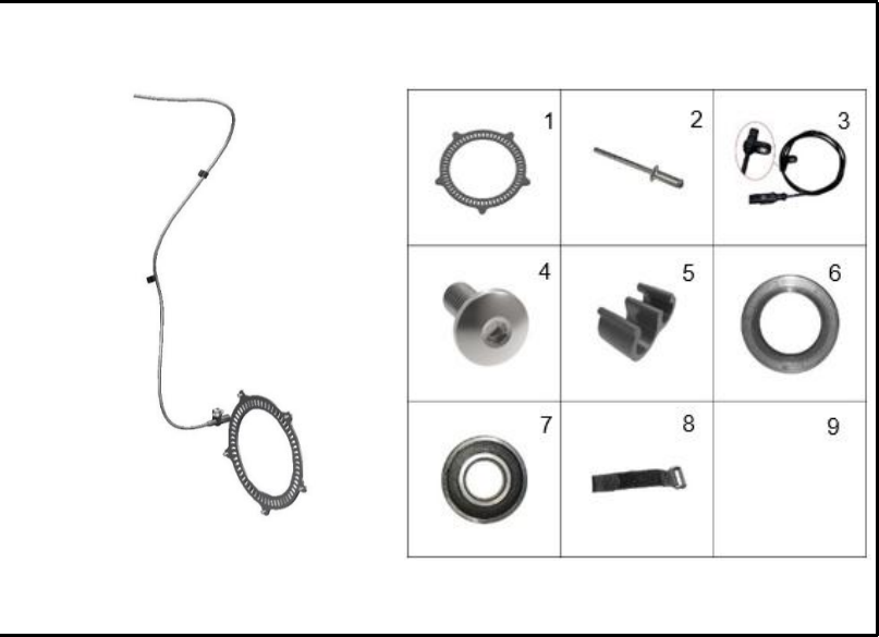
FIGURA 51: RUEDA FONICA RUEDA DELANTERA
