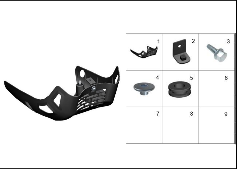
FIGURA 15: CUBIERTA INFERIOR
