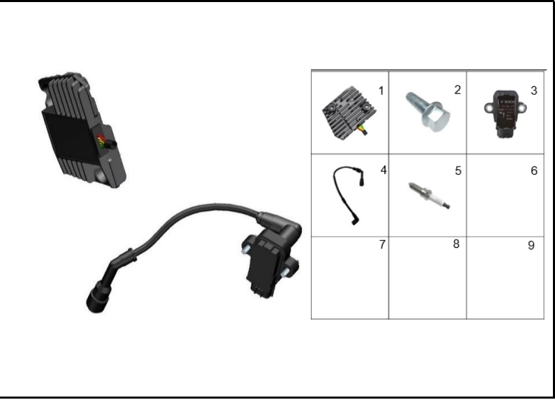
FIGURA 64: REGULADOR
