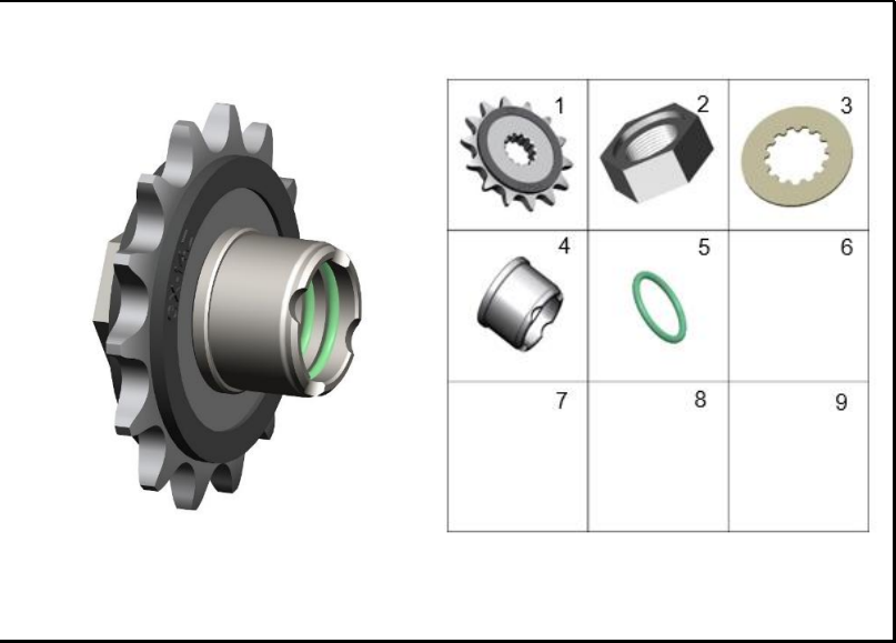
FIGURA 108: PIÑÓN DE SALIDA
