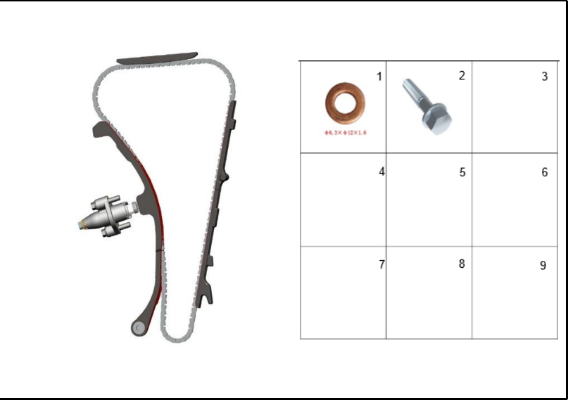
FIGURA 124: CADENILLA DE DISTRIBUCIÓN 2
