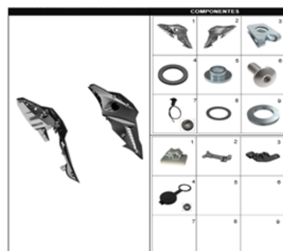
FIGURA N° 23: CUBIERTAS LATERALES
