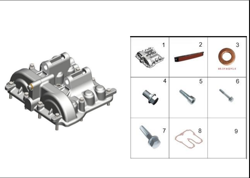
FIGURA 99: TAPA CULATA
