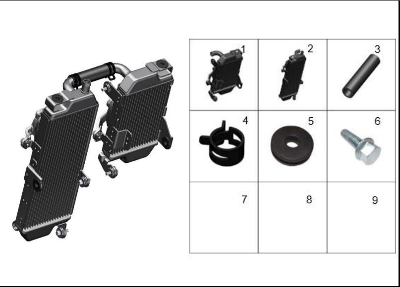
FIGURA 88: RADIADOR
