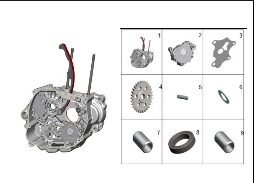
FIGURA 114: CARCASA DERECHA
