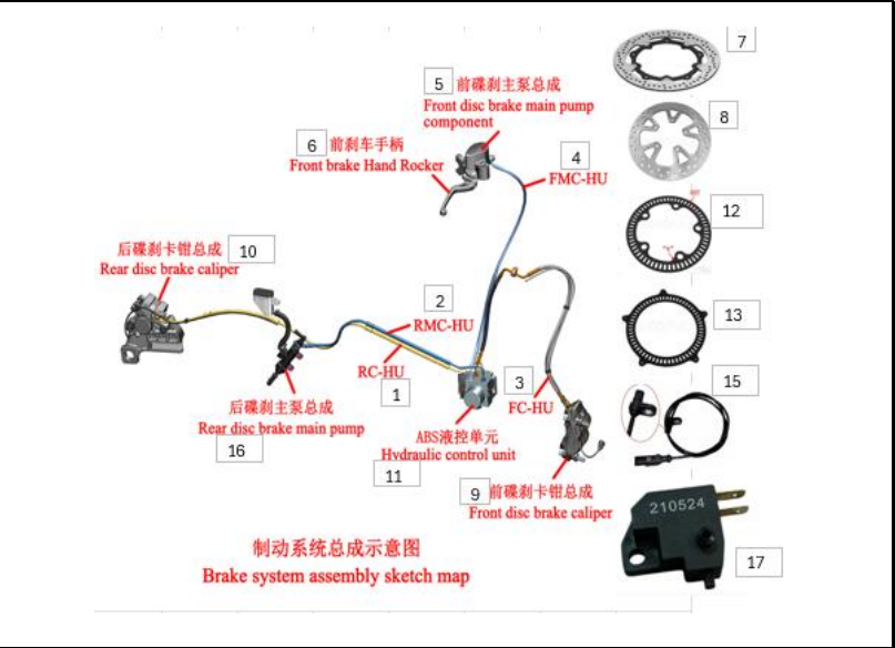
FIGURA 125: SISTEMA DE FRENOS
