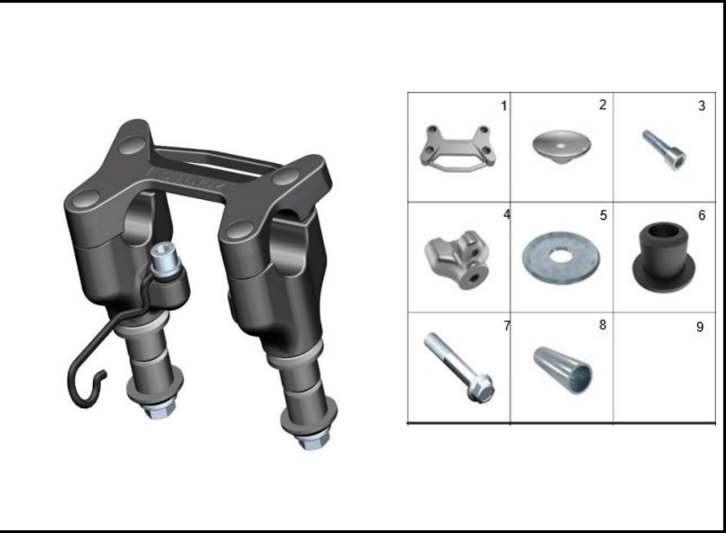
FIGURA 37: SOPORTE MANUBRIO
