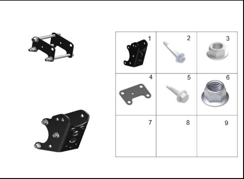
FIGURA 69: SOPORTE MOTOR
