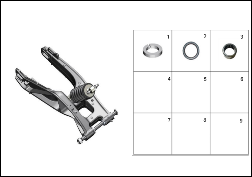
FIGURA 49: BRAZO OSCILANTE 2
