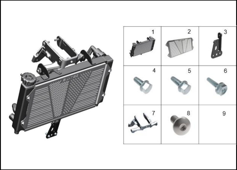
FIGURA 90: RADIADOR
