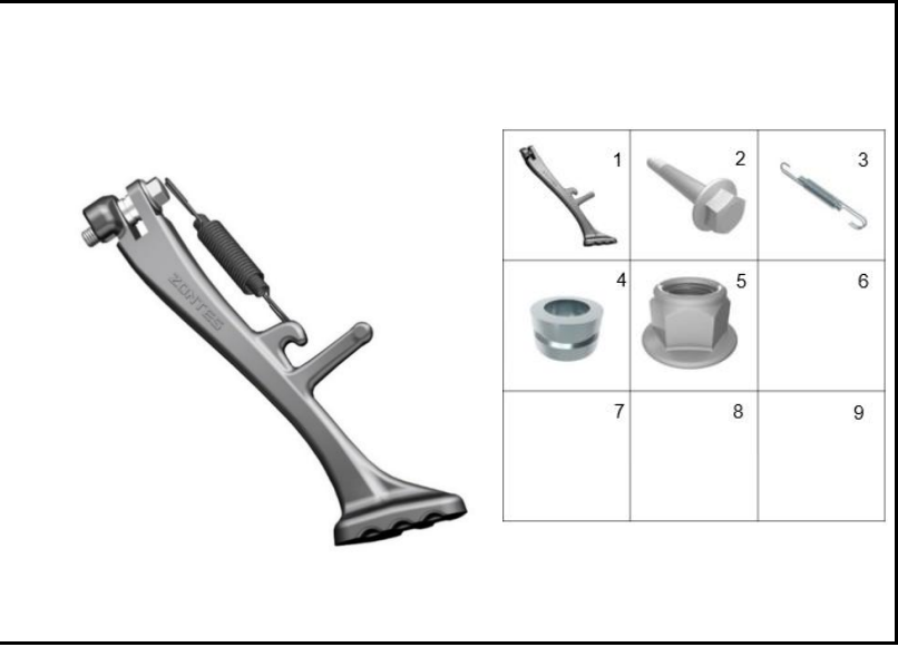
FIGURA 70: SOPORTE LATERAL
