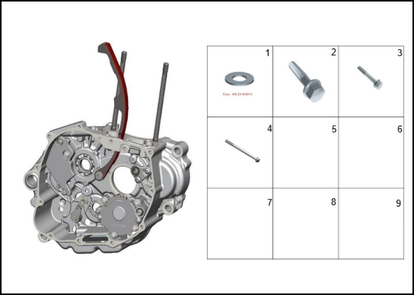
FIGURA 115: CARCASA DERECHA 2
