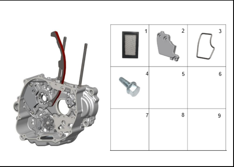
FIGURA 116: CARCASA DERECHA 4
