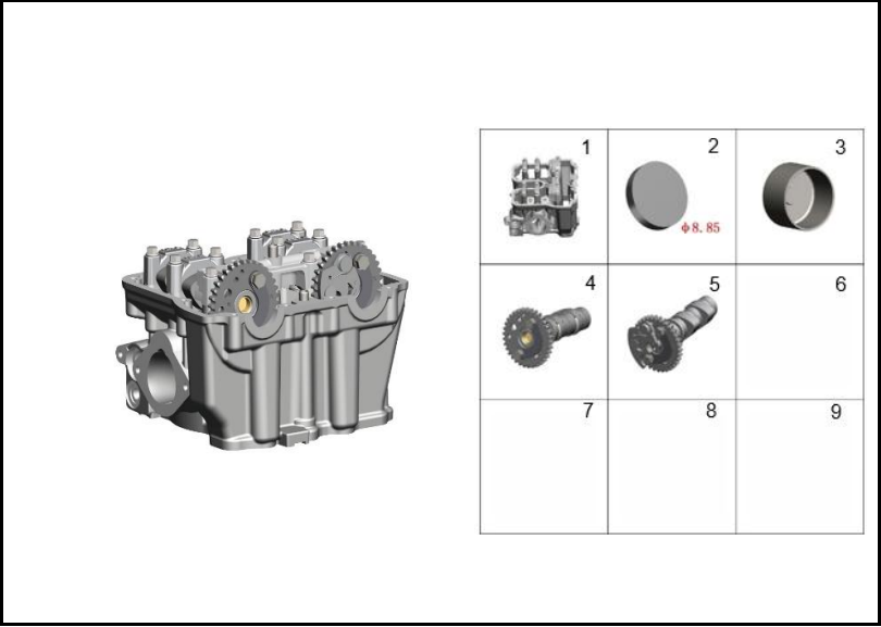
FIGURA 98: CULATA 3
