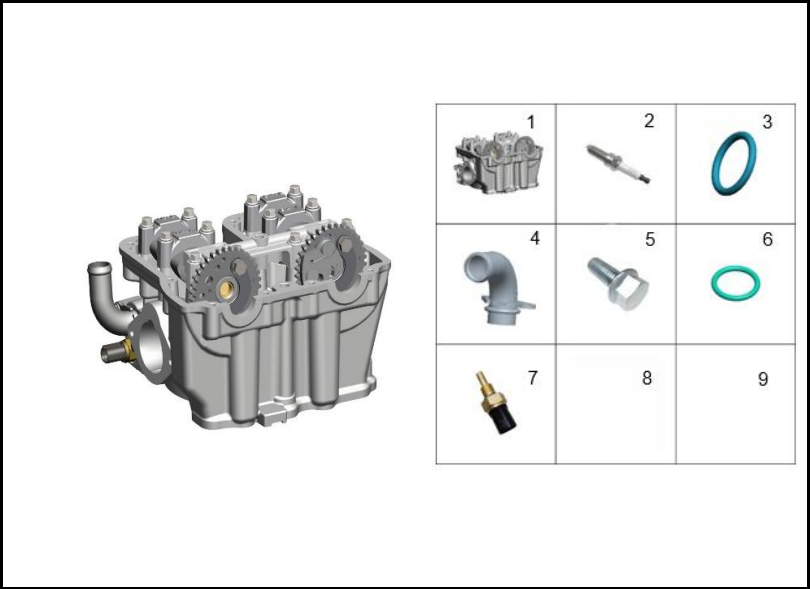
FIGURA 97: CULATA 2
