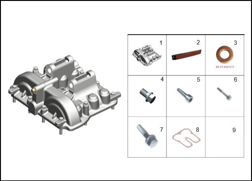
FIGURA 100: TAPA CULATA
