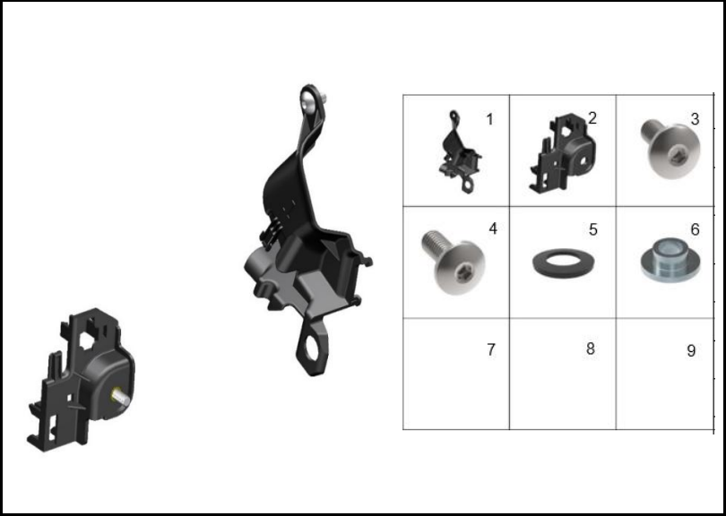
FIGURA 65: CUBIERTA Y SOPORTES
