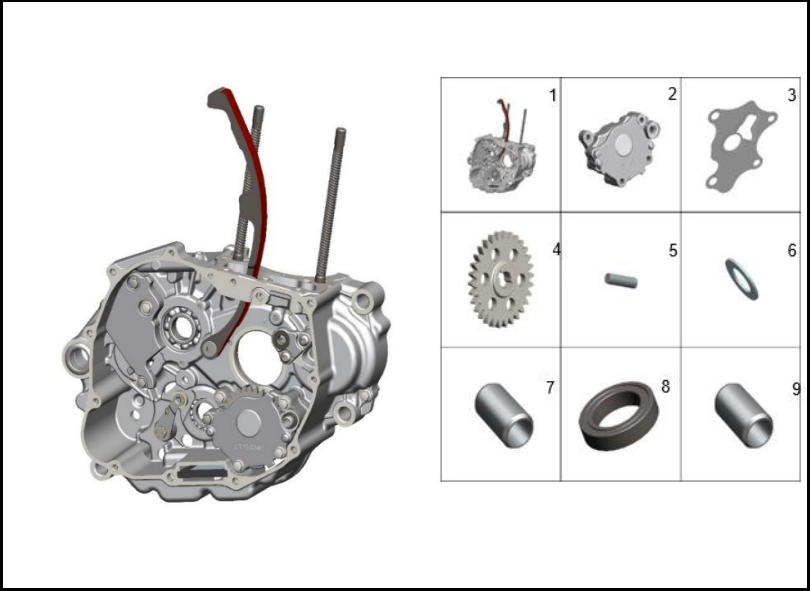
FIGURA 115: CARCASA DERECHA
