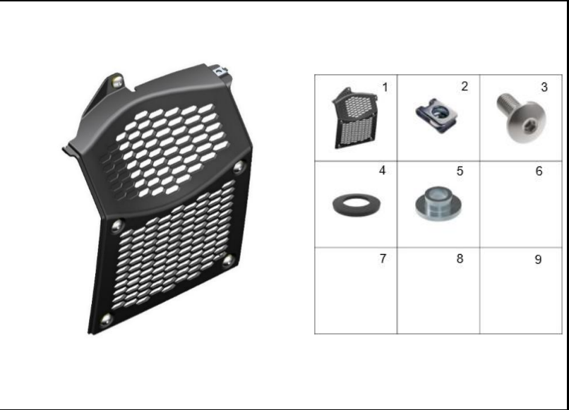
FIGURA 19: CUBIERTA MEDIA INFERIOR
