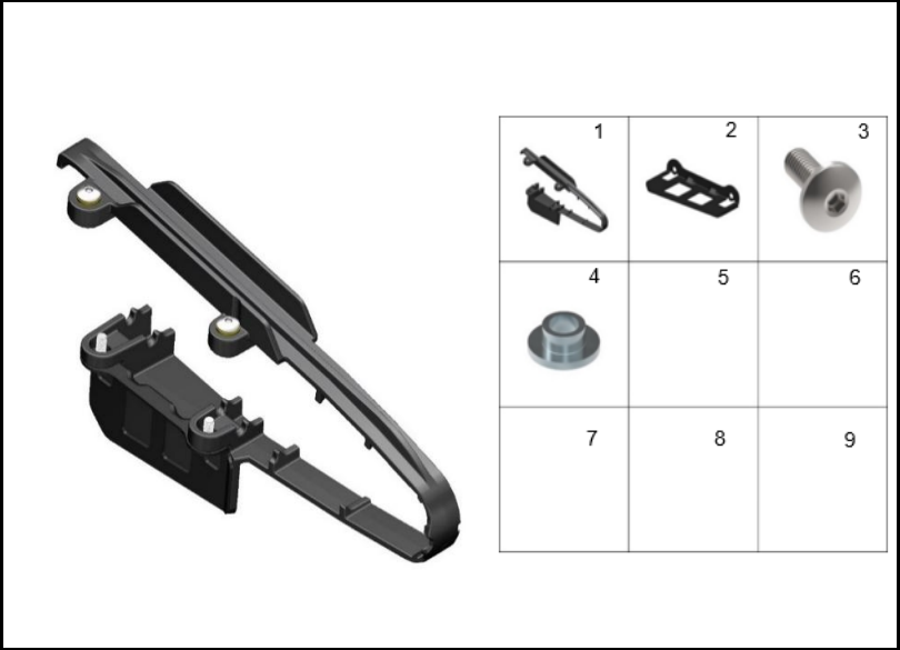
FIGURA 50: DESLIZADOR CADENA
