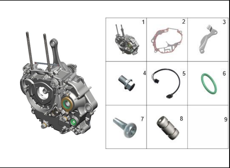
FIGURA 111: CARCASA IZQUIERDA
