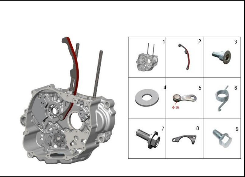
FIGURA 116: CARCASA DERECHA 3
