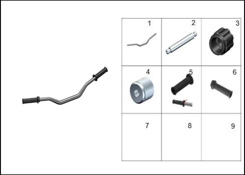
FIGURA 33: MANUBRIO
