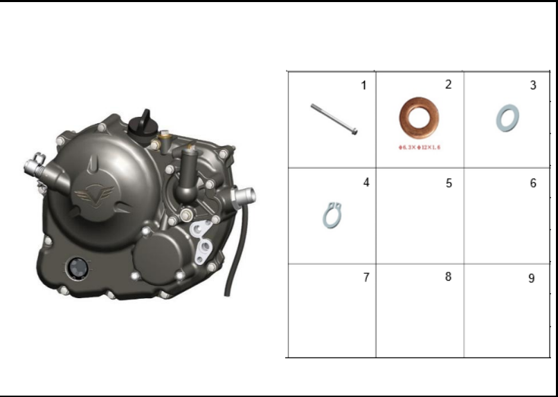
FIGURA 121: TAPA CARTER DERECHA 2
