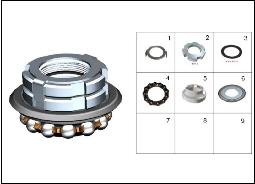
FIGURA 42: CUNAS DIRECCIÓN
