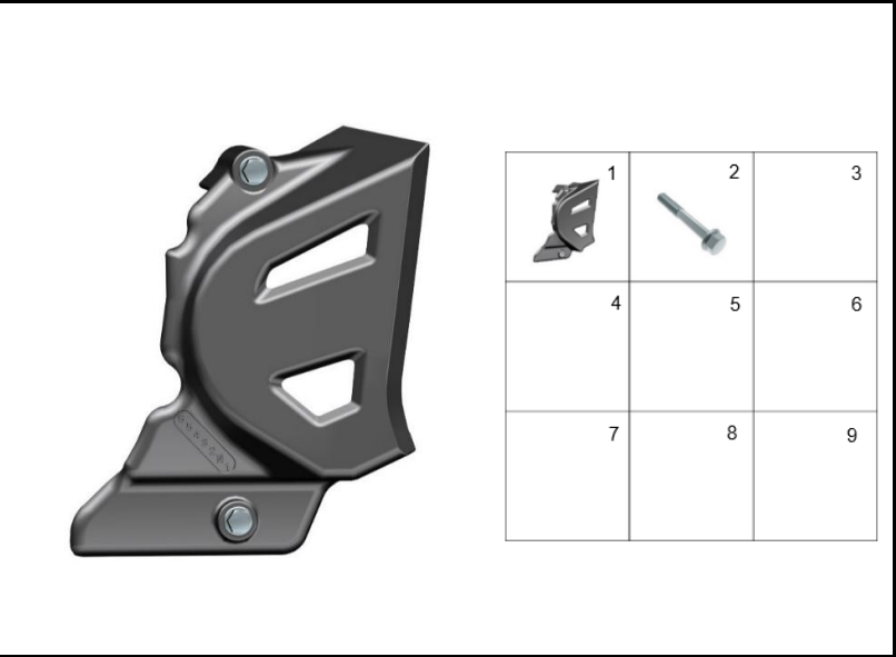
FIGURA 75: TAPA TRASERA IZQUIERDA MOTOR
