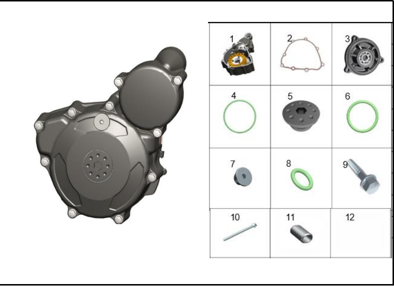
FIGURA 118: TAPA CÁRTER IZQ
