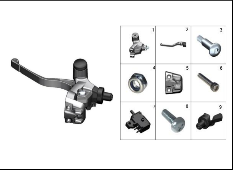
FIGURA 36: LEVA DE CLUTCH
