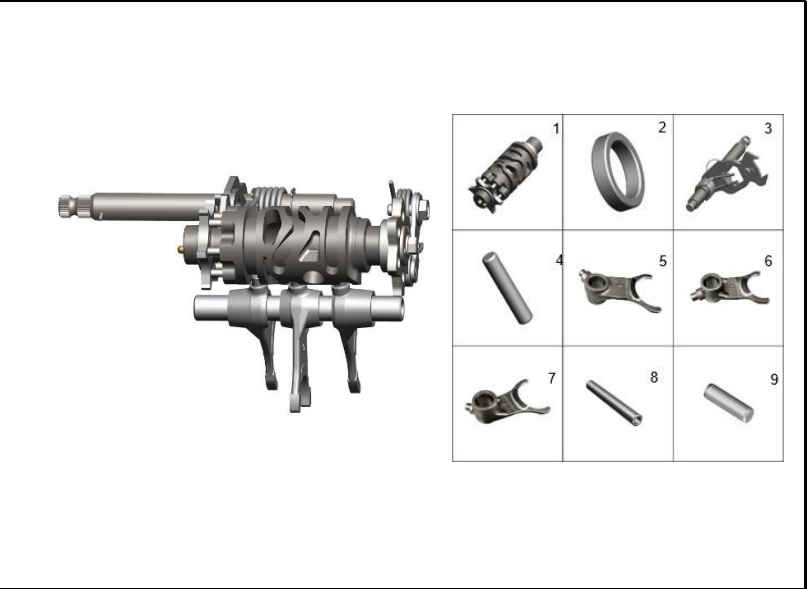
FIGURA 110: EJE DE CAMBIOS
