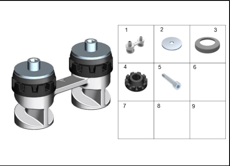
FIGURA 12: SOPORTE TANQUE DE COMBUSTIBLE
