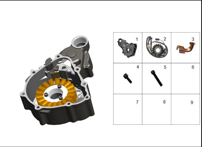
FIGURA 119: CUBIERTA CARCASA MOTOR IZQUIERDA
