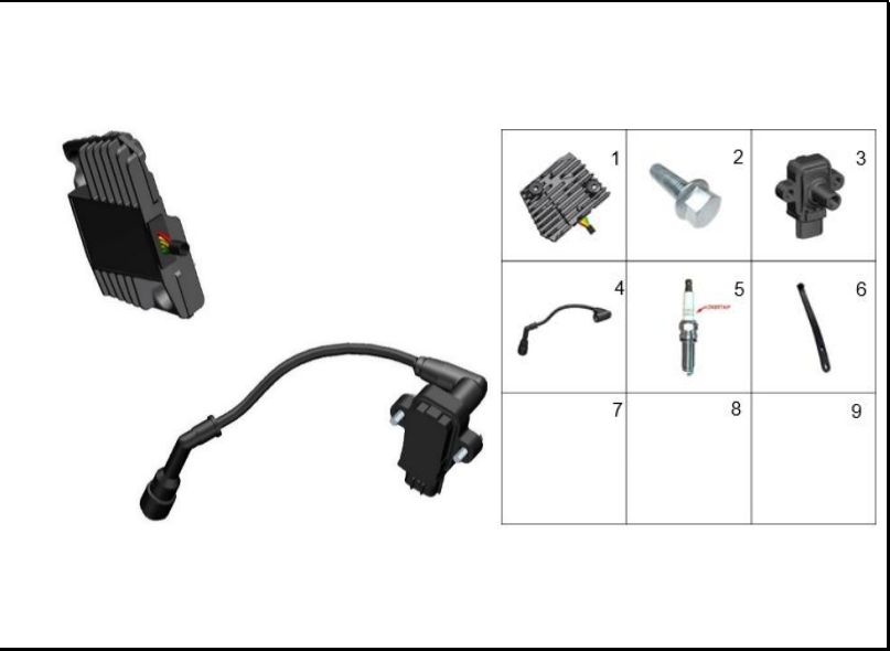
FIGURA 63: REGULADOR
