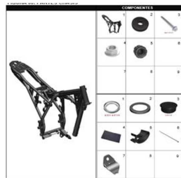
FIGURA N° 60: PA R T E S CHA S I S
