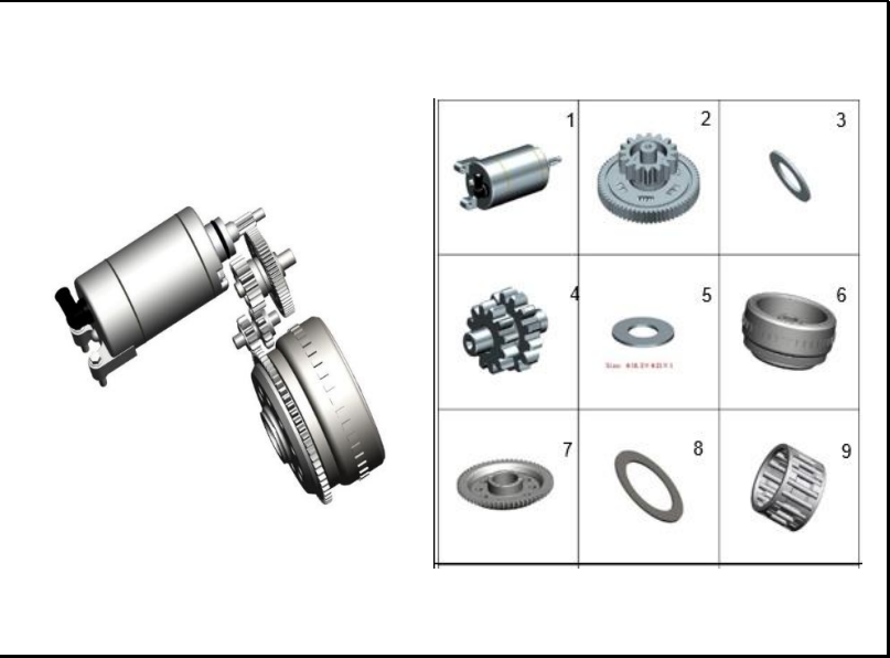
FIGURA 124: MOTOR DE ARRANQUE
