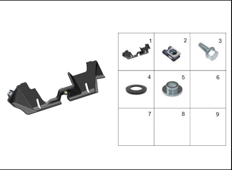
FIGURA 15: CUBIERTA INTERMEDIA TANQUE DE AGUA
