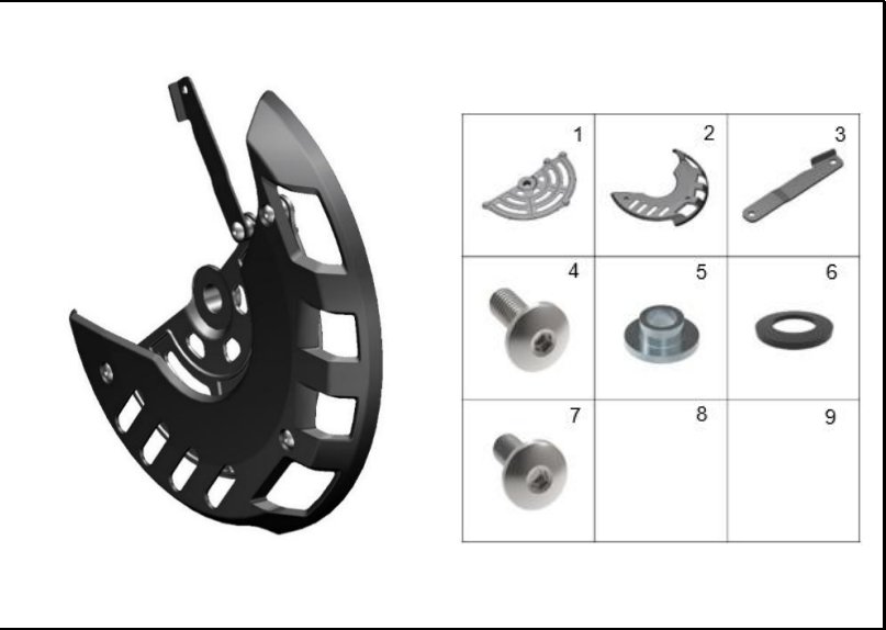
FIGURA 32: CUBIERTA DISCO FRENO DELANTERO
