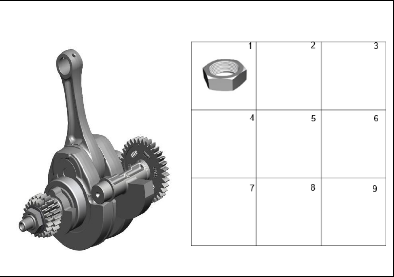
FIGURA 114: CIGÜEÑAL 2
