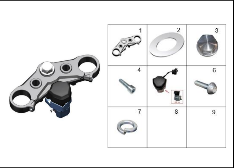
FIGURA 41: SOPORTE TUBOS SUSPENSIÓN DELANTERA
