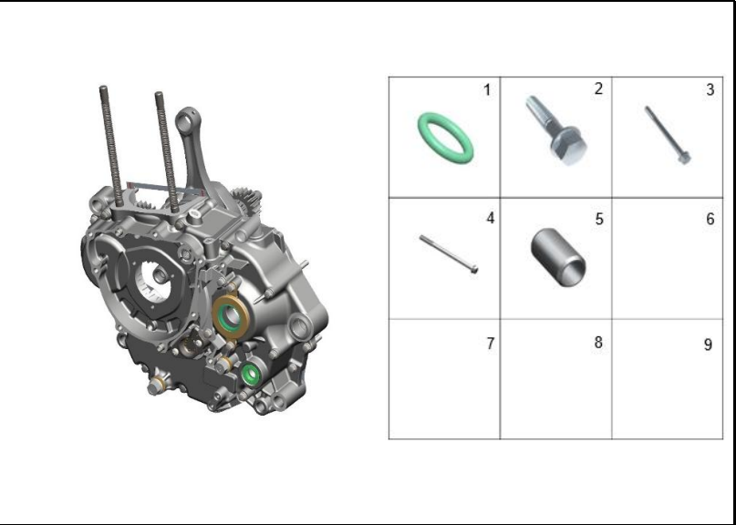
FIGURA 111: CARCASA IZQUIERDA 2
