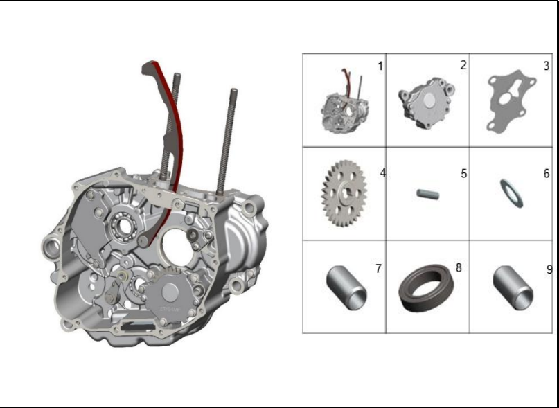
FIGURA 115: CARCASA DERECHA
