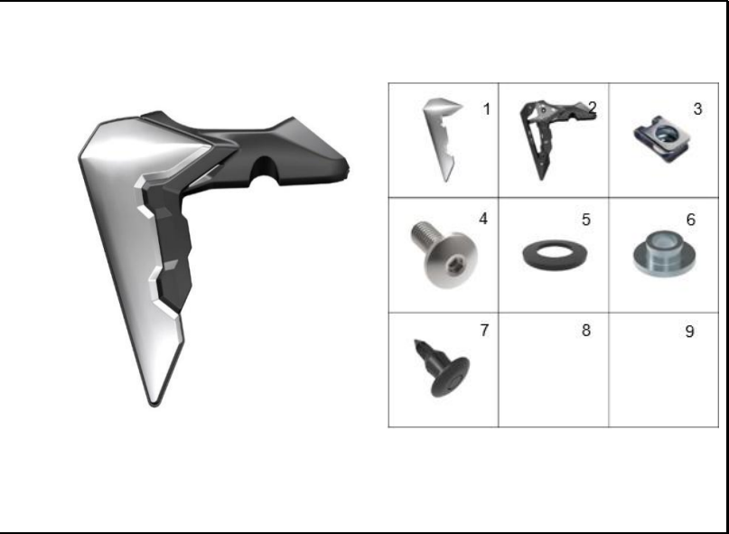
FIGURA 13: CUBIERTA INFERIOR IZQUIERDA TANQUE AGUA
