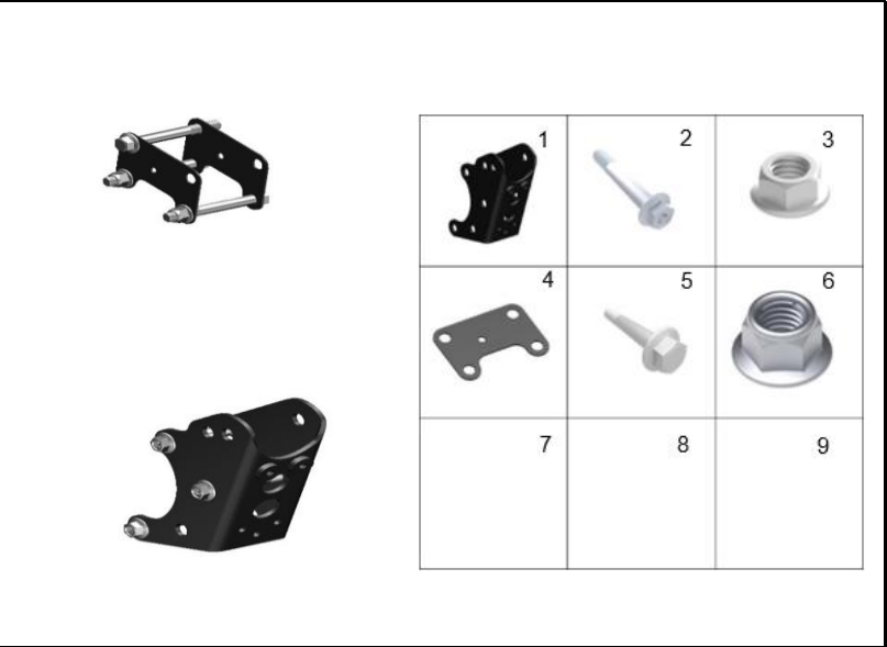
FIGURA 69: SOPORTE MOTOR
