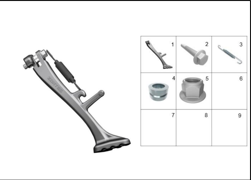
FIGURA 70: SOPORTE LATERAL
