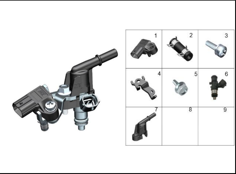
FIGURA 73: SOPORTE INYECTOR
