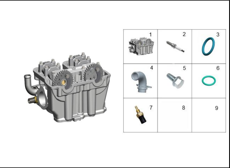
FIGURA 97: CULATA 2
