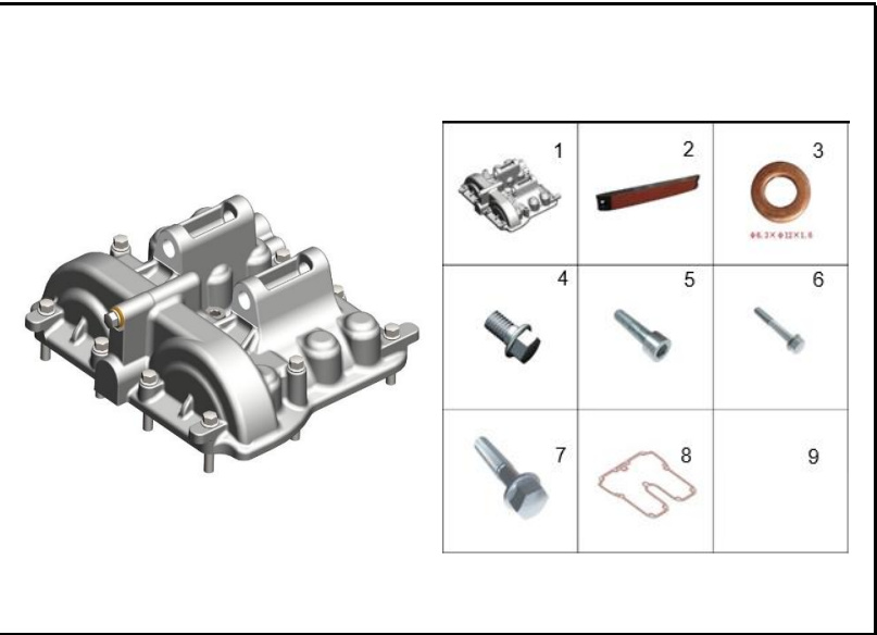
FIGURA 100: TAPA CULATA
