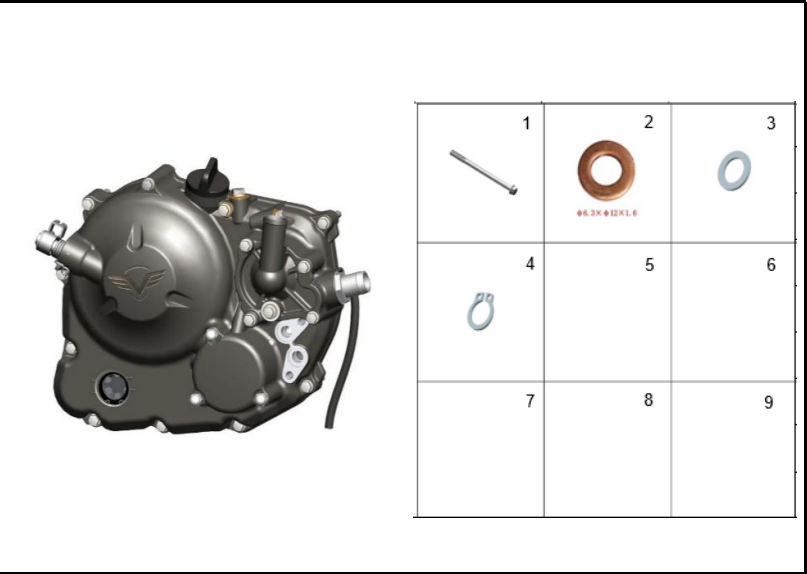
FIGURA 121: TAPA CARTER DERECHA 2
