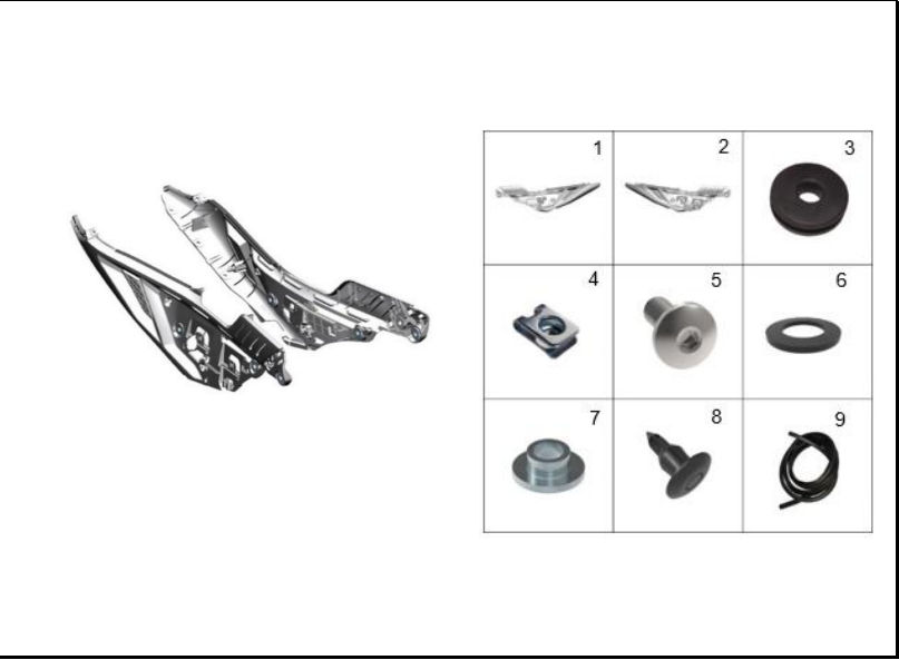
FIGURA 16: PLATINA IZQUIERDA CUBIERTA INFERIOR
