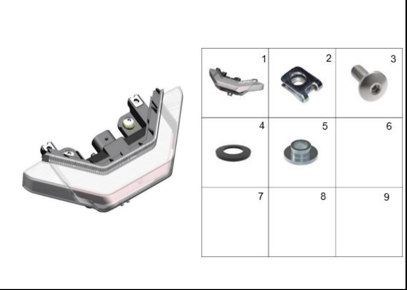
FIGURA 22: STOP TRASERO
