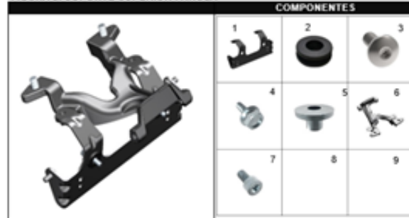
FIGURA 2: SOPORTE SUPERIOR FAROLA
