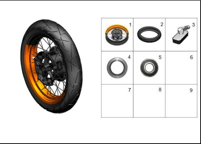
FIGURA 46: RUEDA DELANTERA – RIN NARANJA,NEGRO
