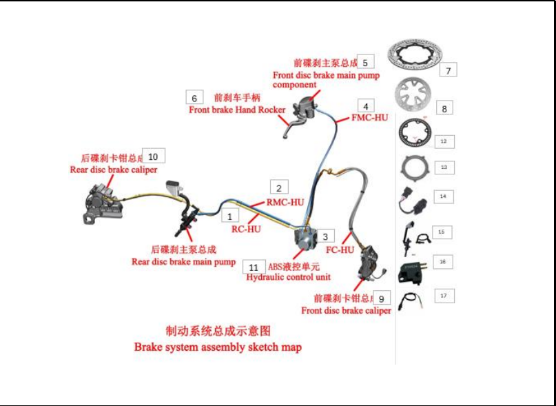
FIGURA 69A SISTEMA DE FRENOS
