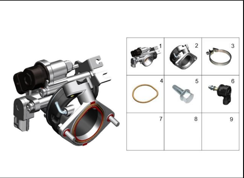
FIGURA 72: CUERPO DE INYECCIÓN
