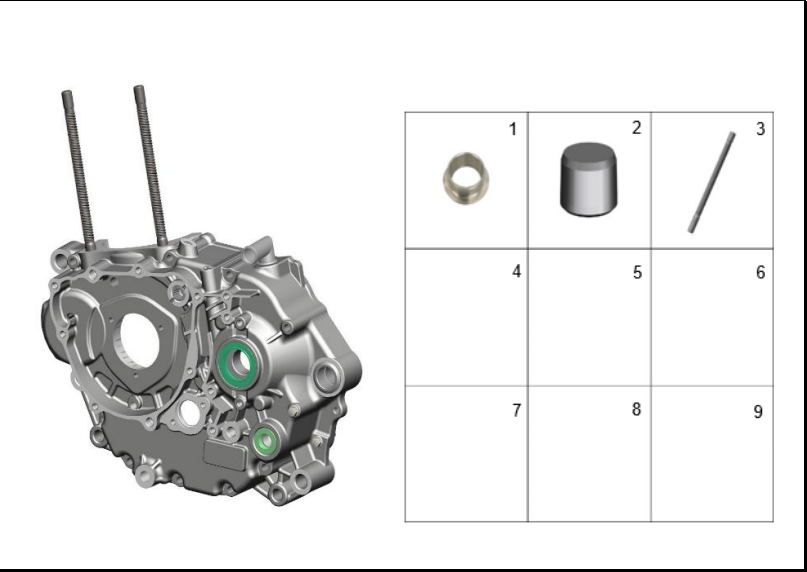
FIGURA 113: CARCASA IZQUIERDA 5
