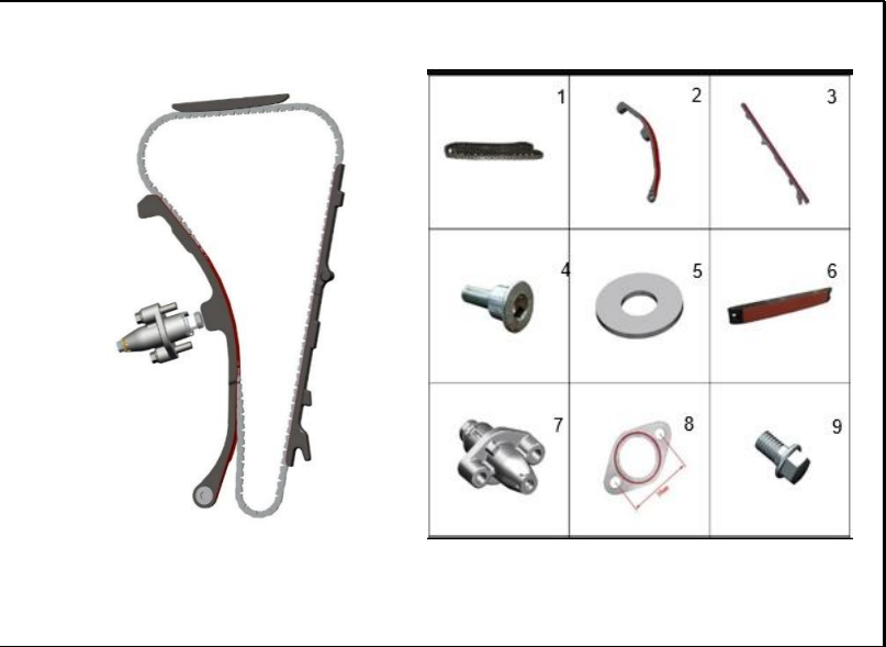
FIGURA 125: CADENILLA DE DISTRIBUCIÓN
