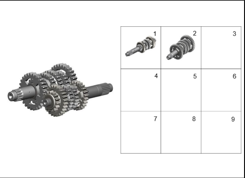
FIGURA 108: TRANSMISIÓN
