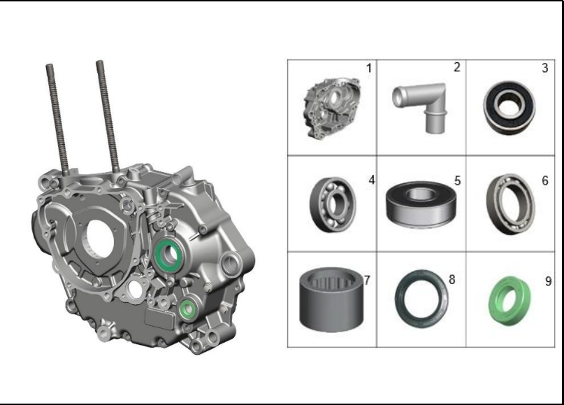
FIGURA 113: CARCASA IZQUIERDA 4
