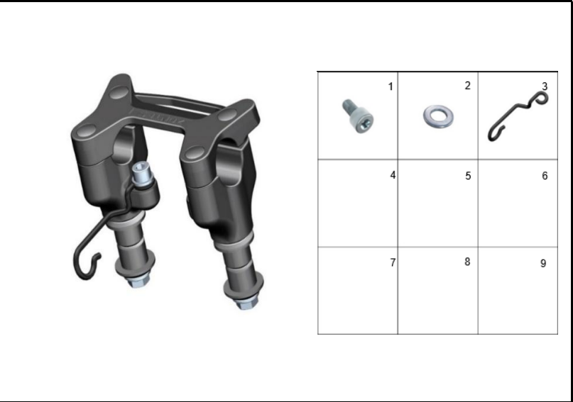
FIGURA 37: SOPORTE MANUBRIO 2
