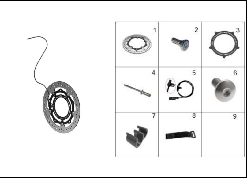
FIGURA 48: RUEDA FONICA RUEDA DELANTERA
