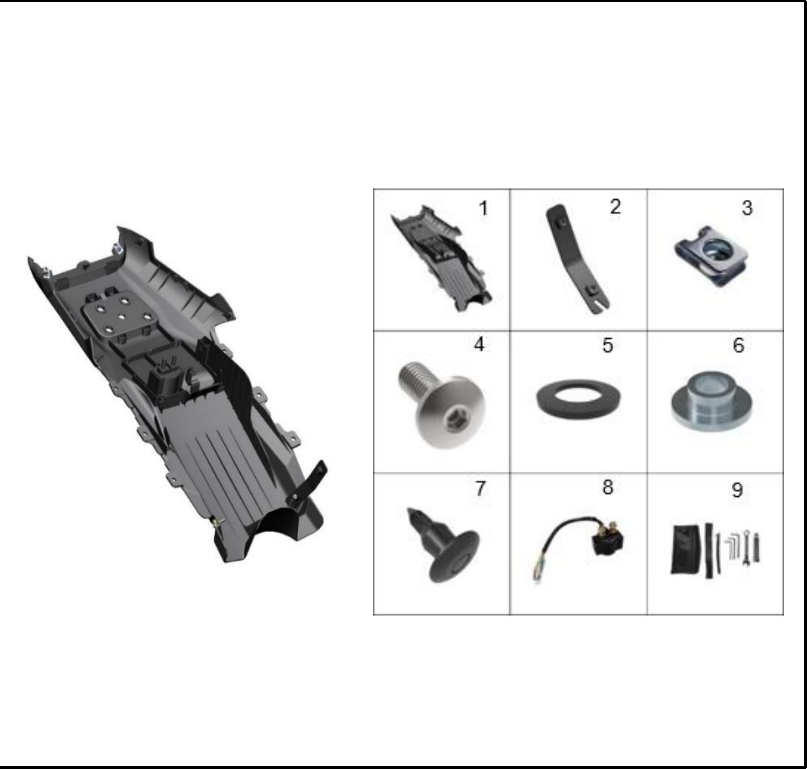
FIGURA 23: GUARDABARRO TRASERO
