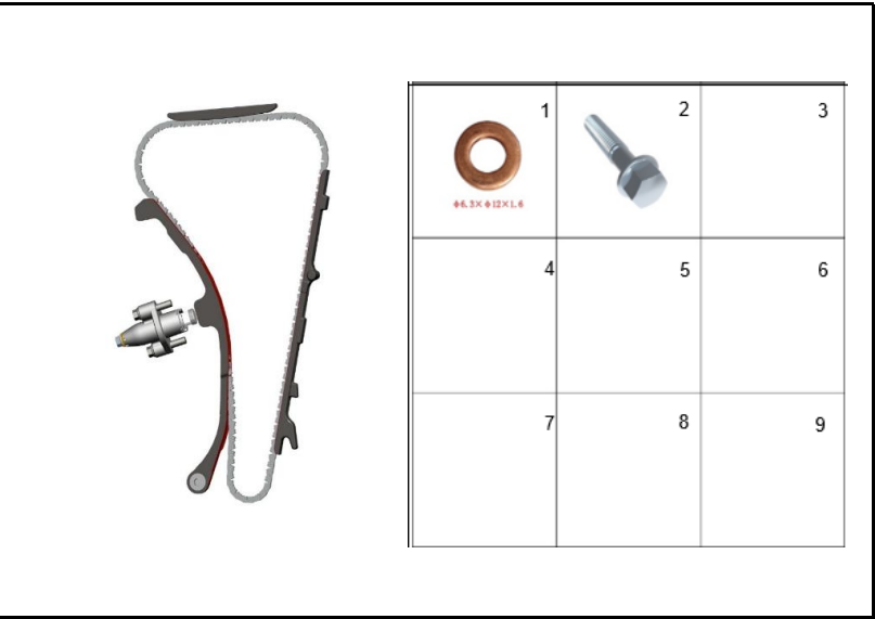
FIGURA 125: CADENILLA DE DISTRIBUCIÓN 2
