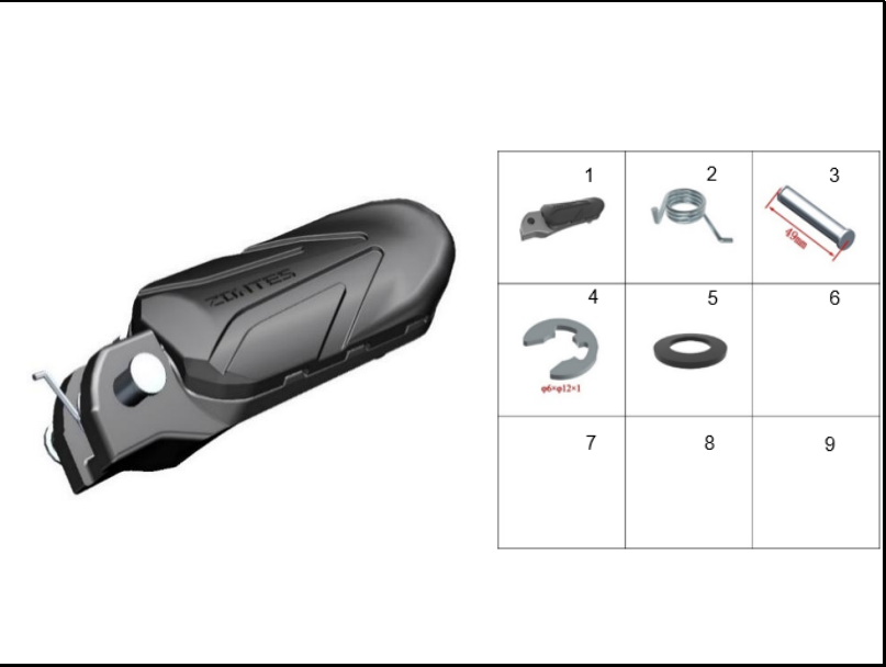
FIGURA 79: REPOSAPIE DELANTERO IZQUIERDO
