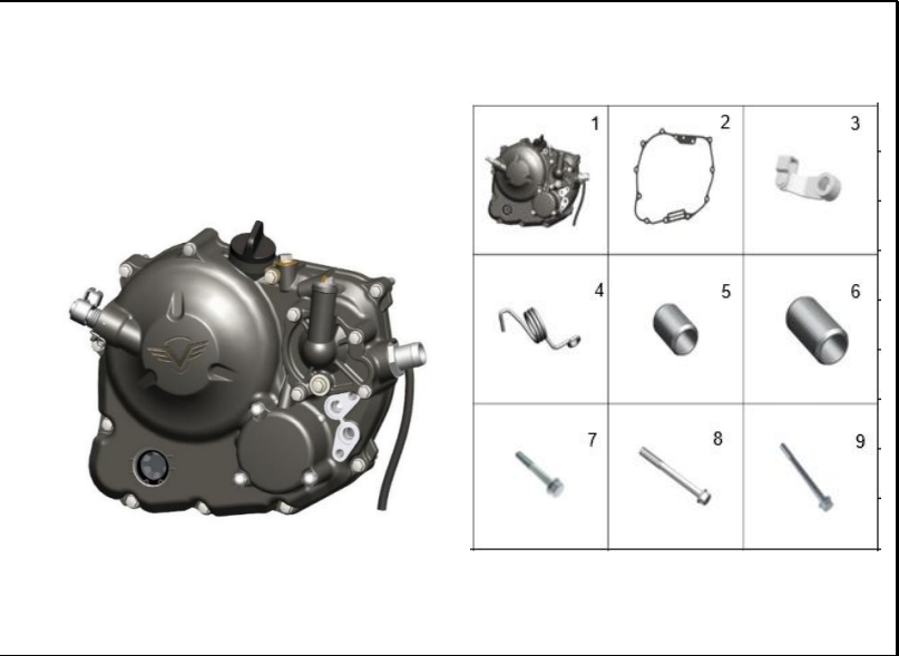
FIGURA 121: TAPA CARTER DERECHA
