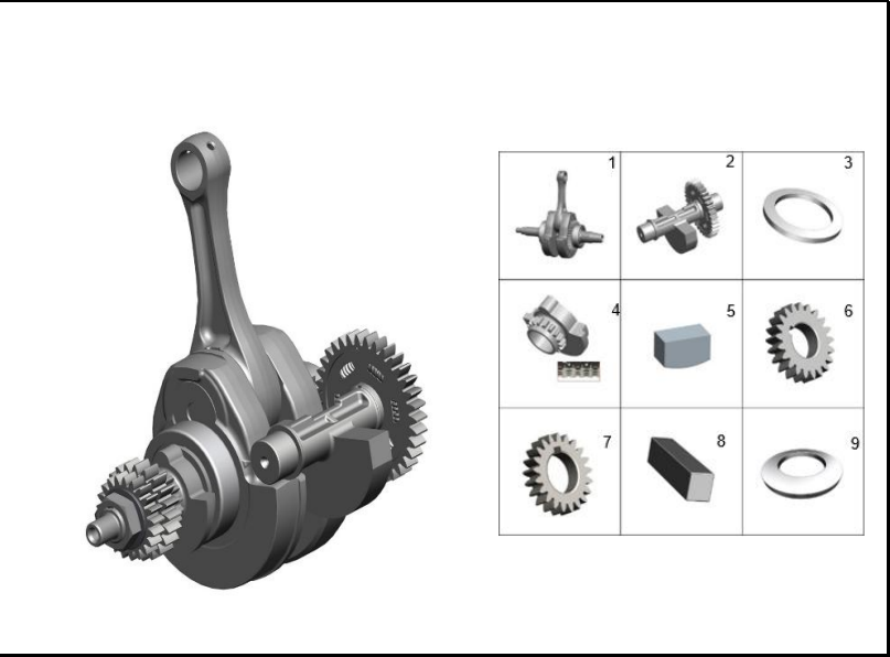
FIGURA 114: CIGÜEÑAL
