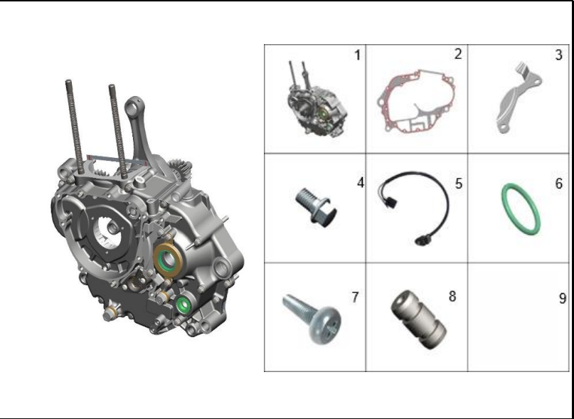
FIGURA 111: CARCASA IZQUIERDA
