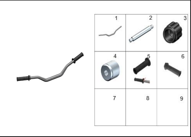
FIGURA 33: MANUBRIO
