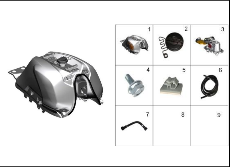
FIGURA 9: TANQUE DE COMBUSTIBLE
