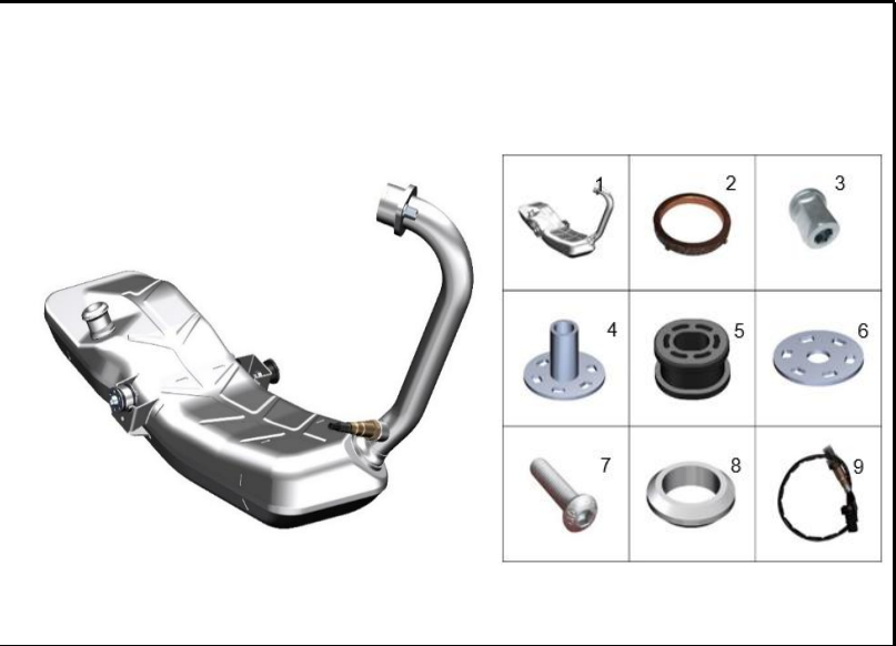
FIGURA 76: SILENCIADOR
