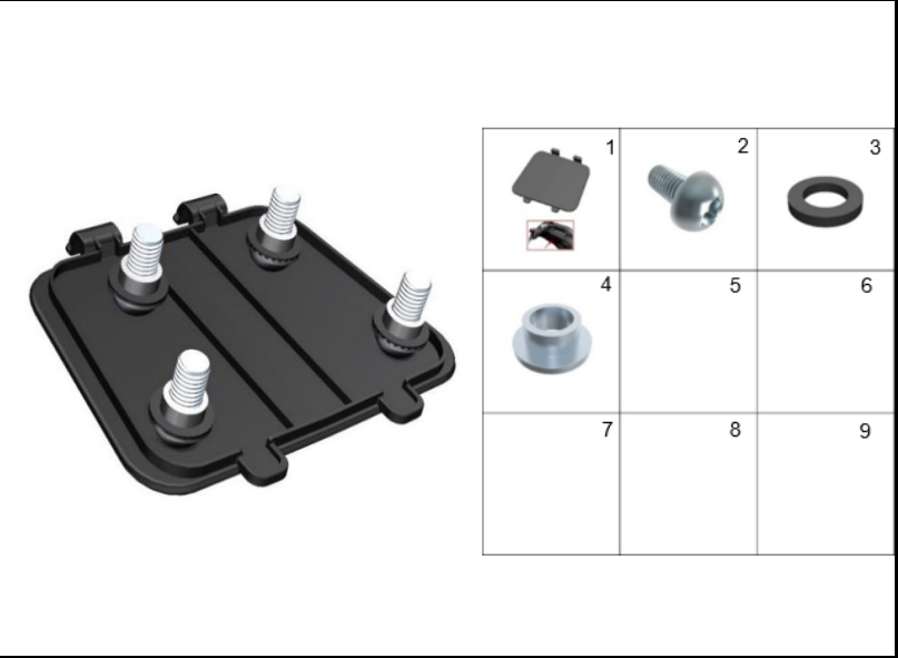
FIGURA 27: TAPA CUBIERTA TRASERA
