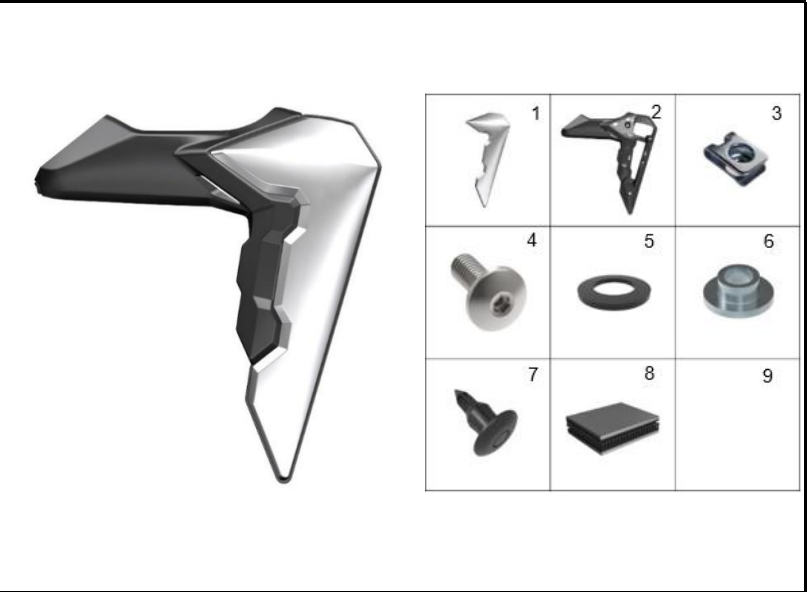
FIGURA 14: CUBIERTA INFERIOR DERECHA TANQUE AGUA
