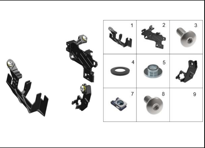
FIGURA 66: SOPORTES
