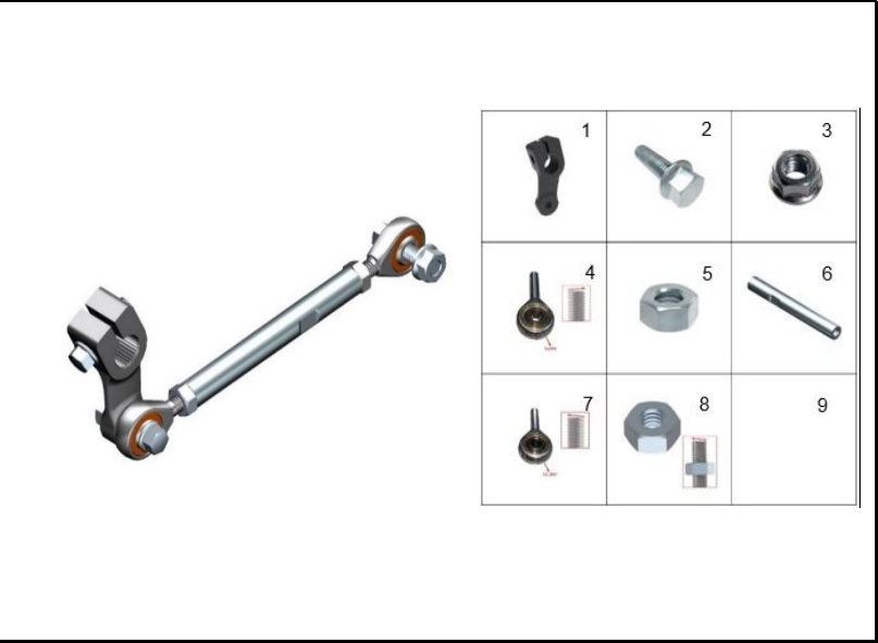
FIGURA 81: MUÑON PEDAL DE CAMBIOS
