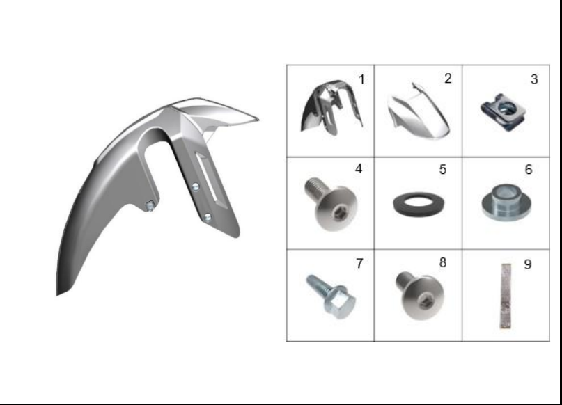
FIGURA 8: GUARDABARRO DELANTERO
