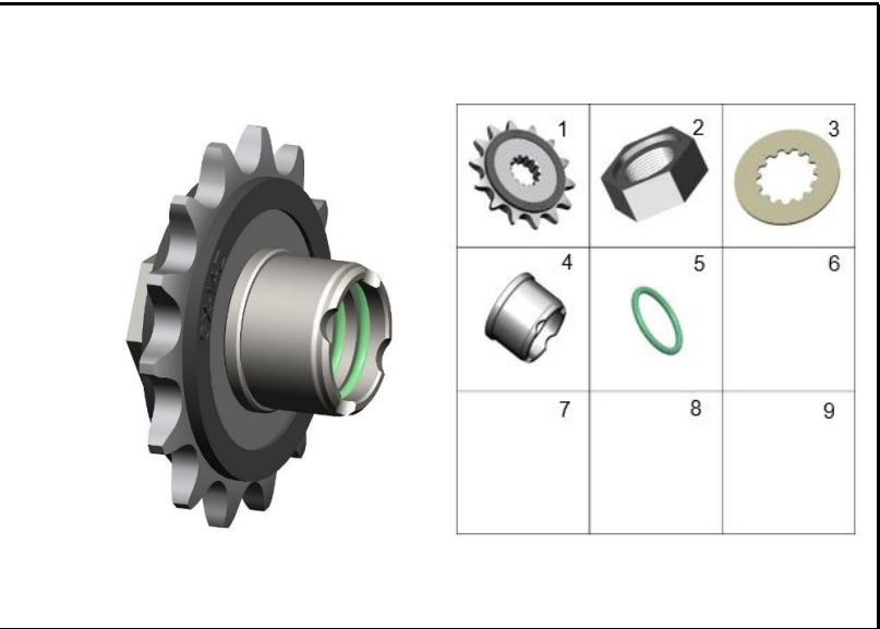
FIGURA 109: PIÑÓN DE SALIDA
