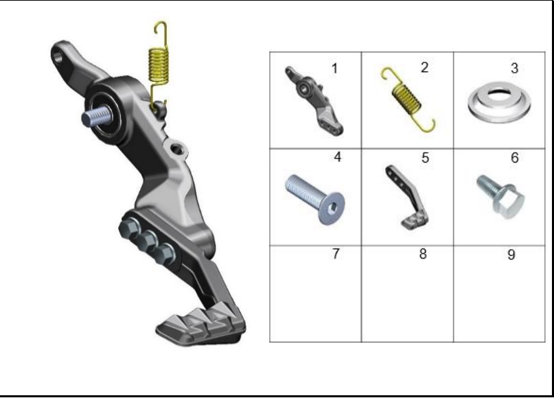
FIGURA 86: PEDAL DE FRENO
