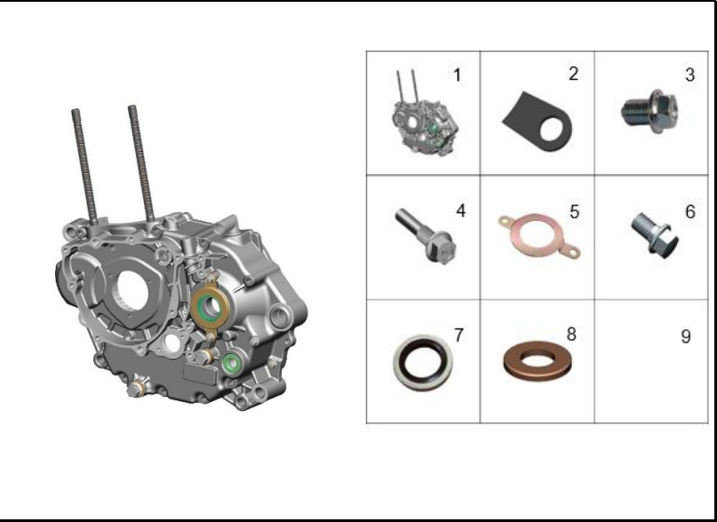
FIGURA 112: CARCASA IZQUIERDA 3
