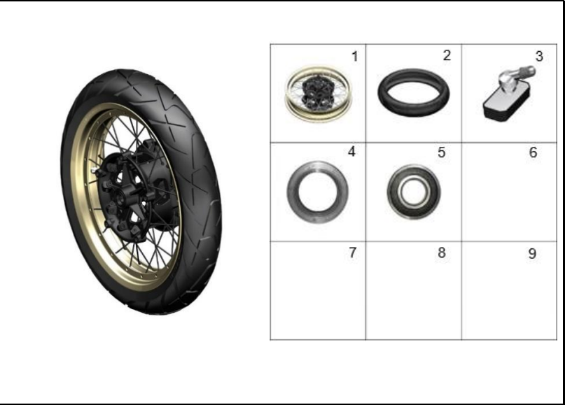
FIGURA 47: RUEDA DELANTERA – RIN DORADO
