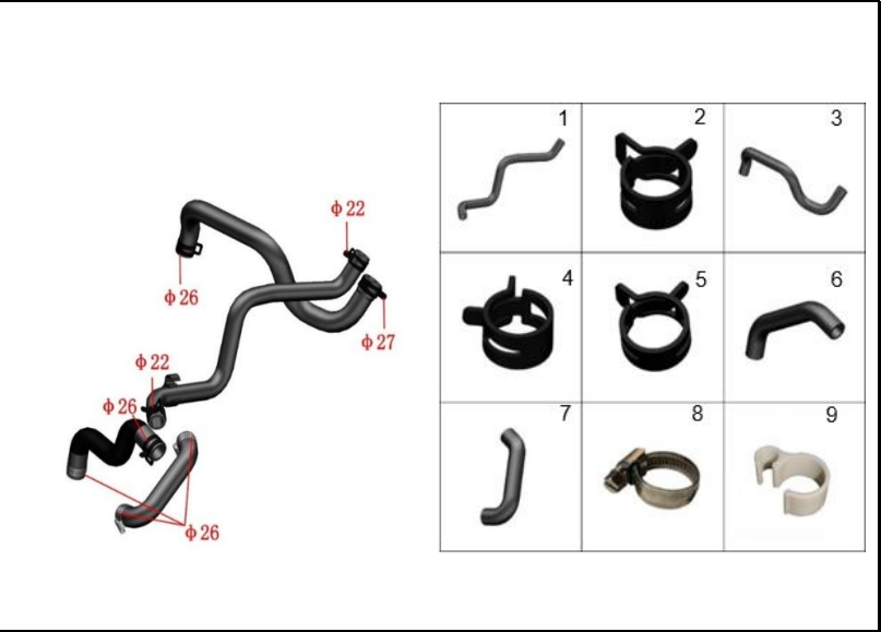
FIGURA 91: MANGUERAS DE DESFOGUE
