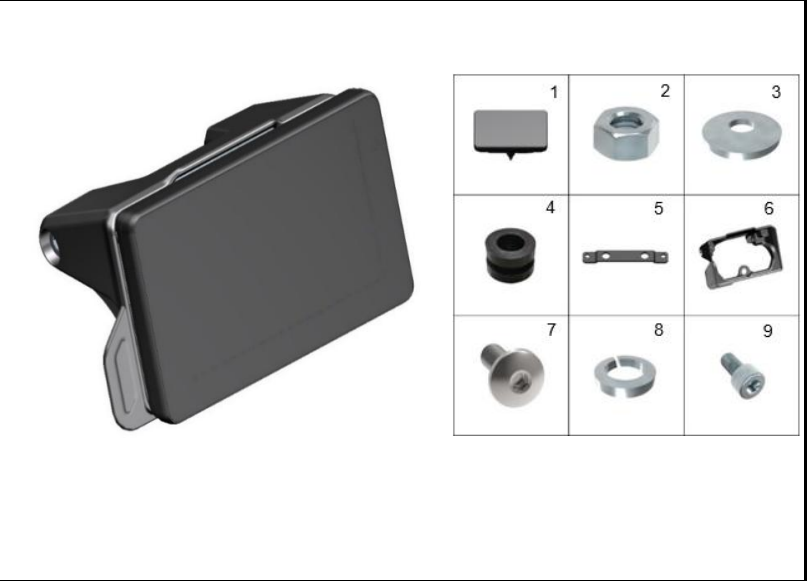
FIGURA 1: VELOCIMETRO
