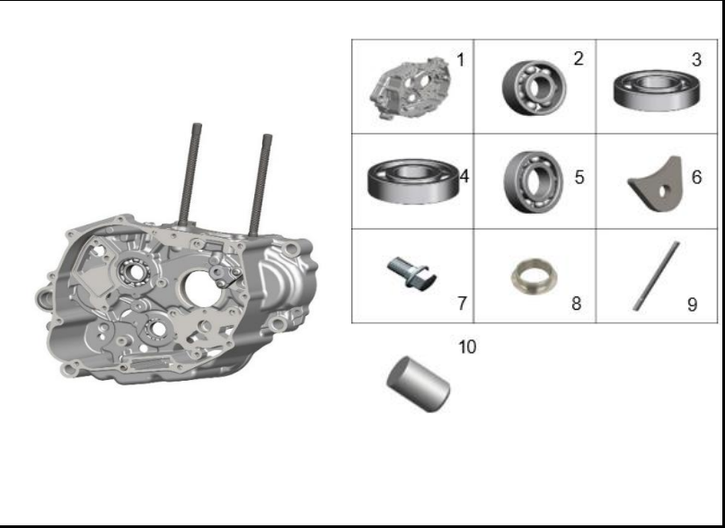
FIGURA 117: CARCASA DERECHA 5
