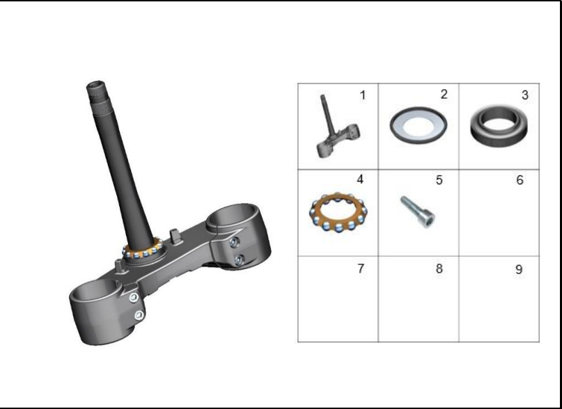
FIGURA 43: HORQUILLA DIRECCIÓN
