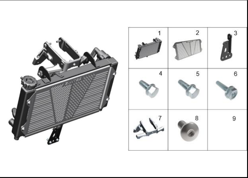
FIGURA 90: RADIADOR
