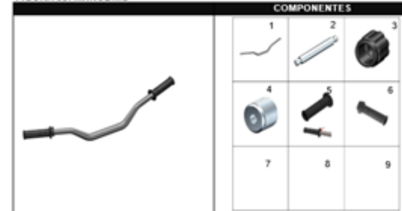
FIGURA 33: MANUBRIO
