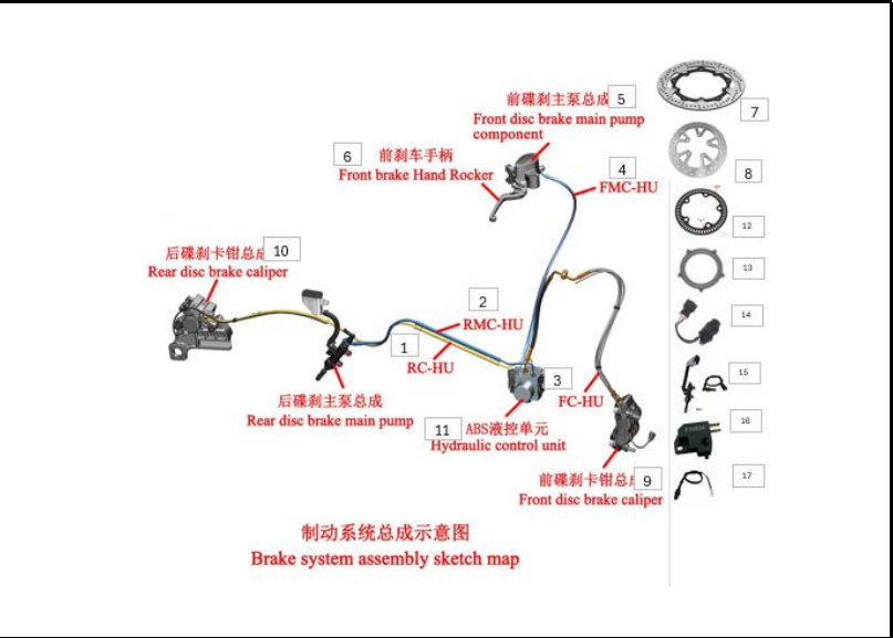
FIGURA 69A SISTEMA DE FRENOS 2
