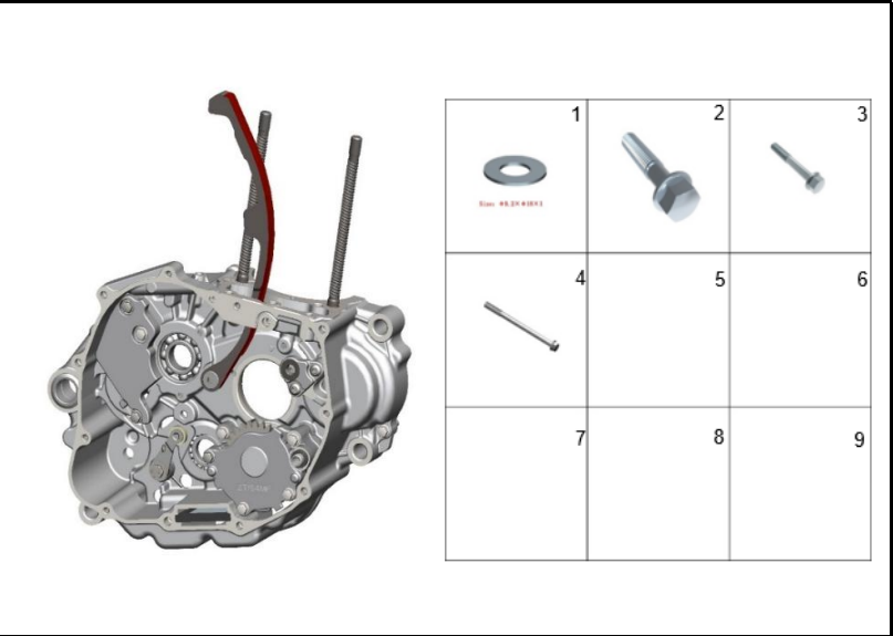
FIGURA 115: CARCASA DERECHA 2
