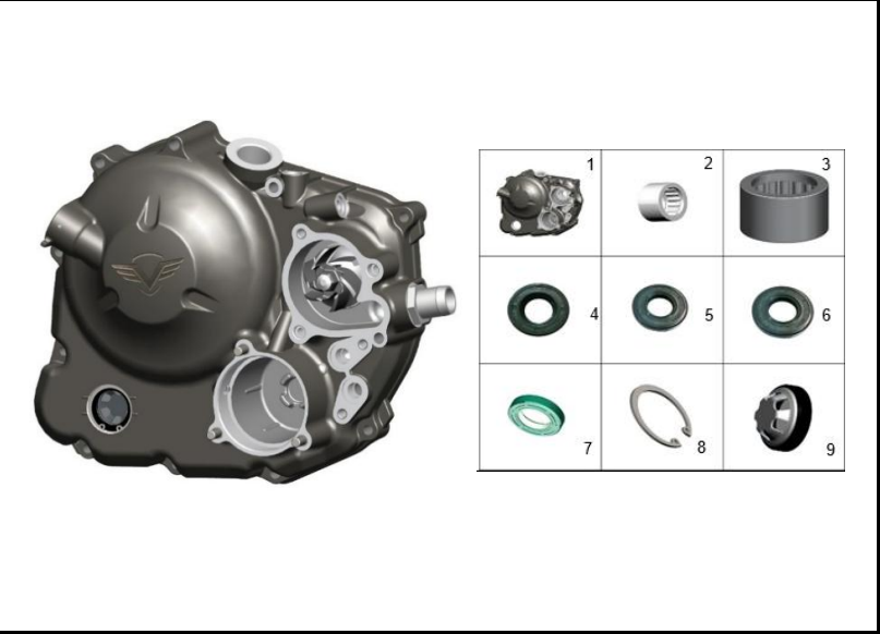
FIGURA 123: CUBIERTA CARCASA MOTOR DERECHA
