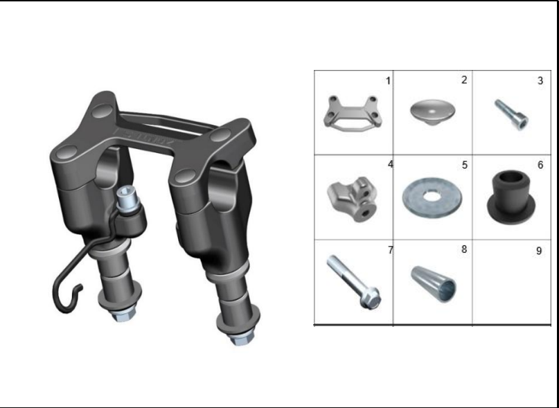
FIGURA 37: SOPORTE MANUBRIO
