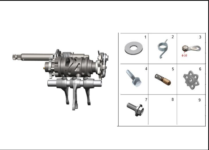
FIGURA 110: EJE DE CAMBIOS 2
