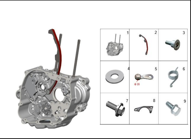
FIGURA 116: CARCASA DERECHA 3
