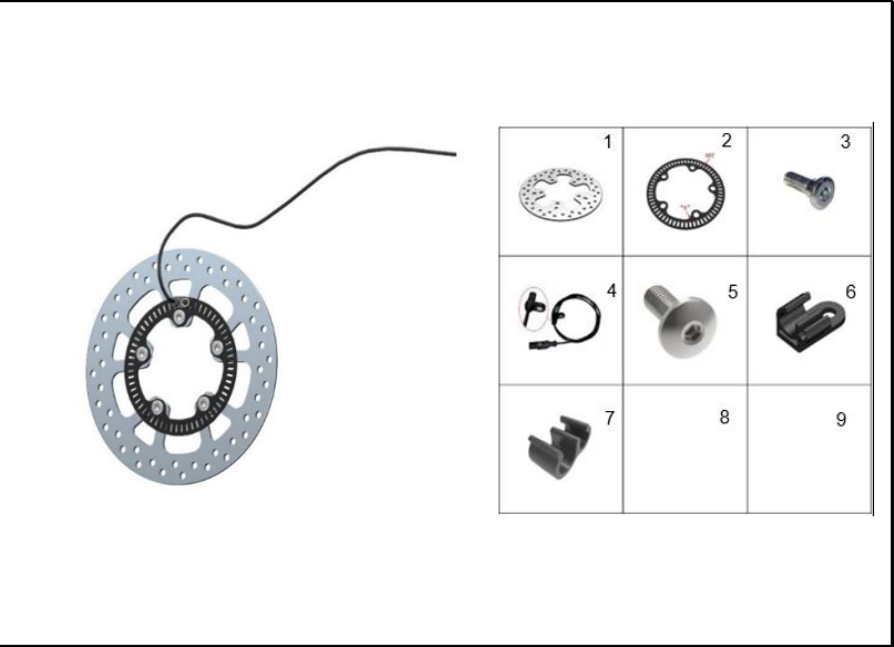
FIGURA 58: RUEDA FÓNICA ABS
