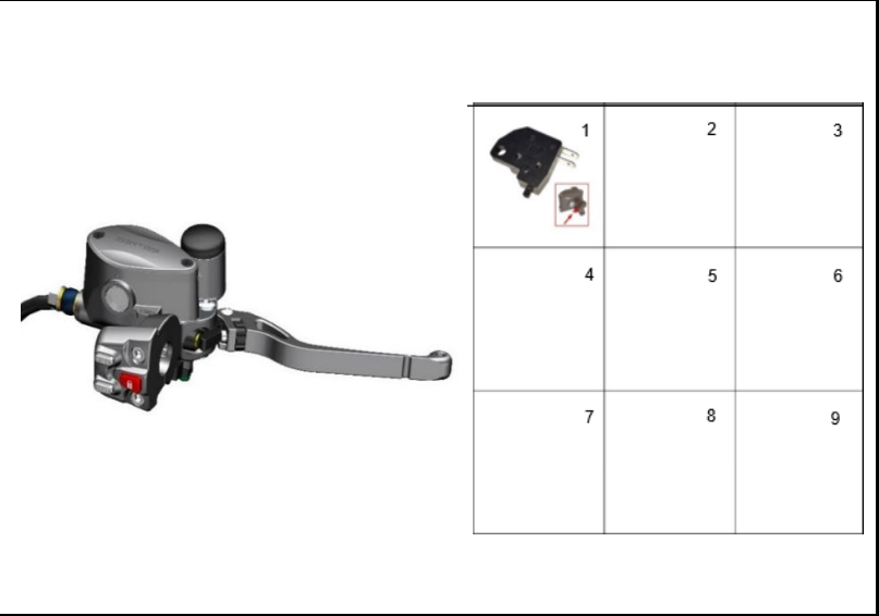
FIGURA 38: LEVA DE FRENO 2
