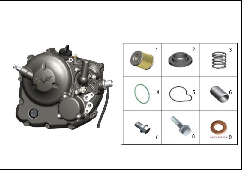
FIGURA 122: TAPA CARTER DERECHA 4
