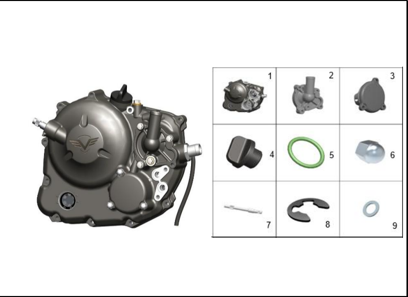
FIGURA 122: TAPA CARTER DERECHA 3
