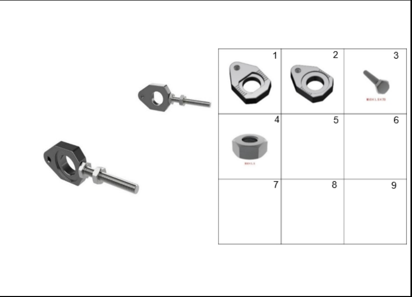
FIGURA 52: TENSORES DE CADENA
