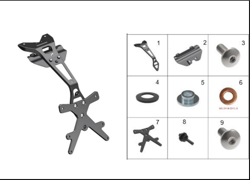
FIGURA 30: SOPORTE GUARDABARRO TRASERO
