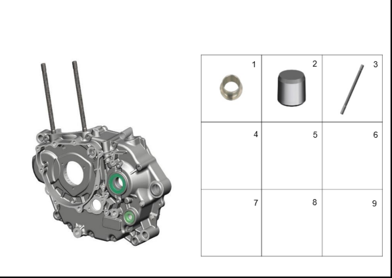
FIGURA 116: CARCASA IZQUIERDA 5
