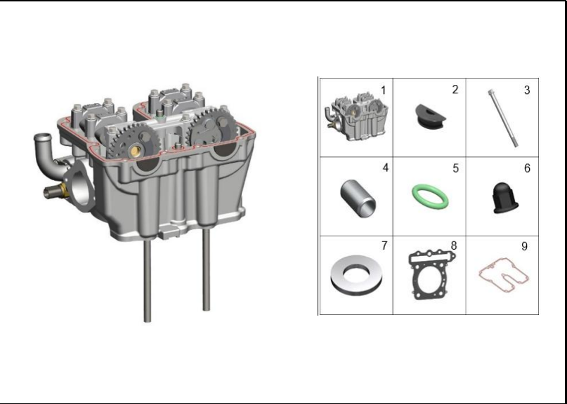
FIGURA 99: CULATA
