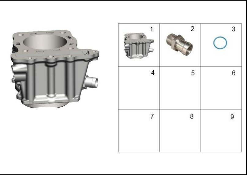
FIGURA 106: CILINDRO SOLO
