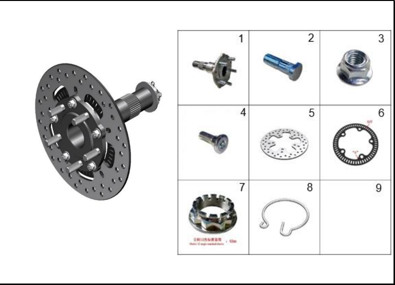
FIGURA 62: EJE TRASERO
