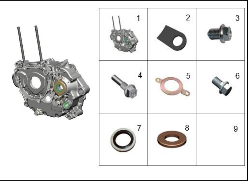
FIGURA 115: CARCASA IZQUIERDA 3
