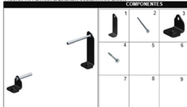
FIGURA 14: PLATINA IZQUIERDA CUBIERTA INFERIOR
