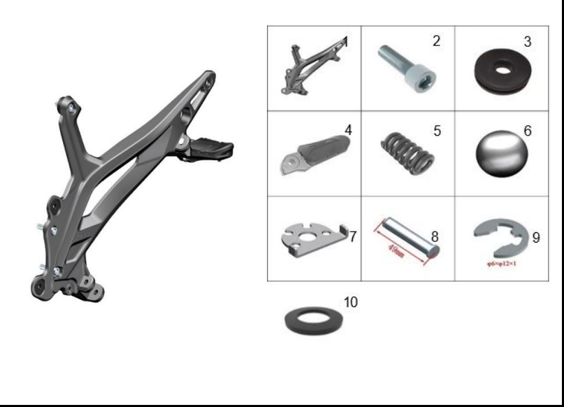
FIGURA 80: SOPORTE REPOSAPIES IZQUIERDO
