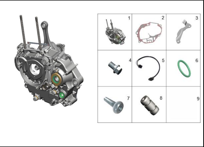
FIGURA 114: CARCASA IZQUIERDA
