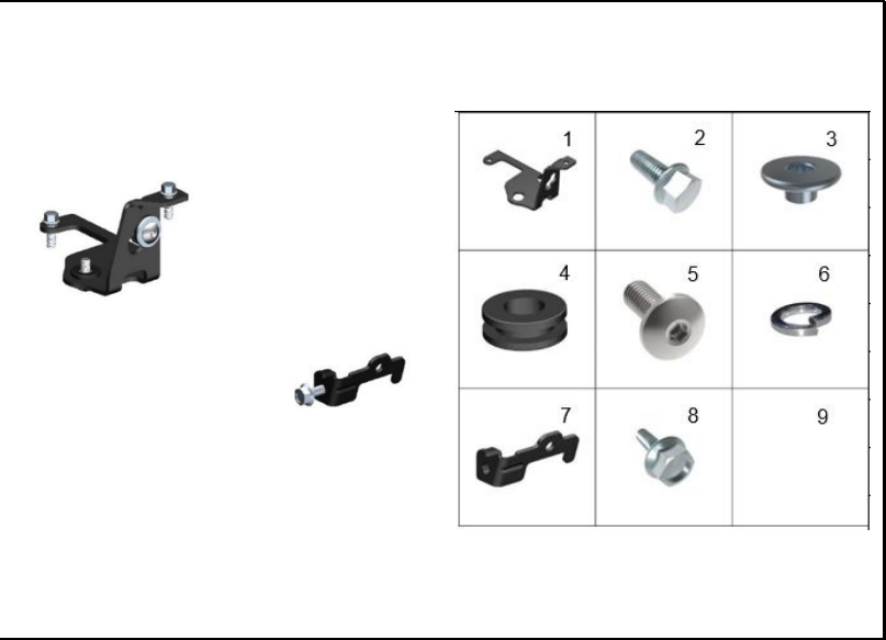
FIGURA 42: SOPORTE MODULO ABS
