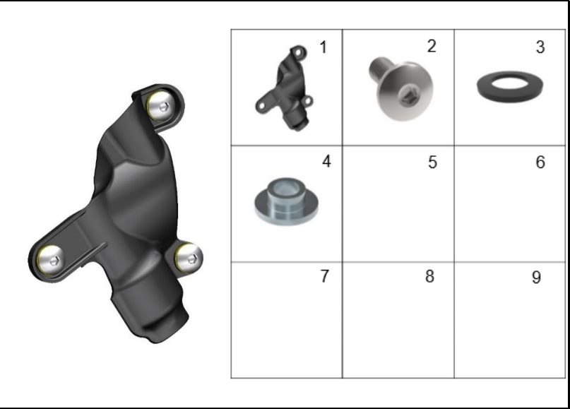
FIGURA 89: CUBIERTA BOMBA DE FRENO TRASERO
