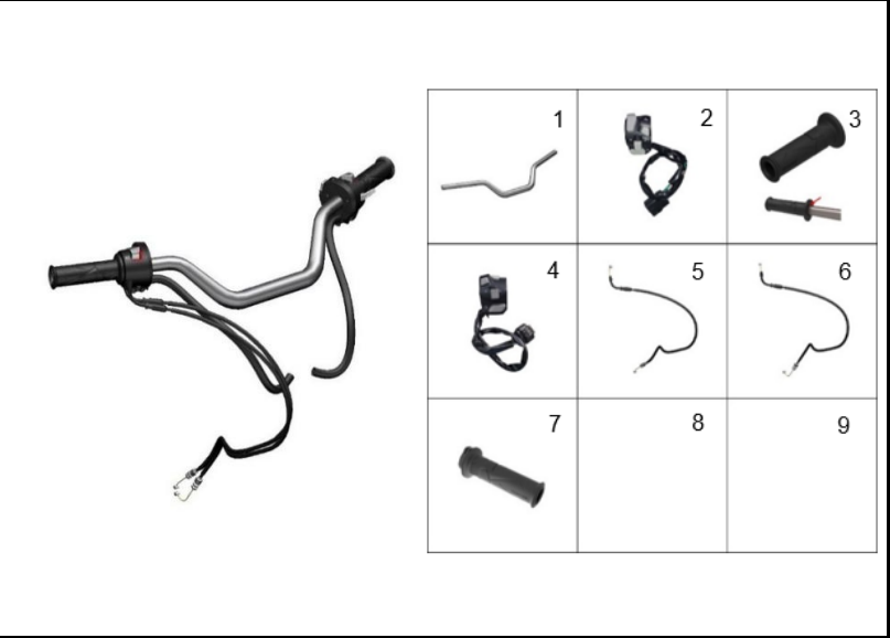
FIGURA 37: MANUBRIO
