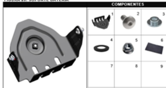
FIGURA 26: SOPORTE BATERIA
