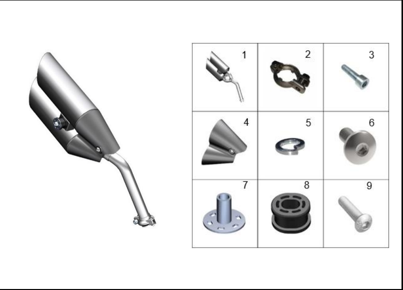
FIGURA 79: PARTE TRASERA SILENCIADOR
