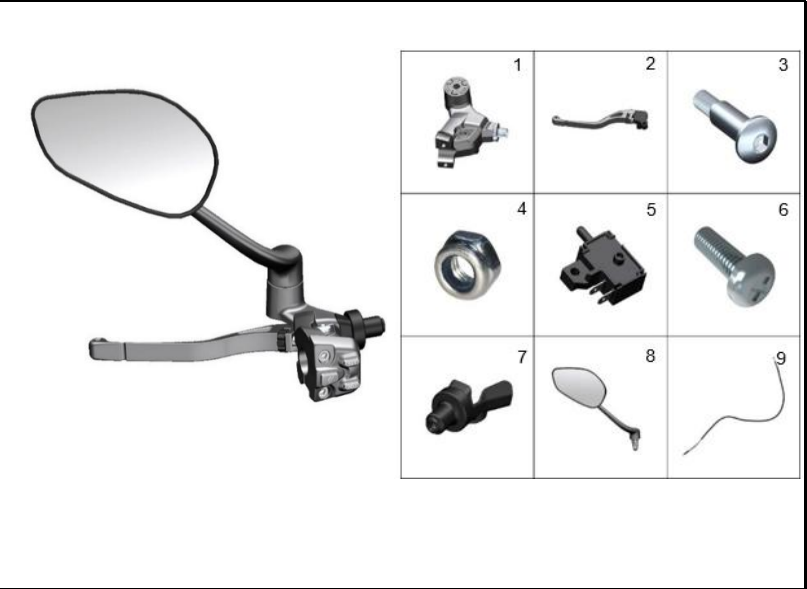
FIGURA 39: LEVA DE CLUTCH – ESPEJO IZQUIERDO
