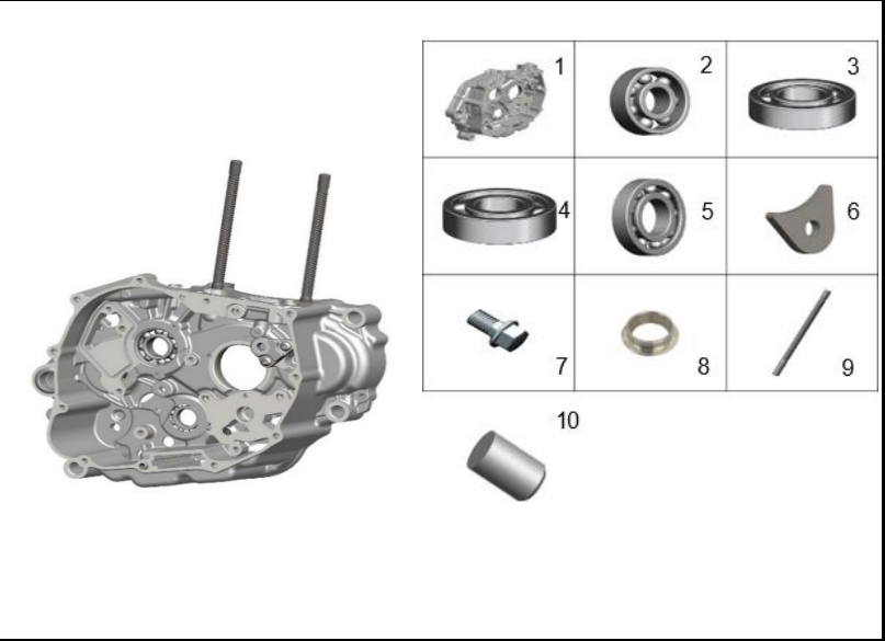
FIGURA 120: CARCASA DERECHA 5
