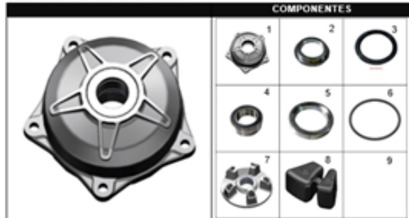
FIGURA 58: PROTECTOR SPROCKET
