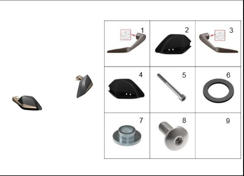
FIGURA 38: CORTAVIENTOS
