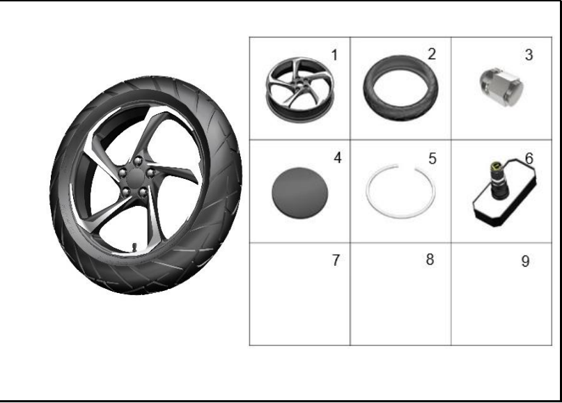
FIGURA 63: RUEDA TRASERA
