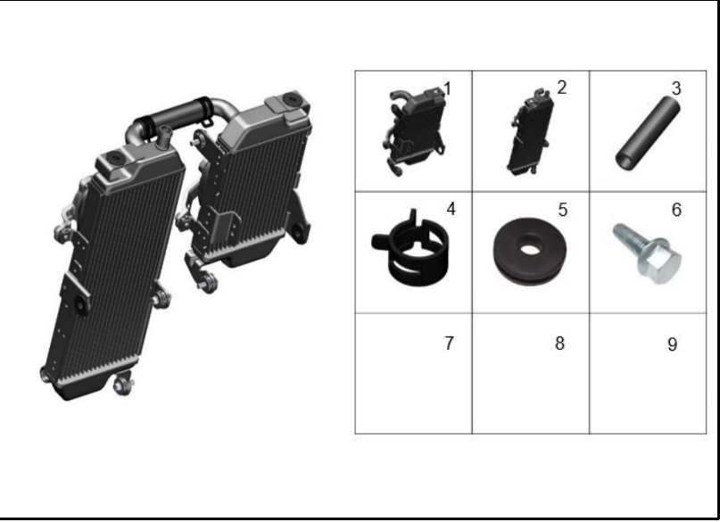
FIGURA 92: RADIADOR
