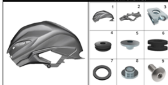
FIGURA 17: CUBIERTA LATERAL IZQUIERDA TANQUE COMBUSTIBLE
