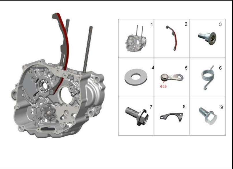
FIGURA 119: CARCASA DERECHA 3
