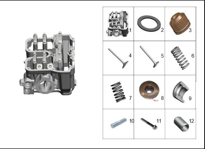
FIGURA 102: CULATA 4
