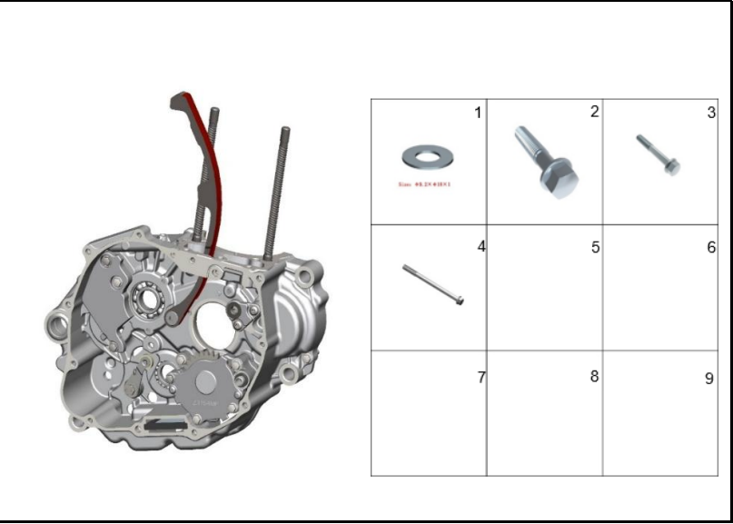
FIGURA 118: CARCASA DERECHA 2
