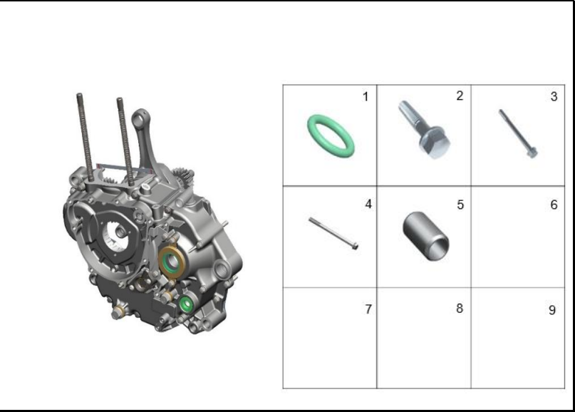
FIGURA 114: CARCASA IZQUIERDA 2
