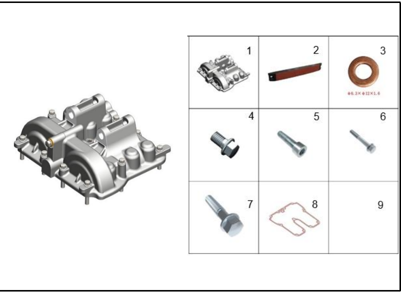
FIGURA 103: TAPA CULATA
