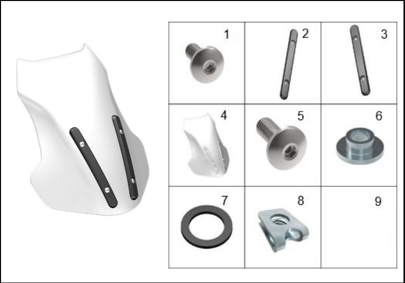
FIGURA 1: VISOR
