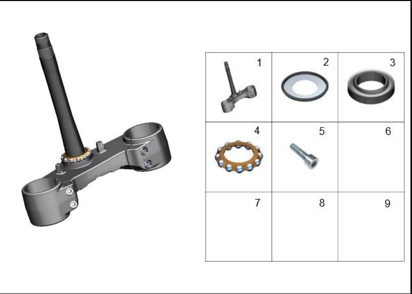
FIGURA 46: HORQUILLA DIRECCIÓN
