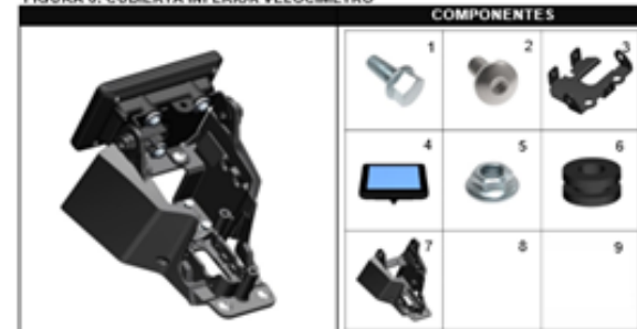
FIGURA 6: CUBIERTA INFERIOR VELOCIMETRO
