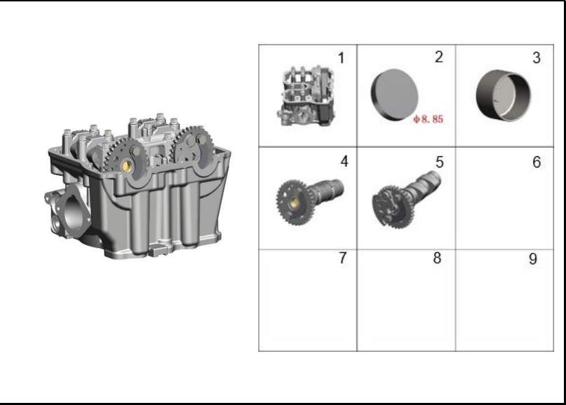
FIGURA 101: CULATA 3
