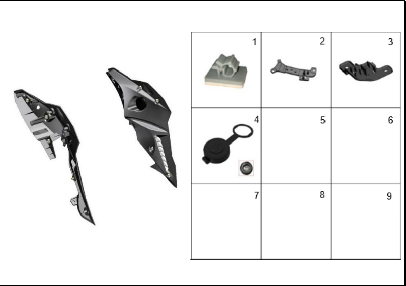
FIGURA 21: CUBIERTAS LATERALES 3
