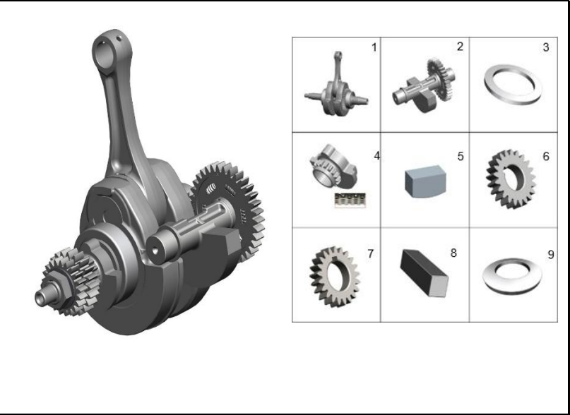
FIGURA 117: CIGÜEÑAL
