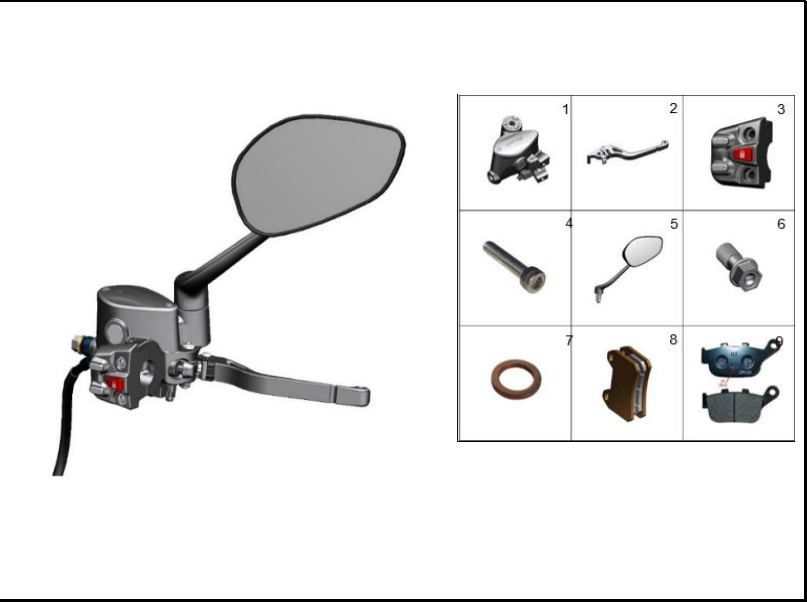
FIGURA 41: LEVA DE FRENO – ESPEJO DERECHO
