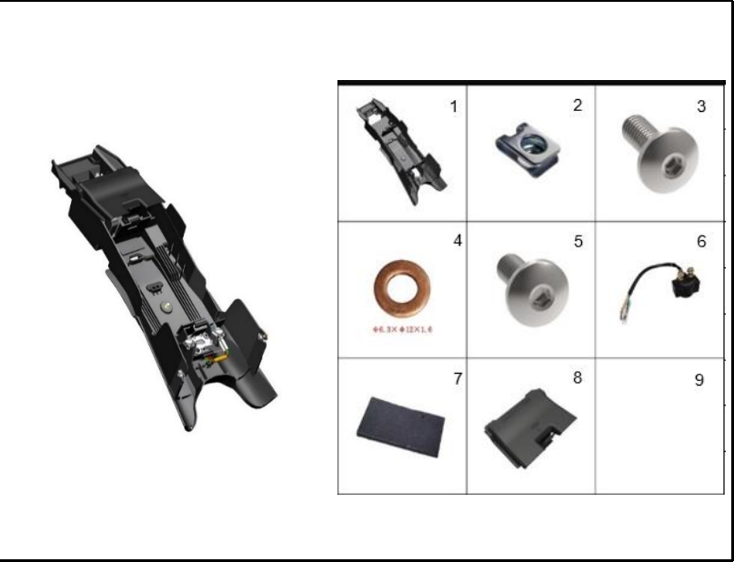
FIGURA 24: GUARDABARRO TRASERO INTERNO
