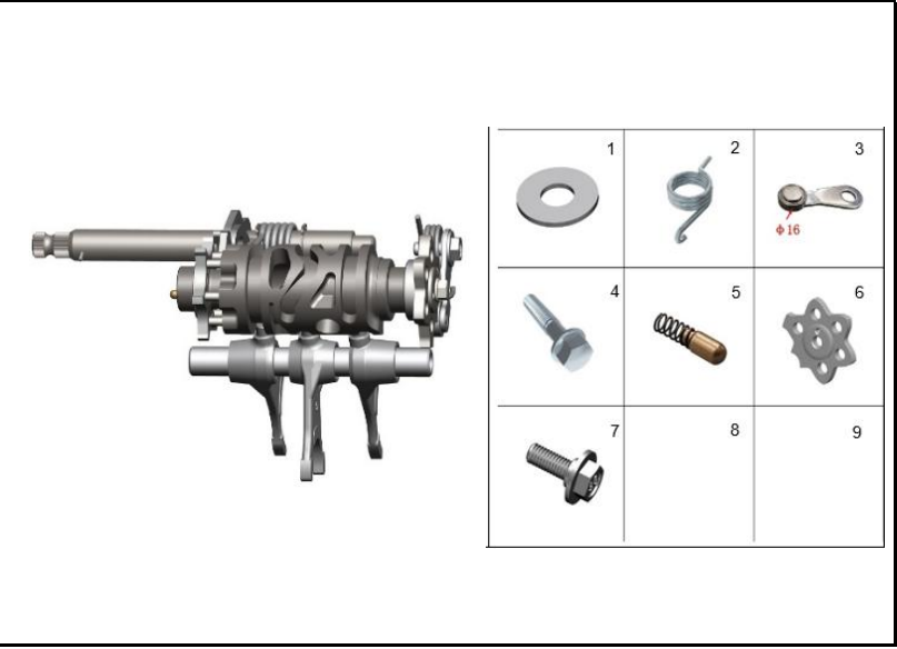
FIGURA 113: EJE DE CAMBIOS 2
