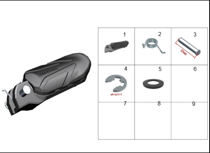
FIGURA 81: REPOSAPIE DELANTERO IZQUIERDO
