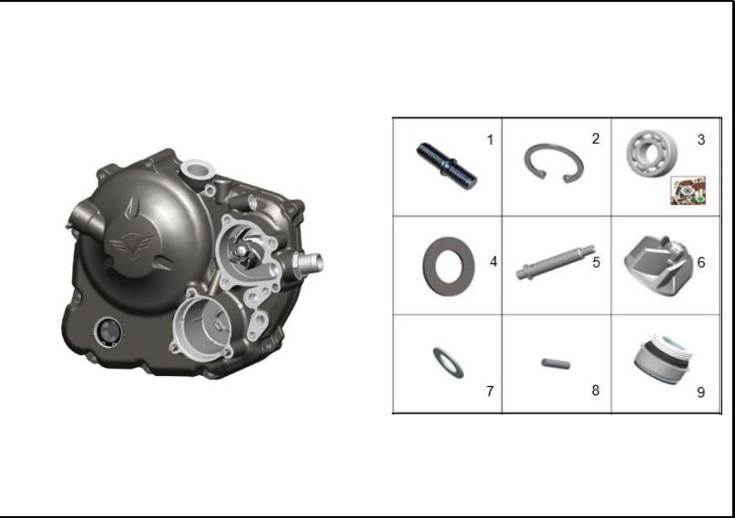
FIGURA 126: CUBIERTA CARCASA MOTOR DERECHA 2
