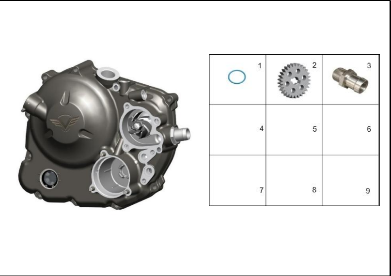
FIGURA 126: CUBIERTA CARCASA MOTOR DERECHA 3
