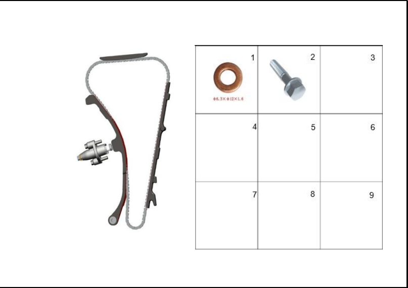
FIGURA 128: CADENILLA DE DISTRIBUCIÓN 2
