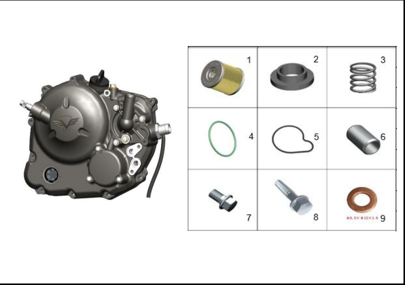
FIGURA 125: TAPA CARTER DERECHA 4
