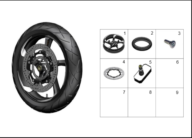
FIGURA 48: RUEDA DELANTERA
