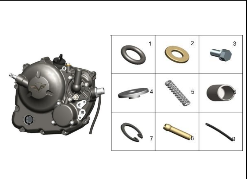
FIGURA 125: TAPA CARTER DERECHA 5
