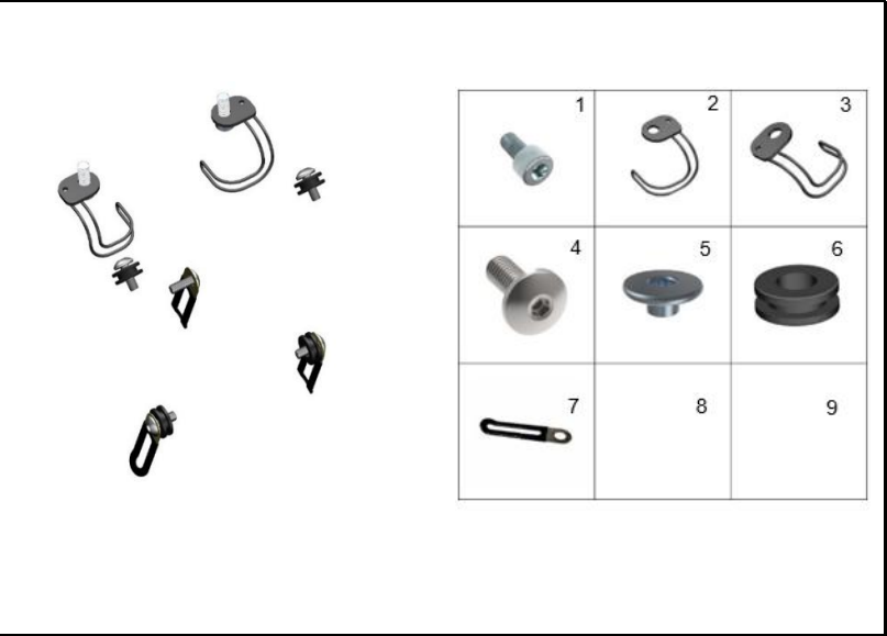
FIGURA 9: GUIAS
