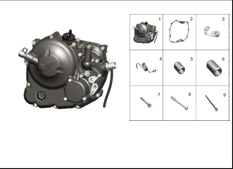
FIGURA 124: TAPA CARTER DERECHA
