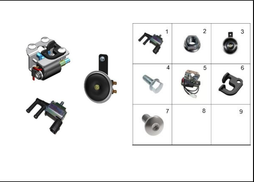
FIGURA 67: PITO Y SEGURO SILLIN
