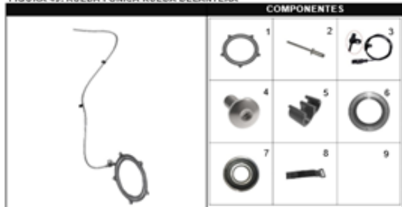
FIGURA 49: RUEDA FONICA RUEDA DELANTERA
