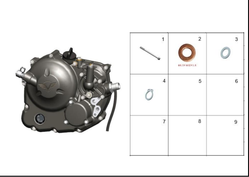
FIGURA 124: TAPA CARTER DERECHA 2
