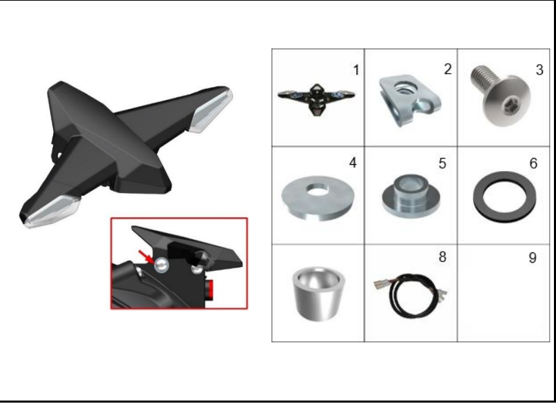
FIGURA 34: SOPORTE DIRECCIONALES COMPLETO
