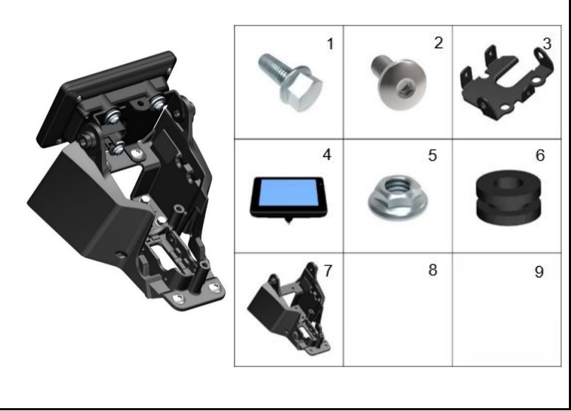
FIGURA 6: CUBIERTA INFERIOR VELOCIMETRO
