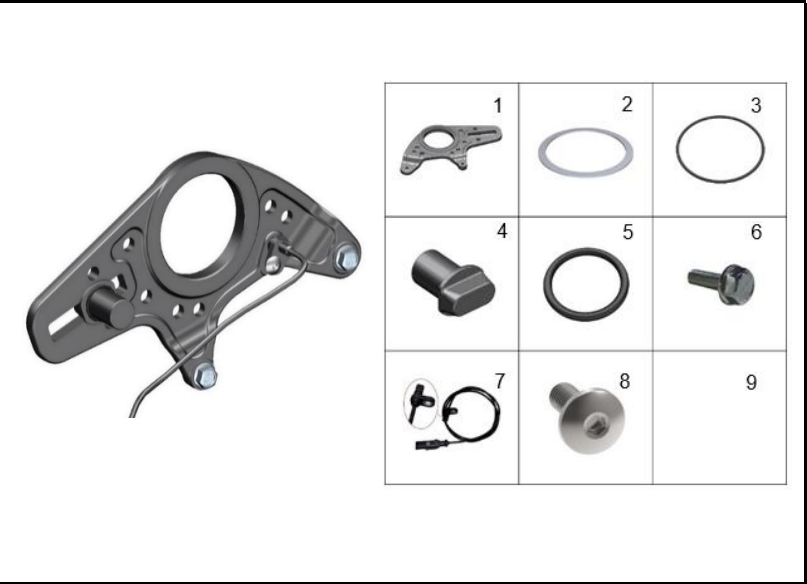
FIGURA 61: SOPORTE FRENO TRASERO
