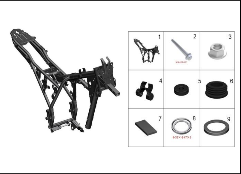
FIGURA 64: PARTES CHASIS
