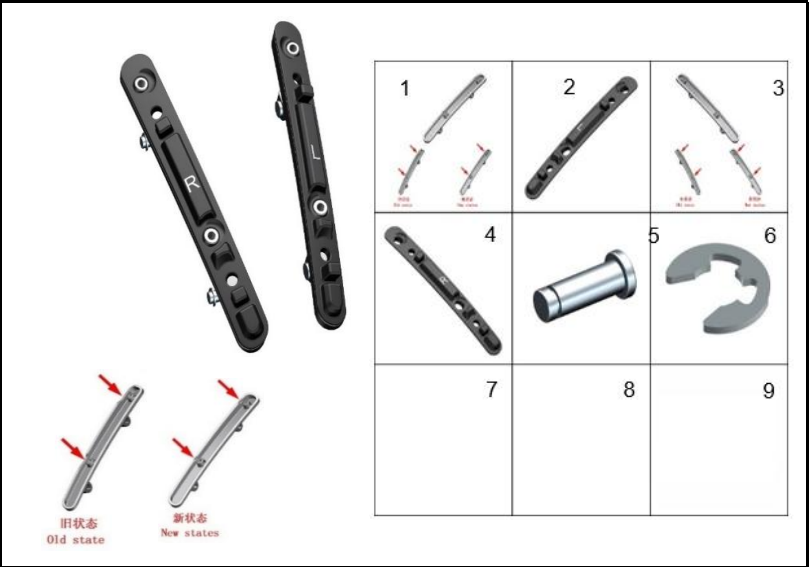
FIGURA 2: SOPORTES VISOR
