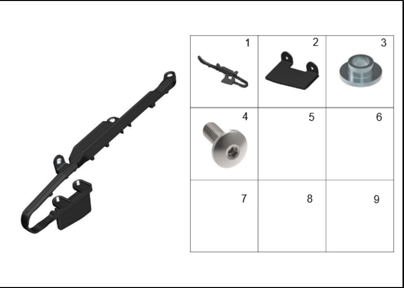
FIGURA 52: DESLIZADOR CADENA
