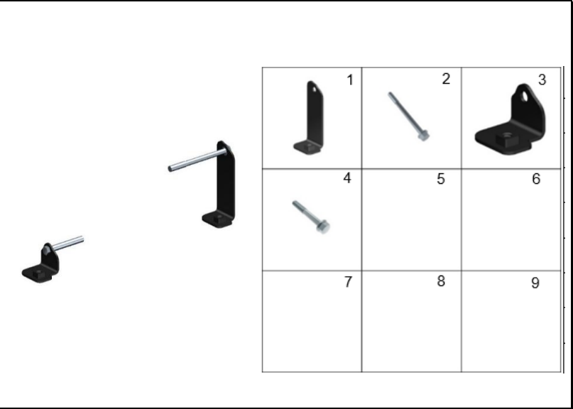
FIGURA 14: PLATINA IZQUIERDA CUBIERTA INFERIOR
