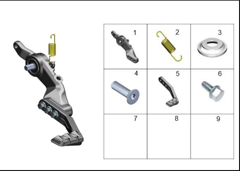
FIGURA 88: PEDAL DE FRENO
