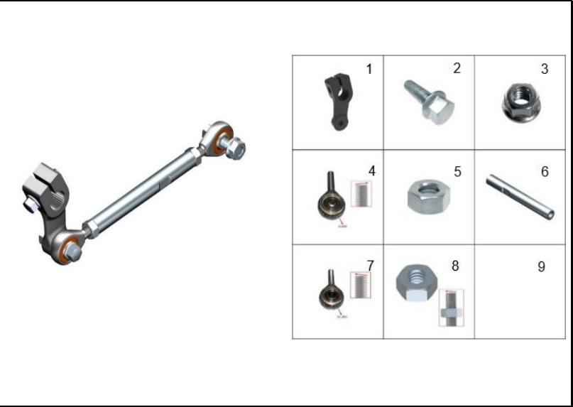
FIGURA 83: MUÑON PEDAL DE CAMBIOS
