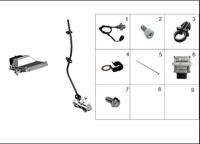
FIGURA 69: SENSOR SOPORTE LATERAL
