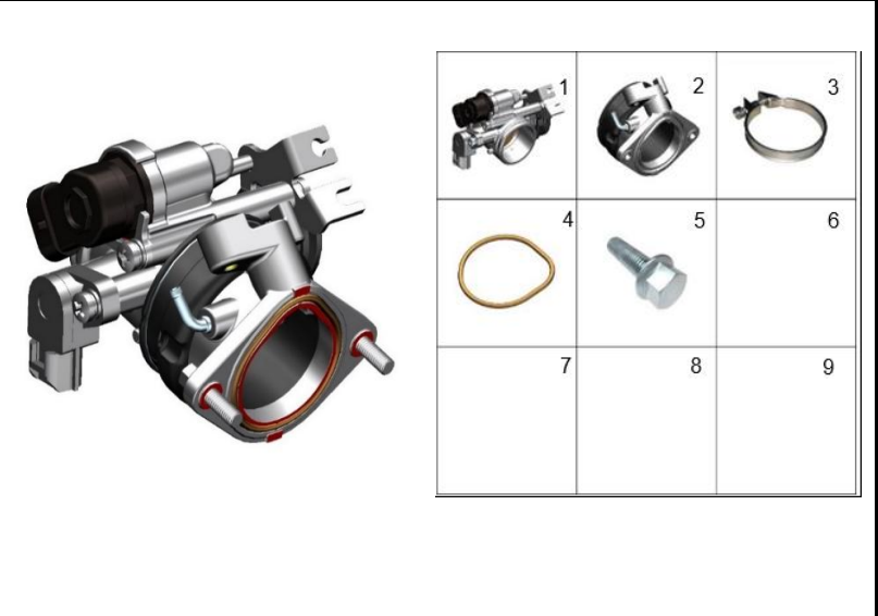
FIGURA 74: CUERPO DE INYECCIÓN
