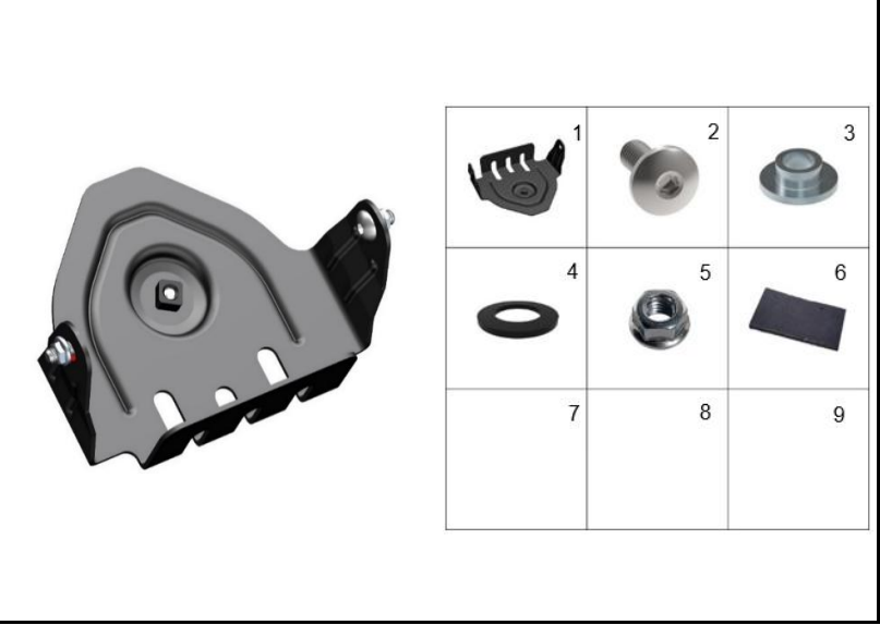
FIGURA 26: SOPORTE BATERIA
