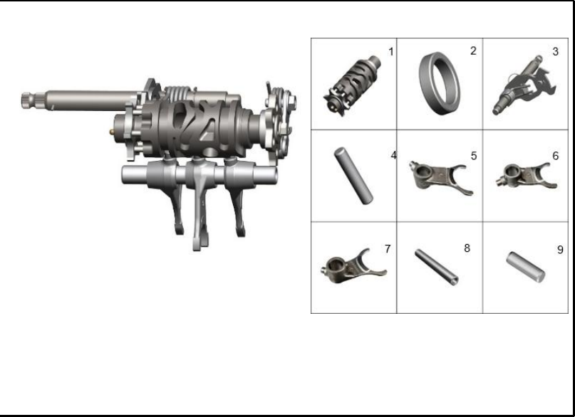
FIGURA 113: EJE DE CAMBIOS
