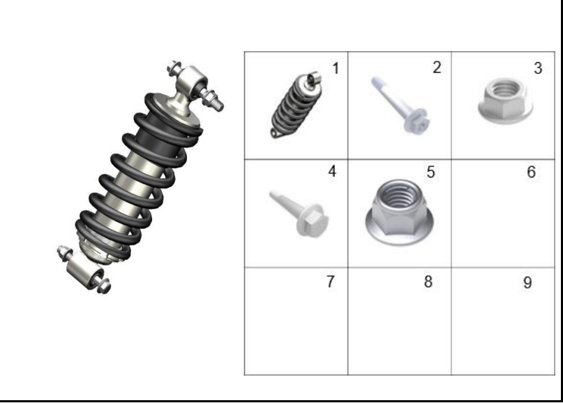
FIGURA 51: AMORTIGUADOR TRASERO
