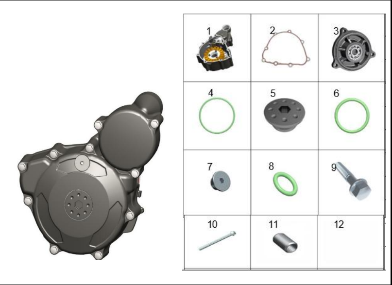
FIGURA 121: TAPA CÁRTER IZQ
