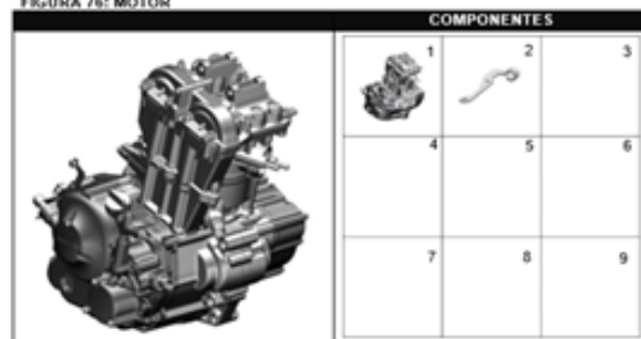
FIGURA 76: MOTOR
