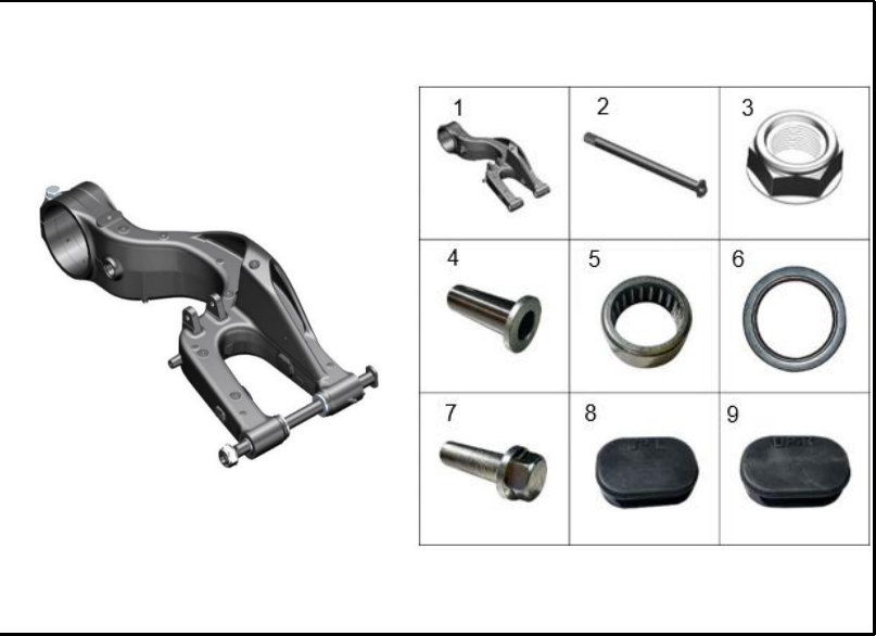
FIGURA 50: BRAZO OSCILANTE
