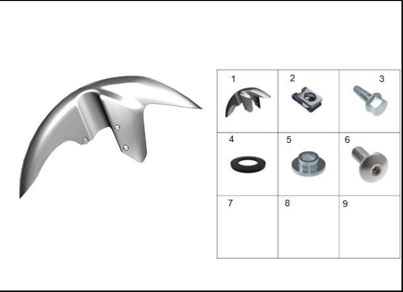
FIGURA 12: GUARDABARRO DELANTERO
