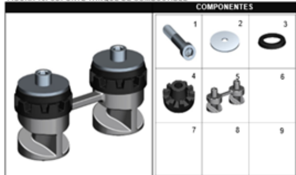
FIGURA 16: SOPORTE TANQUE DE COMBUSTIBLE
