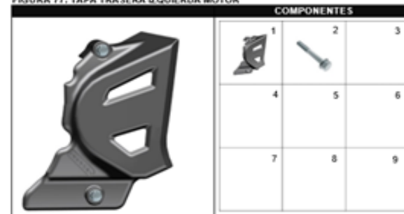
FIGURA 77: TAPA TRASERA IZQUIERDA MOTOR
