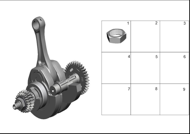
FIGURA 117: CIGÜEÑAL 2
