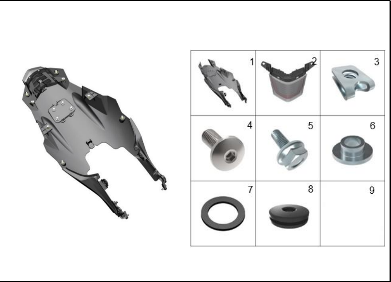
FIGURA 28: COLA INFERIOR
