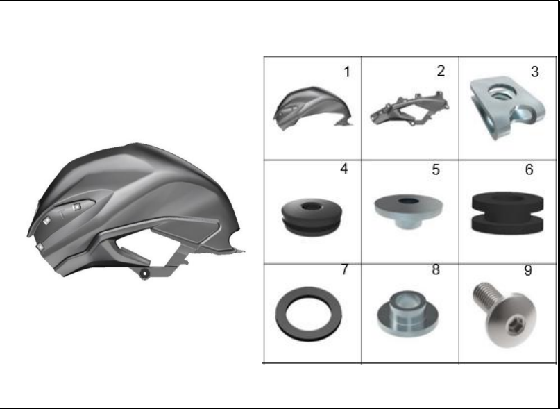
FIGURA 17: CUBIERTA LATERAL IZQUIERDA TANQUE COMBUSTIBLE
