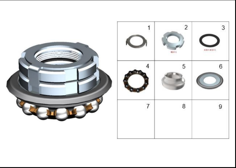
FIGURA 45: CUNAS DIRECCIÓN
