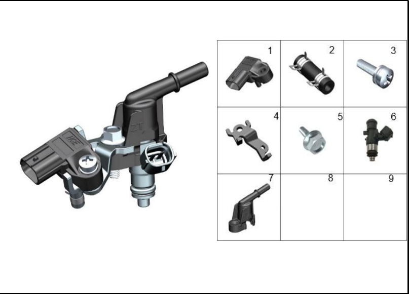
FIGURA 75: SOPORTE INYECTOR
