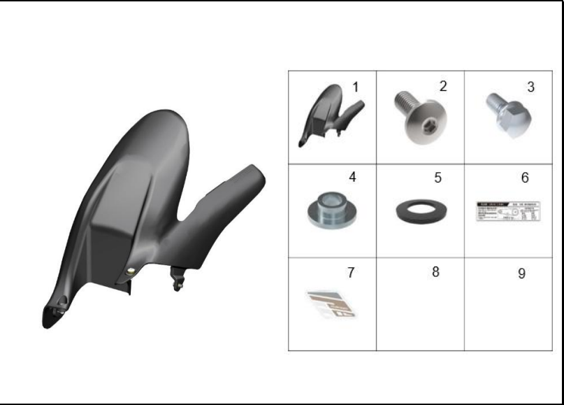
FIGURA 53: GUARDABARRO TRASERO INFERIOR IZQUIERDO
