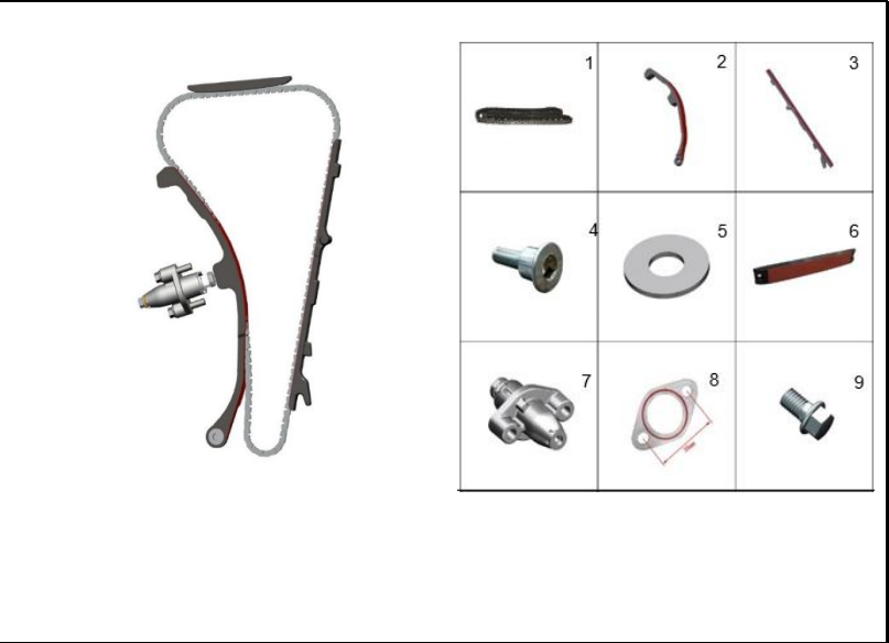
FIGURA 128: CADENILLA DE DISTRIBUCIÓN
