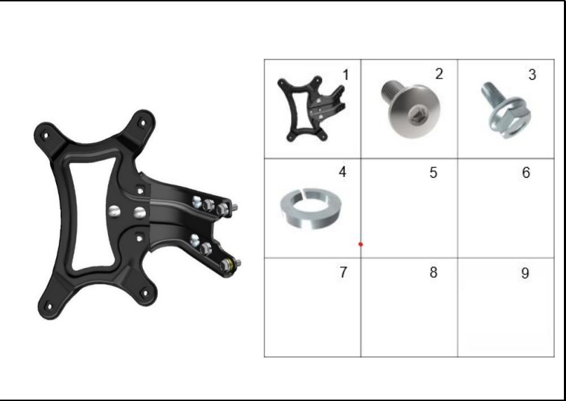
FIGURA 56: SOPORTE GUARDABARRO LLANTA
