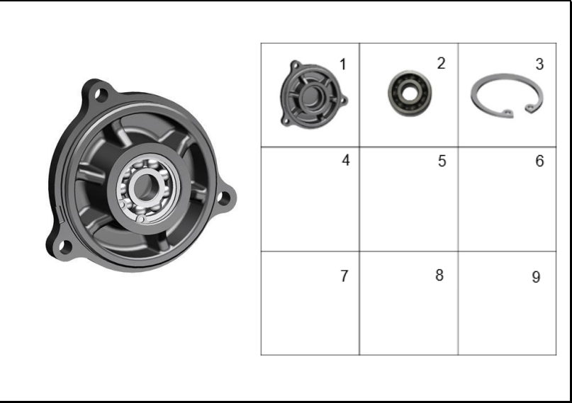
FIGURA 123: TAPA PIÑÓN REDUCTOR ARRANQUE
