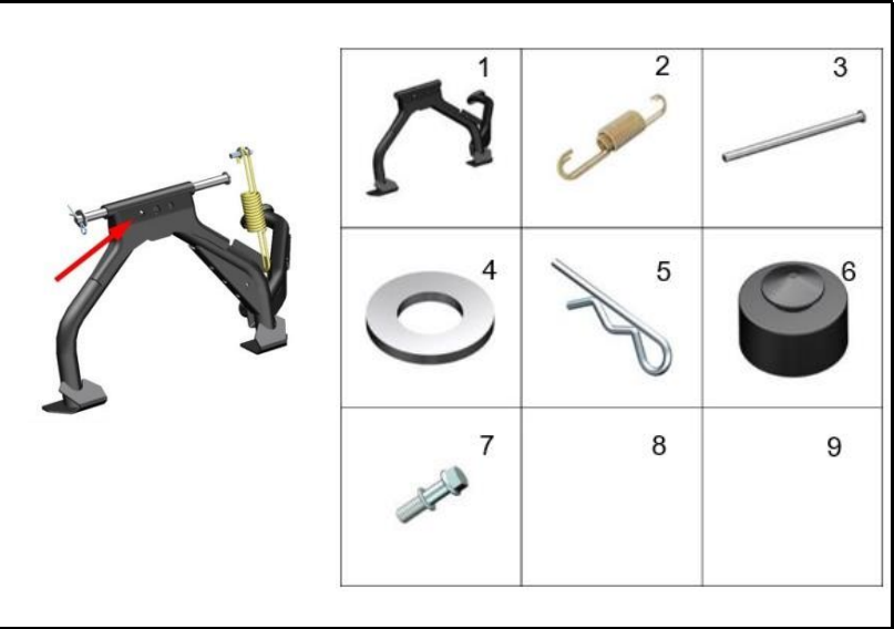
FIGURA 91: SOPORTE CENTRAL
