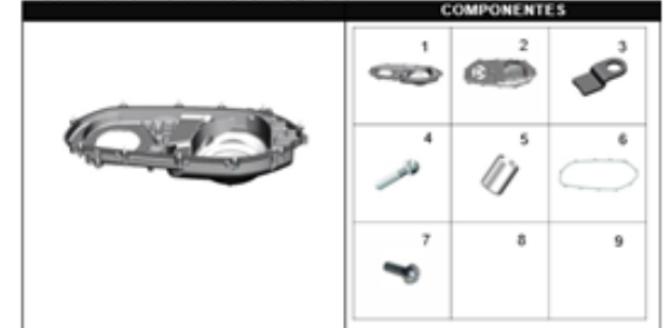
FIGURA 123: CARCASA MOTOR IZQUIERDA
