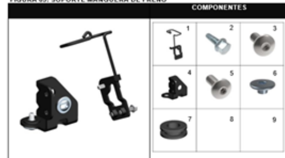
FIGURA 63: SOPORTE MANGUERA DE FRENO
