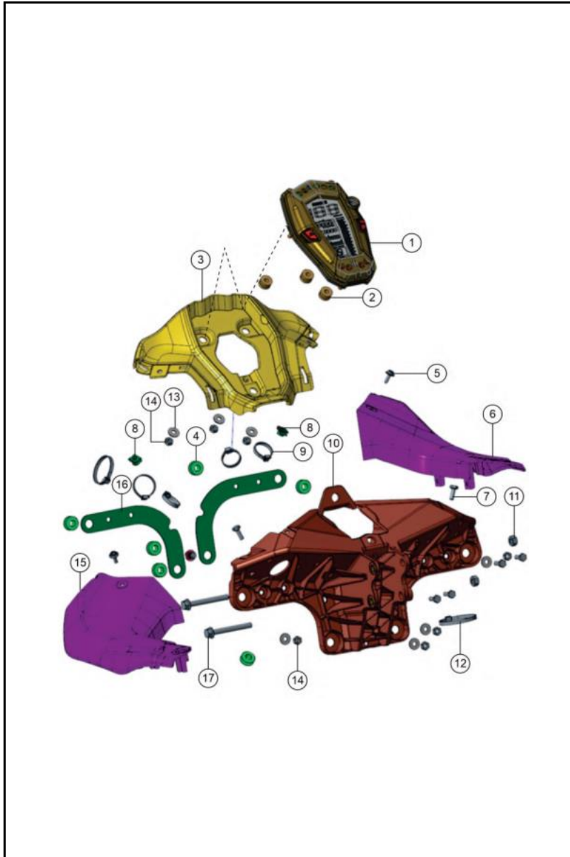
FIGURA N°18: VELOCÍMETRO
