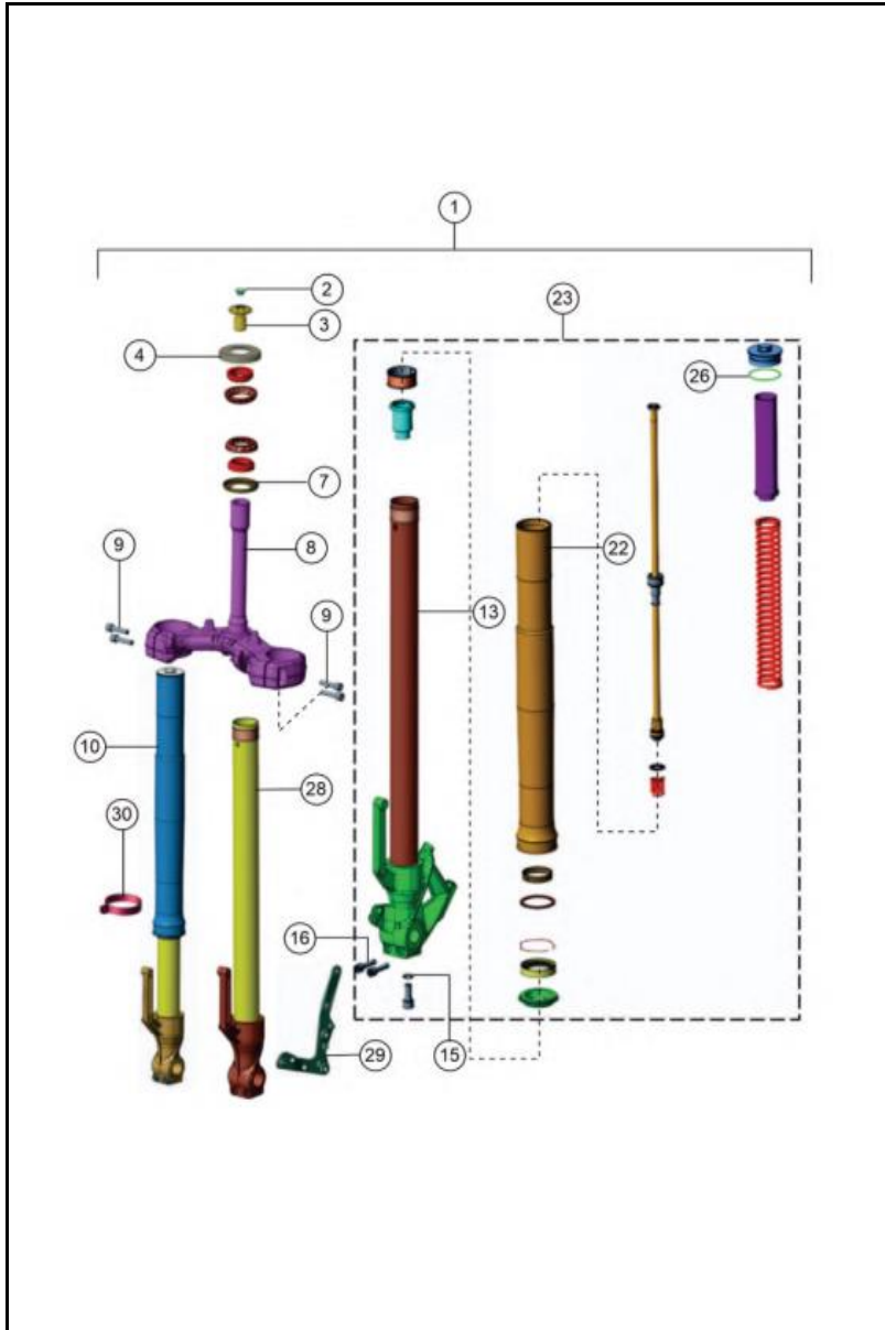
FIGURA N°29 :SUSPENSIÓN DELANTERA
