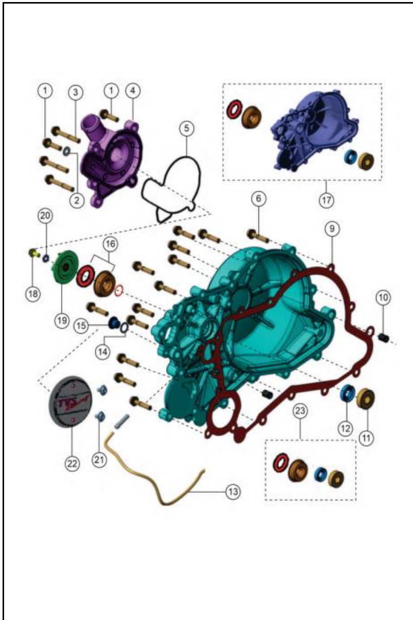
FIGURA N°8: CUBIERTA CLUTCH
