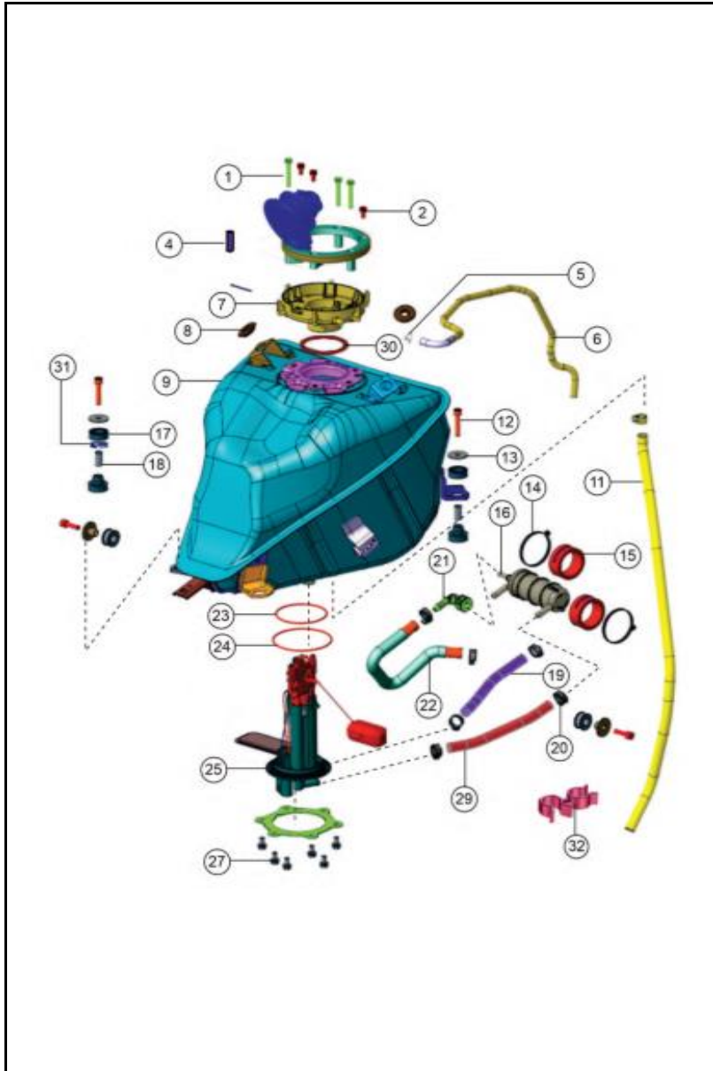
FIGURA N°15 :TANQUE DE GASOLINA
