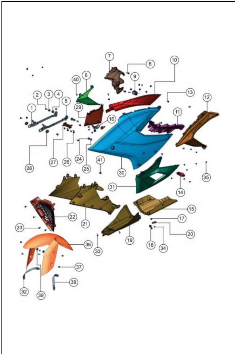
FIGURA N°25: CUBIERTA LADO IZQUIERDO (2/2)
