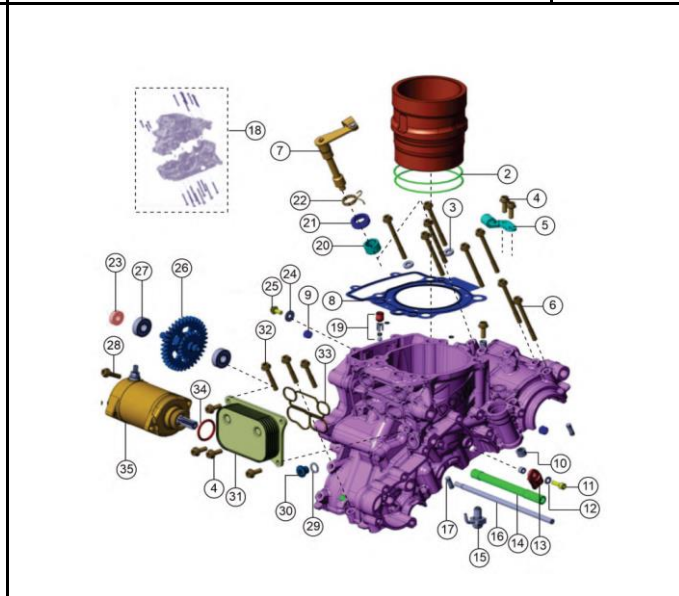
FIG. Nº 5 CARCASA CENTRAL MOTOR SUPERIOR
