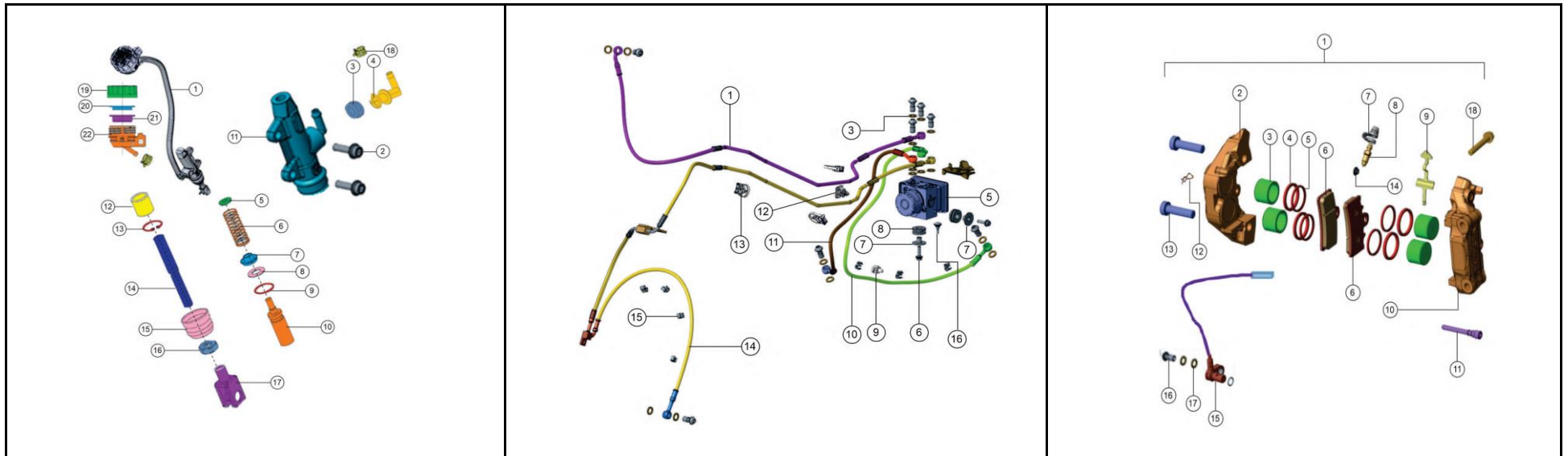
BOMBA FRENO TRASERA
