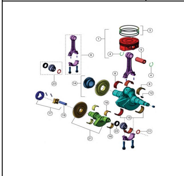
FIG. Nº 4 PISTÓN / CIGÜEÑAL
