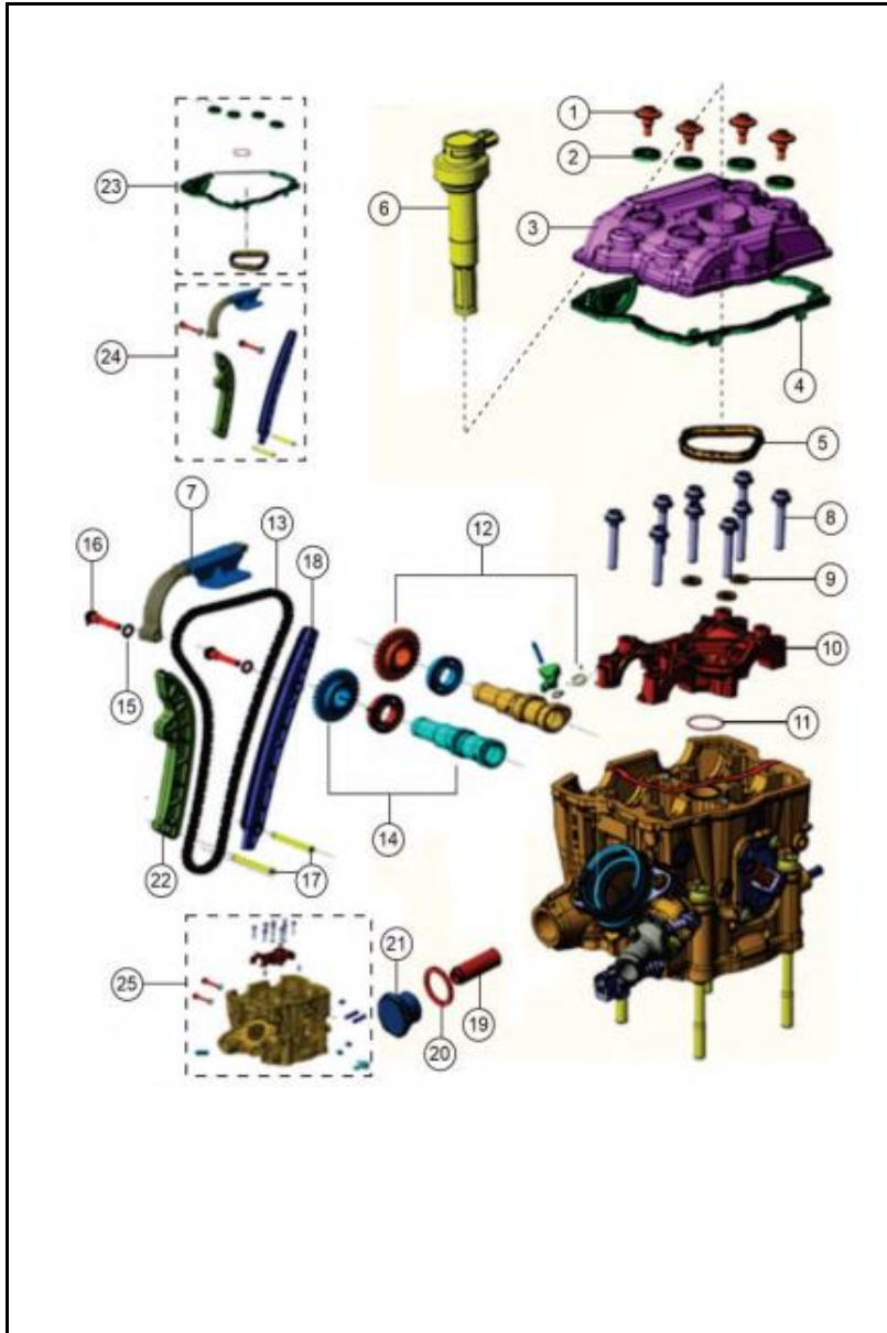
FIGURA N° 1: CUBIERTA CULATA / EJE DE LEVAS
