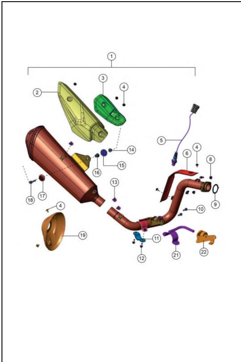
FIGURA N°12: SILENCIADOR
