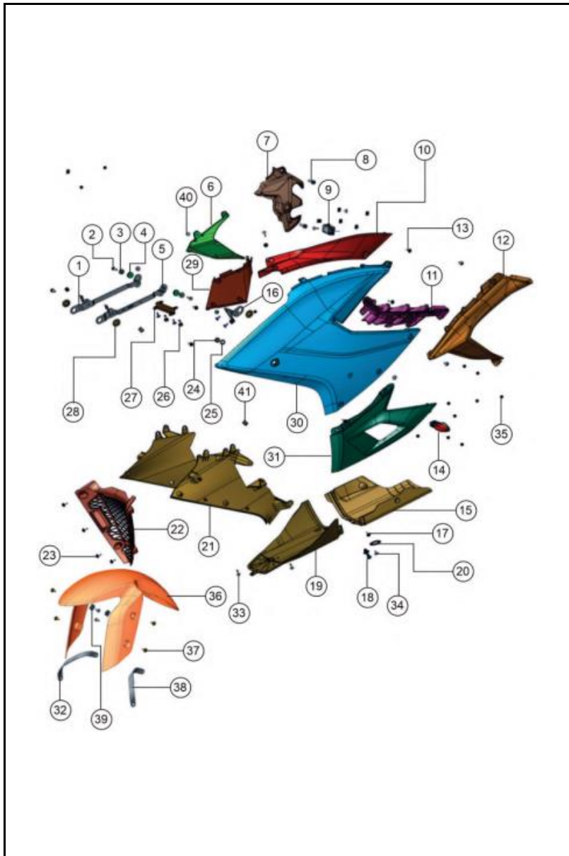
FIGURA N°25: CUBIERTA LADO IZQUIERDO (1/2)
