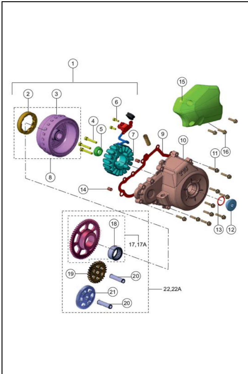
FIGURA N°7: CUBIERTA VOLANTE / VOLANTE
