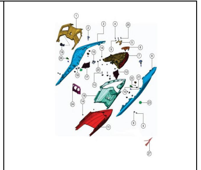
STOP / CUBIERTAS TRASERAS
