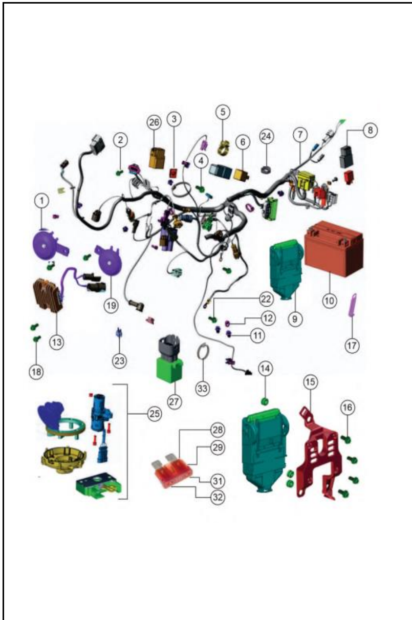
FIGURA N°38: EQUIPO ELECTRICO (2/2)
