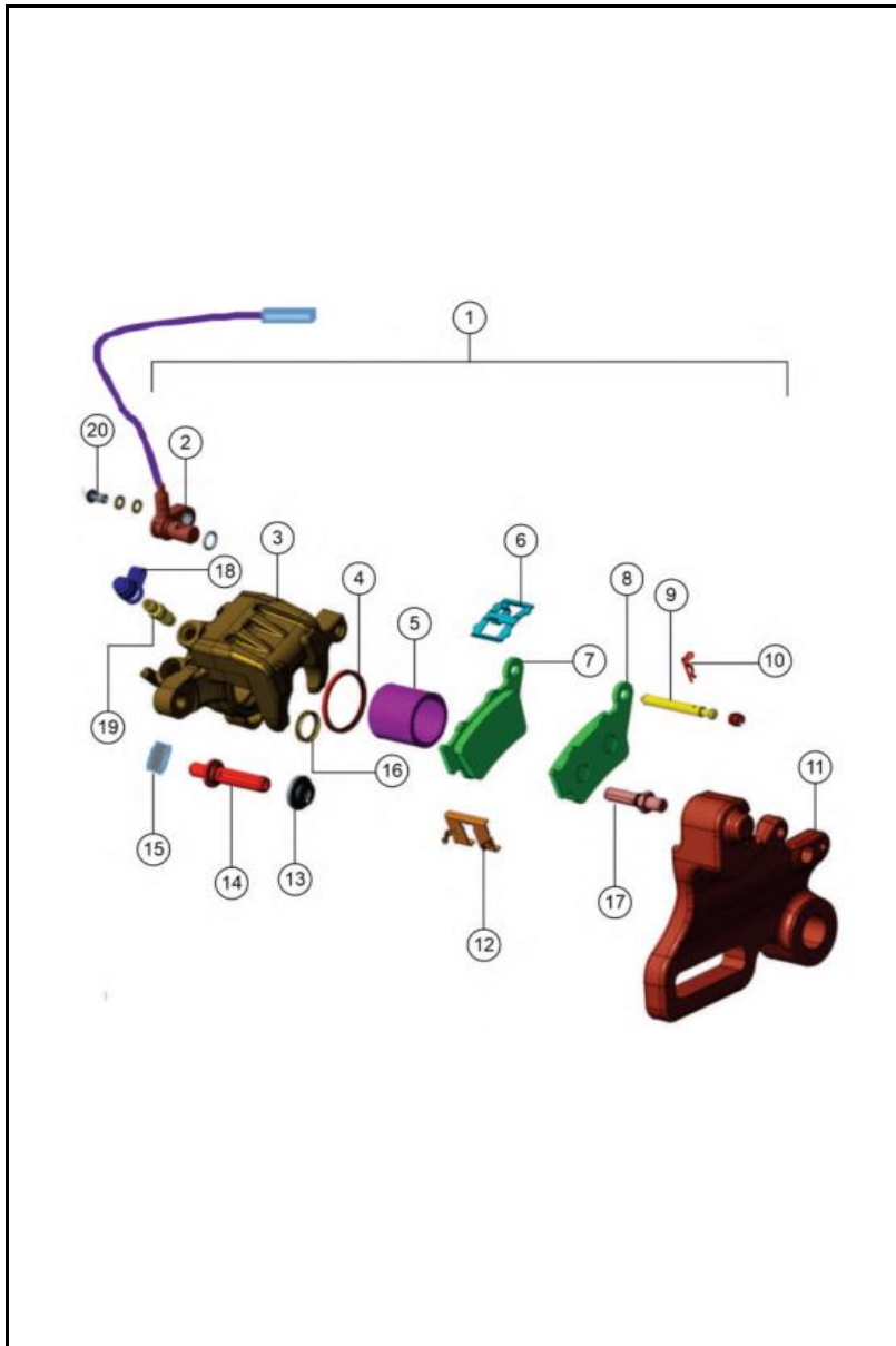
FIGURA N°36: CALIPER TRASERO
