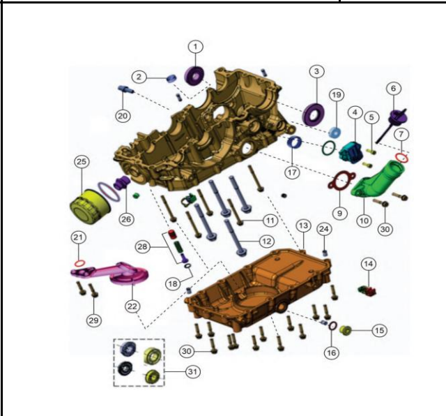
FIG. Nº 6 CARCASA MOTOR CENTRAL INFERIOR
