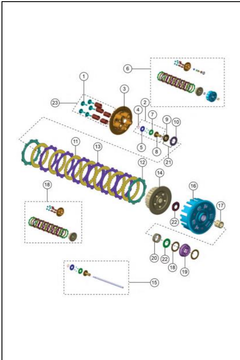
FIGURA N°9: CLUTCH
