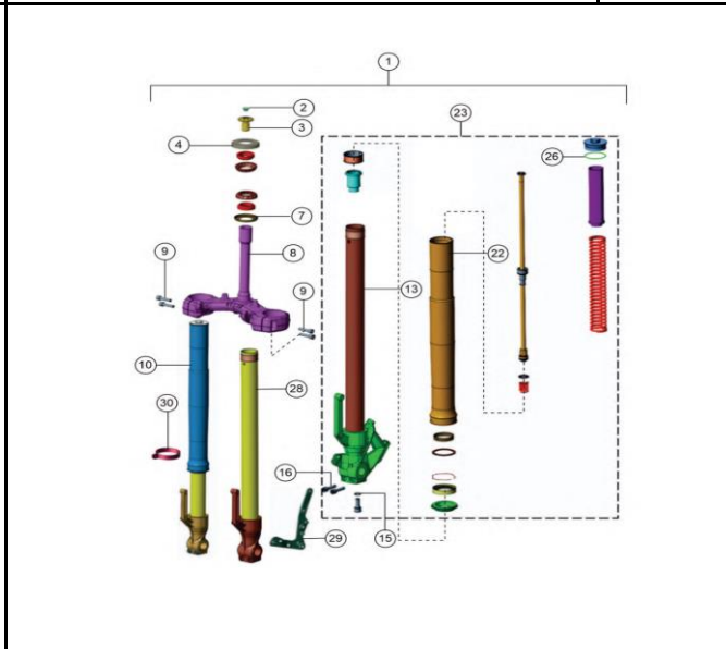
SUSPENSIÓN DELANTERA
