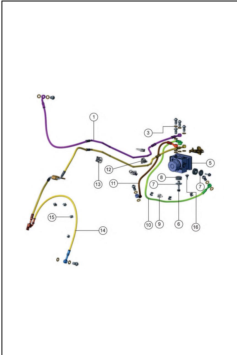
FIGURA N°32: SISTEMA ABS
