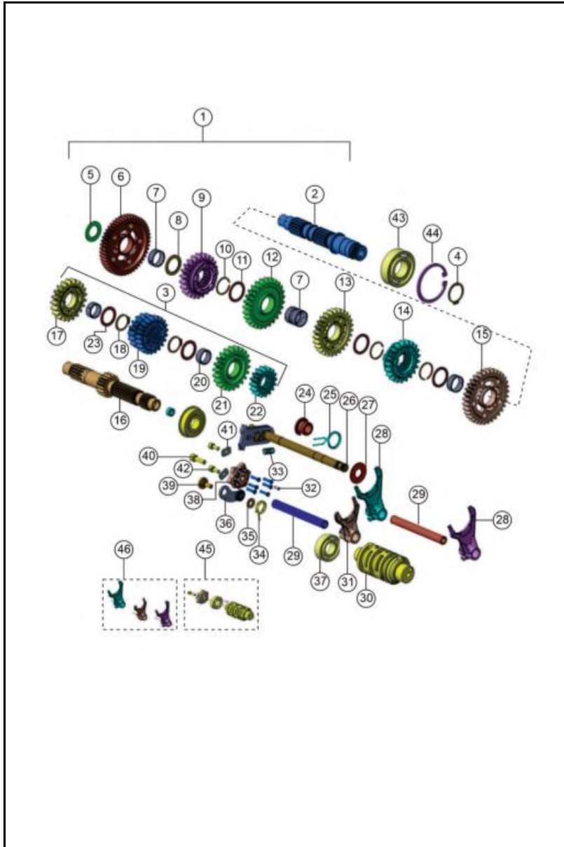
FIGURA N°10: TRANSMISIÓN (1/2)
