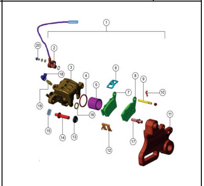
PAG. Nº 50, 51 CALIPER TRASERO
