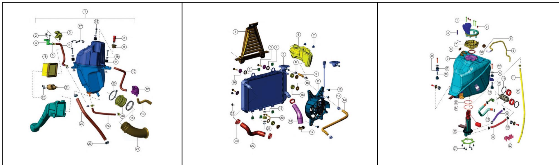
CAJA FILTRO AIRE
