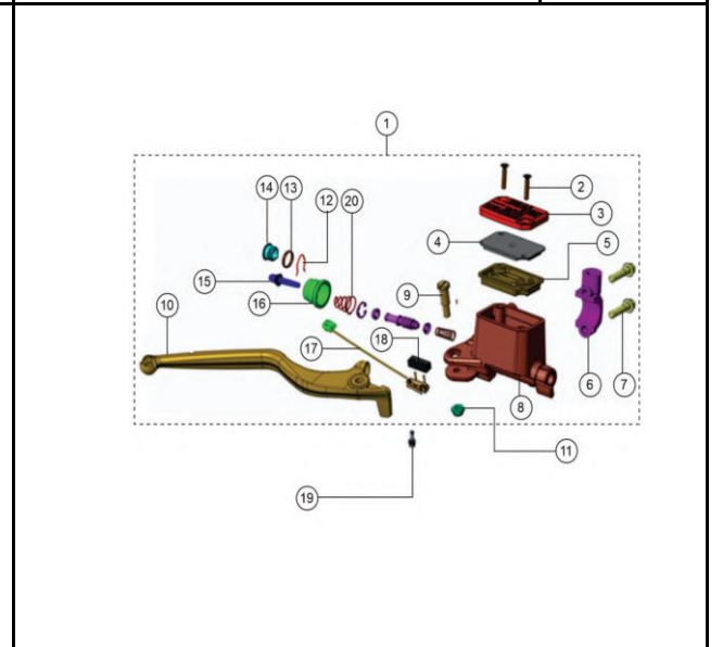
BOMBA FRENO DELANTERA
