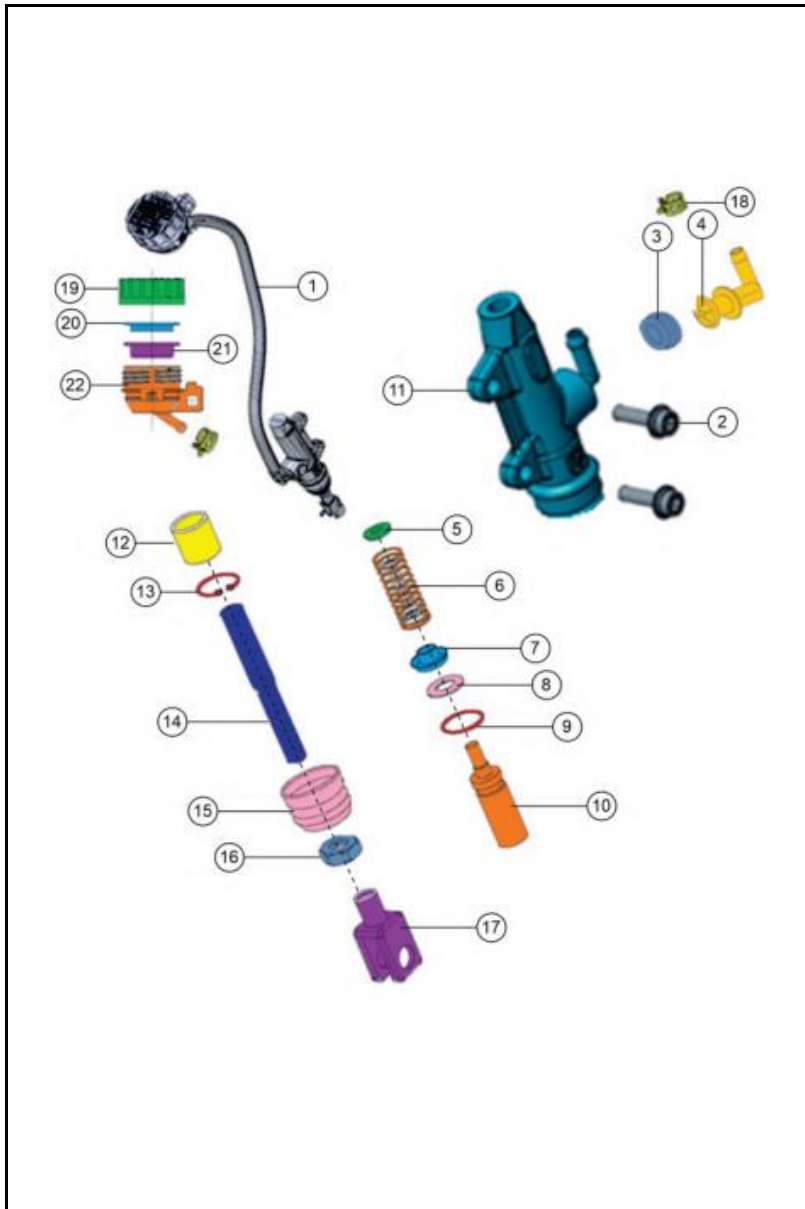
FIGURAN° 31: BOMBA FRENO TRASERA
