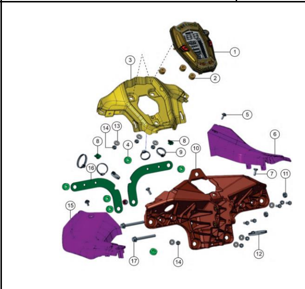
VELOCÍMETRO
