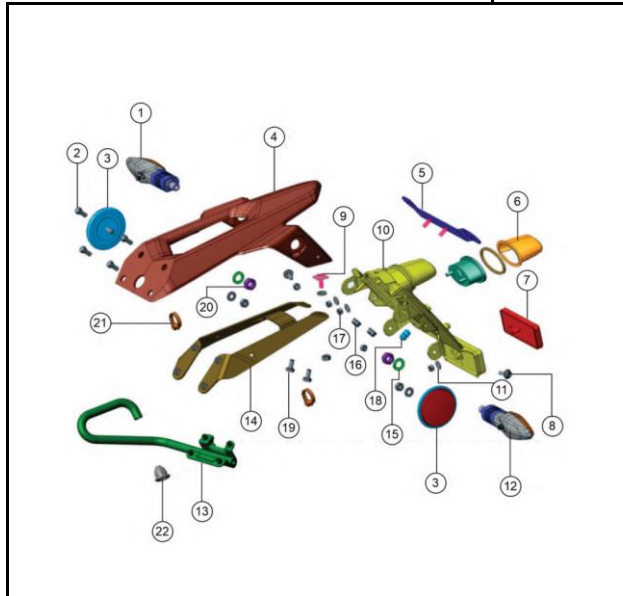
GUARDABARRO TRASERO
