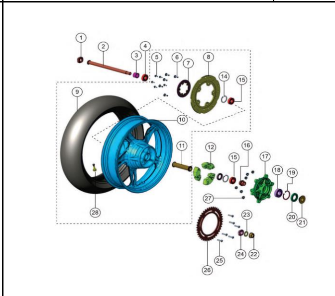
PAG. Nº 49 RUEDA TRASERA
