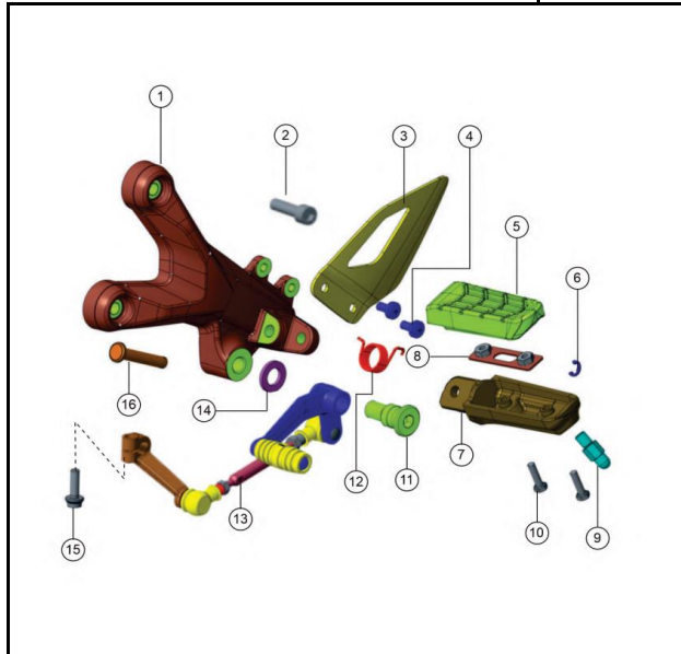
REPOSAPIÉ DELANTERO IZQUIERDO
