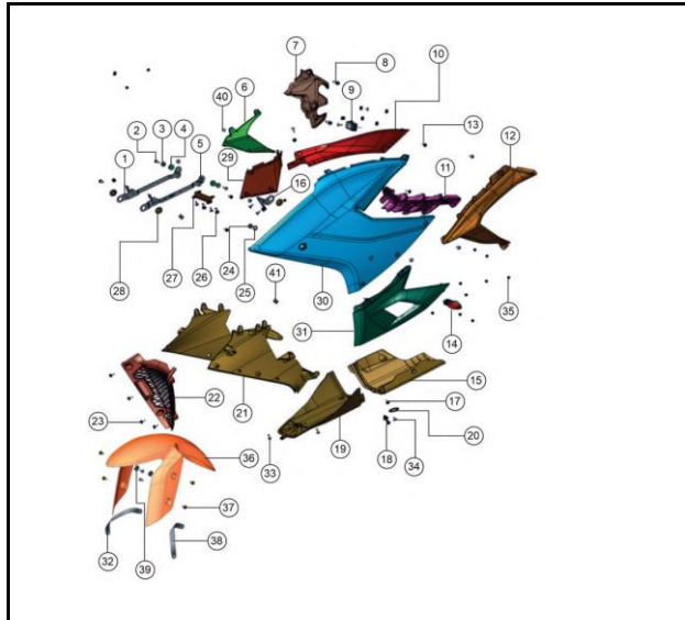
CUBIERTA LADO IZQUIERDO
