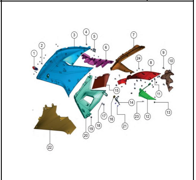
CUBIERTA LADO DERECHO
