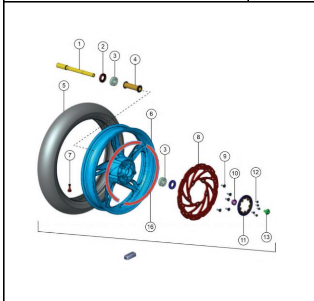
RUEDA DELANTERA
