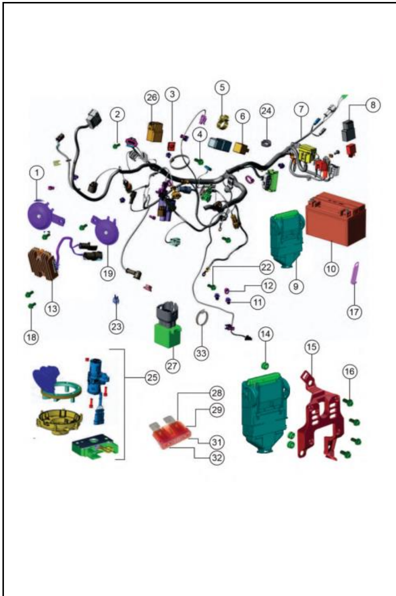
FIGURA N°38: EQUIPO ELECTRICO (1/2)
