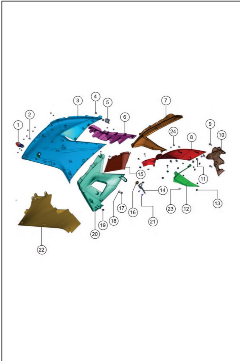
FIGURA N°24: CUBIERTA LADO DERECHO
