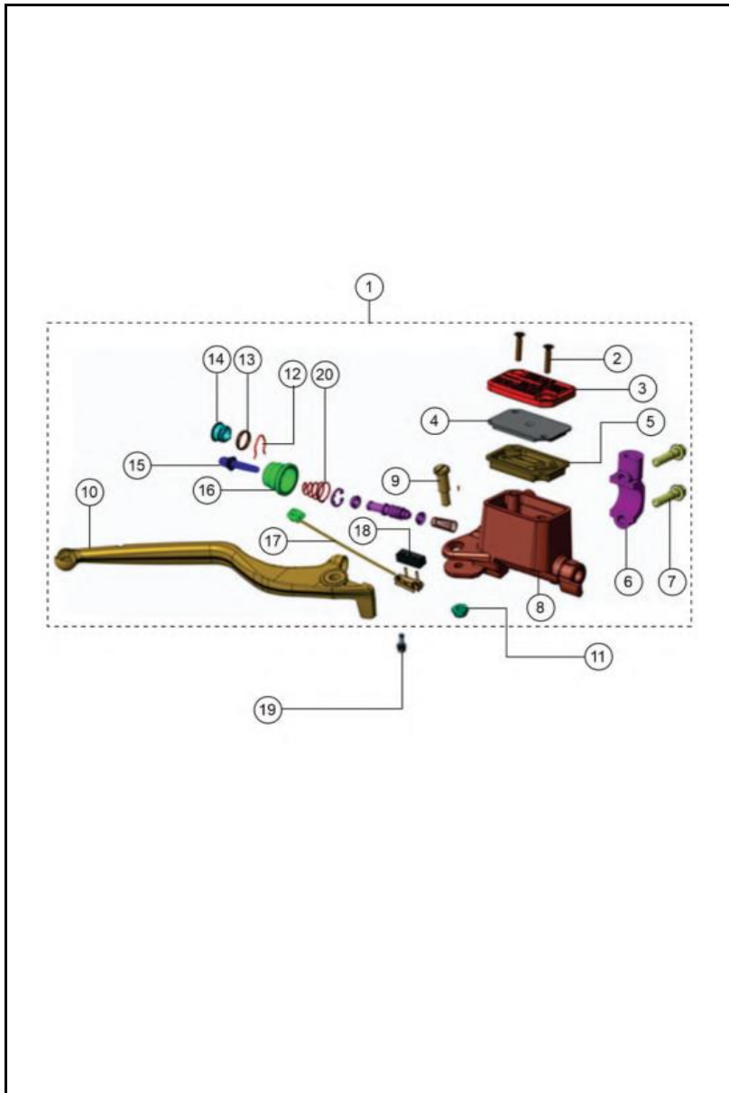
FIGURAN° 30: BOMBA FRENO DELANTERA
