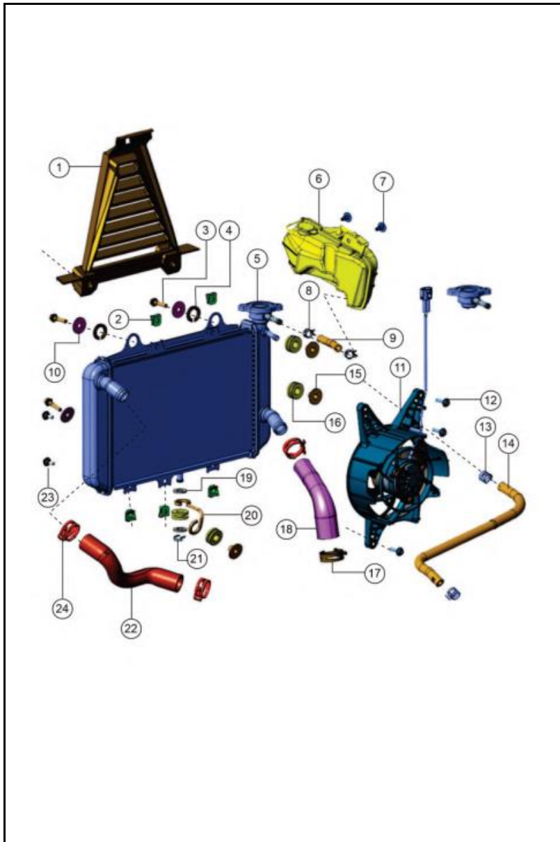
FIGURA N°14: RADIADOR (1/2)
