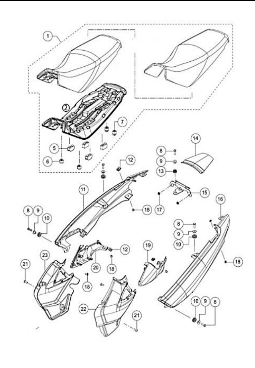
FIGURA N° 24: SILLÍN / CUBIERTAS
