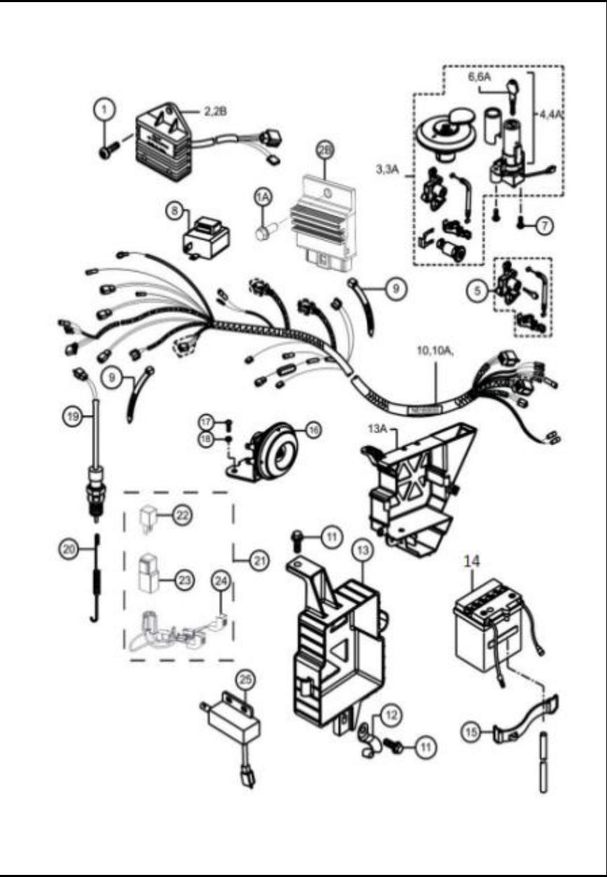
FIGURA N° 32: EQUIPO ELÉCTRICO (1/2)
