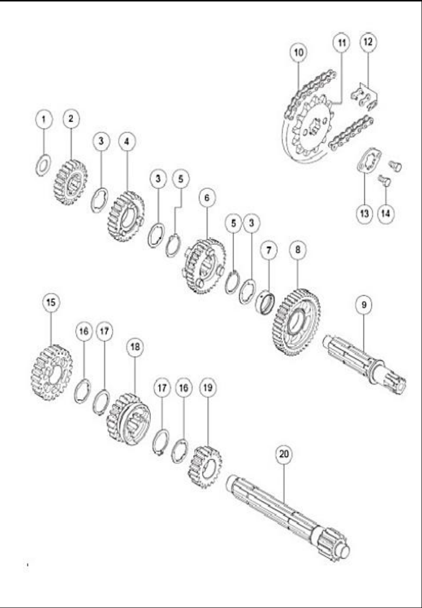
FIGURA N° 11: TRANSMISIÓN
