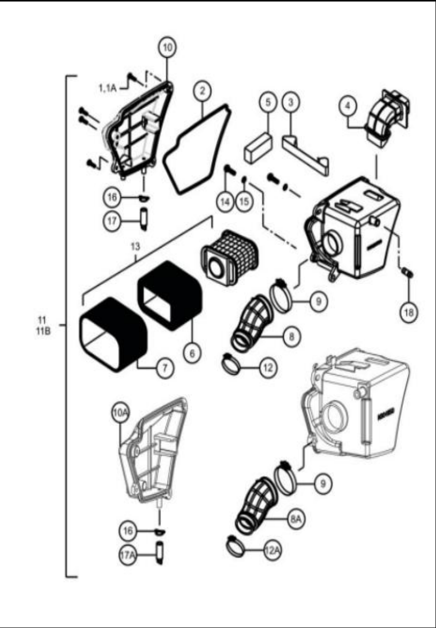
FIGURA N° 12: FILTRO DE AIRE
