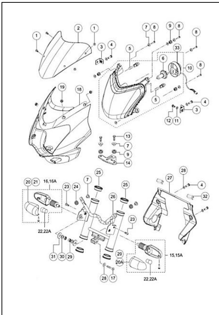
FIGURA N° 23 : FAROLA (1/2)
