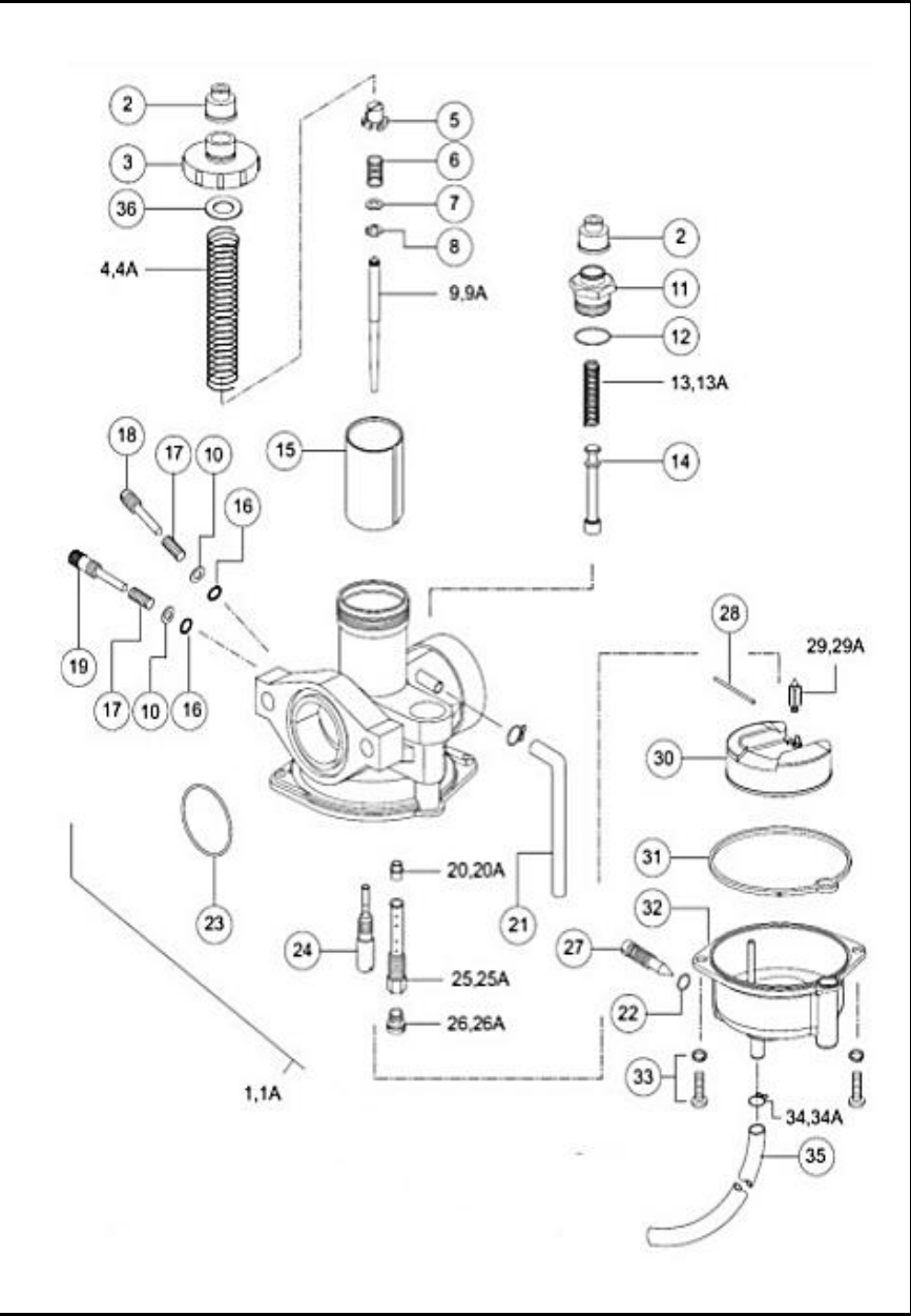
FIGURA N° 15: CARBURADOR (1/2)
