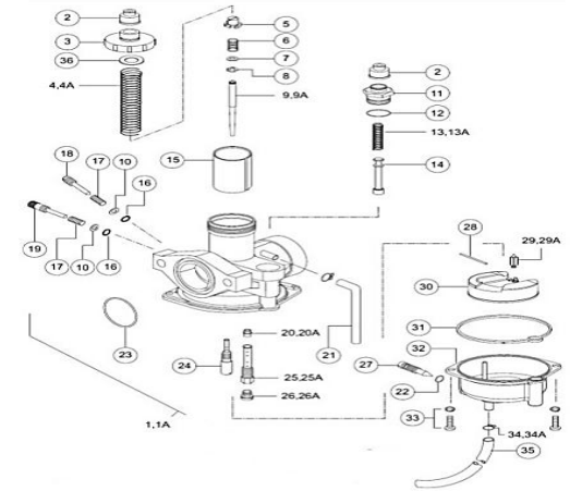
FIGURA N° 15: CARBURADOR
