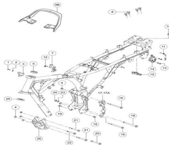
FIGURA N° 17: CHASIS
