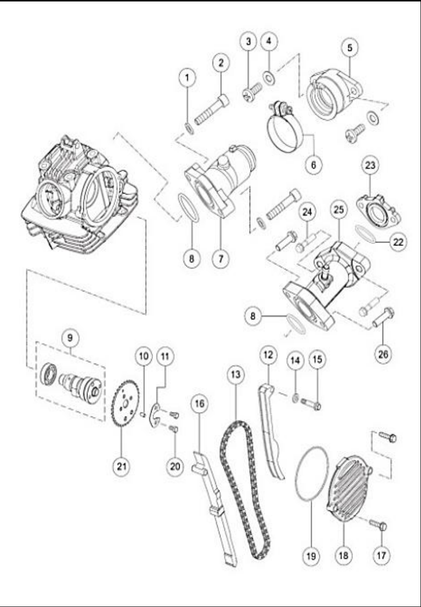
FIGURA N° 2: EJE DE LEVAS
