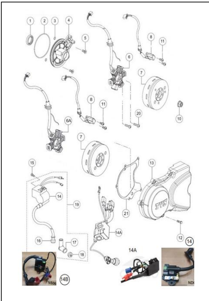
FIGURA N° 7: CUBIERTA VOLANTE (KS)
