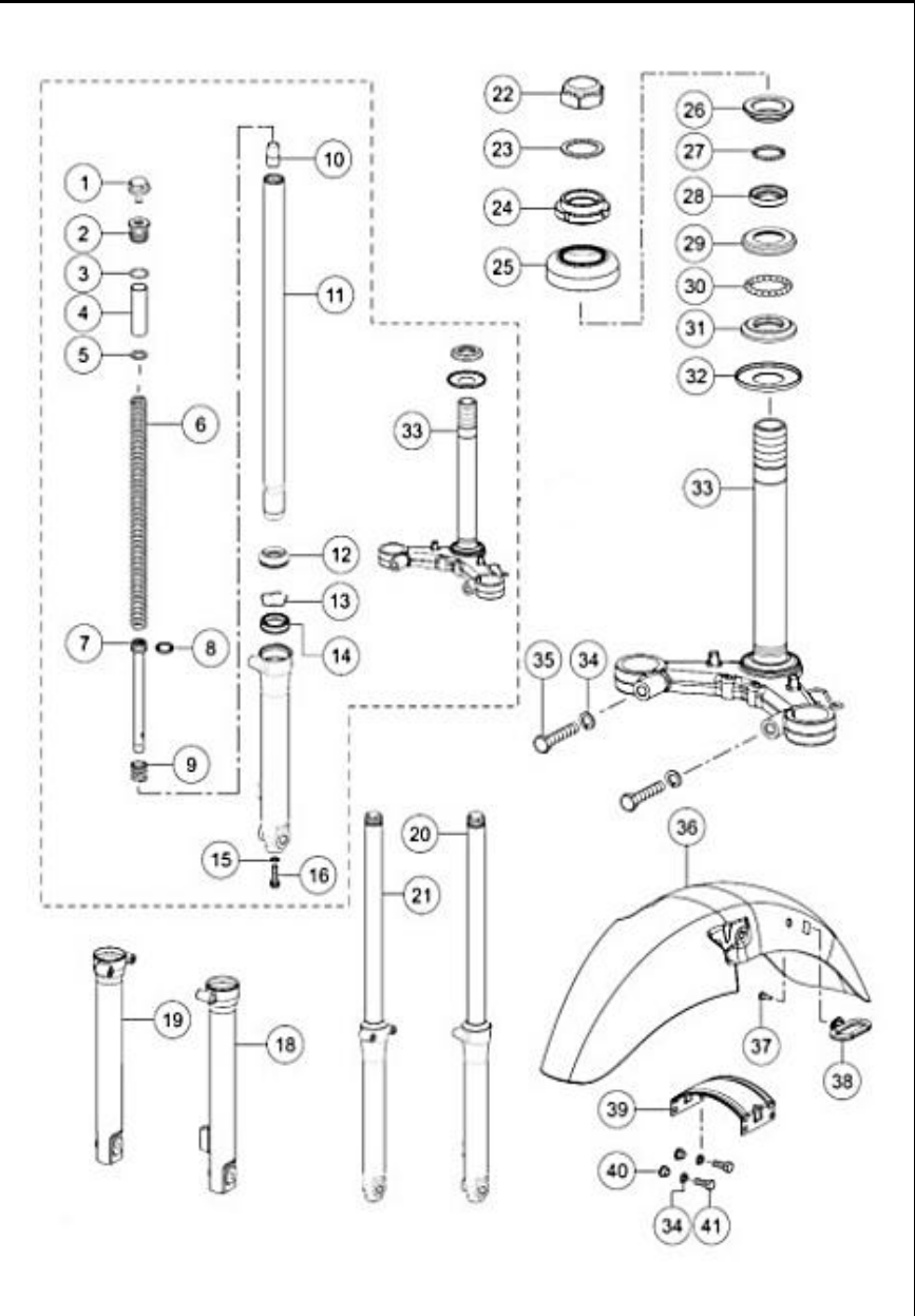
FIGURA N° 27: SUSPENSIÓN DELANTERA (1/2)
