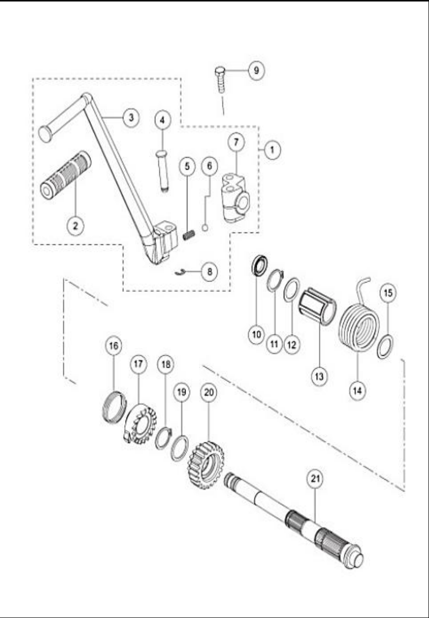
FIGURA N° 10: PEDAL CRANK
