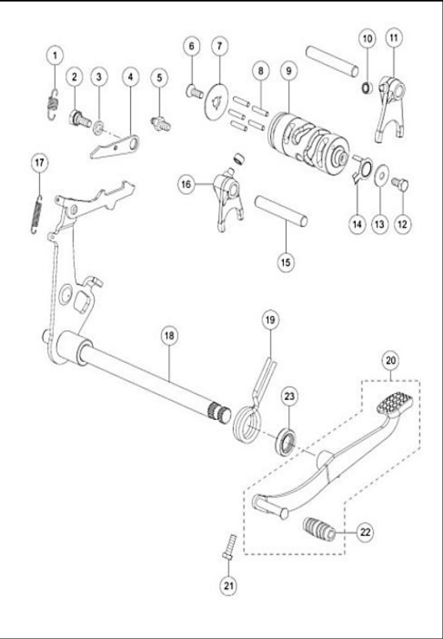
FIGURA N° 9: SELECTOR CAMBIOS
