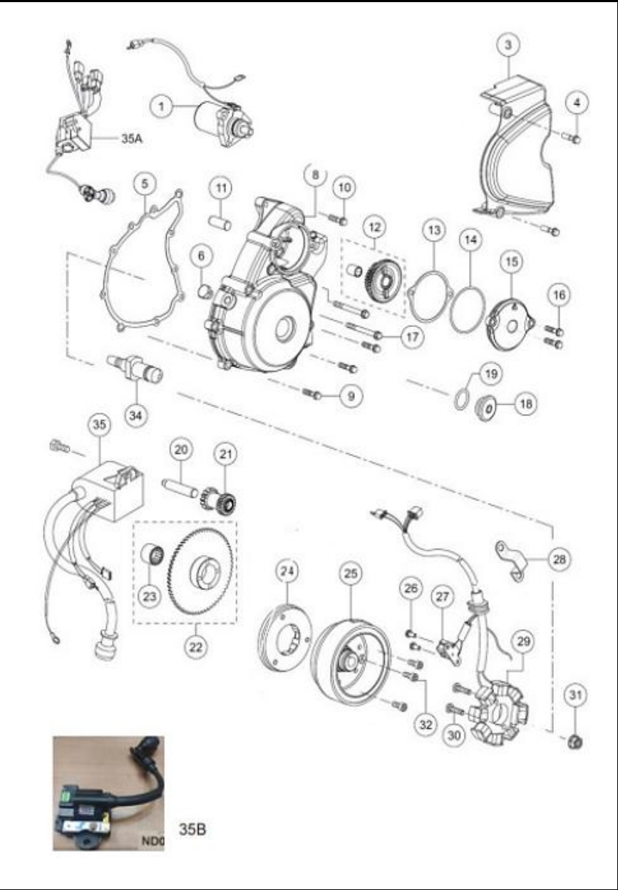
FIGURA N° 8: CUBIERTA VOLANTE (ES) (1/2)
