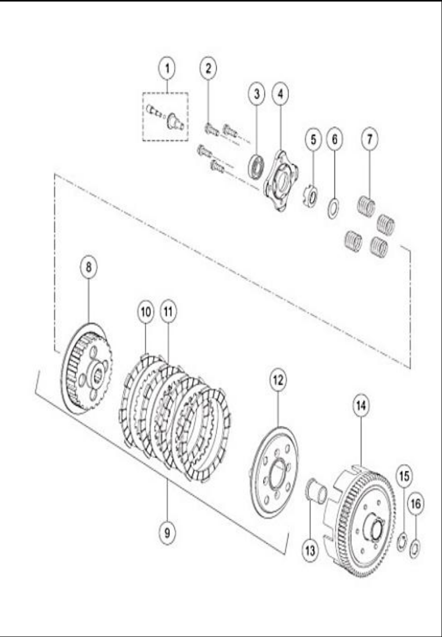
FIGURA N° 6: CLUTCH
