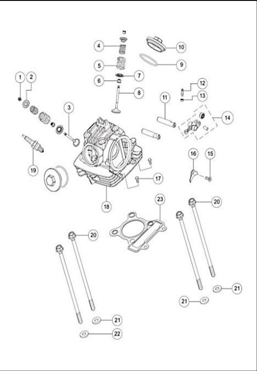
FIGURA N° 1: CULATA
