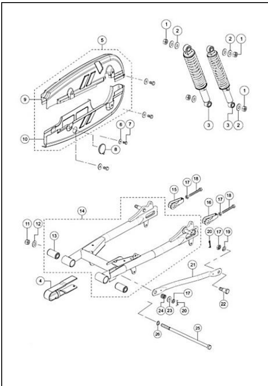
FIGURA N° 35: BRAZO OSCILANTE / AMORTIGUADOR
