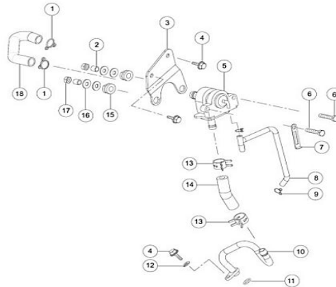
FIGURA N° 14: INYECCIÓN AIRE SECUNDARIO
