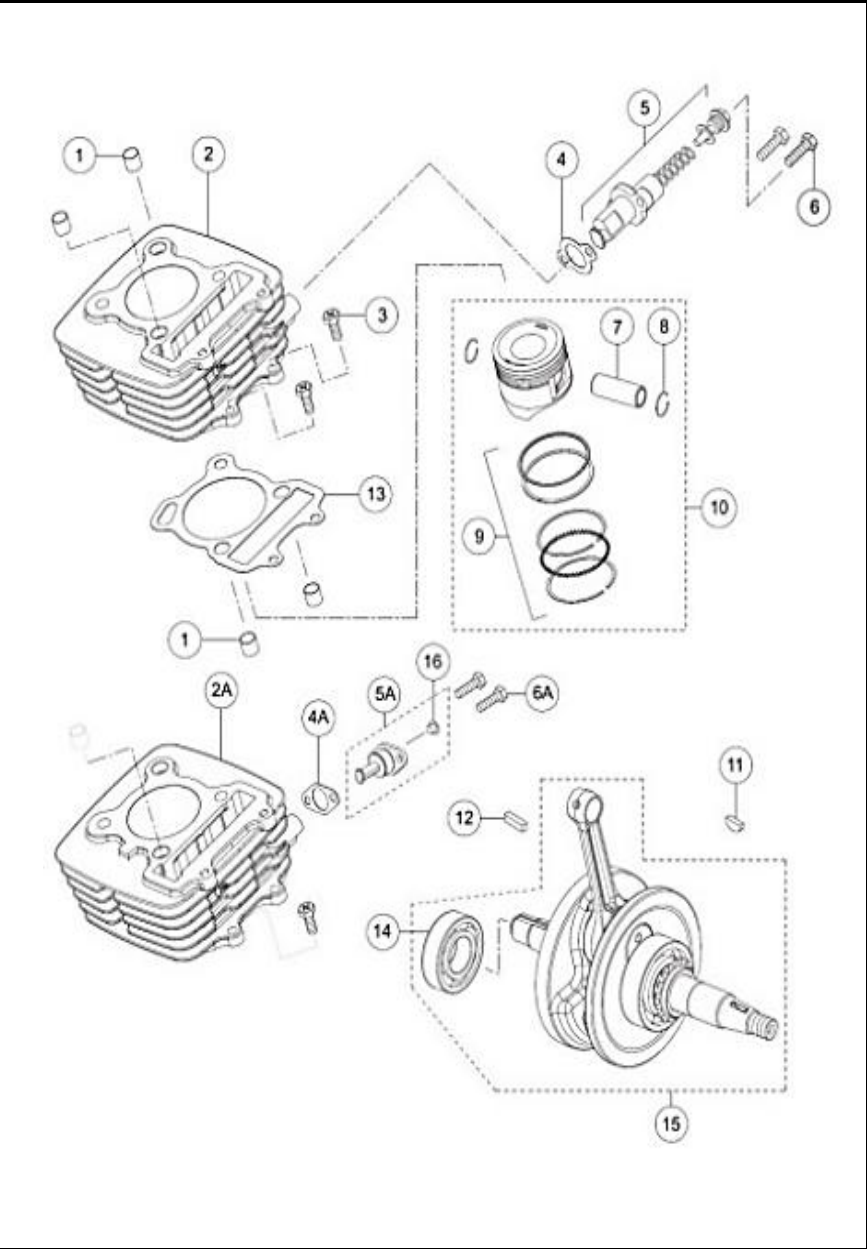
FIGURA N° 3: CILINDRO Y PISTÓN
