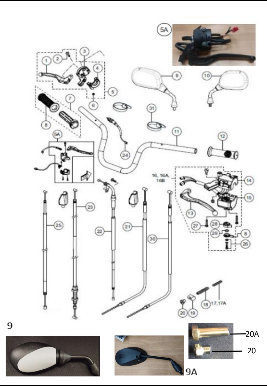
FIGURA N° 20: MANUBRIO (1/2)
