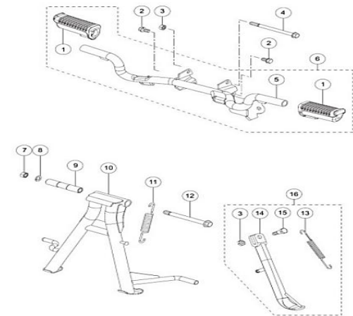
FIGURA N° 18: REPOSAPIE DELANTERO
