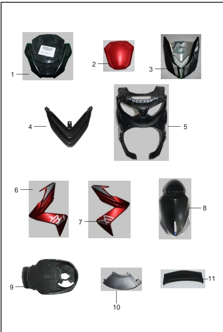
FIGURA N° 9: CUBIERTAS FRONTALES
