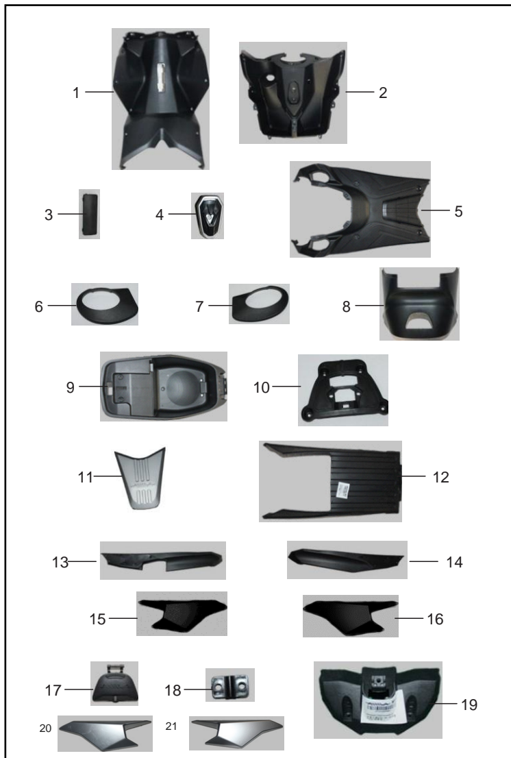
FIGURA N° 10: CUBIERTAS CENTRALES
