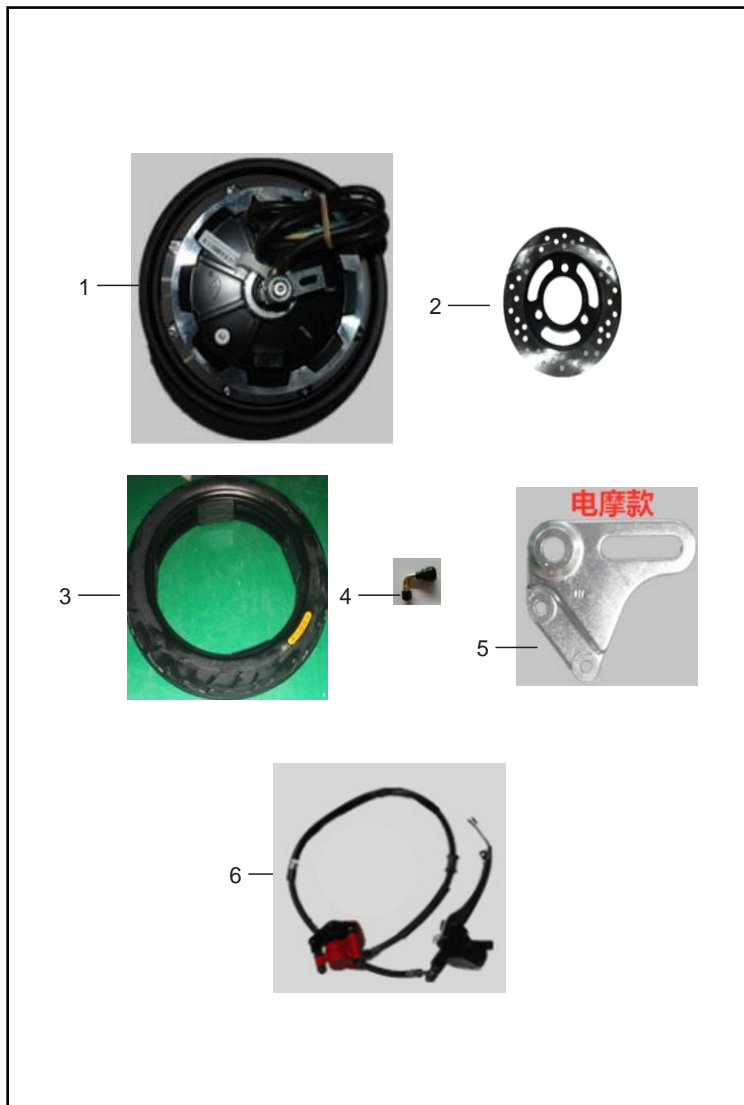
FIGURA N° 5: RUEDA TRASERA - FRENO TRASERO
