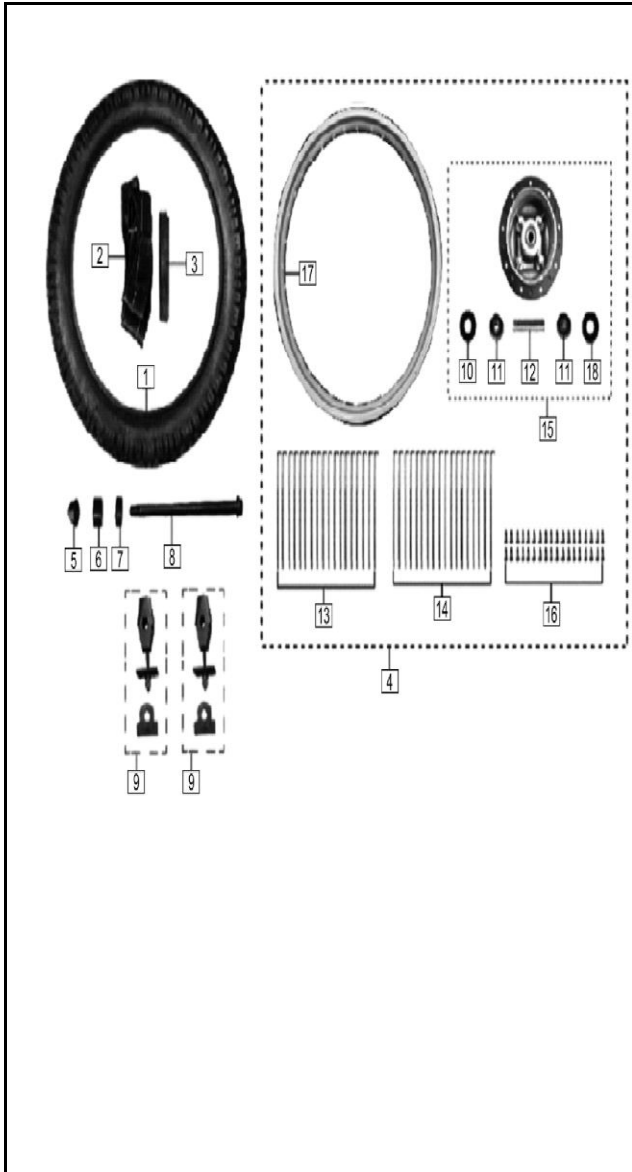
FIGURA N° 37: RUEDA TRASERA
