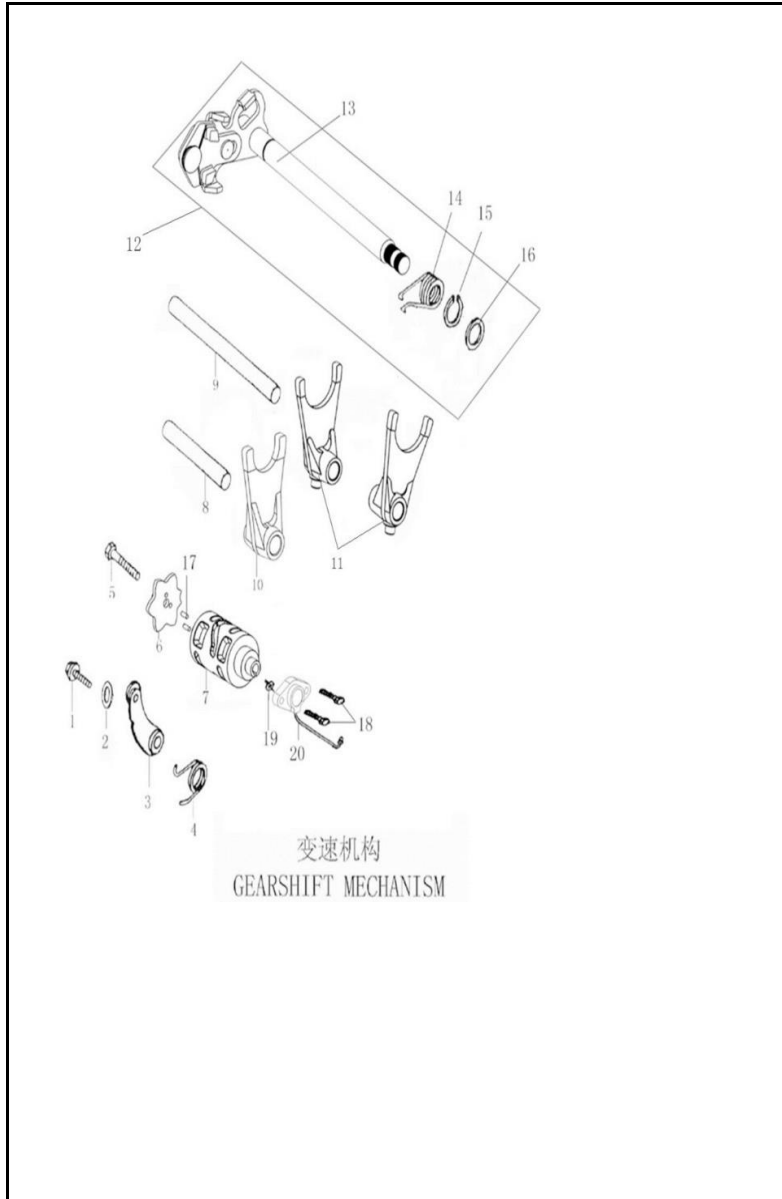
FIGURA N° 9: EJE CAMBIOS - EJE SELECTOR CAMBIOS
