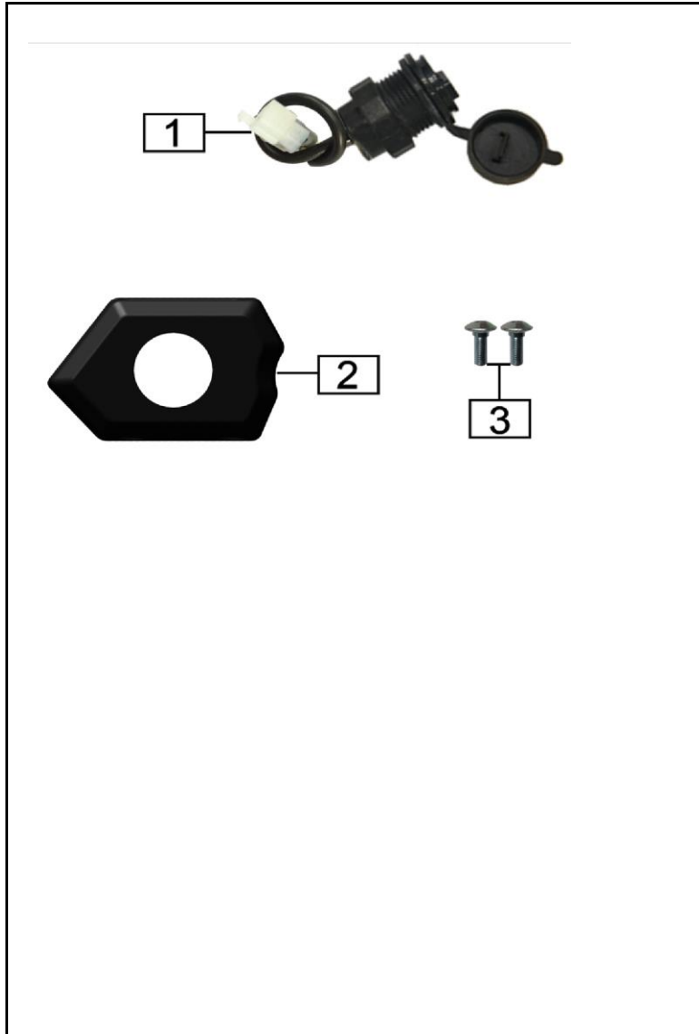
FIGURA N° 47: CARGADOR MOVIL
