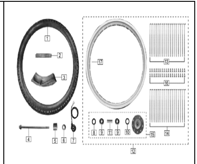
FIG. N° 33 RUEDA DELANTERA
