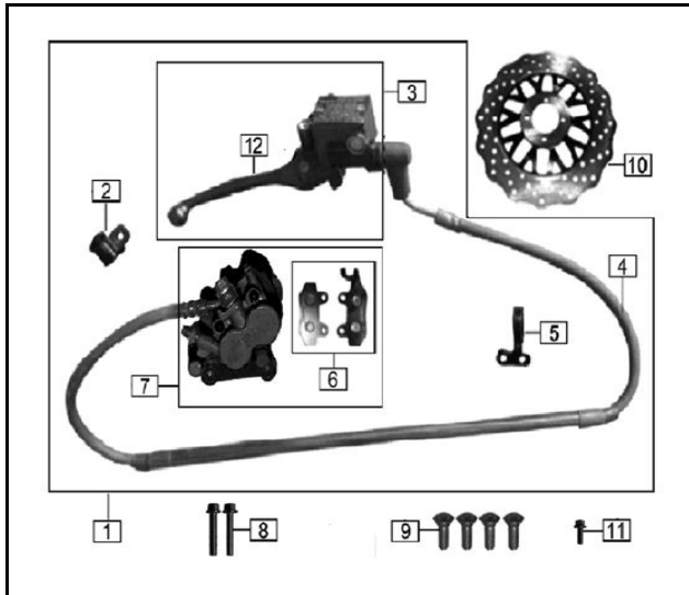
FIG. N° 31 BOMBA FRENO DELANTERO
