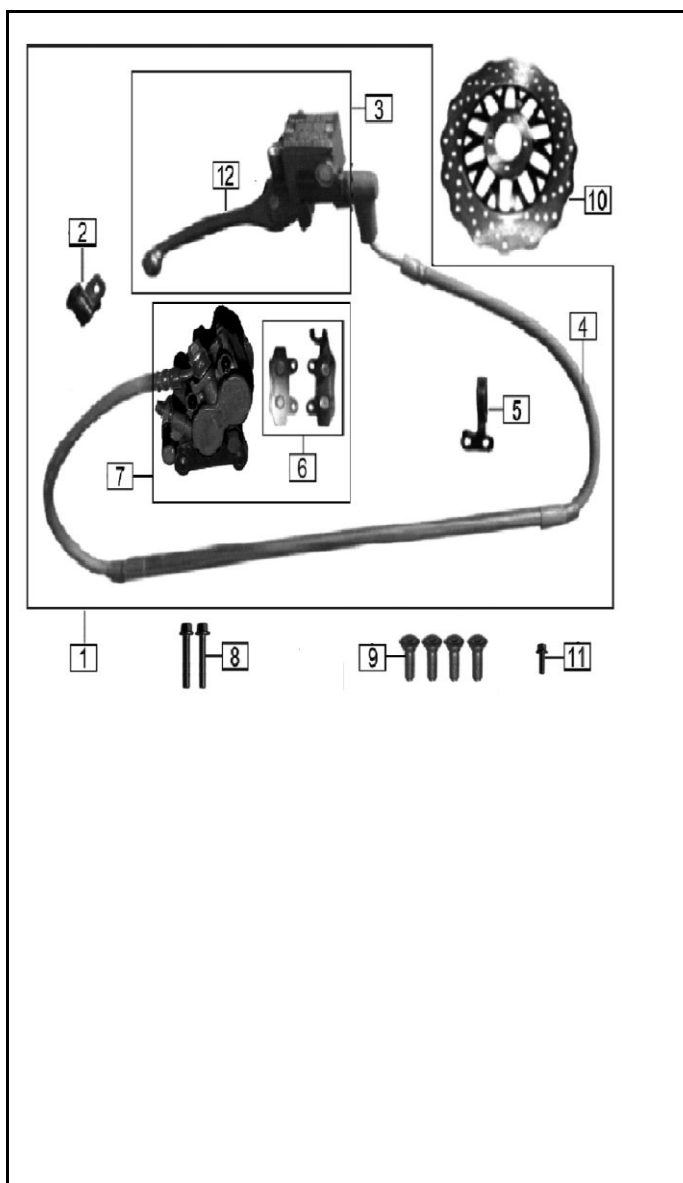
FIGURA N° 34: BOMBA FRENO DELANTERO
