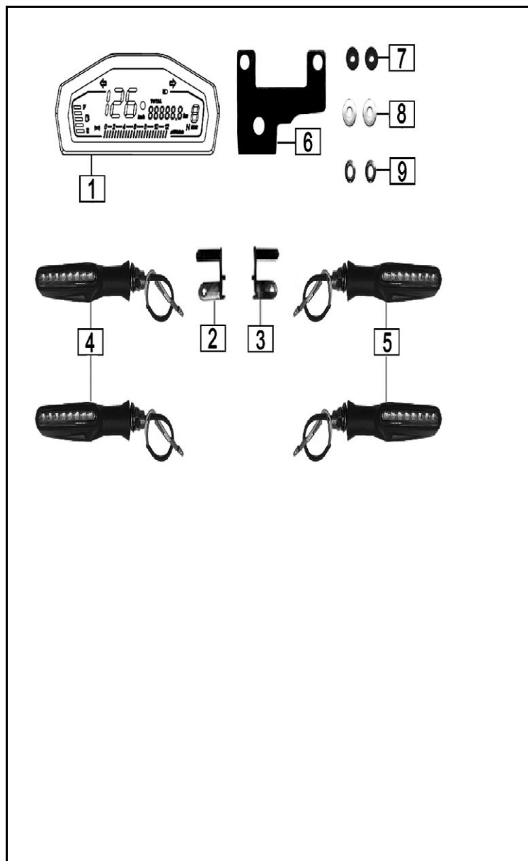
FIGURA N° 14: VELOCIMETRO - DIRECCIONALES DELANTERAS
