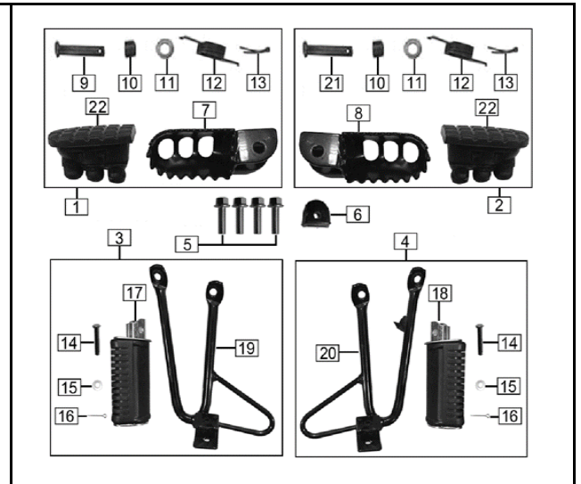
FIG. Nº 27: REPOSAPIE CONDUCTOR - REPOSAPIE PASAJERO
