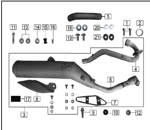
FIG. Nº 25: SILENCIADOR
