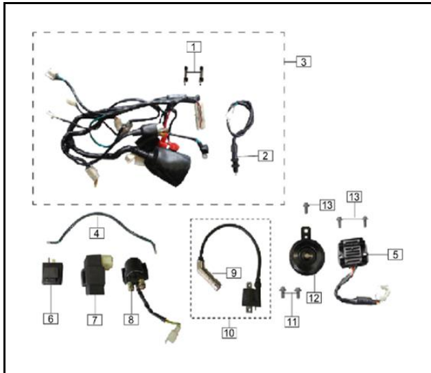
FIG. Nº 19: SISTEMA ELECTRICO
