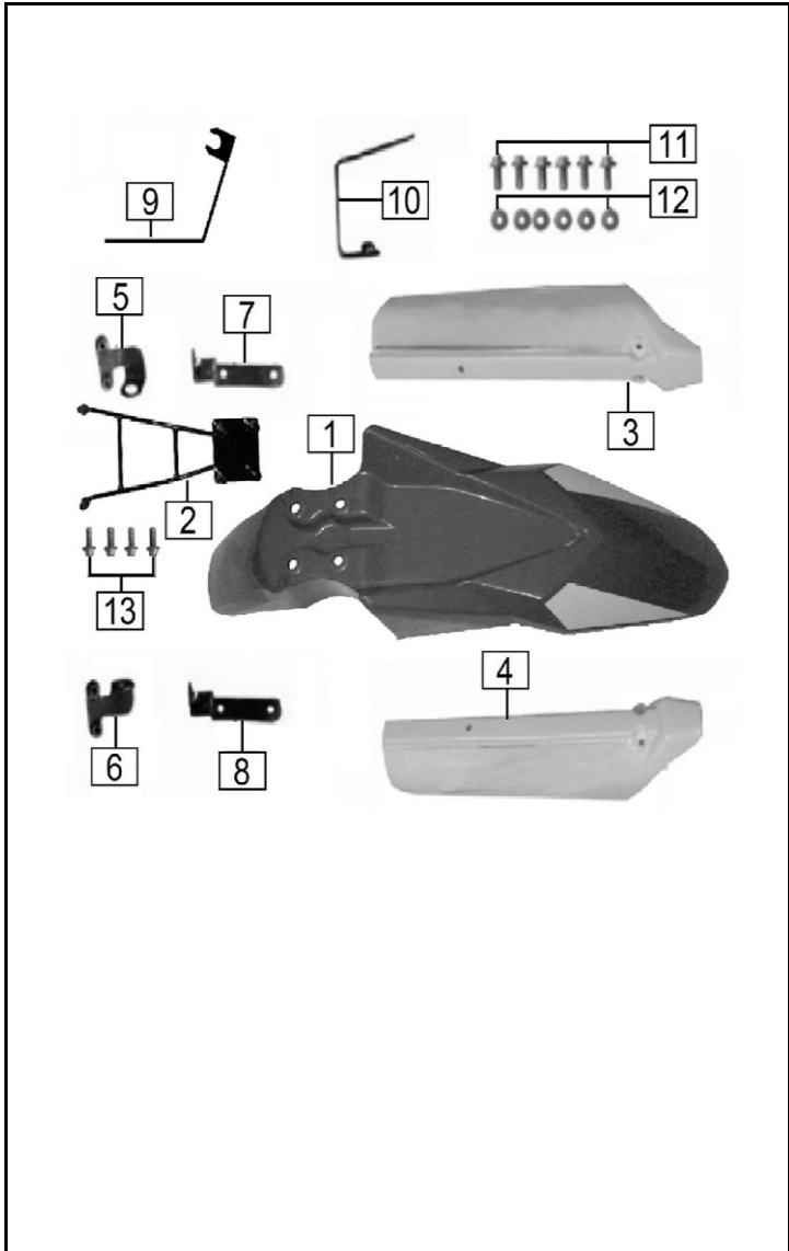
FIGURA N° 33: GUARDABARRO DELANTERO
