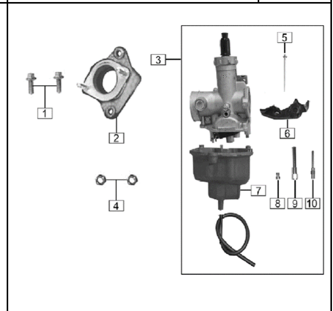
FIG. Nº 24: CARBURADOR
