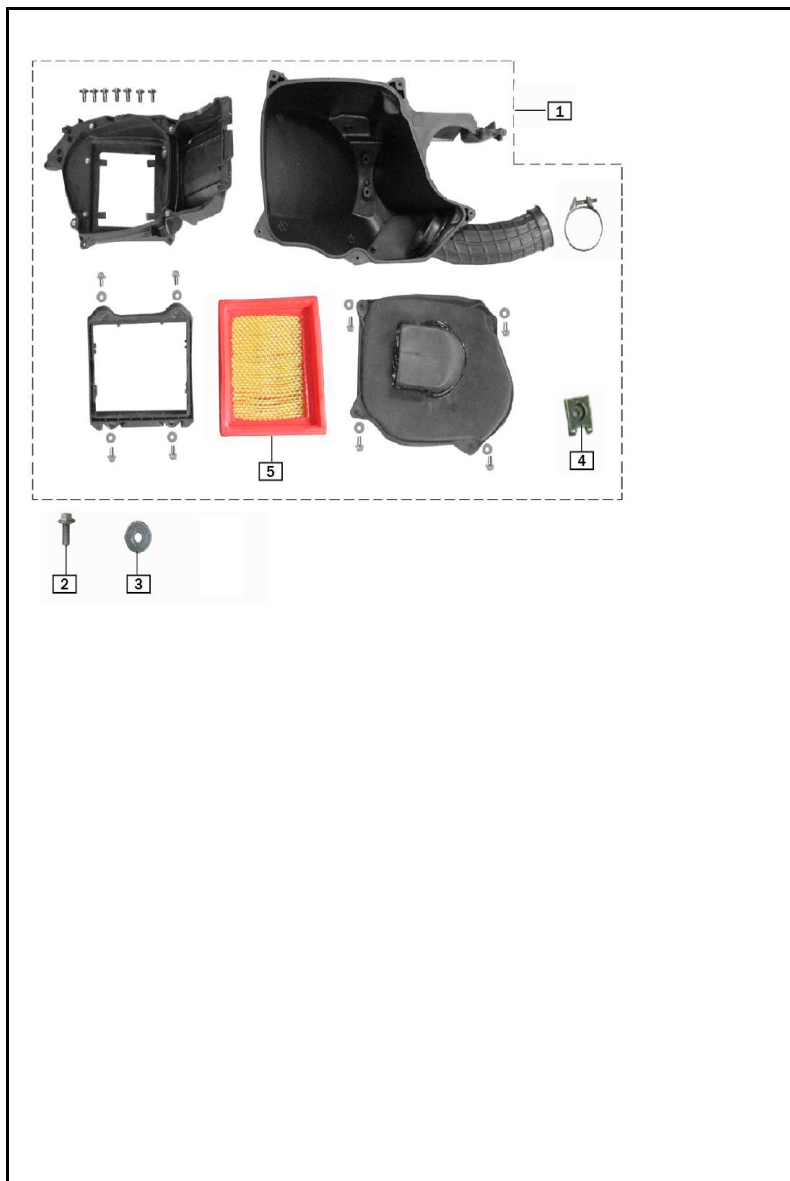
FIGURA N° 26: CAJA FILTRO AIRE
