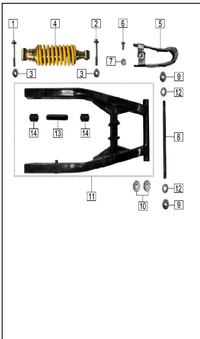
FIGURA N° 38: BRAZO OSCILANTE - MONOSHOCK
