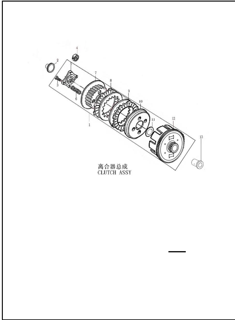
FIGURA N° 4: CLUTCH
