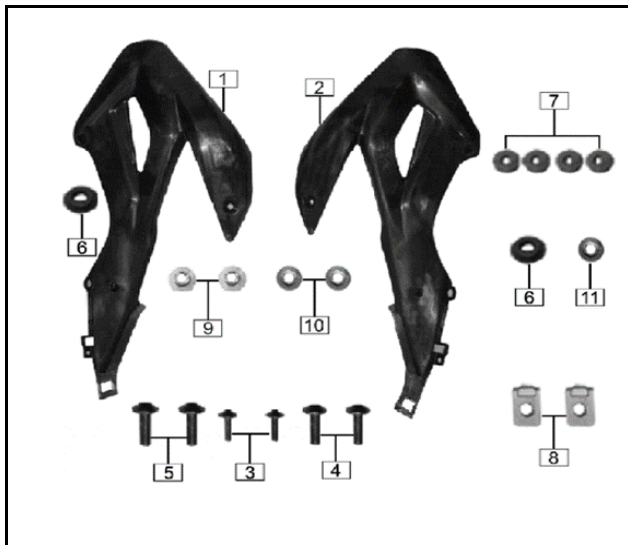
FIG. Nº 37 ENFOCADORES
