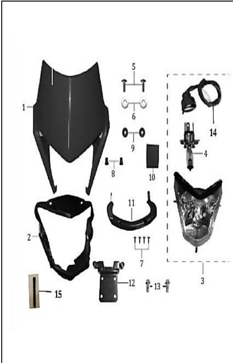
FIGURA N° 13: FAROLA - CARENAJE FAROLA CAMO PRO
