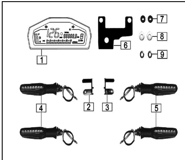
FIG. Nº 13: VELOCIMETRO - DIRECCIONALES DELANTERAS
