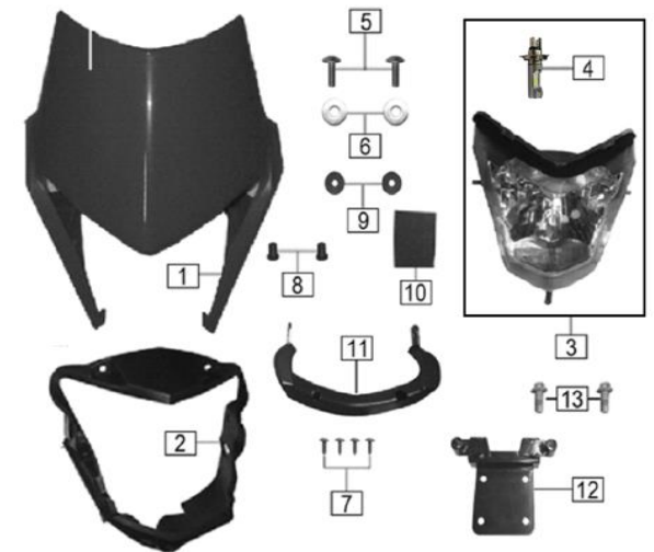
FIG. Nº 12: FAROLA - CARENAJE FAROLA
