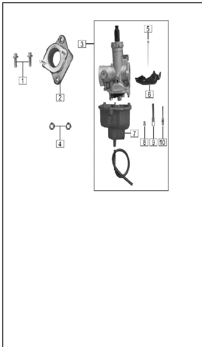
FIGURA N° 27: CARBURADOR
