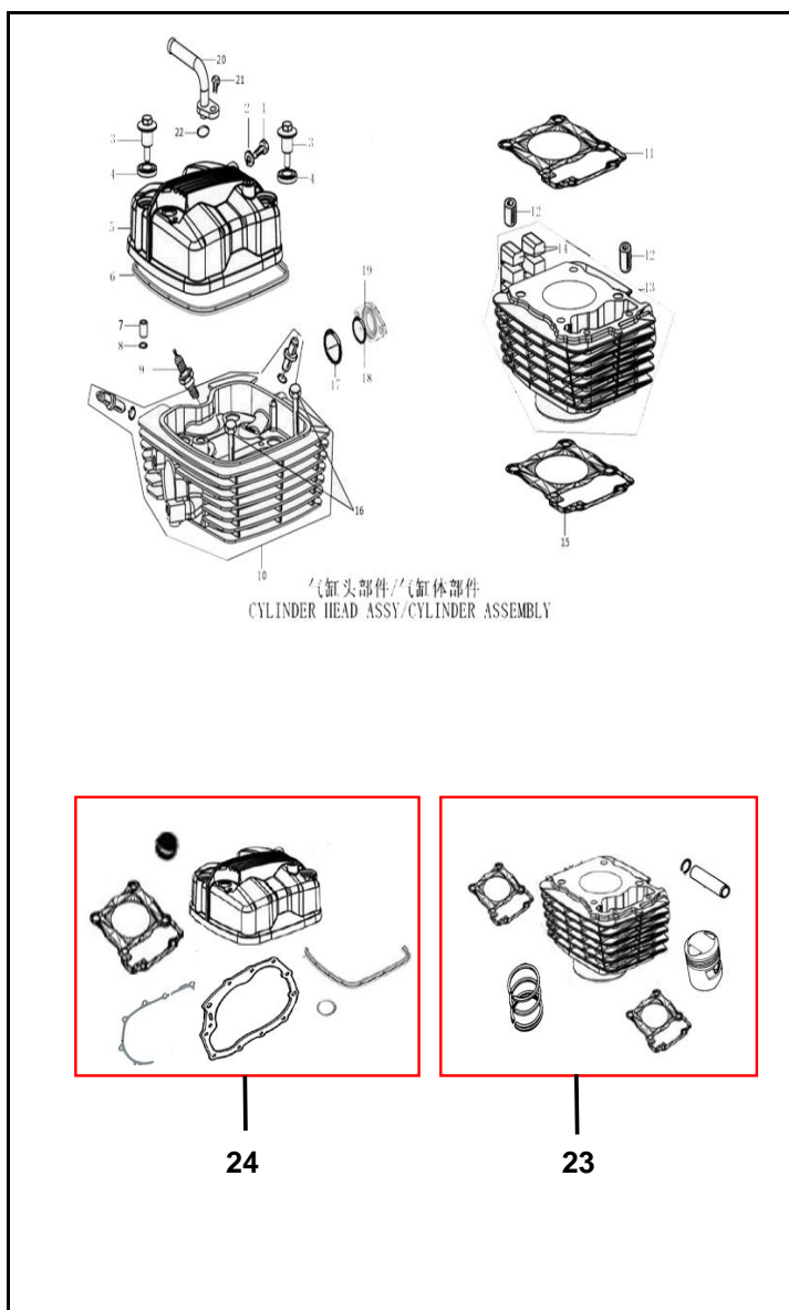
FIGURA N° 1: CULATA - CILINDRO MOTOR
