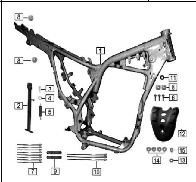
FIG. Nº 41 COMPLEMENTOS CHASIS - GATO LATERAL
