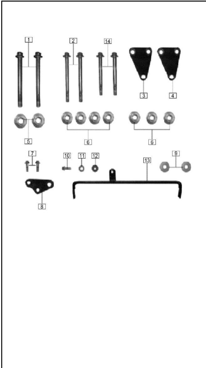
FIGURA N° 45: SOPORTE MOTOR
