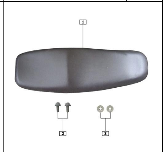
FIG. Nº 18: SILLIN
