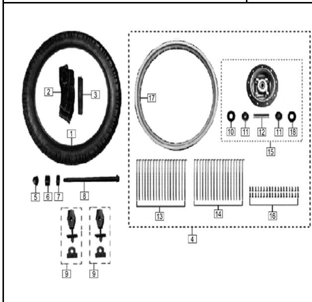
FIG. N° 34 RUEDA TRASERA
