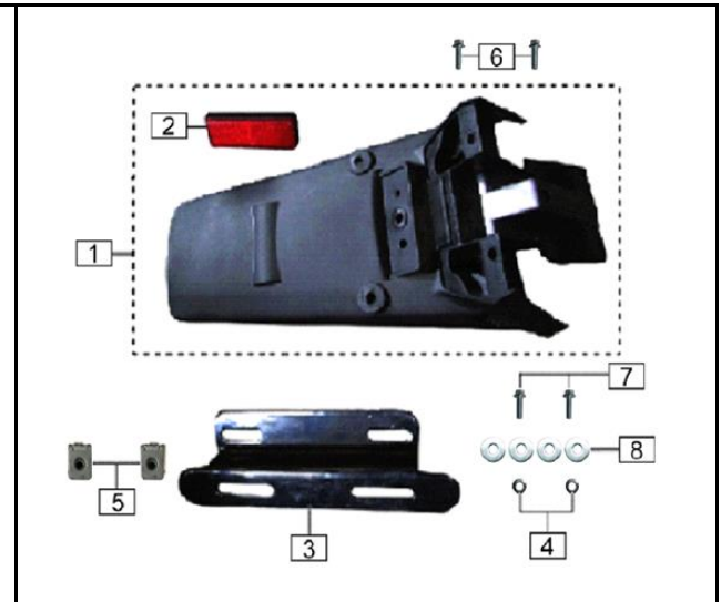
FIG. Nº 21: GUARDABARRO TRASERO
