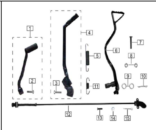
FIG. Nº 26: PEDAL CAMBIOS - PEDAL FRENO - PEDAL CRANK
