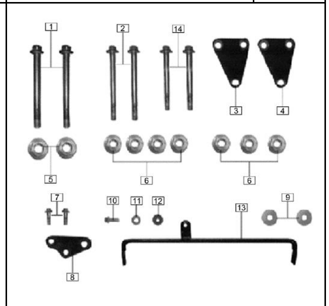
FIG. Nº 42 SOPORTE MOTOR
