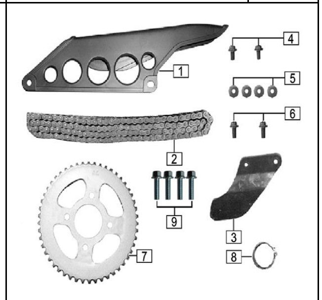
FIG. N° 36 SPROCKET - CADENA
