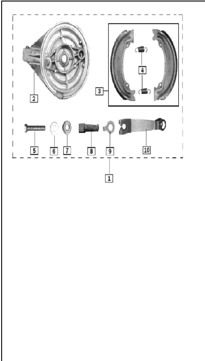
FIGURA N° 35: PORTA BANDAS TRASERO
