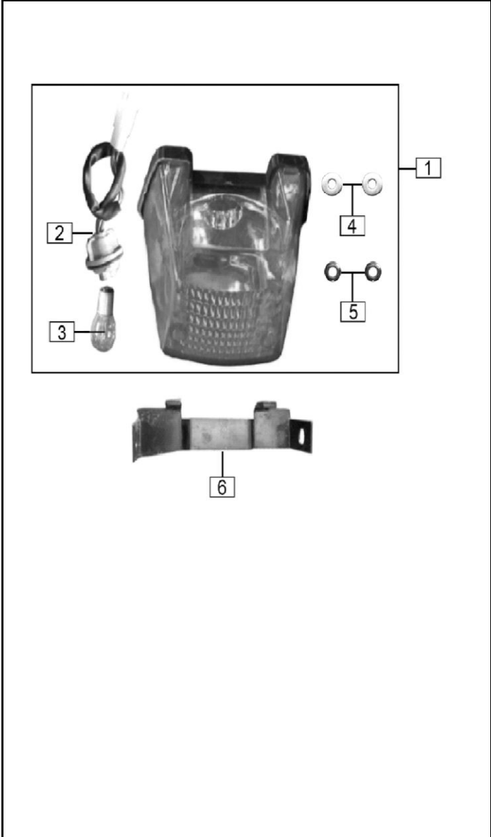
FIGURA N° 25: STOP - DIRECCIONALES TRASERAS
