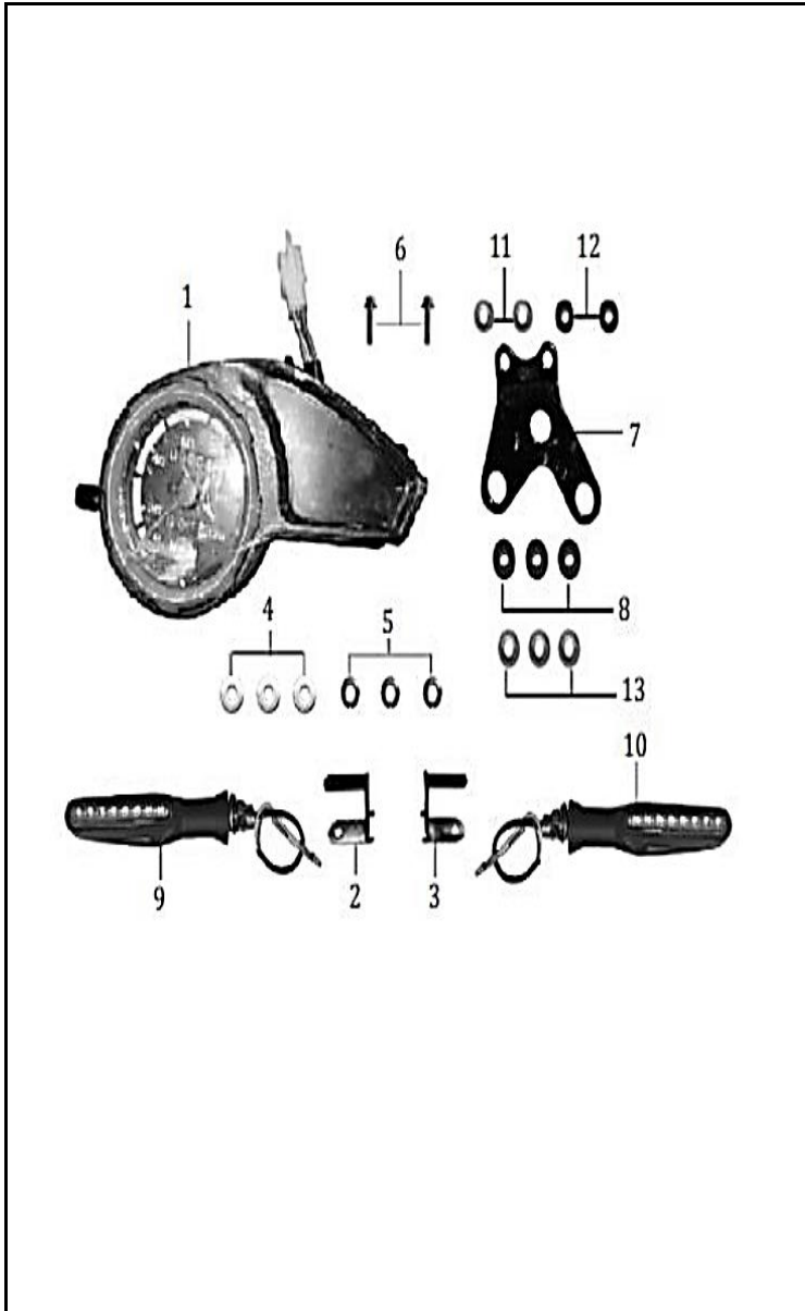
FIGURA N° 15: VELOCIMETRO - DIRECCIONALES DELANTERAS CAMO PRO
