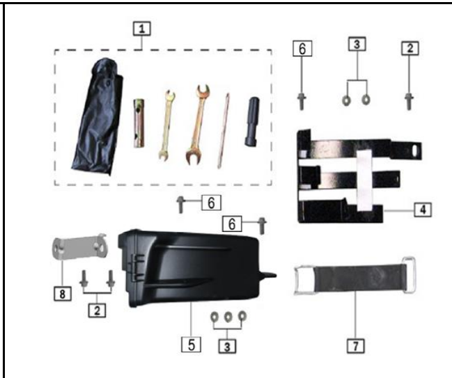
FIG. Nº 20: CAJA HERRAMIENTAS
