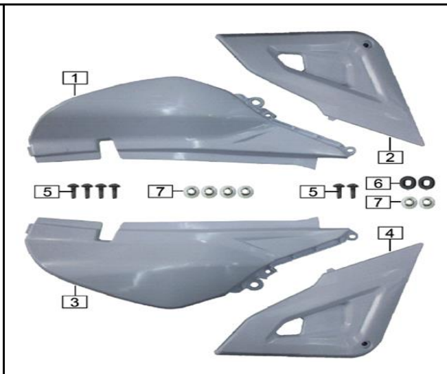
FIG. Nº 38 TAPA LATERAL - CUBIERTA SILLIN
