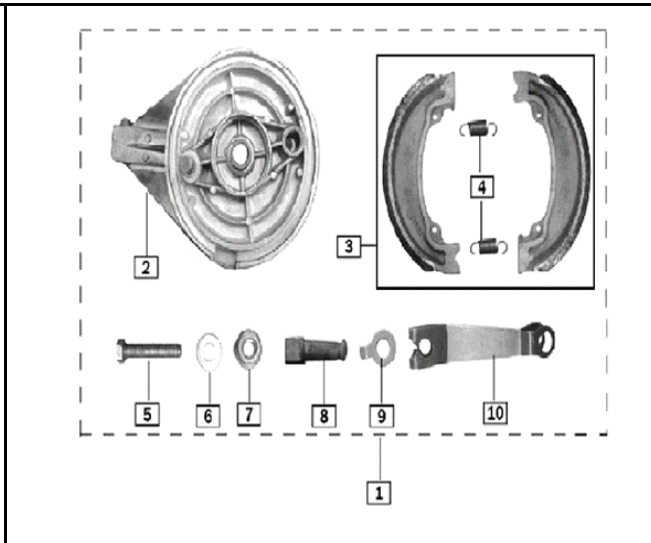
FIG. N° 32 PORTA BANDAS TRASERO
