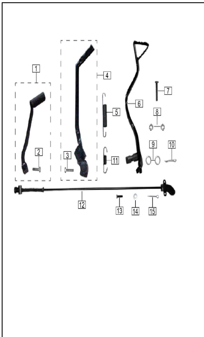
FIGURA N° 29: PEDAL CAMBIOS - PEDAL FRENO - PEDAL CRANK
