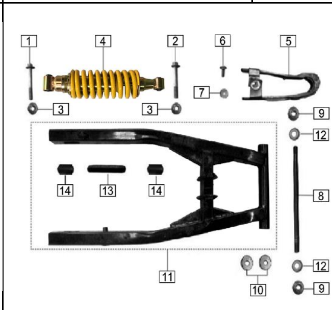
FIG. N° 35 BRAZO OSCILANTE - MONOSHOCK
