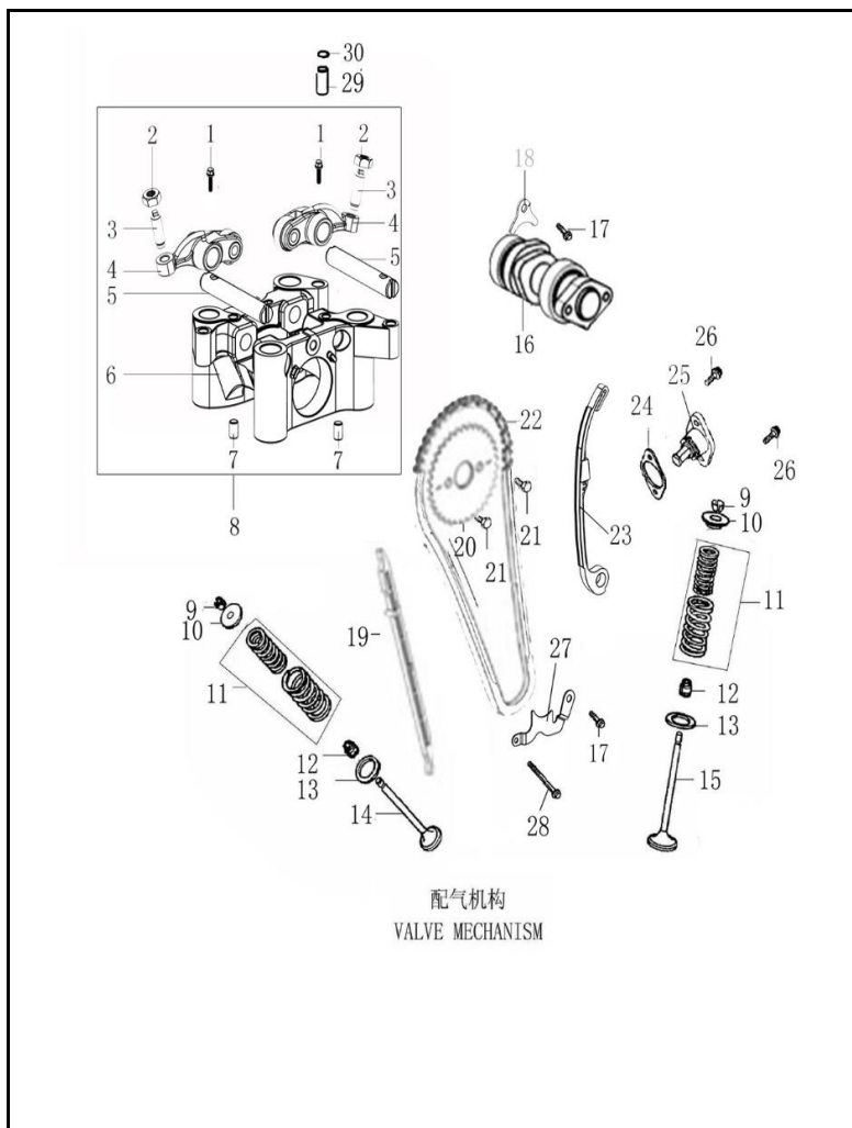
FIGURA N° 2: EJE LEVAS - VALVULAS (2/1)
