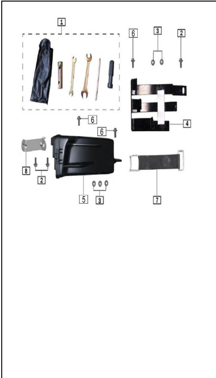
FIGURA N° 23: CAJA HERRAMIENTAS
