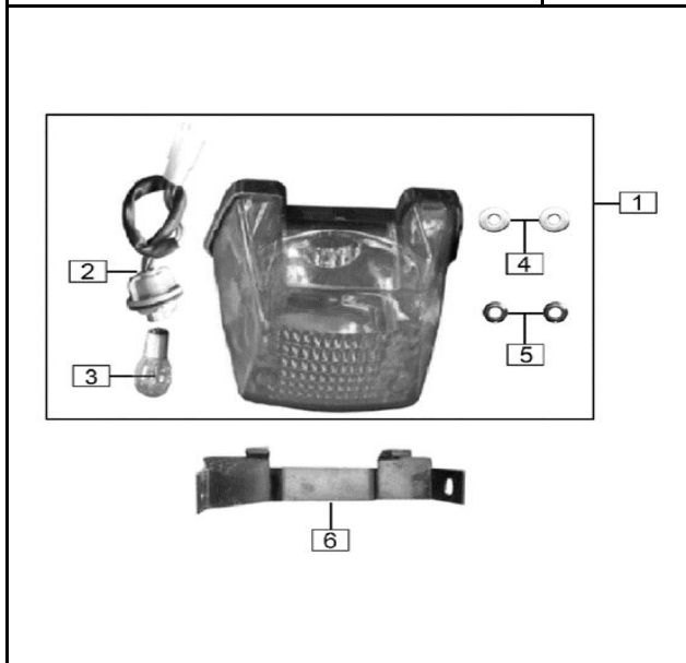
FIG. Nº 22: STOP - DIRECCIONALES TRASERAS
