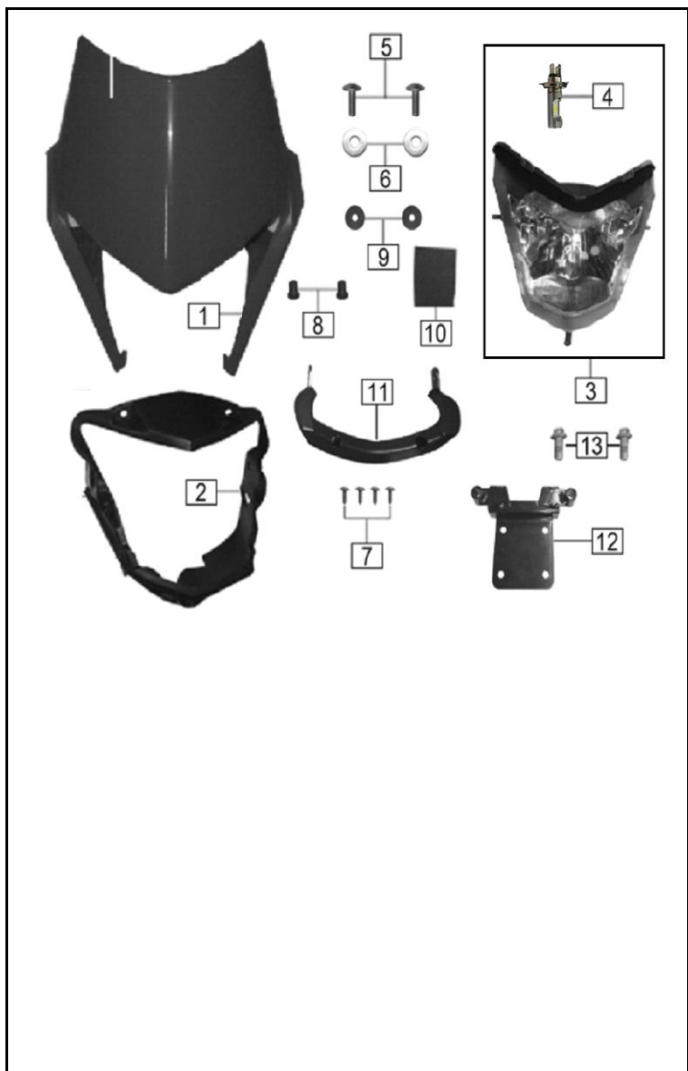
FIGURA N° 12: FAROLA - CARENAJE FAROLA
