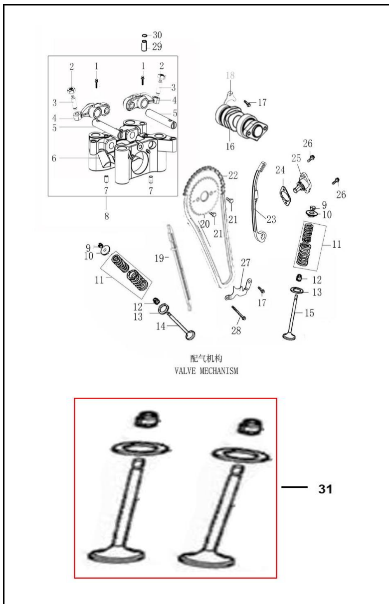
FIGURA N° 2: EJE LEVAS - VALVULAS (2/2)
