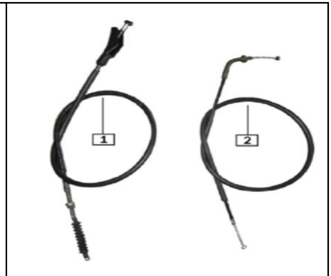
FIG. Nº 15: CABLES
