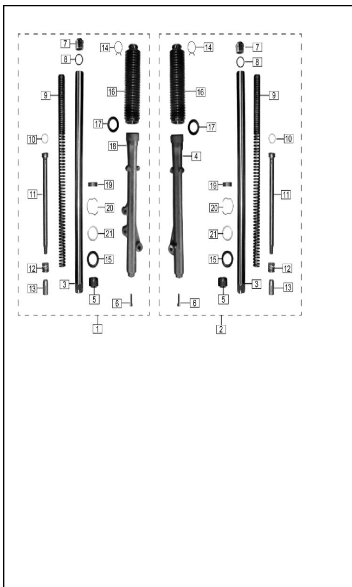
FIGURA N° 32: SUSPENSION DELANTERA
