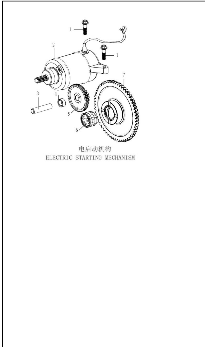
FIGURA N° 11: MOTOR DE ARRANQUE
