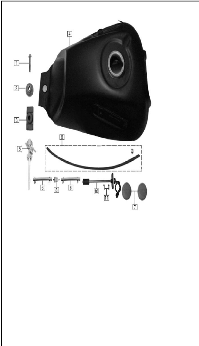
FIGURA N° 20: TANQUE GASOLINA
