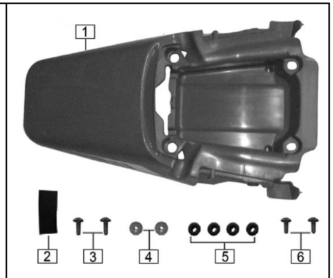
FIG. Nº 39 CUBIERTA STOP
