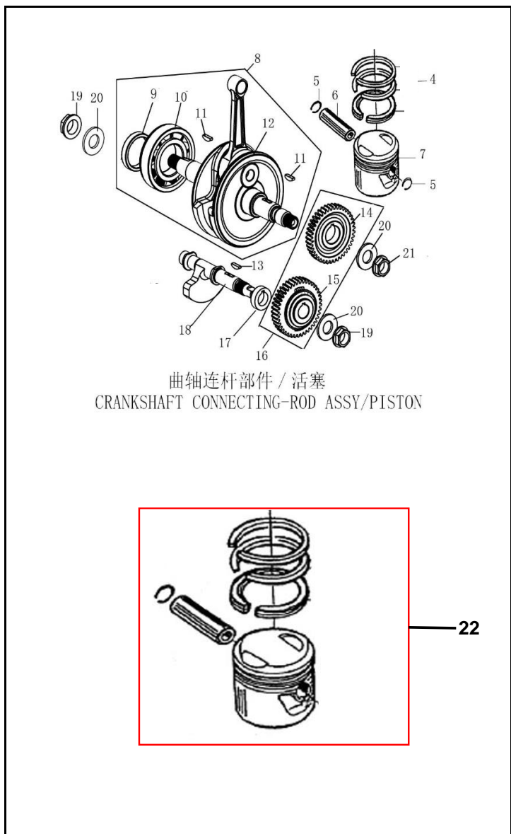
FIGURA N° 7: CIGÜENAL - BALANCEADOR - PISTON
