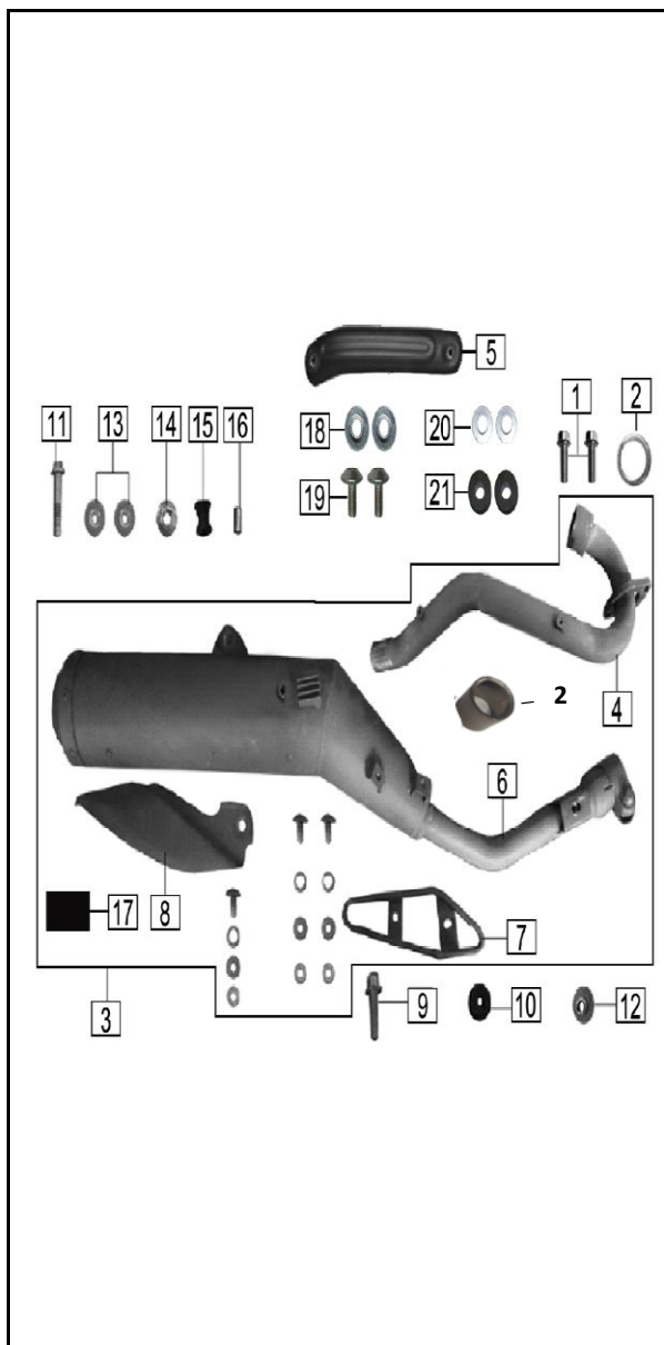
FIGURA N° 28: SILENCIADOR
