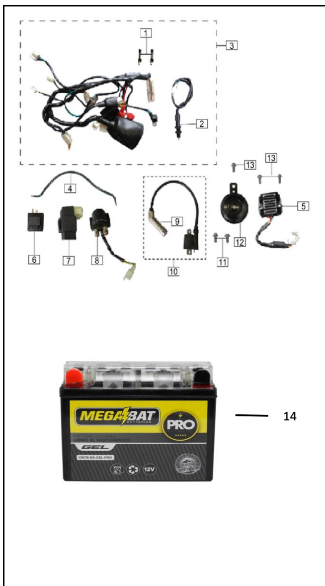
FIGURA N° 22: SISTEMA ELECTRICO
