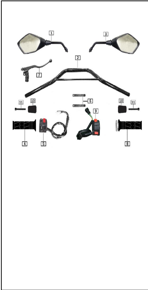
FIGURA N° 18: MANUBRIO - ESPEJOS
