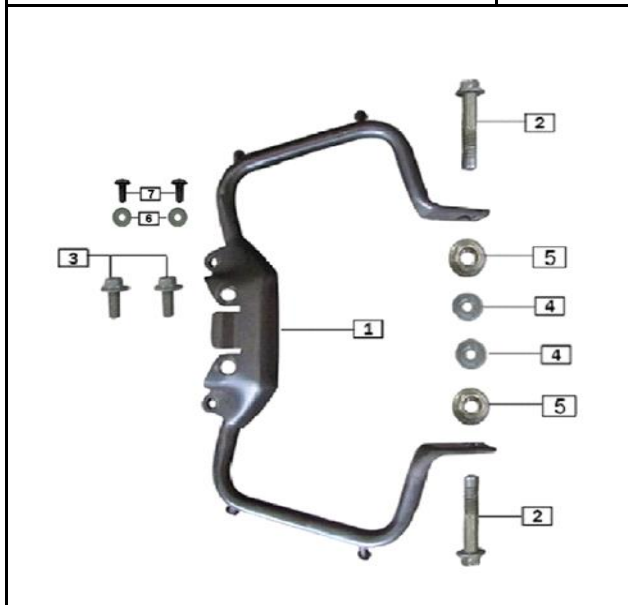
FIG. Nº 40 AGARRADERA PASAJERO
