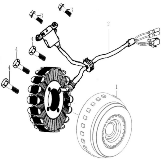
磁电机总成 MAGNETO COMP
