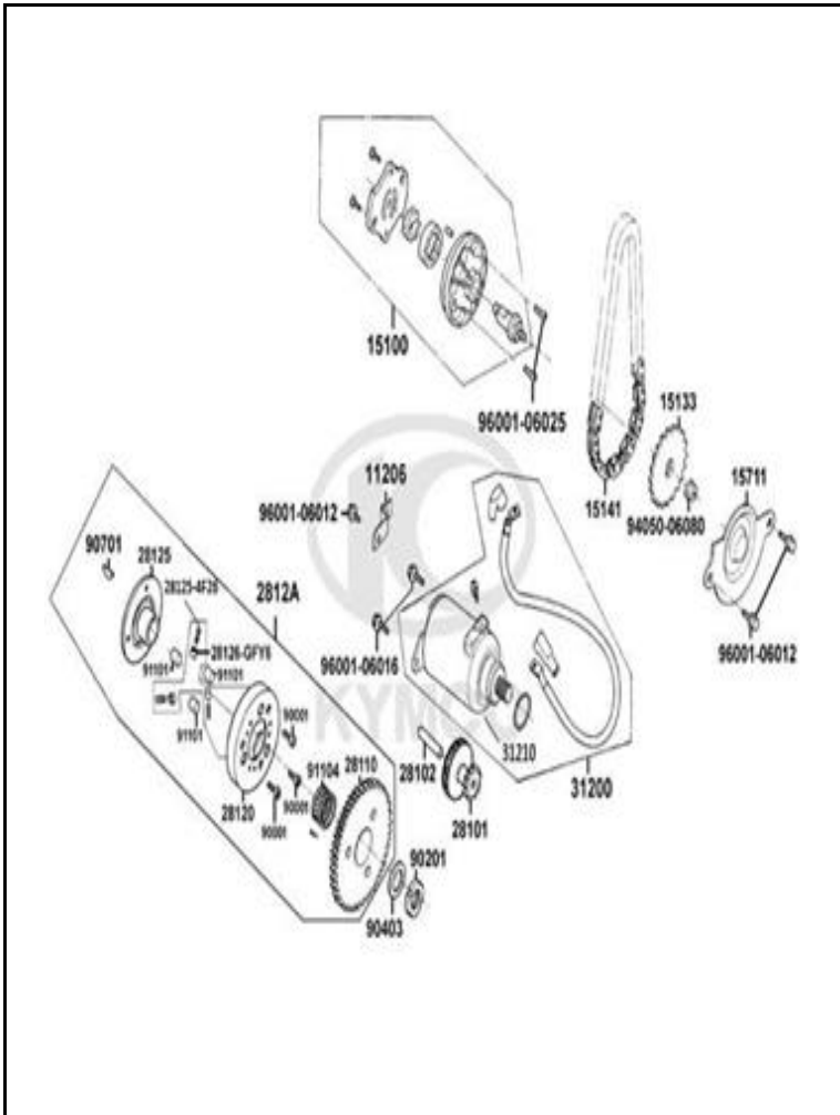
FIGURA N° 6: MOTOR DE ARRANQUE - BOMBA DE ACEITE
