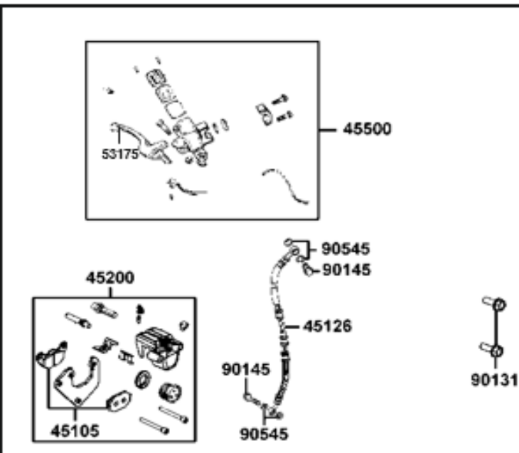
FIGURA 13: BOMBA DE FRENO
