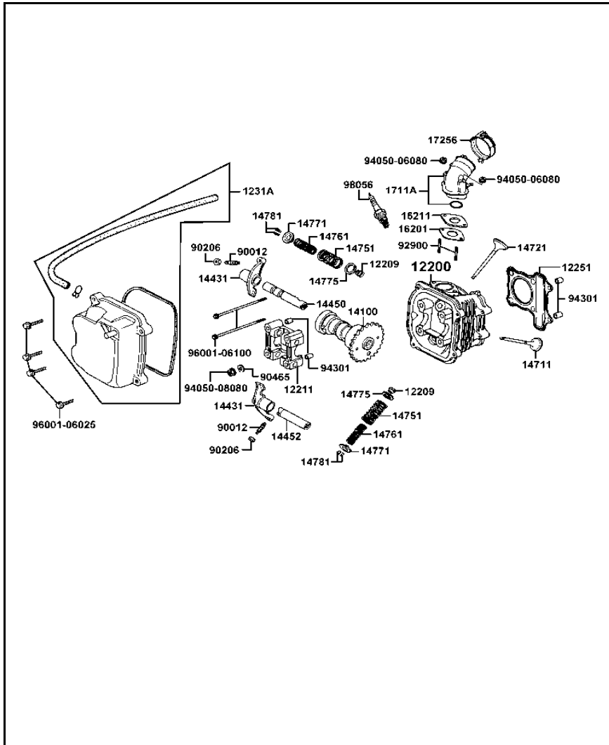
FIGURA N°2: CULATA
