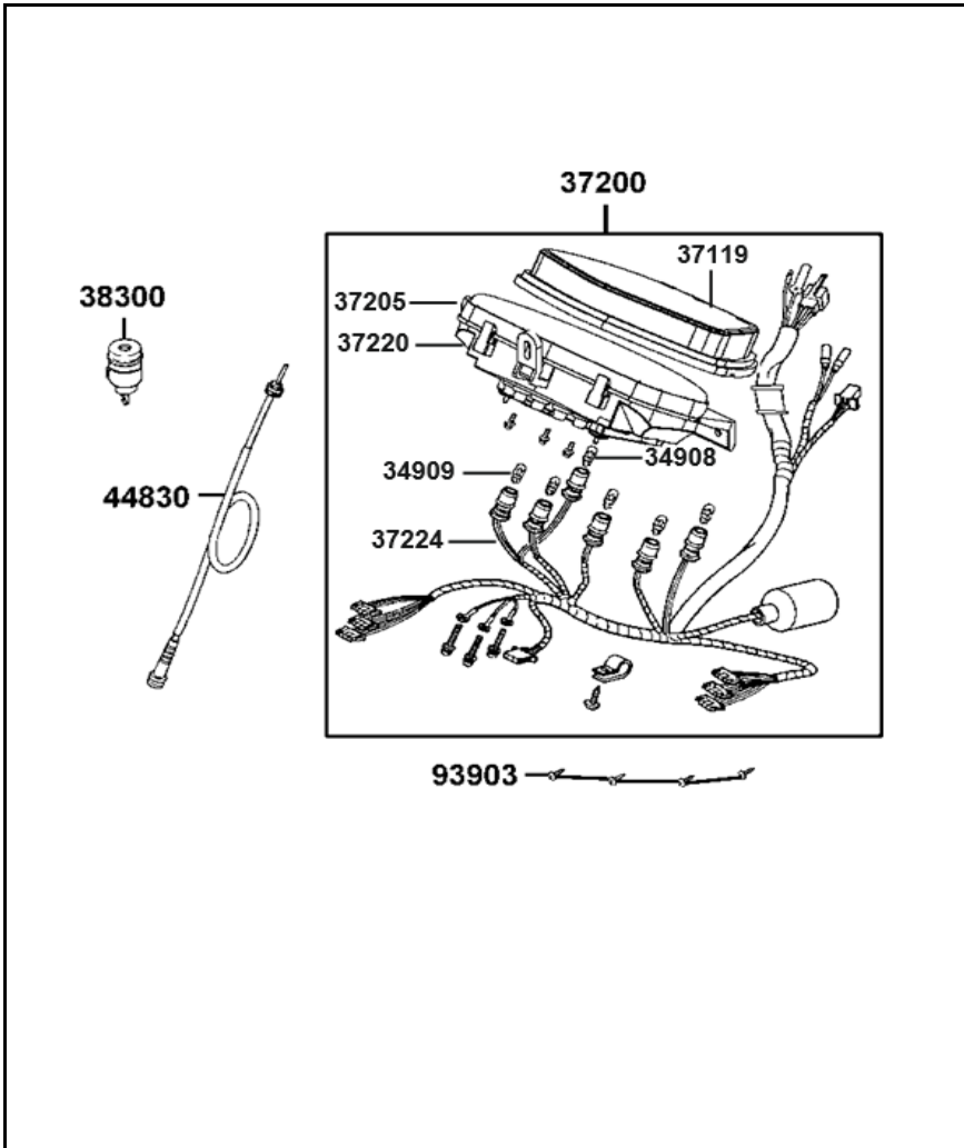
FIGURA N°11: VELOCIMETRO
