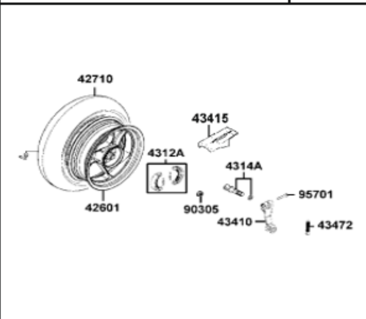
FIGURA 17: RIN TRASERO
