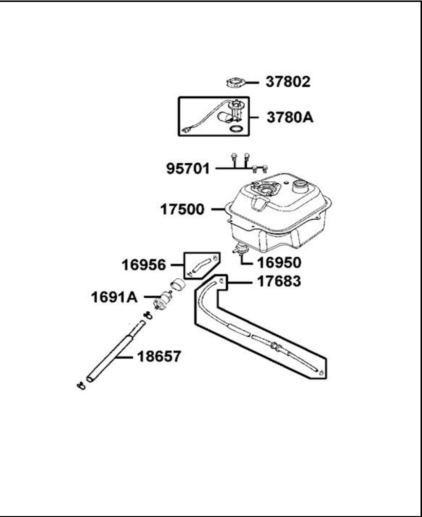
FIGURA N°19: TANQUE DE COMBUSTIBLE
