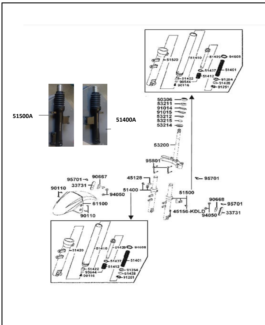
FIGURA N°15: SUSPENSIÓN DELANTERA
