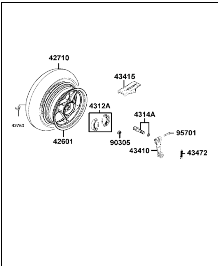
FIGURA N°17: RIN TRASERO
