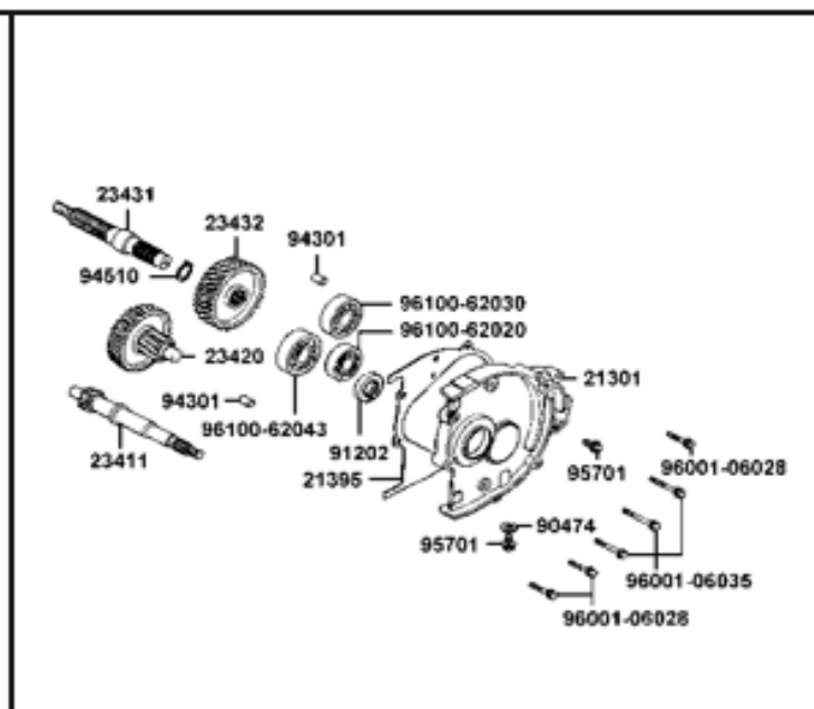
FIGURA 8: TRANSMISIÓN
