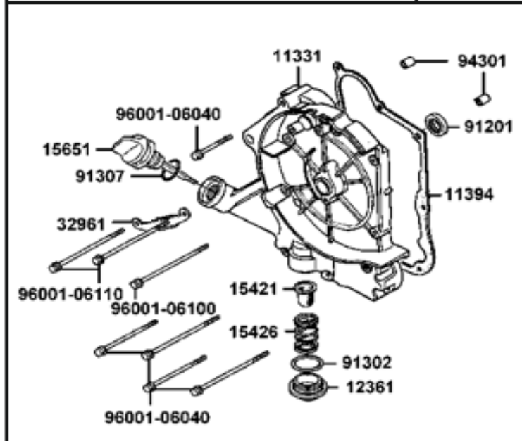
FIGURA 4: CUBIERTA MOTOR DERECHA
