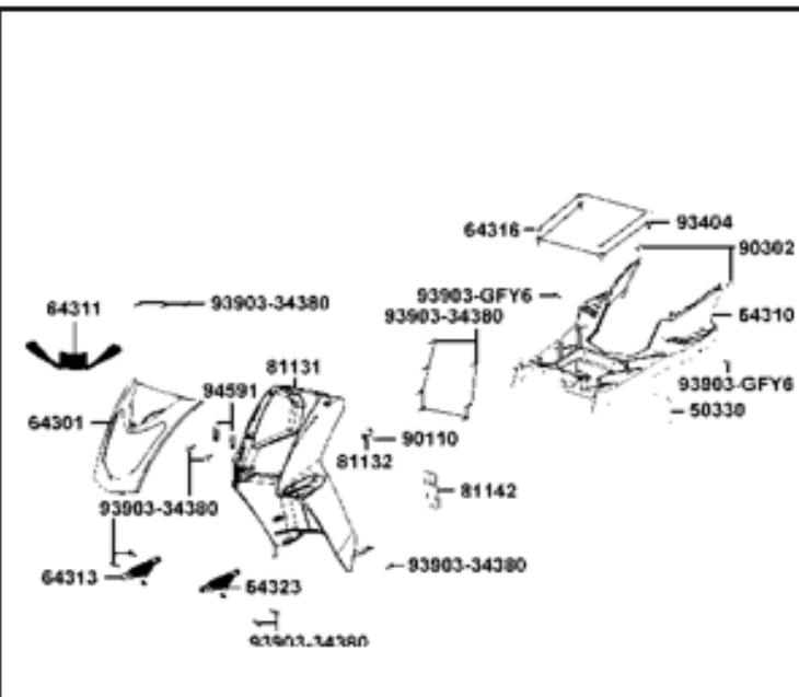
FIGURA 14: CUBIERTAS
