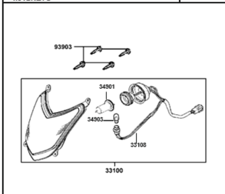
FIGURA 10: FAROLA
