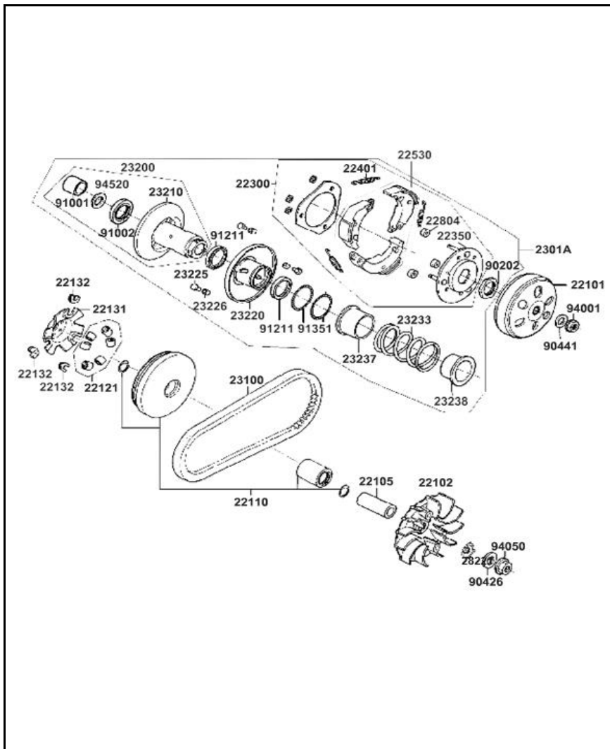
FIGURA N°5: CLUTCH CENTRIFUGO
