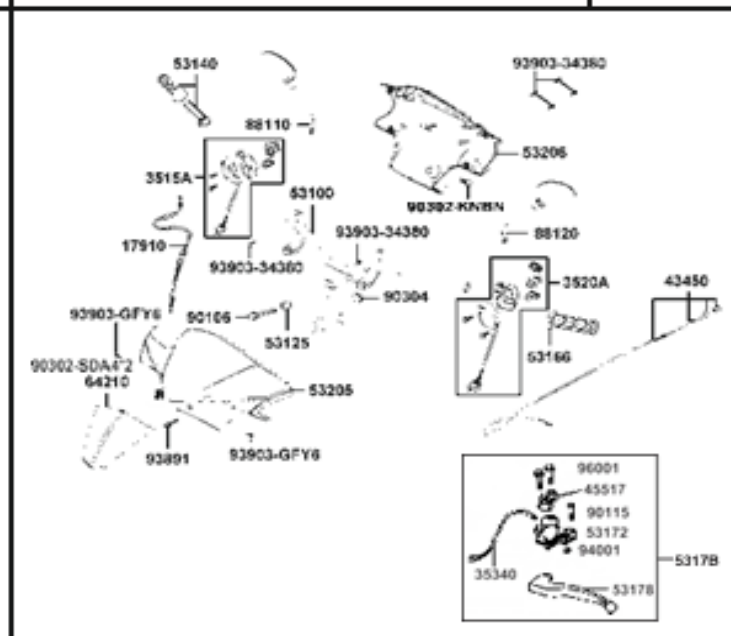
FIGURA 12: MANUBRIO - CUBIERTAS MANUBRIO
