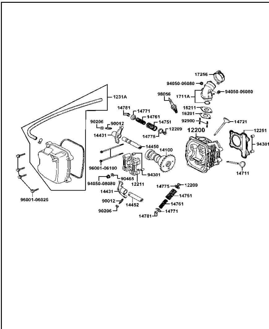
FIGURA N°2: CULATA
