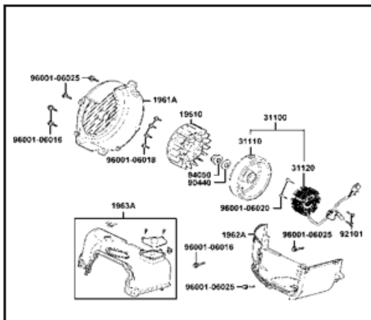
FIGURA 7: CUBIERTA VENTILADOR - MAGNETO
