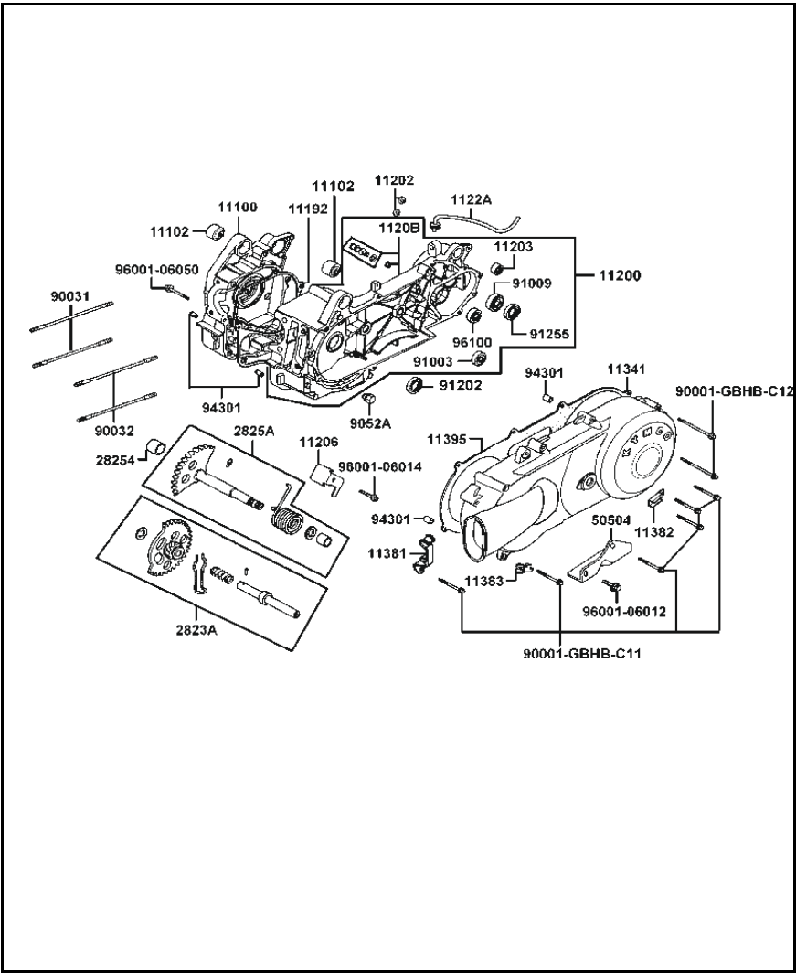
FIGURA N°1: CARCASAS
