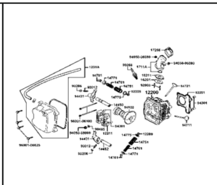
FIGURA 2: CULATA
