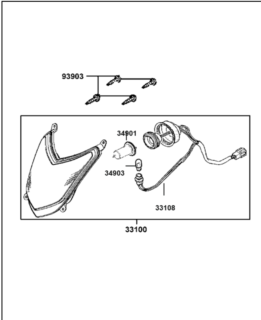
FIGURA N°10: FAROLA
