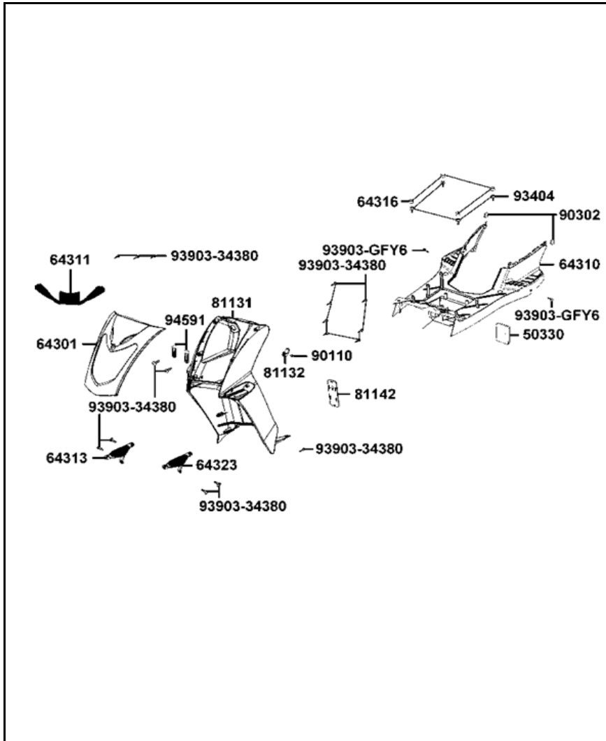
FIGURA N°14: CUBIERTAS
