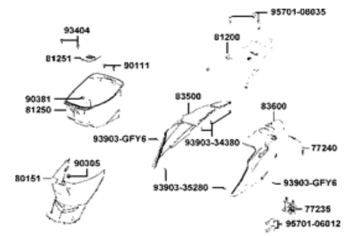
FIGURA 21: CUBIERTAS LATERALES - GUANTERA
