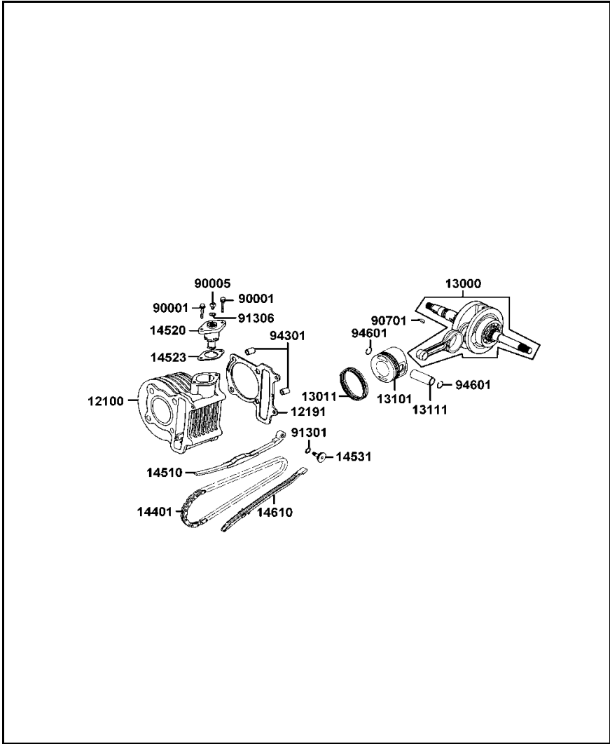
FIGURA N°3: CILINDRO - PISTÓN - CIGÜEÑAL
