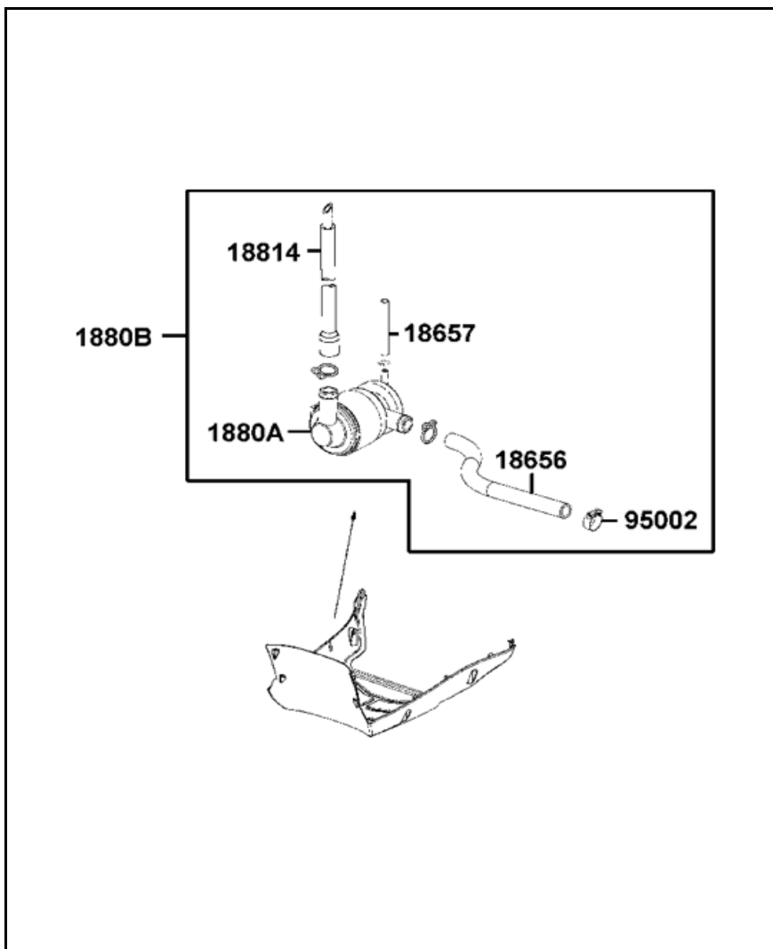
FIGURA N°30: FILTRO DE GASES
