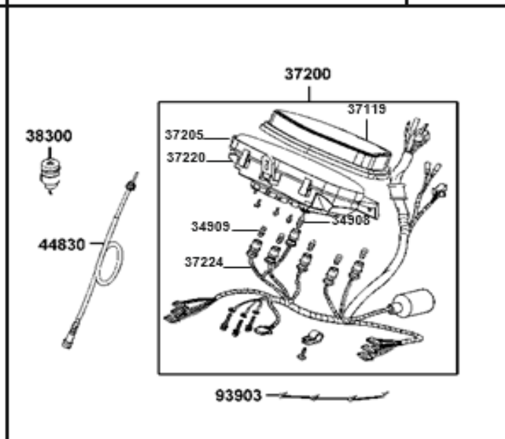
FIGURA 11: VELOCÍMETRO
