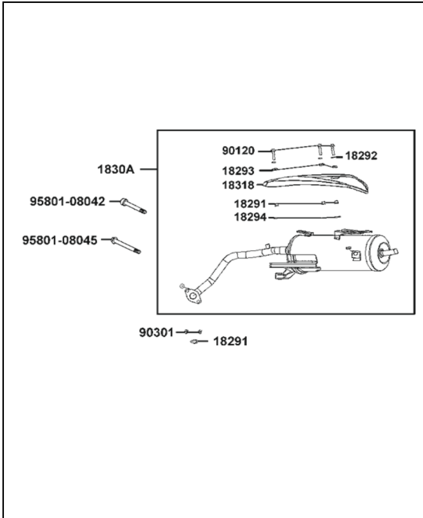
FIGURA N°23: SILENCIADOR
