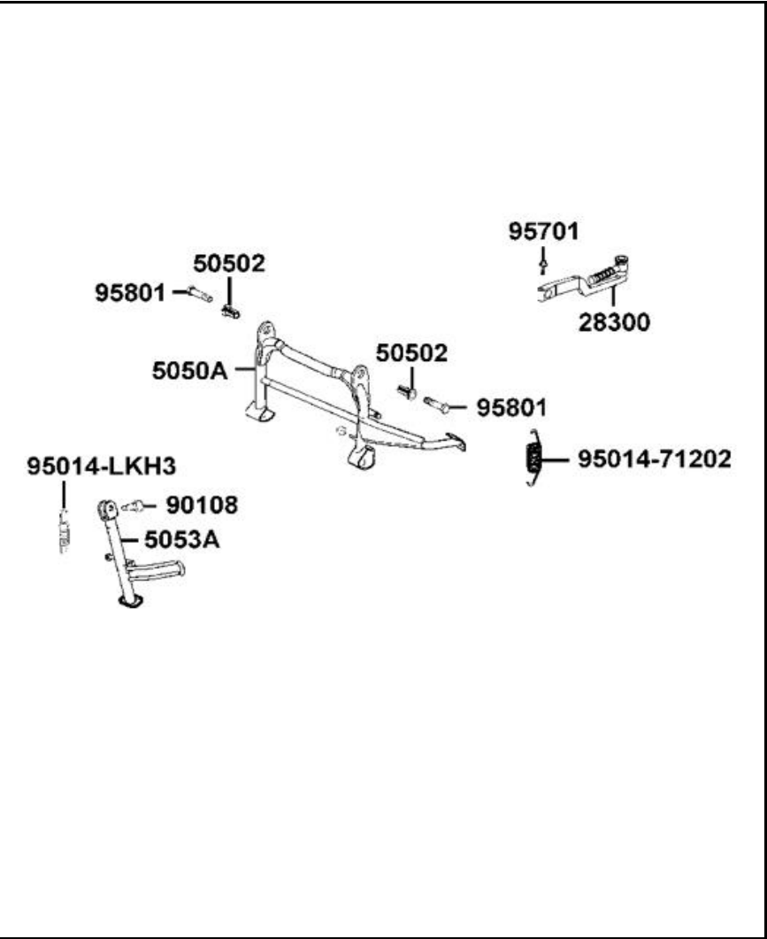
FIGURA N°24: GATO LATERAL - PEDAL CRANK
