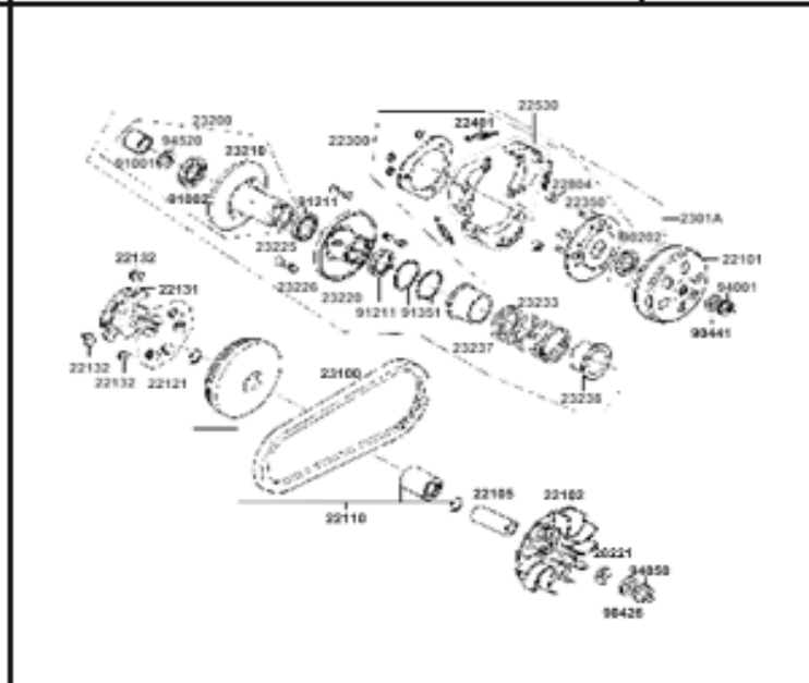
FIGURA 5: CLUTCH CENTRIFUGO
