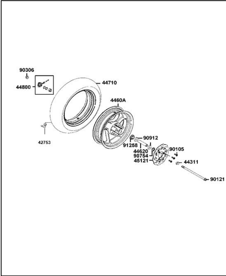
FIGURA N°16: RIN DELANTERO
