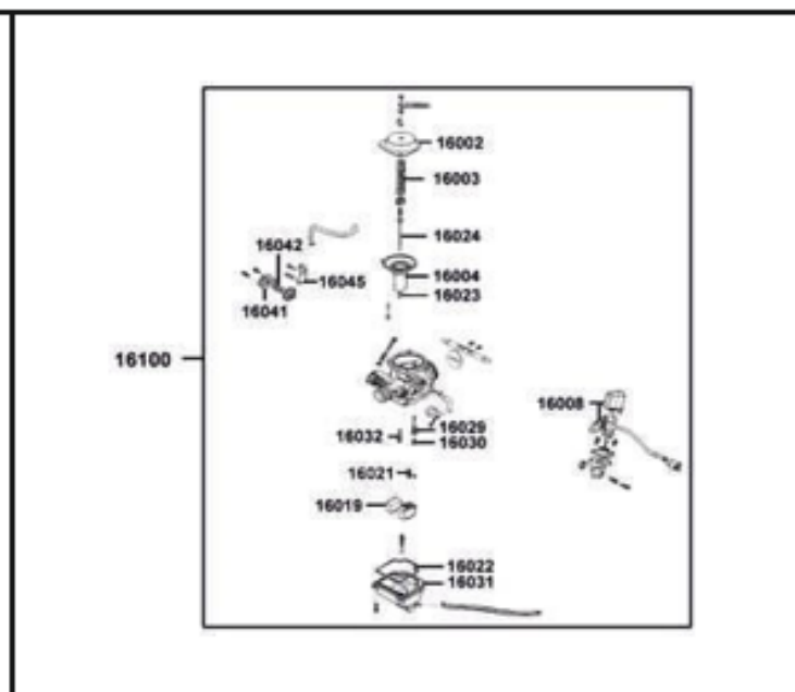
FIGURA 9: CARBURADOR
