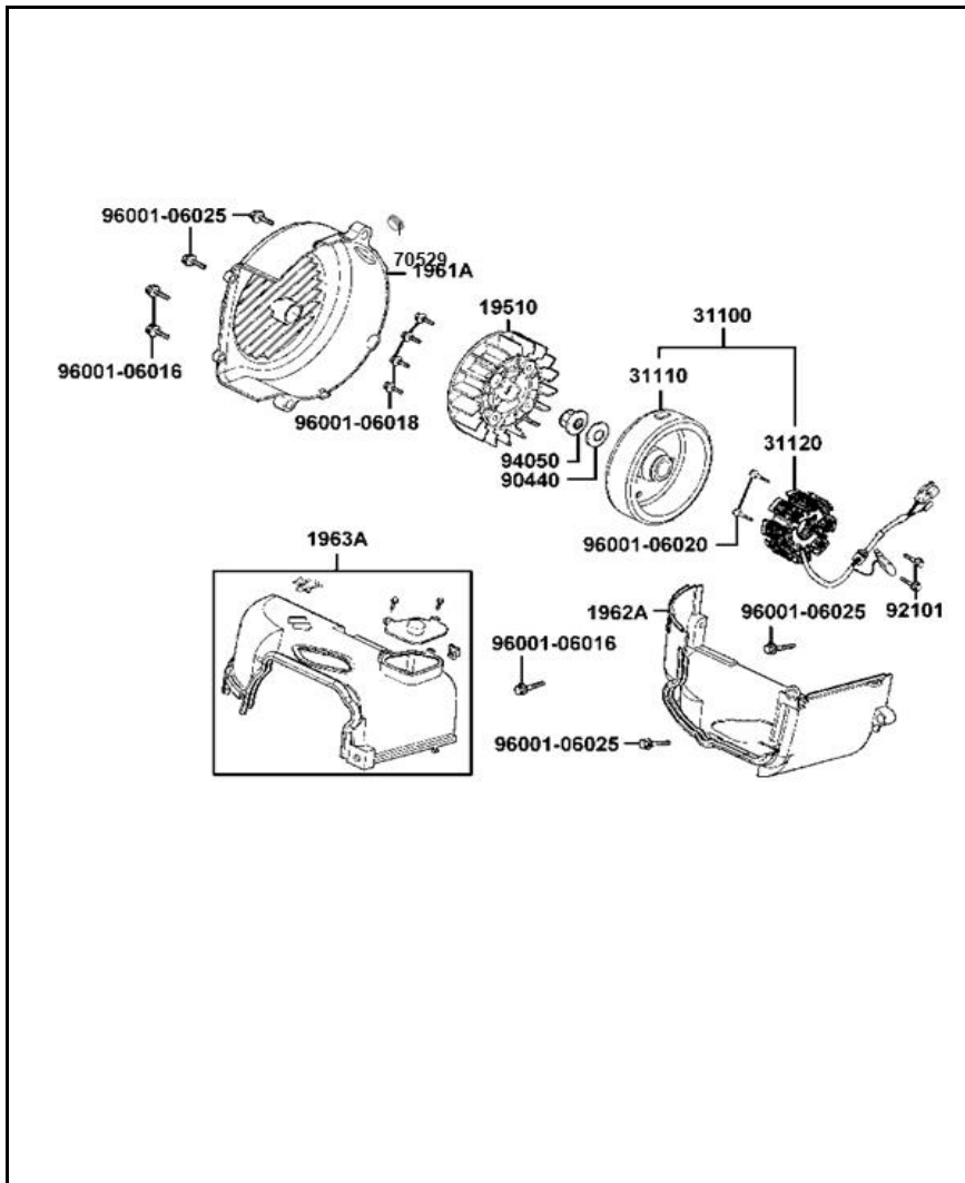
FIGURA N°7: CUBIERTA VENTILADOR - MAGNETO
