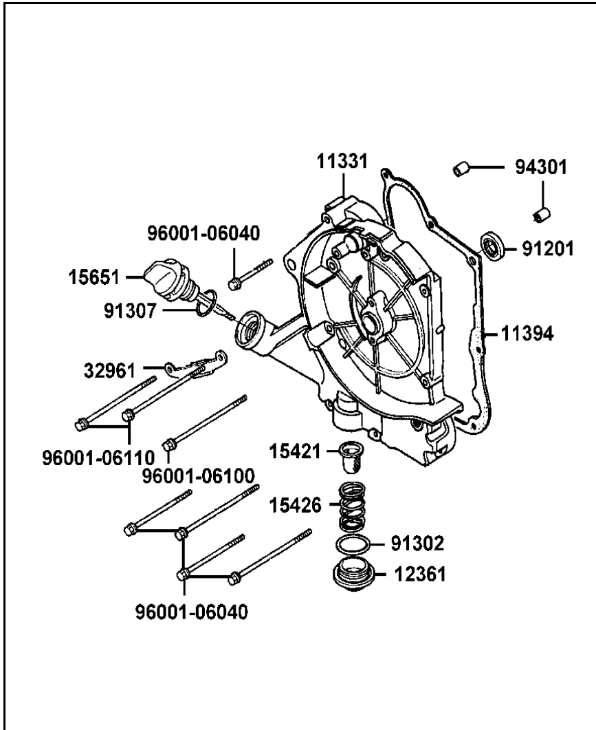
FIGURA N°4: CUBIERTA MOTOR DERECHA
