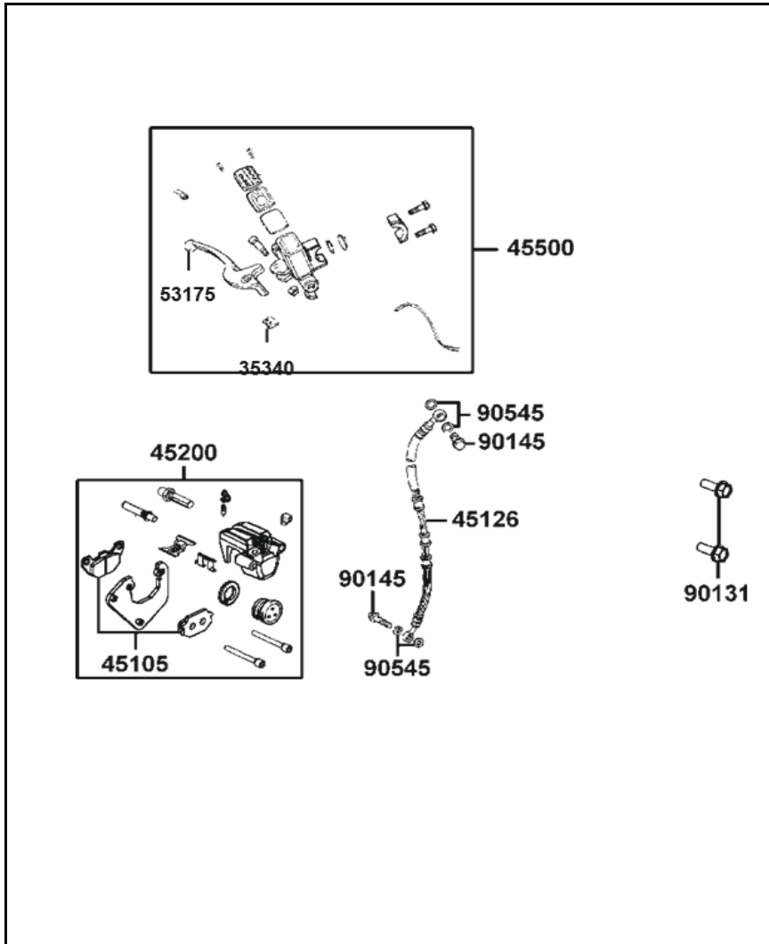
FIGURA N°13: BOMBA DE FRENO
