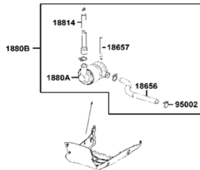
FIGURA 30: FILTRO DE GASES
