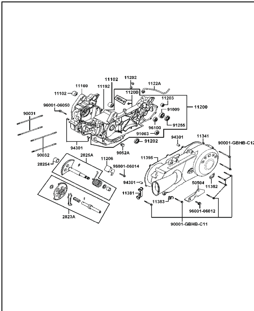
FIGURA N°1: CARCASAS
