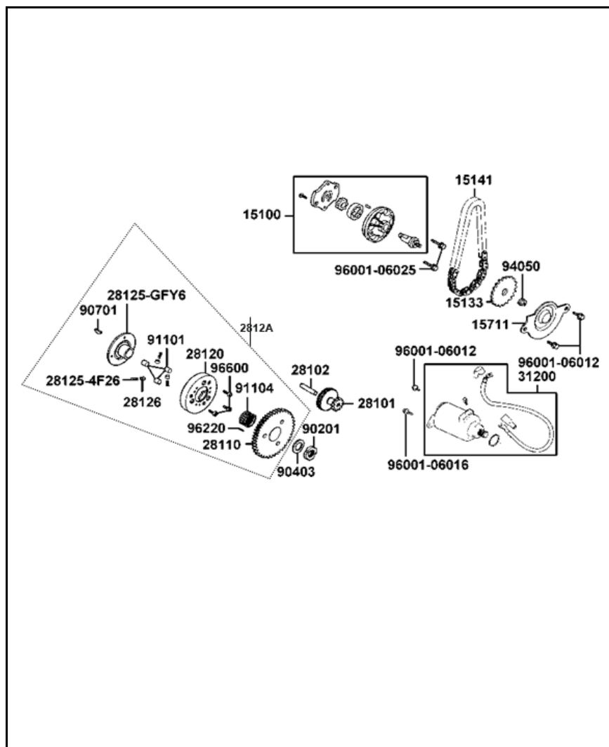
FIGURA N°6: MOTOR DE ARRANQUE - BOMBA DE ACEITE
