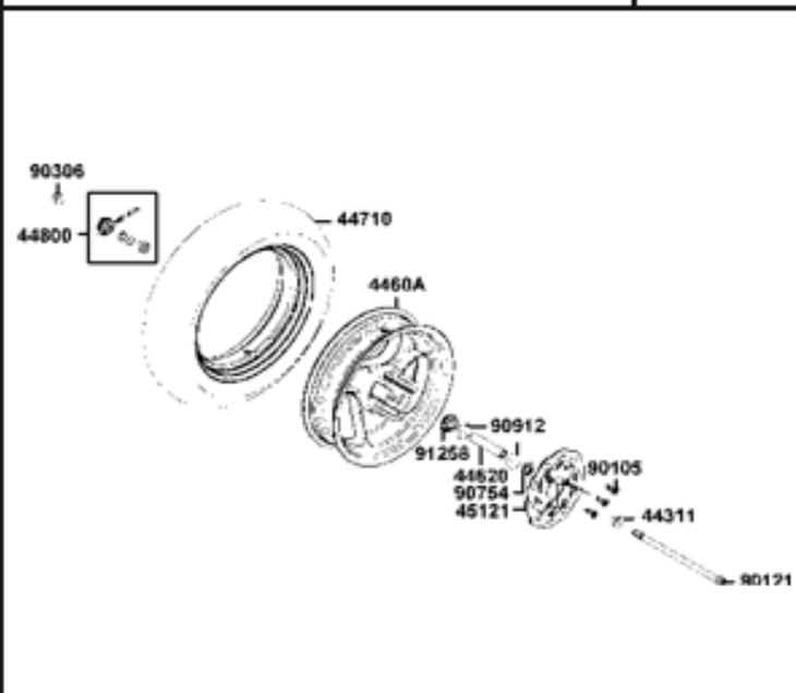
FIGURA 16: RIN DELANTERO
