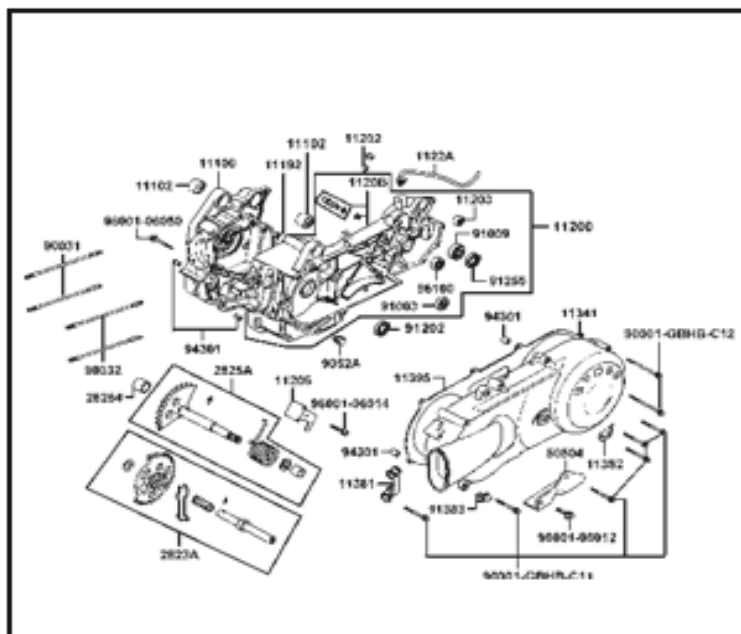
FIGURA 1: CARCASAS
