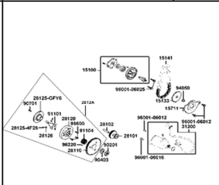
FIGURA 6: MOTOR DE ARRANQUE - BOMBA DE ACEITE
