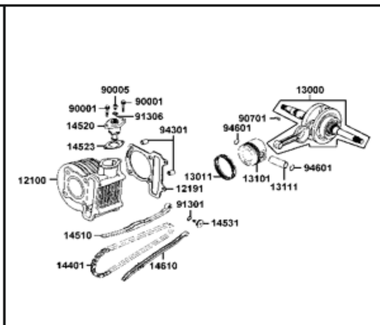
FIGURA 3: CILINDRO - PISTÓN - CIGUEÑAL
