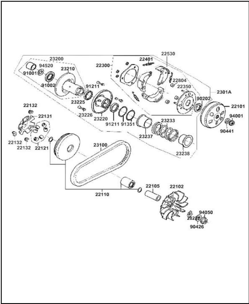
FIGURA N°5: CLUTCH CENTRIFUGO
