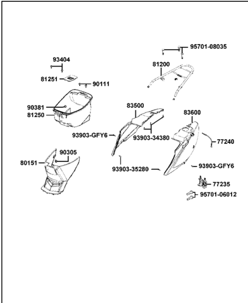
FIGURA N°21: CUBIERTAS LATERALES - GUANTERA
