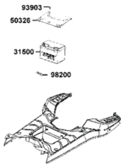
FIGURA 20: BATERIA
