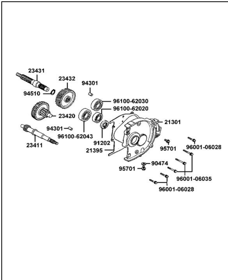
FIGURA N°8: TRANSMISIÓN
