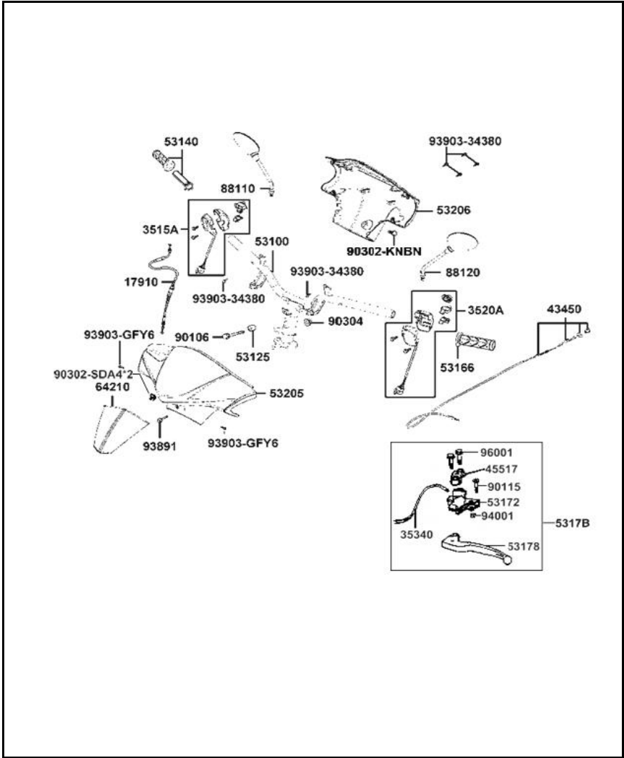
FIGURA N°12: MANUBRIO - CUBIERTAS MANUBRIO
