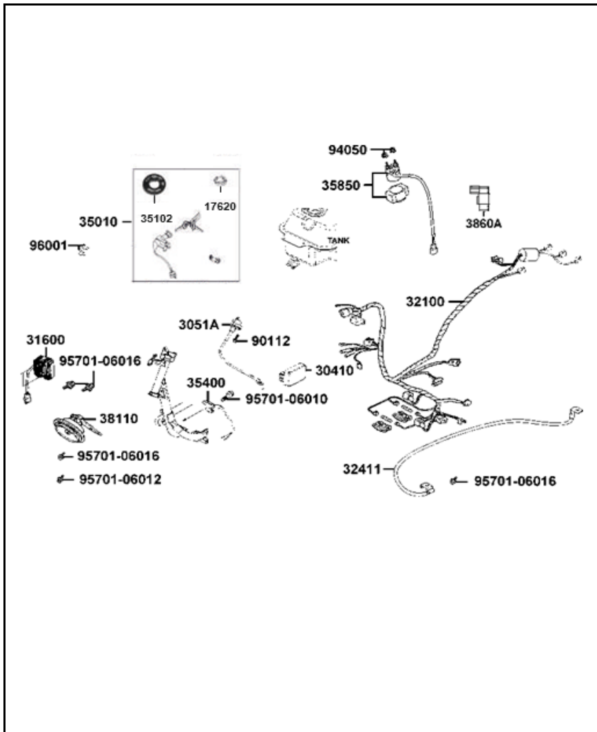
FIGURA N°28: SISTEMA ELÉCTRICO
