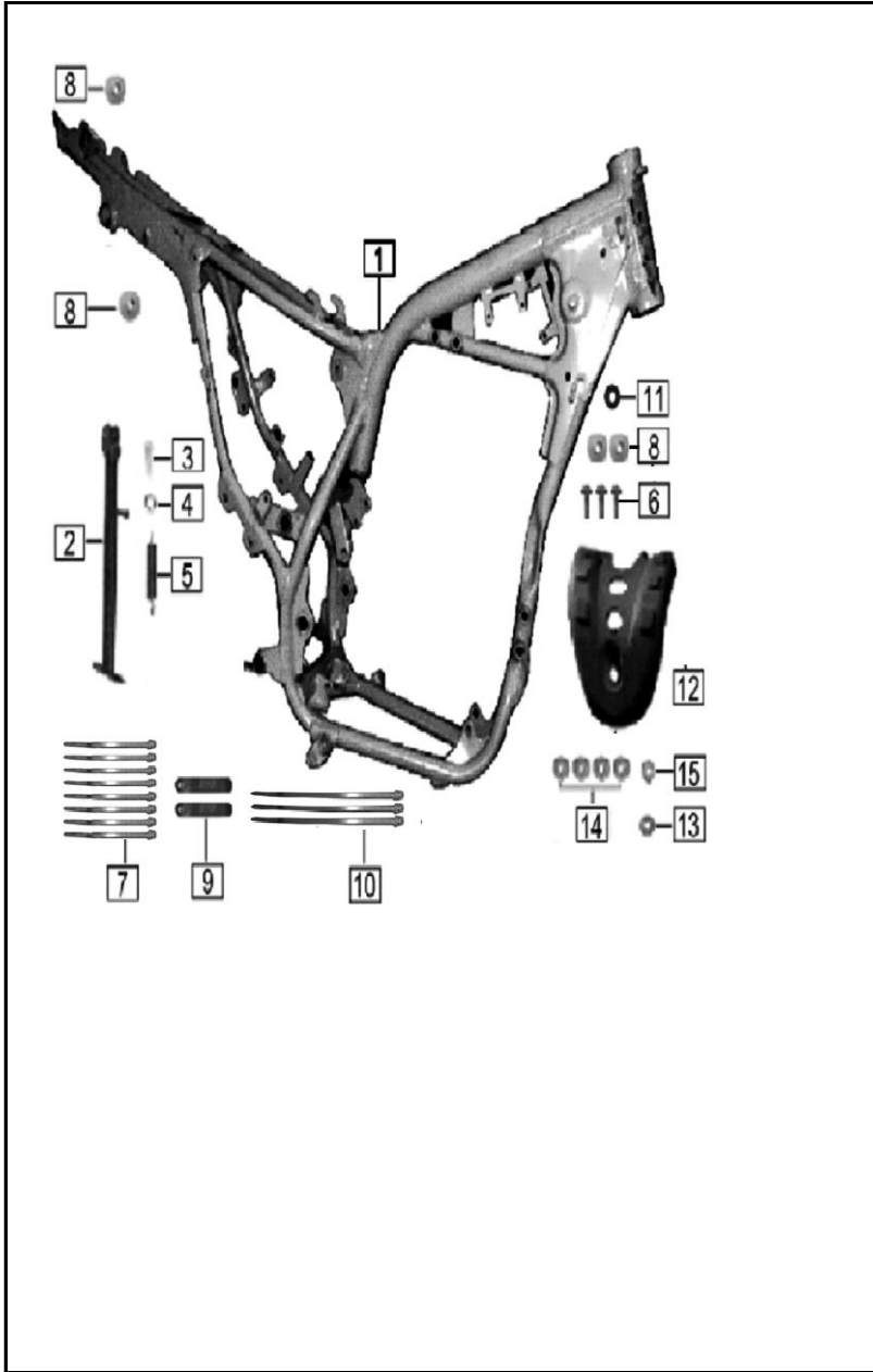
FIGURA N° 44: COMPLEMENTOS CHASIS - GATO LATERAL
