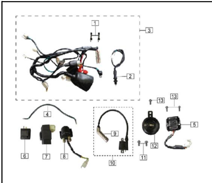
FIG. Nº 19: SISTEMA ELECTRICO
