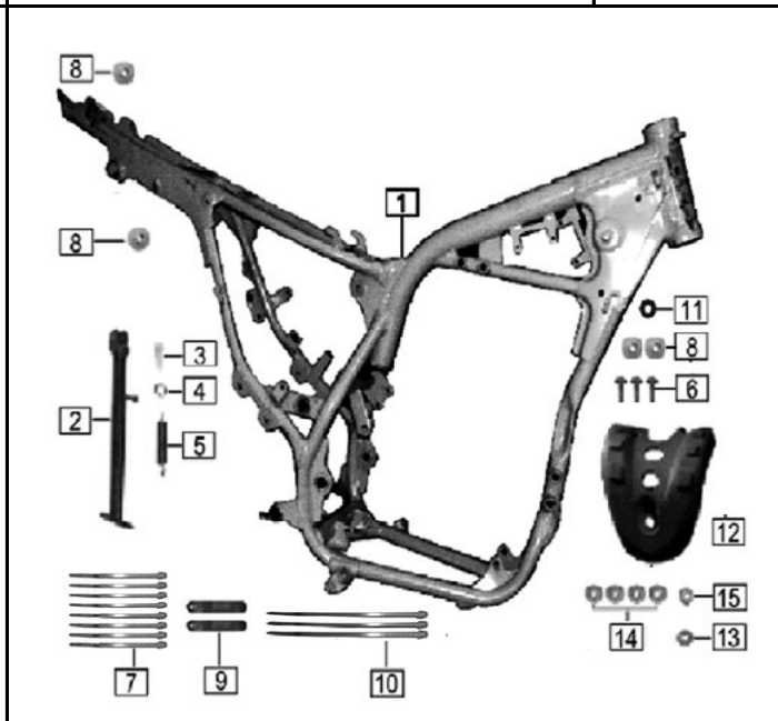
FIG. Nº 41 COMPLEMENTOS CHASIS - GATO LATERAL
