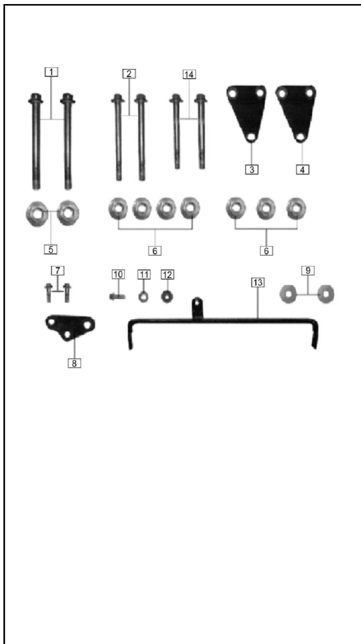
FIGURA N° 45: SOPORTE MOTOR
