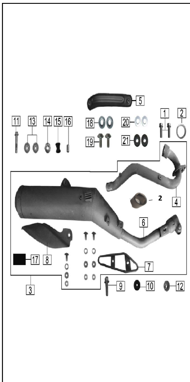
FIGURA N° 28: SILENCIADOR
