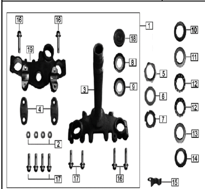
FIG. Nº 28 ESPIGA CENTRAL - CABEZA ESPIGA
