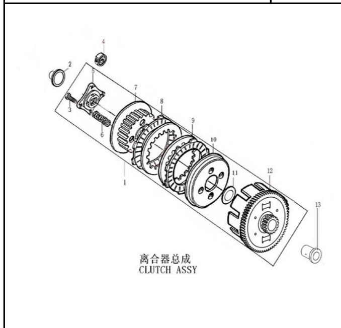
FIG. Nº 4: CLUTCH
