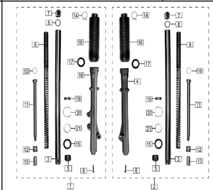
FIG. Nº 29 SUSPENSION DELANTERA
