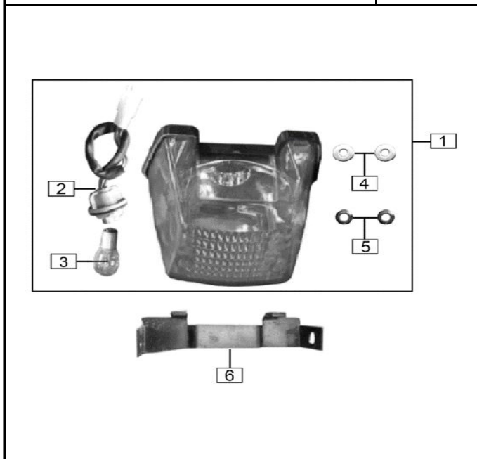
FIG. Nº 22: STOP - DIRECCIONALES TRASERAS
