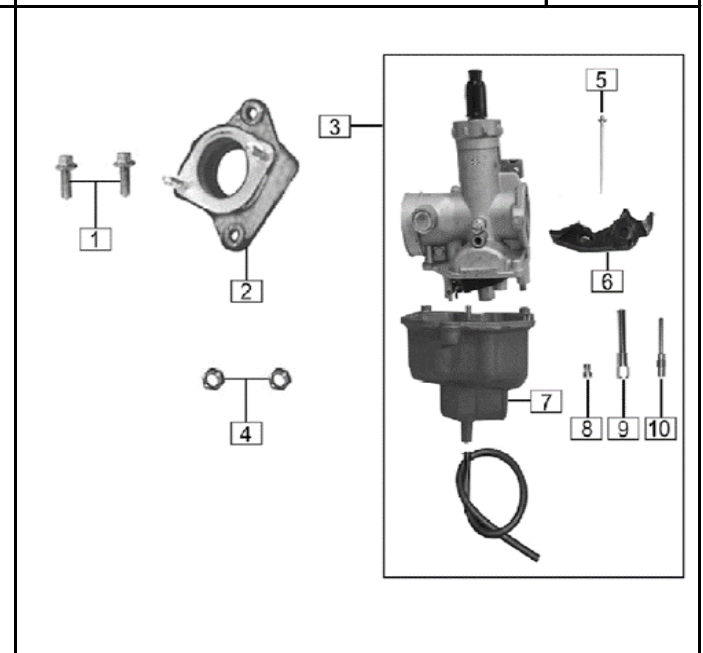
FIG. Nº 24: CARBURADOR
