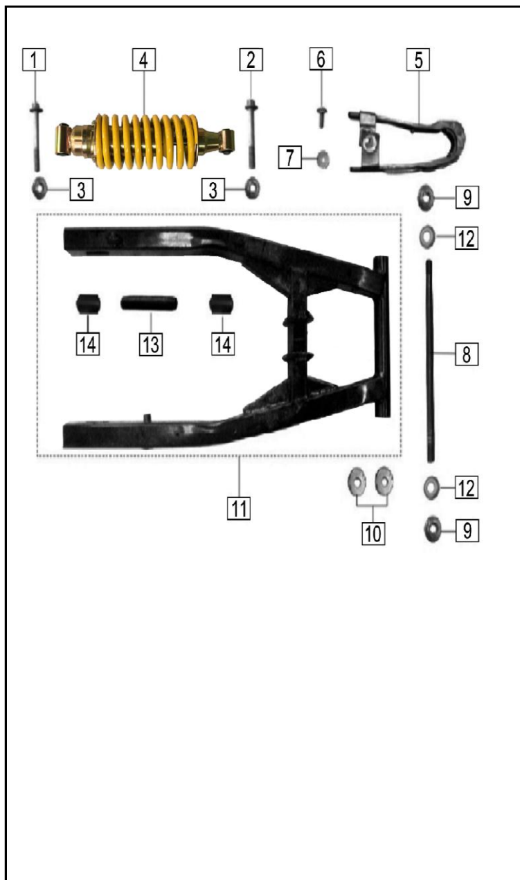
FIGURA N° 38: BRAZO OSCILANTE - MONOSHOCK
