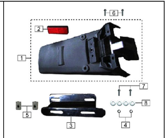
FIG. Nº 21: GUARDABARRO TRASERO
