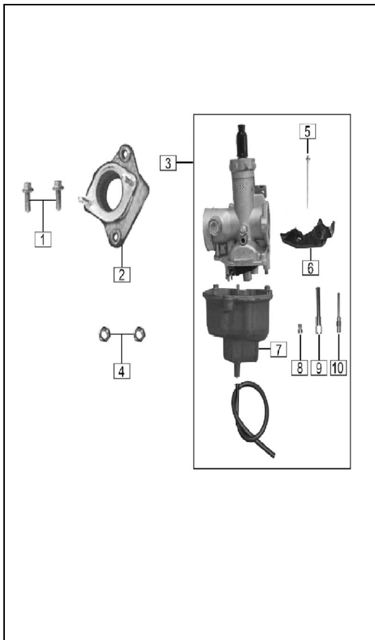
FIGURA N° 27: CARBURADOR
