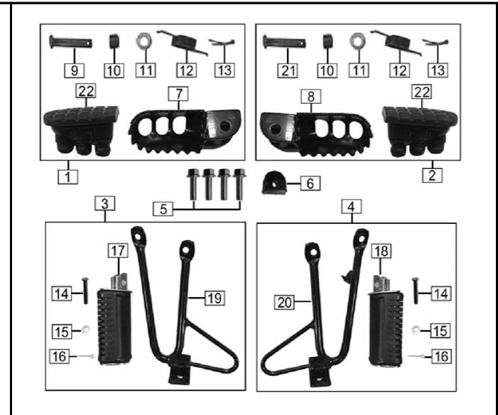
FIG. Nº 27: REPOSAPIE CONDUCTOR - REPOSAPIE PASAJERO
