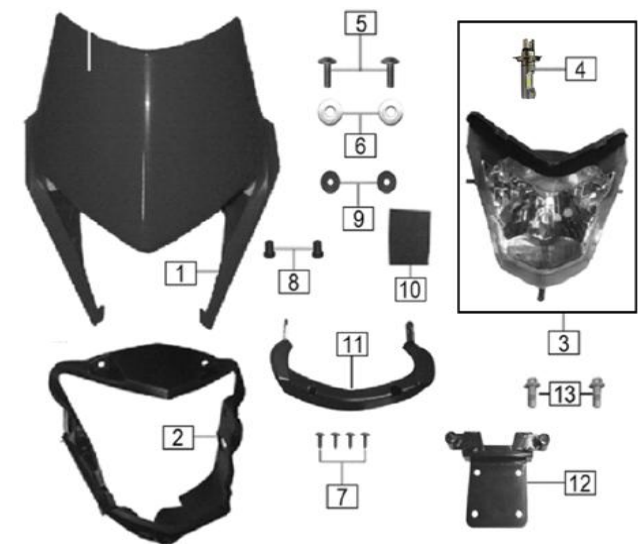
FIG. Nº 12: FAROLA - CARENAJE FAROLA
