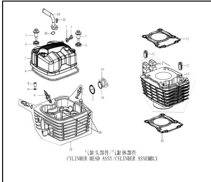
FIG. Nº 1: CULATA - CILINDRO MOTOR
