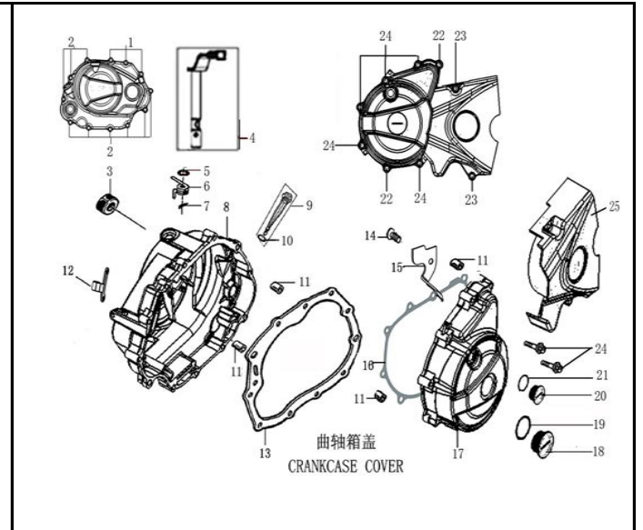
FIG. Nº 3: CUBIERTA CLUTCH - CUBIERTA VOLANTE
