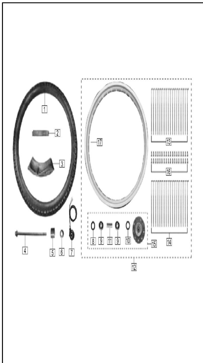
FIGURA N° 36: RUEDA DELANTERA
