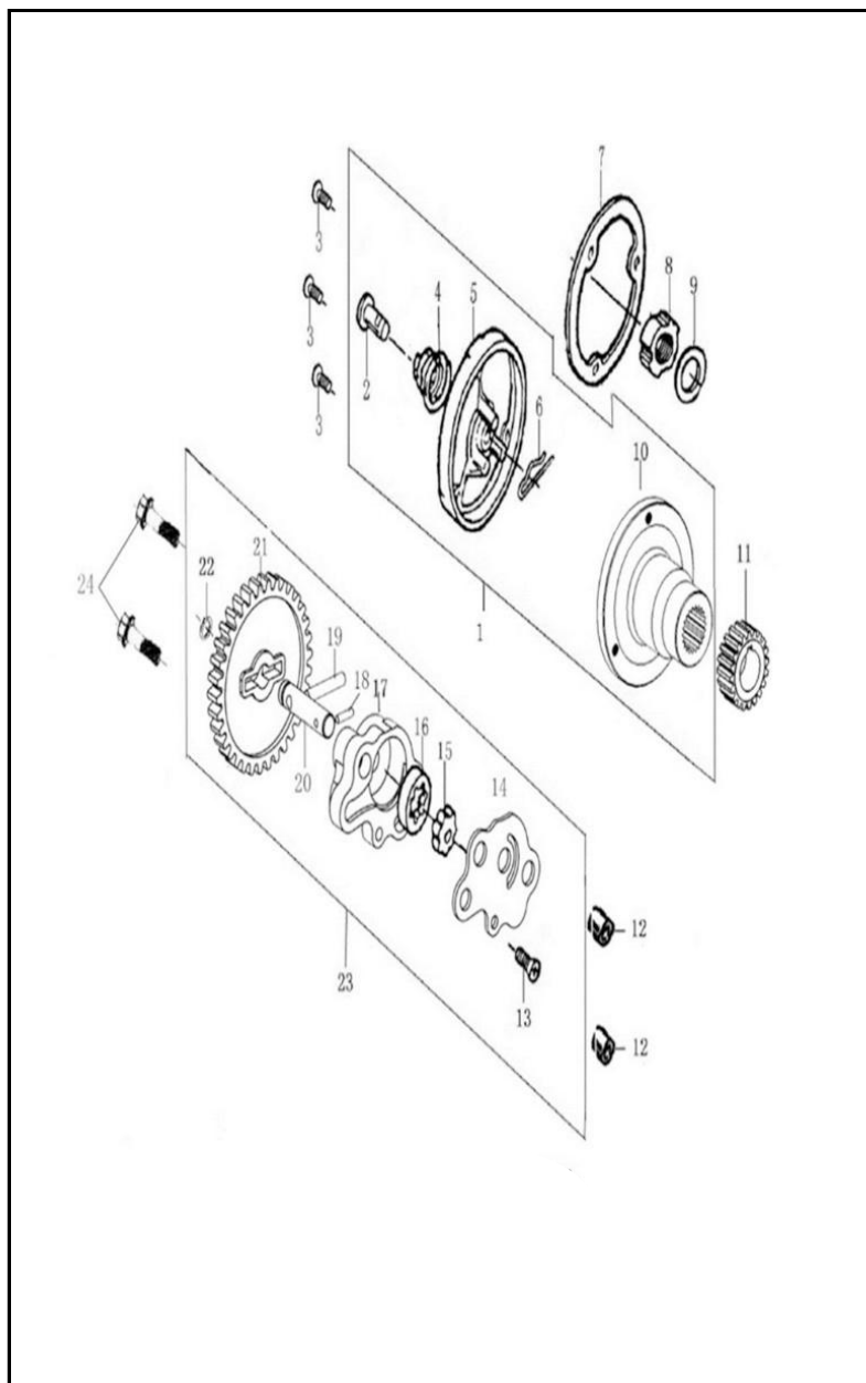
FIGURA N° 5: BOMBA ACEITE - FILTRO CENTRIFUGO ACEITE
