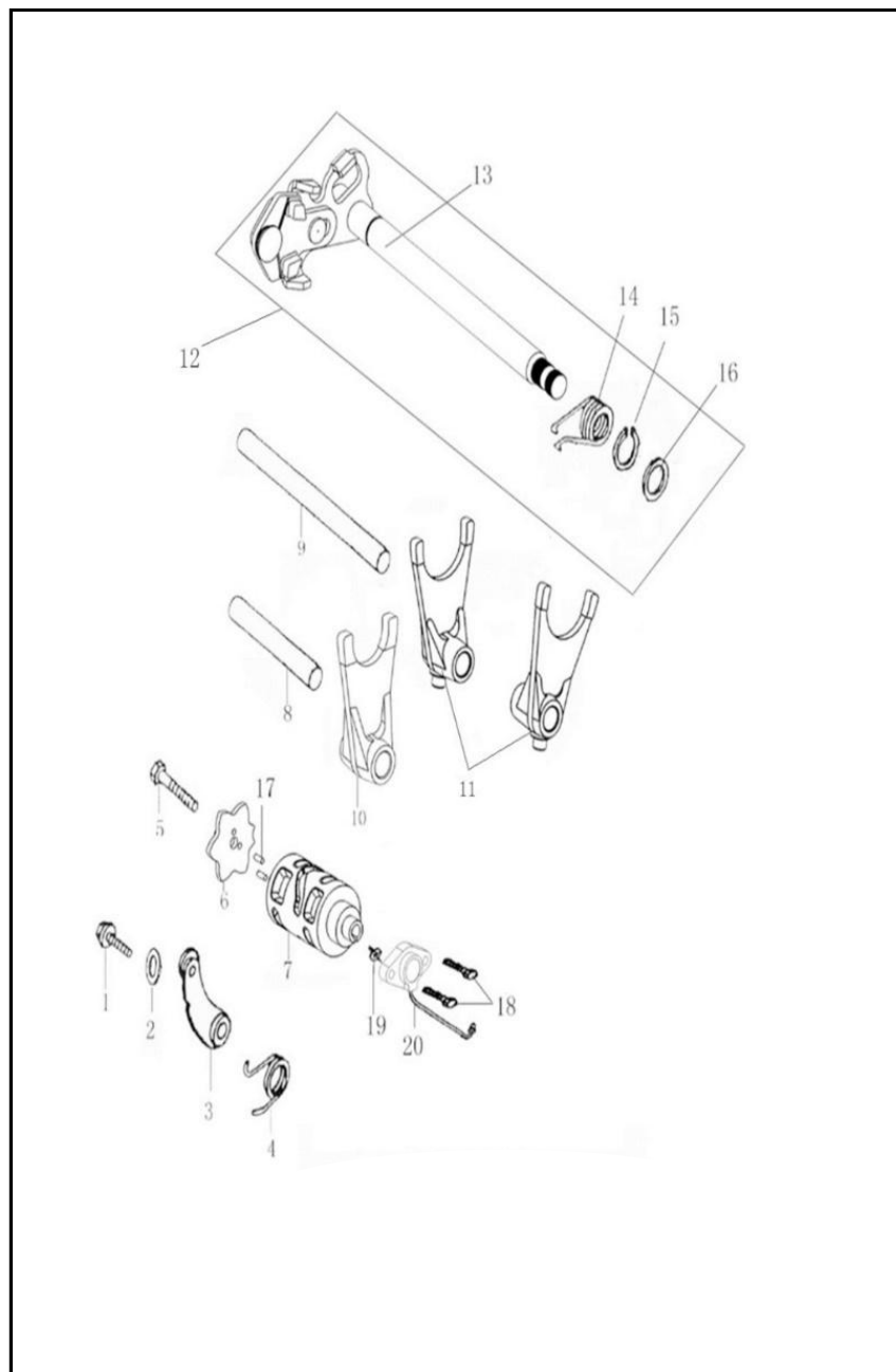
FIGURA N° 9: EJE CAMBIOS - EJE SECTOR CAMBIOS
