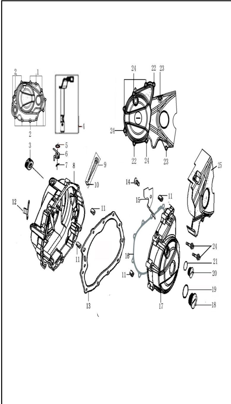
FIGURA N° 3: CUBIERTA CLUTCH - CUBIERTA VOLANTE
