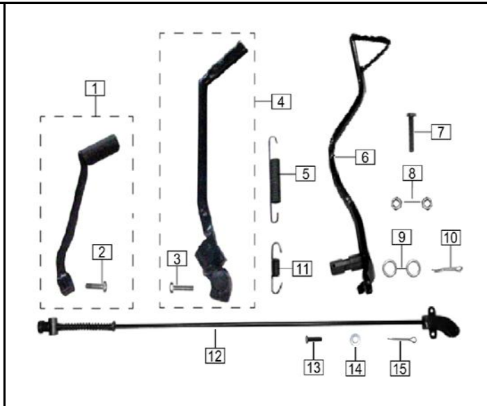
FIG. Nº 26: PEDAL CAMBIOS - PEDAL FRENO - PEDAL CRANK
