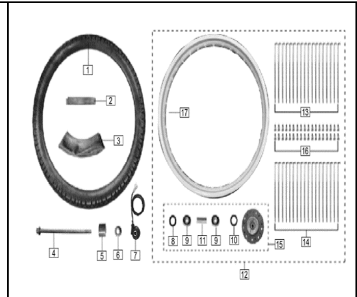
FIG. Nº 33 RUEDA DELANTERA
