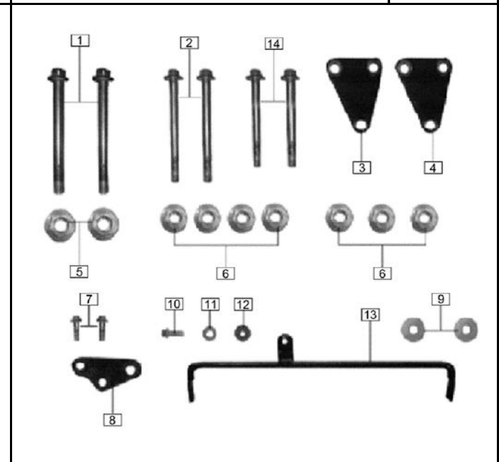
FIG. Nº 42 SOPORTE MOTOR
