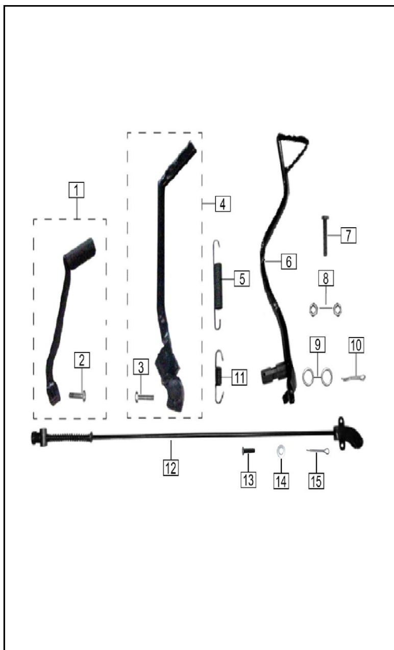
FIGURA N° 29: PEDAL CAMBIOS - PEDAL FRENO - PEDAL CRANK
