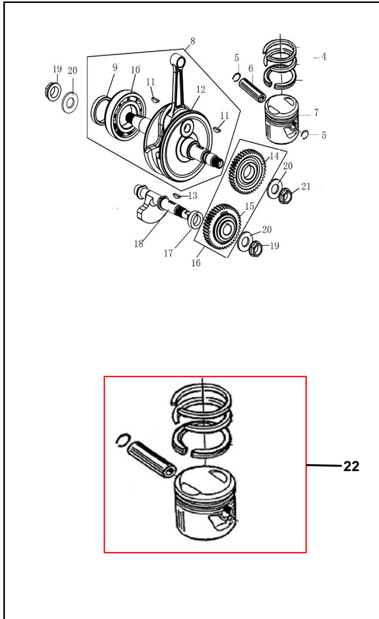
FIGURA N° 7: CIGÜEÑAL - BALANCEADOR - PISTON
