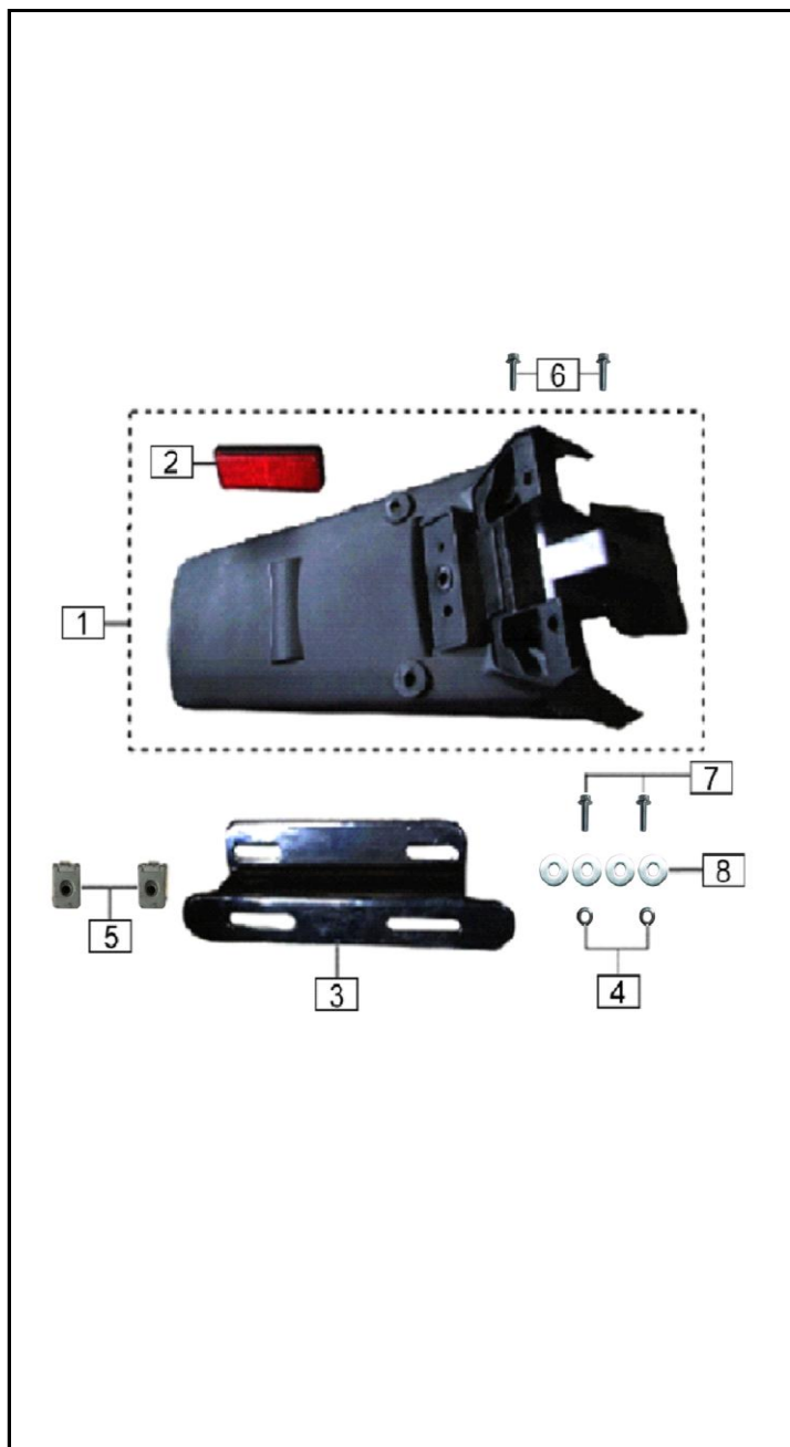
FIGURA N° 24: GUARDABARRO TRASERO
