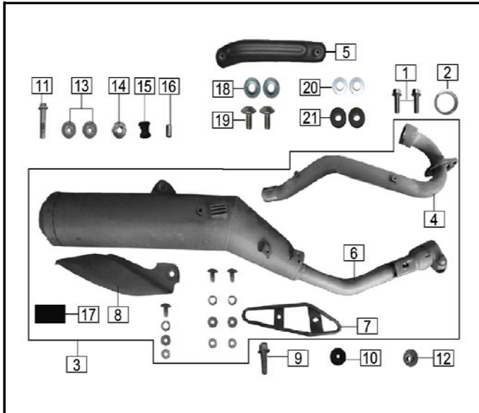
FIG. Nº 25: SILENCIADOR
