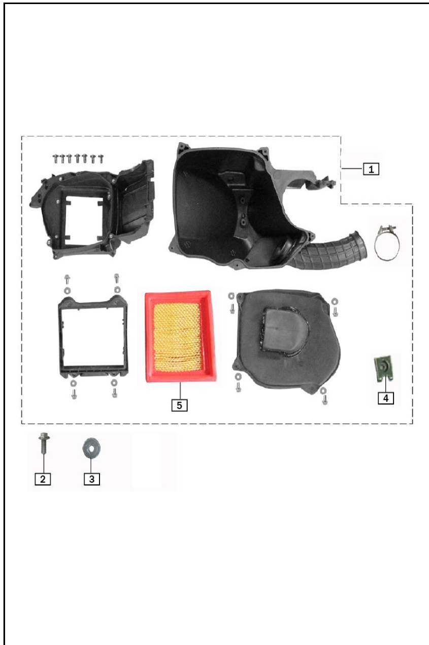
FIGURA N° 26: CAJA FILTRO AIRE
