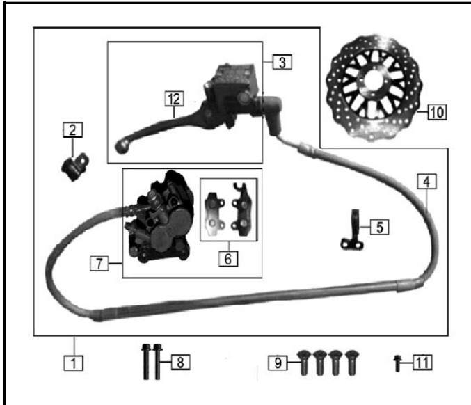
FIG. Nº 31 BOMBA FRENO DELANTERO
