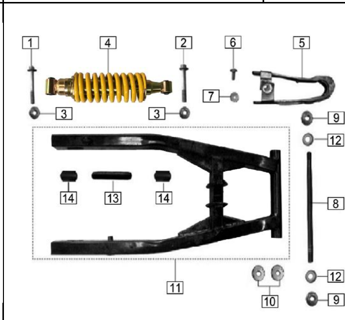
FIG. Nº 35 BRAZO OSCILANTE - MONOSHOCK
