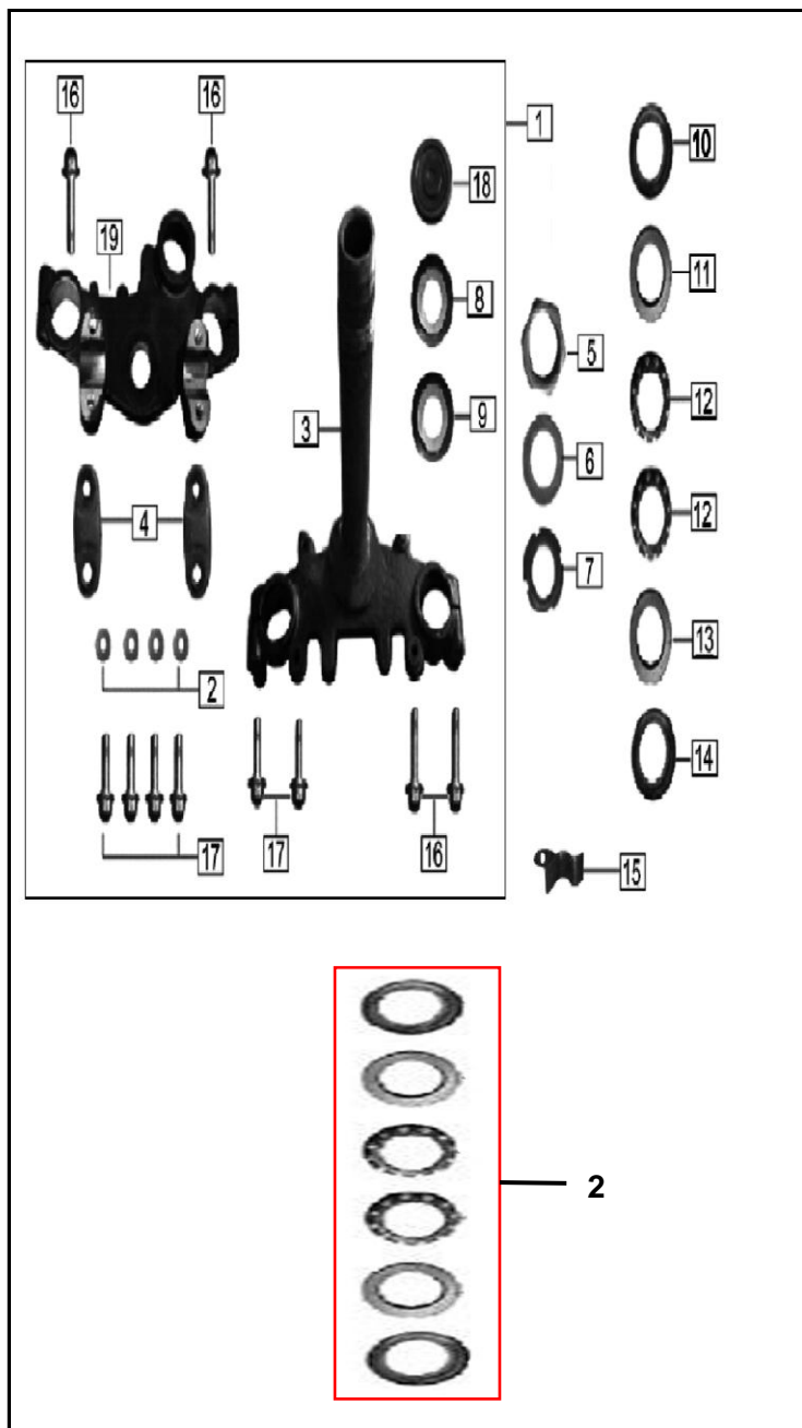
FIGURA N° 31: ESPIGA CENTRAL - CABEZA ESPIGA
