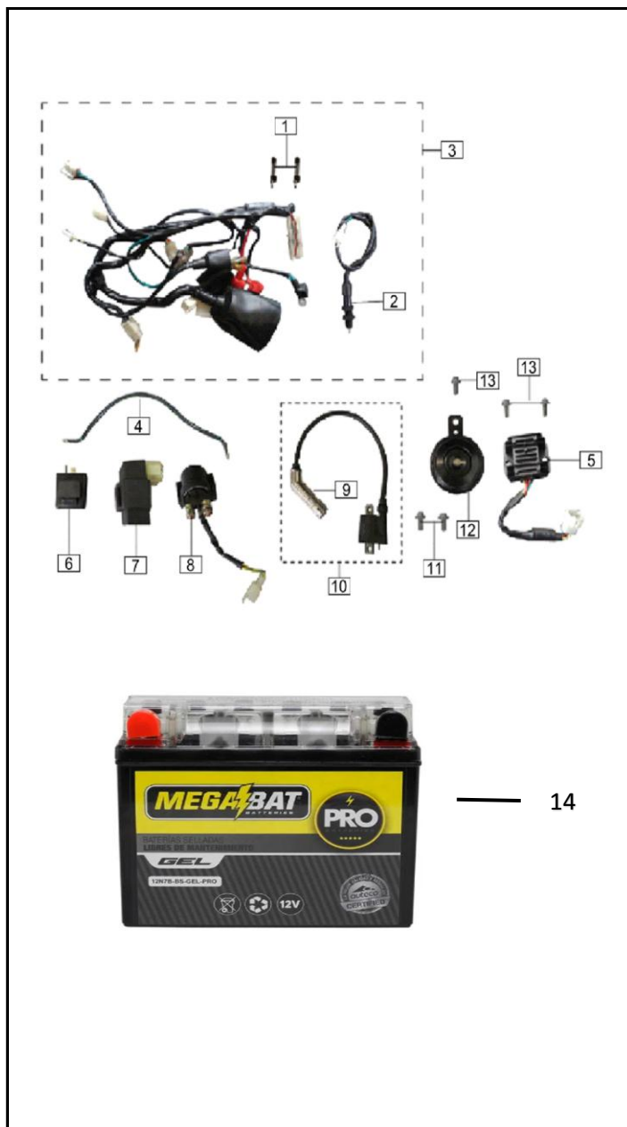
FIGURA N° 22: SISTEMA ELECTRICO
