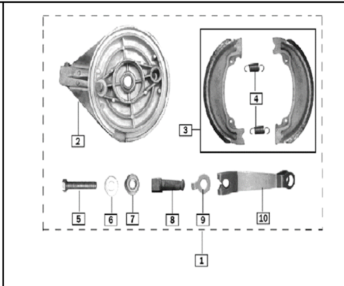
FIG. Nº 32 PORTA BANDAS TRASERO
