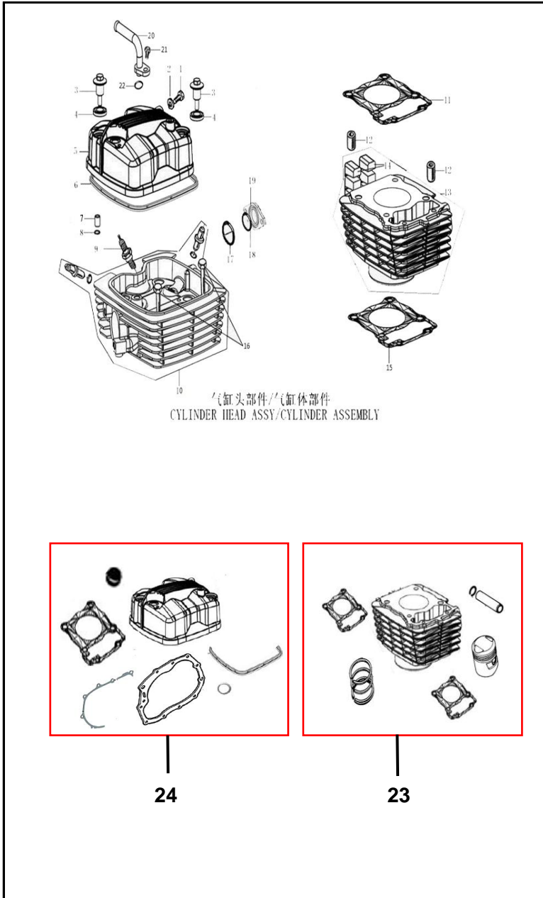
FIGURA N° 1: CULATA - CILINDRO MOTOR
