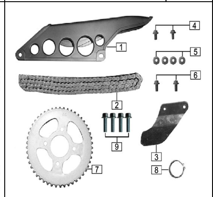
FIG. Nº 36 SPROCKET - CADENA
