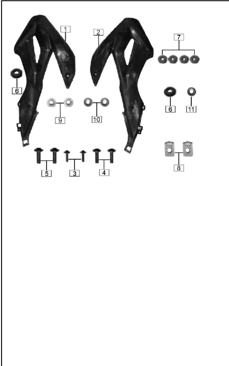
FIGURA N° 40: ENFOCADORES
