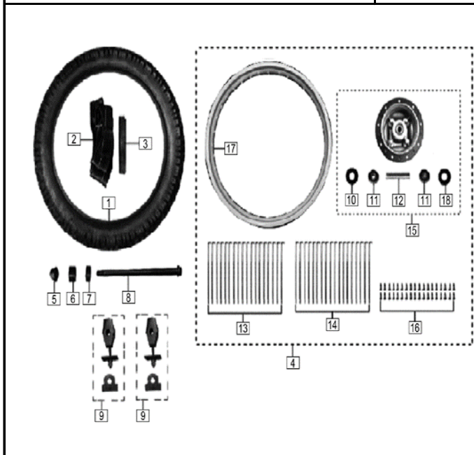
FIG. Nº 34 RUEDA TRASERA
