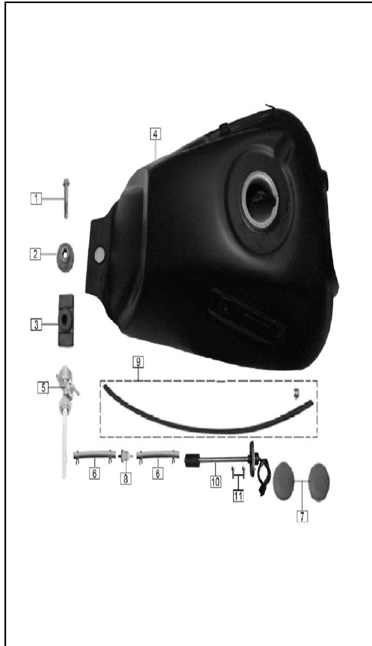
FIGURA N° 20: TANQUE GASOLINA
