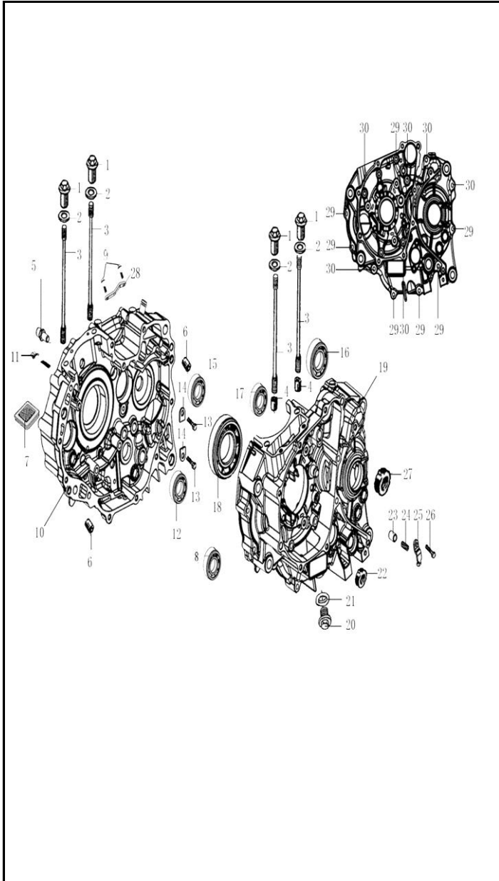
FIGURA N° 6: CARCASAS (1/2)
