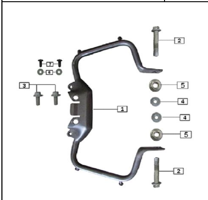
FIG. Nº 40 AGARRADERA PASAJERO
