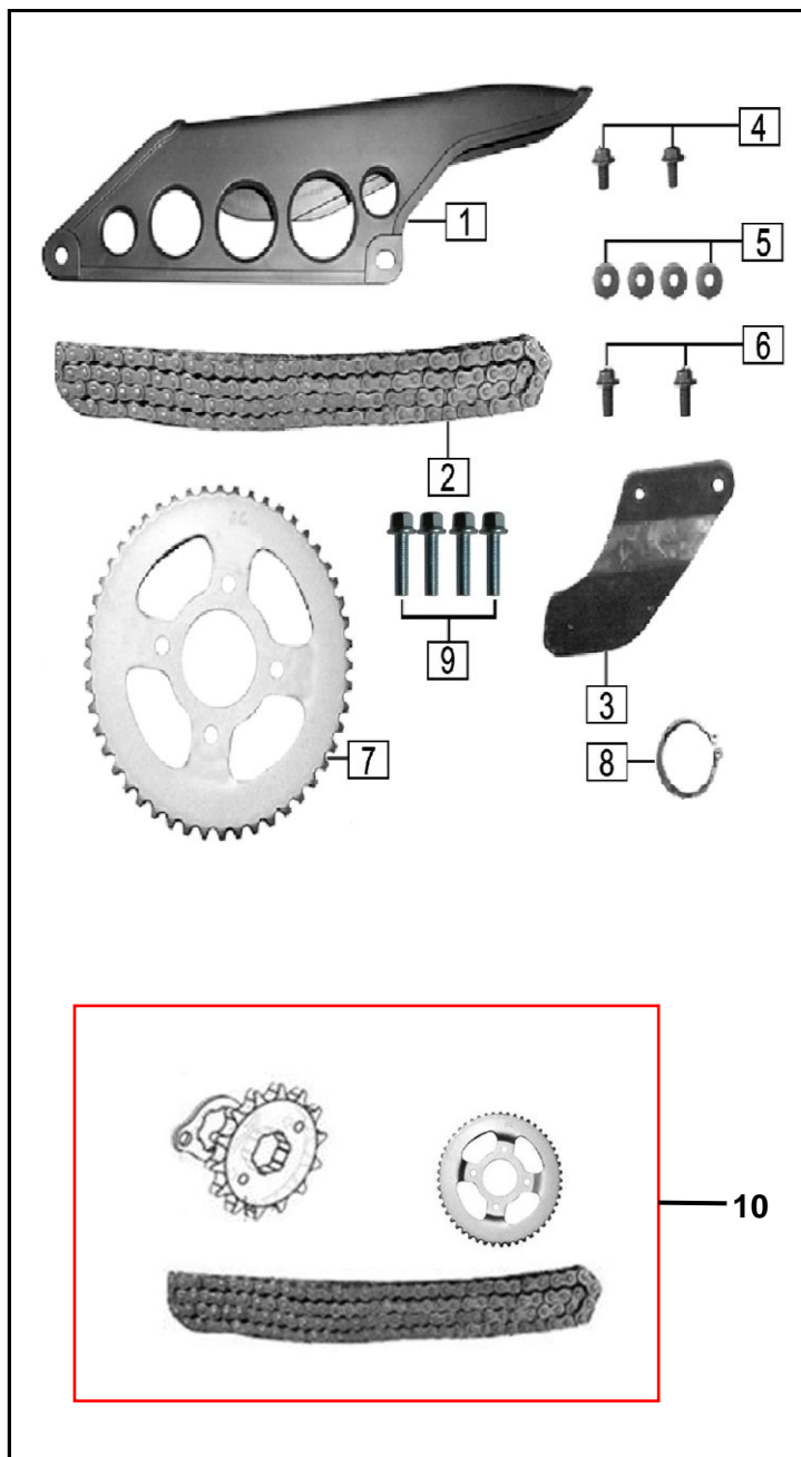
FIGURA N° 39: SPROCKET - CADENA
