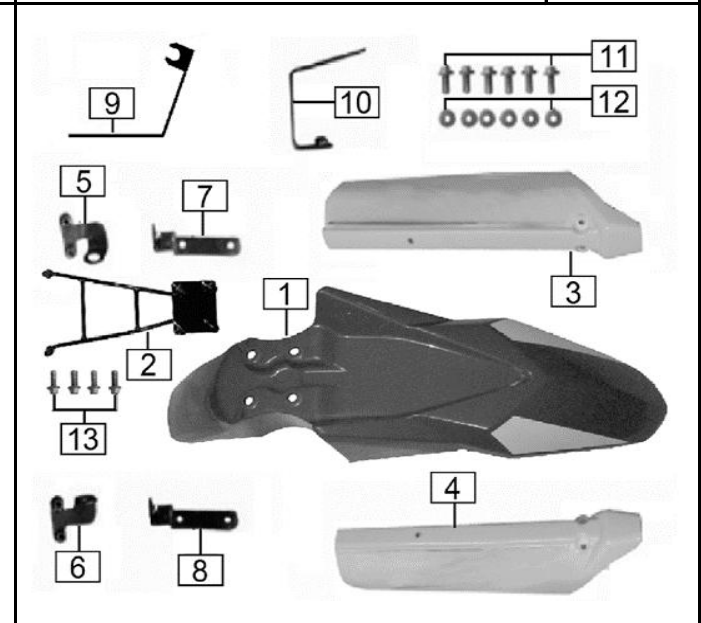
FIG. Nº 30 GUARDABARRO DELANTERO
