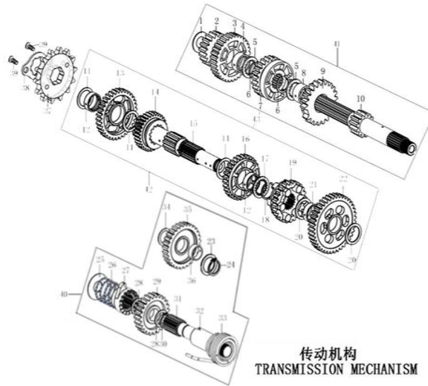
FIG. Nº 8: TRANSMISSION
