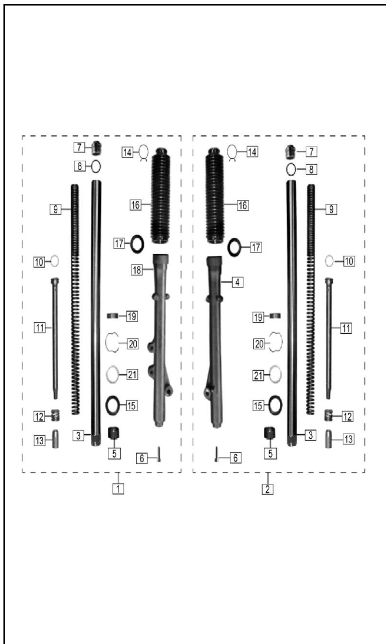
FIGURA N° 32: SUSPENSION DELANTERA
