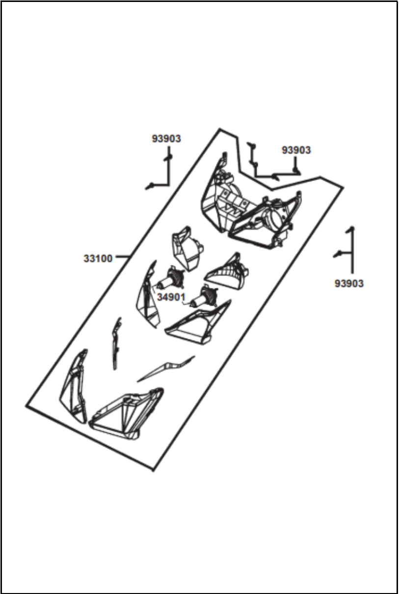
FIGURA N° 10: FAROLA
