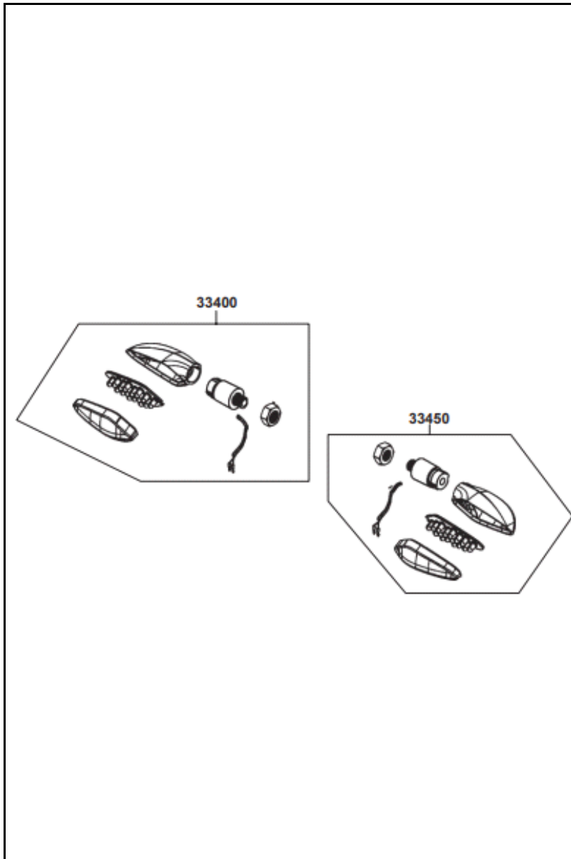
FIGURA N° 26: DIRECCIONALES DELANTERAS
