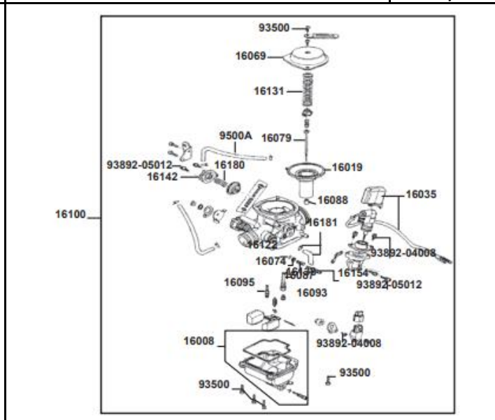
FIG. Nº 5 CARBURADOR
