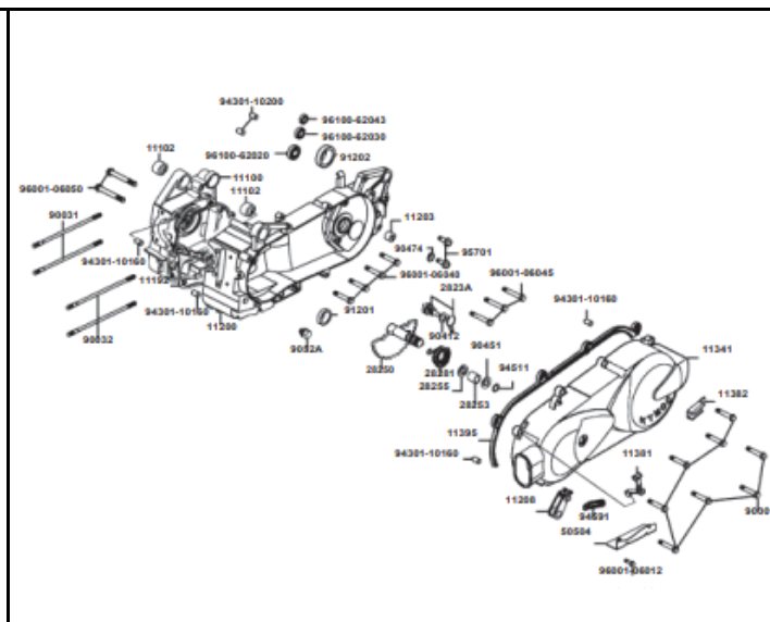
FIG. Nº 2 CARCASAS
