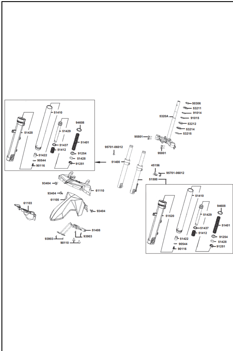
FIGURA N° 15: SUSPENSIÓN DELANTERA
