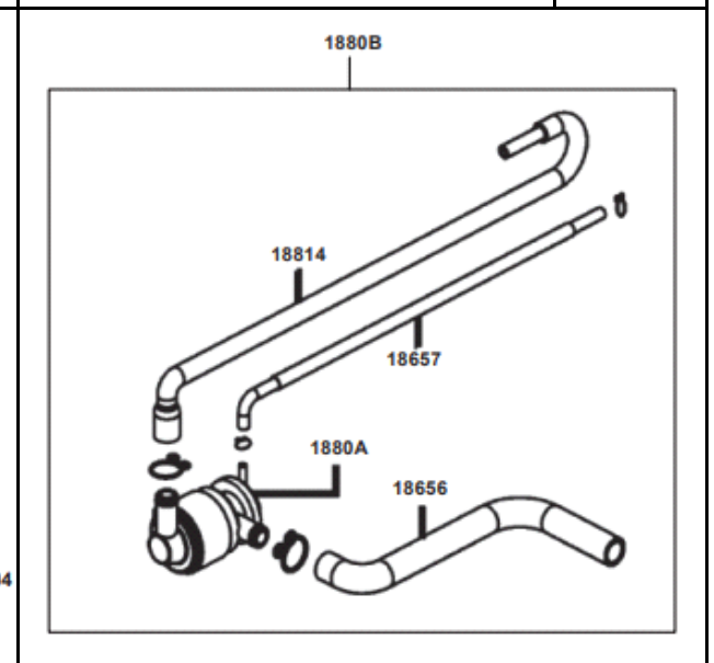
FIG. Nº 30 SISTEMA DE INYECCIÓN DE AIRE
