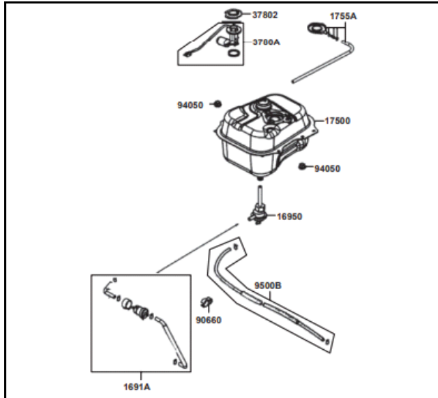
FIG. Nº 19 TANQUE DE COMBUSTIBLE
