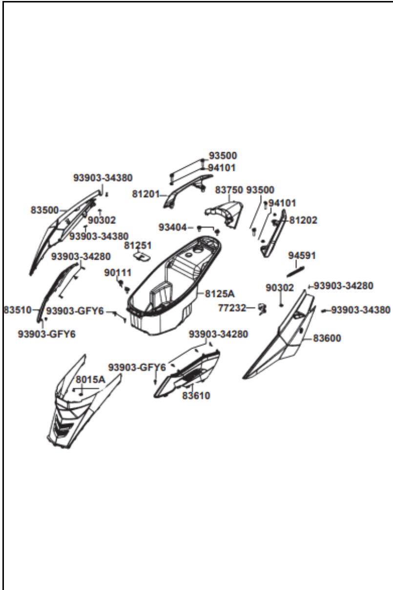
FIGURA N° 22: CUBIERTAS LATERALES - GUANTERA
