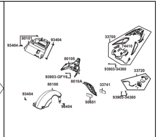
FIG. Nº 27 STOP - GUARDABARRO TRASERO
