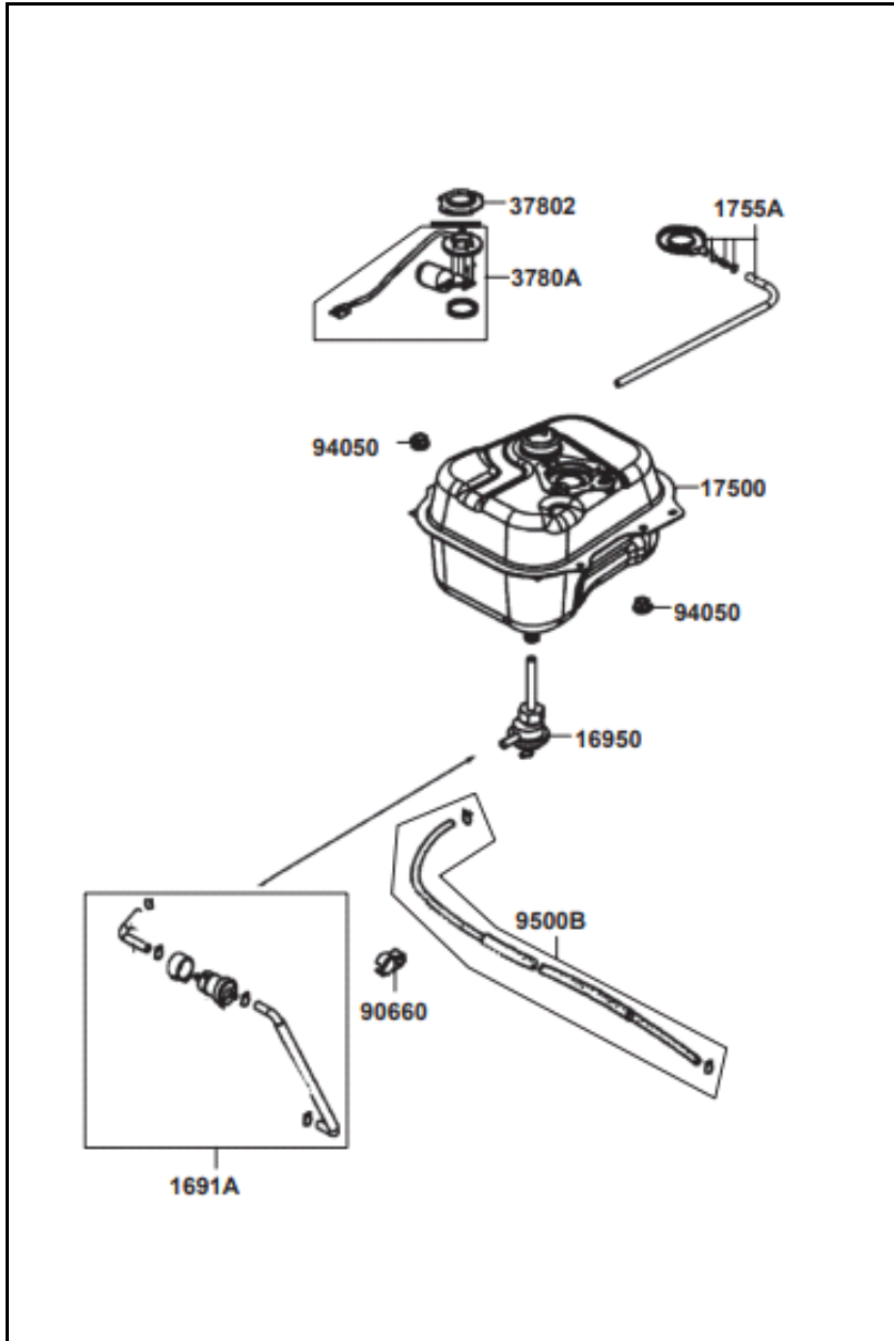
FIGURA N° 19: TANQUE DE COMBUSTIBLE
