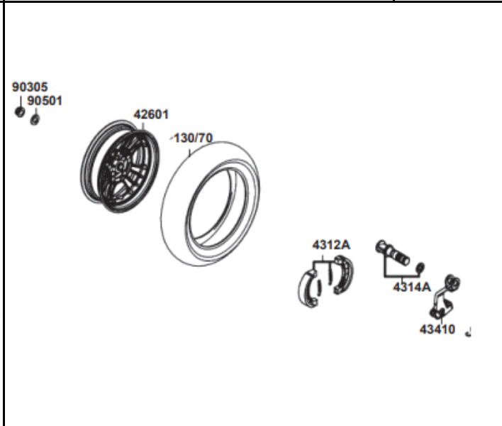
FIG. Nº 17 RIN TRASERO
