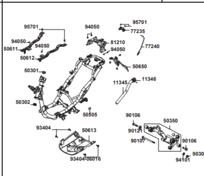
FIG. Nº 29 CHASIS
