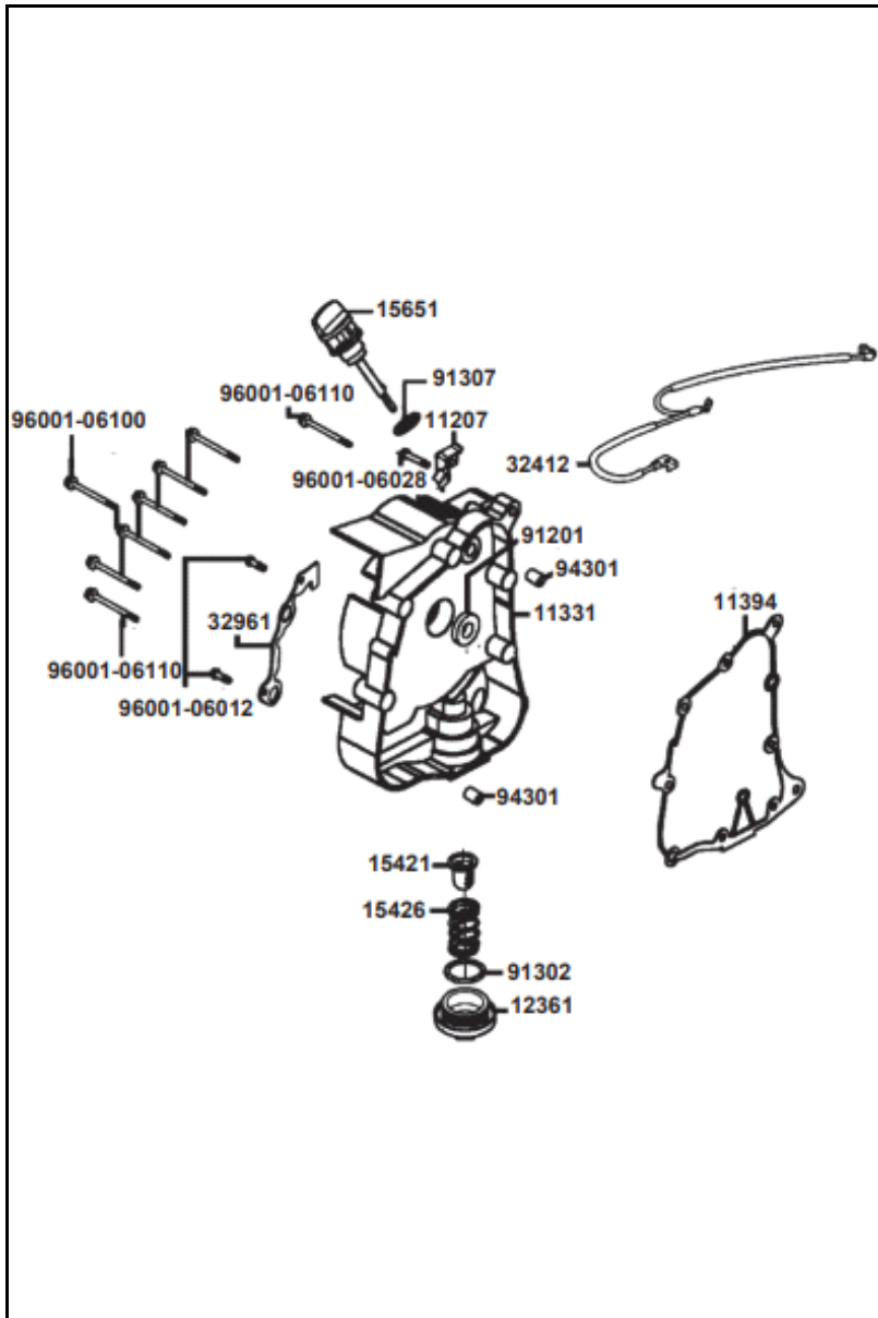
FIGURA N° 4: CUBIERTA MOTOR DERECHA
