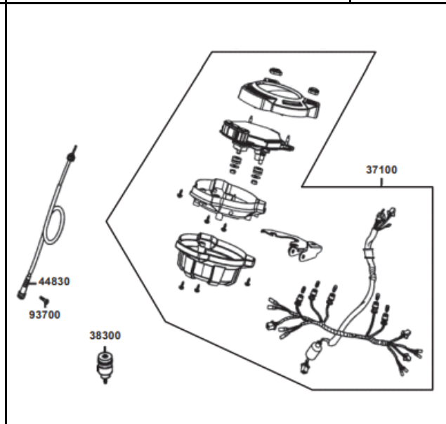
FIG. Nº 12 VELOCÍMETRO
