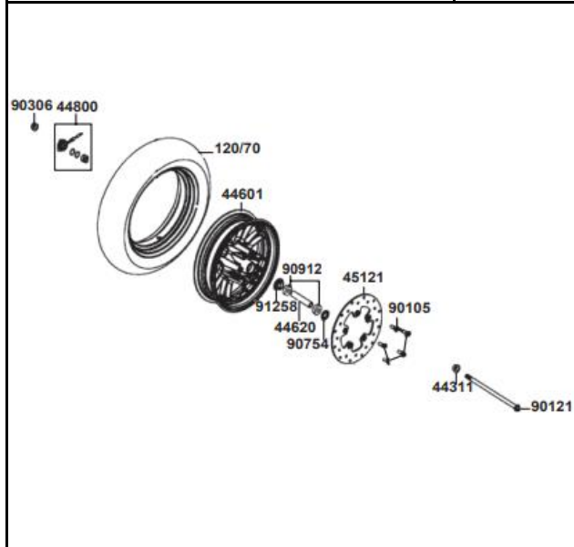
FIG. Nº 16 RIN DELANTERO
