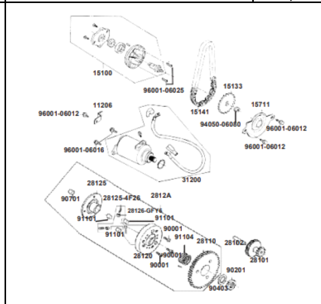
FIG. Nº 6 MOTOR DE ARRANQUE - BOMBA DE ACEITE
