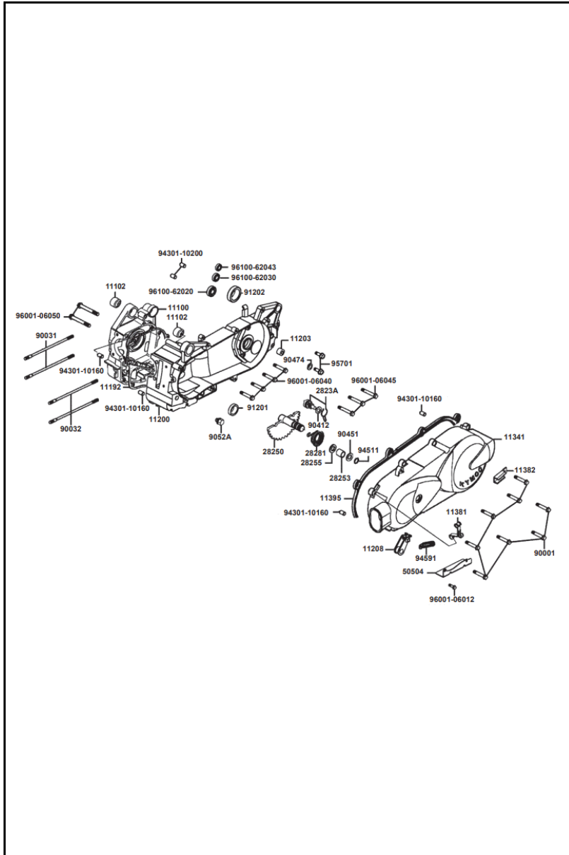
FIGURA N° 2: CARCASAS
