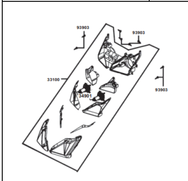
FIG. Nº 10 FAROLA
