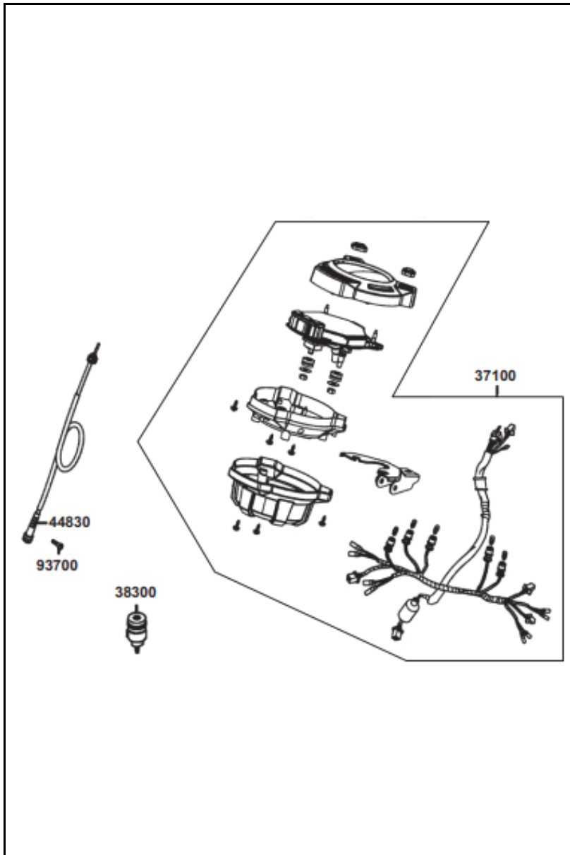
FIGURA N° 12: VELOCÍMETRO
