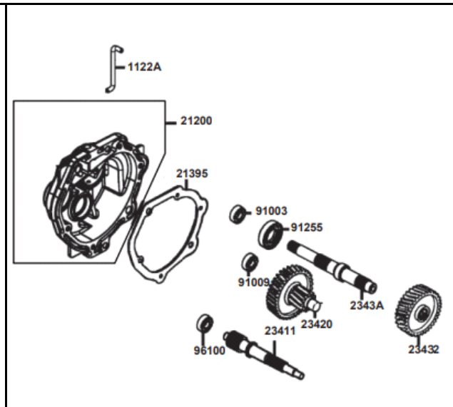
FIG. Nº 9 TRANSMISIÓN
