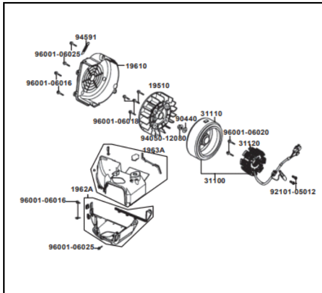
FIG. Nº 7 CUBIERTA VENTILADOR - MAGNETO
