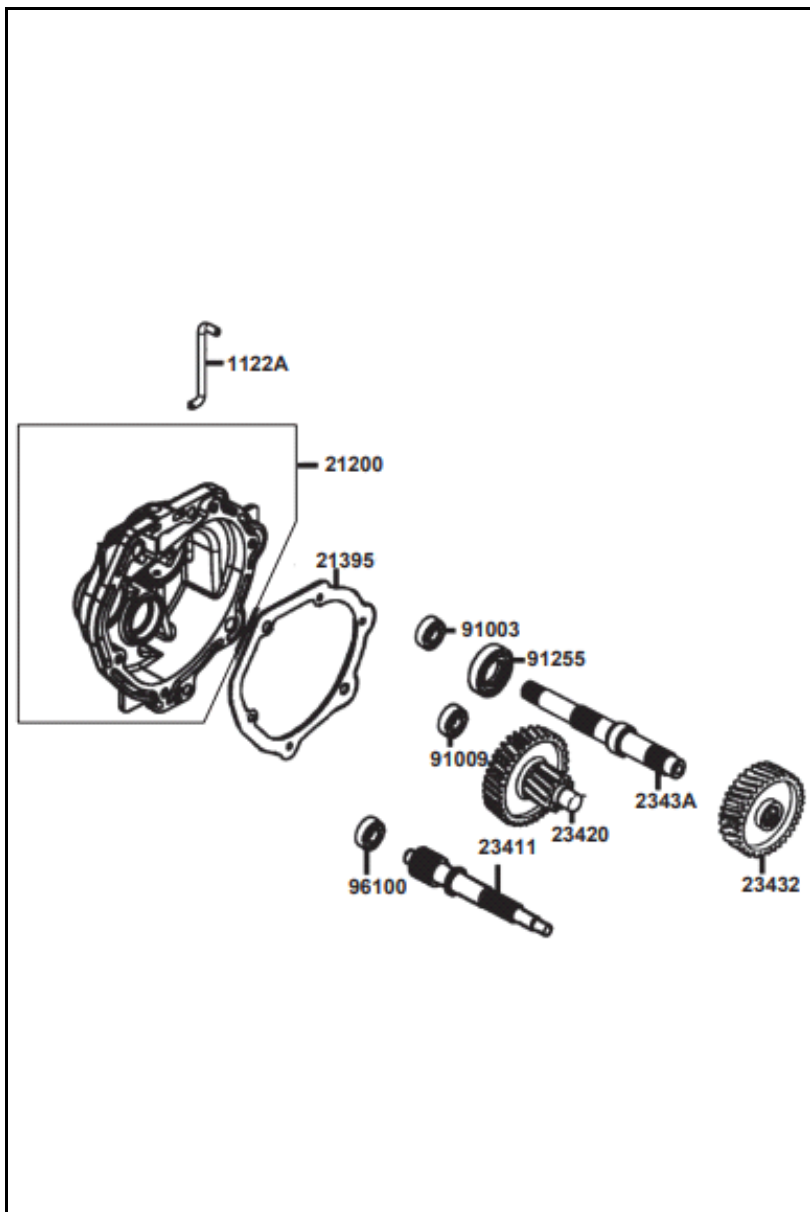
FIGURA N° 9: TRANSMISIÓN
