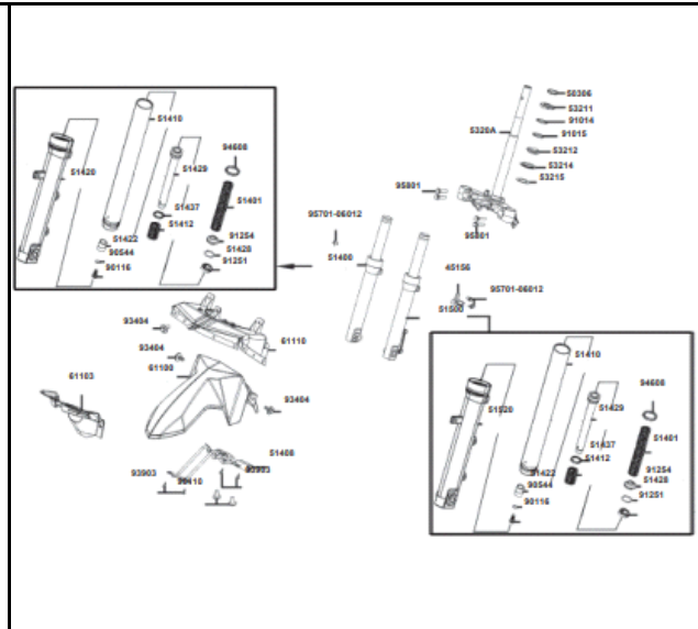
FIG. Nº 15 SUSPENSIÓN DELANTERA
