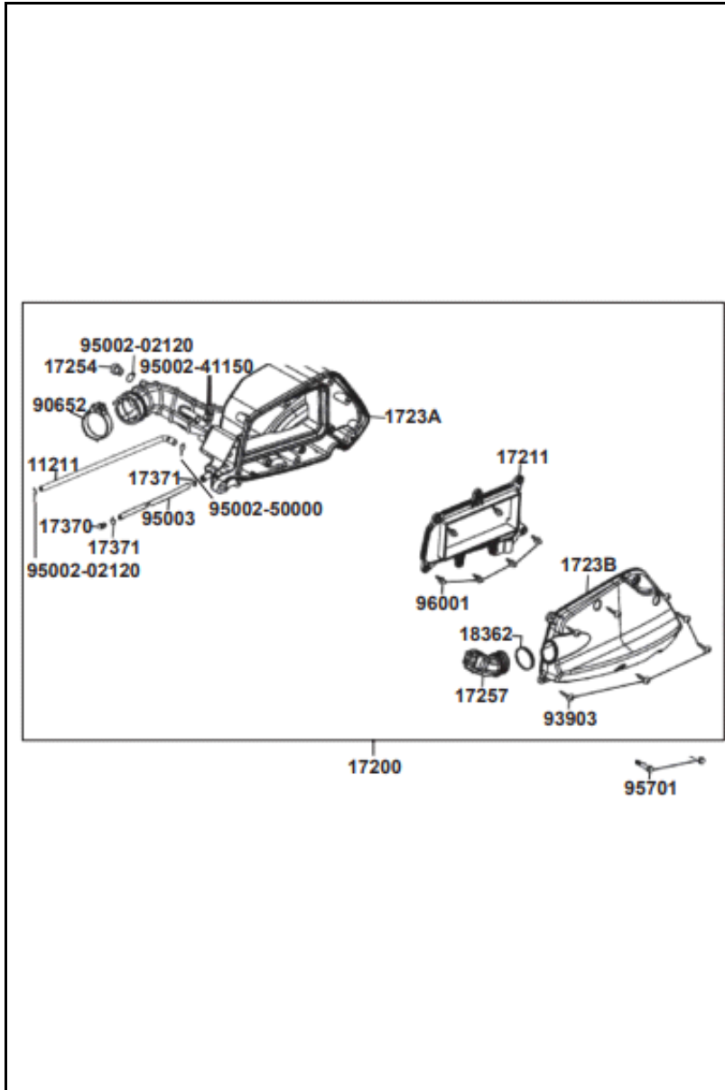
FIGURA N° 21: FILTRO DE AIRE
