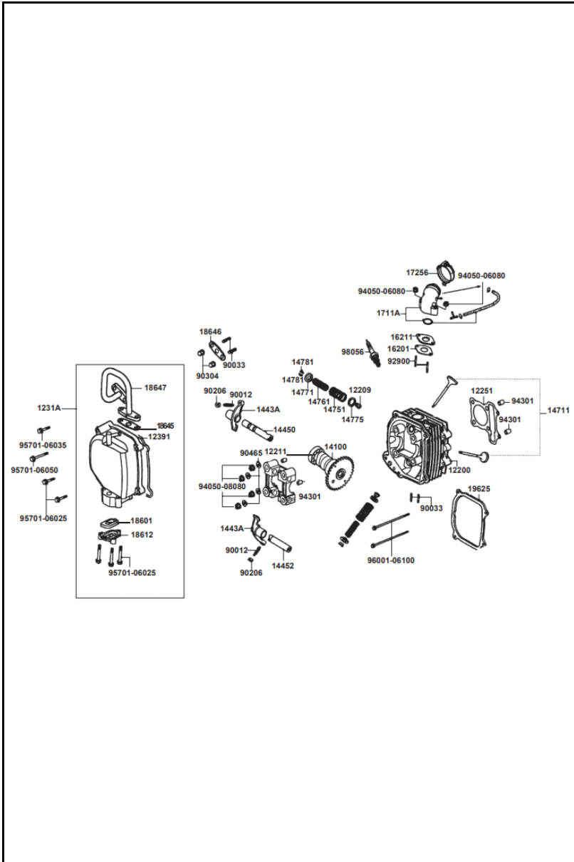
FIGURA N° 3: CULATA
