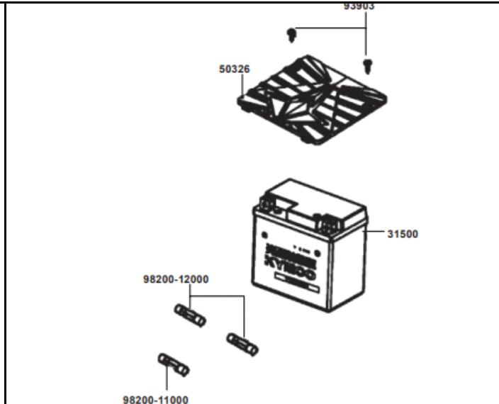
FIG. Nº 20 BATERÍA
