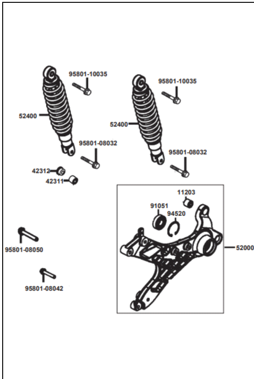
FIGURA N° 25: AMORTIGUADOR
