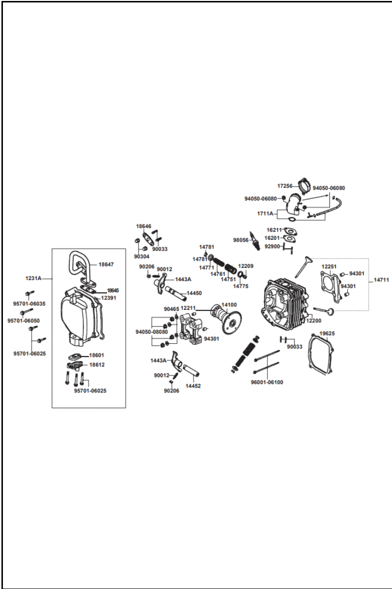
FIGURA N° 3: CULATA
