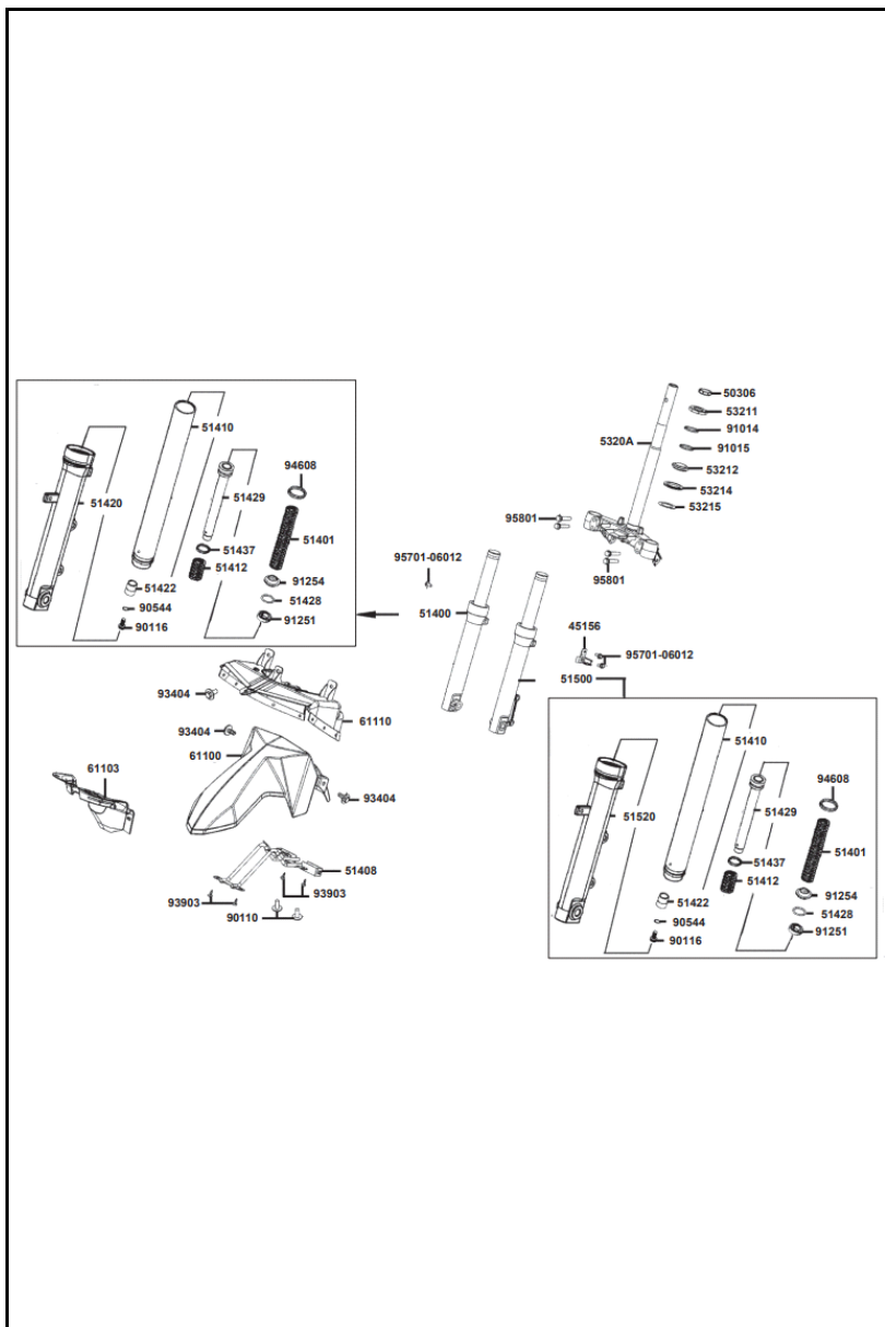
FIGURA N° 15: SUSPENSIÓN DELANTERA
