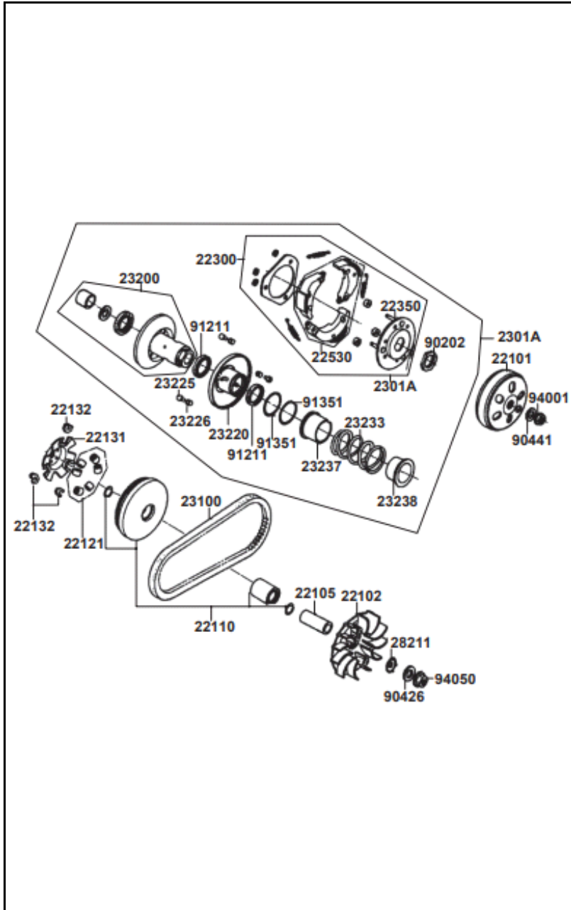
FIGURA N° 8: CLUTCH CENTRIFUGO
