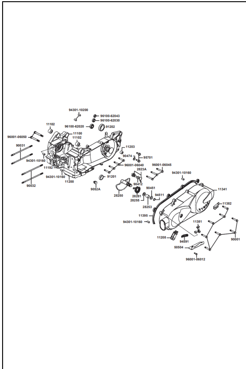
FIGURA N° 2: CARCASAS
