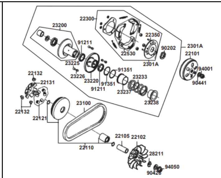
FIG. Nº 8 CLUTCH CENTRIFUGO
