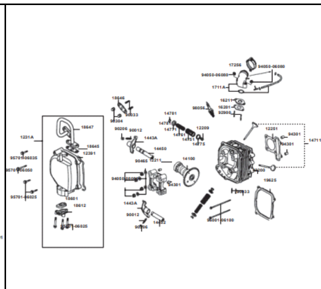
FIG. Nº 3 CULATA
