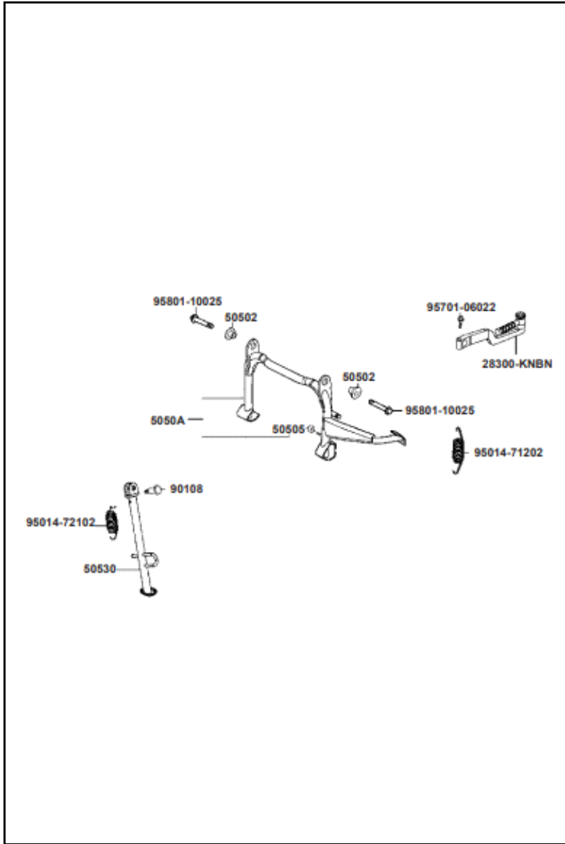
FIGURA N° 24: GATO LATERAL - PEDAL CRANK
