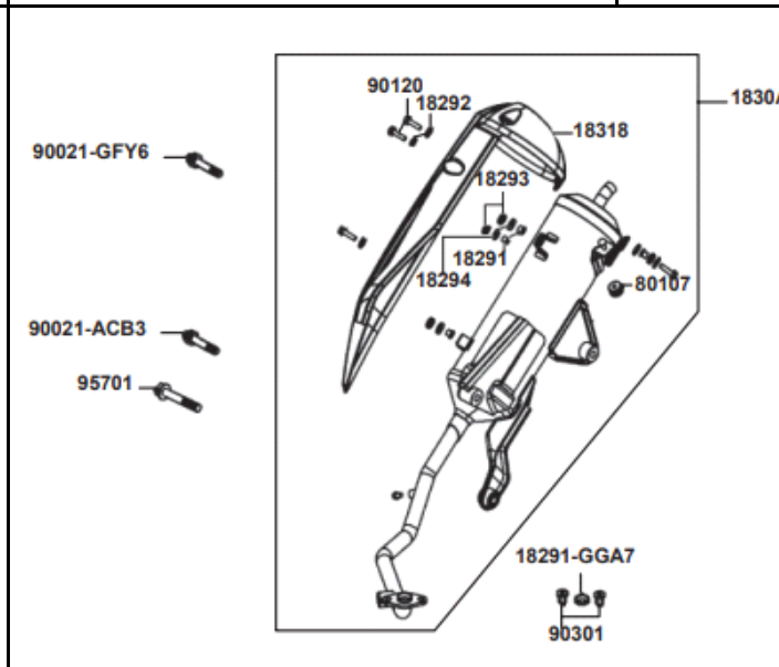
FIG. Nº 23 SILENCIADOR
