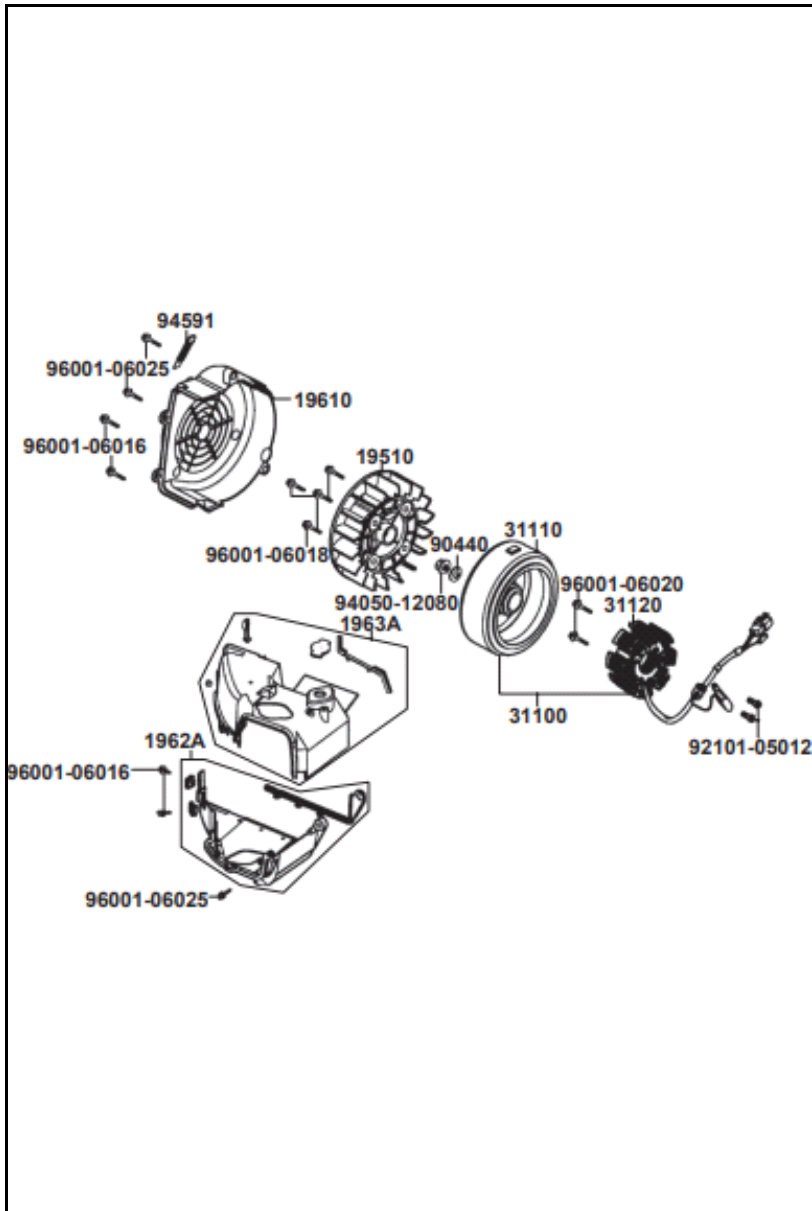
FIGURA N° 7: CUBIERTA VENTILADOR - MAGNETO
