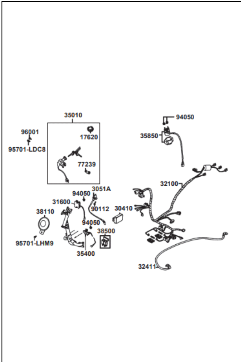
FIGURA N° 28: SISTEMA ELÉCTRICO
