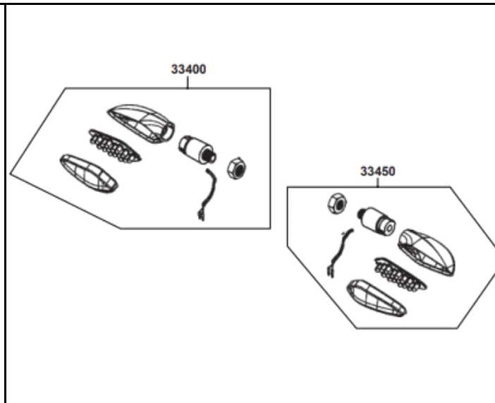
FIG. Nº 26 DIRECCIONALES DELANTERAS
