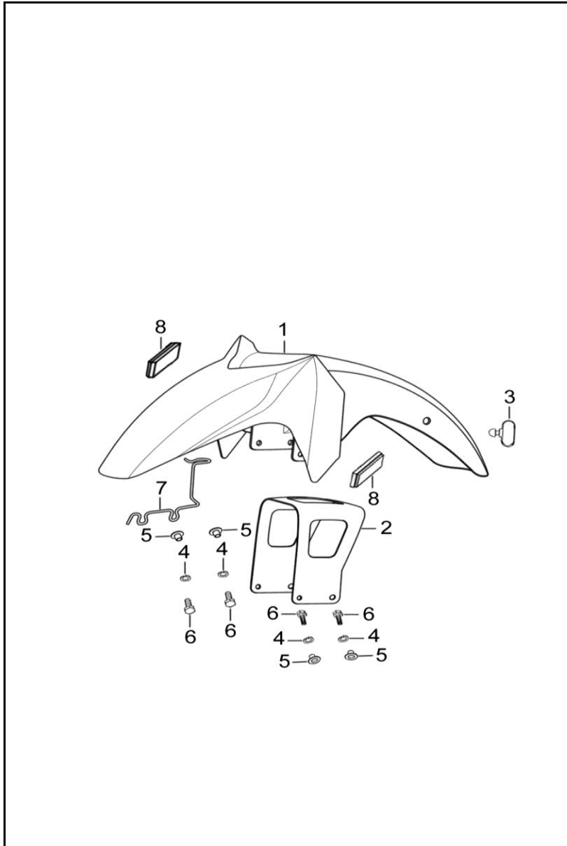
FIGURA N° 22: GUARDABARRO DELANTERO
