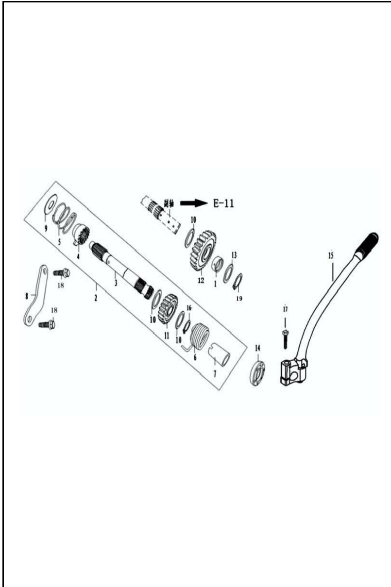
FIGURA N° 12: PEDAL CRANK - EJE CRANK
