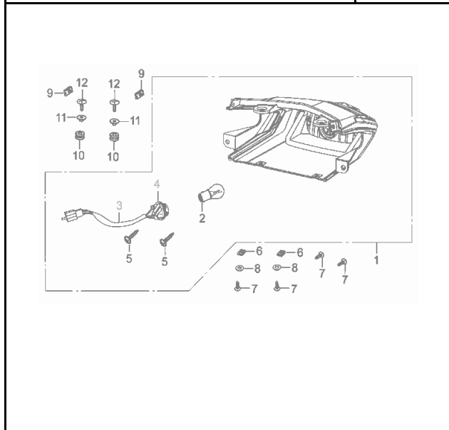
FIG. Nº 40: STOP
