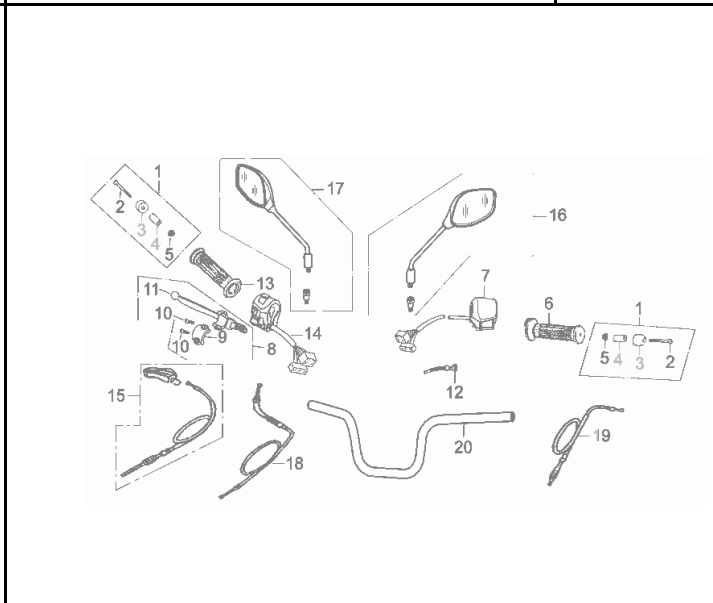
FIG. Nº 17: MANUBRIO - ESPEJOS - CABLES
