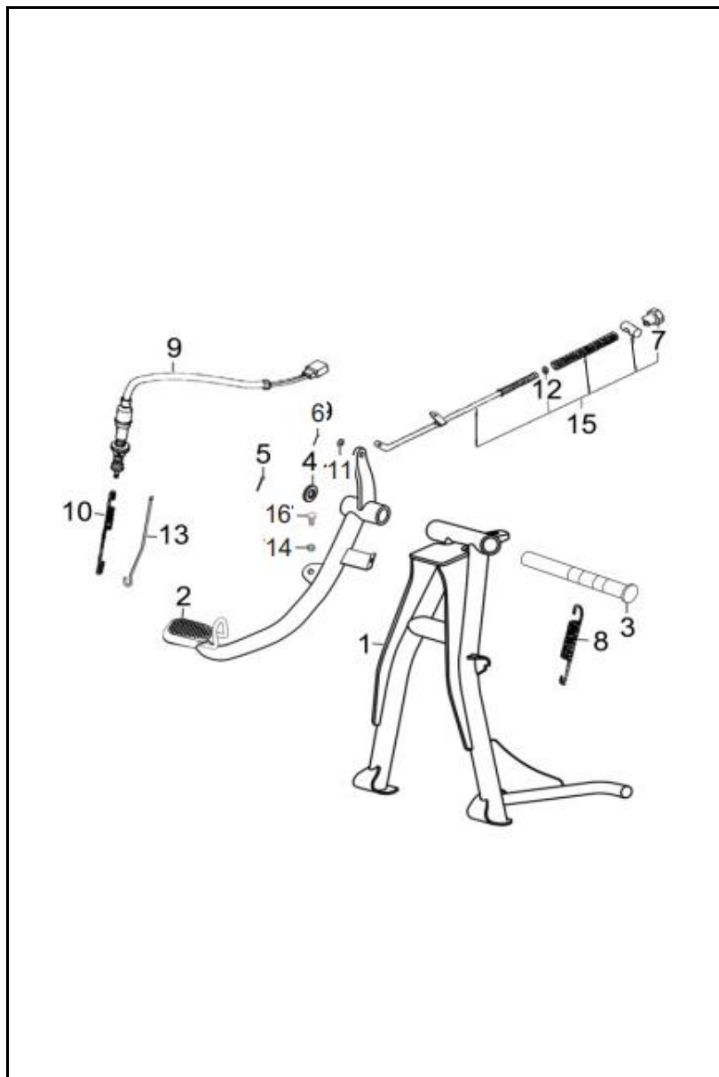
FIGURA N° 29: GATO CENTRAL - PEDAL FRENO
