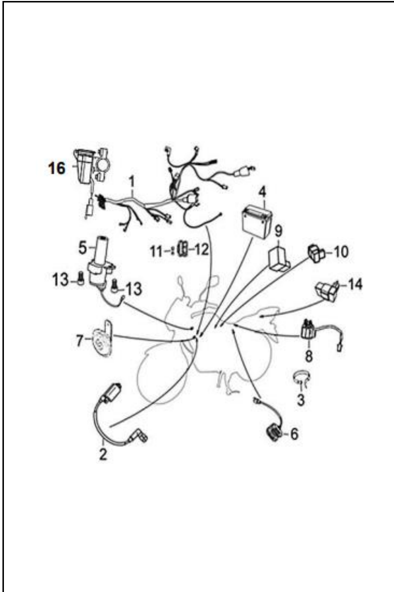
FIGURA N° 37: INSTALACIÓN ELÉCTRICA
