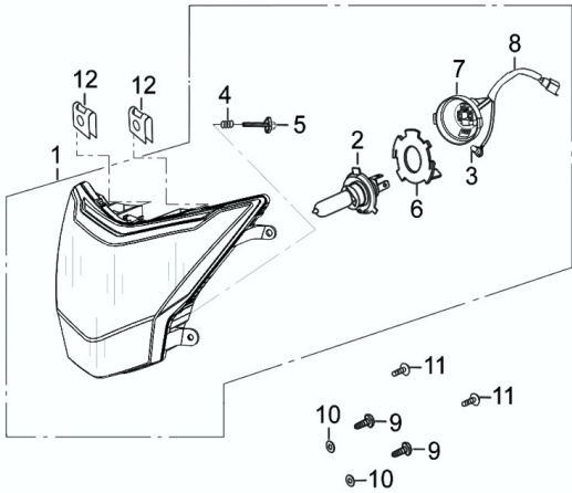
FIG. Nº 19: FAROLA
