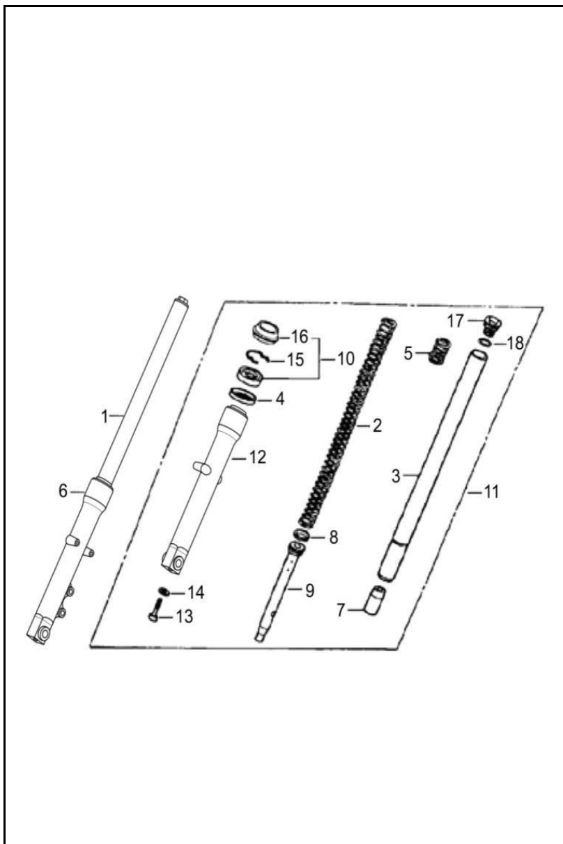
FIGURA N° 23: SUSPENSIÓN DELANTERA
