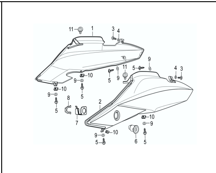
FIG. Nº 38: CUBIERTA SILLÍN
