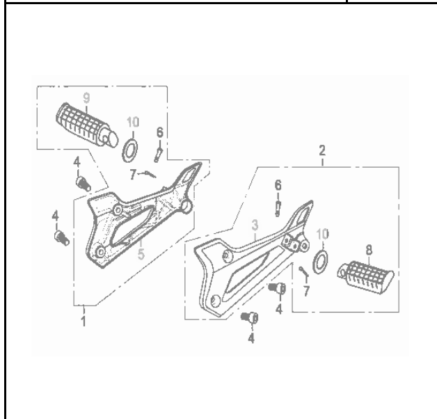
FIG. Nº 34: SOPORTE REPOSAPIE - PASAJERO
