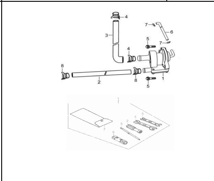
FIG. Nº 41: VÁLVULA DE AIRE - ESTUCHE HERRAJE
