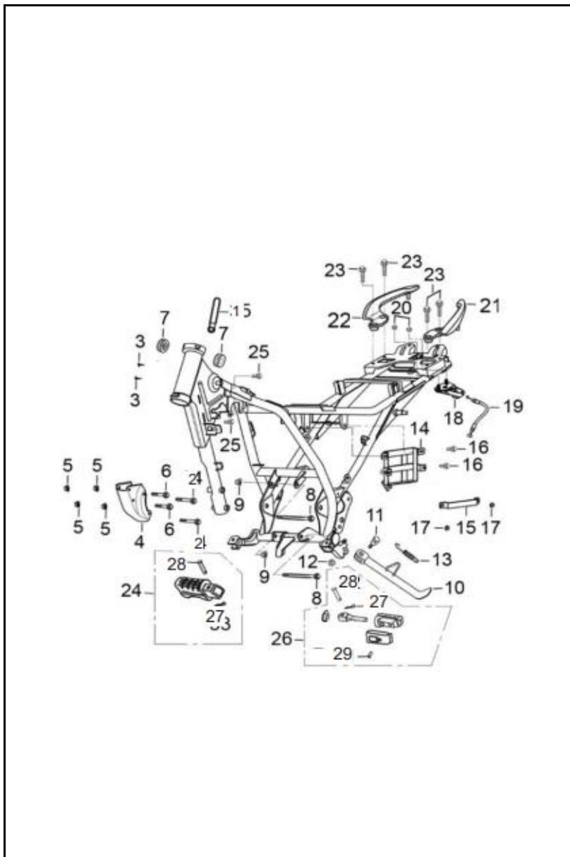
FIGURA N° 16: COMPLEMENTOS CHASIS - GATO LATERAL (2/2)
