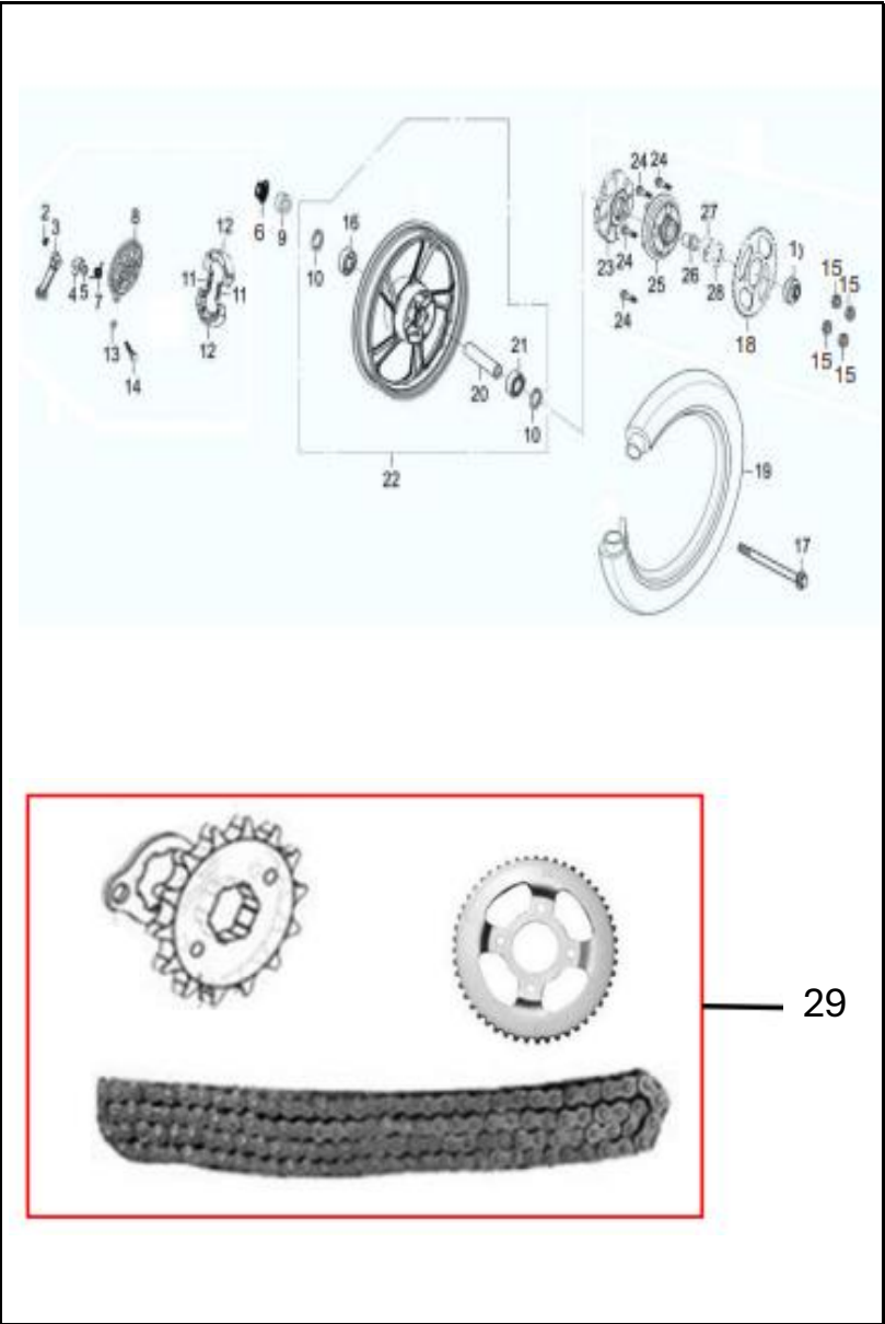
FIGURA N° 33: RUEDA TRASERA (2/2)
