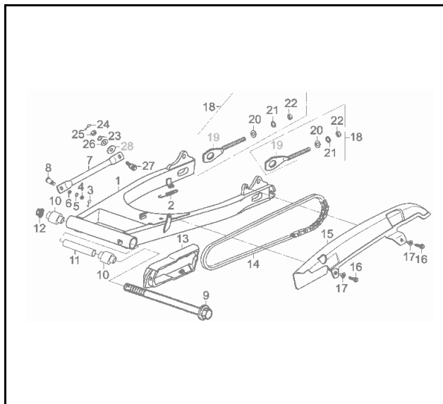
FIG. Nº 31: BRAZO OSCILANTE
