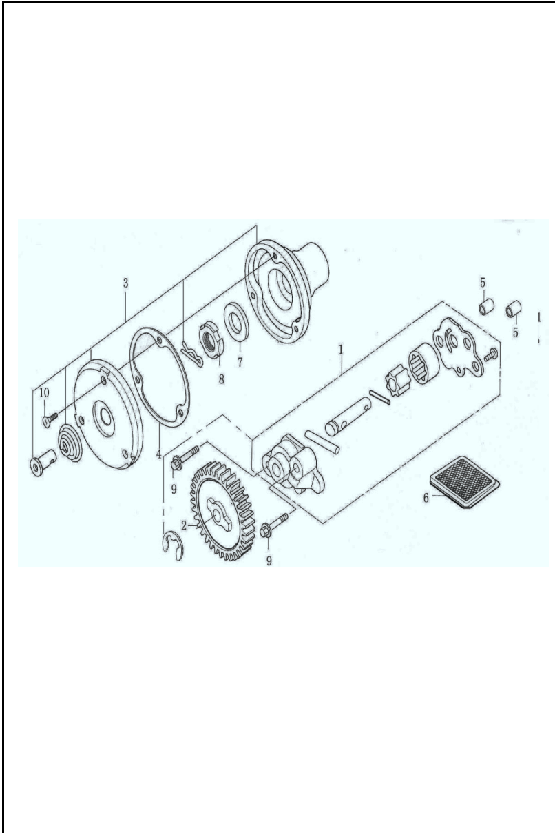
FIGURA N° 7: BOMBA ACEITE - FILTRO CENTRIFUGO ACEITE
