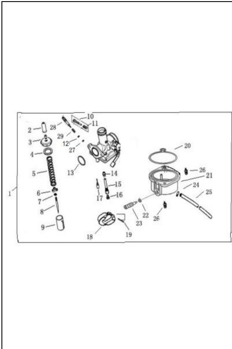
FIGURA N° 13: CARBURADOR (1/2)
