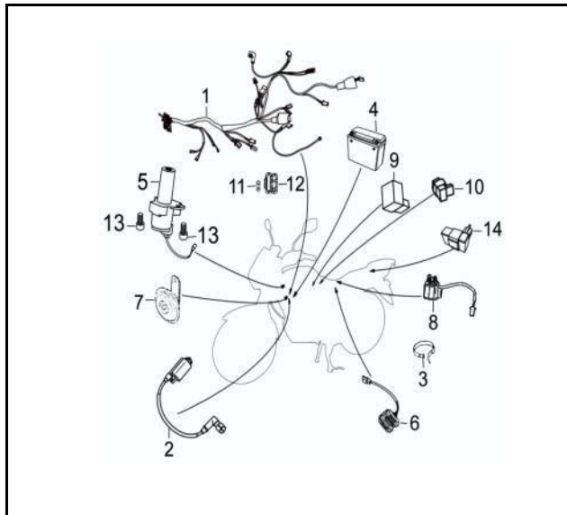
FIG. Nº 37: INSTALACIÓN ELÉCTRICA
