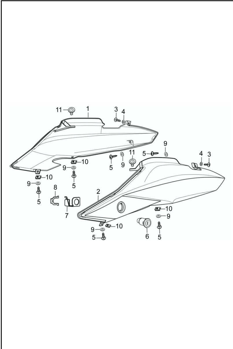
FIGURA N° 38: CUBIERTA SILLÍN
