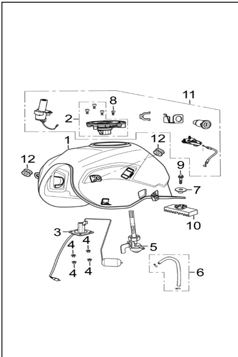
FIGURA N° 26: TANQUE GASOLINA
