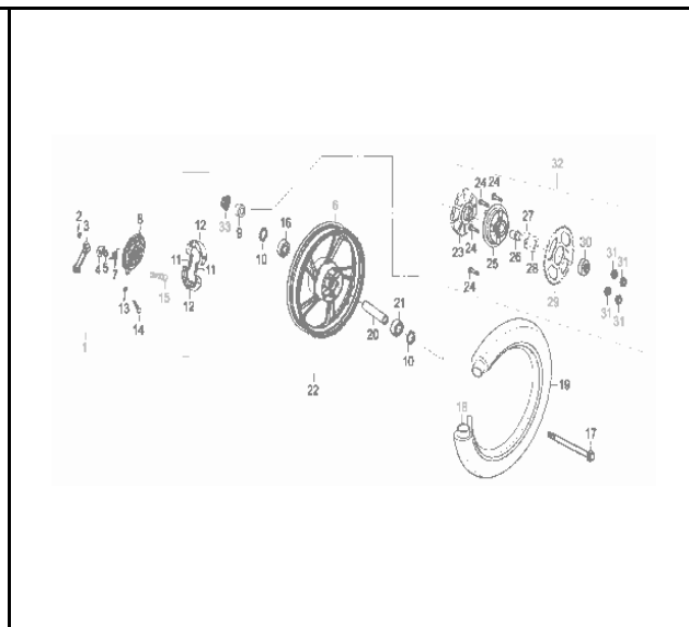
FIG. Nº 33: RUEDA TRASERA
