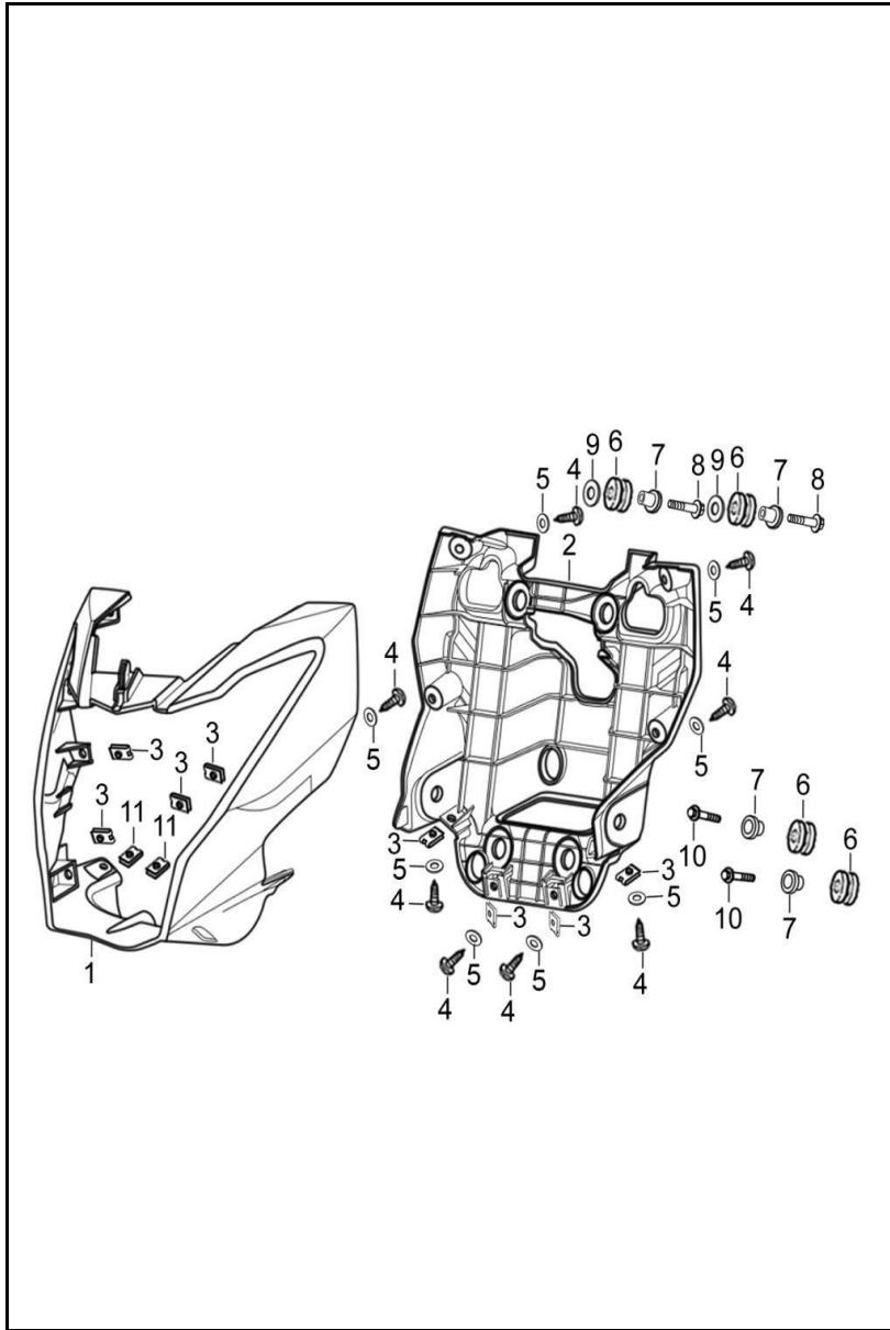
FIGURA N° 20: CARENAJE FAROLA
