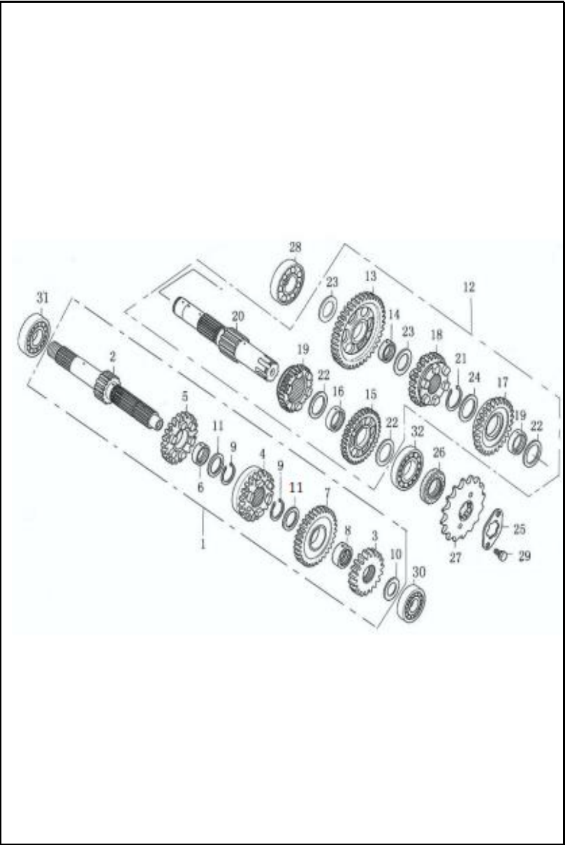
FIGURA N° 10: TRANSMISIÓN (2/2)
