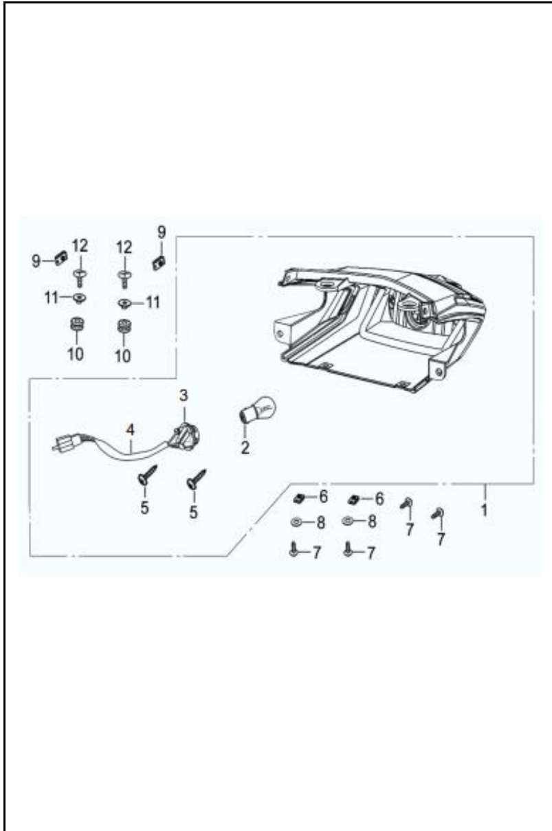
FIGURA N° 40: STOP
