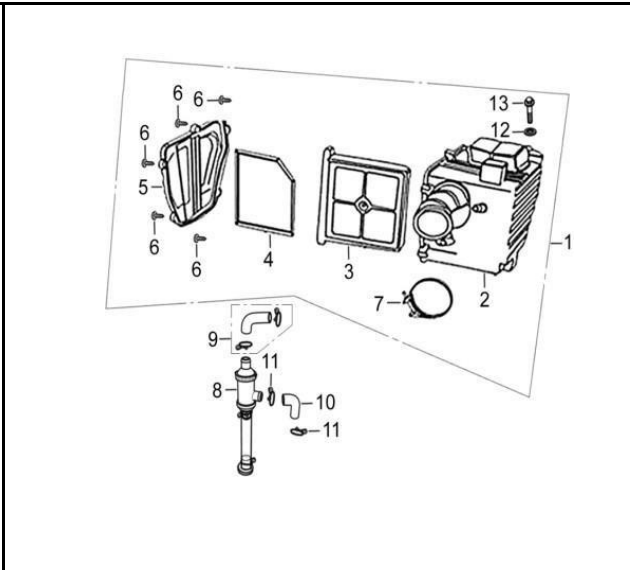
FIG. Nº 15: CAJA FILTRO AIRE
