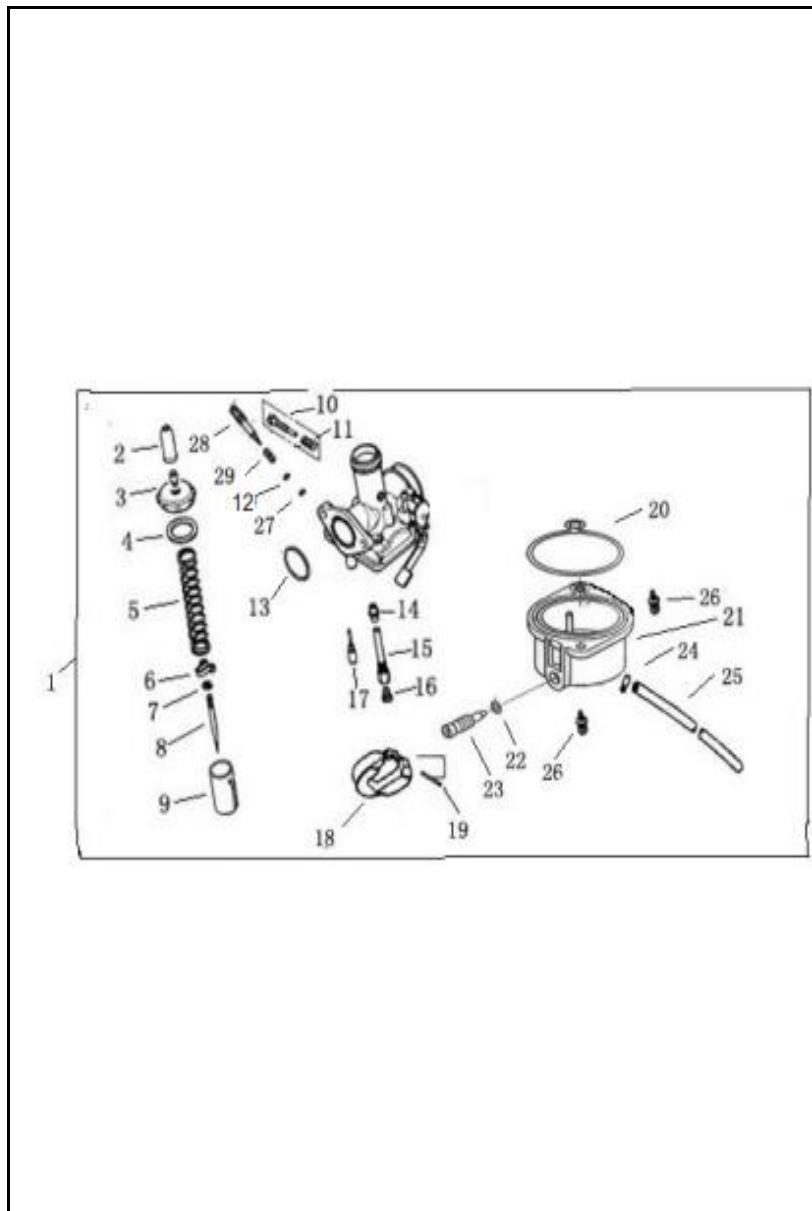
FIGURA N° 13 : CARBURADOR (2/2)
