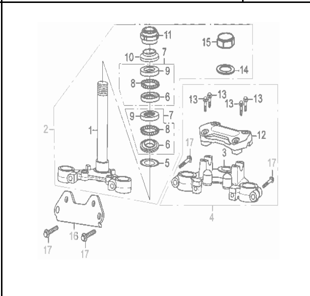
FIG. Nº 18: ESPIGA CENTRAL - CABEZA ESPIGA
