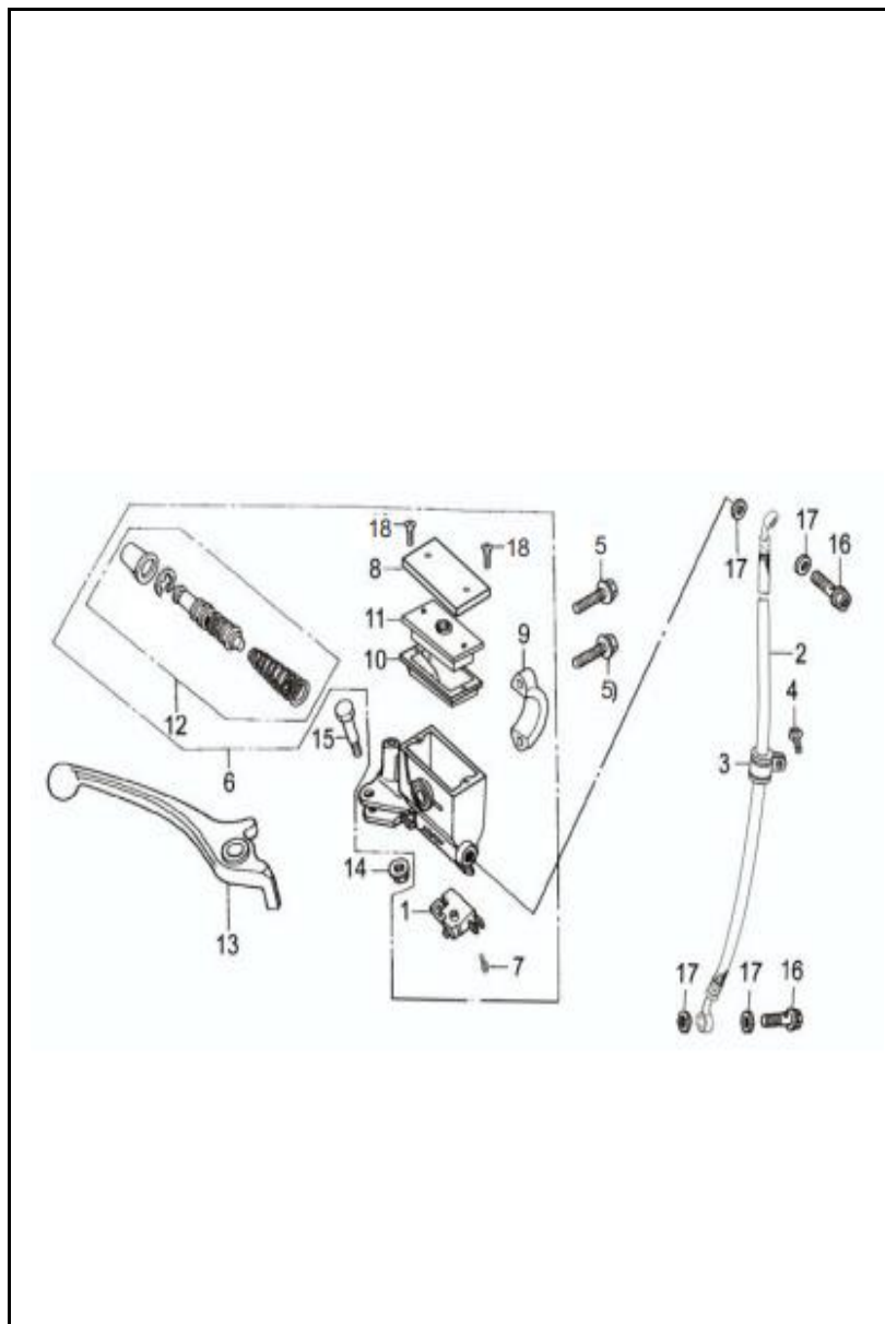
FIGURA N° 24: BOMBA FRENO DELANTERO
