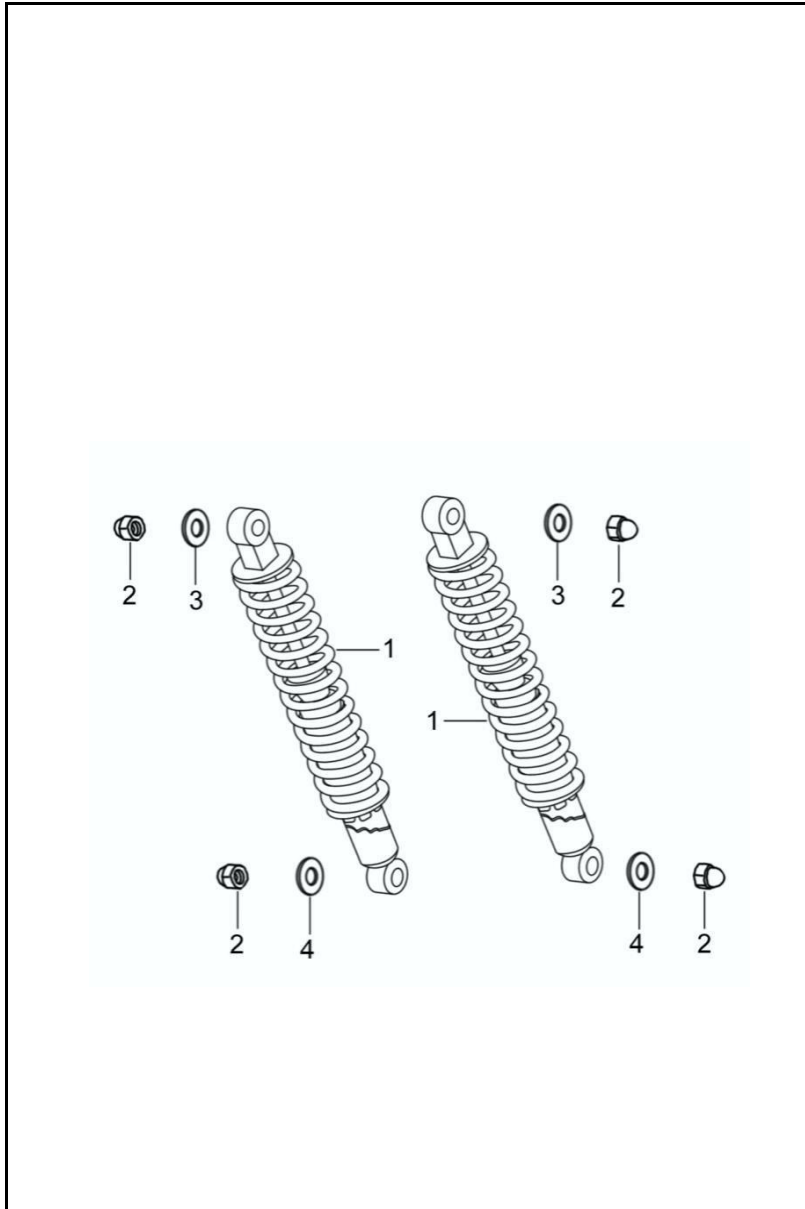
FIGURA N° 35: AMORTIGUADOR
