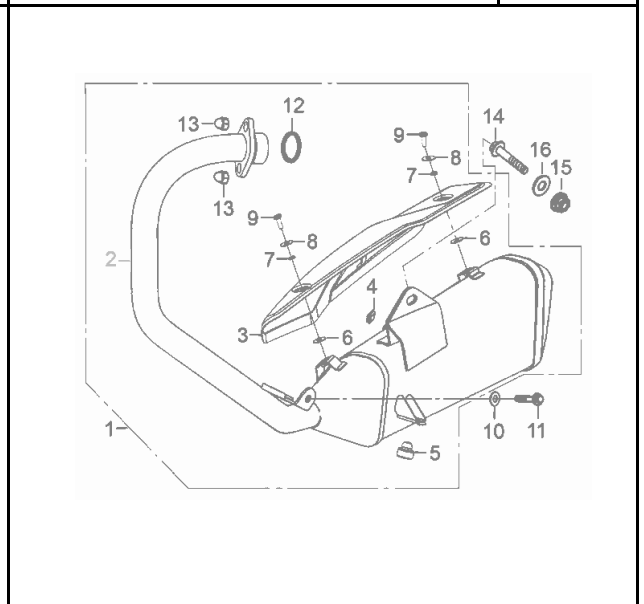
FIG. Nº 30: SILENCIADOR
