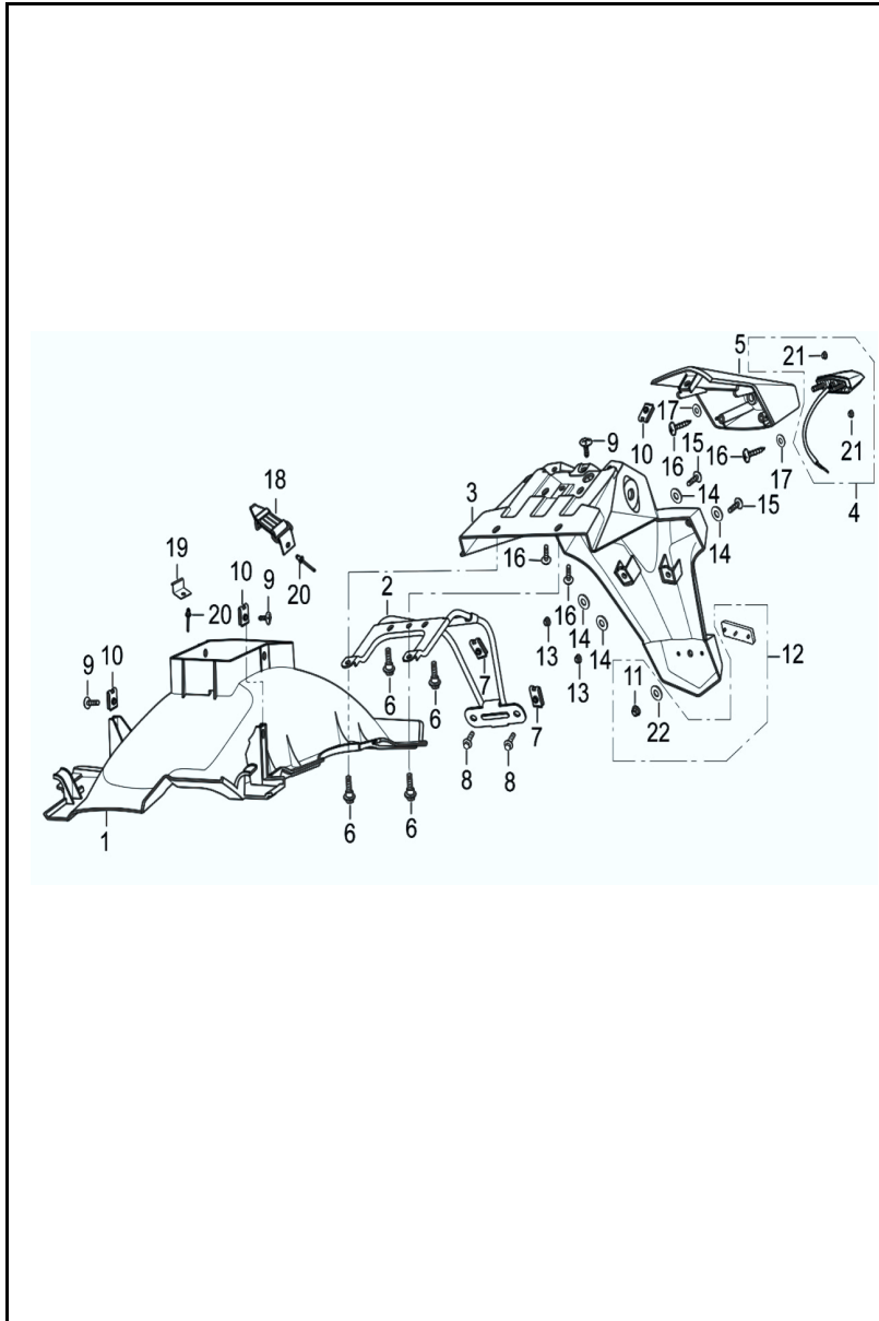
FIGURA N° 36: GUARDABARRO TRASERO
