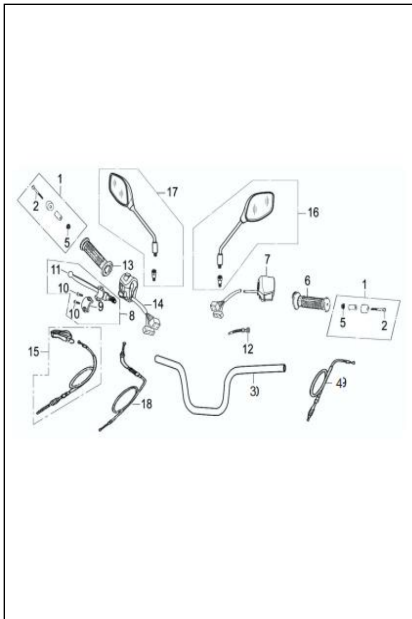
FIGURA N° 17: MANUBRIO - ESPEJOS - CABLES
