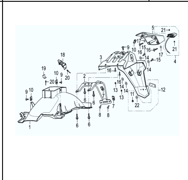
FIG. Nº 36: GUARDABARRO TRASERO
