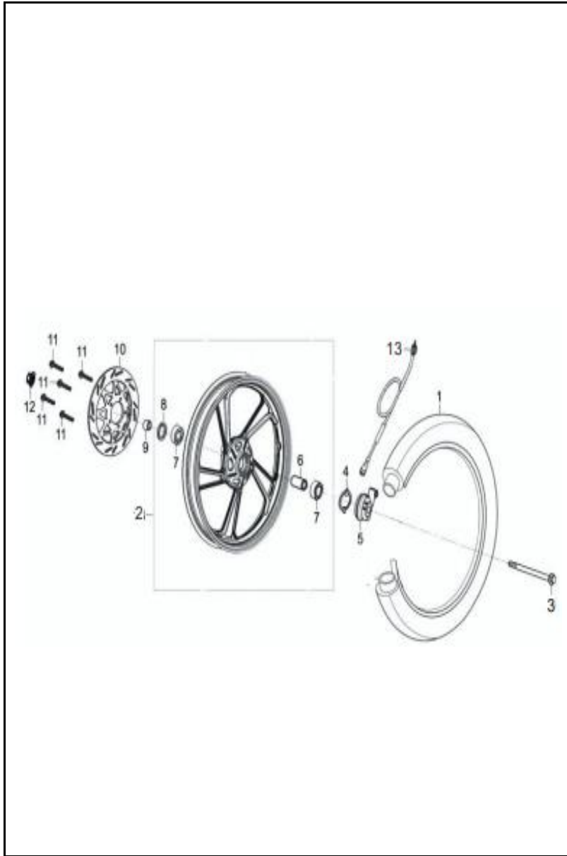
FIGURA N° 32: RUEDA DELANTERA
