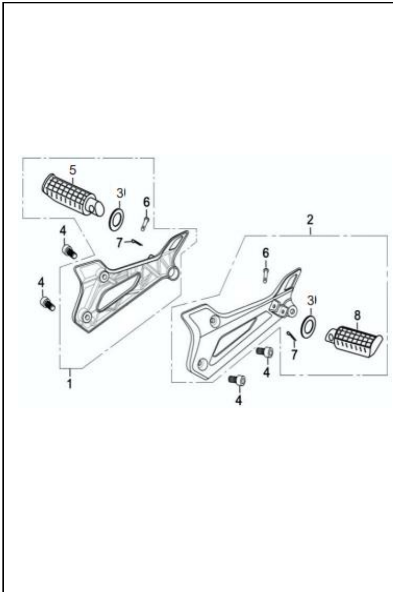
FIGURA N° 34: SOPORTE REPOSAPIE PASAJERO
