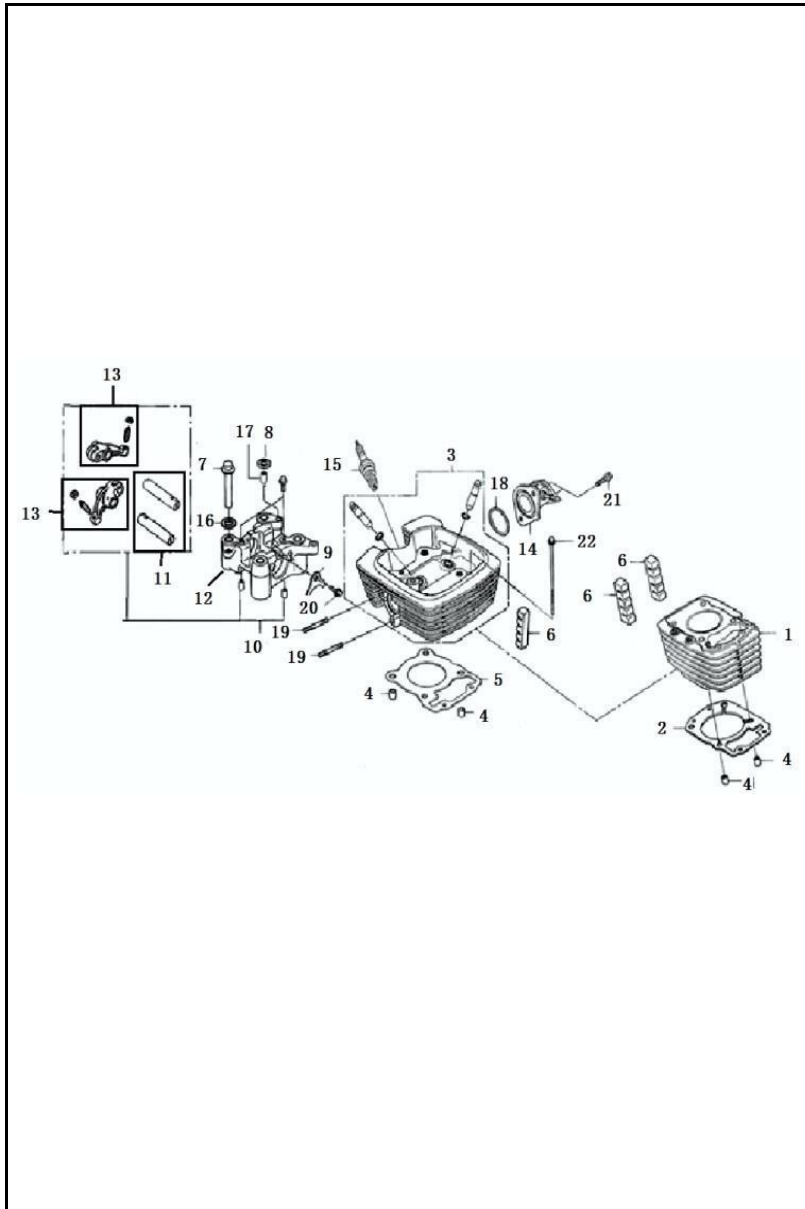
FIGURA N° 1: CILINDRO - CULATA
