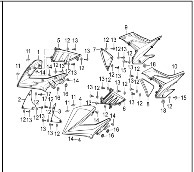
FIG. Nº 27: CUBIERTAS
