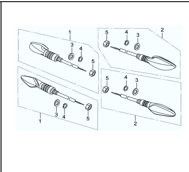
FIG. Nº 39: DIRECCIONALES
