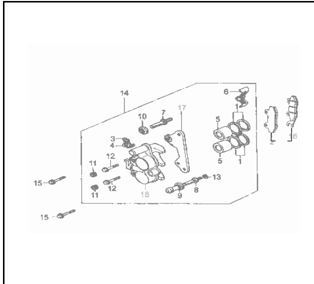
FIG. Nº 25: CALIPER DELANTERO
