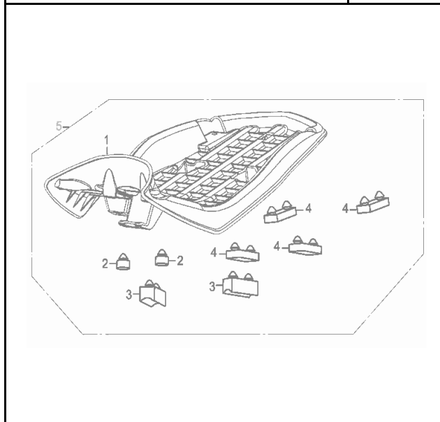
FIG. Nº 28: SILLÍN
