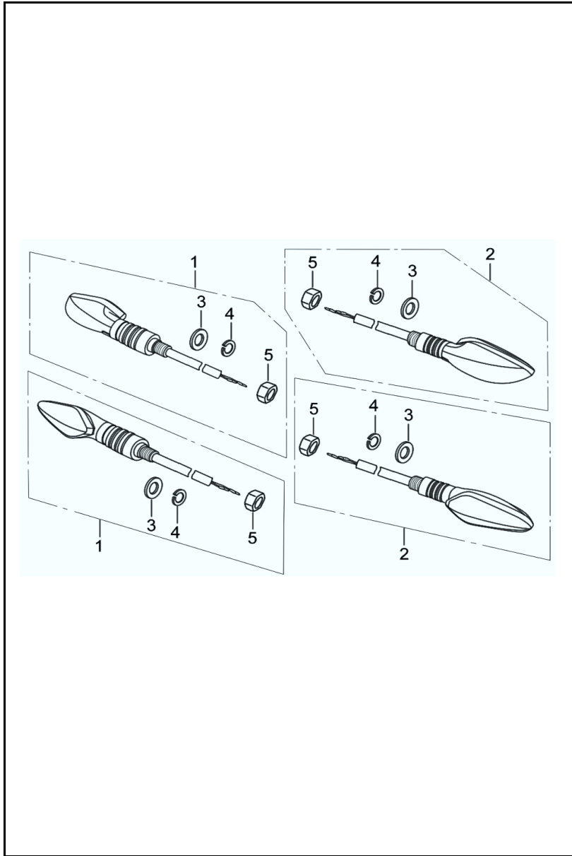
FIGURA N° 39: DIRECCIONALES
