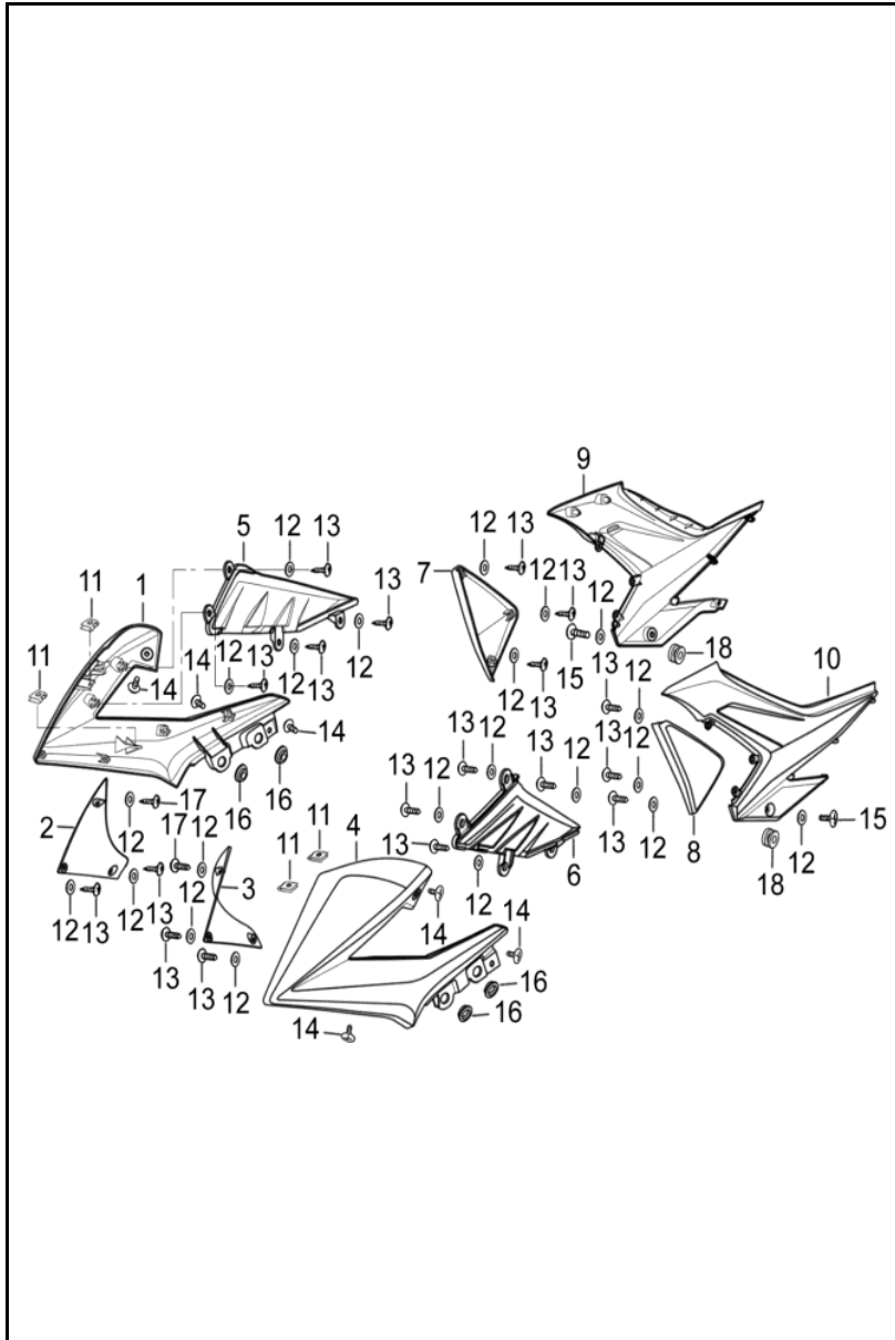
FIGURA N° 27: CUBIERTAS
