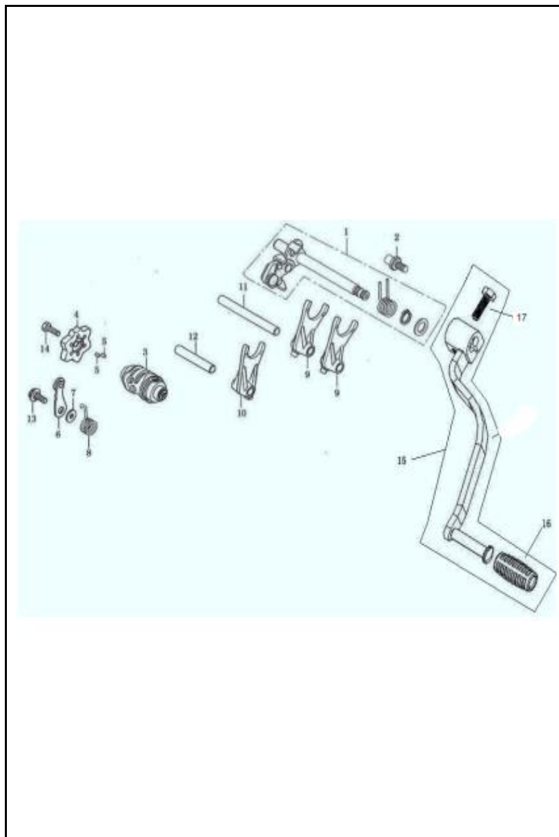
FIGURA N° 11: EJE CAMBIOS - PEDAL CAMBIOS
