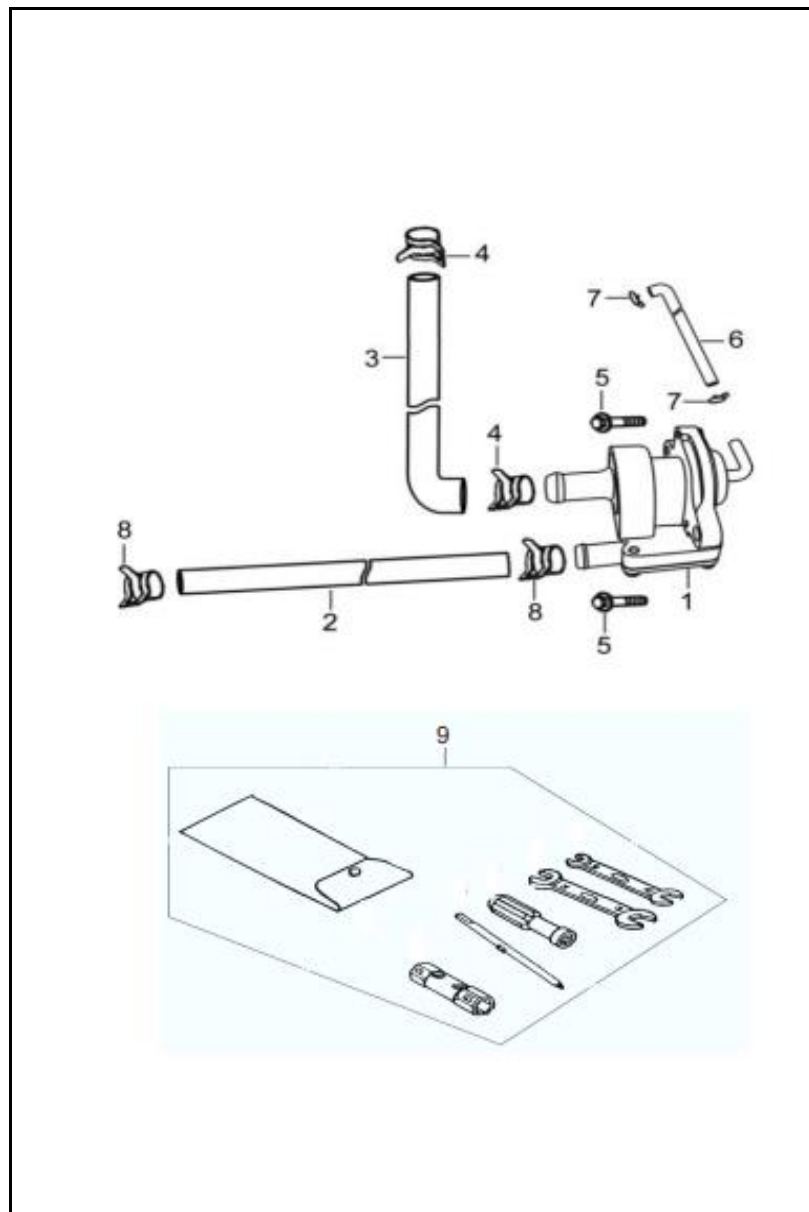
FIGURA Nº 41: VÁLVULA DE AIRE - ESTUCHE HERRAMIENTA
