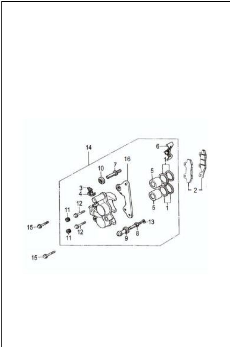
FIGURA N° 25: CALIPER DELANTERO
