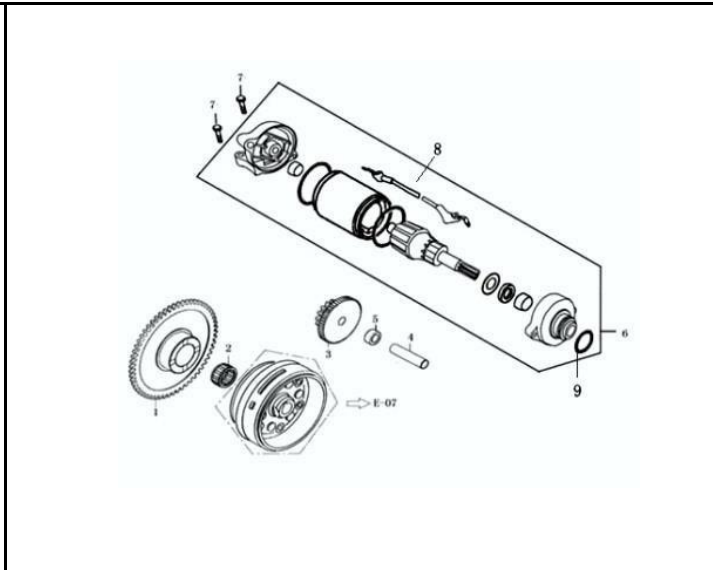
FIG. Nº 14: MOTOR DE ARRANQUE
