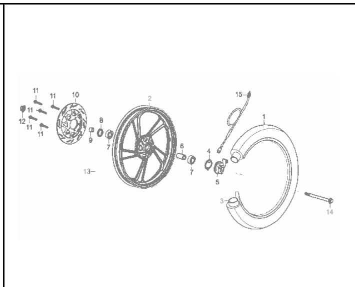
FIG. Nº 32: RUEDA DELANTERA
