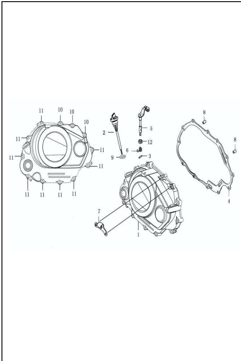
FIGURA N° 4: CUBIERTA CLUTCH
