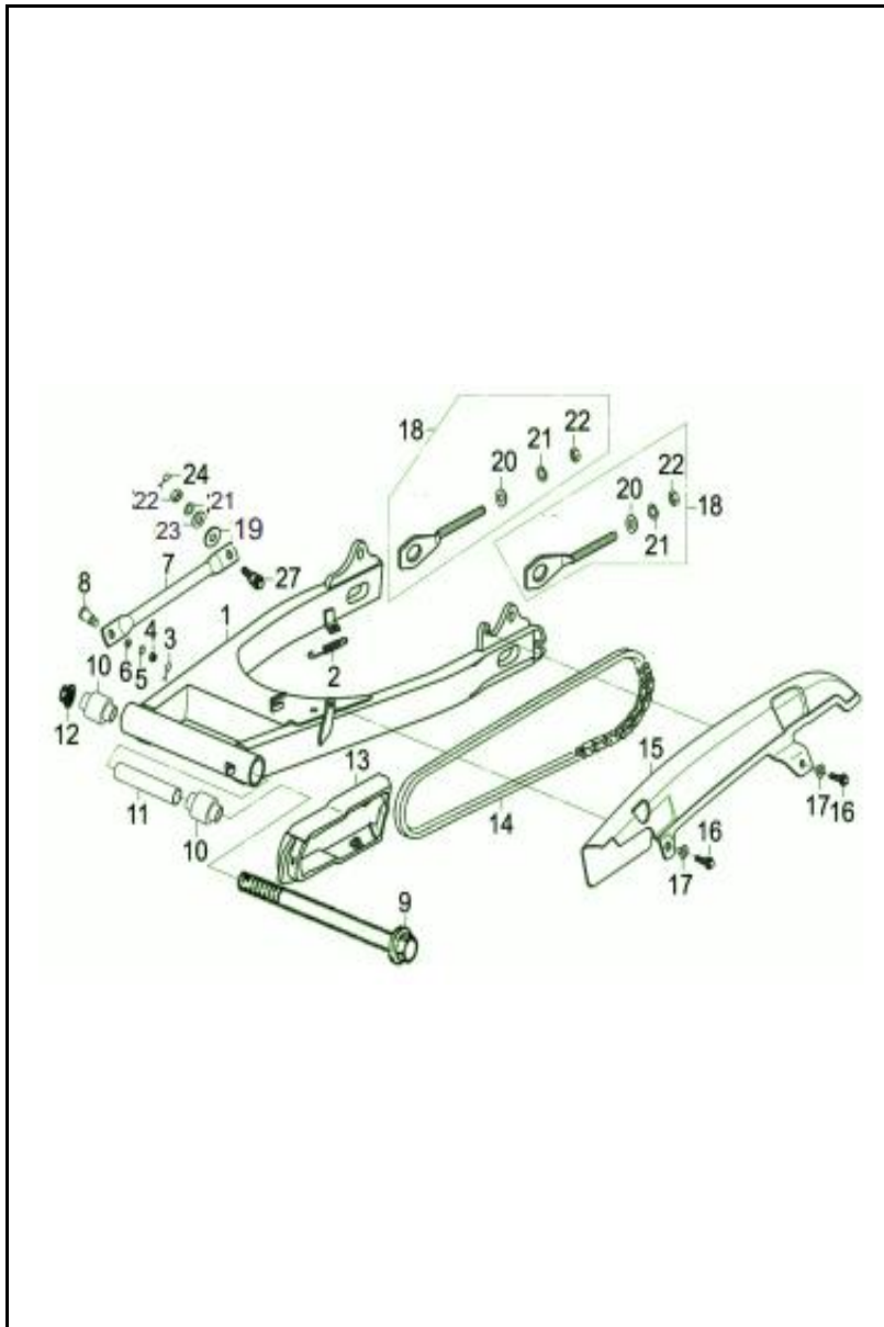
FIGURA N° 31: BRAZO OSCILANTE
