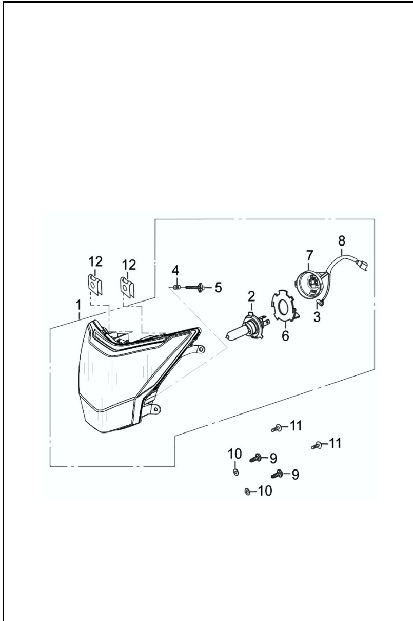
FIGURA N° 19: FAROLA
