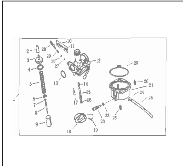
FIG. Nº 13: CARBURADOR
