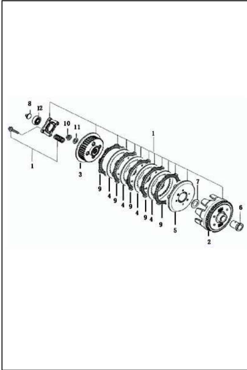
FIGURA N° 5: CLUTCH
