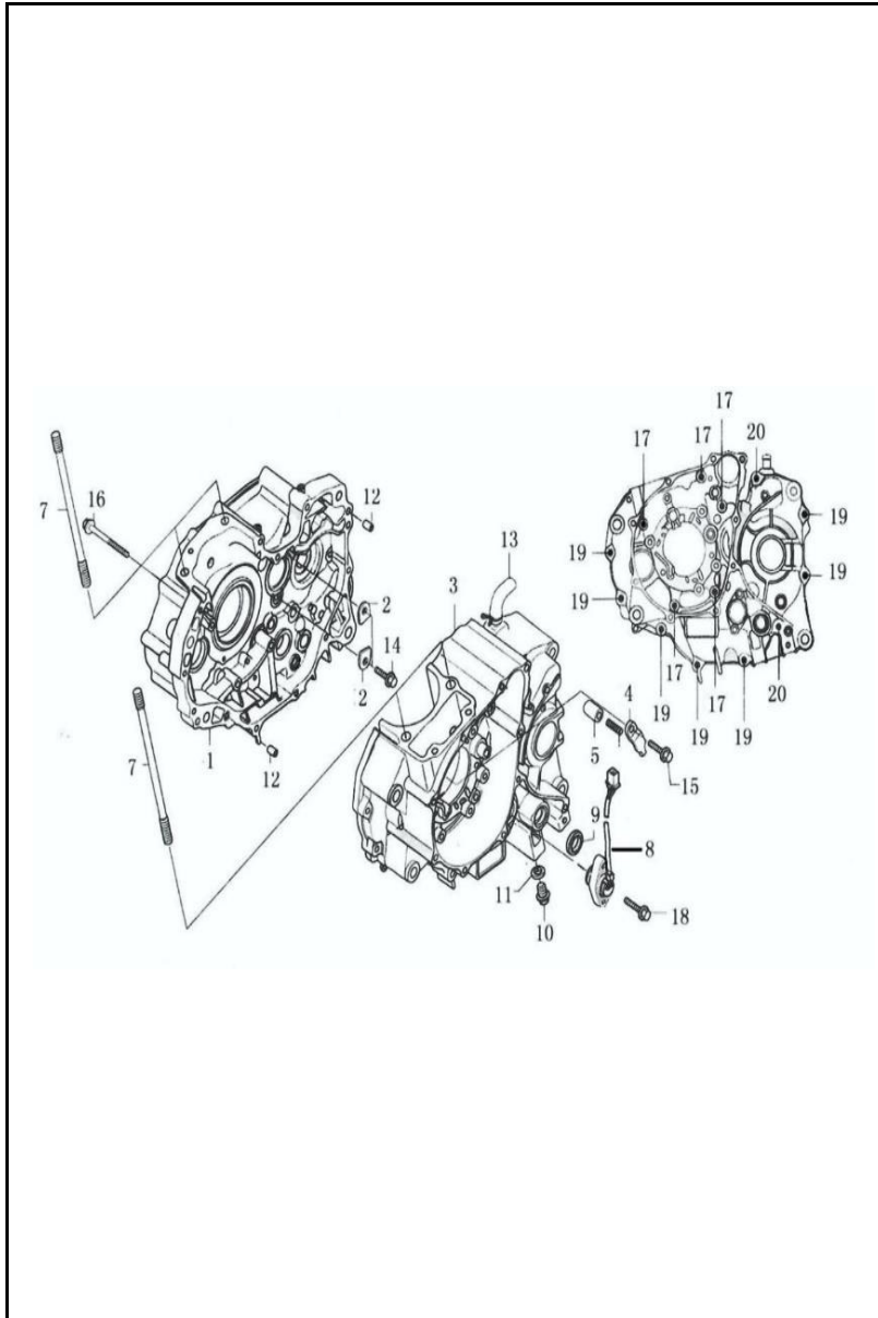
FIGURA N° 8: CARCASAS
