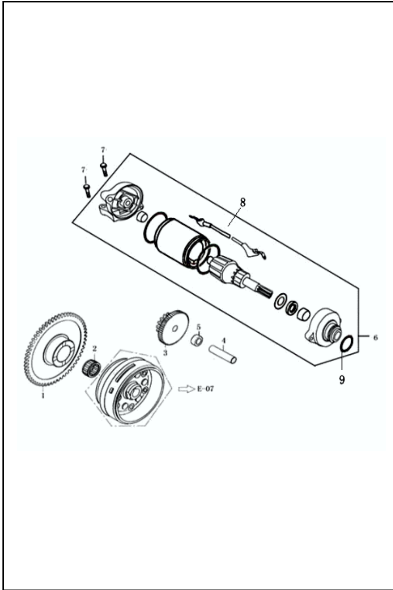
FIGURA N° 14: MOTOR DE ARRANQUE
