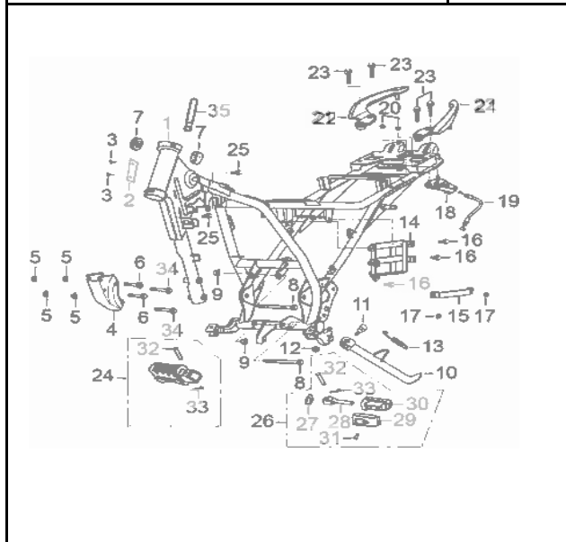
FIG. Nº 16: COMPLEMENTOS CHASIS - GATO LATERAL
