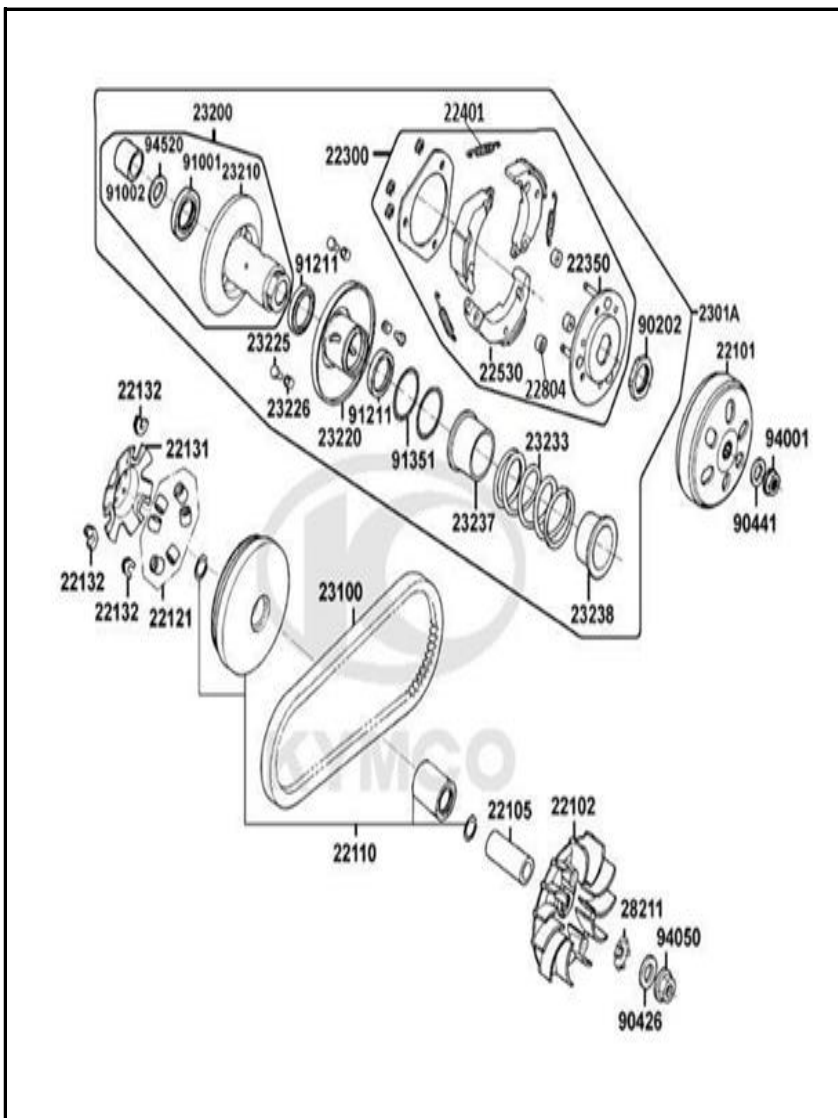
FIGURA N° 5: CLUTCH CENTRIFUGO 1/2
