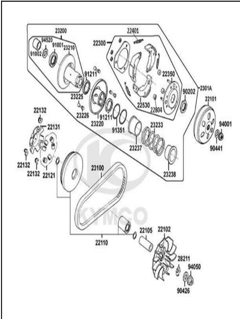
FIGURA N° 5: CLUTCH CENTRIFUGO 2/2
