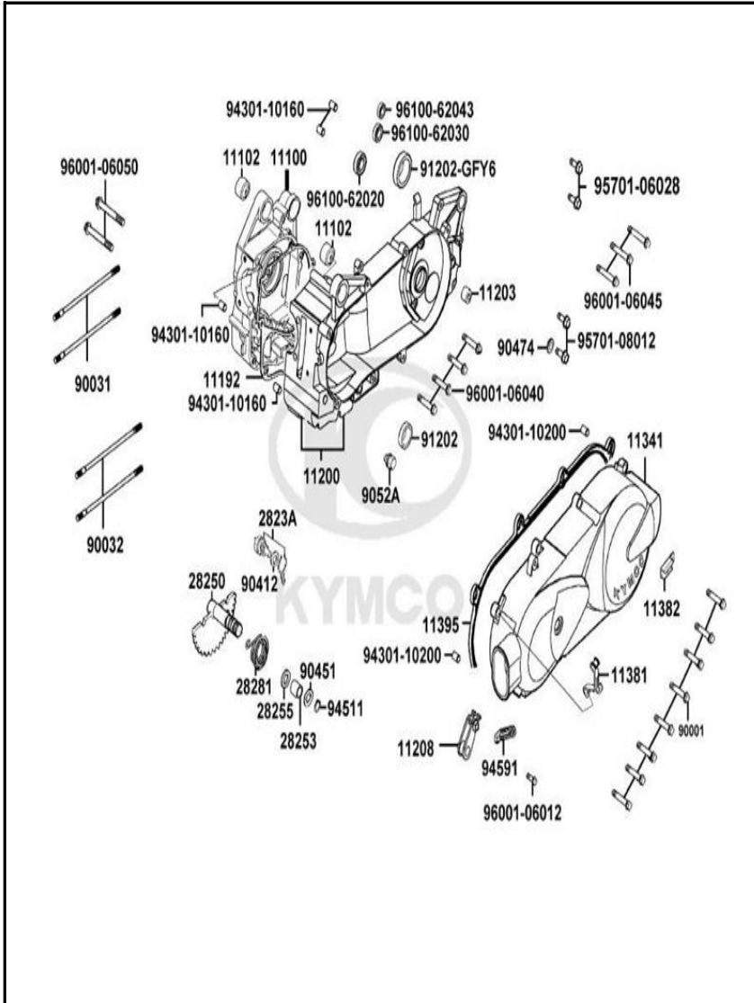
FIGURA N° 1: CARCASAS 1/2
