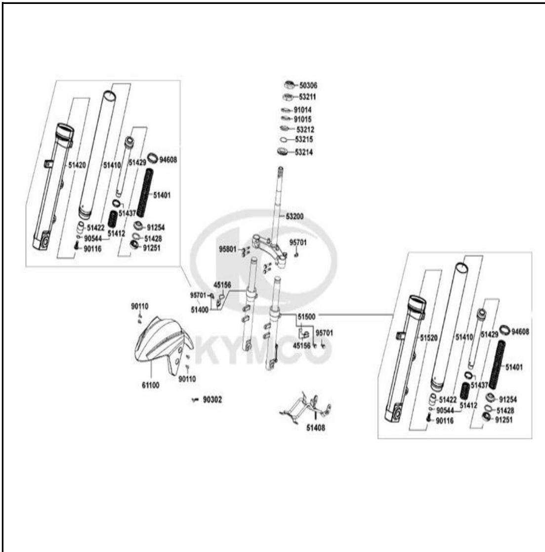
FIGURA N° 15: SUSPENSION DELANTERA 2/2
