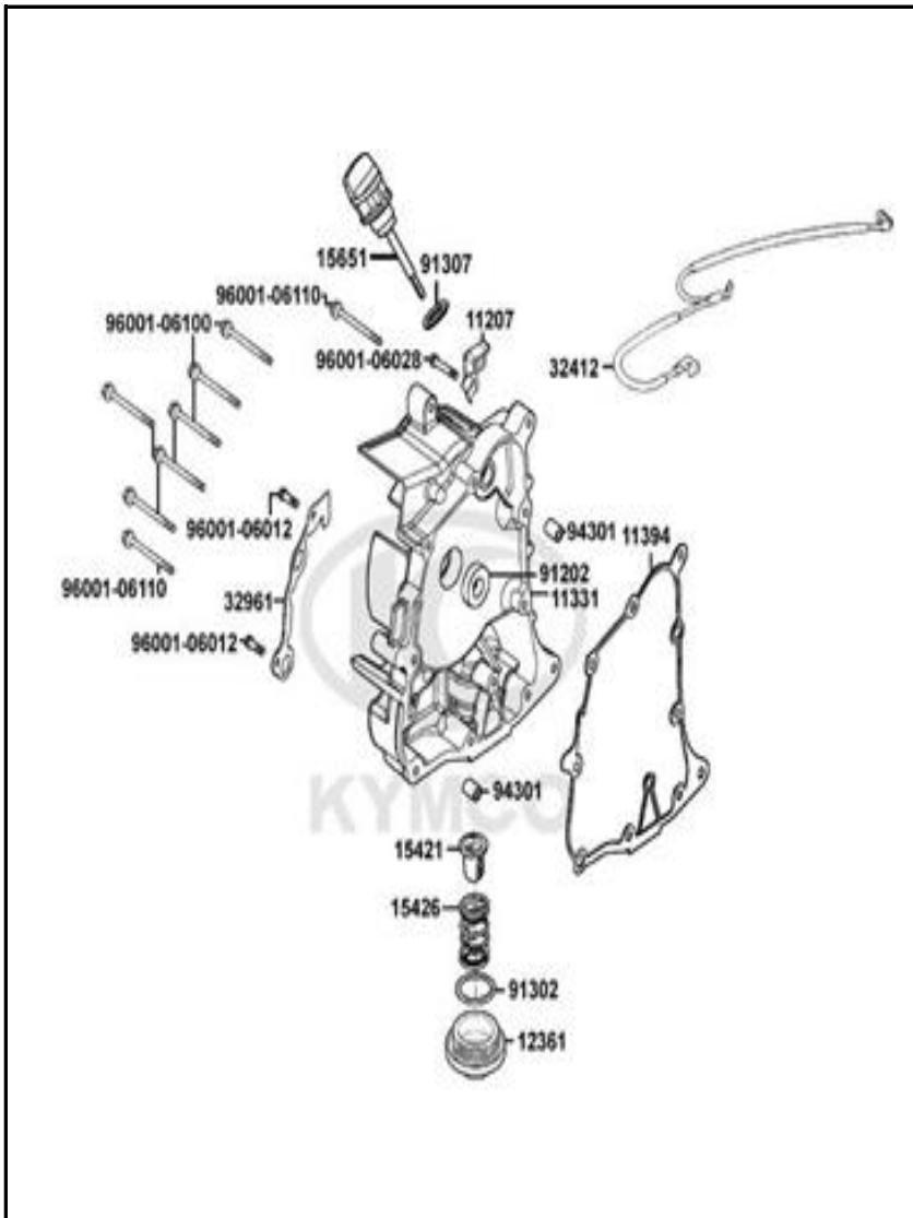
FIGURA N° 4: CUBIERTA MOTOR DERECHA
