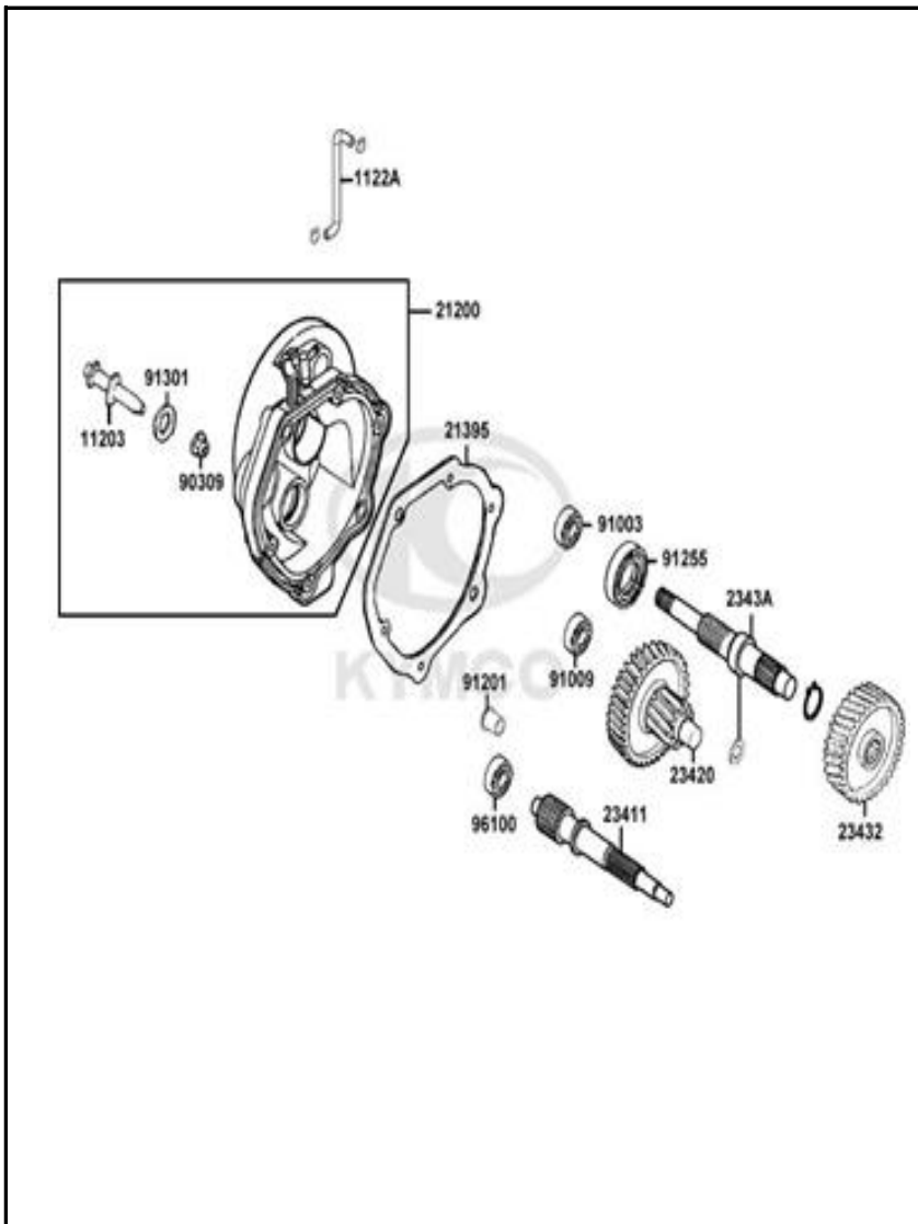
FIGURA N° 8: TRANSMISIÓN
