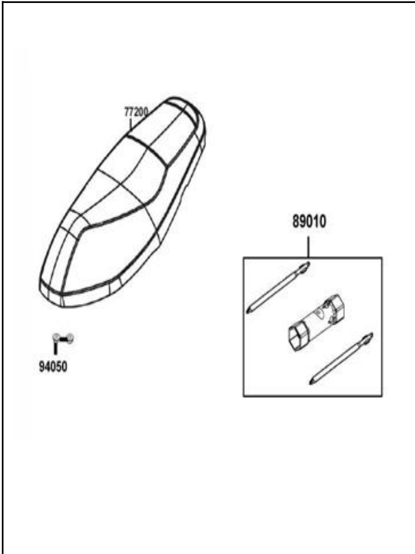
FIGURA N° 18: SILLIN
