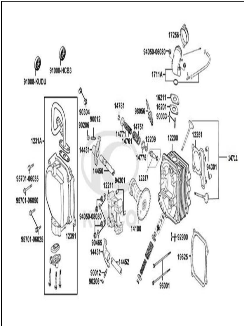
FIGURA N° 2: CULATA 1/2
