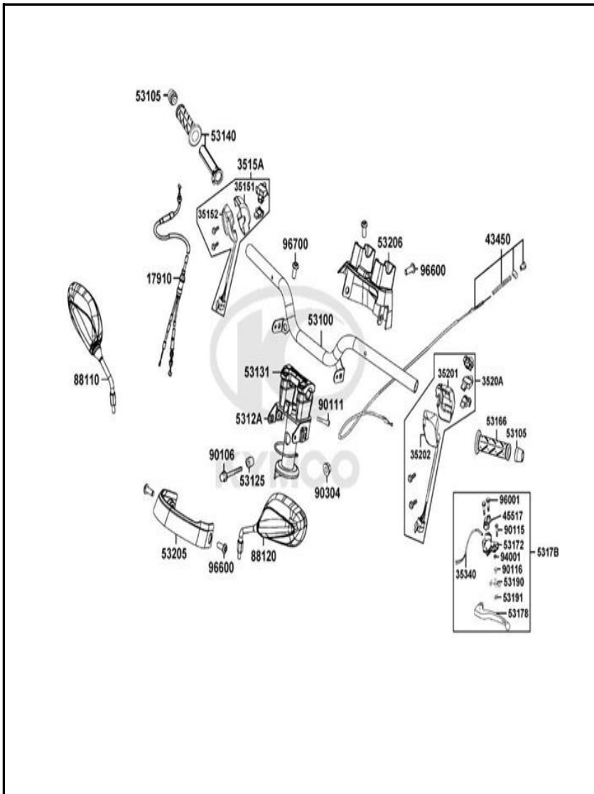
FIGURA N° 12: MANUBRIO - CUBIERTAS MANUBRIO 2/2
