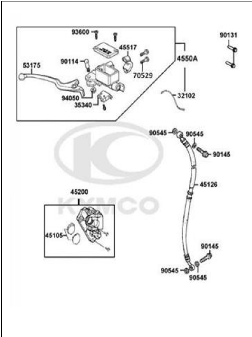
FIGURA N° 13: BOMBA FRENO DELANTERO
