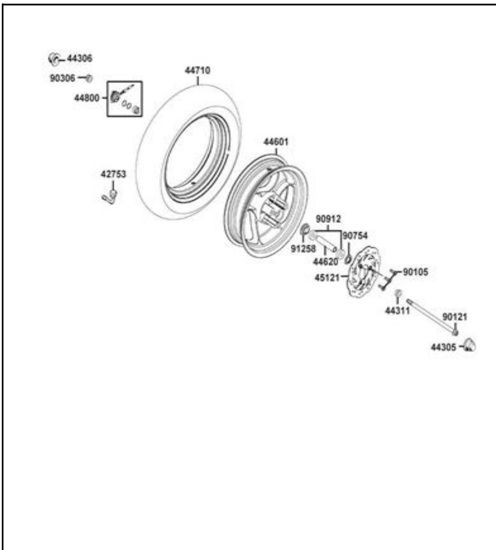
FIGURA N° 16: RIN DELANTERO
