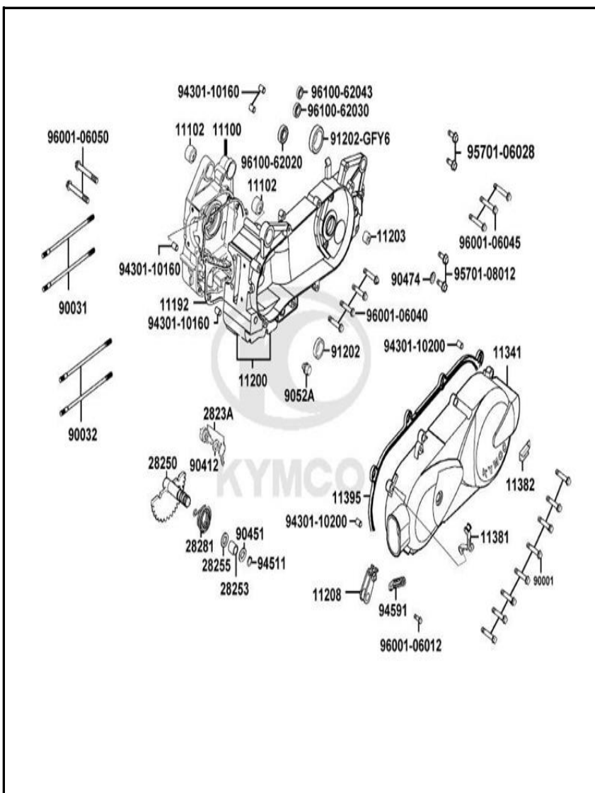
FIGURA N° 1: CARCASAS 2/2
