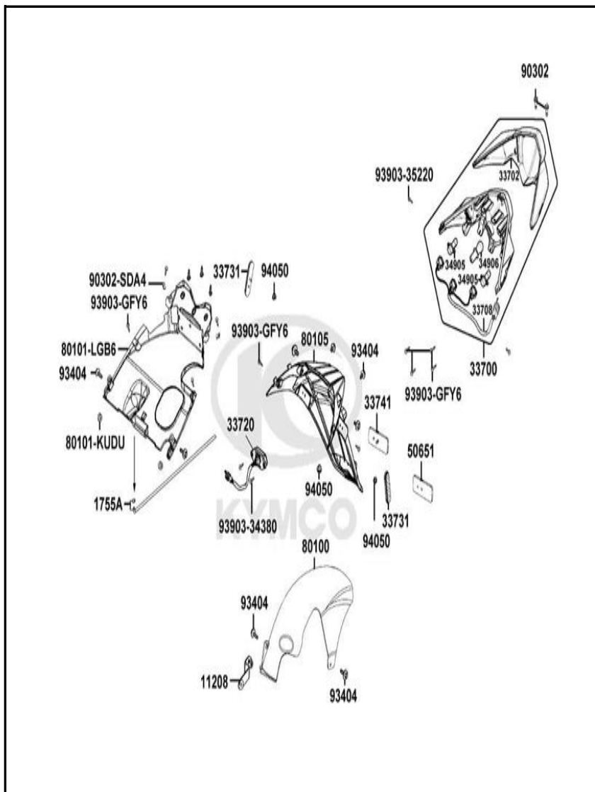
FIGURA N° 27: GUARDABARRO TARSERO
