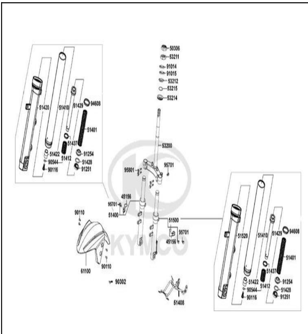
FIGURA N° 15: SUSPENSION DELANTERA 1/2
