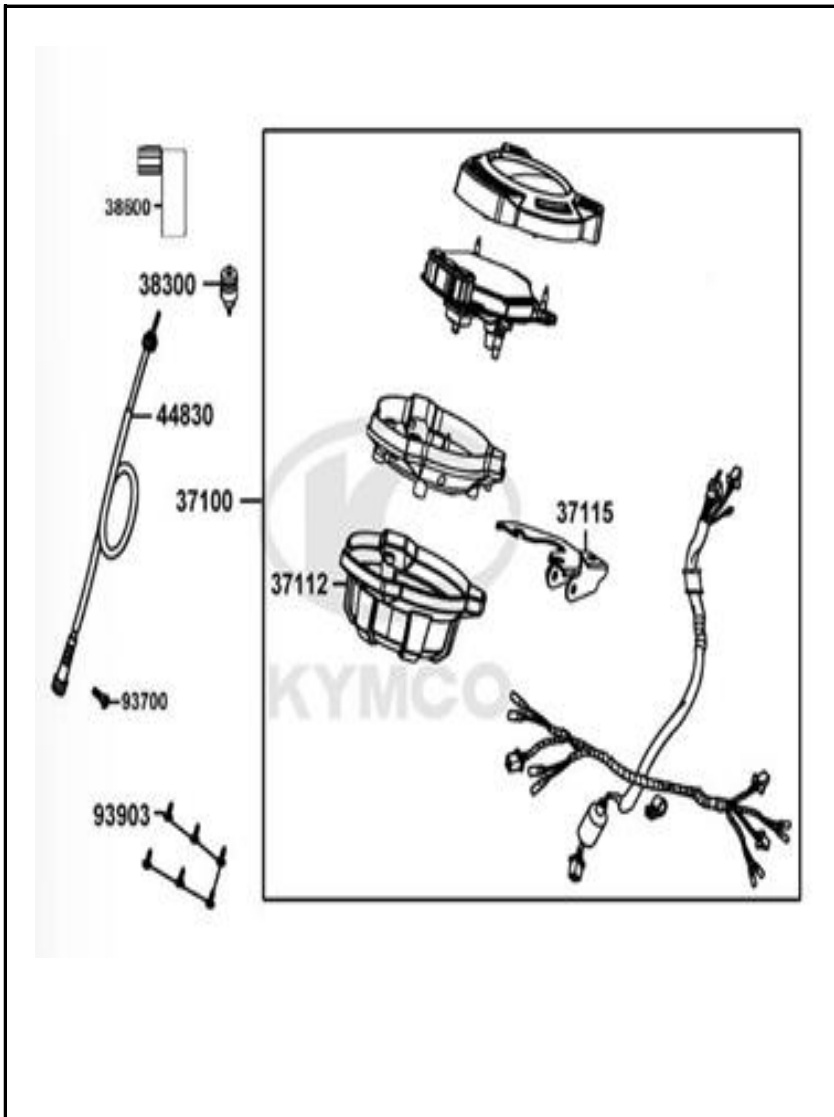
FIGURA N° 11: VELOCÍMETRO
