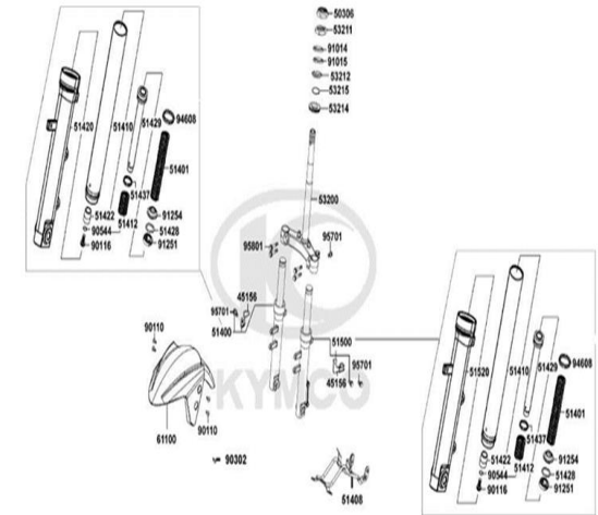
FIG. N° 15 SUSPENSION DELANTERA
