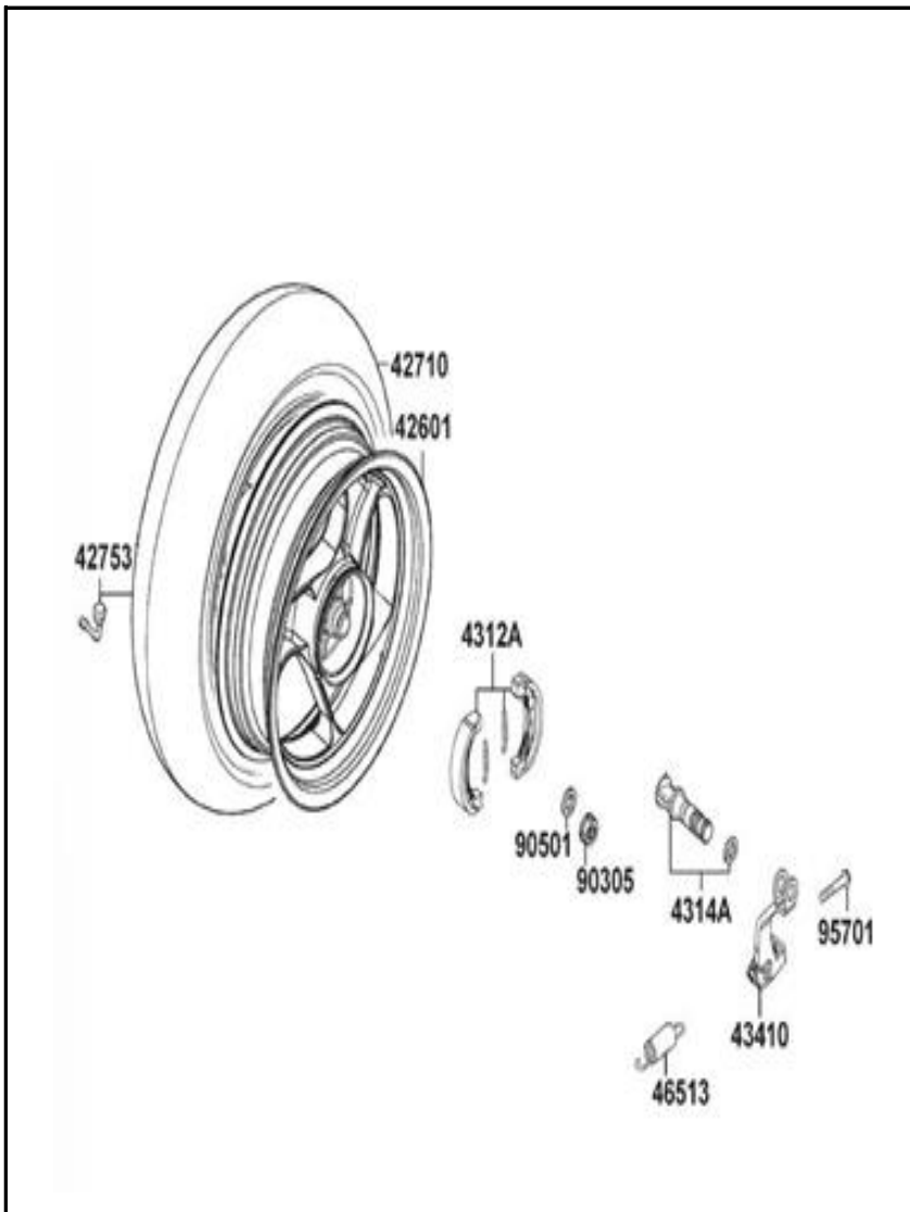
FIGURA N° 17: RIN TRASERO
