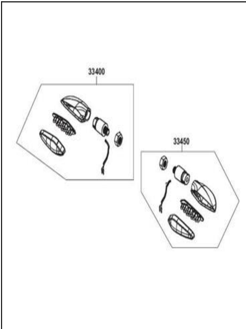
FIGURA N° 26: DIRECCIONALES
