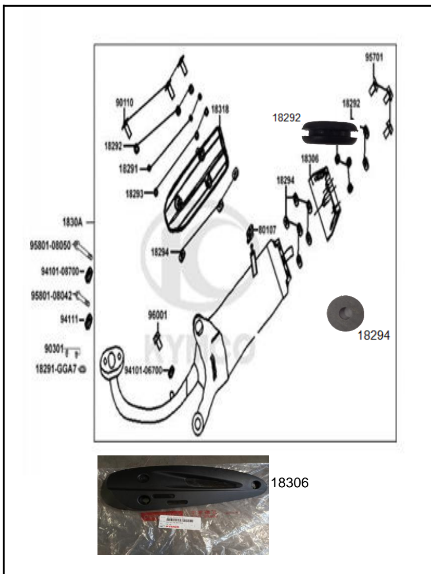
FIGURA N° 23: SILENCIADOR
