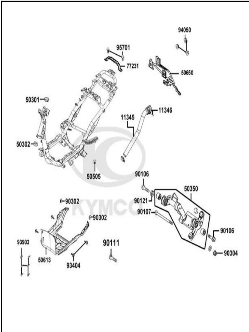
FIGURA N° 29: CHASIS
