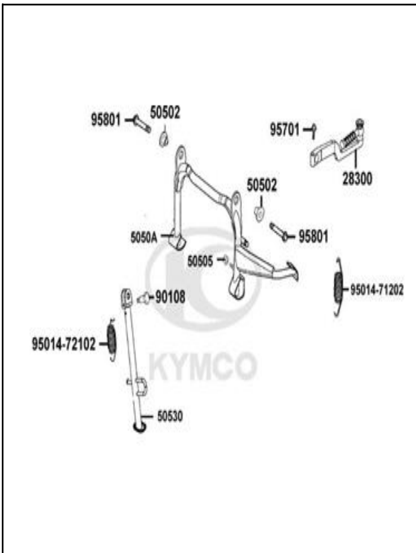
FIGURA N° 24: PEDAL CRANK
