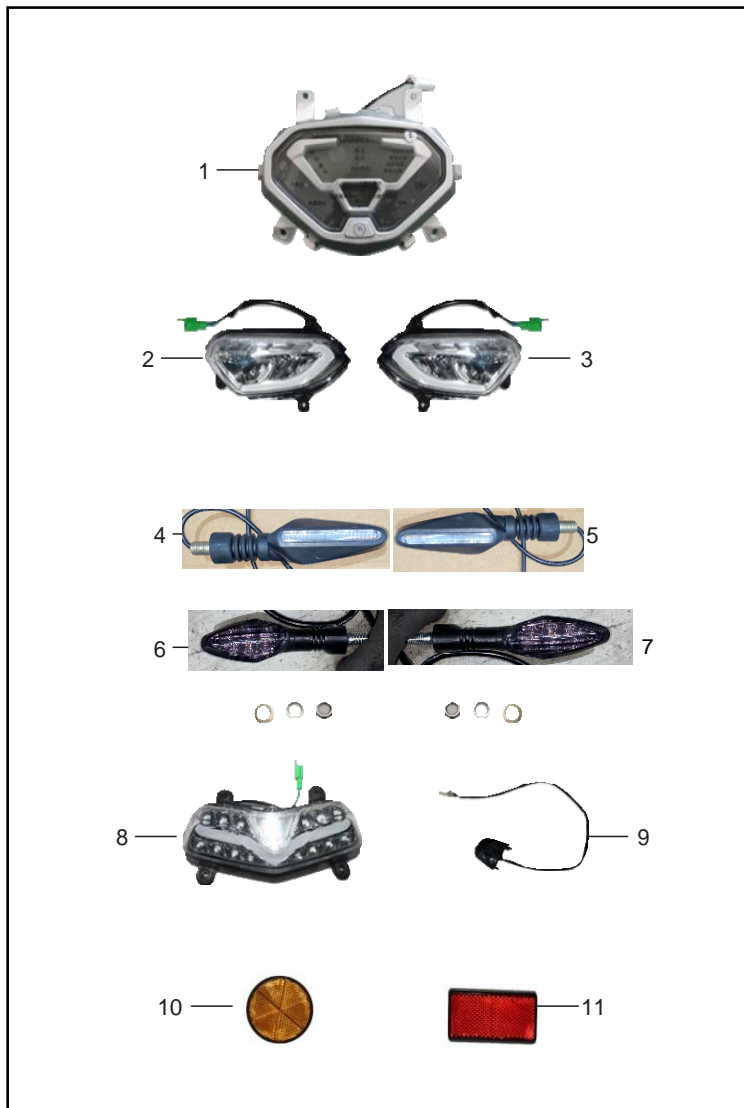
FIGURA N° 1: VELOCÍMETRO - FAROLA - DIRECCIONALES - STOP
