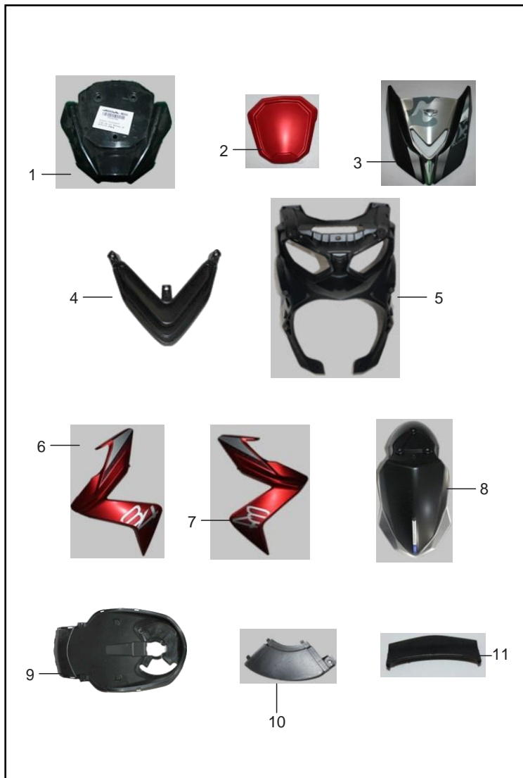
FIGURA N° 9: CUBIERTAS FRONTALES
