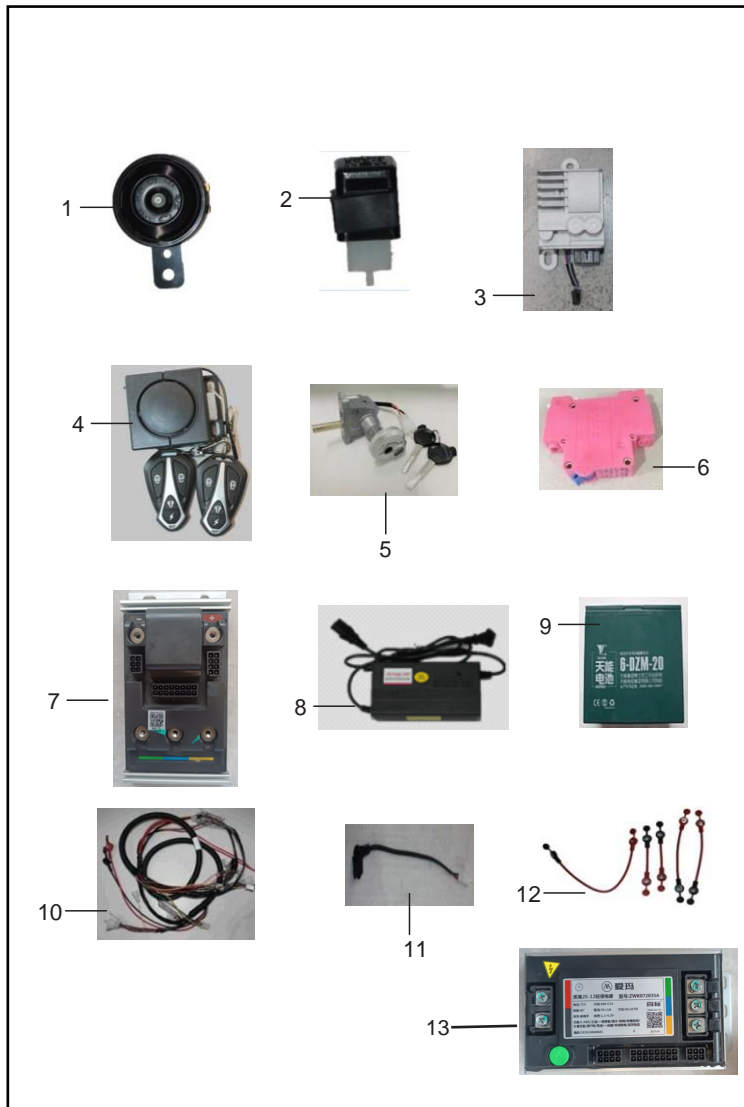
FIGURA N° 8: EQUIPO ELECTRICO
