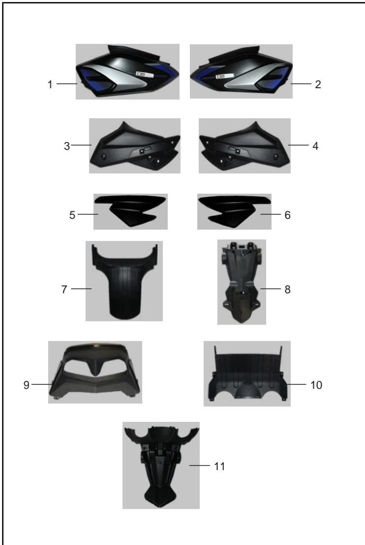
FIGURA N° 11: GUARDABARRO TRASERO - CUBIERTAS TRASERAS
