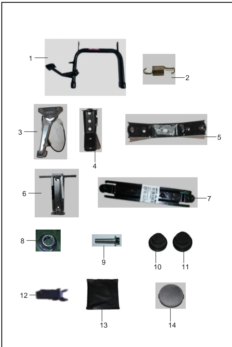
FIGURA N° 7: GATO CENTRAL - GATO LATERAL - COMPLEMENTOS CHASIS
