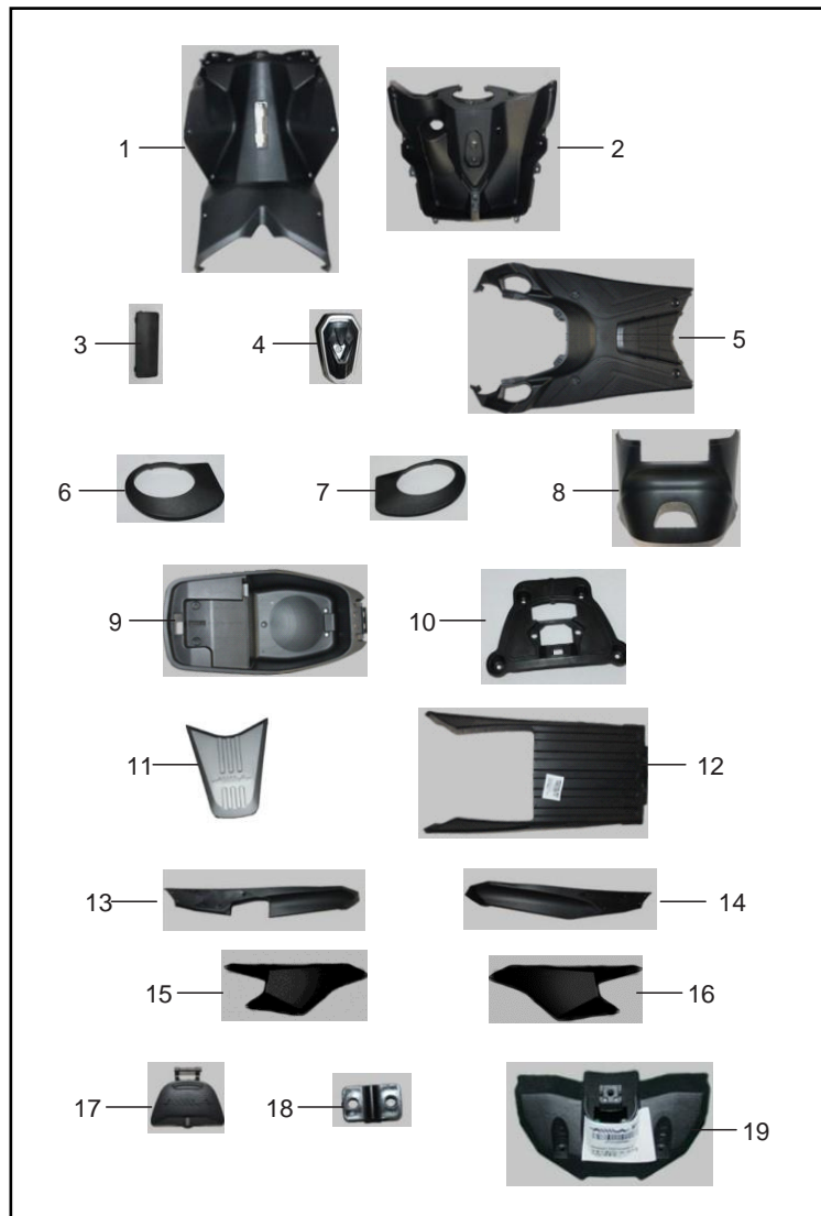
FIGURA N° 10: CUBIERTAS CENTRALES
