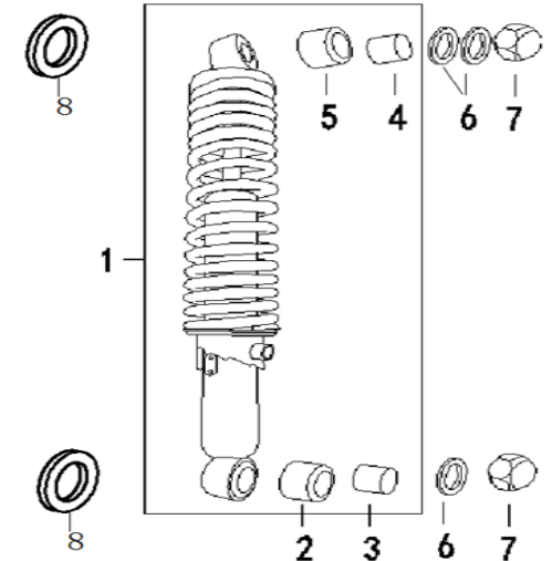
FIG. Nº 39 AMORTIGUADOR TRASERO
