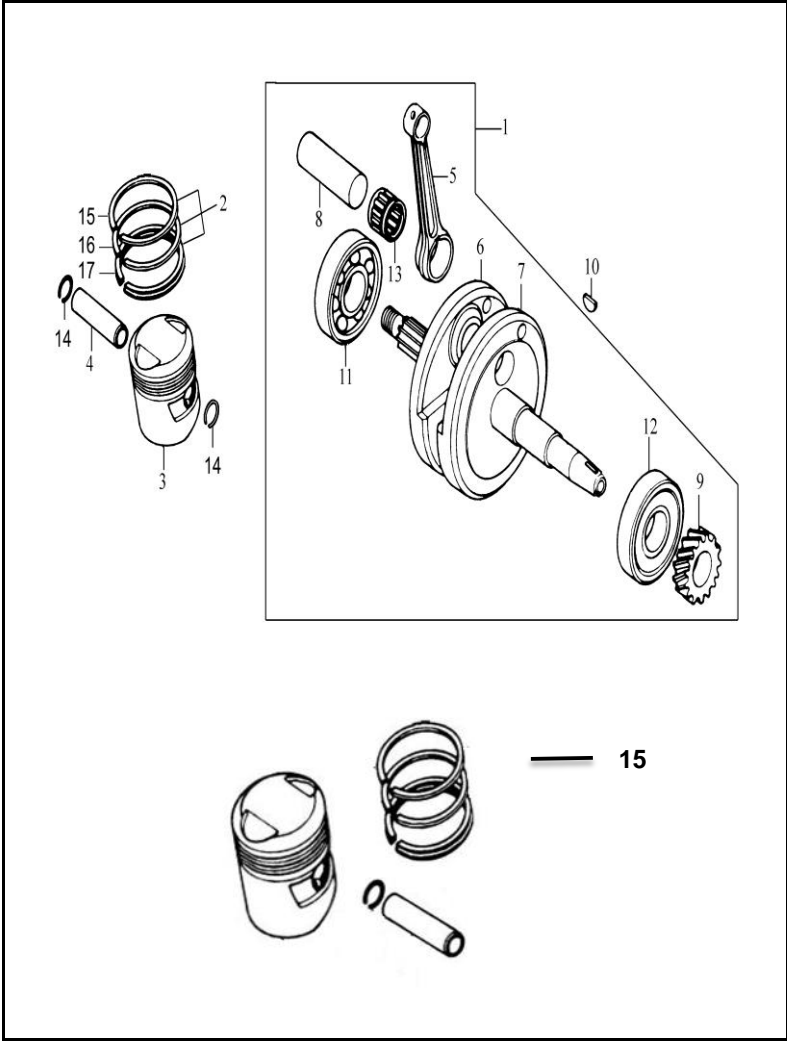
FIGURA N° 9: CIGÜEÑAL - PISTON
