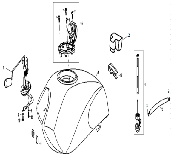
FIG. Nº 29 TANQUE GASOLINA
