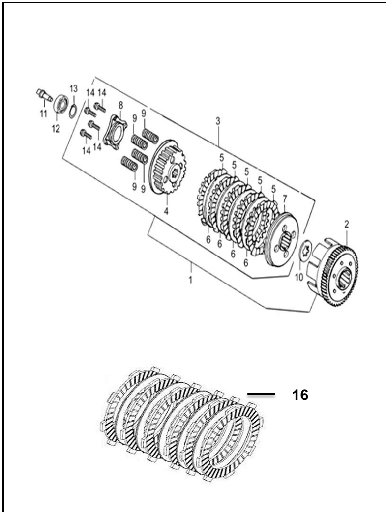
FIGURA N° 4: CLUTCH (5 DISCOS)
