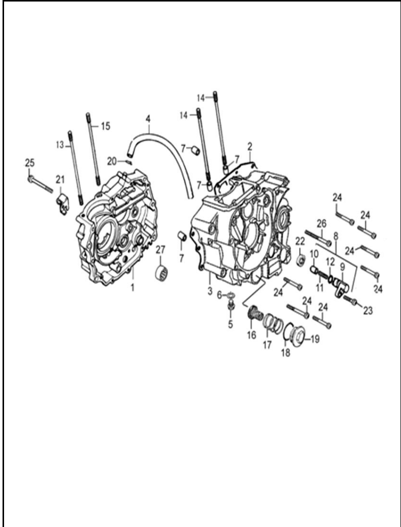
FIGURA N° 8: CARCASAS (2/2)
