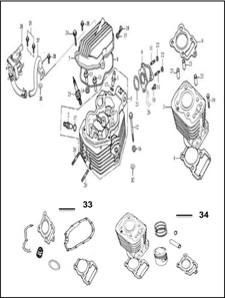
FIGURA N° 1: CULATA - CILINDRO (2/2)
