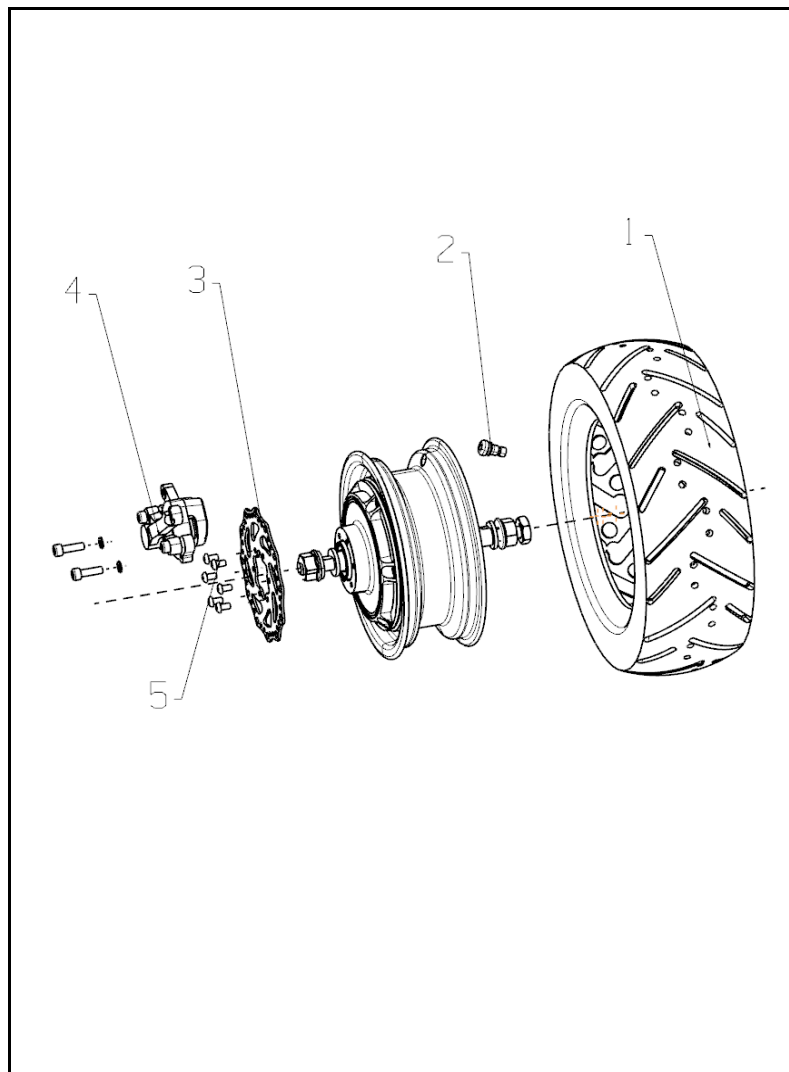
FIGURA N° 12: RUEDA TRASERA
