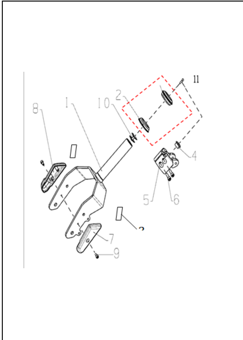
FIGURA N° 5: HORQUILLA DELANTERA
