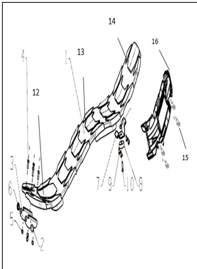
FIGURA N° 8: PISO REPOSAPIES
