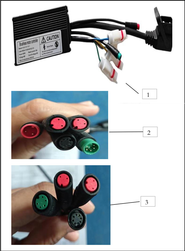
FIGURA N° 15: RAMALES - CONTROLADOR
