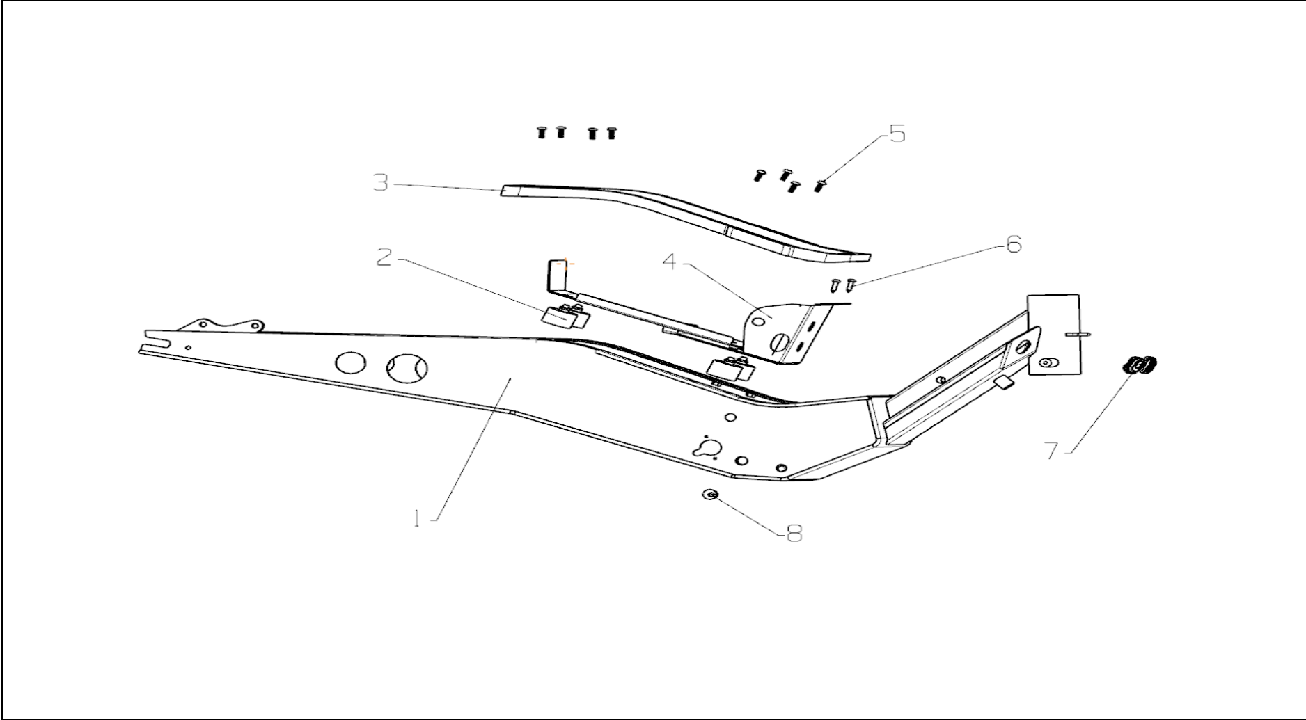
FIGURA N° 7: PARTES DEL CHASIS
