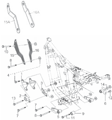
FIGURA N° 24: SOPORTES DE MOTOR (PULSAR 180 UG)
