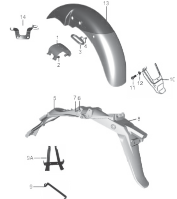
FIGURA N° 28: GUARDABARRO DELANTERO/ GUARDABARRO TRASERO
