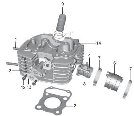
FIGURA N° 3: CULATA
