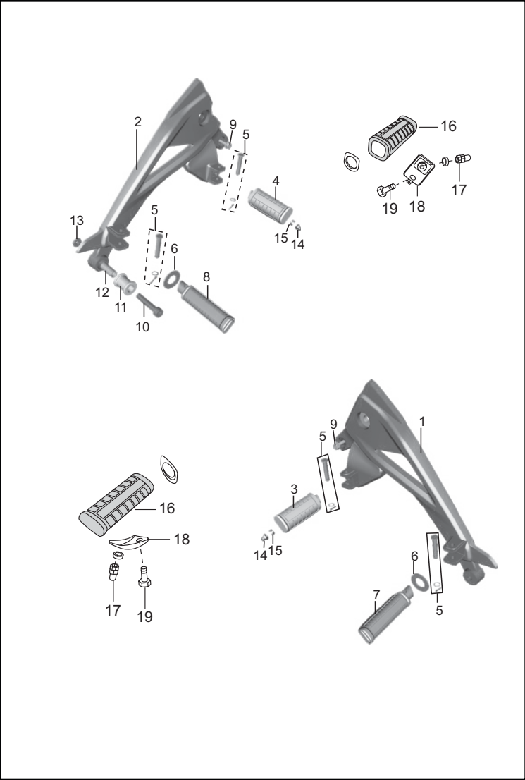
FIGURA N° 27: REPOSAPIES
