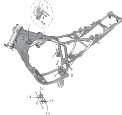
FIGURA N° 24A: SOPORTES DE MOTOR (PULSAR 180 GT BS-IV)
