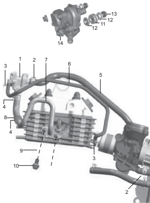
FIGURA N° 2: SISTEMA SAI
