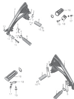
FIGURA N° 27: REPOSAPIES
