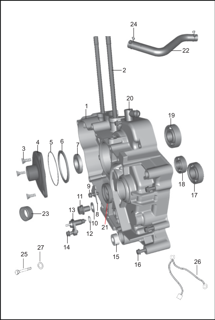
FIGURA N° 13: CARCASA IZQUIERDA (1/2)
