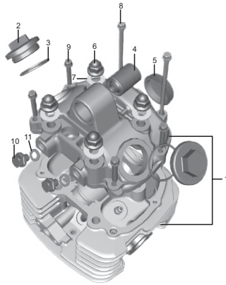
FIGURA N° 1: CUBIERTA CULATA
