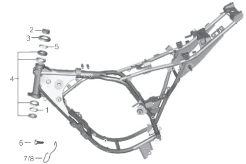
FIGURA N° 25: CHASIS
