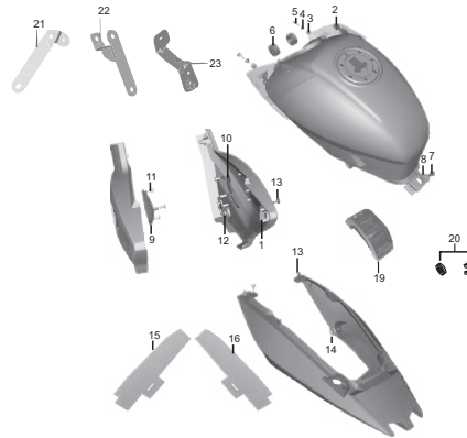
FIGURA N° 40: COMPLEMENTOS TANQUE GASOLINA / TAPAS LATERALES / CUBIERTA SILLÍN
