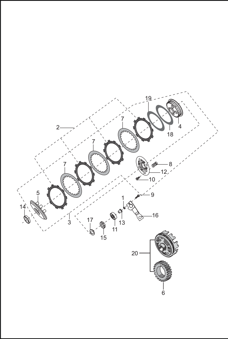
FIGURA N° 16: CLUTCH
