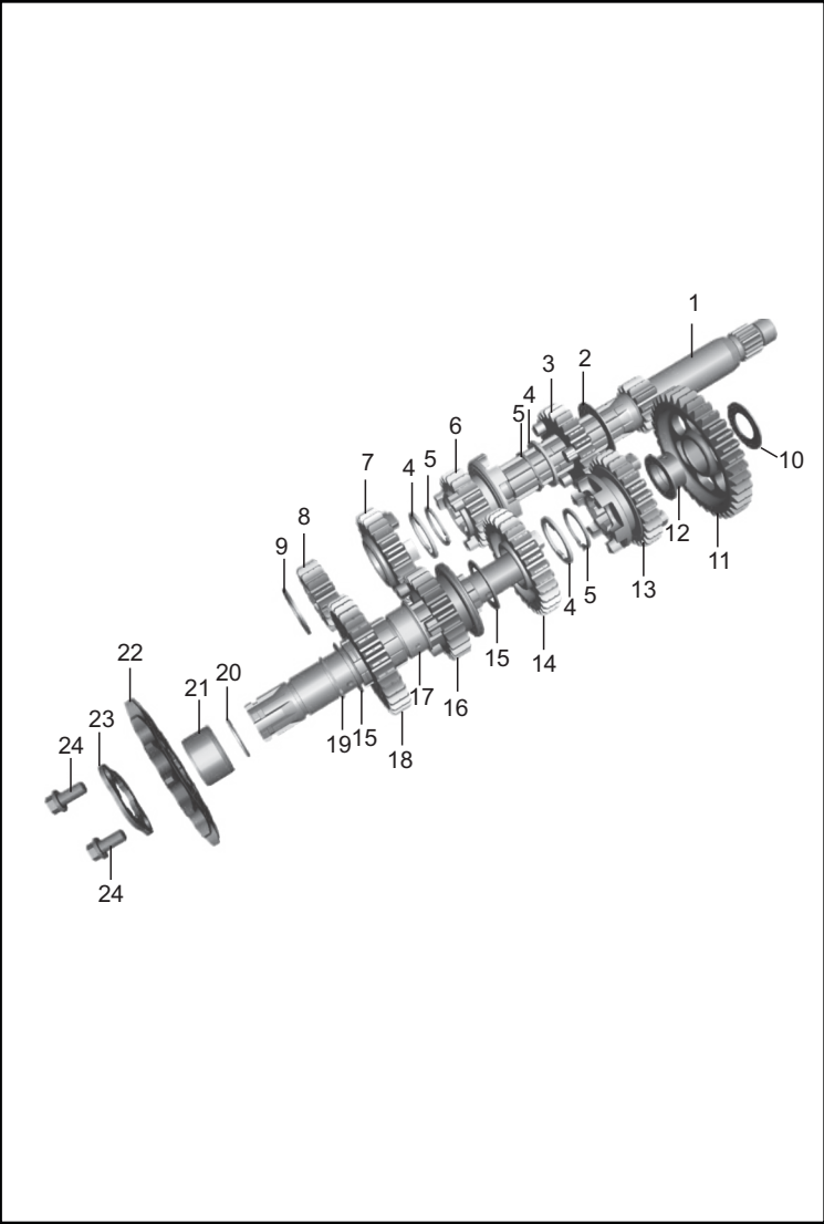
FIGURA N° 9: TRANSMISIÓN (1/2)
