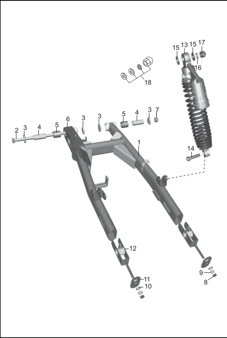
FIGURA N° 26: AMORTIGUADOR TRASERO / BRAZO OSCILANTE
