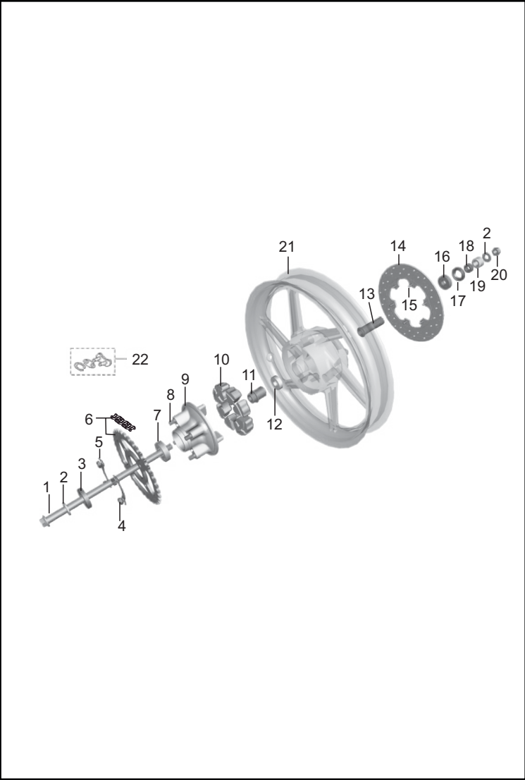
FIGURA N° 34A: RUEDA TRASERA (PULSAR 180 GT BS-IV)
