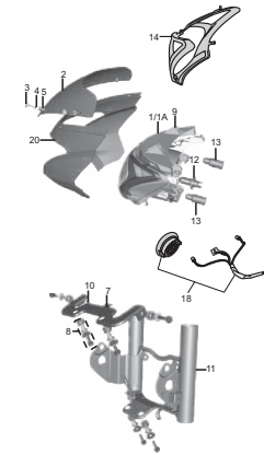
FIGURA N° 44: FAROLA
