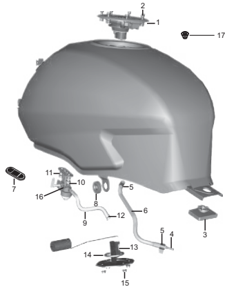
FIGURA N° 39: GRIFO GASOLINA / MEDIDOR GASOLINA
