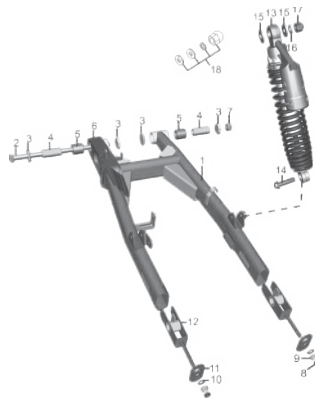
FIGURA N° 26: AMORTIGUADOR TRASERO / BRAZO OSCILANTE
