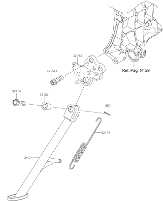
FIGURA N° 36: GATO LATERAL
