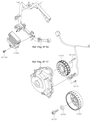
FIGURA N° 22: VOLANTE - PLATO BOBINAS
