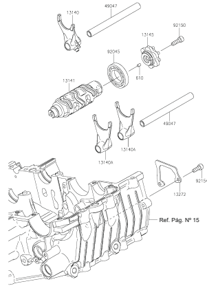
FIGURA N° 12: SELECTOR DE CAMBIOS
