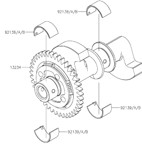
FIGURA N° 9: BALANCEADOR
