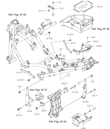
FIGURA N° 30: SOPORTES DE MOTOR
