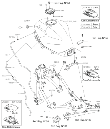
FIGURA N° 48: TANQUE DE GASOLINA
