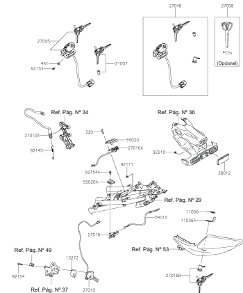
FIGURA N° 57: SWICHE DE ENCENDIDO
