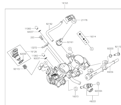
FIGURA N° 18: SISTEMA DE INYECCIÓN
