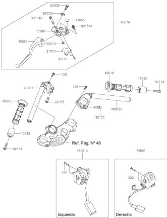
FIGURA N° 46: MANUBRIO
