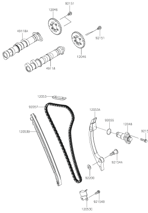
FIGURA N° 7: EJE DE LEVAS / TENSOR CADENILLA
