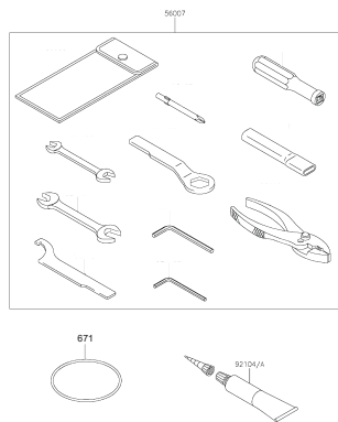
FIGURA N° 58: HERRAMIENTAS
