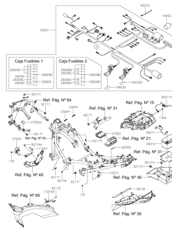
FIGURA N° 56: SISTEMA ELÉCTRICO
