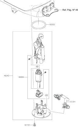
FIGURA N° 19: BOMBA DE GASOLINA
