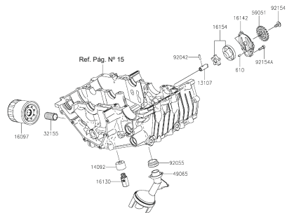
FIGURA Nº 21: BOMBA ACEITE
