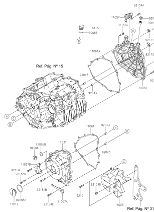
FIGURA N° 16: CUBIERTA MOTOR
