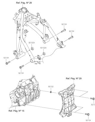
FIGURA N° 29: COMPLEMENTOS CHASIS
