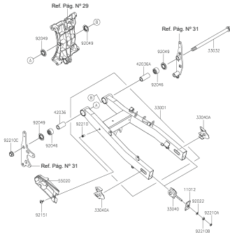
FIGURA N° 31: BRAZO OSCILANTE
