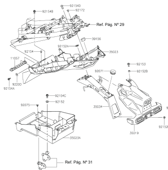
FIGURA N° 35: GUARDABARRO TRASERO
