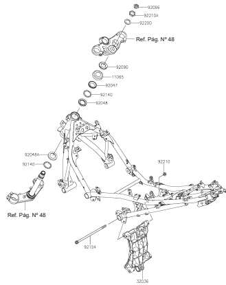
FIGURA N° 28: CHASIS
