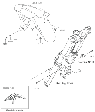
FIGURA N° 34: GUARDABARRO DELANTERO
