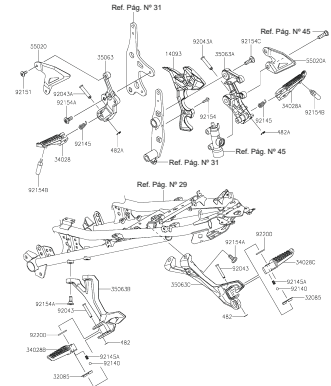
FIGURA N° 33: REPOSAPIES
