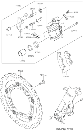
FIGURA N° 43: DISCO FRENO DELANTERO CALIPER DELANTERO
