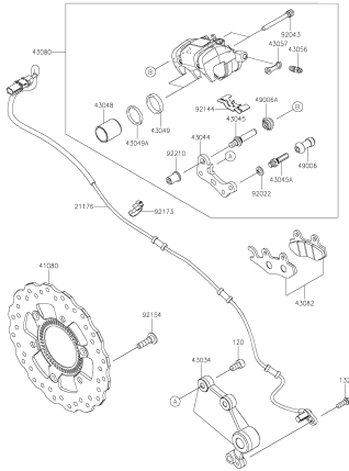
FIGURA Nº 45: DISCO FRENO TRASERO CALIPER TRASERO
