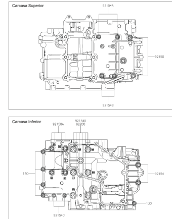
FIGURA N° 15: TORNILLOS CARCASA MOTOR
