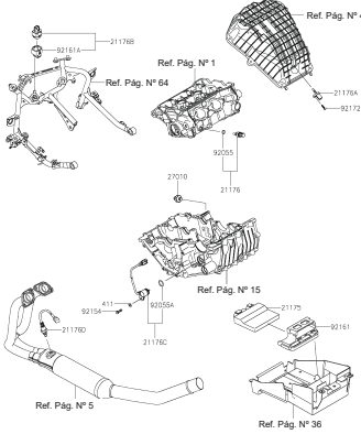
FIGURA N° 20: UNIDAD DE CONTROL ELÉCTRICA (E.C.U.)
