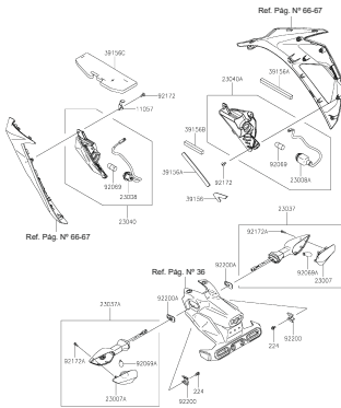
FIGURA N° 55: DIRECCIONALES
