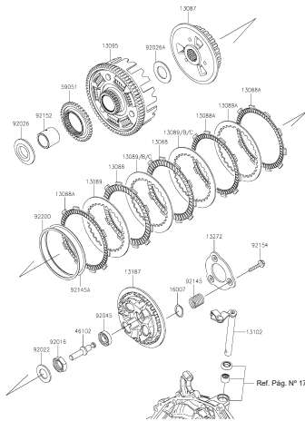
FIGURA N° 10: CLUTCH
