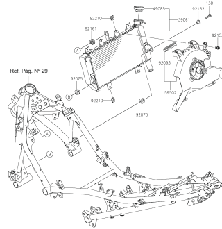
FIGURA N° 26: RADIADOR
