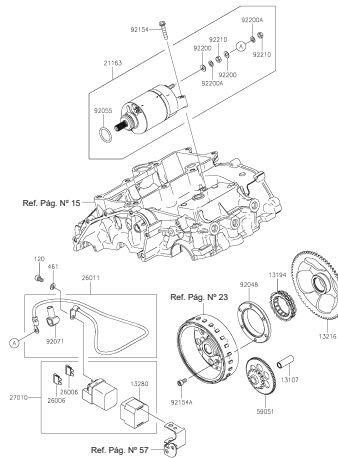
FIGURA N° 24: MOTOR DE ARRANQUE
