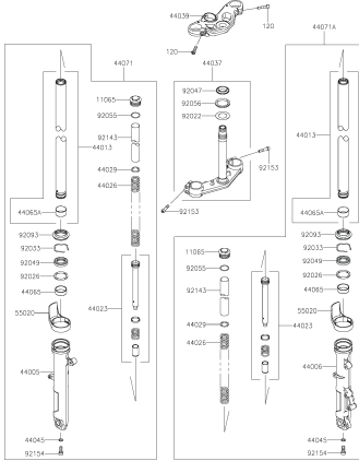
FIGURA N° 47: SUSPENSIÓN DELANTERA
