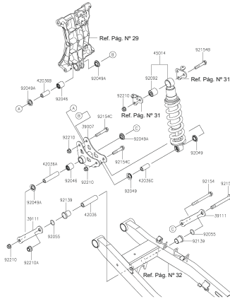
FIGURA N° 32: AMORTIGUADOR
