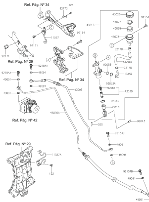
FIGURA N° 44: BOMBA FRENO TRASERO
