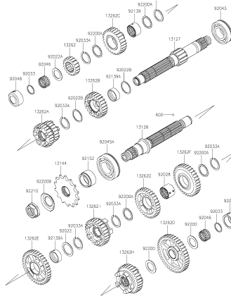
FIGURA N° 11: TRANSMISIÓN
