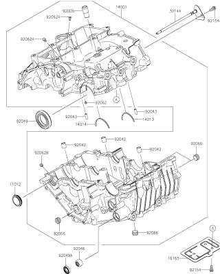
FIGURA N° 14: CARCASA MOTOR
