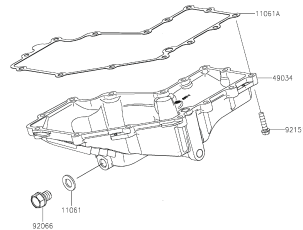
FIGURA Nº 17: CARTER ACEITE
