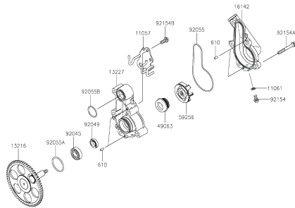
FIGURA N° 25: BOMBA DE AGUA
