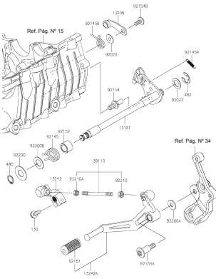
FIGURA N° 13: EJE DE CAMBIOS
