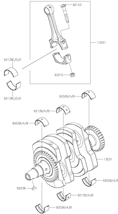
FIGURA N° 8: CIGÜEÑAL
