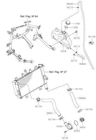
FIGURA N° 27: TANQUE DE RESERVA
