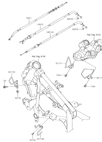
E-13: CABLES
