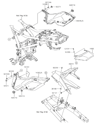
E-14: CUBIERTA SILLÍN / GUARDACADENA
