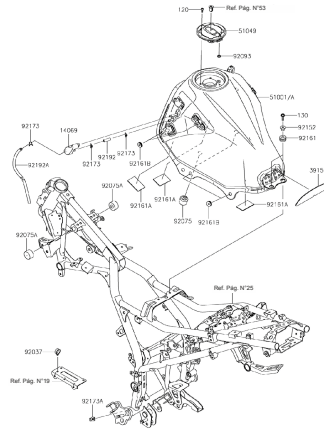
E-10: TANQUE DE GASOLINA
