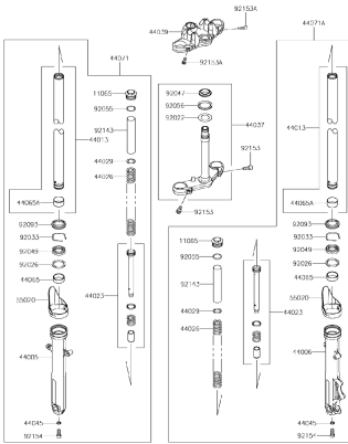
E-9: SUSPENSIÓN DELANTERA
