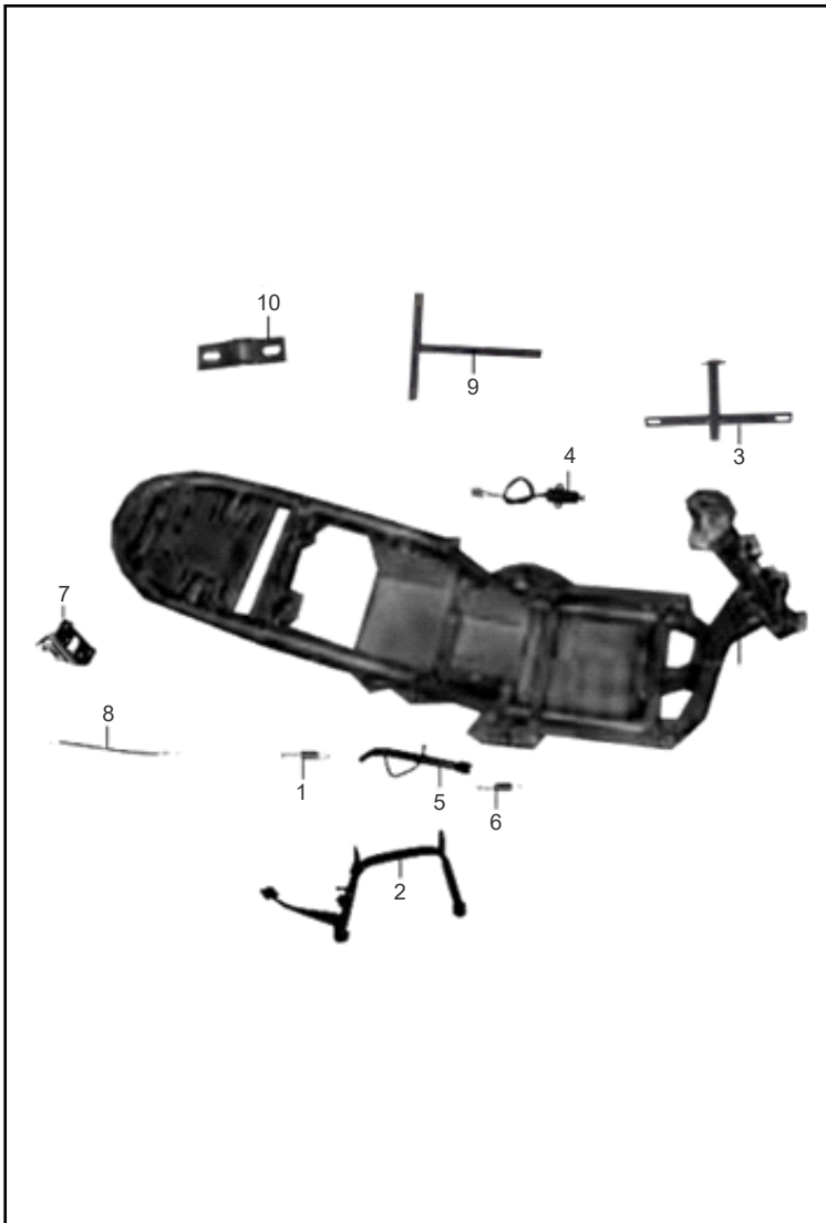
FIGURA N° 04: CHASIS
