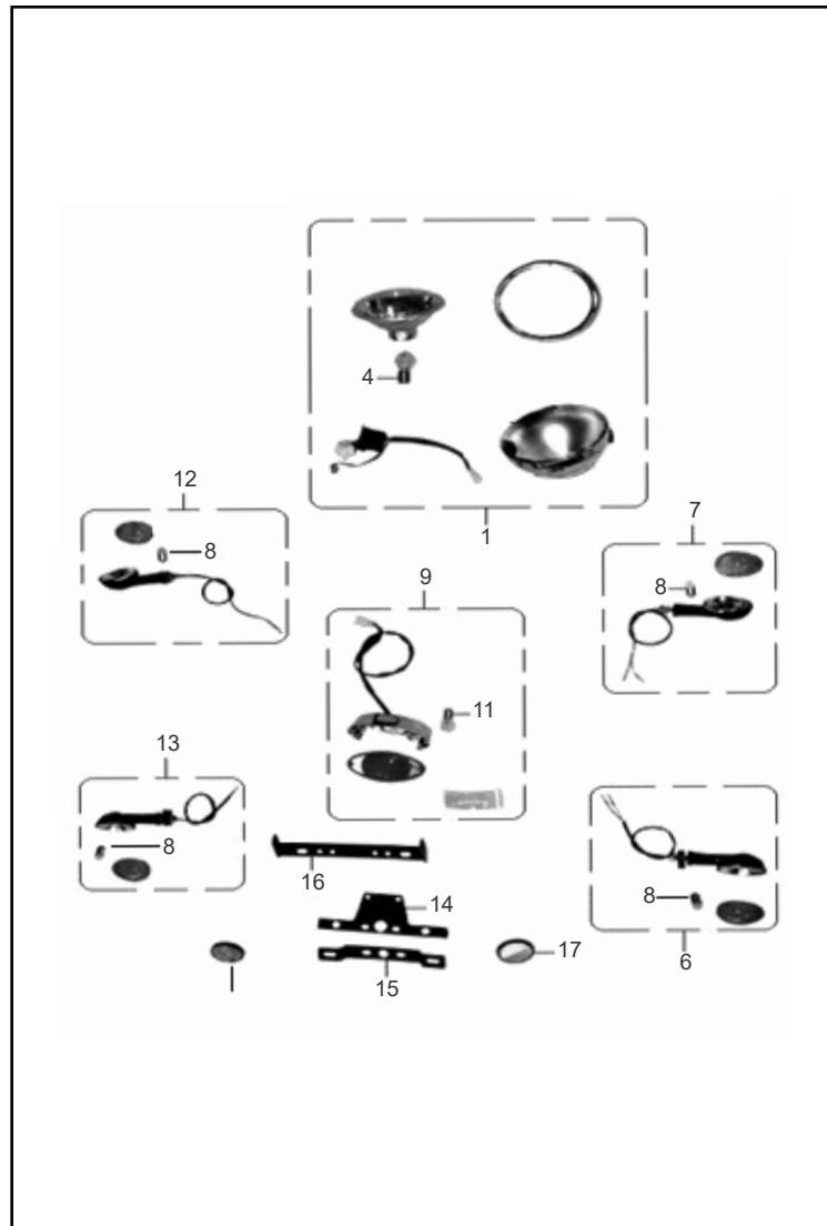
FIGURA N° 08: LUCES
