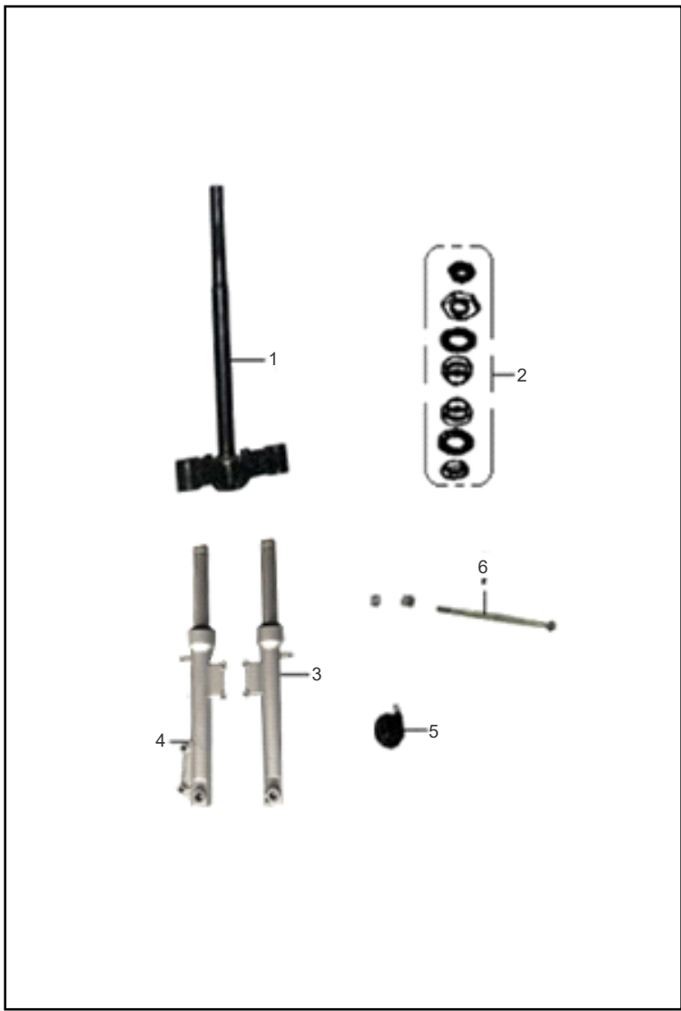
FIGURA N° 05: SUSPENSIÓN DELANTERA
