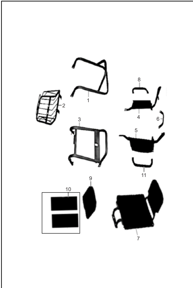
FIGURA N° 11: PARRILLAS Y SOPORTES
