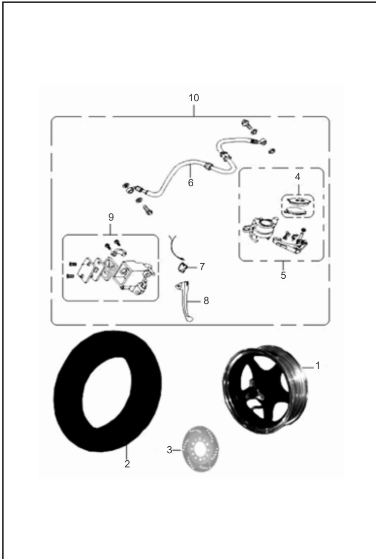
FIGURA N° 03: RUEDA DELANTERA
