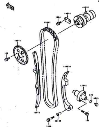
B-8 Camshaft(s)/Tensioner
