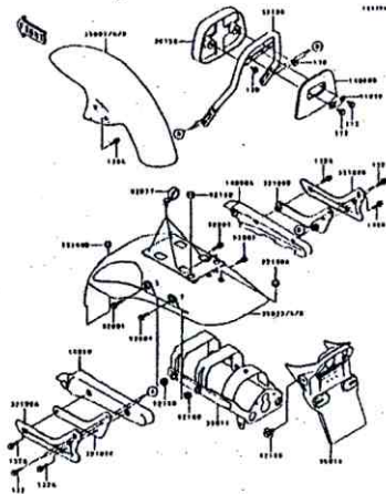
D-10 Fenders(BN175-A3)
