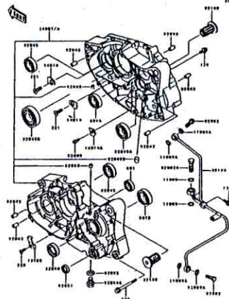
B-14 Crankcase
