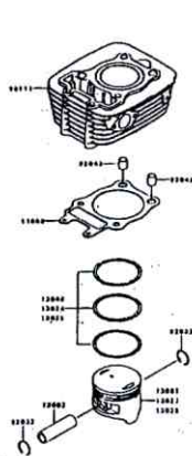
B-4 Cylinder/Piston(s)
