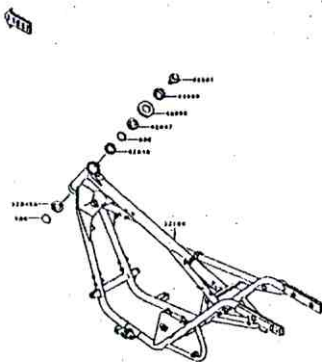
D-3 Frame
