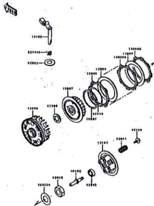
B-10 Clutch
