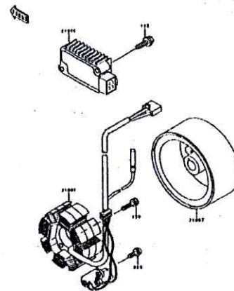
C-9 Generator
