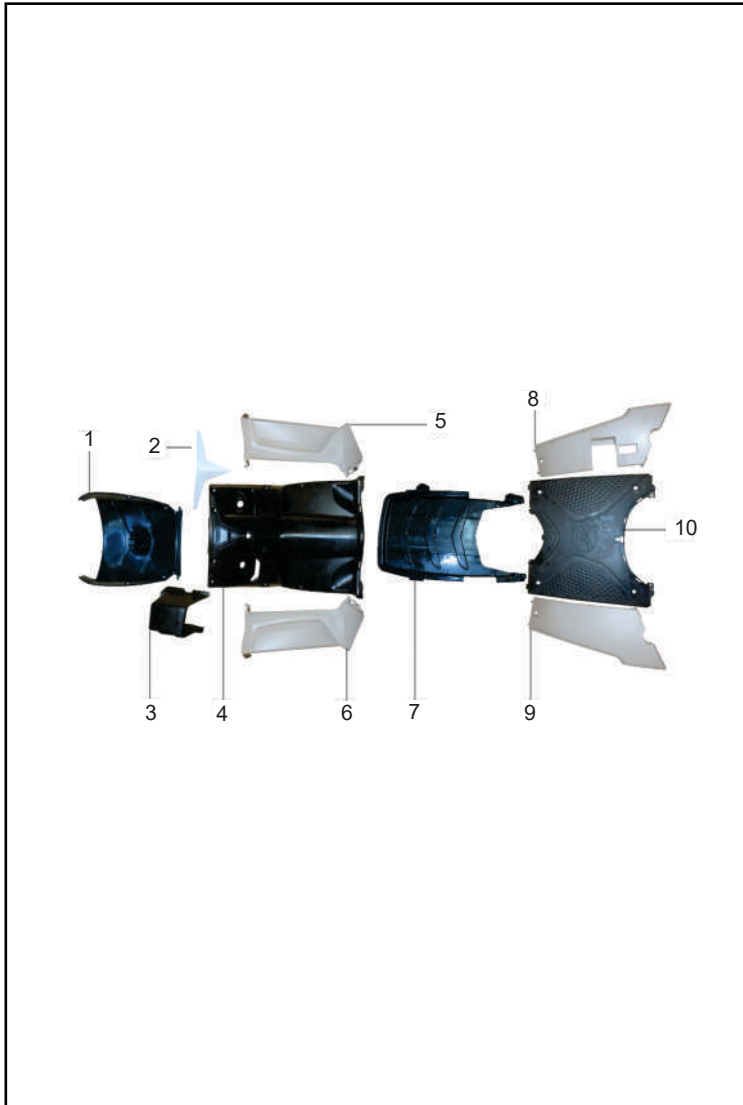
FIGURA N° 4: CUBIERTAS
