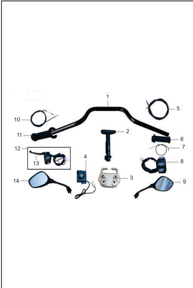
FIGURA N° 1: MANUBRIO - ESPEJOS
