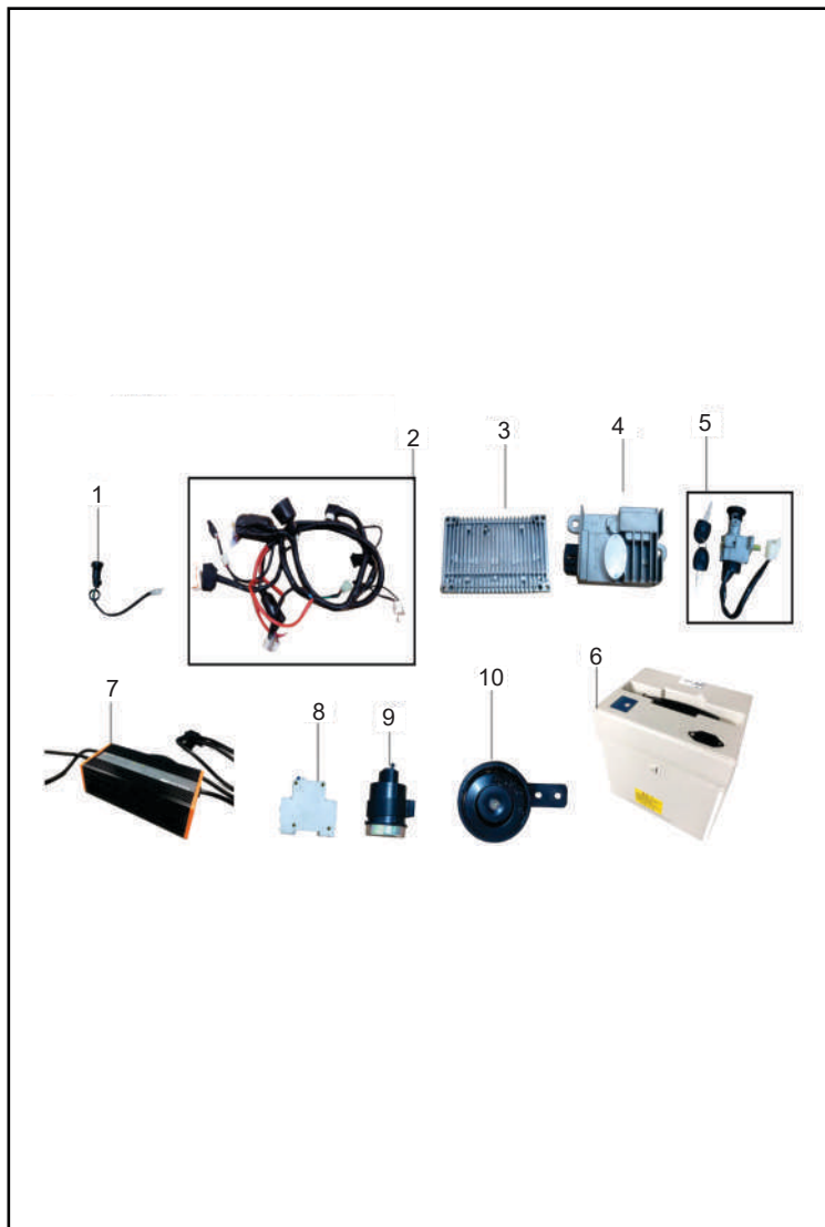
FIGURA N° 14: EQUIPO ELÉCTRICO
