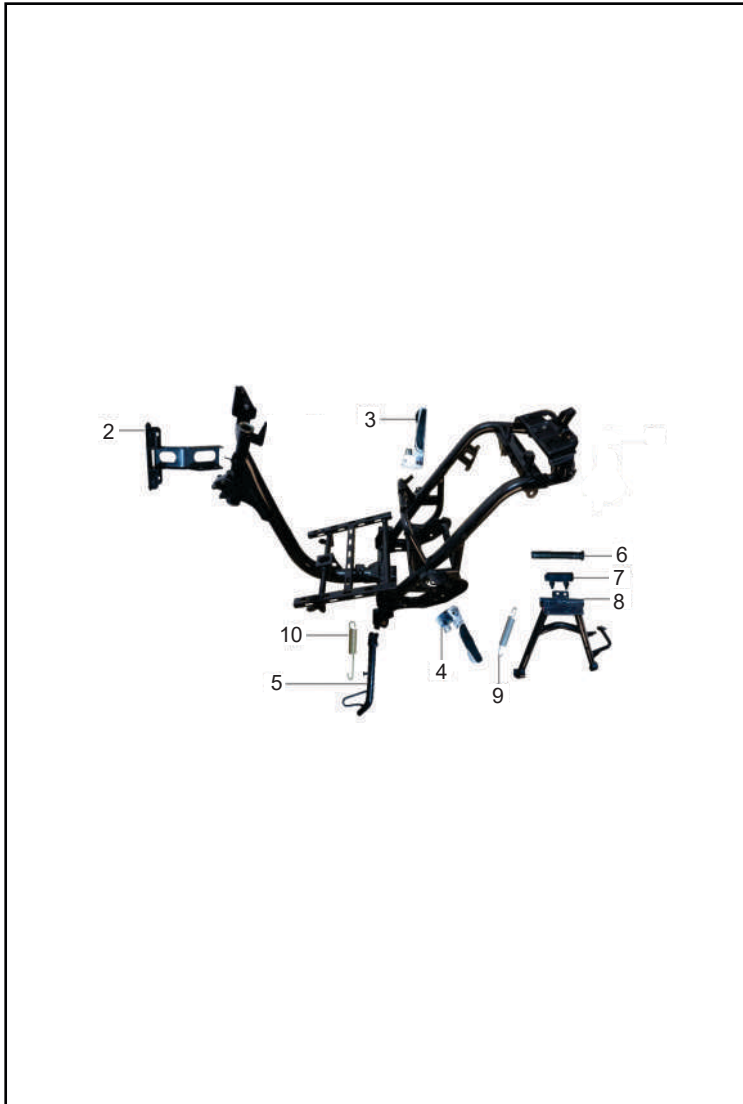
FIGURA N° 13: CHASIS
