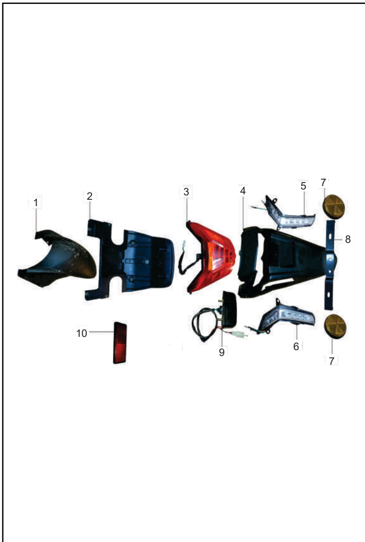
FIGURA N° 7: GUARDABARRO TRASERO - STOP
