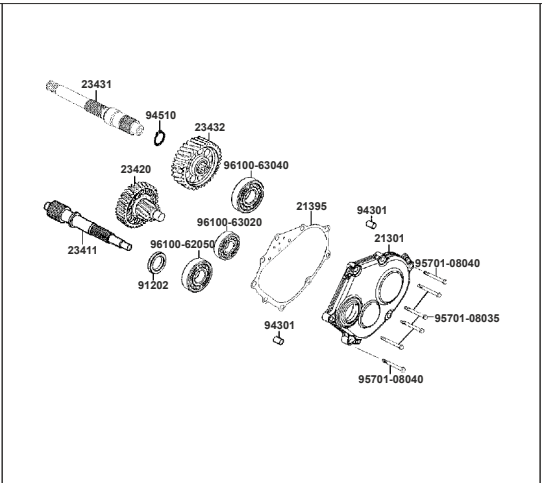
E08: TRANSMISIÓN
