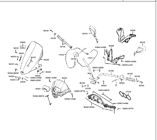
F04: MANUBRIO - CUBIERTAS MANUBRIO
