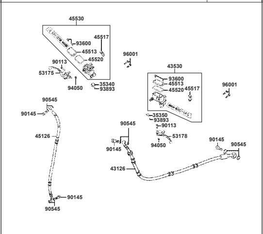
F03: BOMBA DE FRENO
