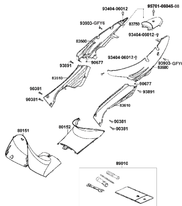
F-15: CARENAJES / TAPAS LATERALES
