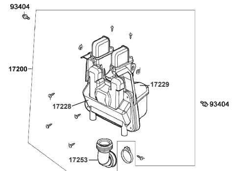
F-16: FILTRO DE AIRE
