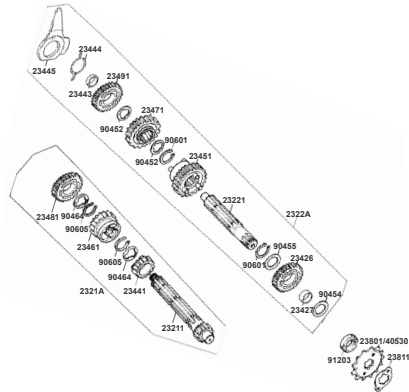
E-16: TRANSMISIÓN
