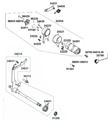
E-17: EJE DE CAMBIOS / SELECTOR DE CAMBIOS
