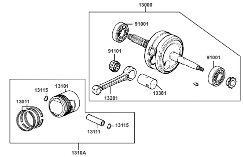
E-15: CIGÜEÑAL / PISTÓN
