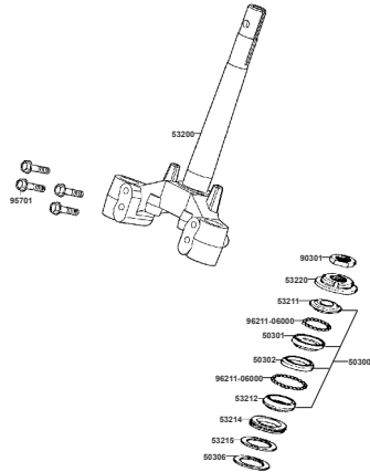
F-06: HORQUILLA
