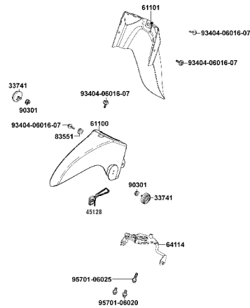
F-07: GUARDABARRO DELANTERO
